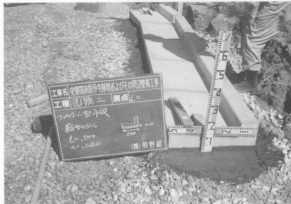
(1) 園路L型側溝付設状況
