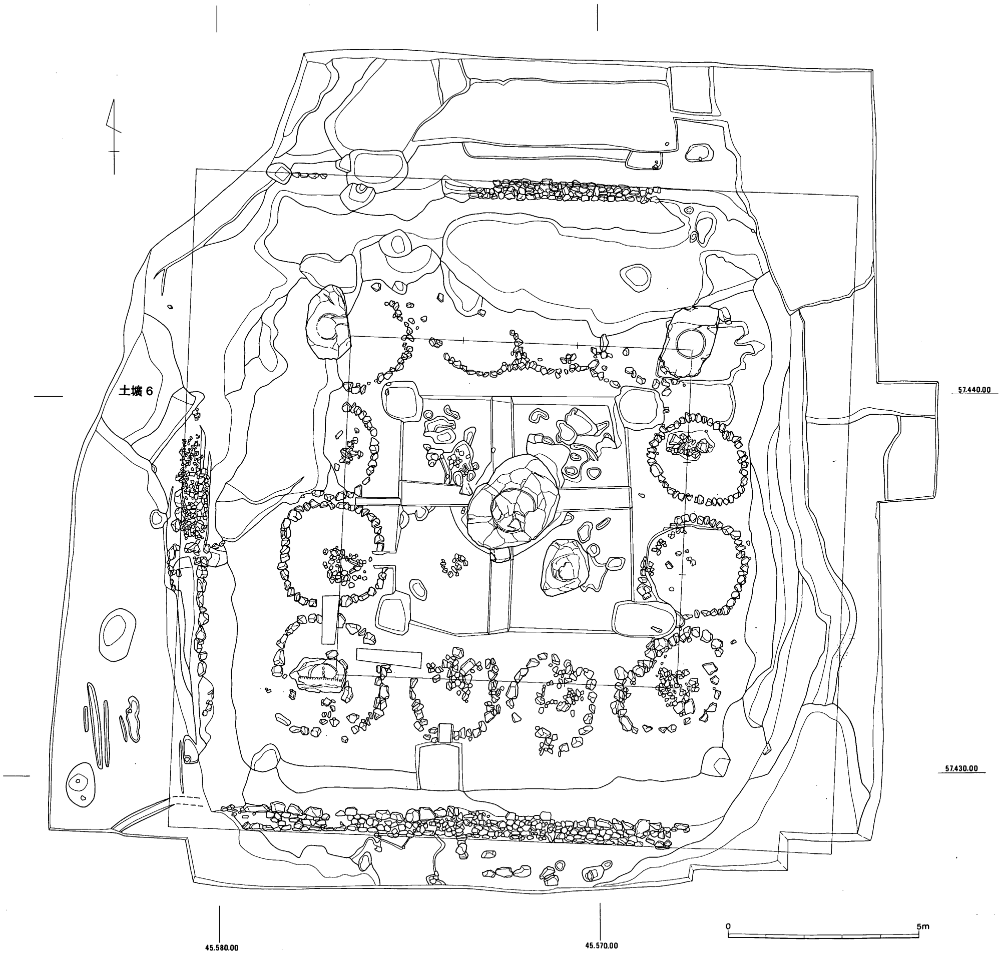
第6図 塔跡遺構実測図 (1/100)
