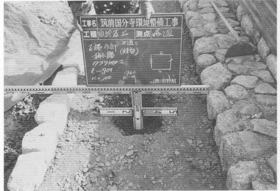
(1) 塔跡雨落溝床路盤工事 (クラッシャーラン敷設)
