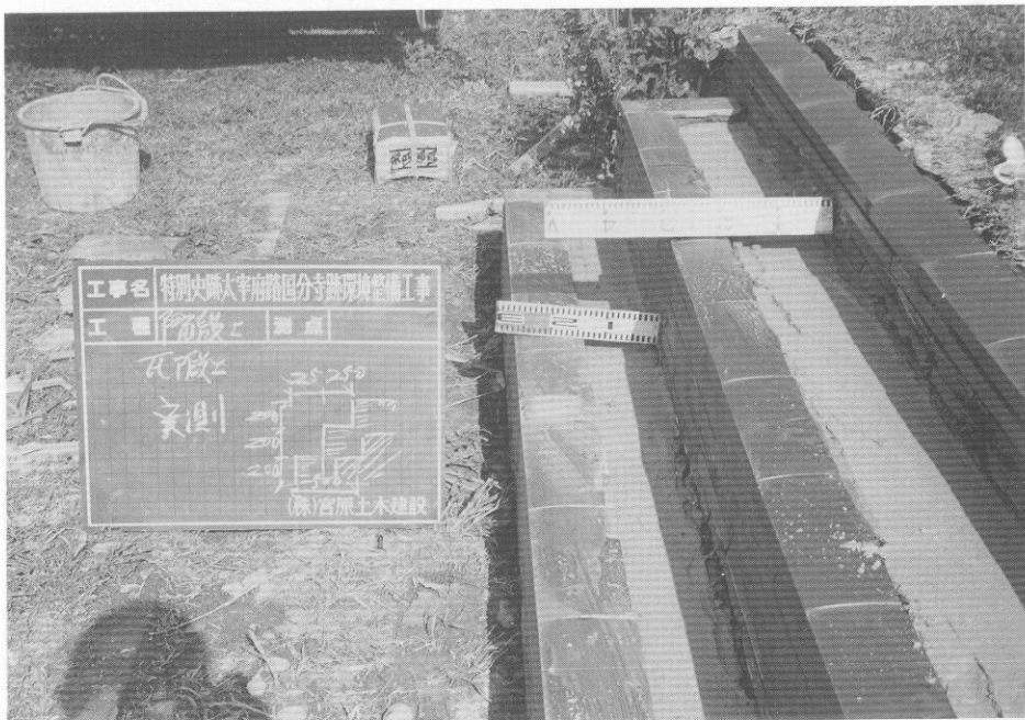
(3) 講堂跡瓦積階段修理工事
