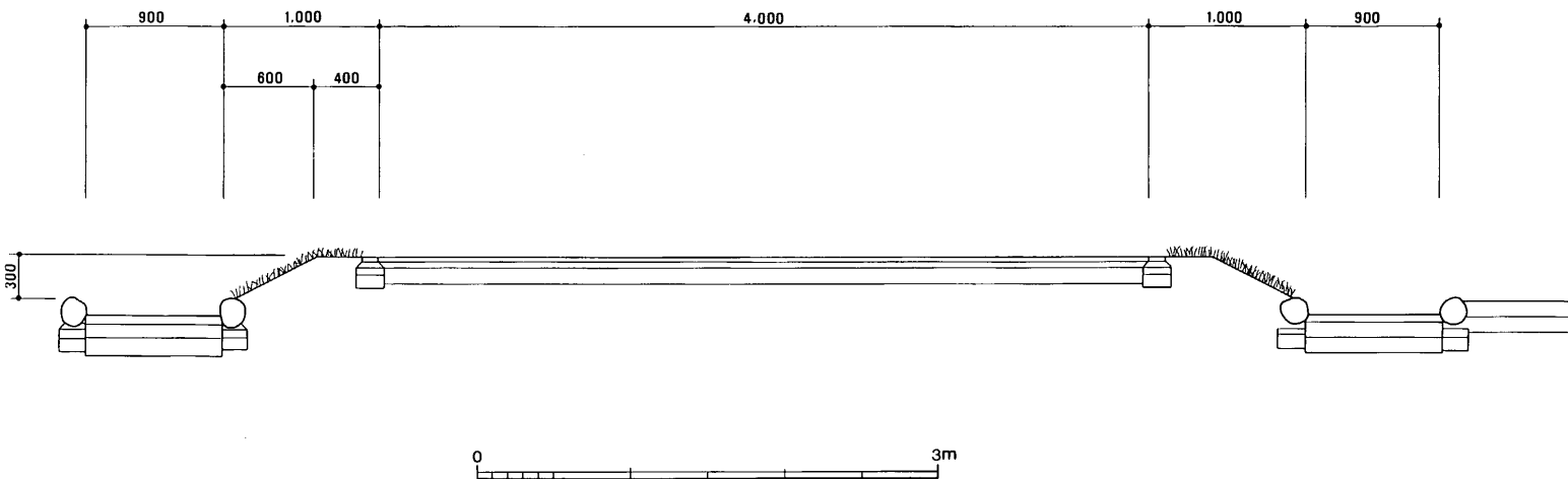
第15図 回廊・雨落溝断面図
