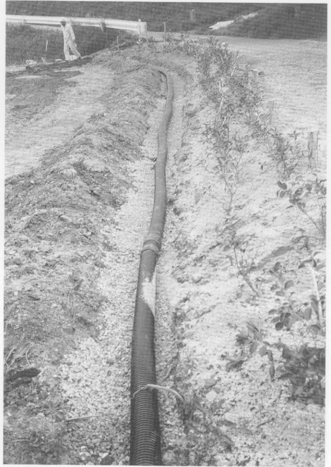
(3) 講堂跡東側暗渠排水管付設状況
