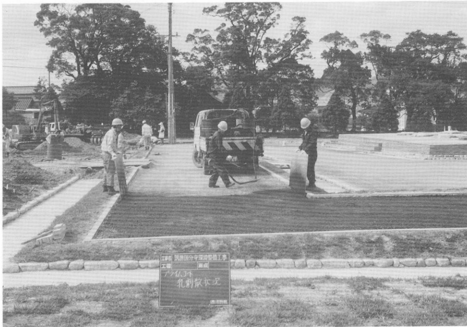
(3) 回廊跡基壇舗装プライムライト乳剤散布状況
