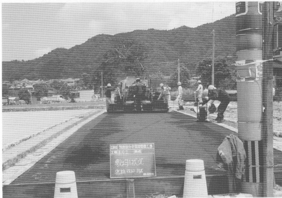
(4) 回廊跡基壇舗装工事
