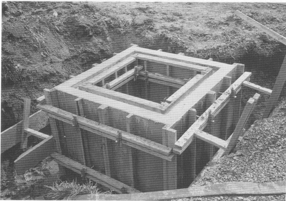
(4) 水路改修溜柵工事
