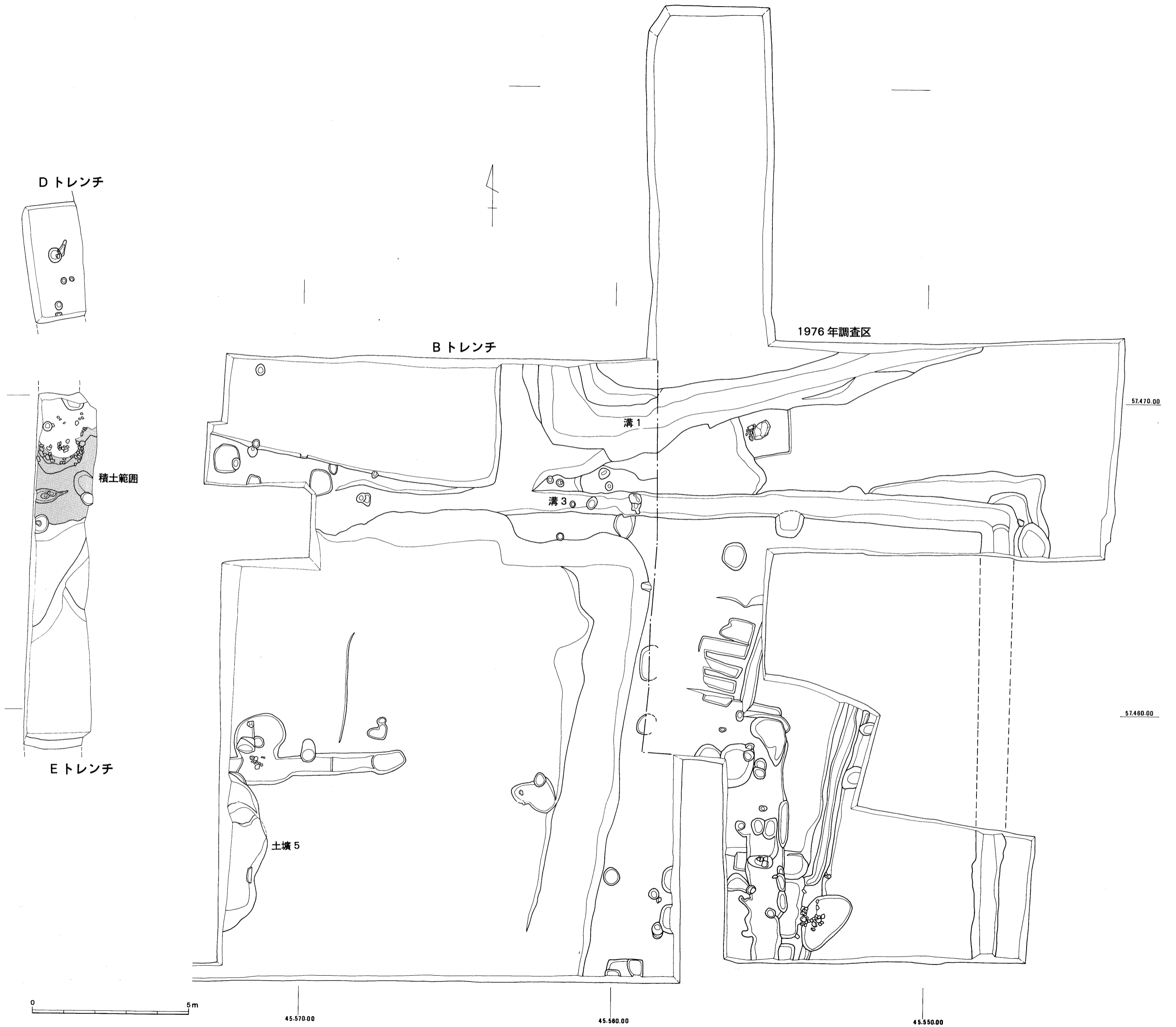
第5図 回廊東北隅遺構実測図 (1/100)
