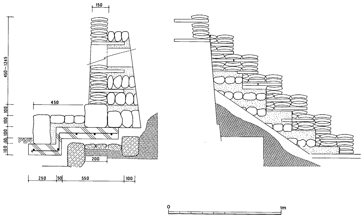
第14図 塔跡瓦積基壇・階段断面図 (1/20)
