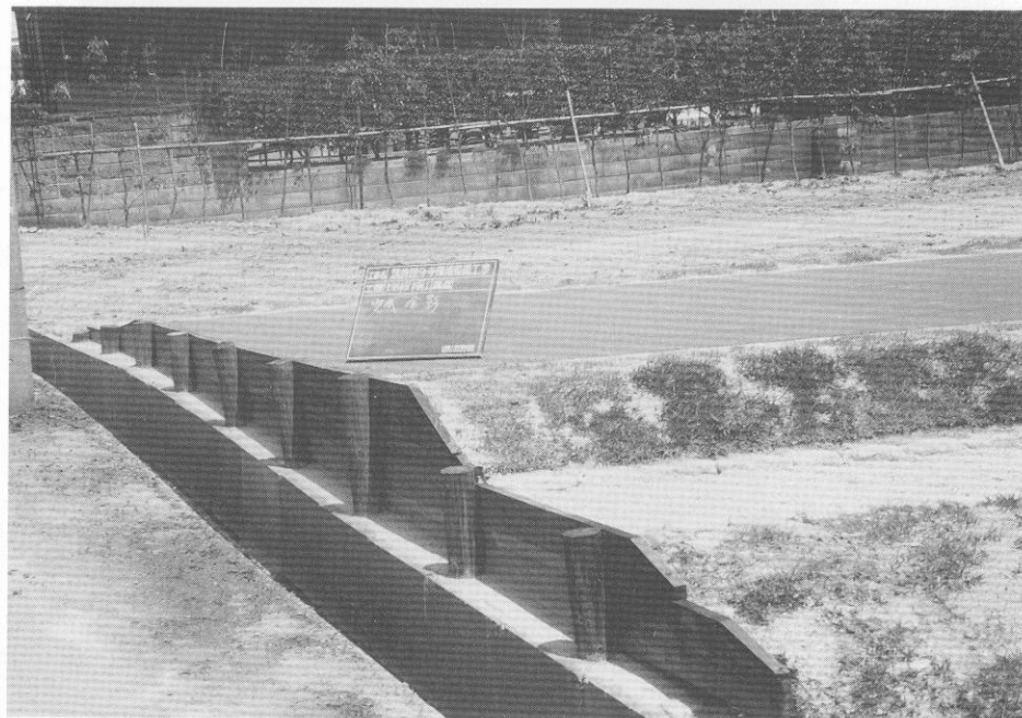
(4) 回廊基壇土留板柵工事
