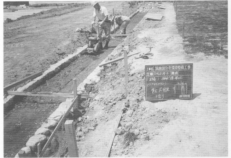
(1) 回廊跡雨落溝床路盤工事
