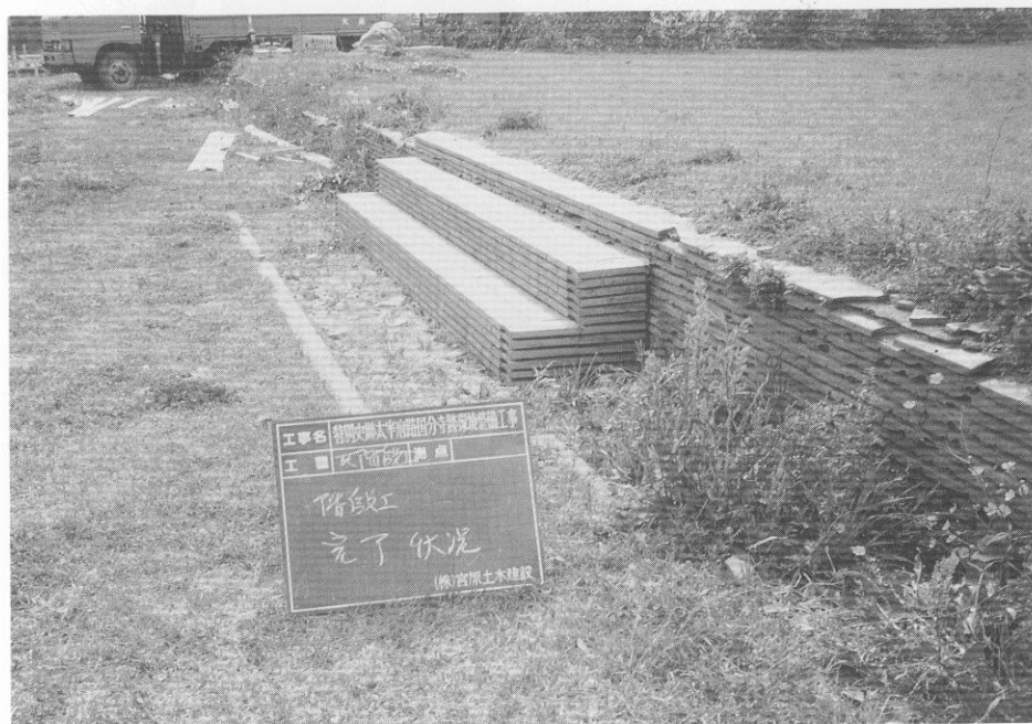
(4) 講堂跡瓦積階段修理完了状況
