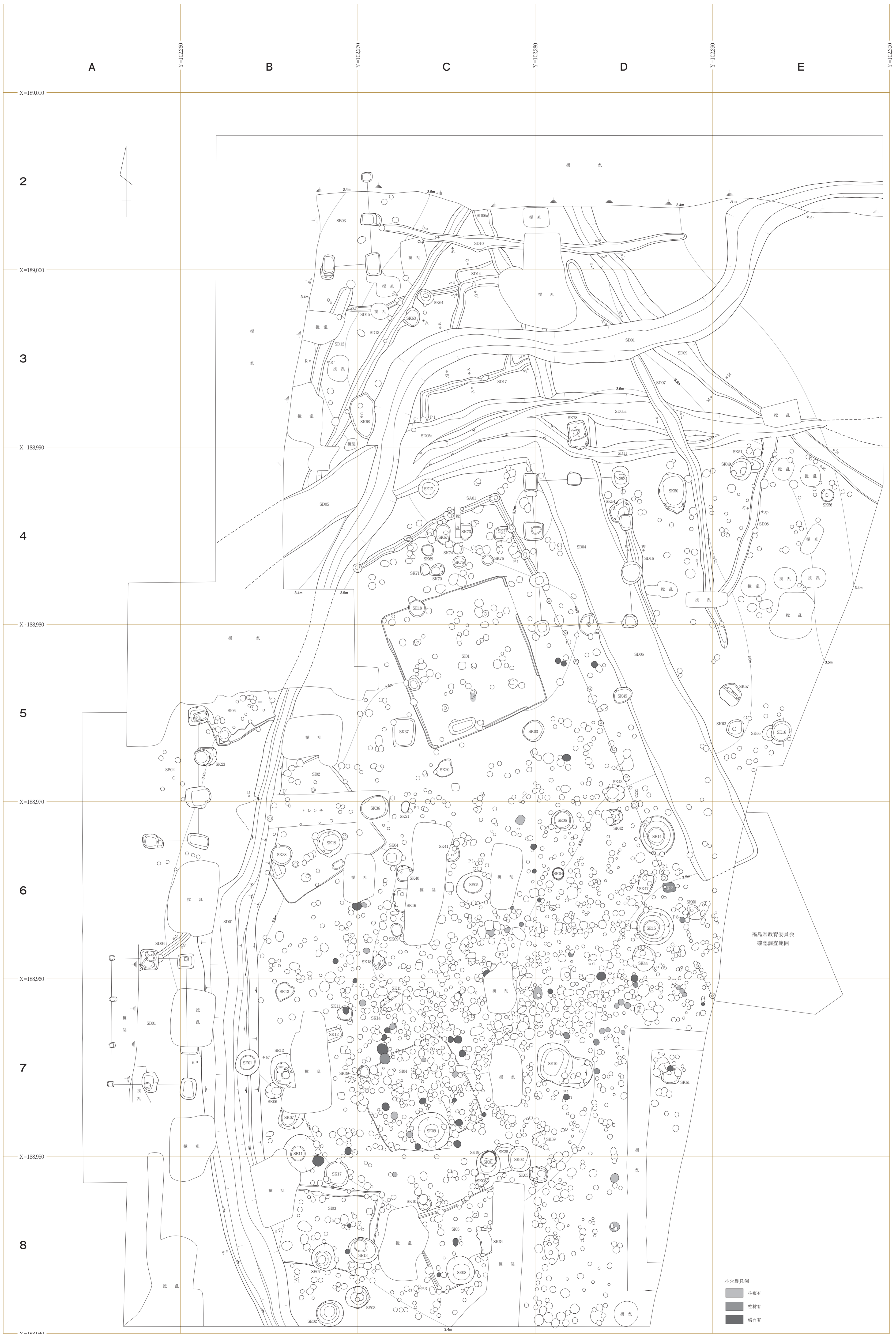
付図1 桶師屋遺跡遺構配置図
