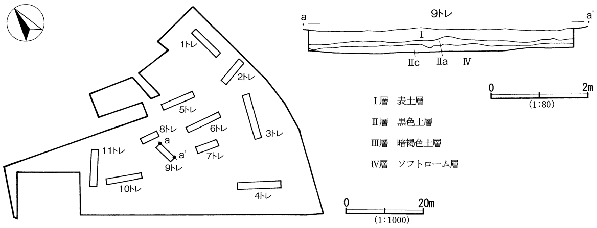
第19図 青柳台遺跡トレンチ配置図
