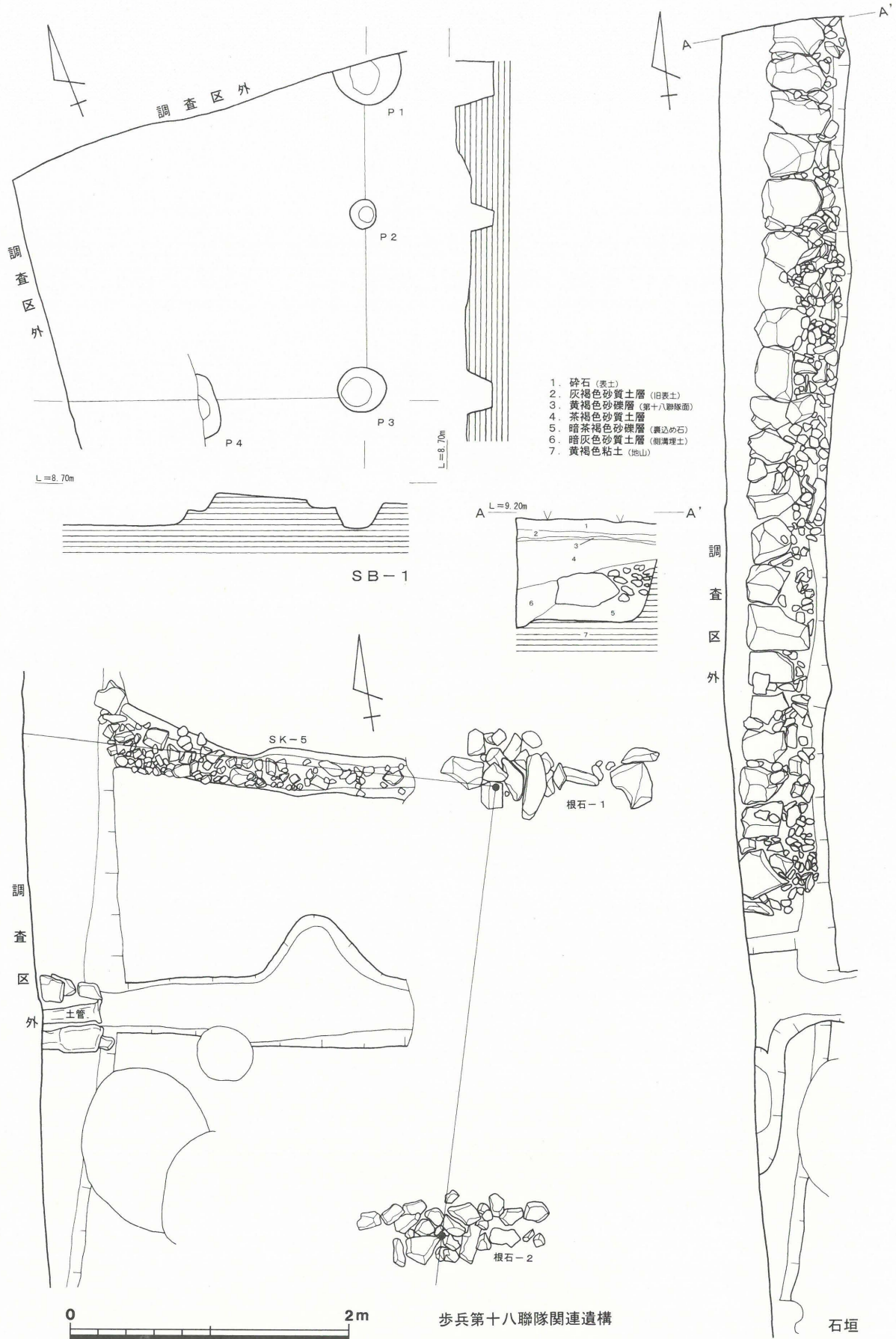
第7図 遺構実測図-1 (1/40)
