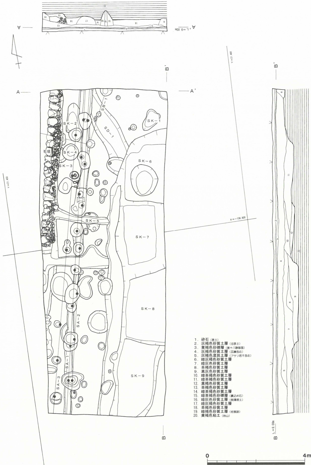
第6図 調査区全体図 (1/80)
