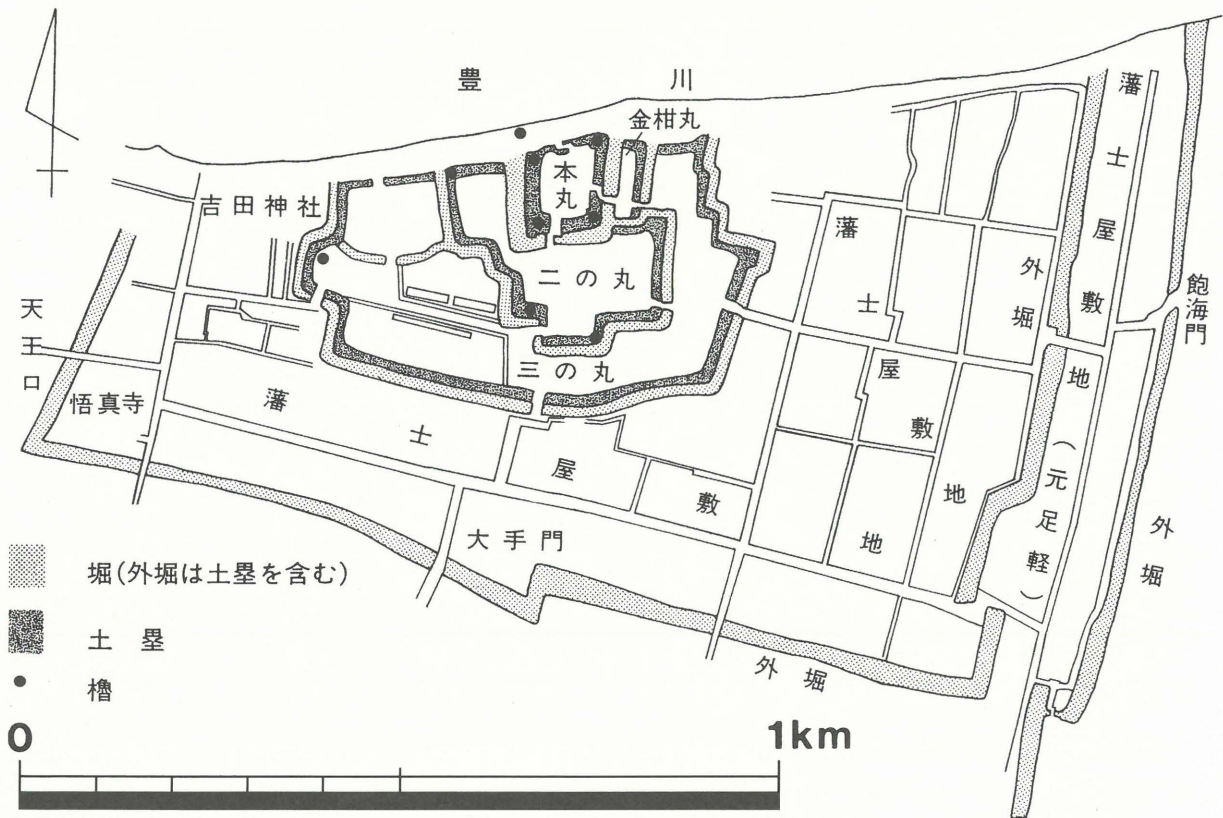
第3図 近世吉田城の構造 (1/10,000)
