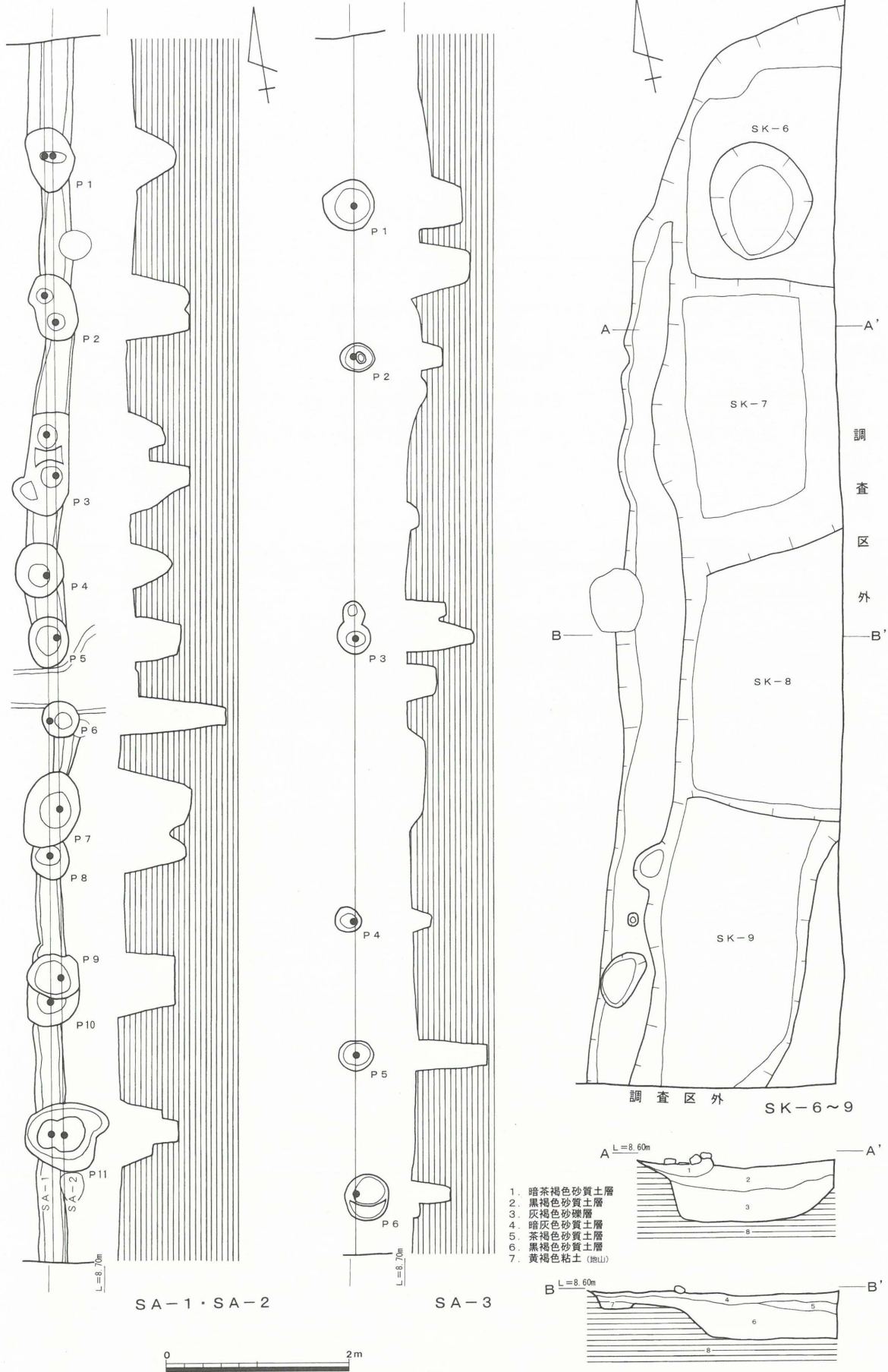
第8図 遺構実測図-2 (1/40)
