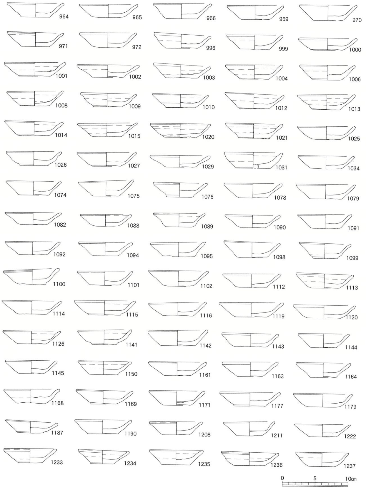
第31図 遺物実測図(皿2 遺構)
