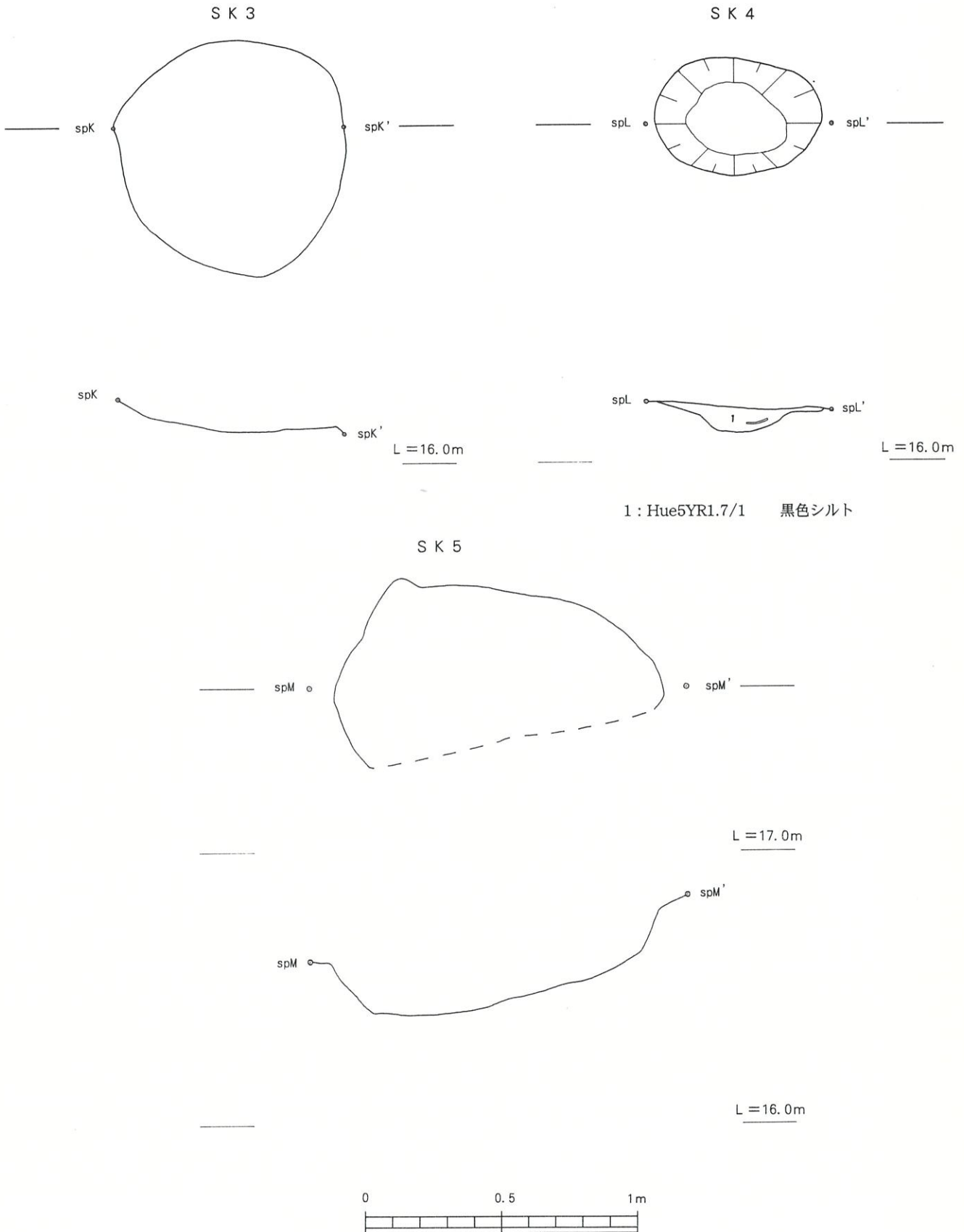
第20図 S K 3 ・ S K 4 ・ S K 5 平面断面図
