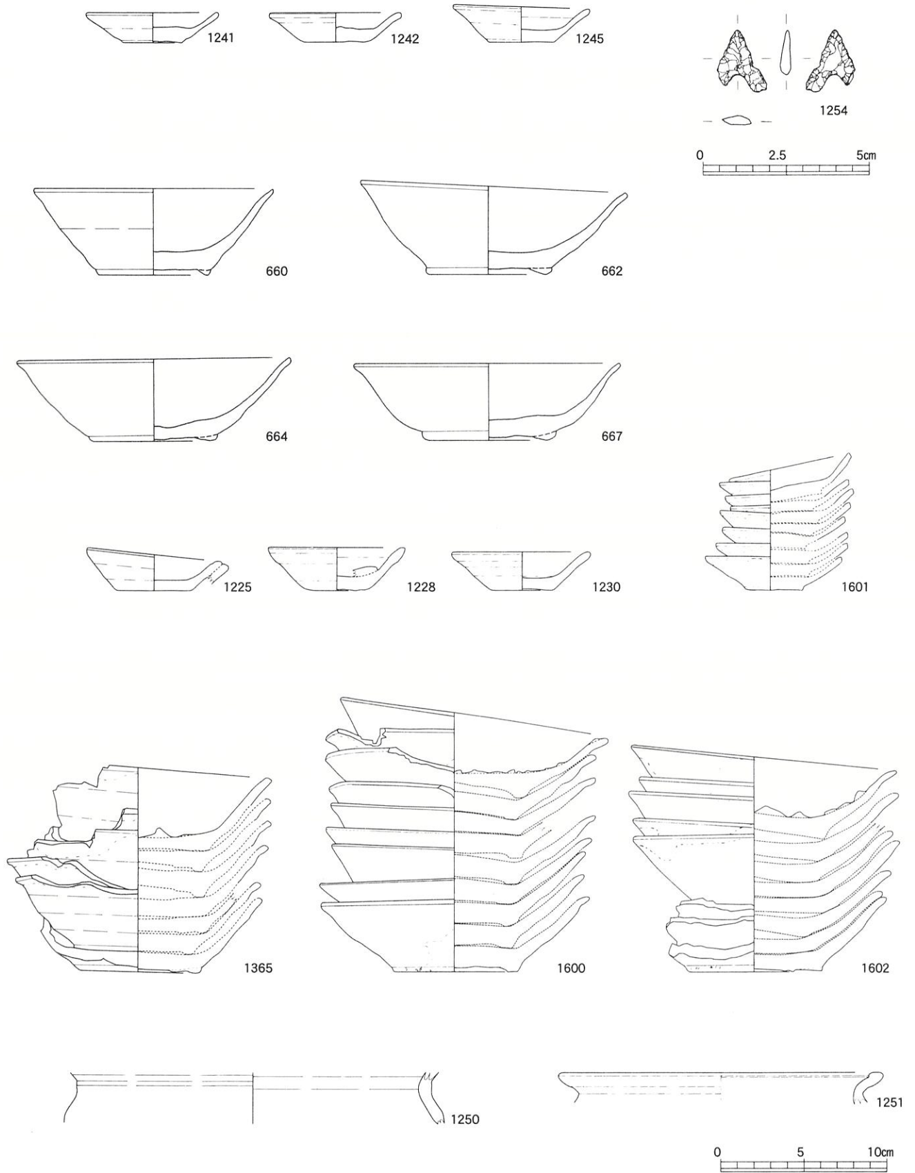
第33図 遺物実測図(その他)
