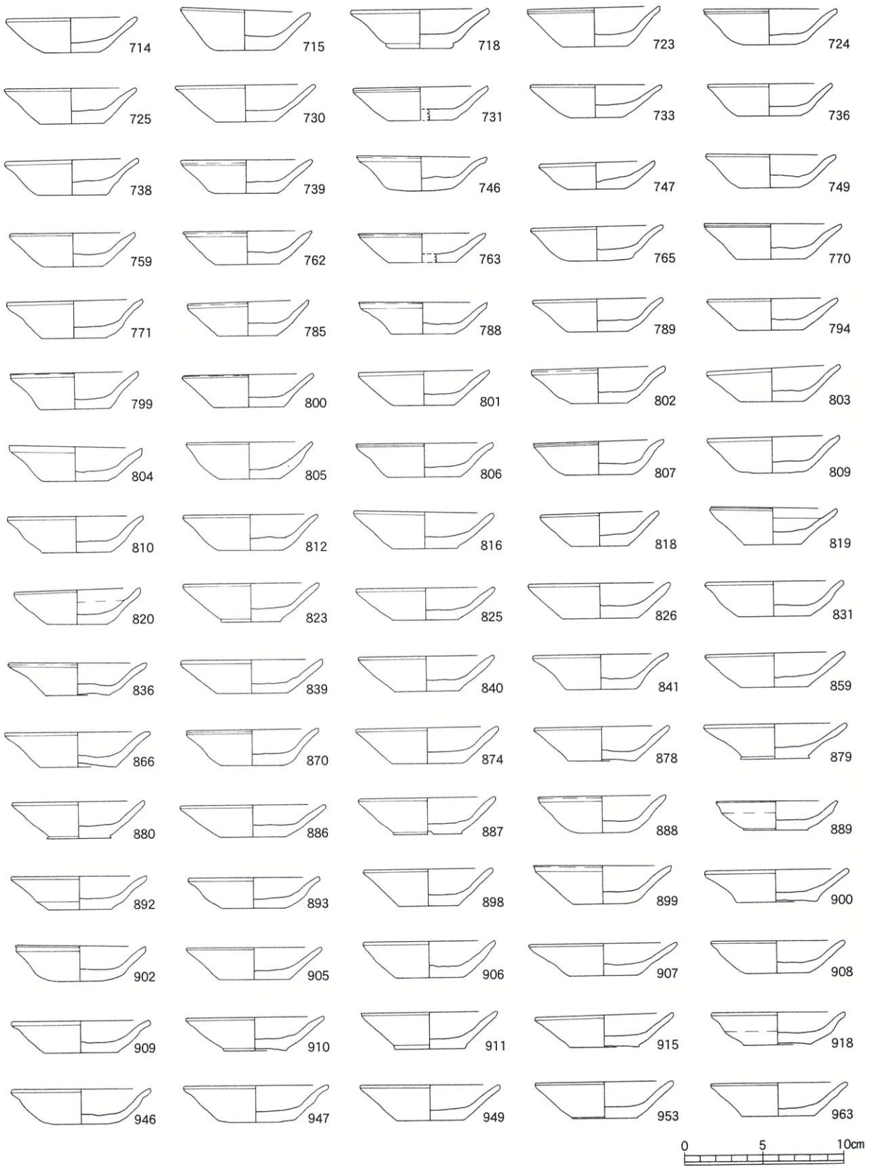
第30図 遺物実測図(皿1 遺構)
