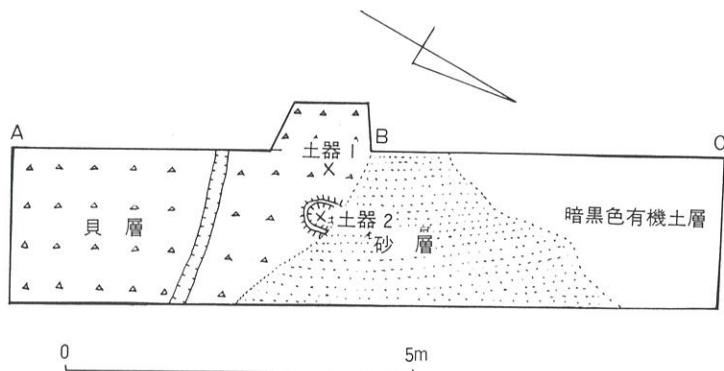
第4図の1 第1トレンチ平面図
