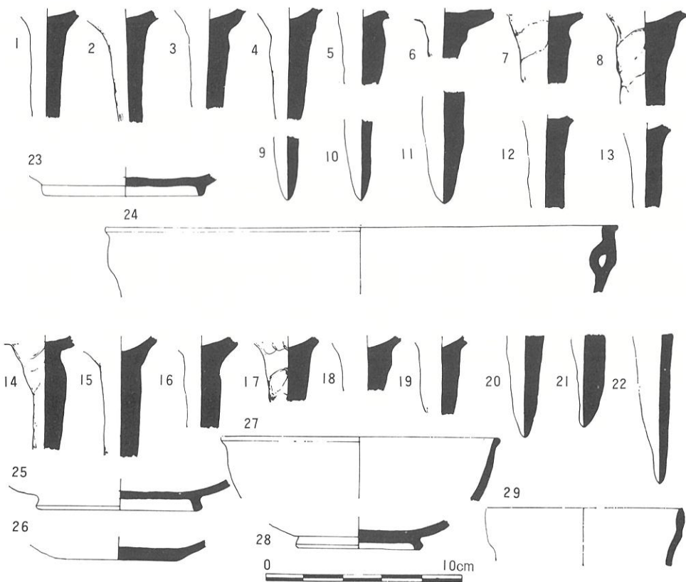
第15図 第3トレンチ出土 遺物実測図
