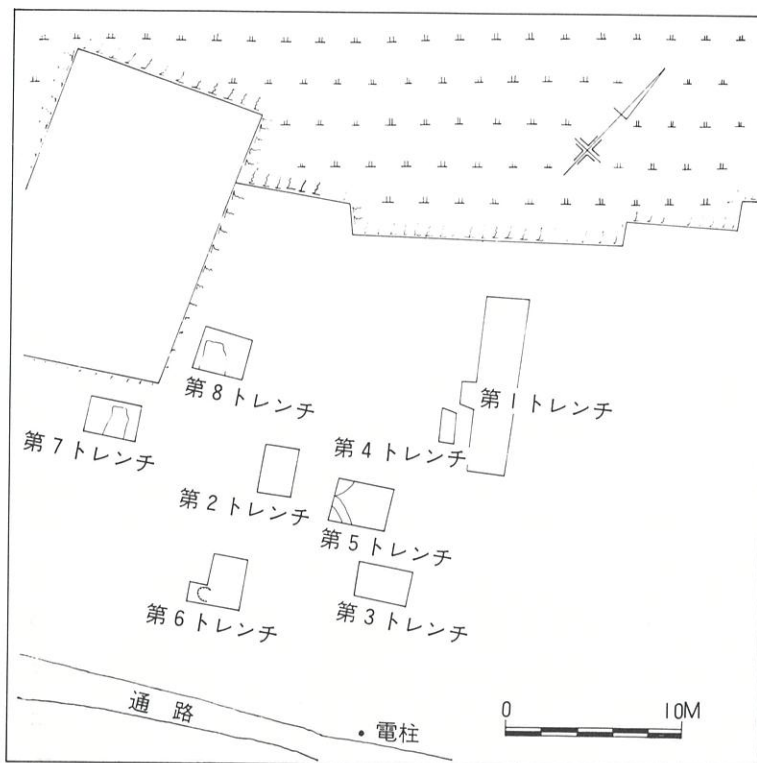
第3図 第1次・第2次発掘区平面図
