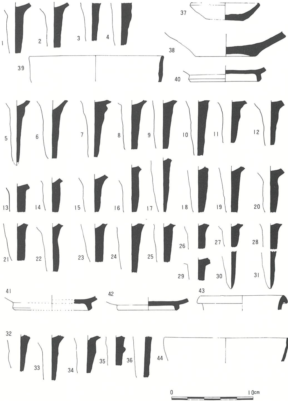
第13図 第2トレンチ出土 遺物実測図
