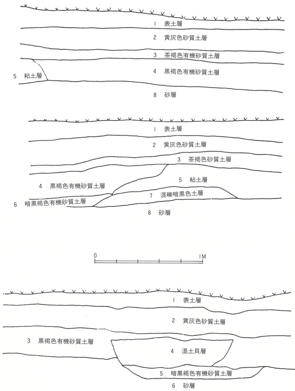
第6図 第2トレンチ・第3トレンチ断面実測図 上段：第2トレンチ北壁 中段：第2トレンチ西壁 下段：第3トレンチ北壁
