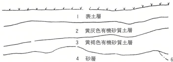
第8図 第6トレンチ断面実測図
