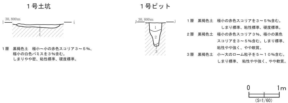
第14図 1号土坑、1号ピット断面図
