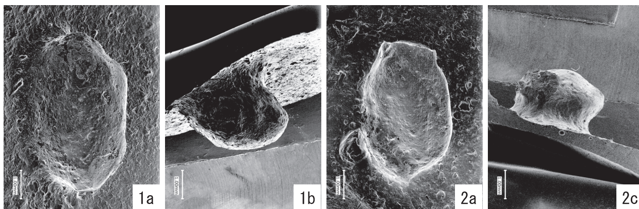
国分宿遺跡 25 次調査出土時圧痕レプリカの走査型電子顕微鏡写真
