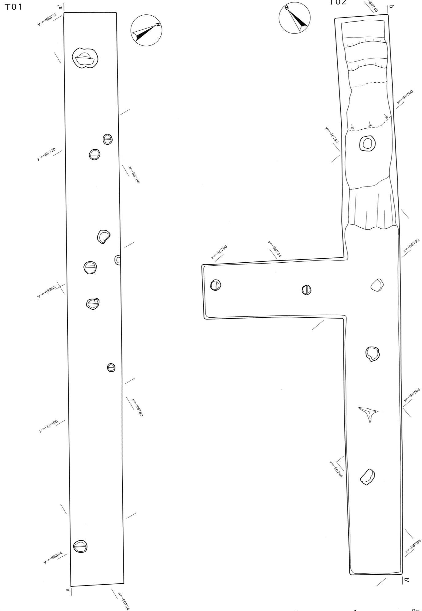
図7 T01T02遺構平面図 (S=1/40)
