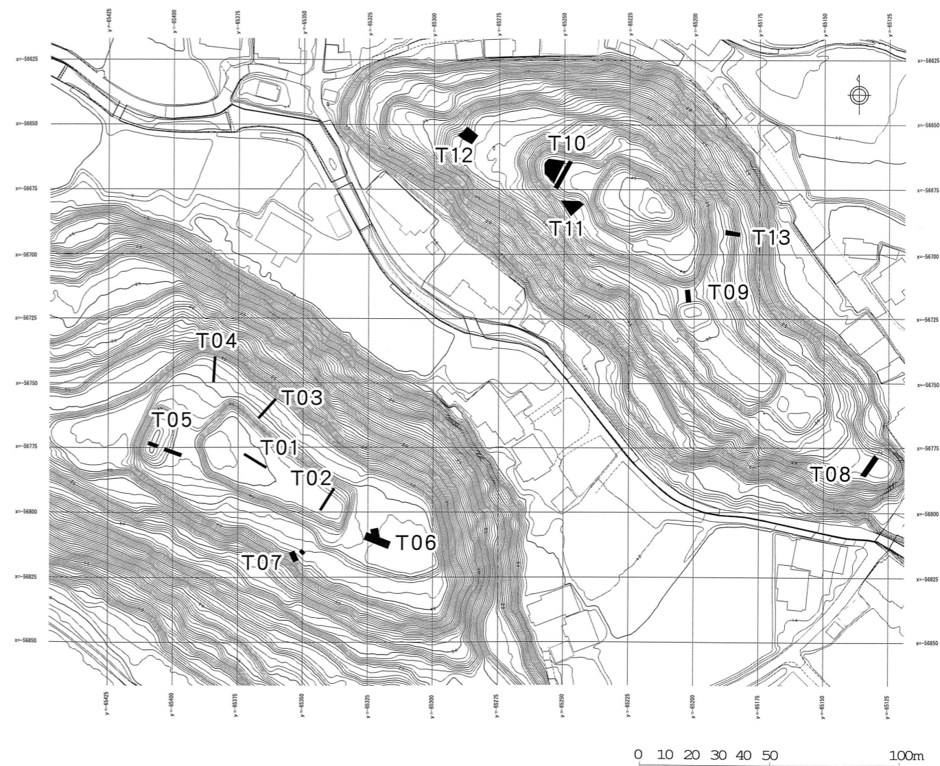
図6 調査トレンチ配置図 (S= 1/2000)
