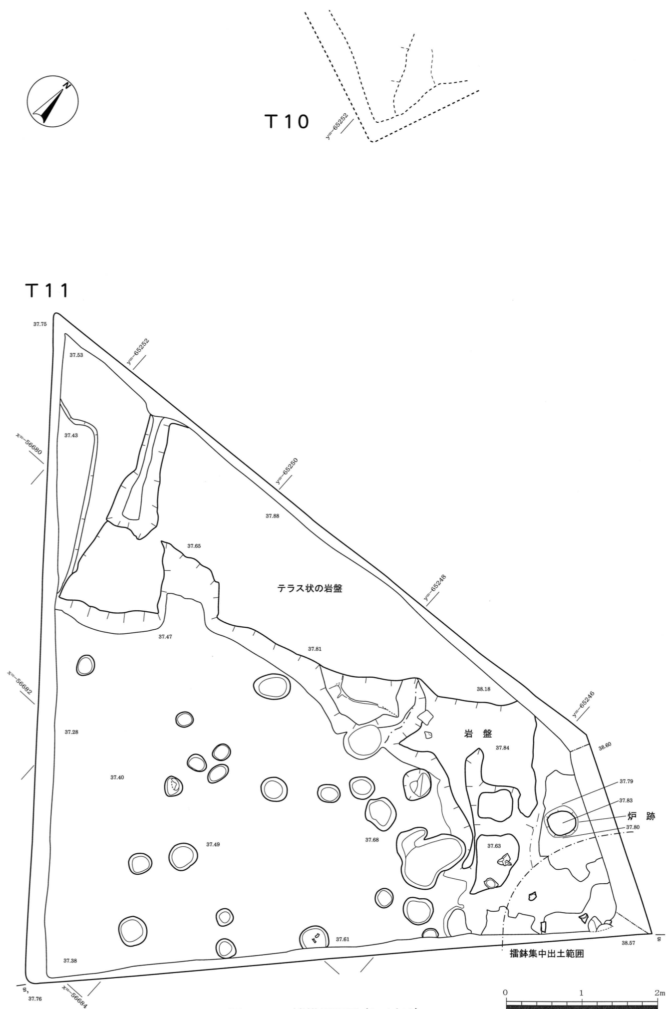
図15 T11遺構平面図(S=1/40)
