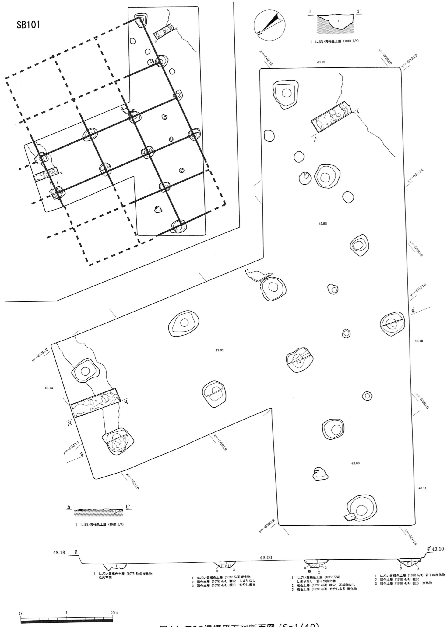
図11 T06遺構平面図断面図 (S=1/40)
