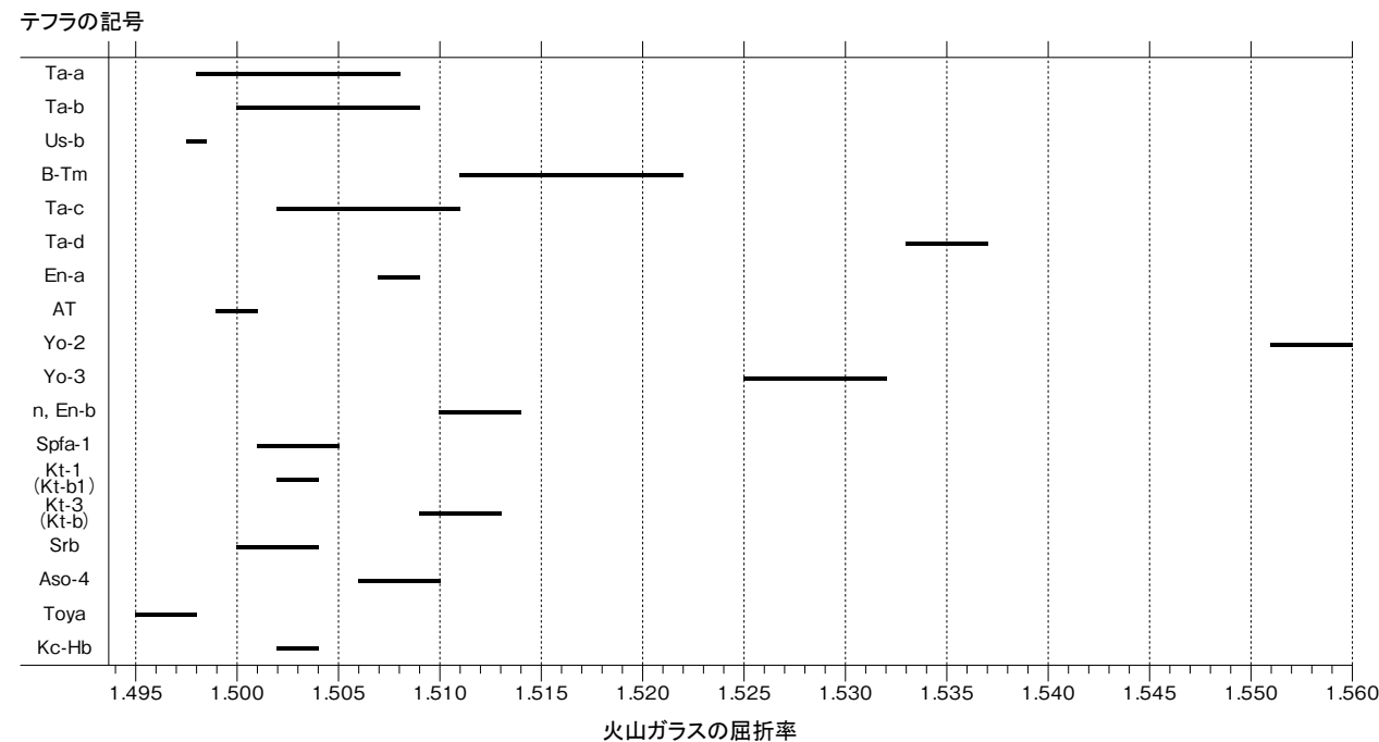
石狩低地帯周辺に分布する可能性のある第四紀後期テフラの火山ガラスの屈折率の分布範囲
