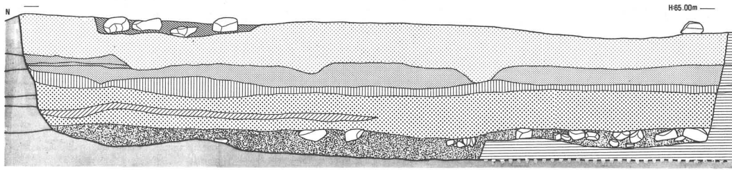
SB1800基壇築成断面図
