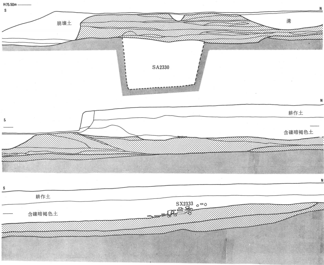
SA2300築成断面図
