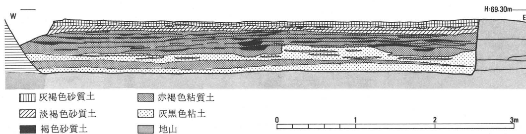
SB3600基壇築成断面図
