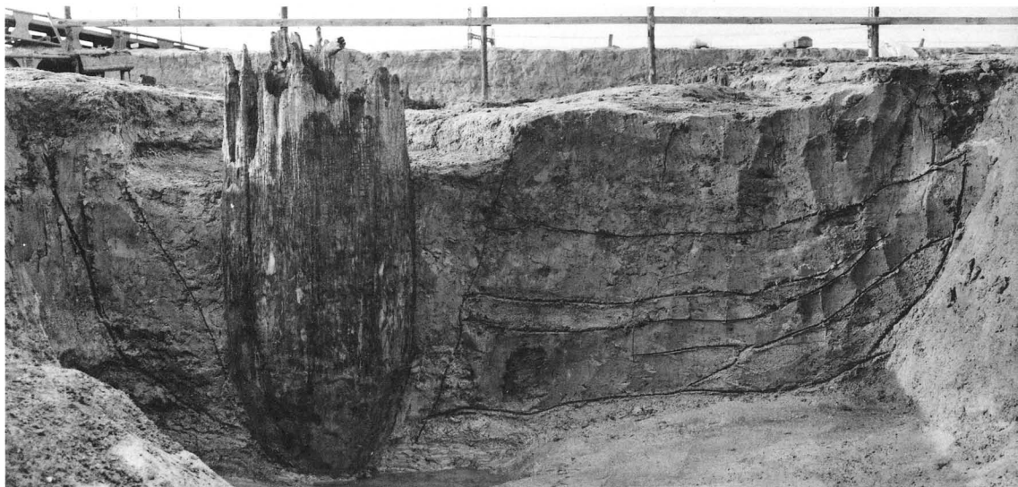
3. SX1830東柱根・ 溝SD1900土層 北から
