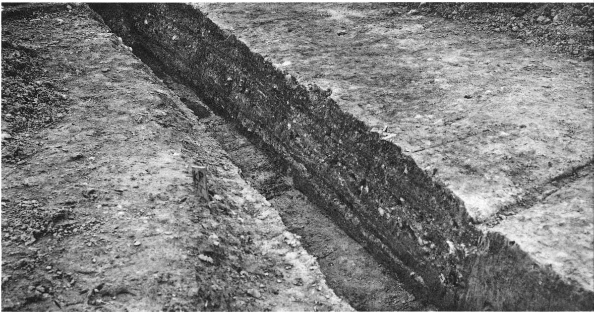
2. 佐伯門SB3600 基壇掘込み地業 と版築 東南から
