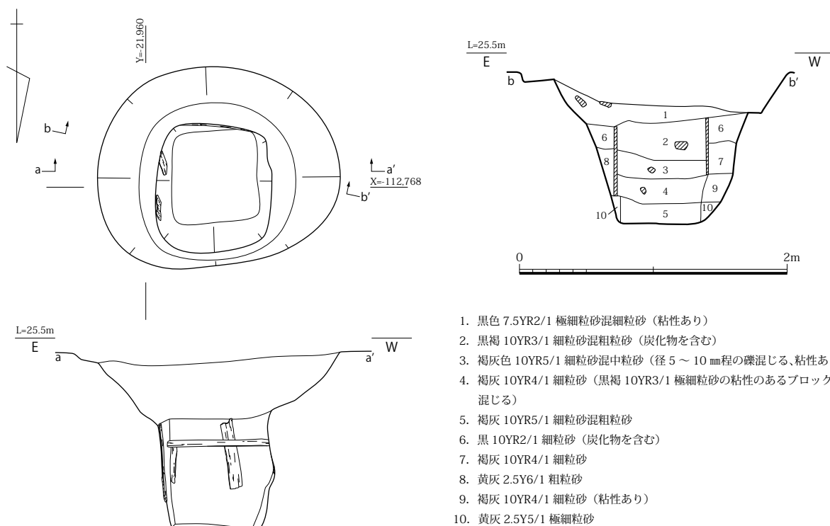
図 66 SE5400 平面・立面・土層断面図 (S=1/40)
