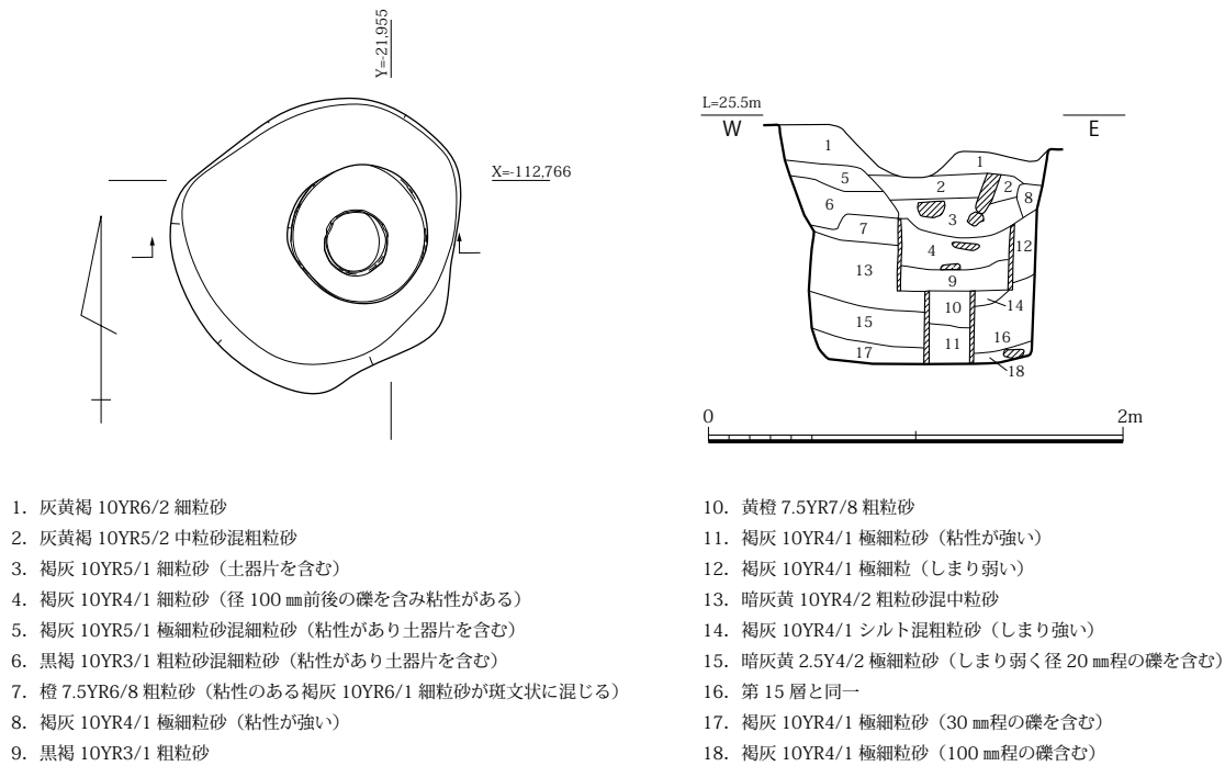
図 69 SE5493 平面・土層断面図 (S=1/40)
