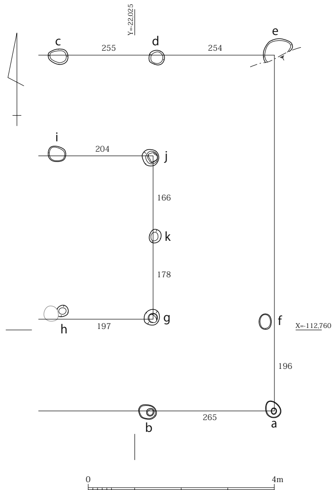
図 54 SB0930 平面図 (S=1/80)
