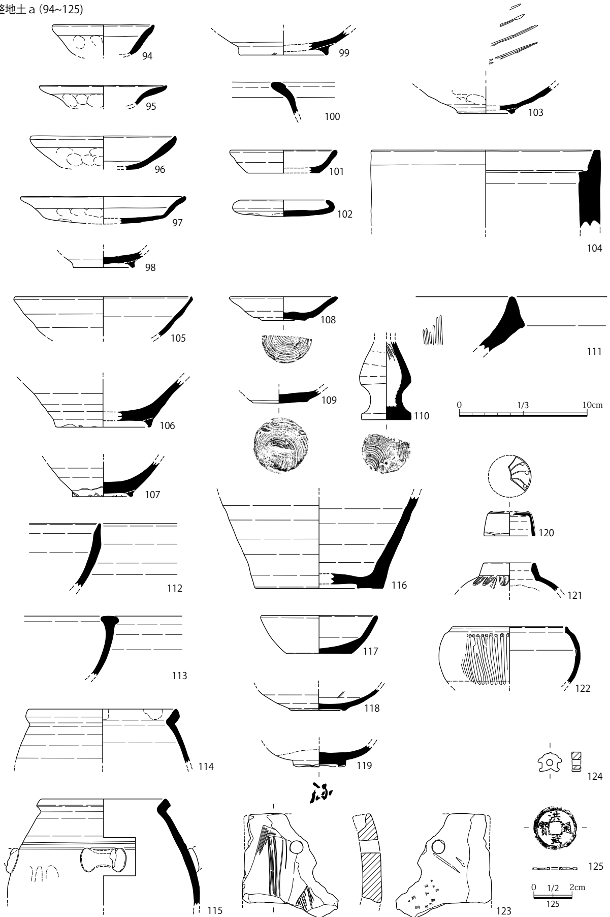
図 23 整地土 a 出土遺物実測図 (S=1/2・1/3)
