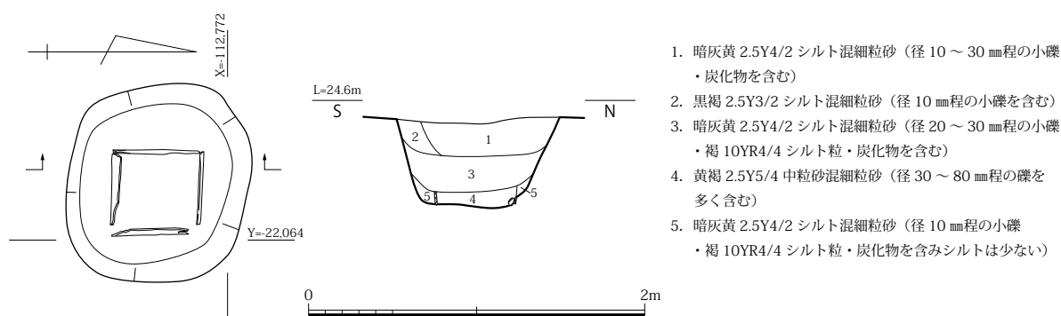
図 108 SE1670 平面・土層断面図 (S=1/40)
