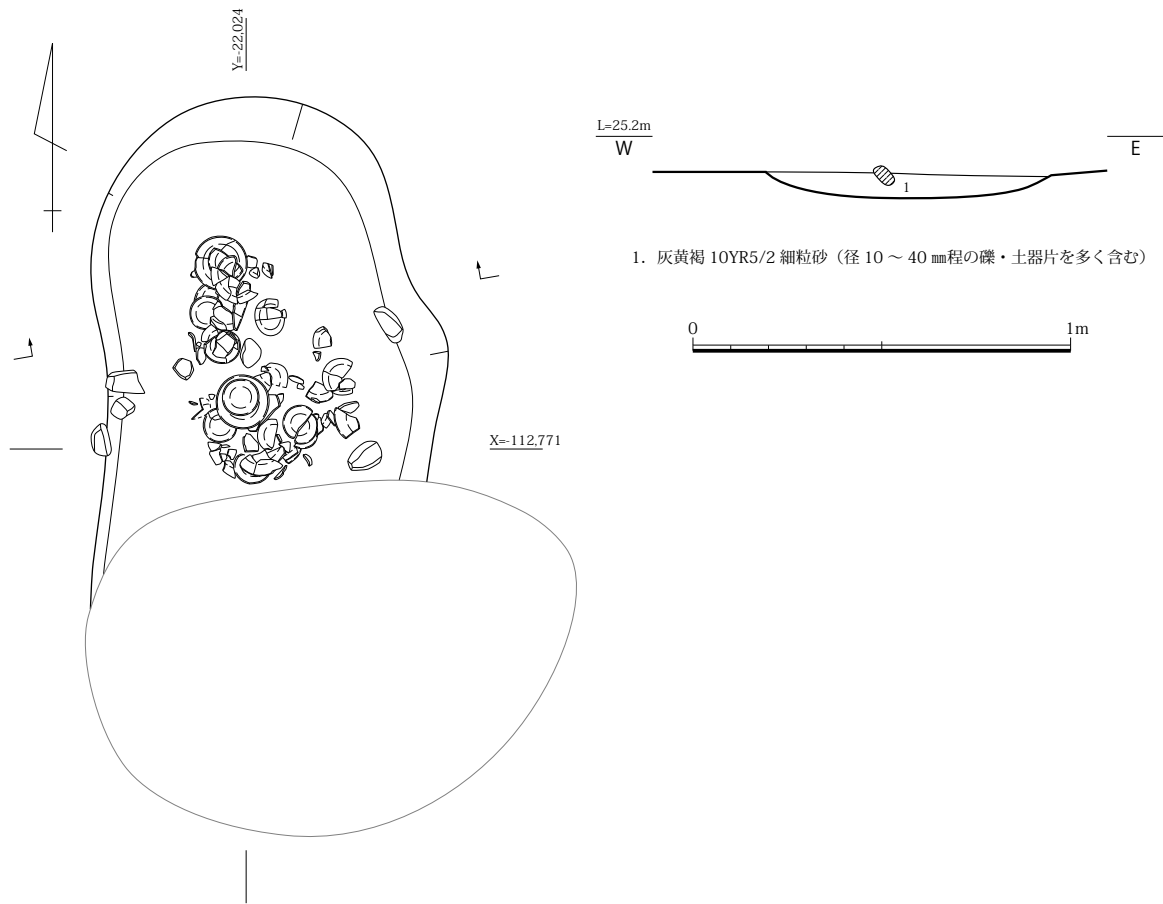
図 116 SK0290 平面・土層断面図 (S=1/20)
