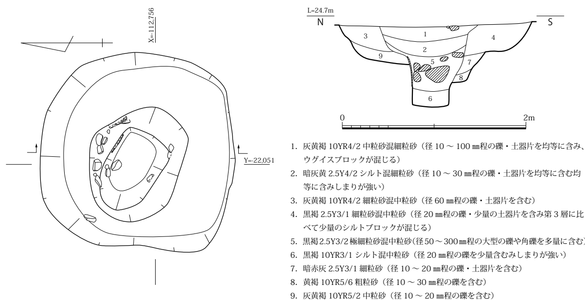
図 136 SE1290 平面・土層断面図 (S=1/40)
