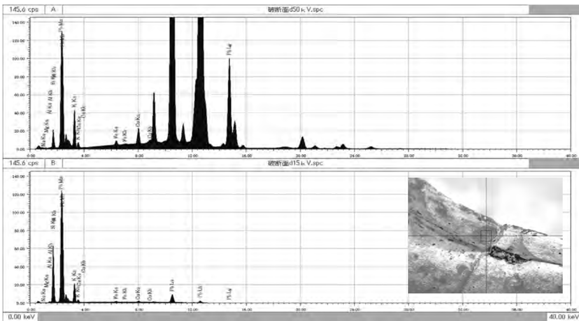
図 184 ガラス水滴欠損部 d の XRF スペクトル (上段 : 50kV、下段 : 15kV)
