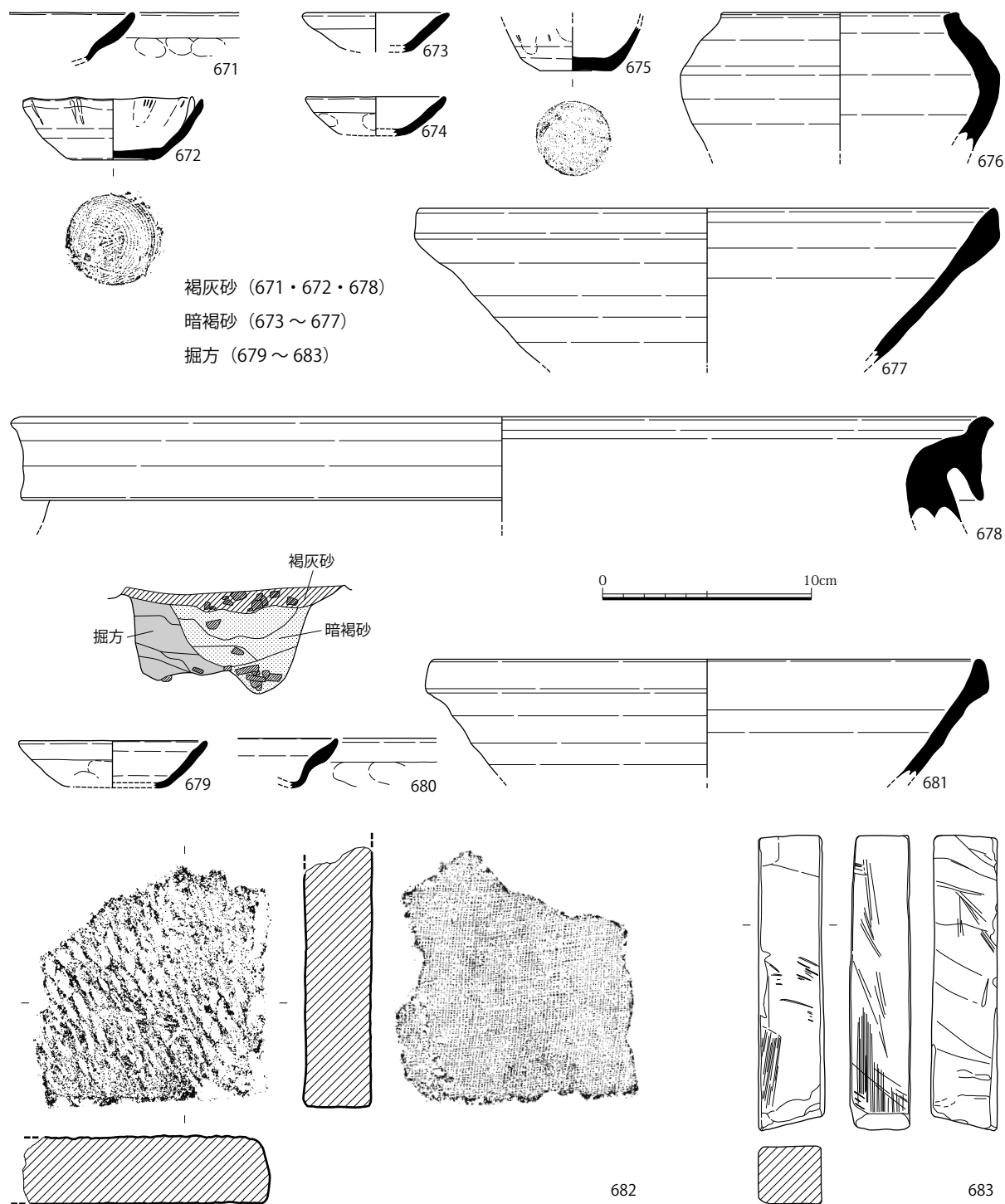
図 155 SE5160 出土遺物実測図 (S=1/3)
