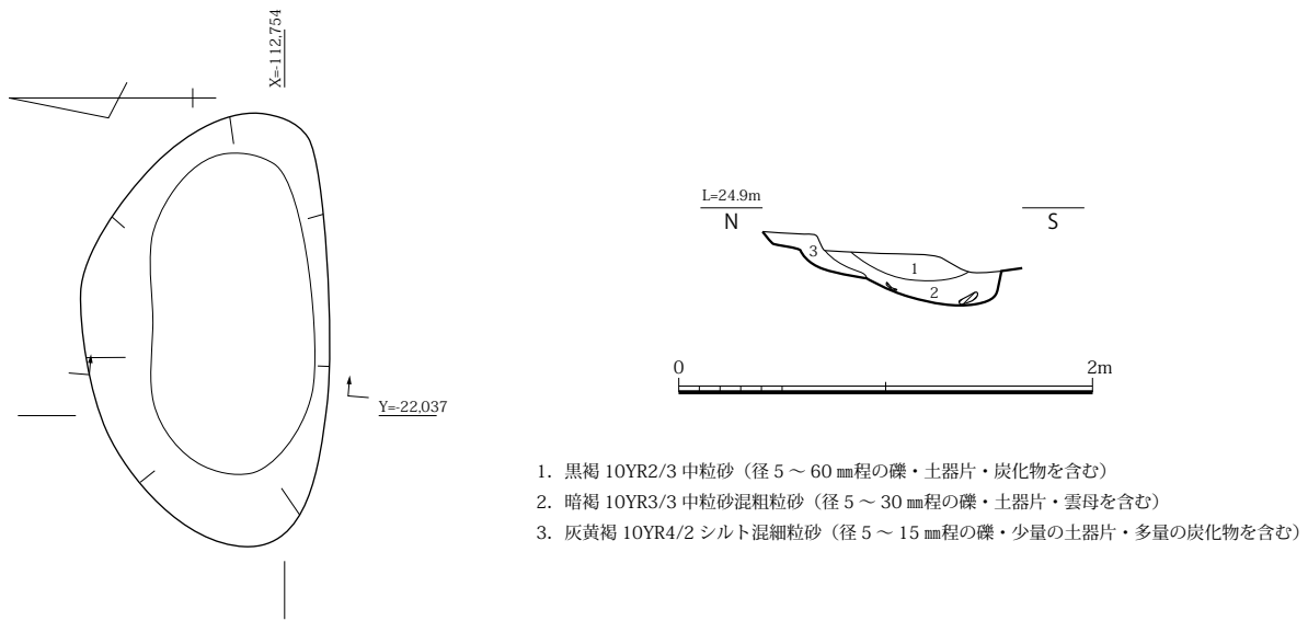
図 144 SK1090 平面・土層断面図 (S=1/40)
