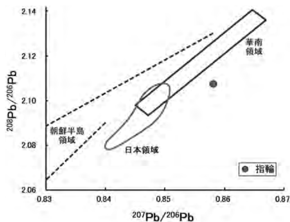
図 178 整地土 2 出土指輪の鉛同位体比 (A 式図)
