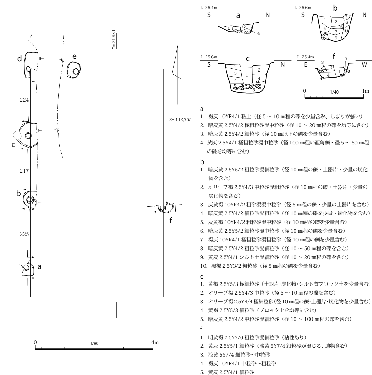
図 43 SB5650 平面・土層断面図 (平面 S=1/80・断面 S=1/40)
