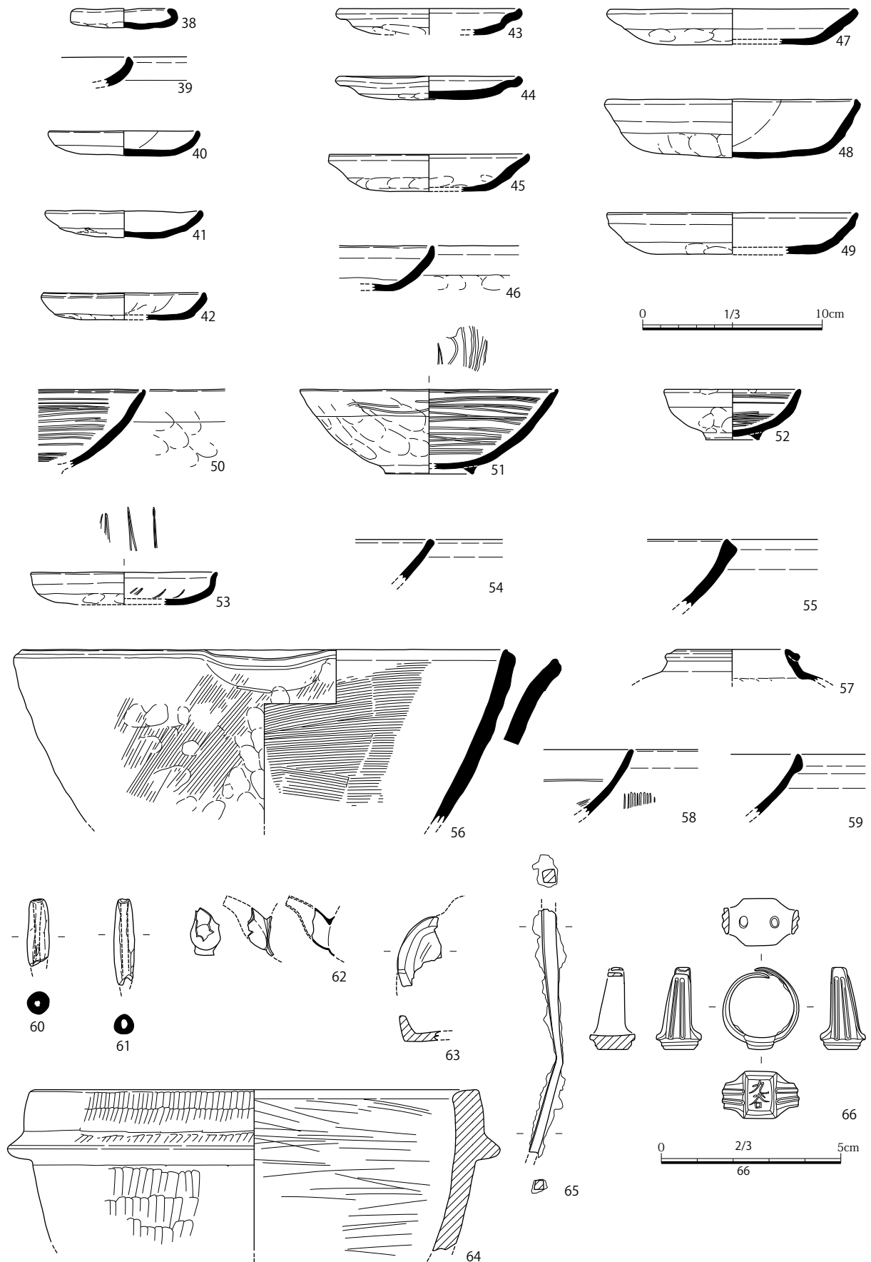
图 21 整地土 2 出土遺物実測図 (S=1/3・2/3)
