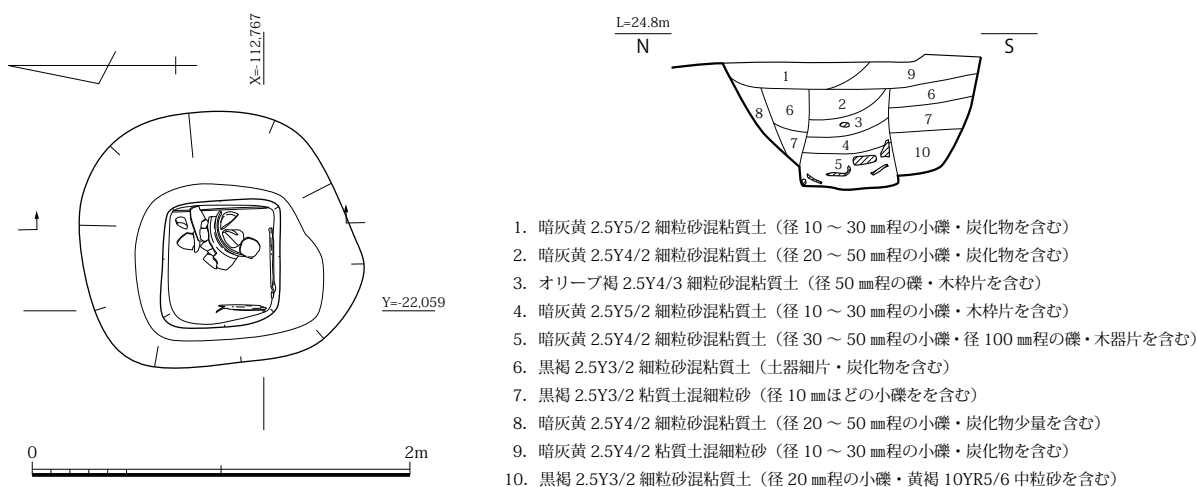
図 106 SE1430 平面・土層断面図 (S=1/40)
