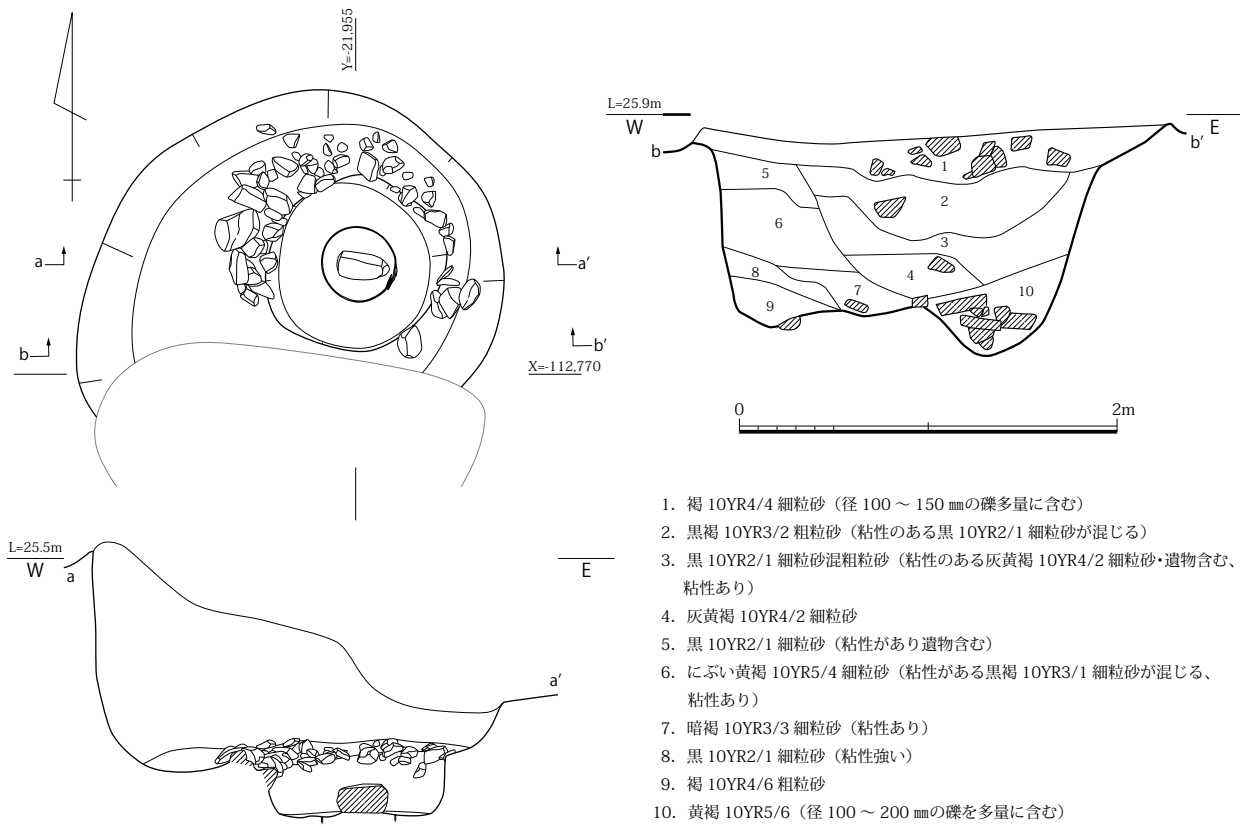
図 141 SE5160 平面・立面・土層断面図 (S=1/40)
