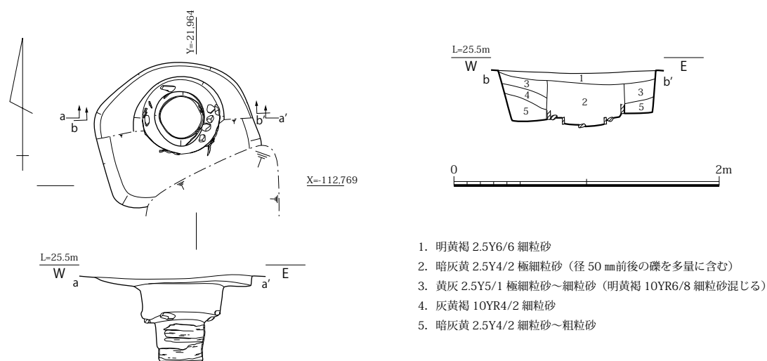
図 63 SE5180 平面・立面・土層断面図 (S=1/40)
