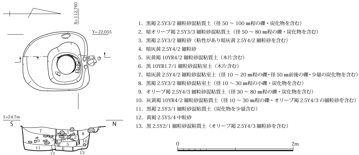
図 101 SE1330 平面・土層断面図 (S=1/40)
