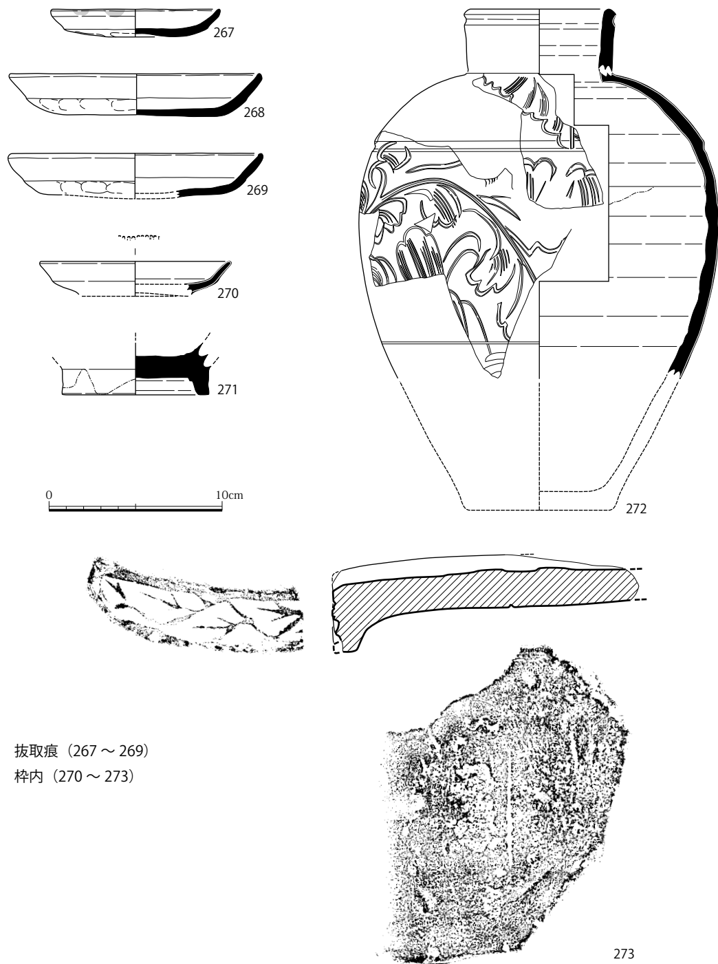
図 82 SE0590 出土遺物実測図 (S=1/3)
