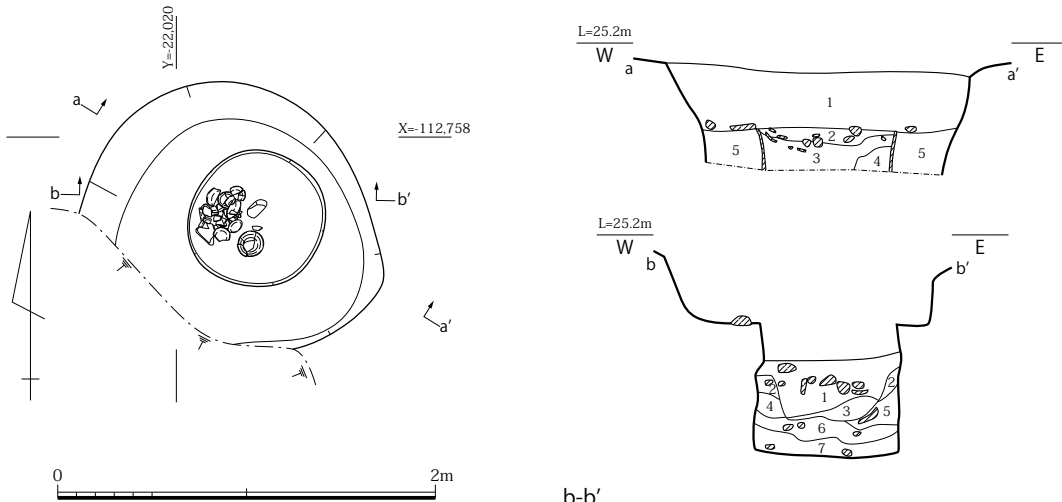
図 95 SD0020・0030・0040 土層断面図 (S=1/40)
