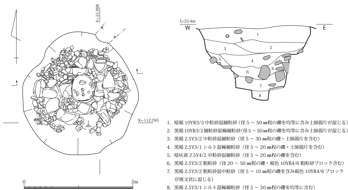
図 97 SE0780 平面・土層断面図 (S=1/40)
