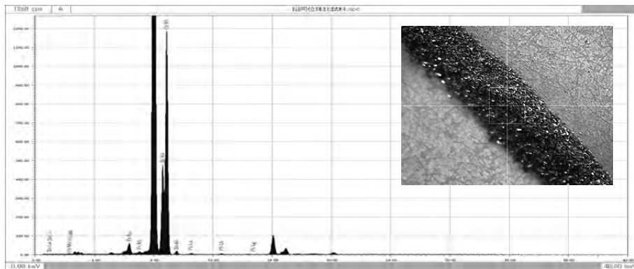
図 174 鉛同位体比測定試料の蛍光 X 線分析スペクトル (試料採取箇所を図 175 に示す。)
