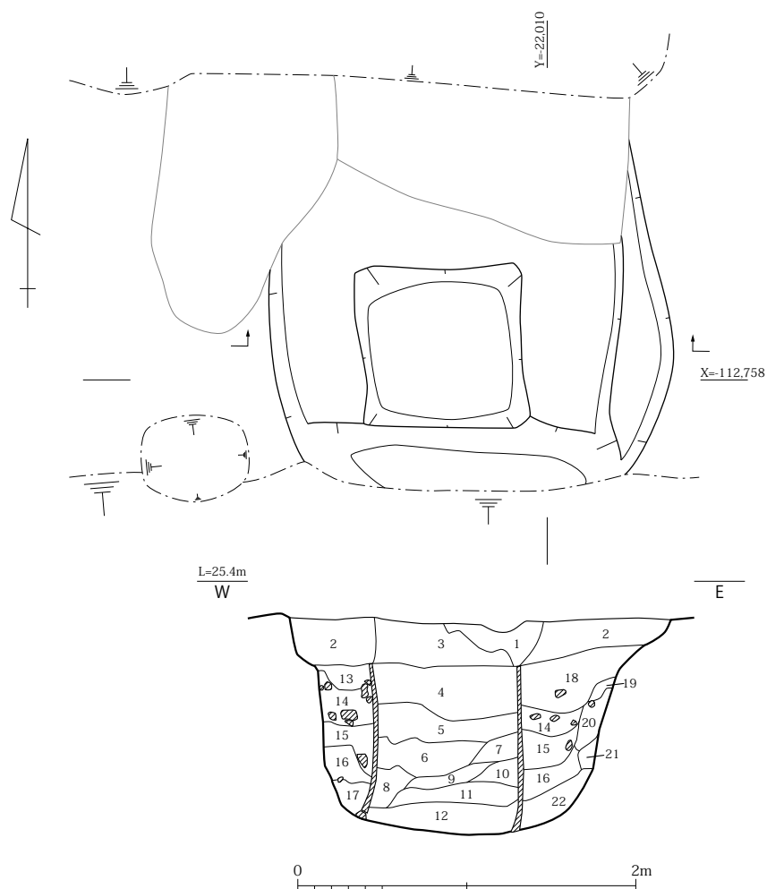
図 133 SD5150 土層断面図 (S=1/40)
