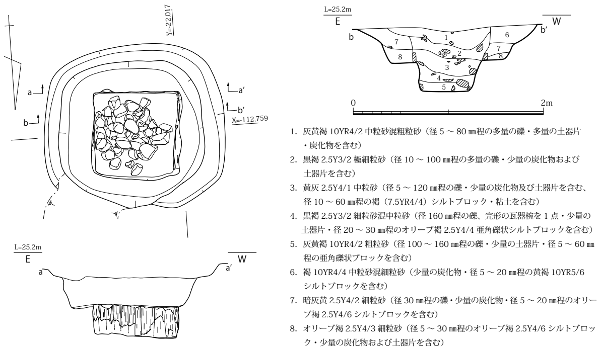
図 56 SE0360 平面・立面・土層断面図 (S=1/40)
