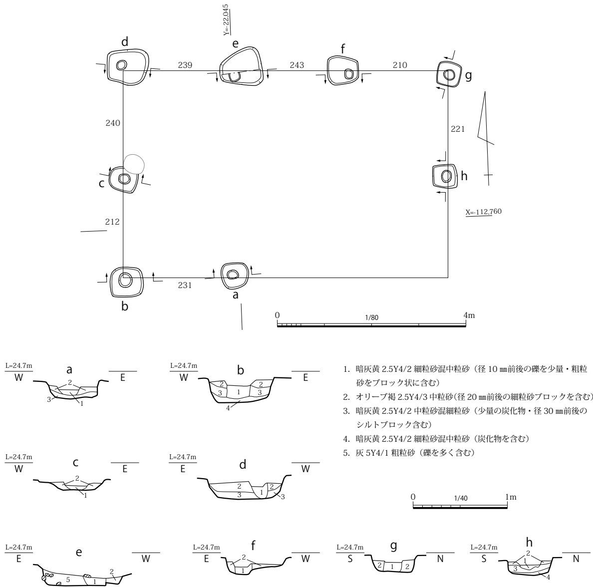
図 39 SB3030 平面・土層断面図 (平面 S=1/80・断面 S=1/40)
