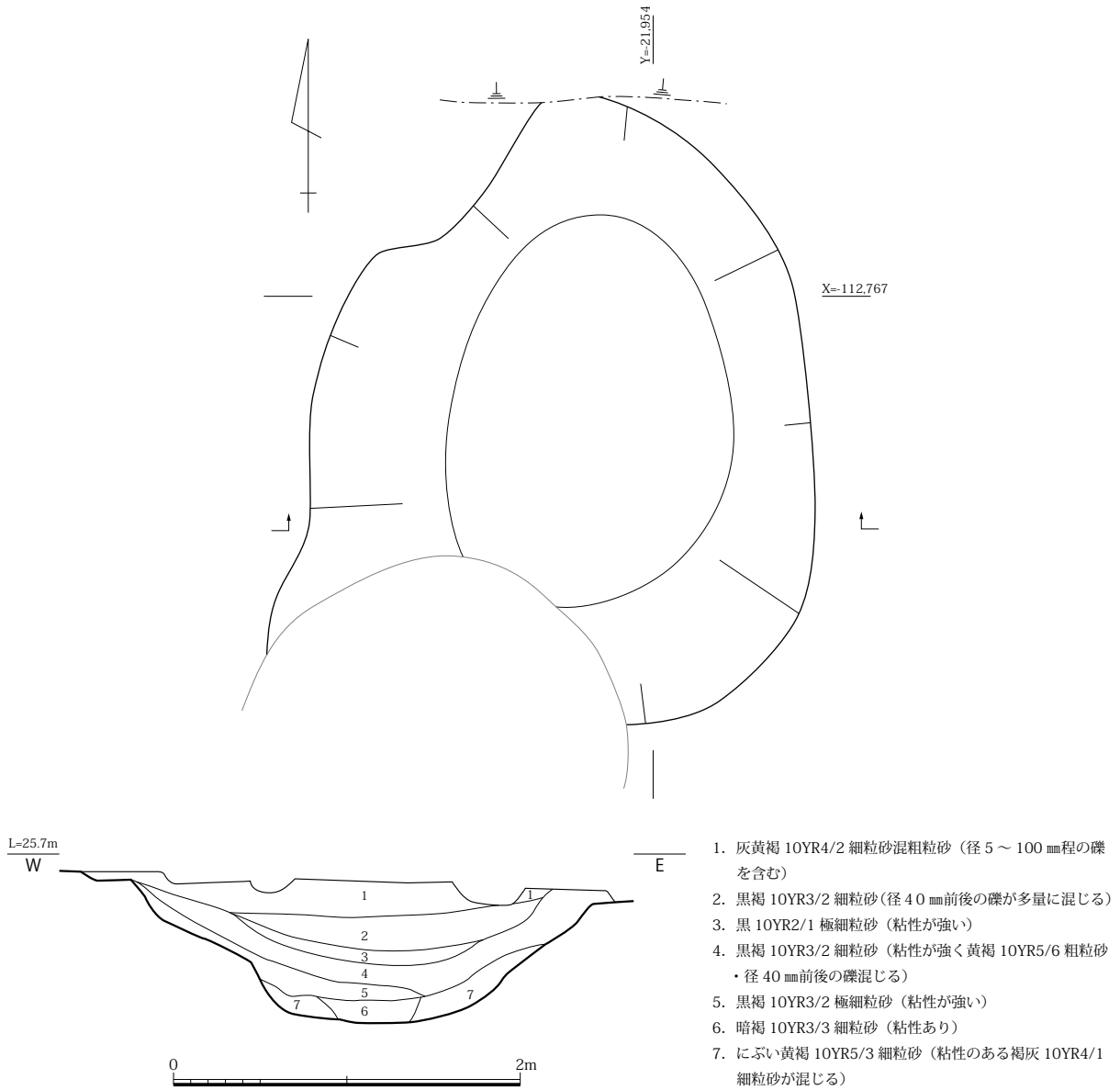
図 140 SE5090 平面・土層断面図 (S=1/40)
