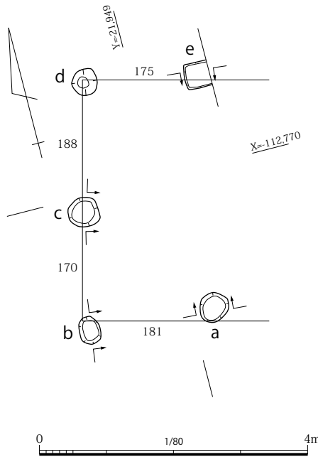
図 27 SB5620 平面・土層断面図 (平面 S=1/80・断面 S=1/40)
