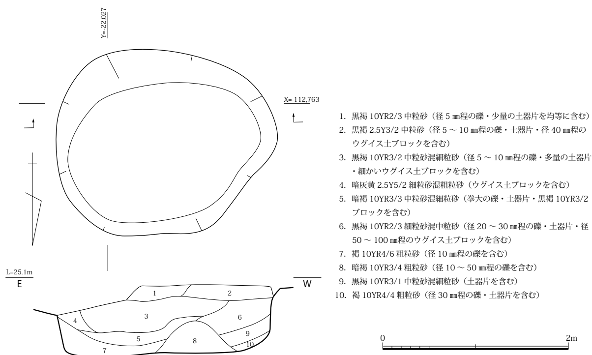
図 115 SK0260 平面・土層断面図 (S=1/40)
