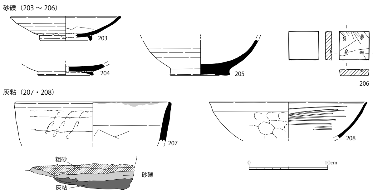
図 51 SD1750 出土遺物実測図 (2) (S=1/3)
