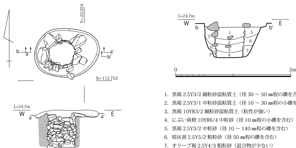
図 105 SE1390 平面・立面・土層断面図 (S=1/40)
