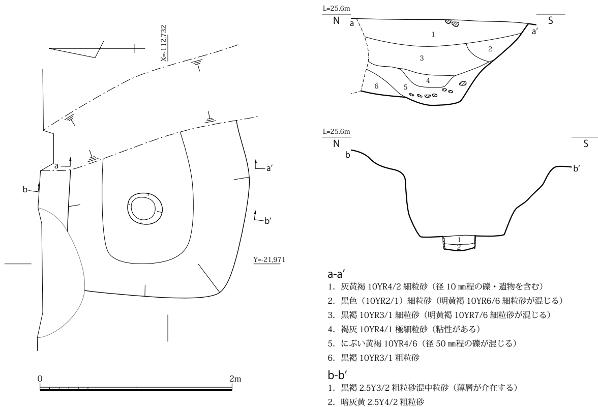
図 64 SE5189 平面・土層断面図 (S=1/40)
