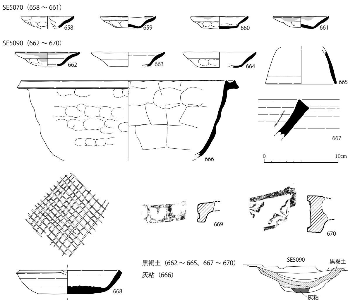
図 154 SE5070・5090 出土遺物実測図 (S=1/3)
