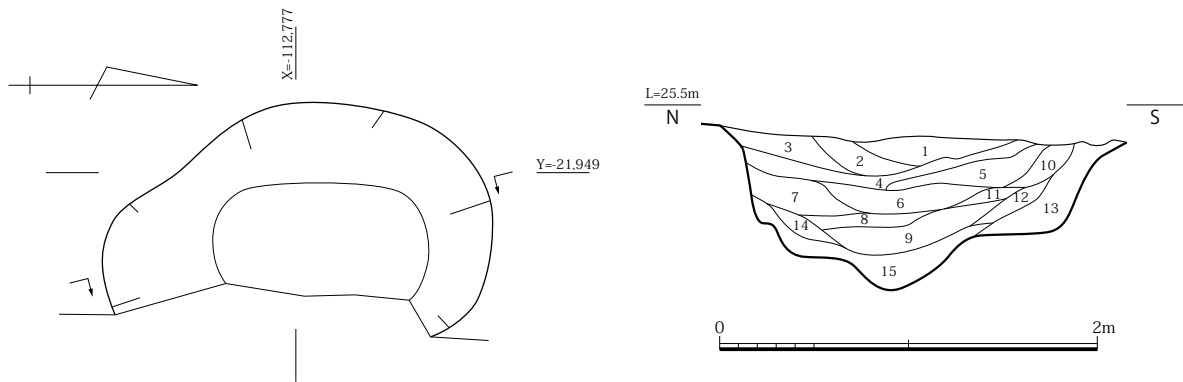
図 76 SK0670 平面・土層断面図 (S=1/40)
