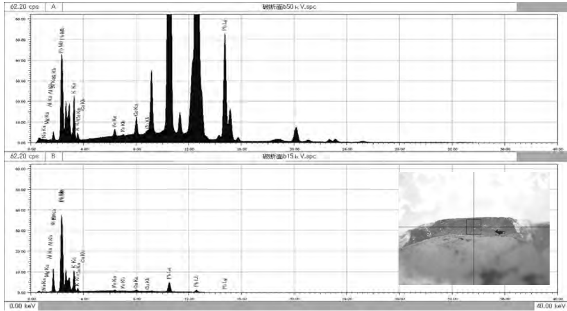
図 182 ガラス水滴欠損部bの XRF スペクトル (上段：50kV、下段：15kV)
