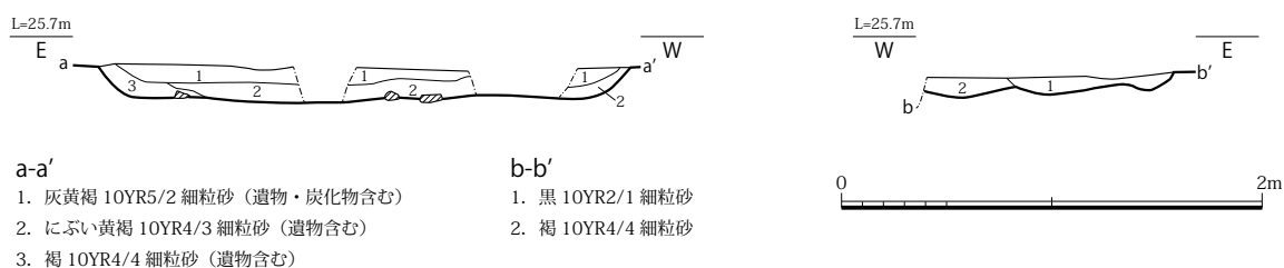
図 133 SD5150 土層断面図 (S=1/40)
