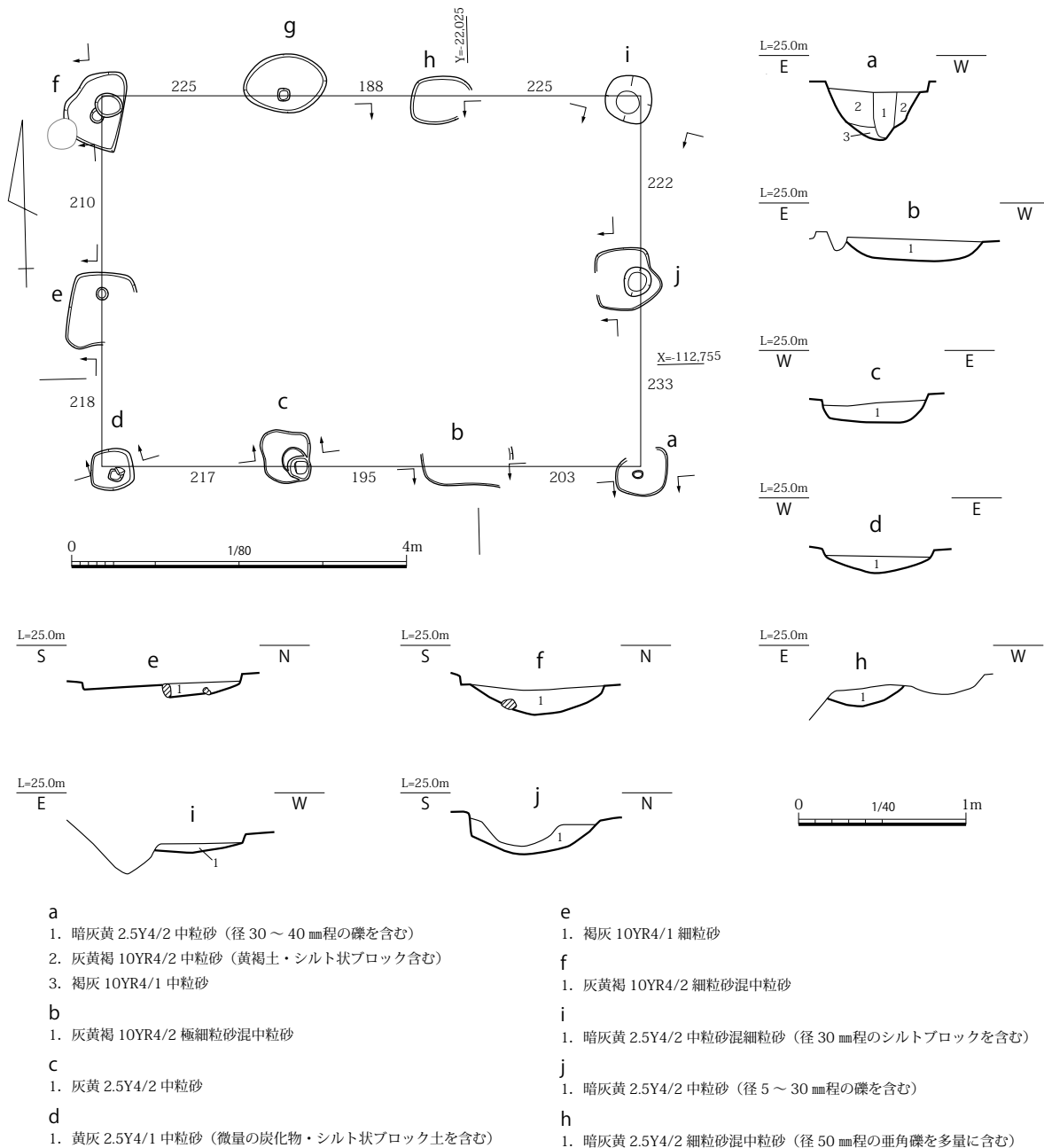
図 36 SB0970 平面・土層断面図 (平面 S=1/80・断面 S=1/40)
