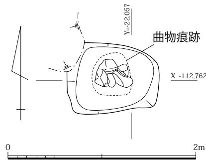
図 46 SE1600 平面図 (S=1/40)
