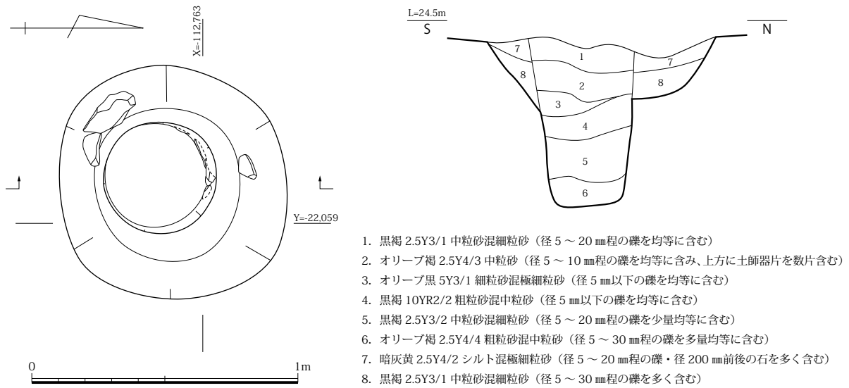
図 103 SE1370 平面・土層断面図 (S=1/40)
