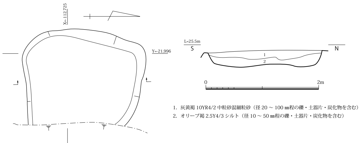
図 147 SK5560 平面・土層断面図 (S=1/40)
