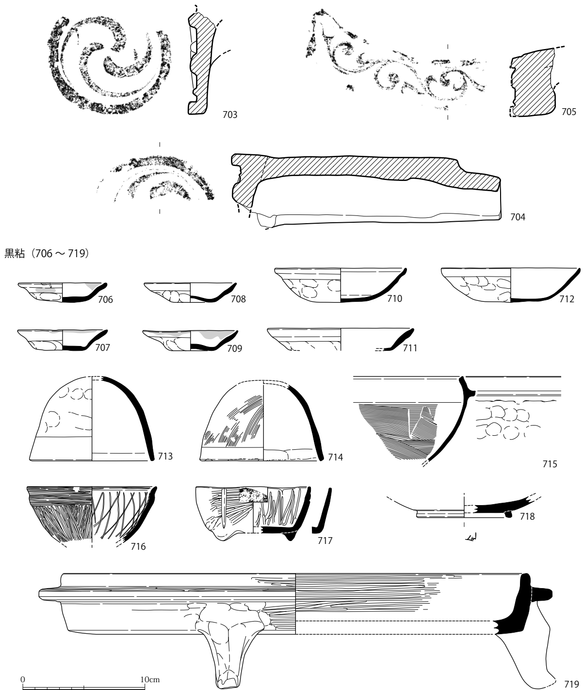
図 158 SG5030 出土遺物実測図 (2) (S=1/3)
