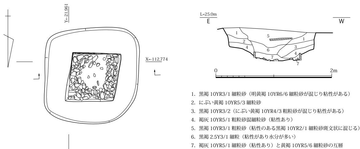
図 109 SE5080 平面・土層断面図 (S=1/40)
