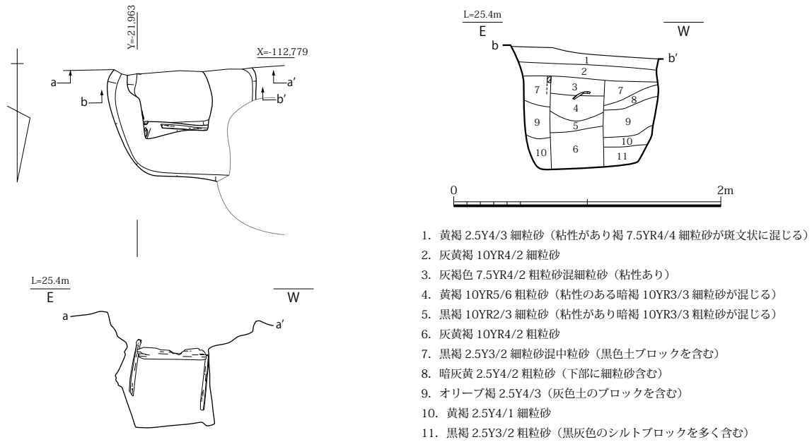
図 110 SE5100 平面・立面・土層断面図 (S=1/40)
