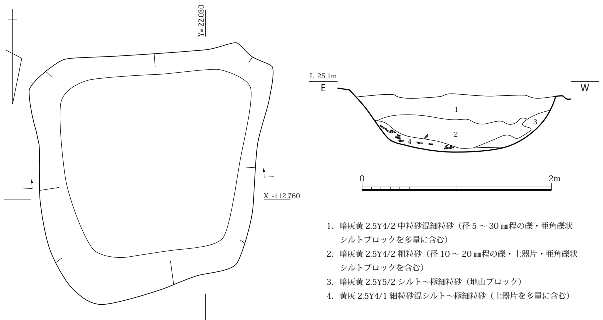
図 75 SK0640 平面・土層断面図 (S=1/40)
