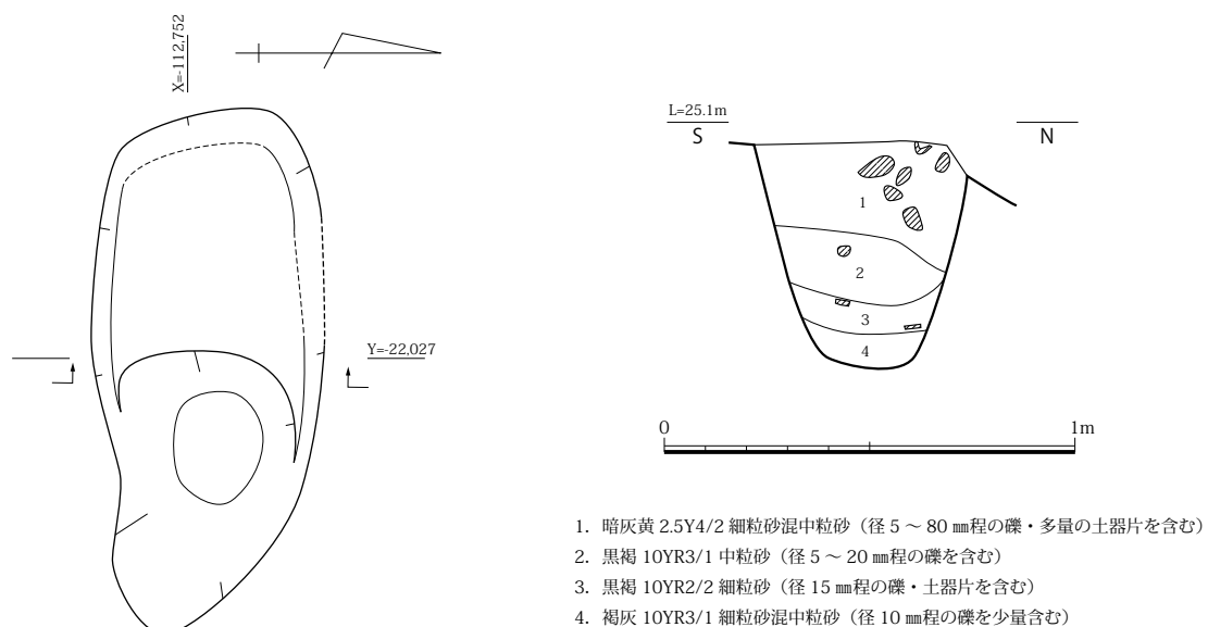
図 73 SK0460 平面・土層断面図 (S=1/20)
