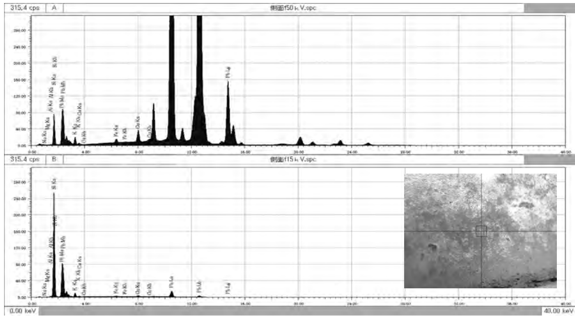
図 186 ガラス水滴表面 f の XRF スペクトル (上段：50kV、下段：15kV)
