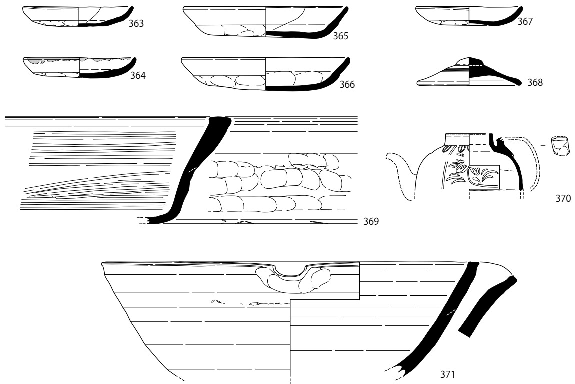
図 90 SK0380・0460 出土遺物実測図 (S=1/3・1/6)
