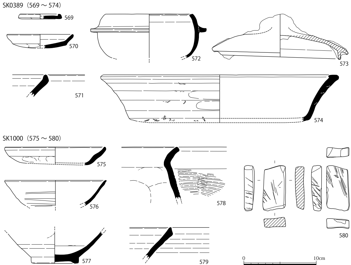
図 131 SK0389・1000 出土遺物実測図 (S=1/3)
