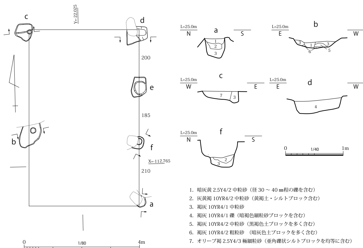
図 37 SB0980 平面・土層断面図 (平面 S=1/80・断面 S=1/40)
