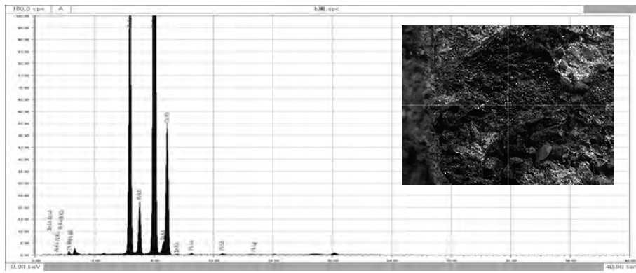
図 172 分析箇所 b の蛍光 X 線分析スペクトル
