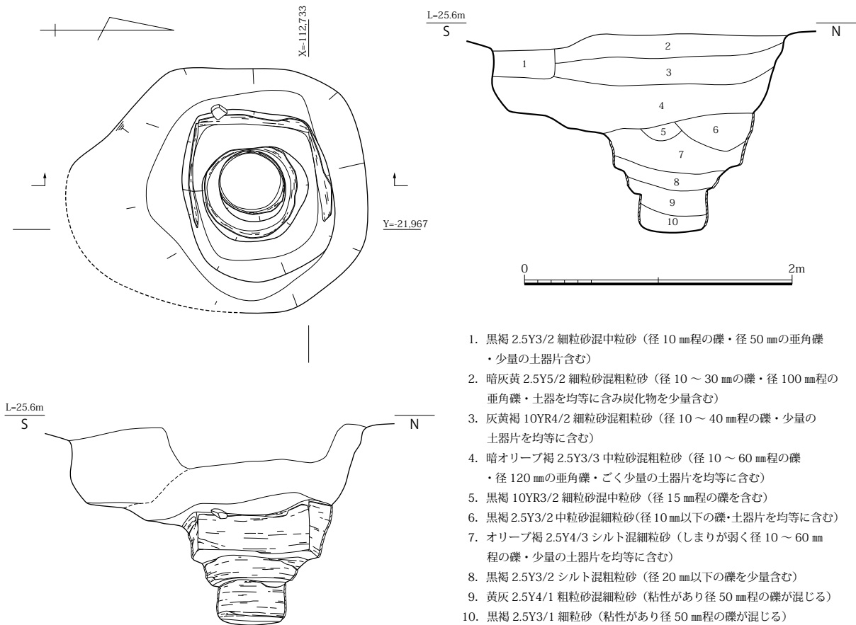
図 114 SE5280 平面・立面・土層断面図 (S=1/40)
