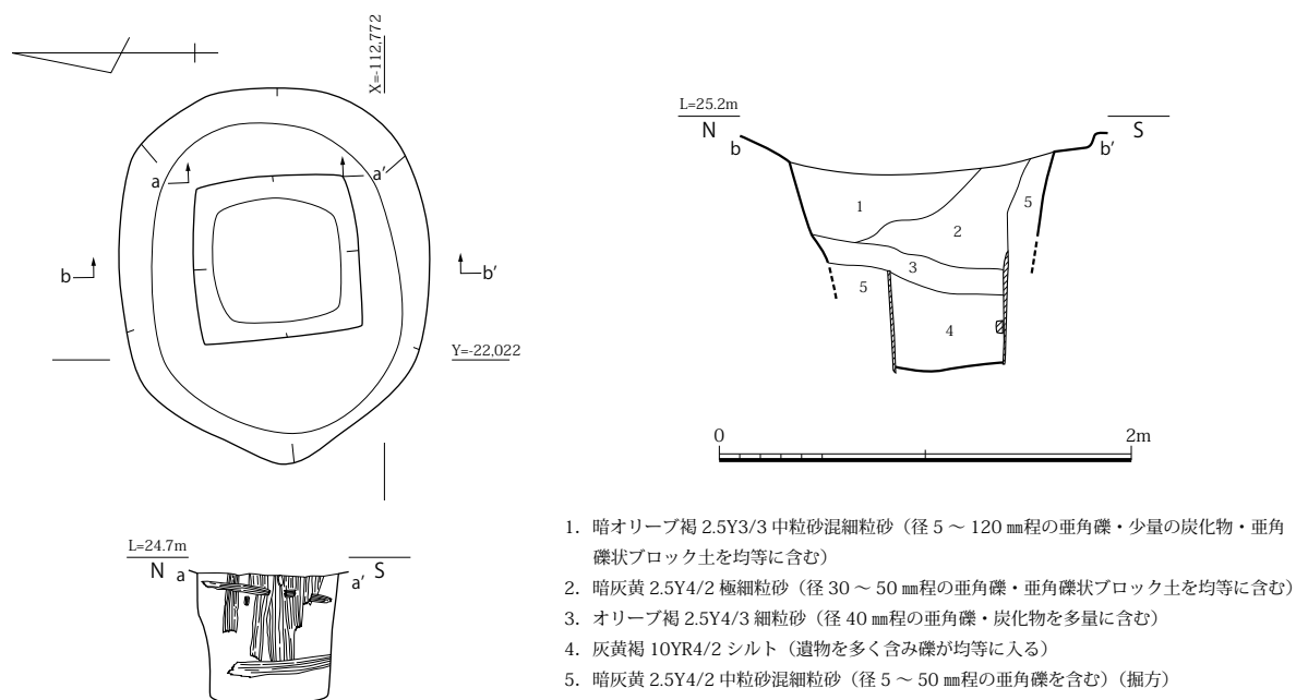
図 59 SE0590 平面・立面・土層断面図 (S=1/40)
