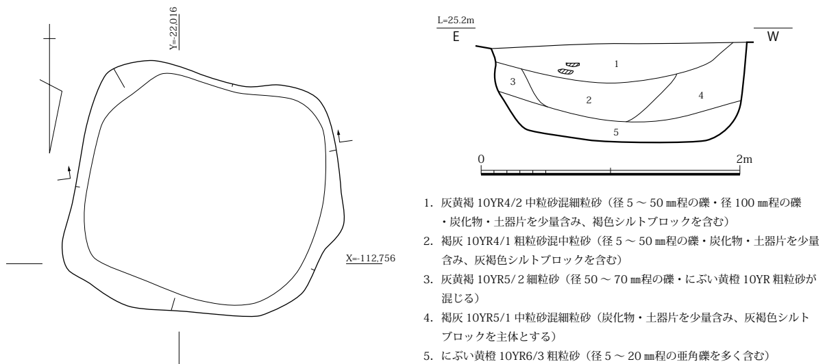
図 57 SE0370 平面・土層断面図 (S=1/40)
