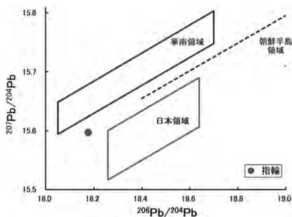
図 179 整地土 2 出土指輪の鉛同位体比 (B 式図)
