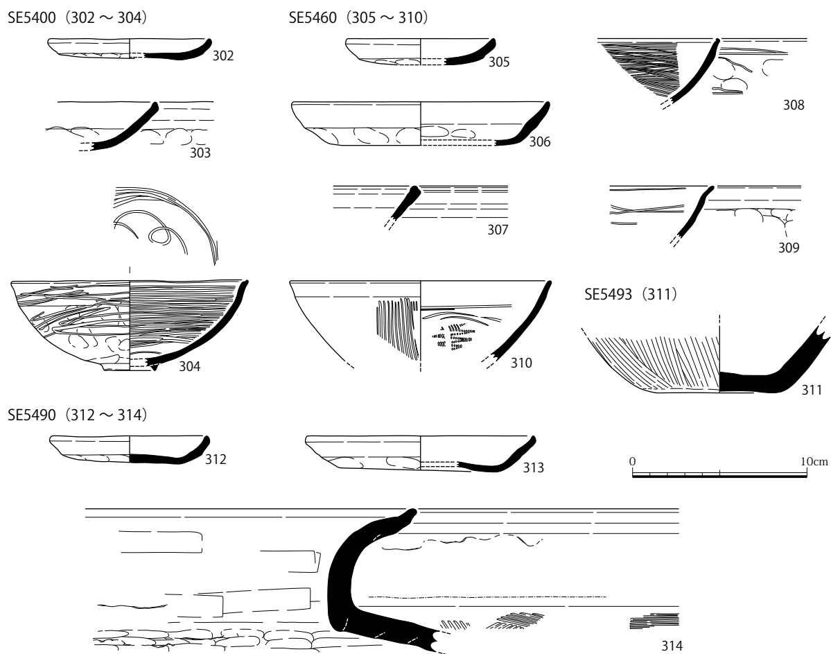
図 86 SE5400・5460・5490・5493 出土遺物実測図 (S=1/3)
