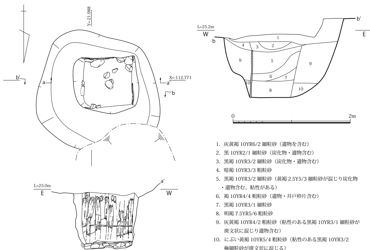
図 112 SE5200 平面・立面・土層断面図 (S=1/40)
