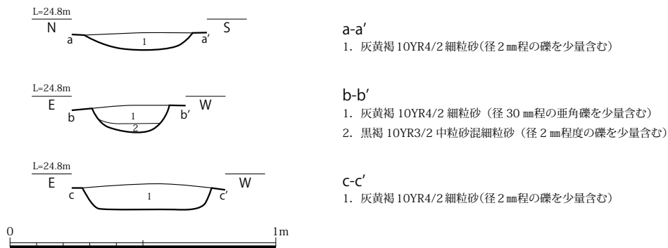
図 44 SD0890 土層断面図 (S=1/20)
