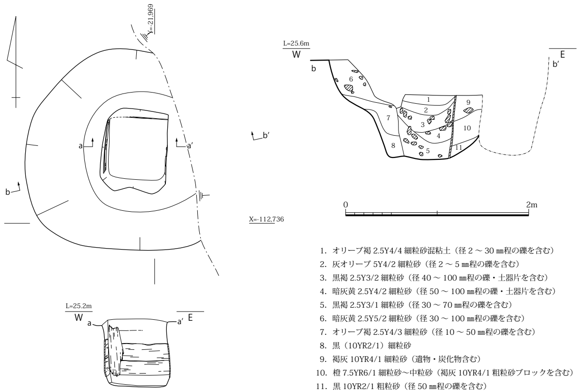
図 113 SE5270 平面・立面・土層断面図 (S=1/40)
