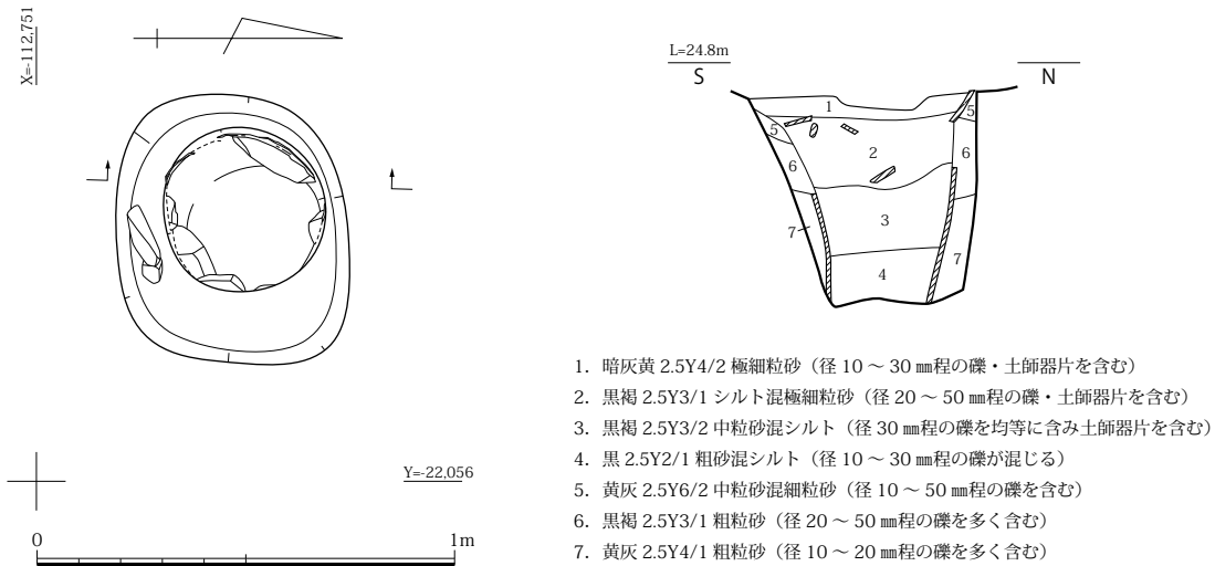
図 102 SE1350 平面・土層断面図 (S=1/20)
