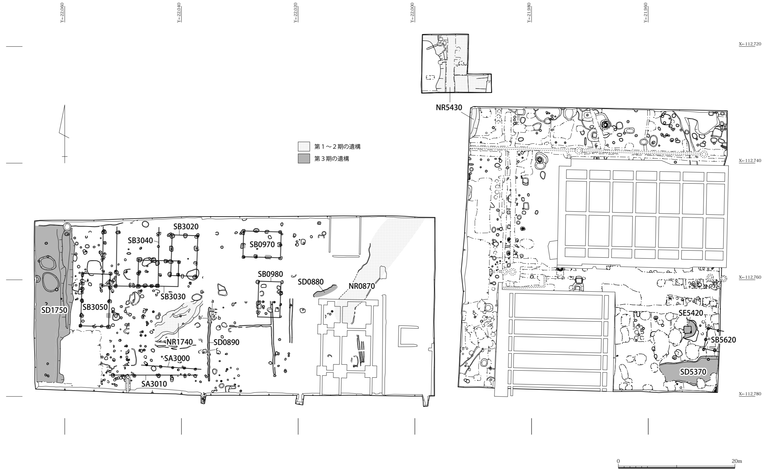
図9 第3・4遺構面遺構配置図 (S=1/400) ※西区西半の遺構は第3遺構面相当
