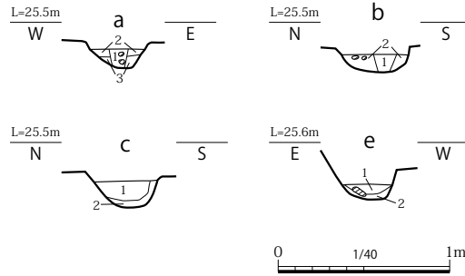
図 26 SD5578 土層断面図 (S=1/40)
