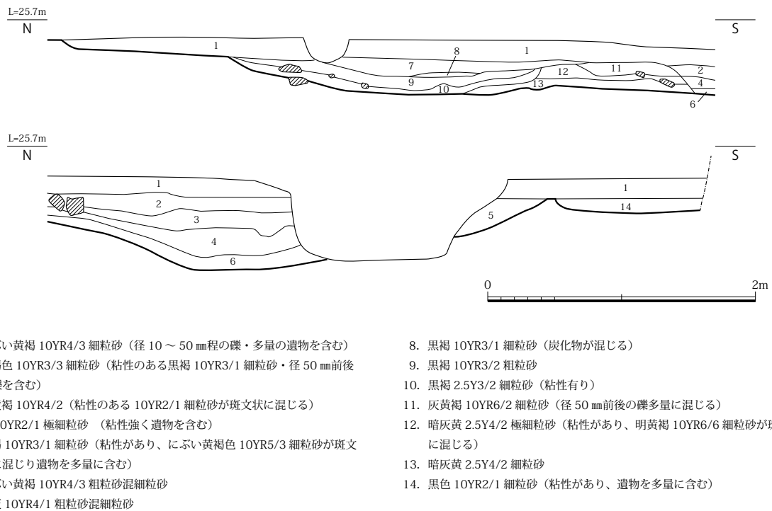
図 143 SG5030 土層断面図 (S=1/40)
