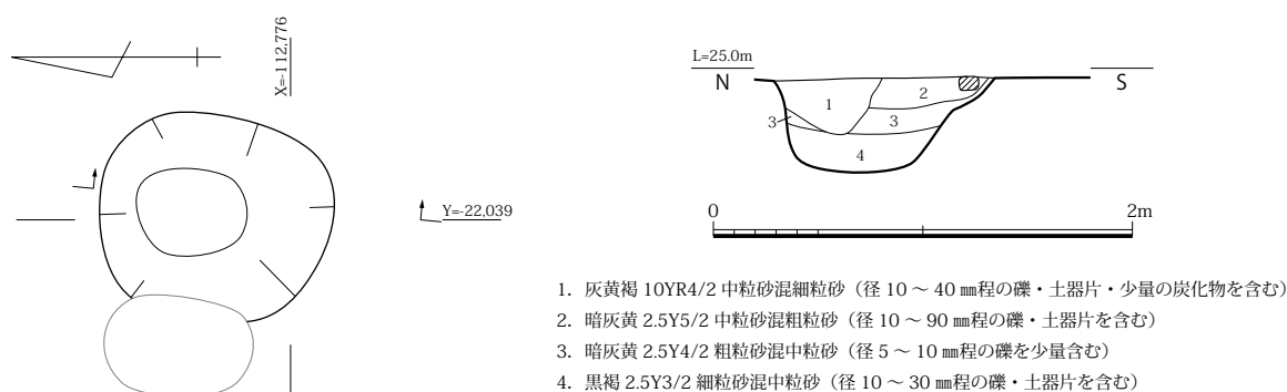
図 118 SK1000 平面・土層断面図 (S=1/40)
