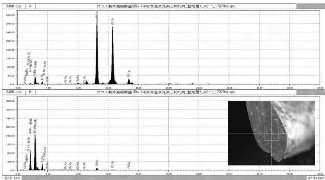
図 181 ガラス水滴破断接合面 a の XRF スペクトル (上段: 50kV、下段: 15kV)
