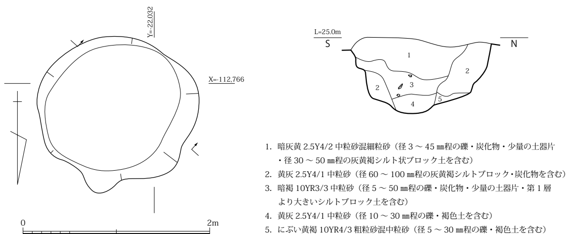
図 58 SE0570 平面・土層断面図 (S=1/40)
