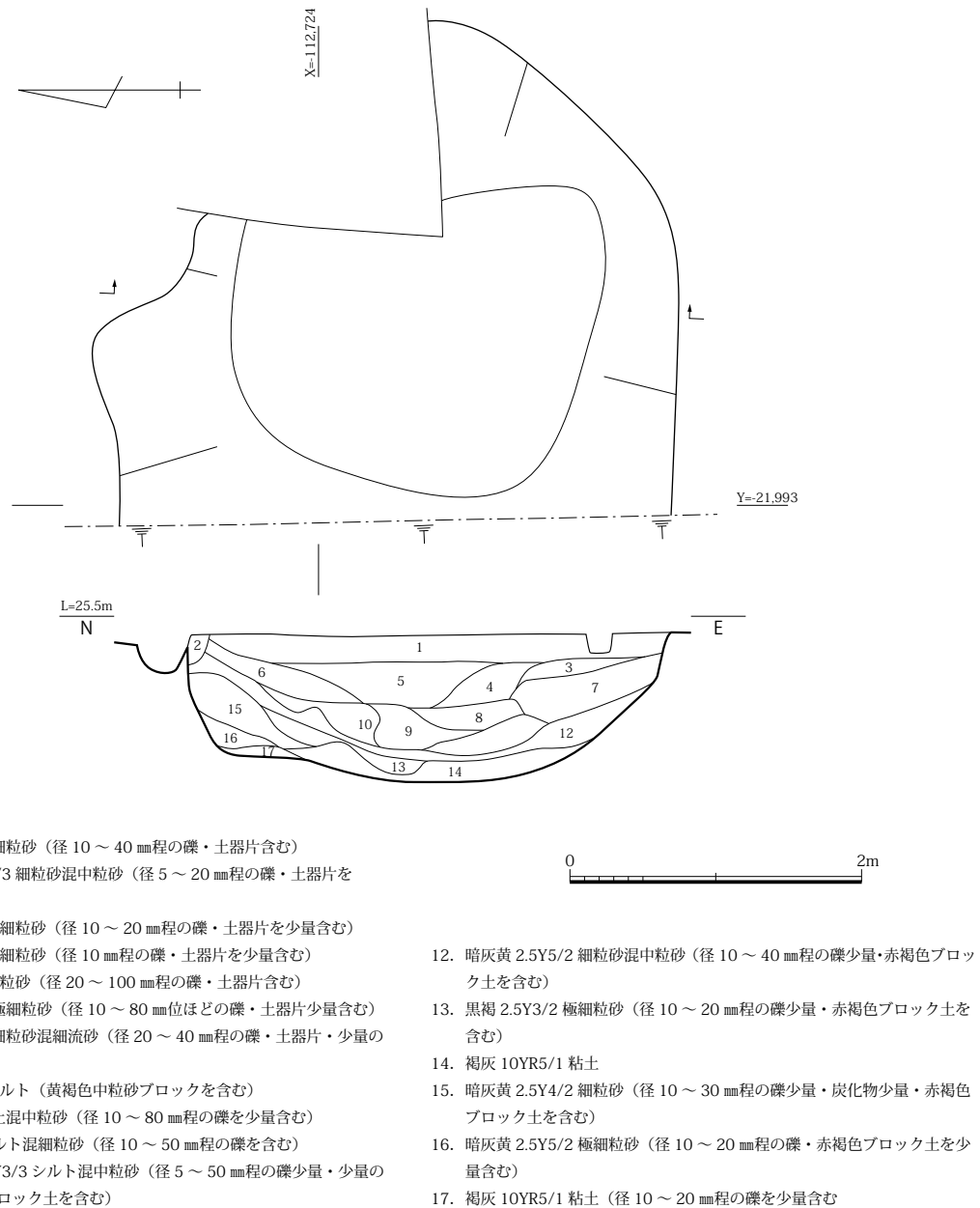
図 148 SK5570 平面・土層断面図 (S=1/50)
