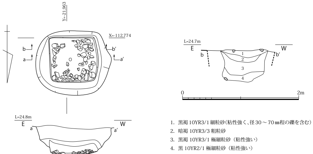
図 139 SE5070 平面・立面・土層断面図 (S=1/40)
