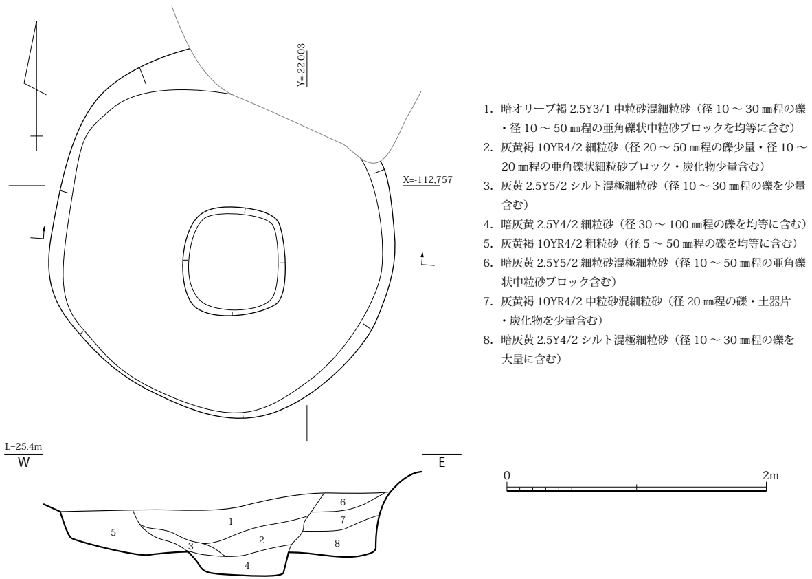
図 60 SE0730 平面・土層断面図 (S=1/40)
