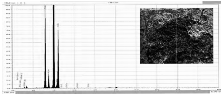
図 173 分析箇所 c の蛍光 X 線分析スペクトル
