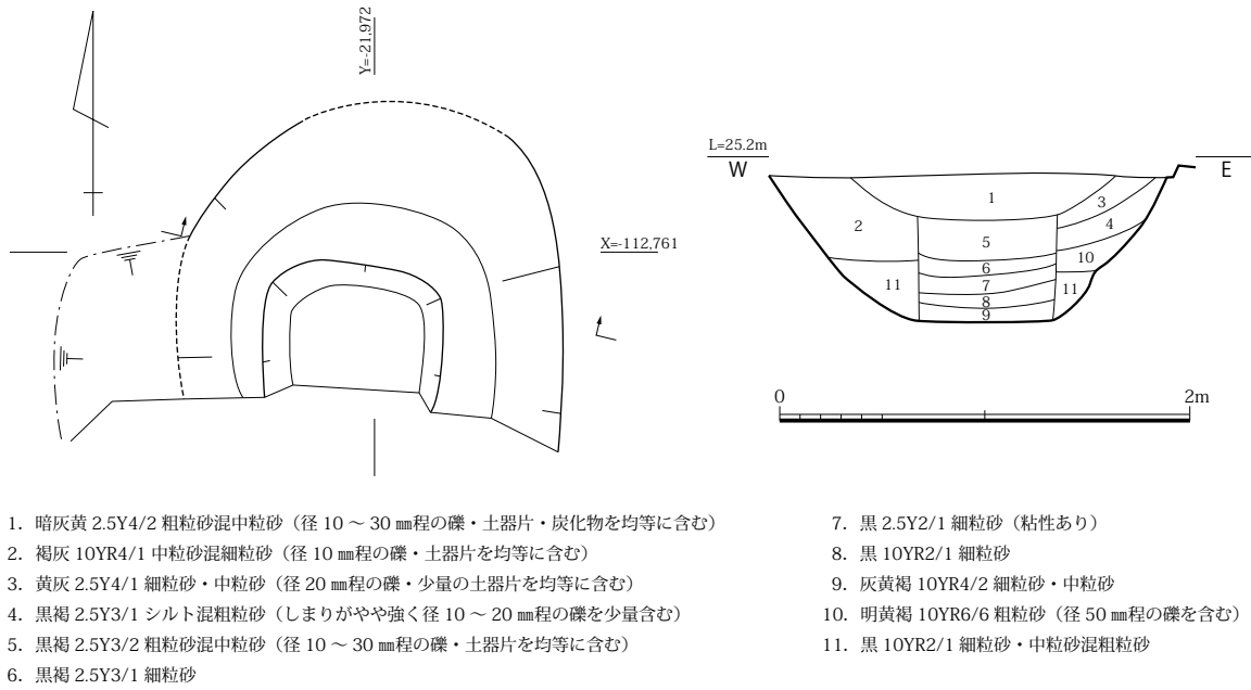
図 68 SE5490 平面・土層断面図 (S=1/40)
