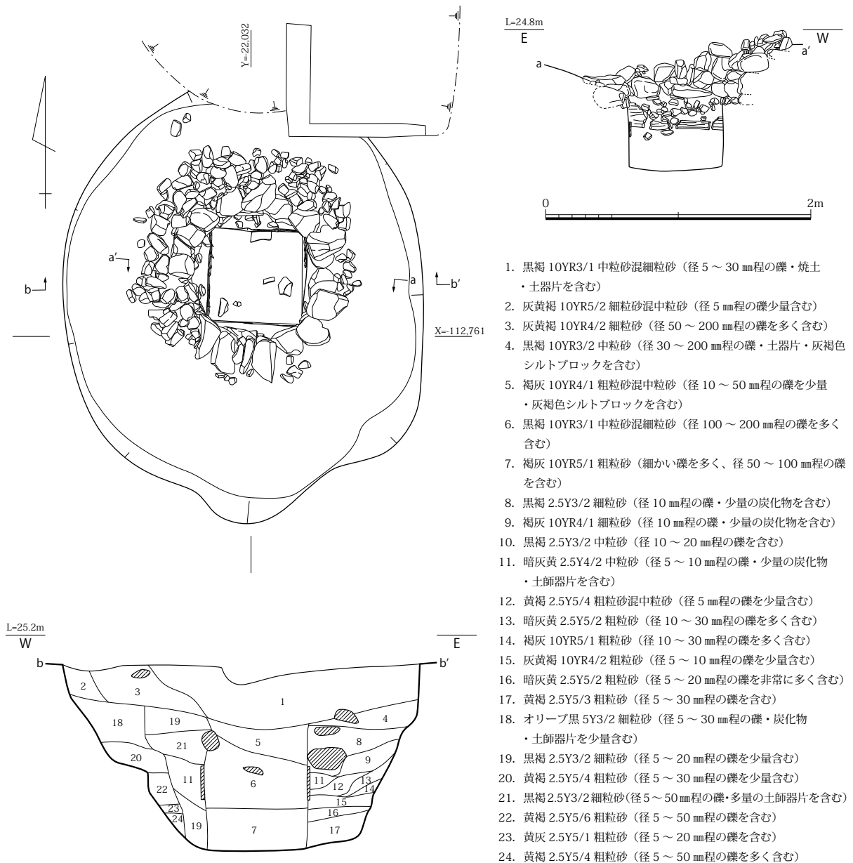
図 135 SE0110 平面・立面・土層断面図 (S=1/40)
