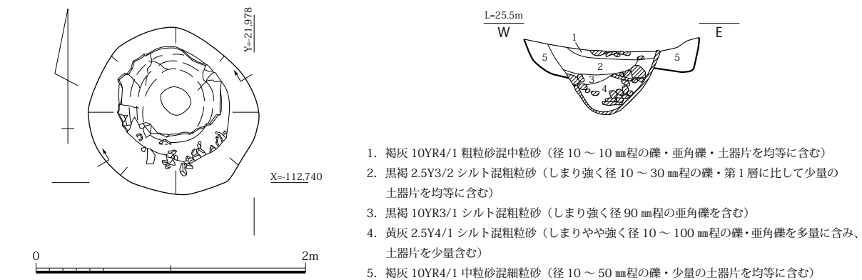
図 142 SE5320 平面・土層断面図 (S=1/40)
