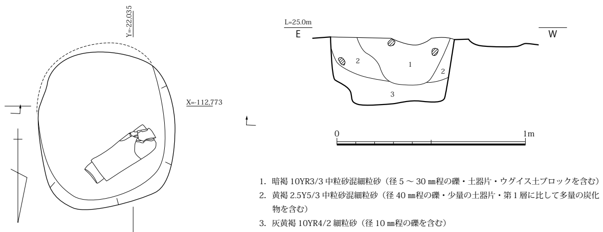
図 72 SK0450 平面・土層断面図 (S=1/20)
