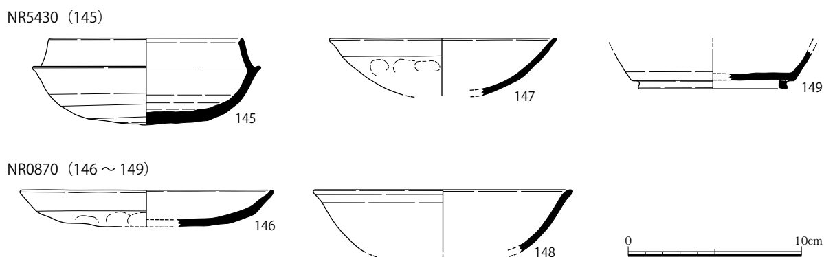
図 25 NR0870・5430 出土遺物実測図 (S=1/3)
