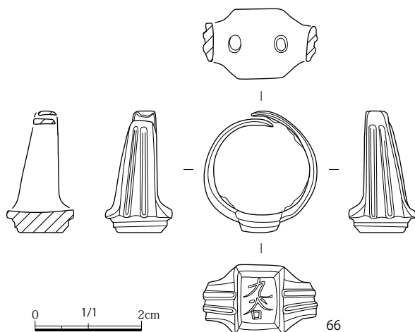
図203 整地土2出土指輪実測図 (S=1/1)
