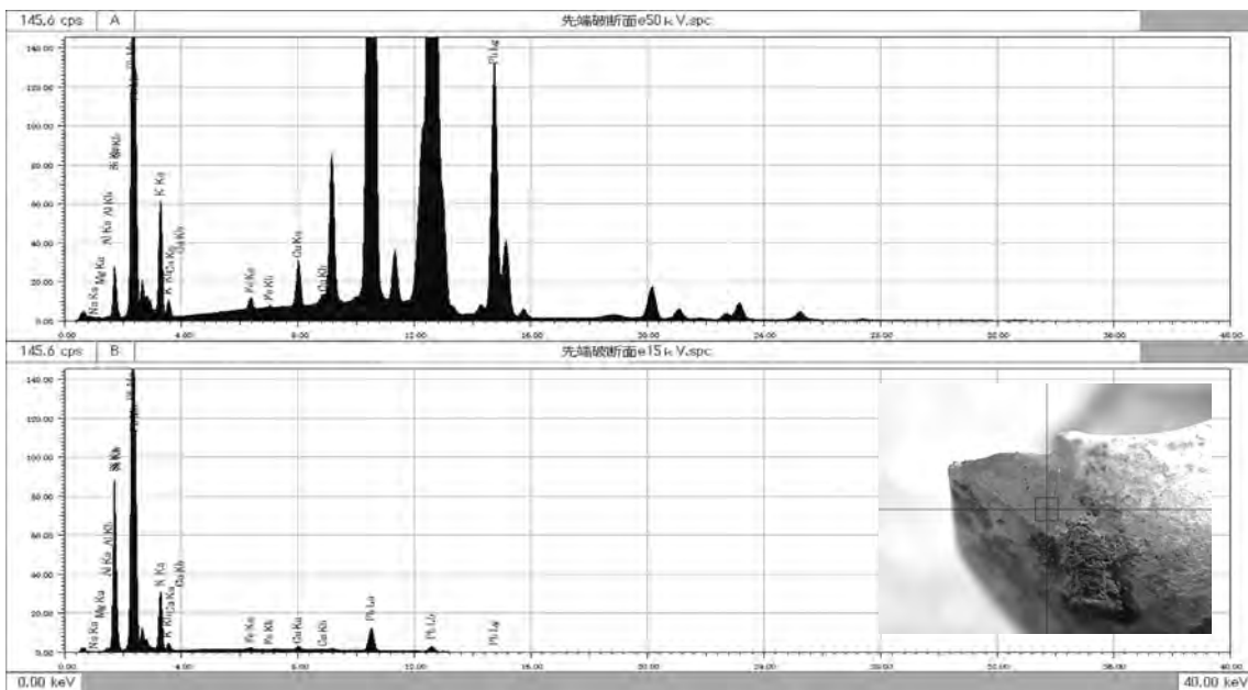
図 185 ガラス水滴欠損部 e の XRF スペクトル (上段 : 50kV、下段 : 15kV)
