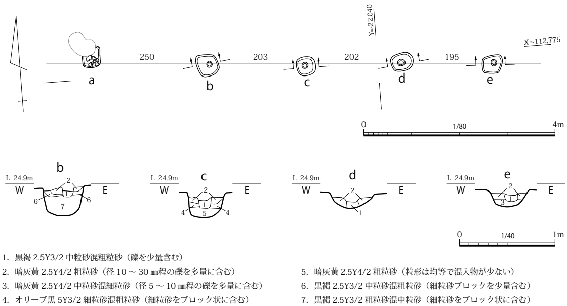
図 33 SA3000 平面・土層断面図 (平面 S=1/80・断面 S=1/40)
