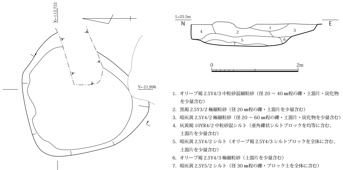
図 146 SK5550 平面・土層断面図 (S=1/50)
