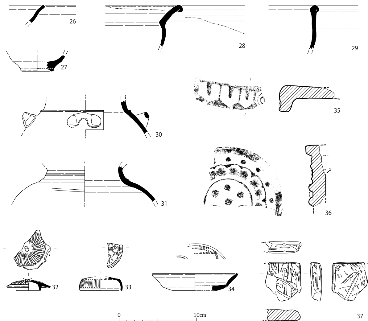
図 20 整地土 1 出土遺物実測図 (2) (S=1/3)
