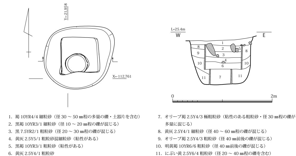
図 67 SE5460 平面・土層断面図 (S=1/40)
