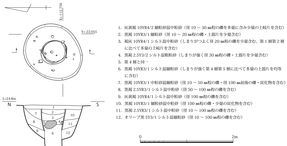
図 104 SE1380 平面・土層断面図 (S=1/40)
