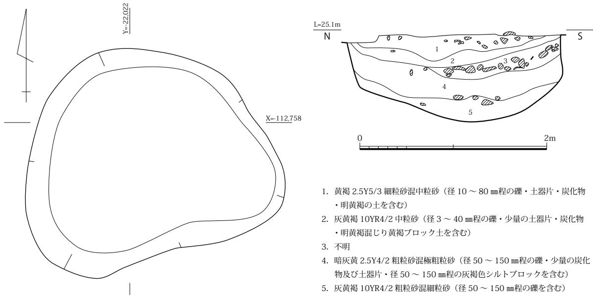
図 74 SK0490 平面・土層断面図 (S=1/40)
