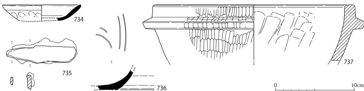
図 160 SK1090・2118・2717・5560 出土遺物実測図 (S=1/3)
