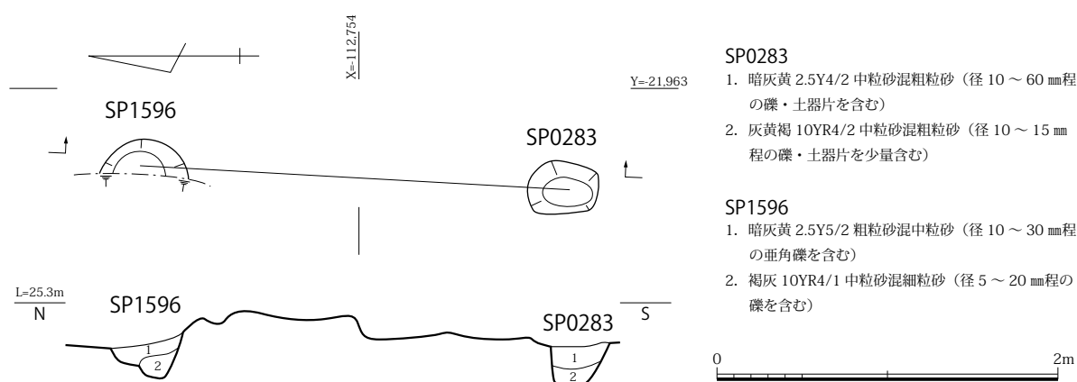
図 119 SP0283・1596 平面・土層断面図 (S=1/40)
