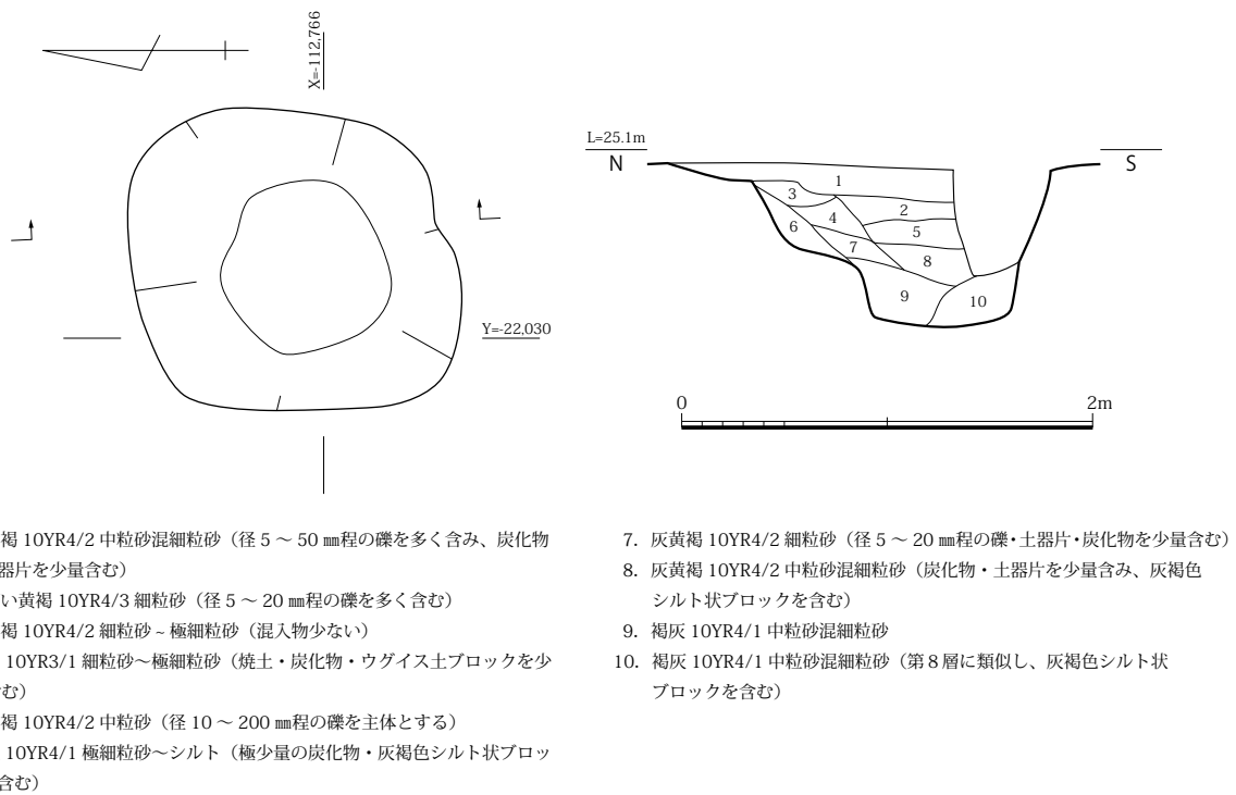
図 117 SK0389 平面・土層断面図 (S=1/40)
