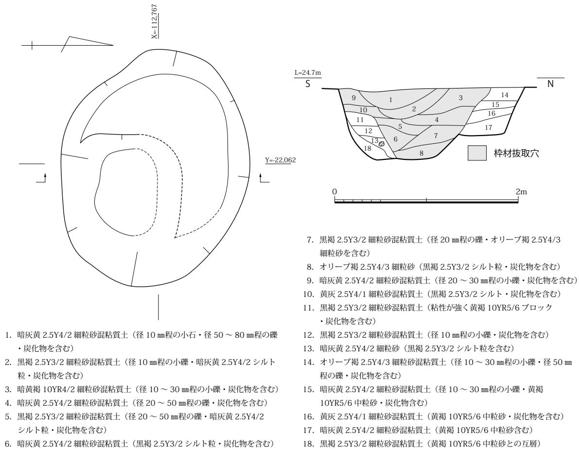
図 107 SE1490 平面・土層断面図 (S=1/40)
