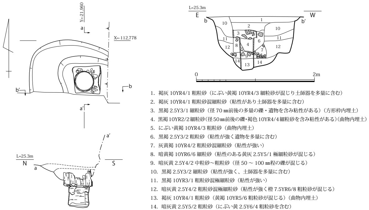
図 111 SE5110 平面・立面・土層断面図 (S=1/40)
