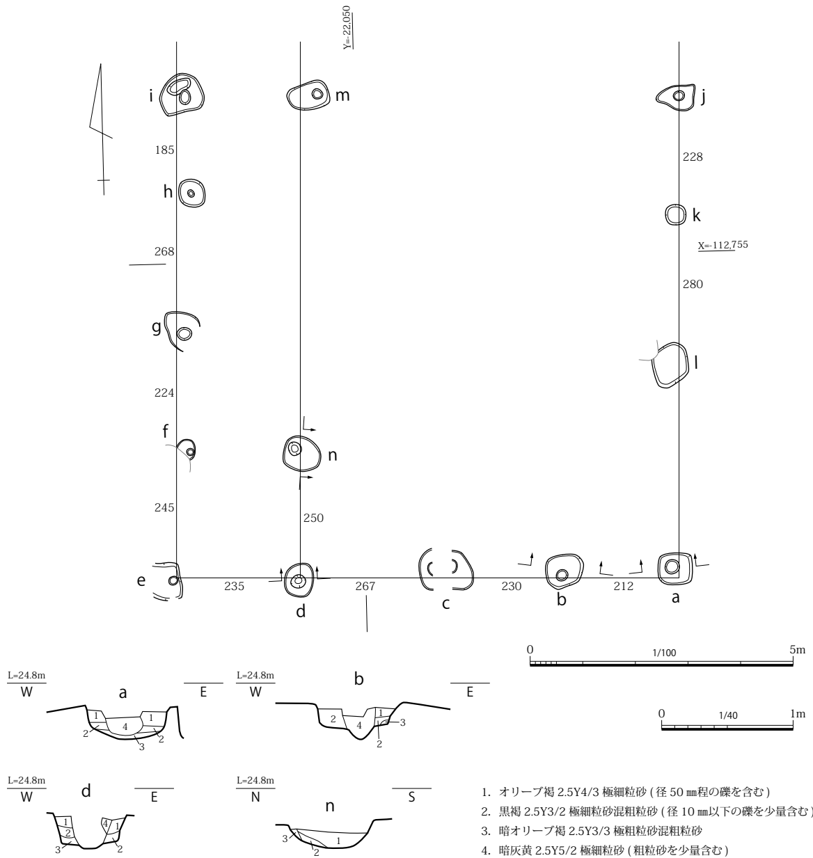
図 40 SB3040 平面・土層断面図 (平面 S=1/100・断面 S=1/40)
