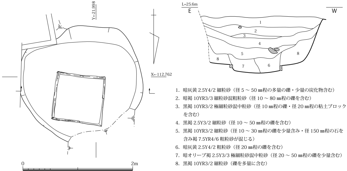
図 61 SE0790 平面・土層断面図 (S=1/40)
