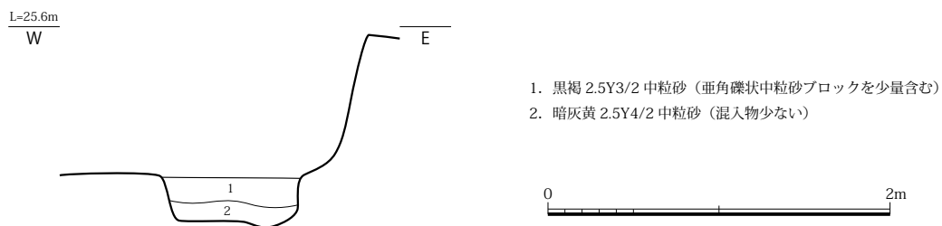
図 65 SE5290 土層断面図 (S=1/40)
