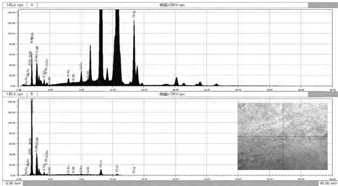
図 183 ガラス水滴表面cの XRF スペクトル (上段：50kV、下段：15kV)
