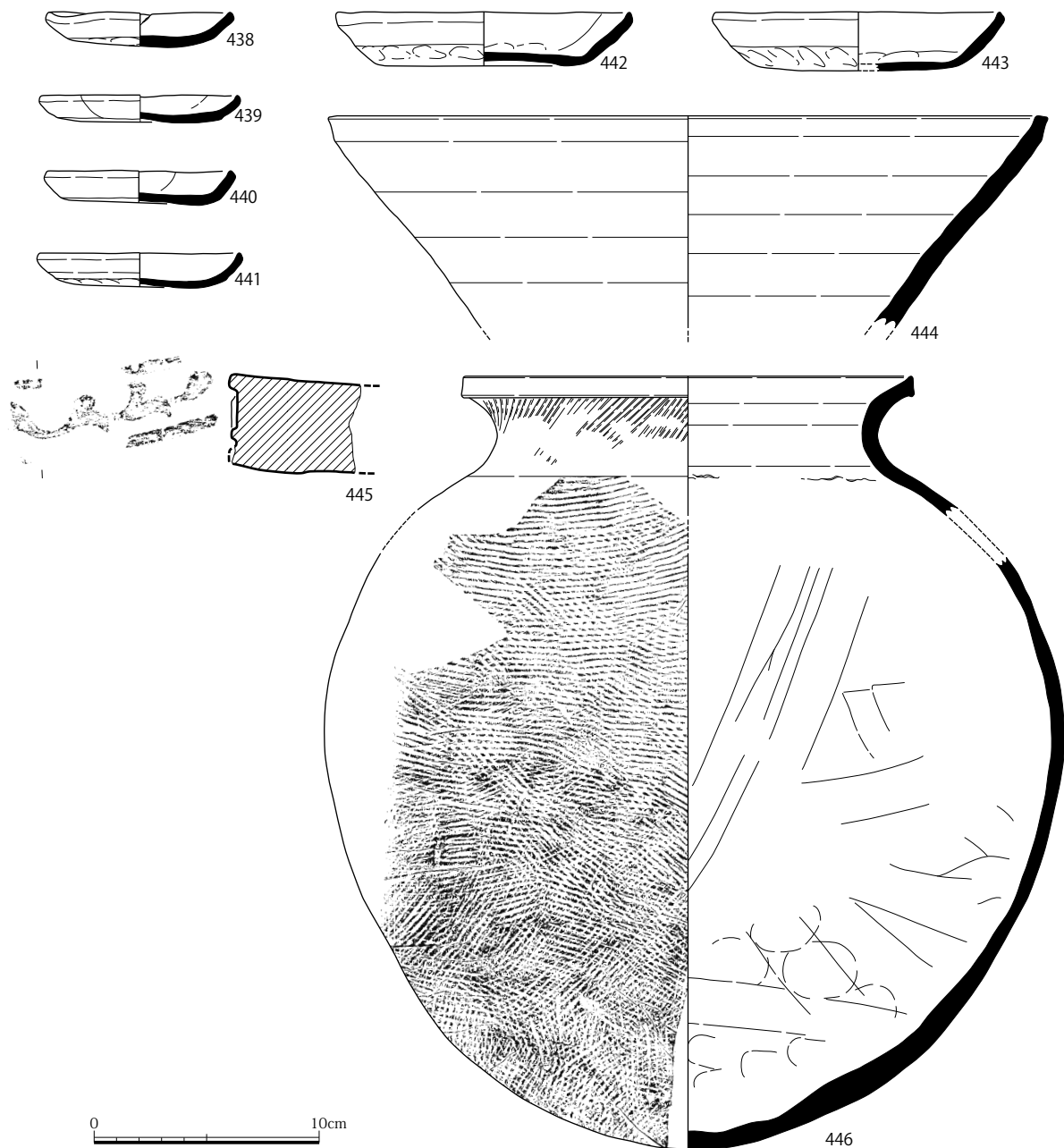
図 121 SE0140 出土遺物実測図 (S=1/3)
