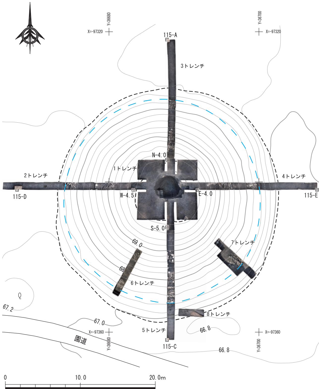
第2図 西都原115号墳調査区配置図(1:250)
