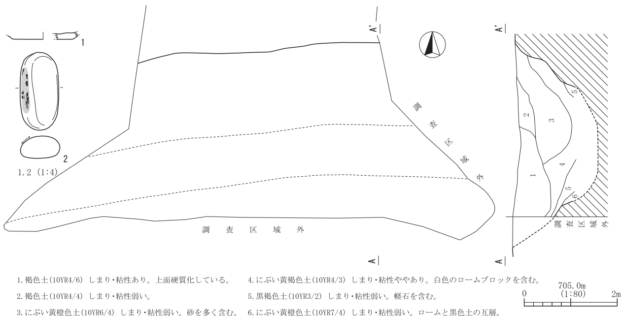
第20図 M1号溝状遺構及び出土遺物実測図
