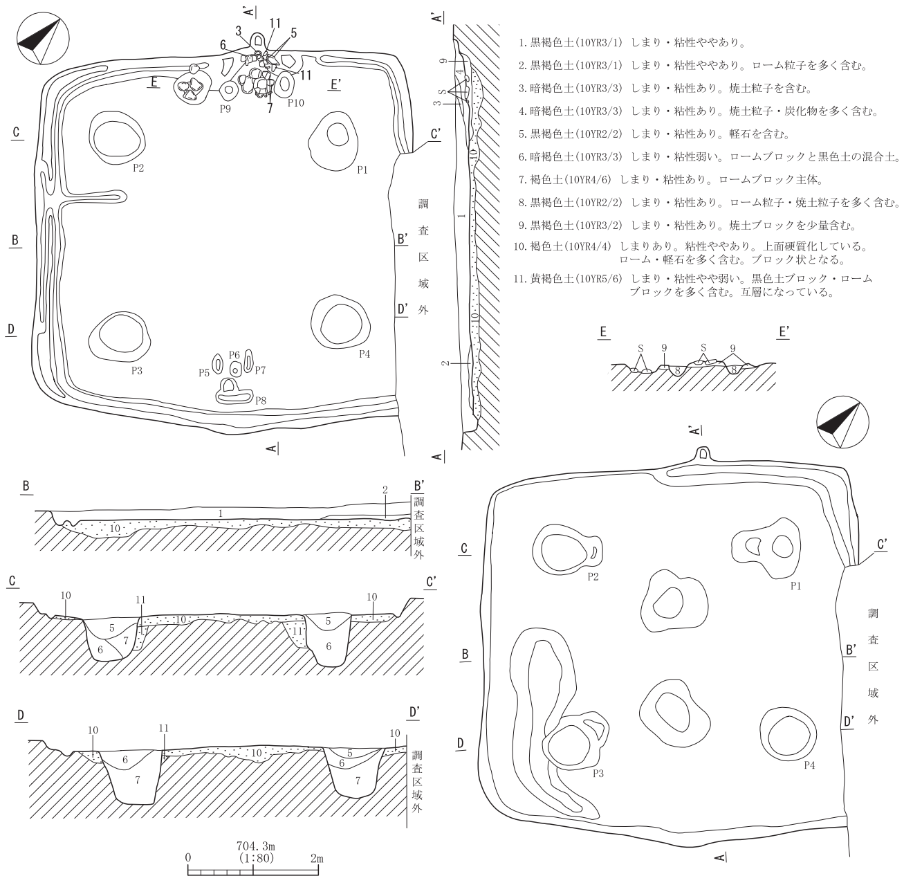
第13図 H5号住居址実測図
