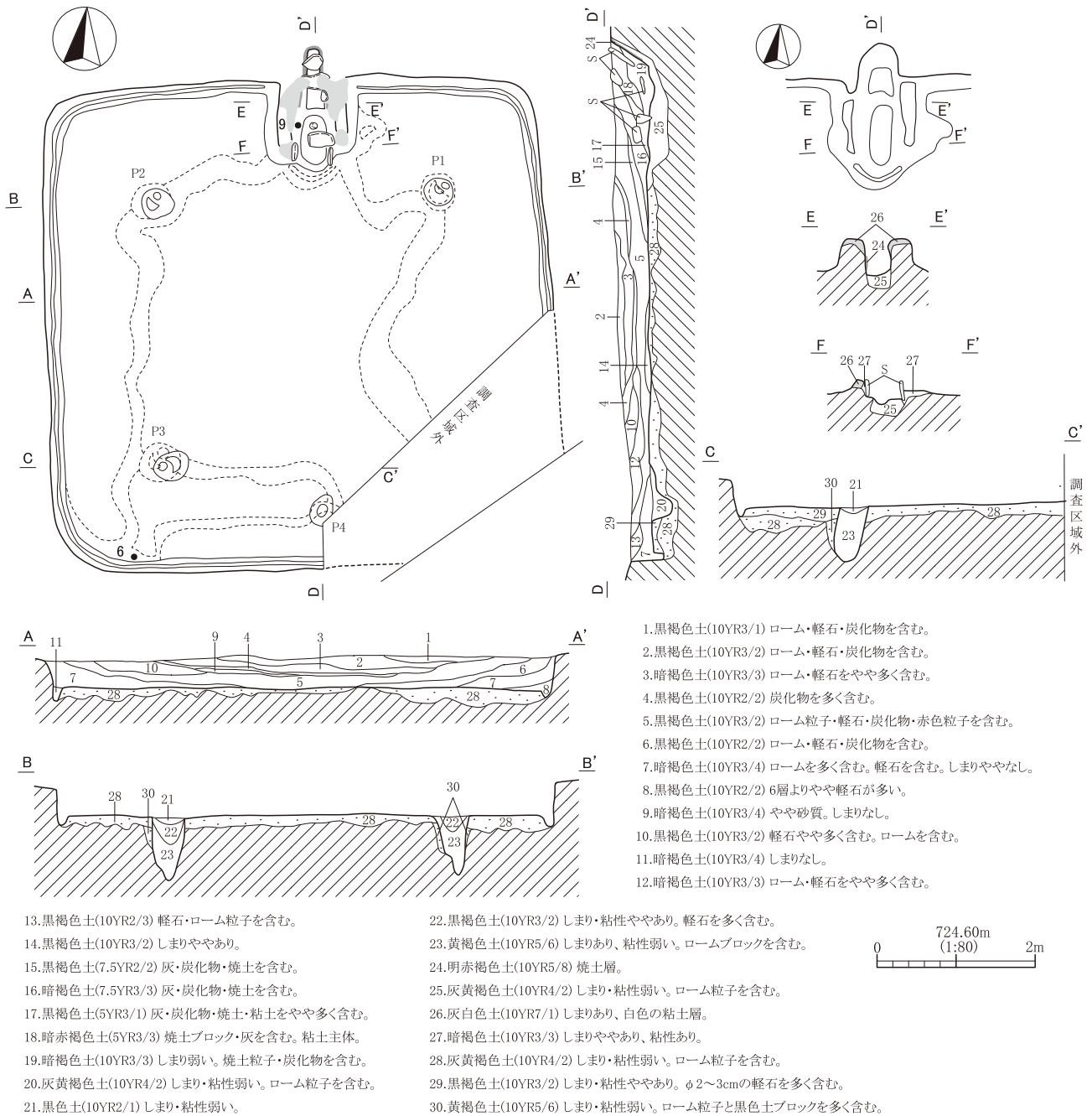
第4図 H1号住居址実測図
