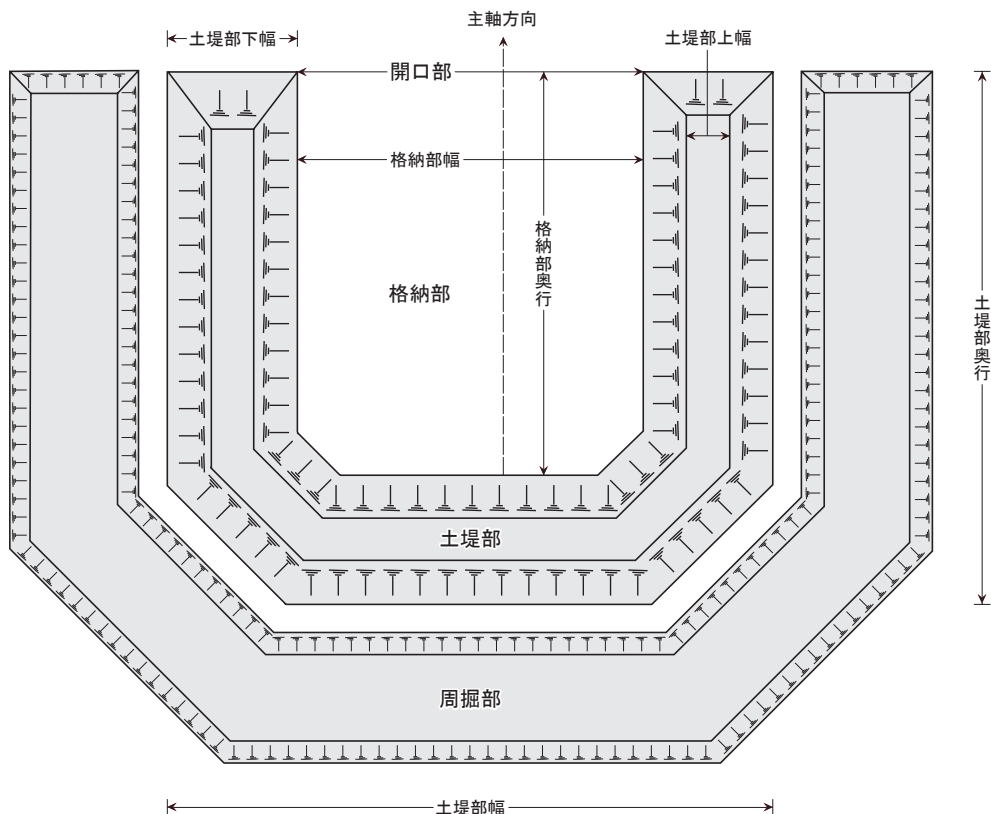
第5図 C字型 無蓋掩体壕の模式図
