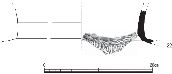
图8 C区溝38・集石遺構39出土遺物実測図(1/4)
