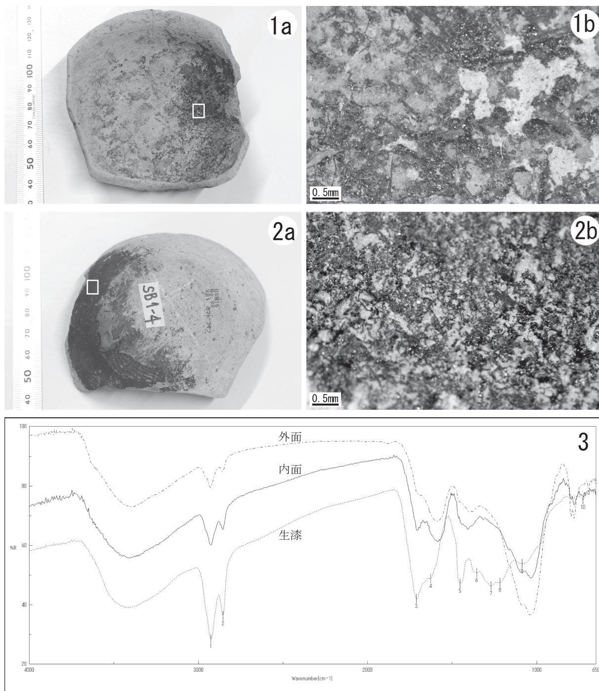
1a 内面付着物(□は1b) 1b 内面付着物の拡大写真と採取位置 2a 外面付着物(□は2b) 2b 外面付着物の拡大写真と採取位置 3 付着物の赤外分光スペクトル図 実線:内面付着物、一点鎖線:外面付着物、点線:生漆、数字:生漆の赤外吸収位置
