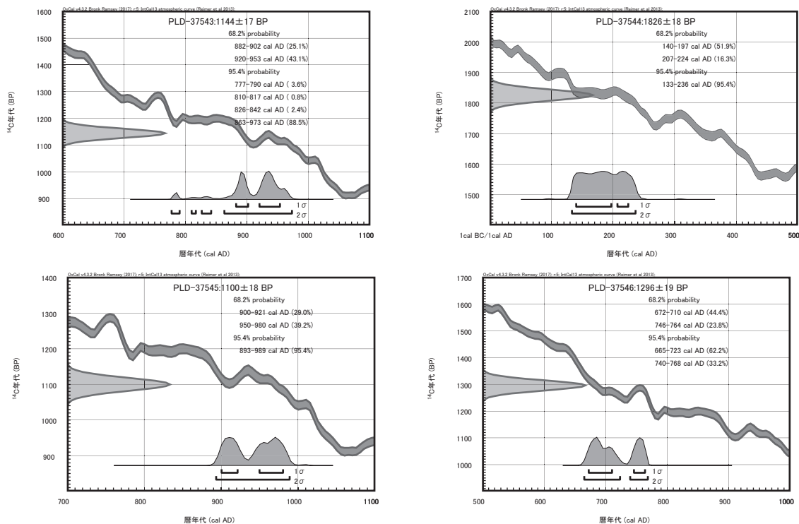
第29図 暦年較正結果
