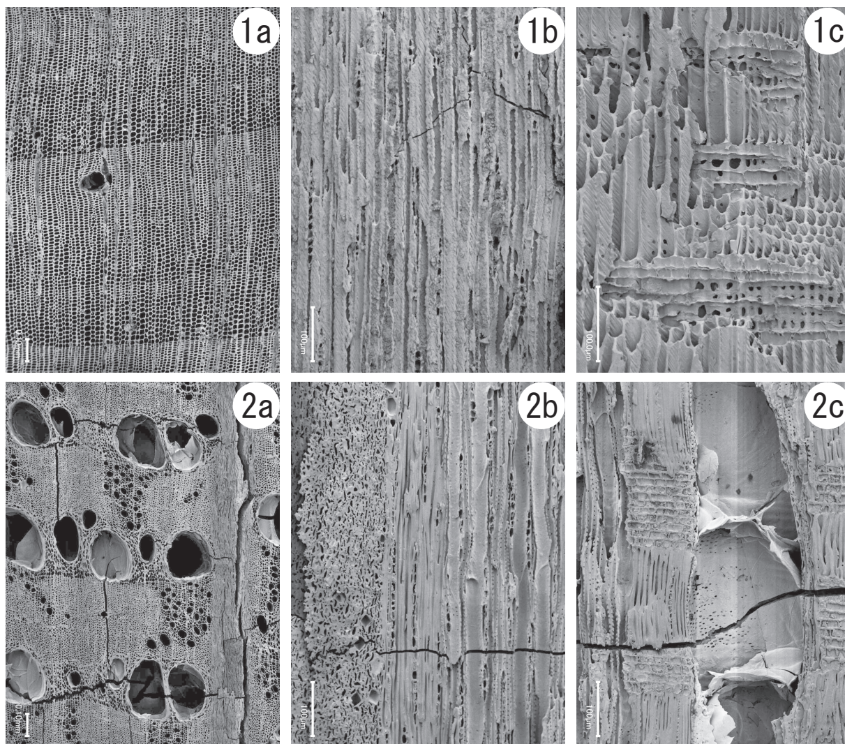
1a-1c. マツ属複維管束亜属(No.4)、2a-2c. コナラ属コナラ節(No.1) a:横断面、b:接線断面、c:放射断面
