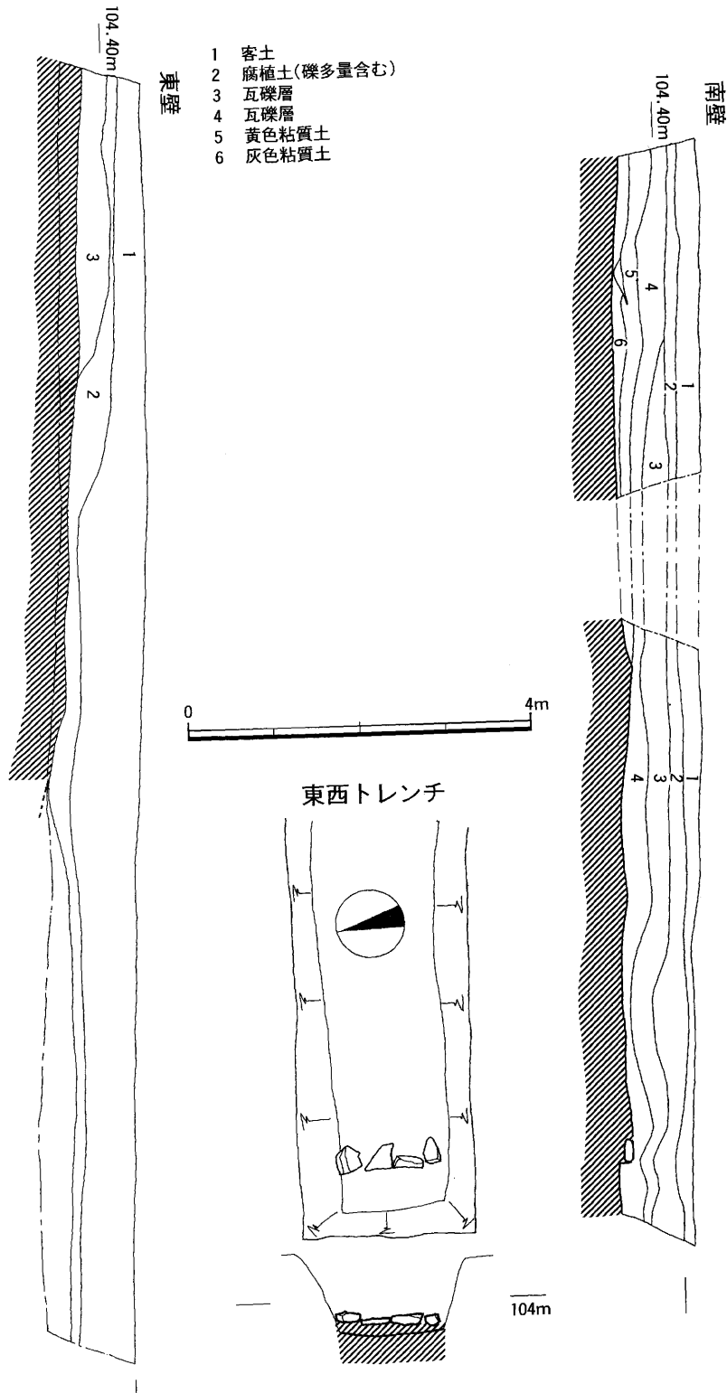
挿図7 Aトレンチ平面及び断面図
