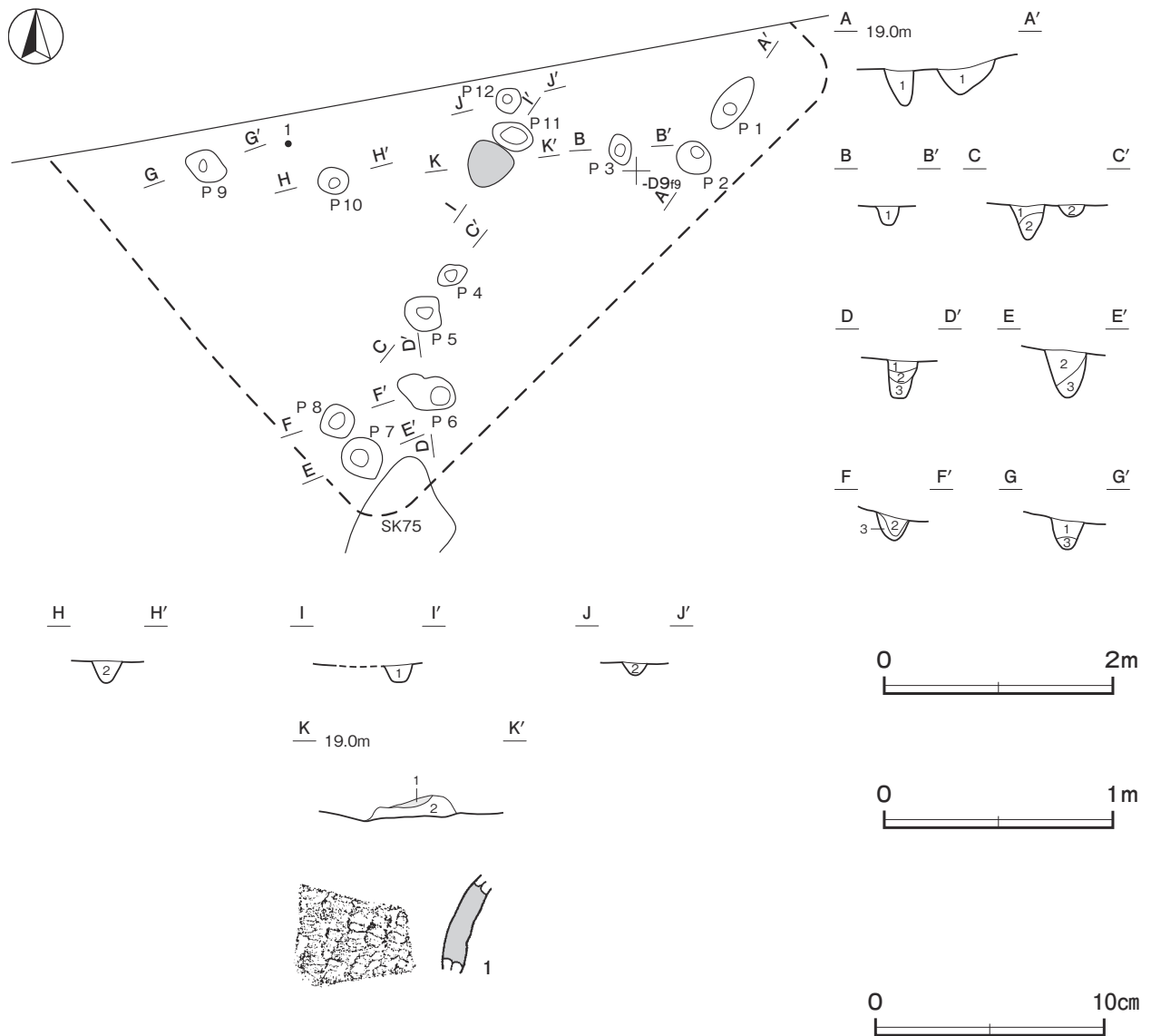
第 362 図 第 36 号 縦穴建物跡・出土遺物実測図
