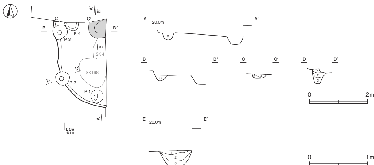
第 194 図 第 46 号竪穴建物跡実測図
