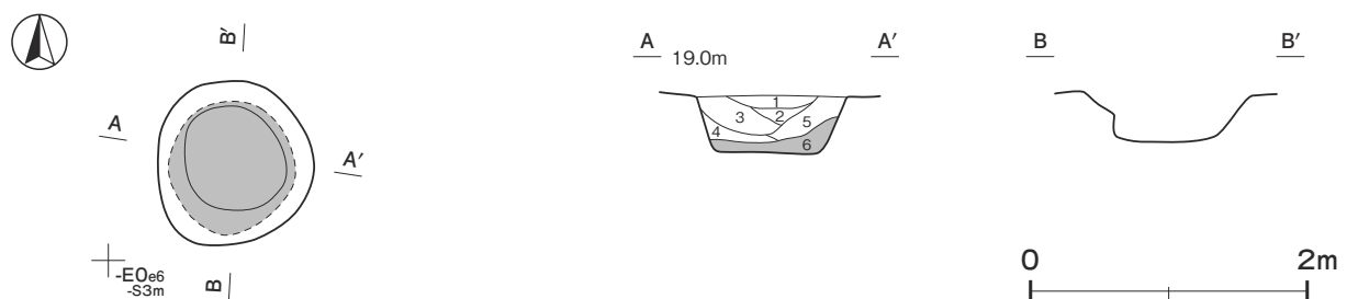
第 417 図 第 1 号粘土貼土坑実測図
