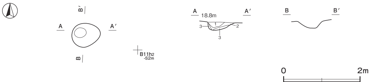
第 424 図 第 129 号土坑実測図
