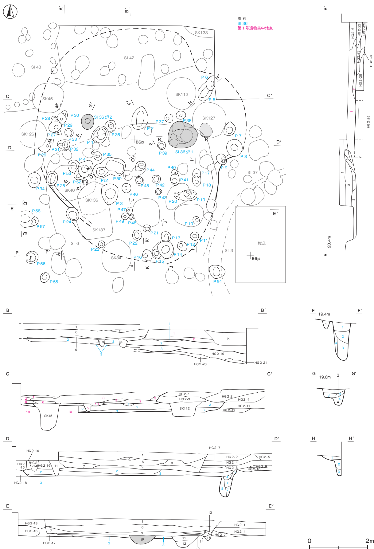
第43図 第6・36号竪穴建物跡，第1号遺物集中地点実測図(2)
