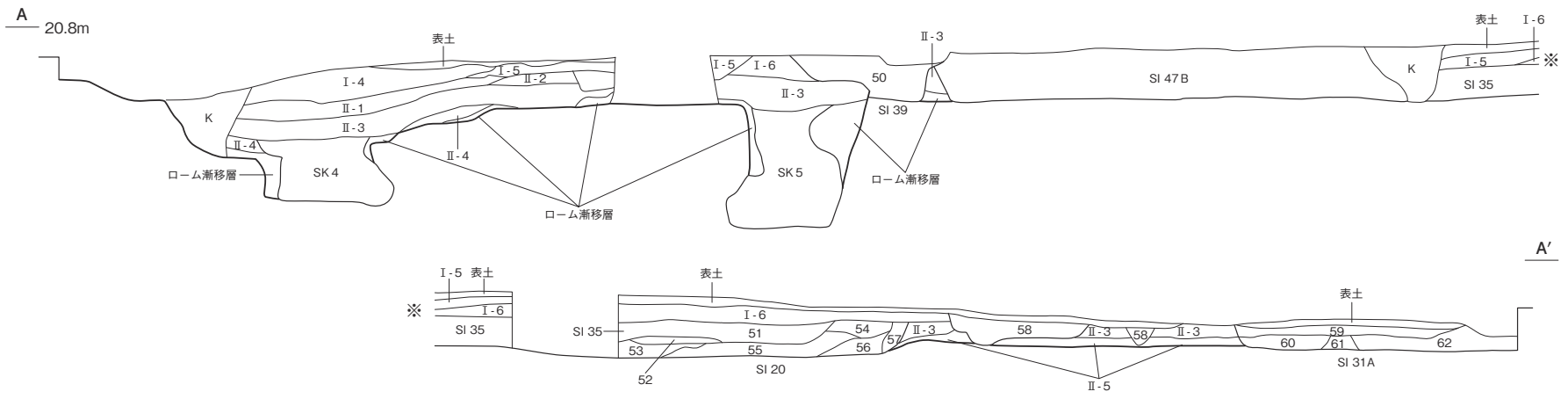
第 265 図 第 2 号遺物包含層実測図 (1)
