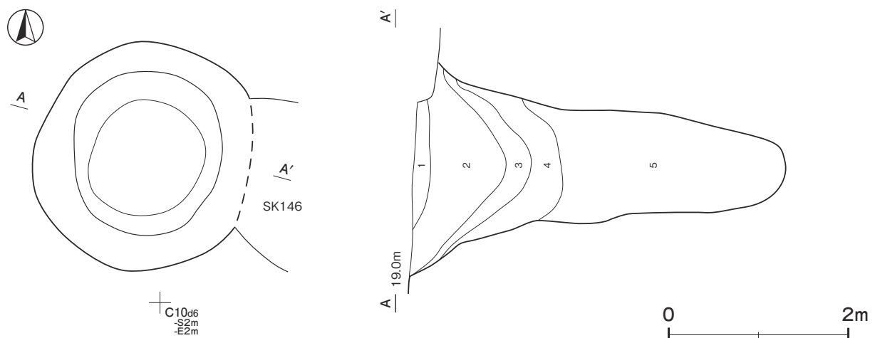
第421図 第8号井戸跡実測図
