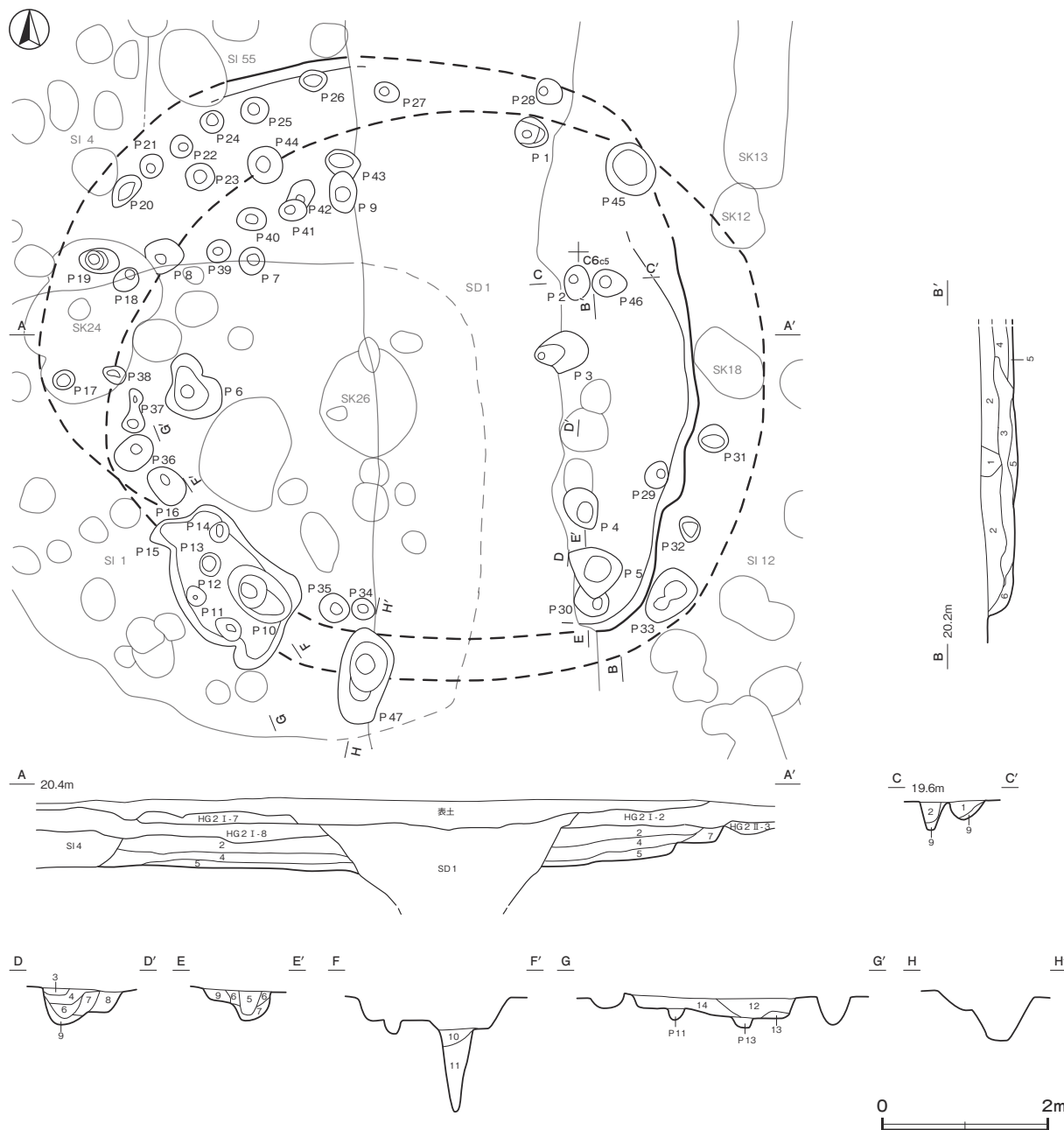
第62図 第7号竪穴建物跡実測図
