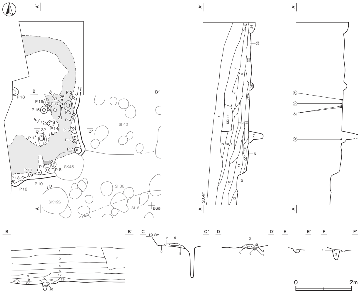
第186図 第43号竪穴建物跡実測図
