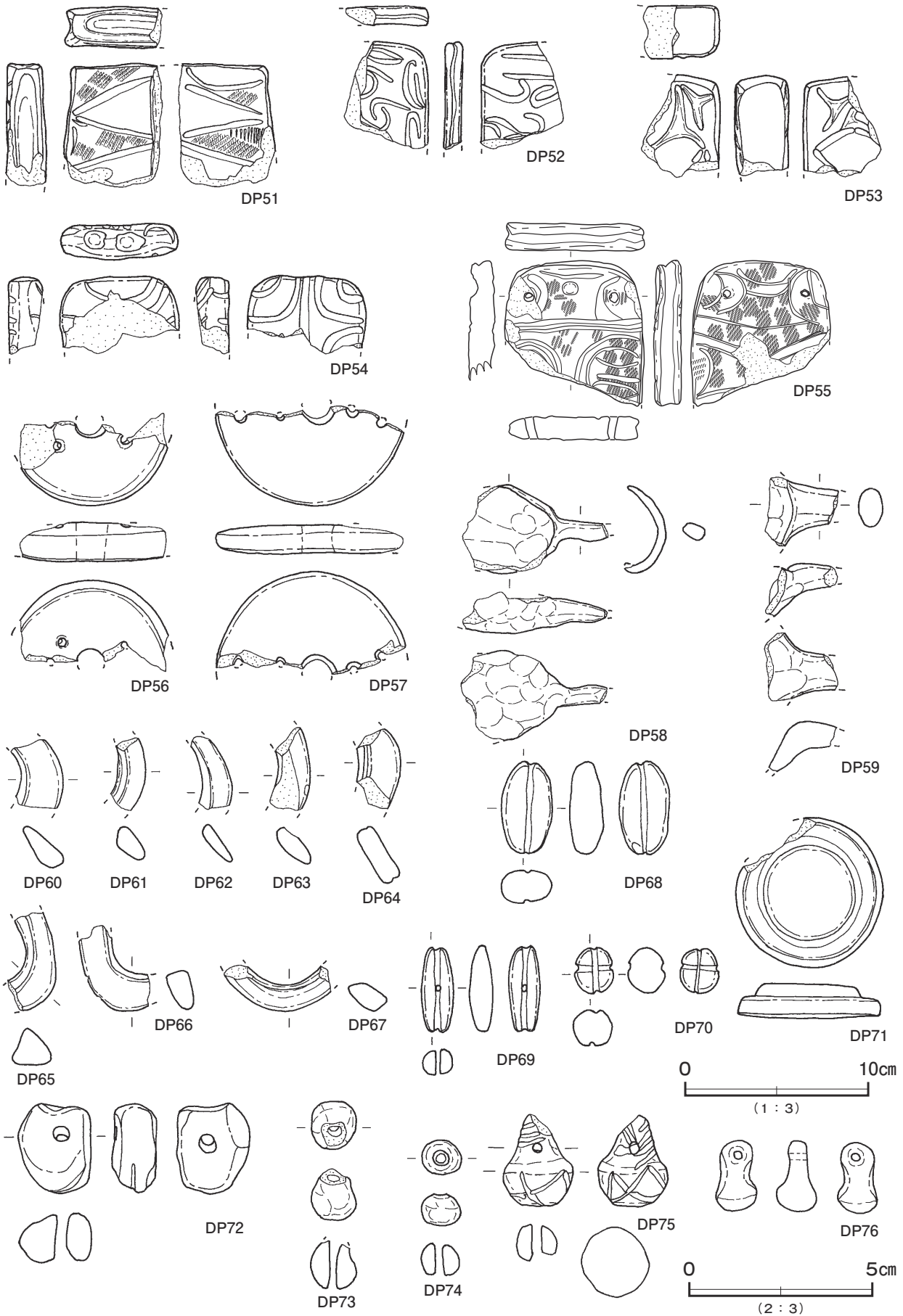
第 308 图 第 2 号遺物包含層出土遺物実測图 (42)
