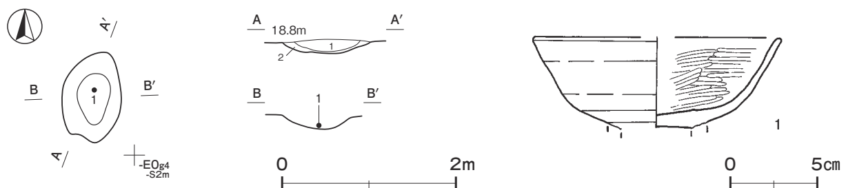
第 406 図 第 93 号土坑・出土遺物実測図
