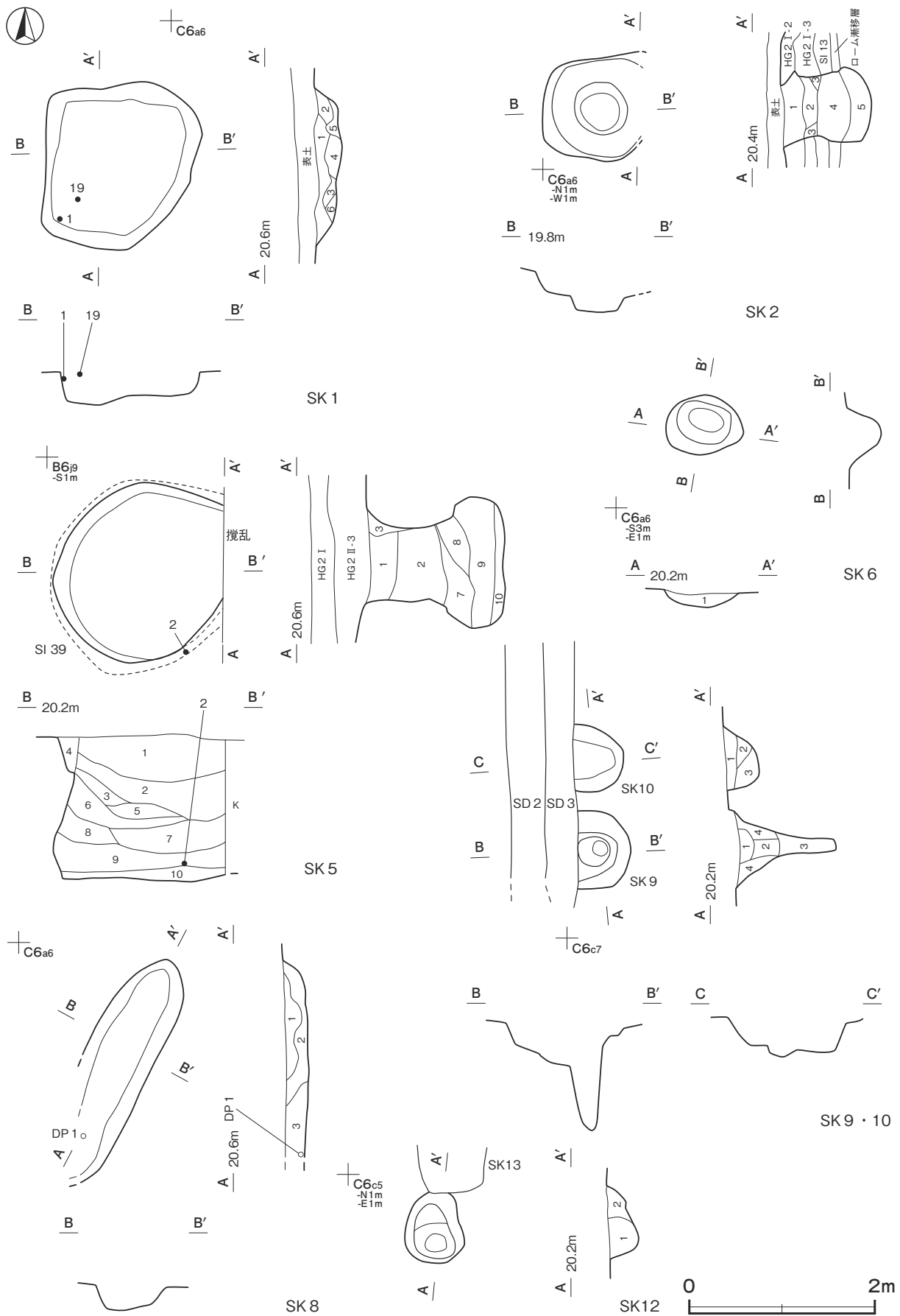
第 222 図 縄文時代の土坑実測図 (1)
