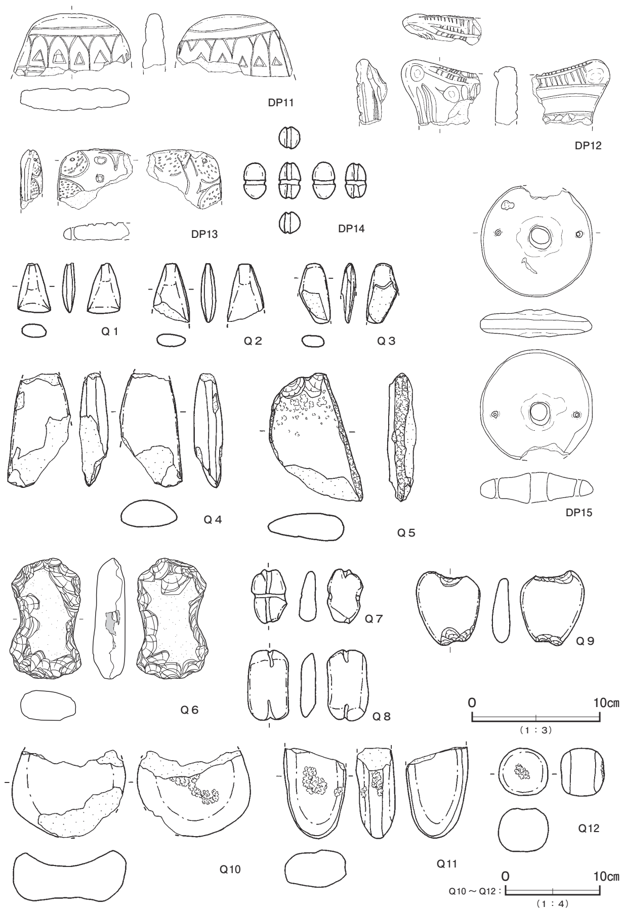
第 128 図 第 22 号 竪穴建物跡出土遺物実測図 (9)
