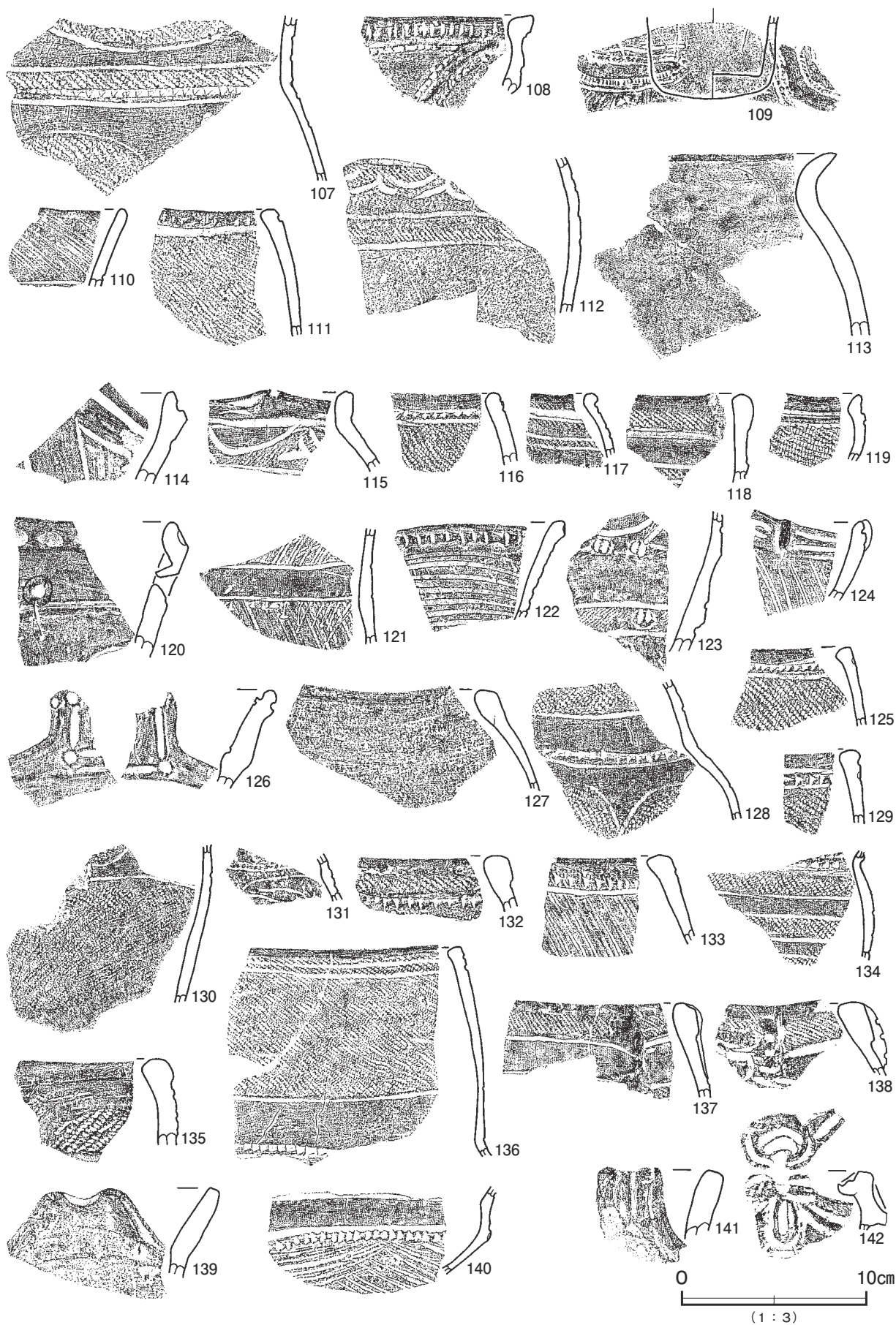
第 162 図 第 35 号 竪穴建物跡出土遺物実測図 (6)
