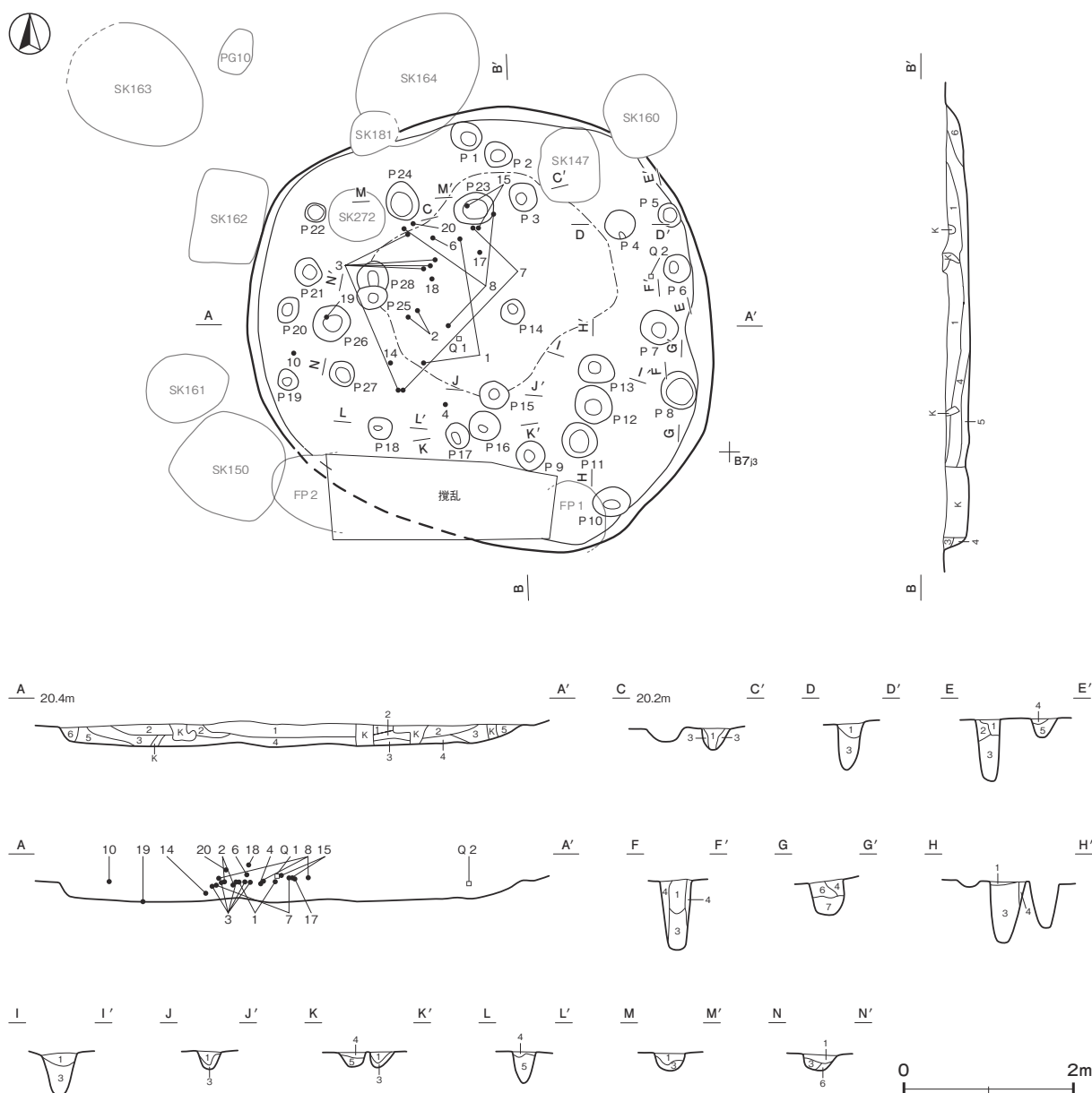
第 196 図 第 48 号 竪穴建物跡実測図
