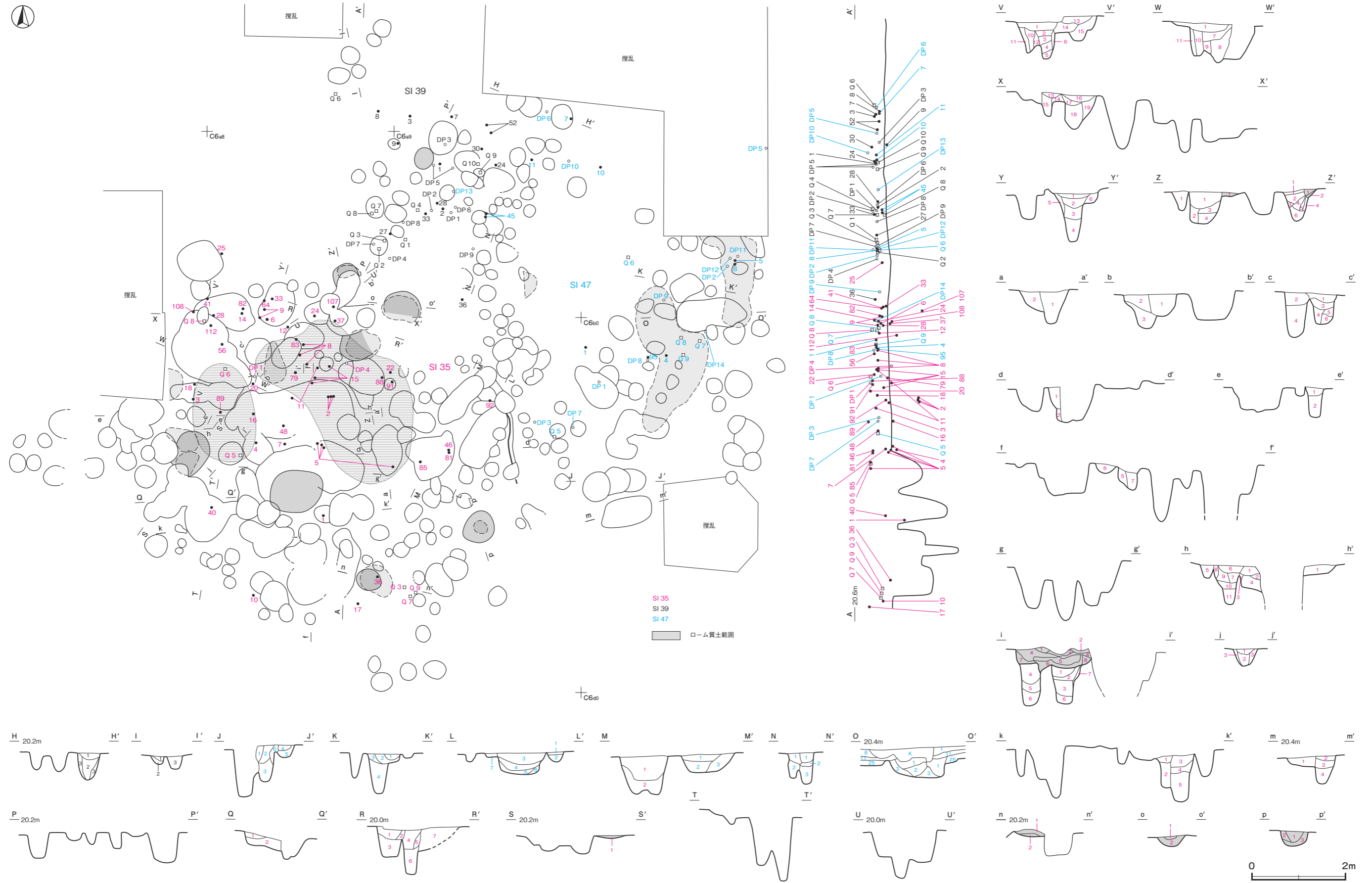
第156図 第35・39・47号竖穴建物跡実測図(2)
