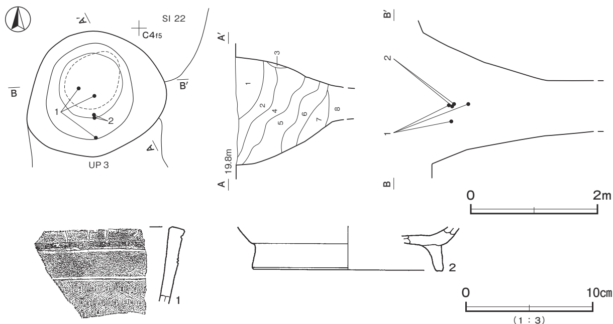
第 341 図 第 1 号井戸跡・出土遺物実測図
