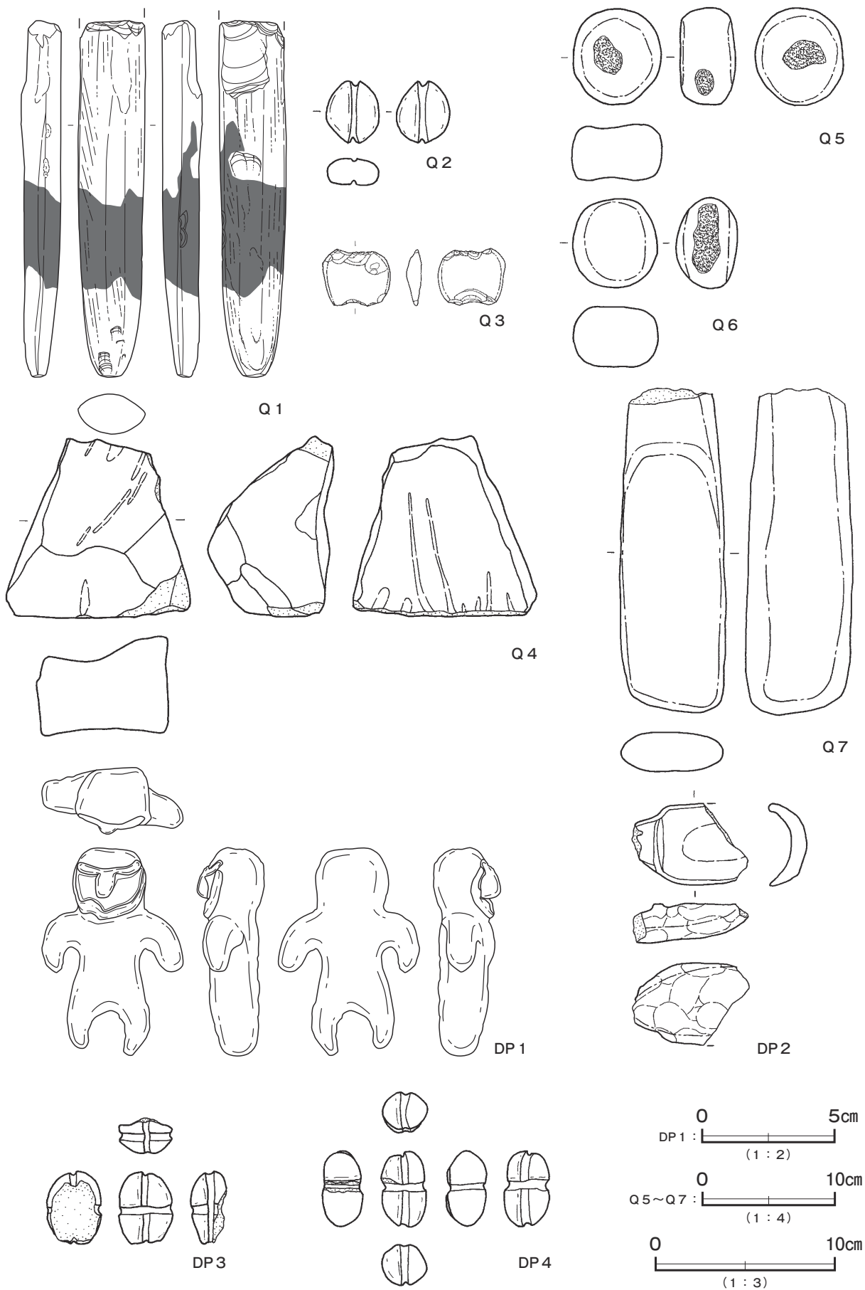
第 101 図 第 15 号 豎穴建物跡出土遺物実測図 (4)
