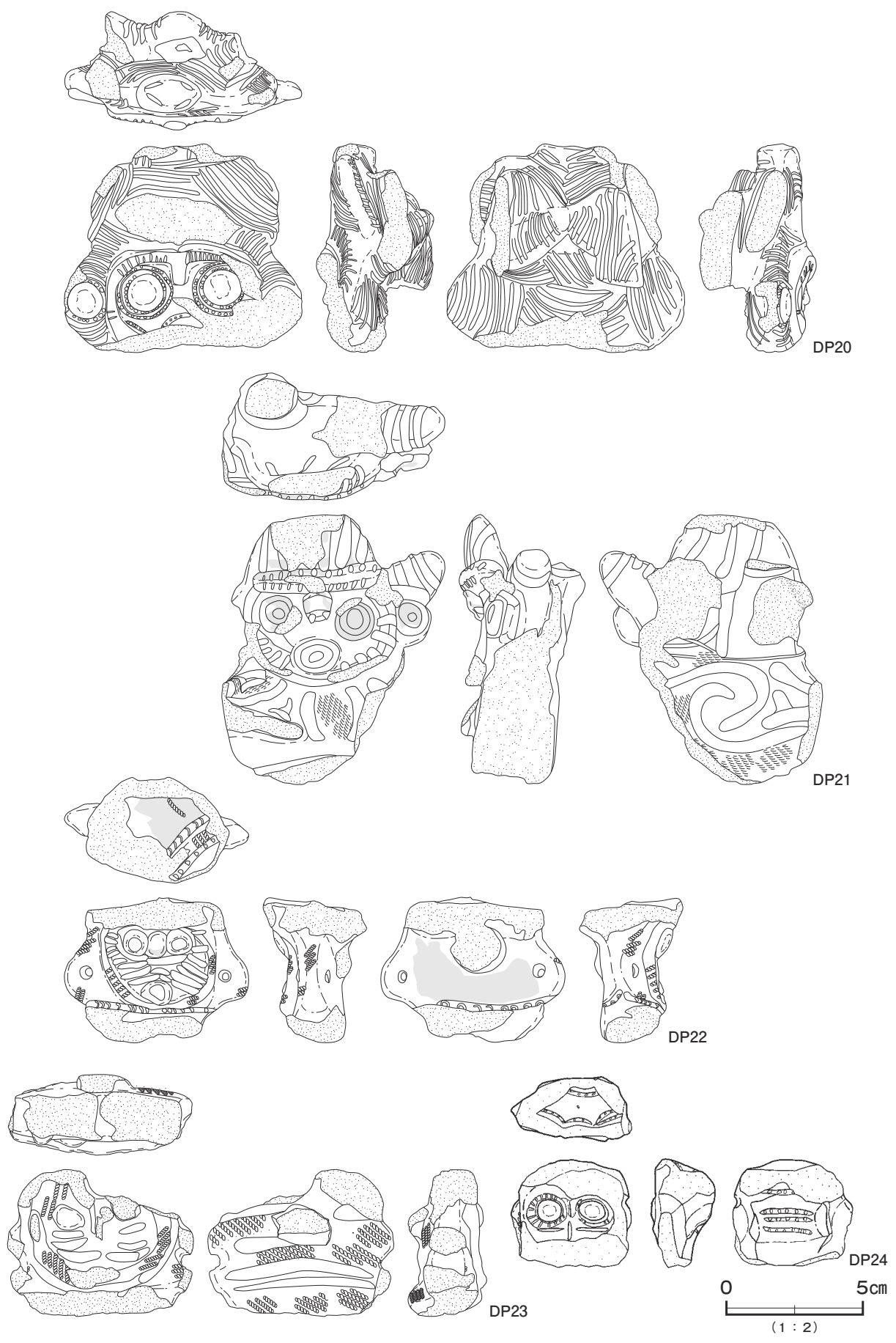
第 304 図 第 2 号遺物包含層出土遺物実測図 (38)
