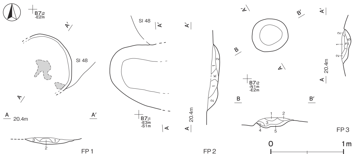
第 261 図 第 1～3号炉跡実測図
