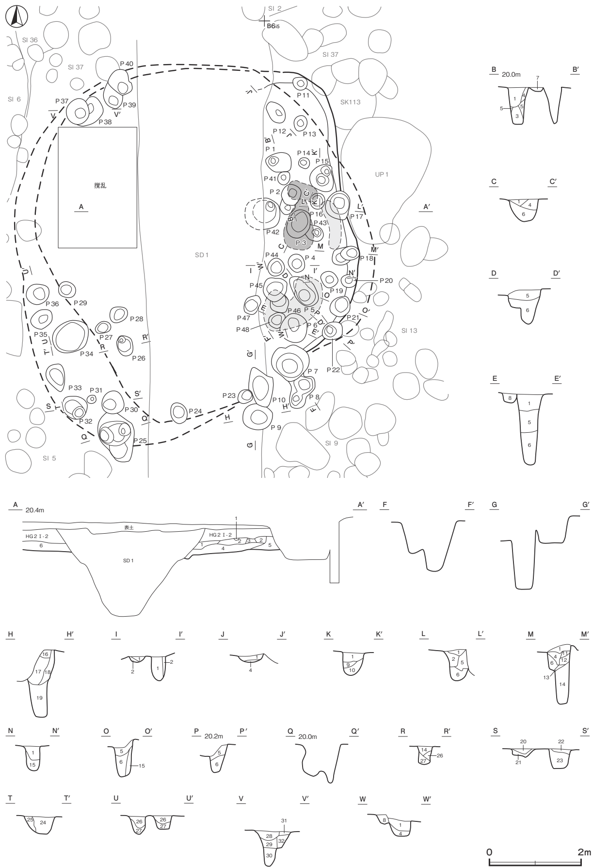
第 20 图 第 3 号竖穴建物跡实测图
