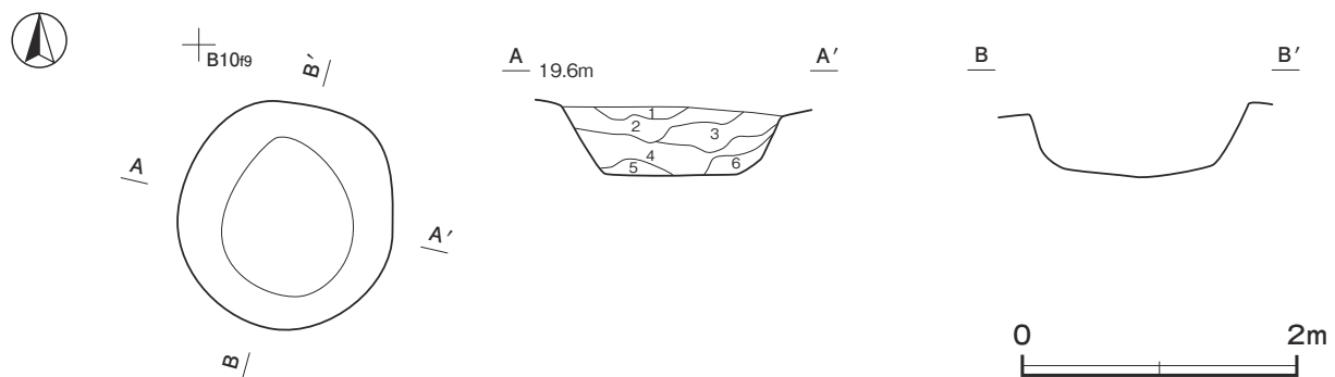
第 368 図 第 151 号土坑実測図
