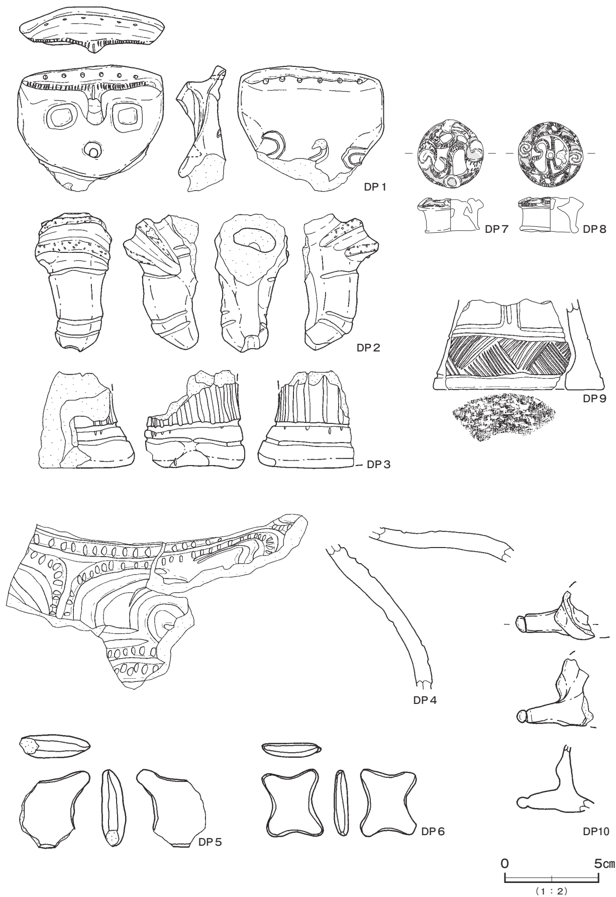
第 127 图 第 22 号竖穴建物跡出土遺物実測图 (8)
