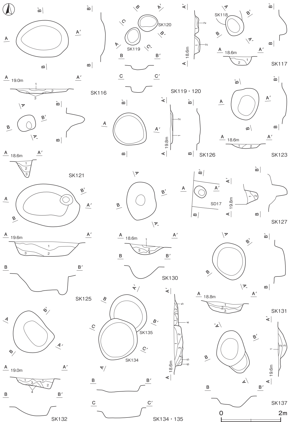
第 442 図 その他の土坑実測図(3)
