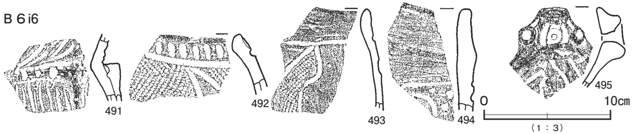
第 284 图 第 2 号遺物包含層出土遺物実測図 (18)
