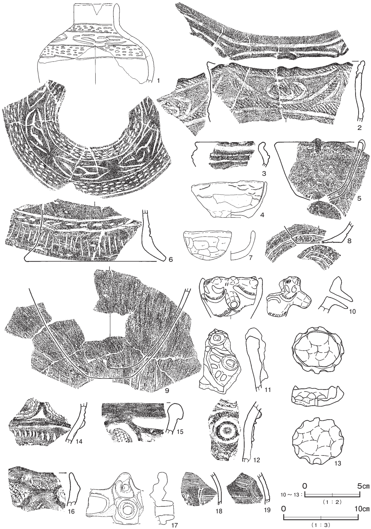
第 120 图 第 22 号竖穴建物跡出土遺物実測图 (1)
