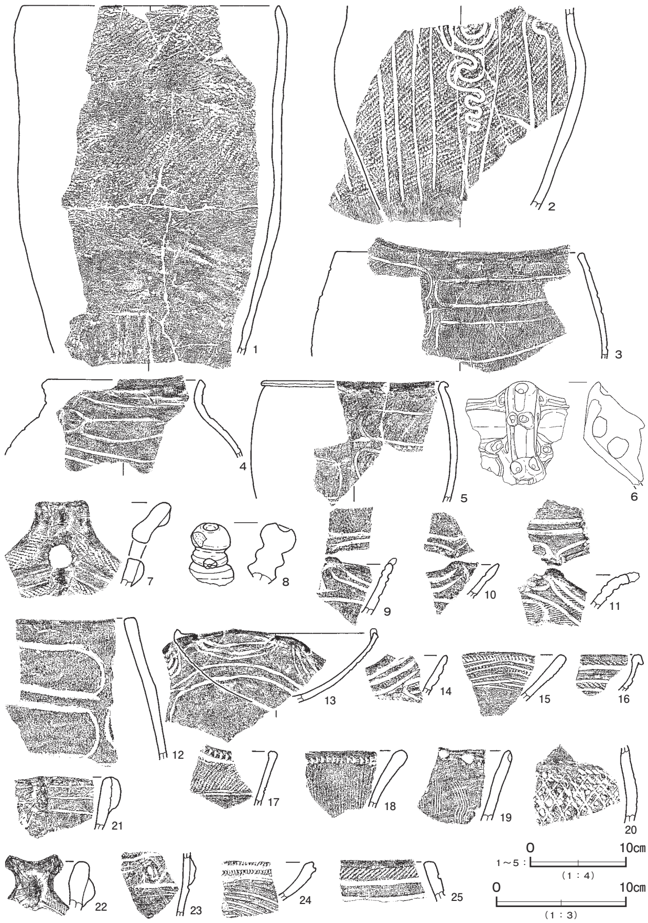
第 40 図 第 19 号豎穴建物跡出土遺物実測図 (1)
