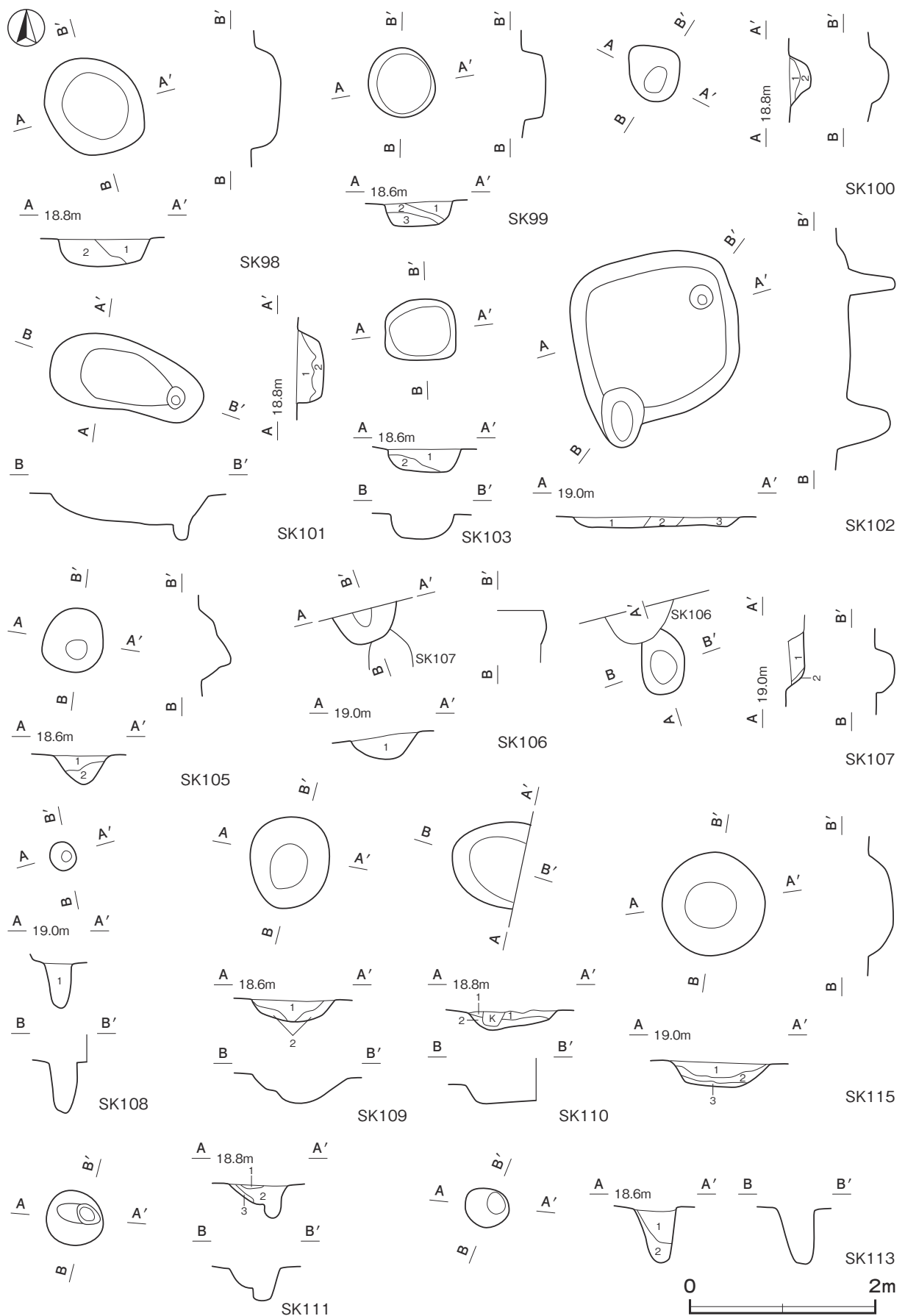
第 441 図 その他の土坑実測図(2)
