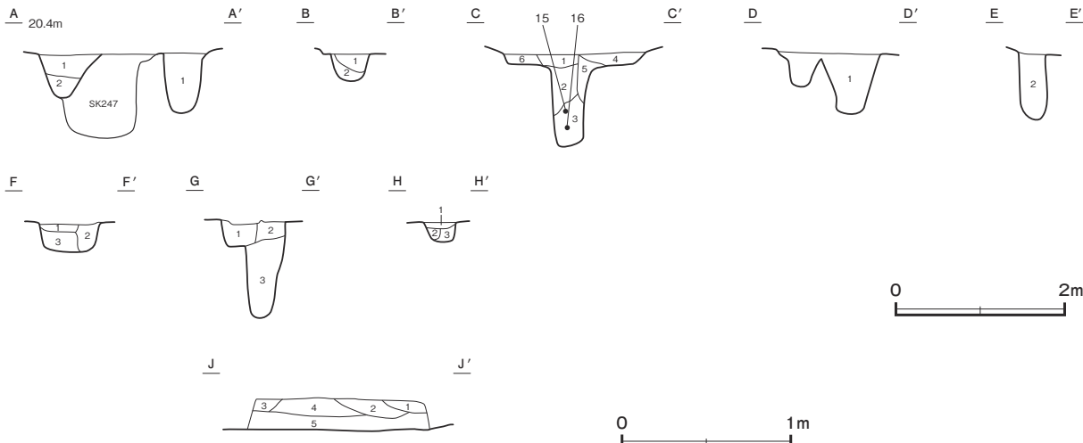
第 202 図 第 53 号 竪穴建物跡実測図
