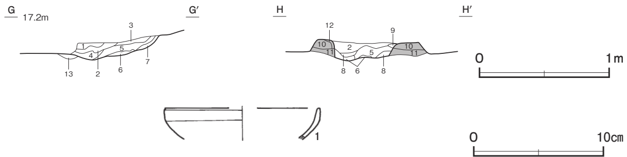
第 372 図 第 43 号竪穴建物跡・出土遺物実測図
