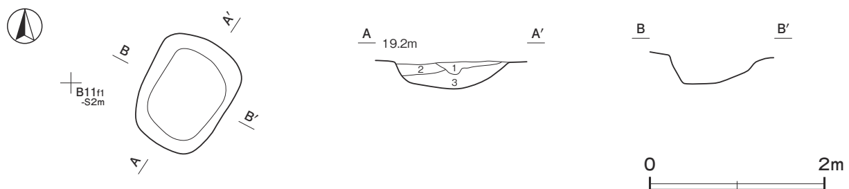
第411図 第153号土坑実測図
