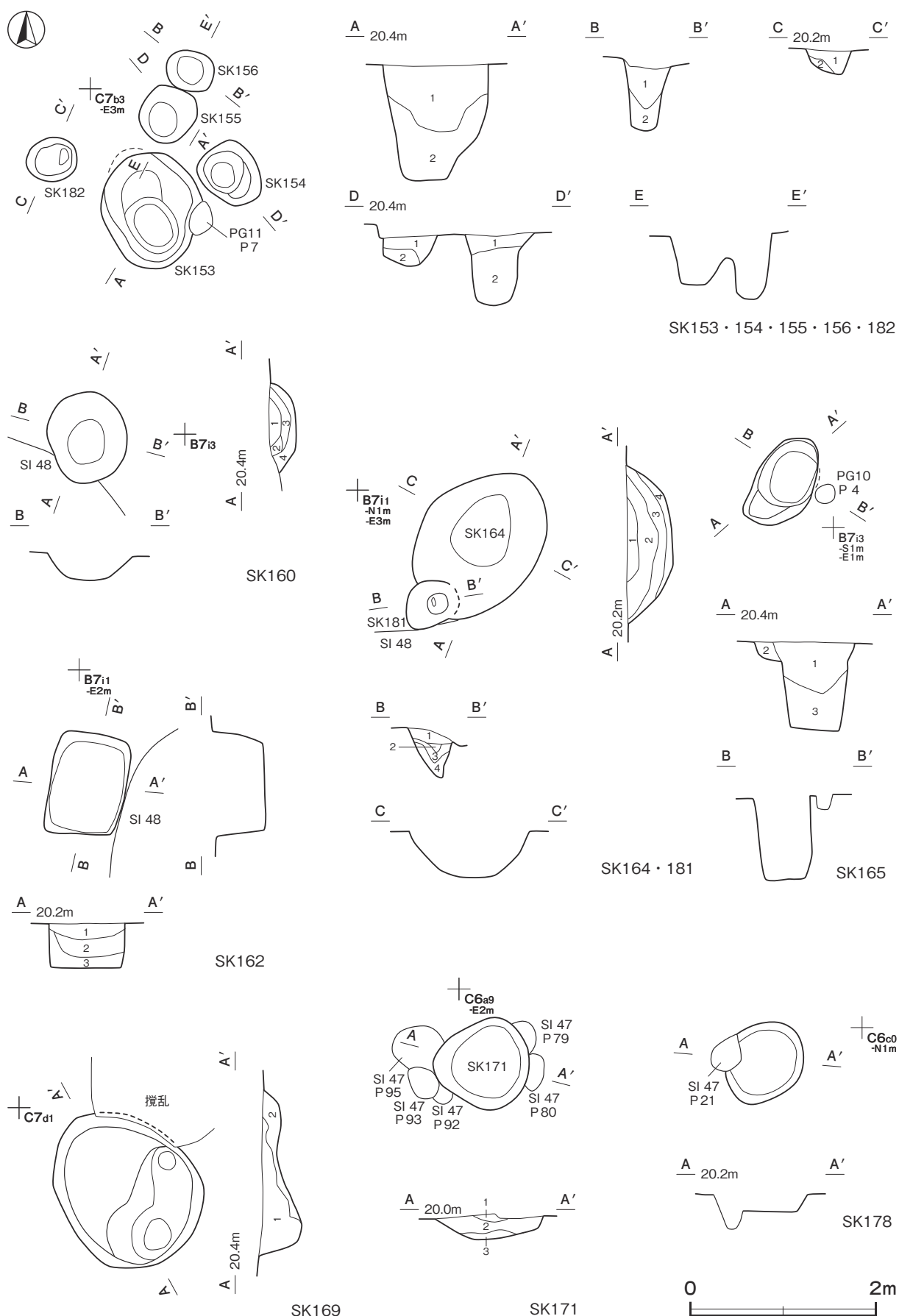
第 233 図 縄文時代の土坑実測図 (12)
