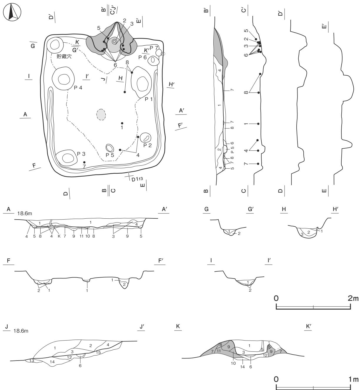
第390図 第34号竈穴建物跡実測図
