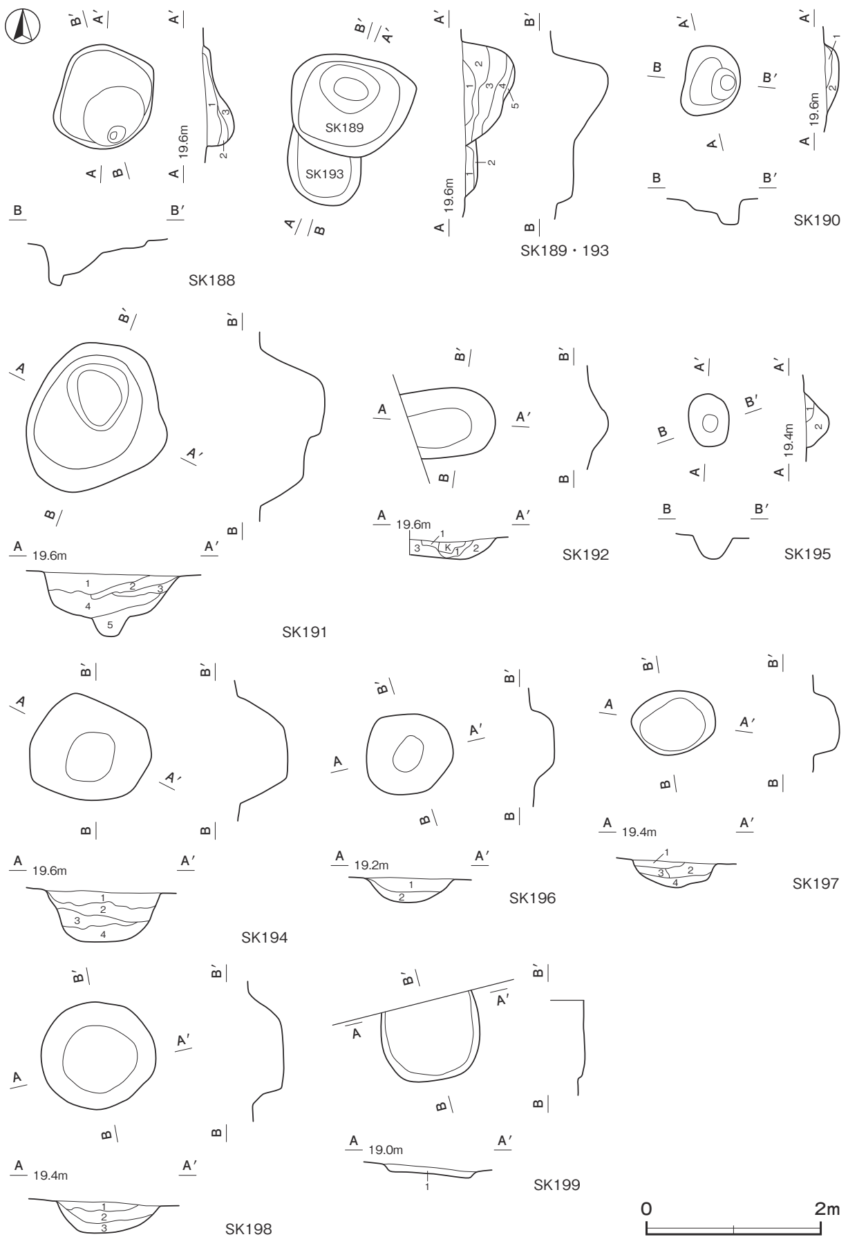
第 447 図 その他の土坑実測図(8)
