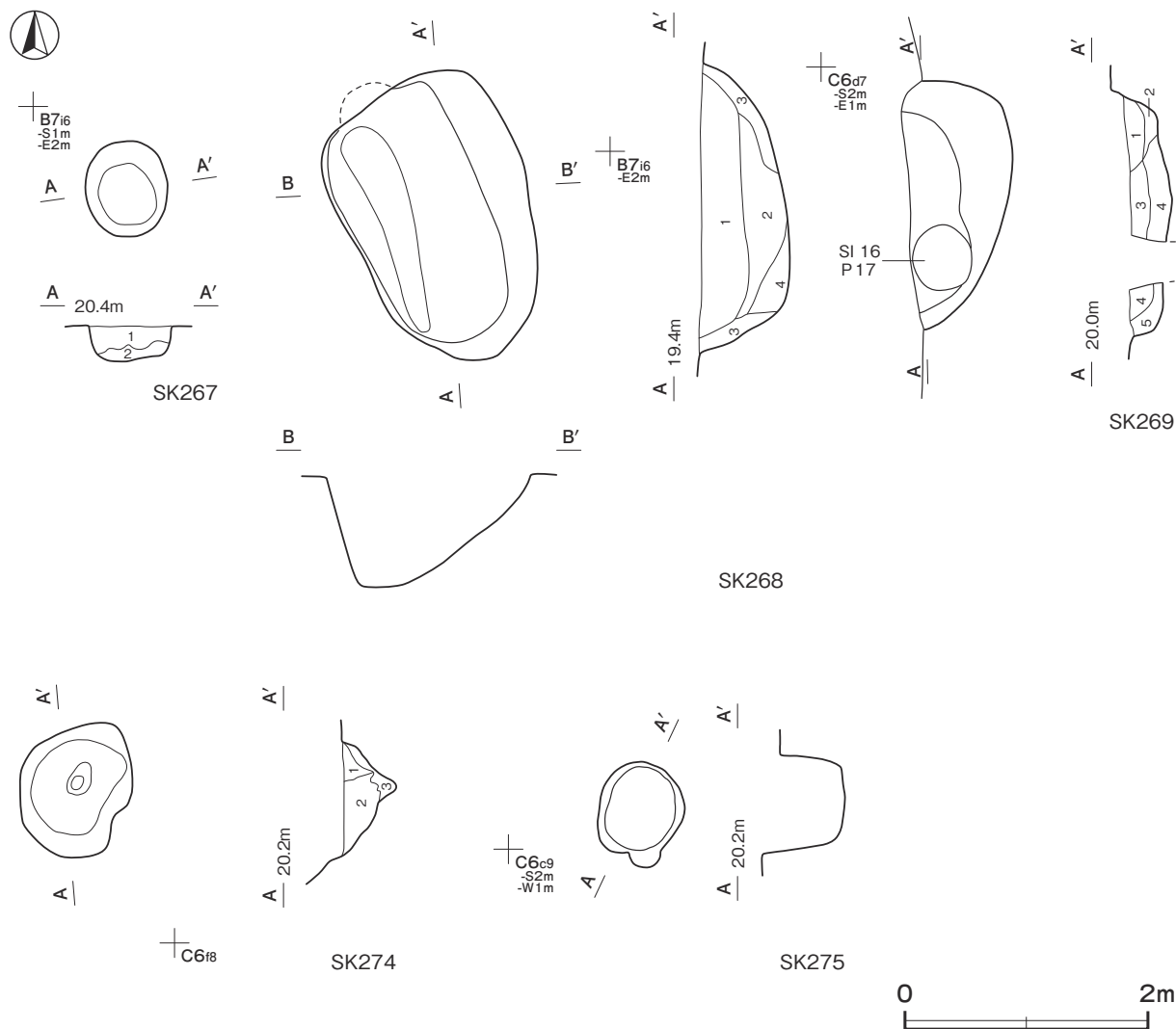
第 238 図 縄文時代の土坑実測図 (17)
