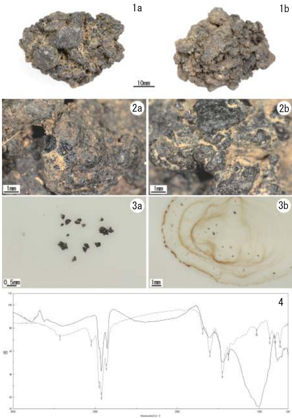
図1 黒色付着礫塊とクロロホルム溶融試験および赤外分光スペクトル図 1a・1b. 黒色付着礫塊 2a・2b. 同拡大写真 3a・3b. クロロホルム溶融試験の前後 4. 赤外分光スペクトル図（実線：黒色付着物，点線と数字：天然アスファルトとその吸収位置）
