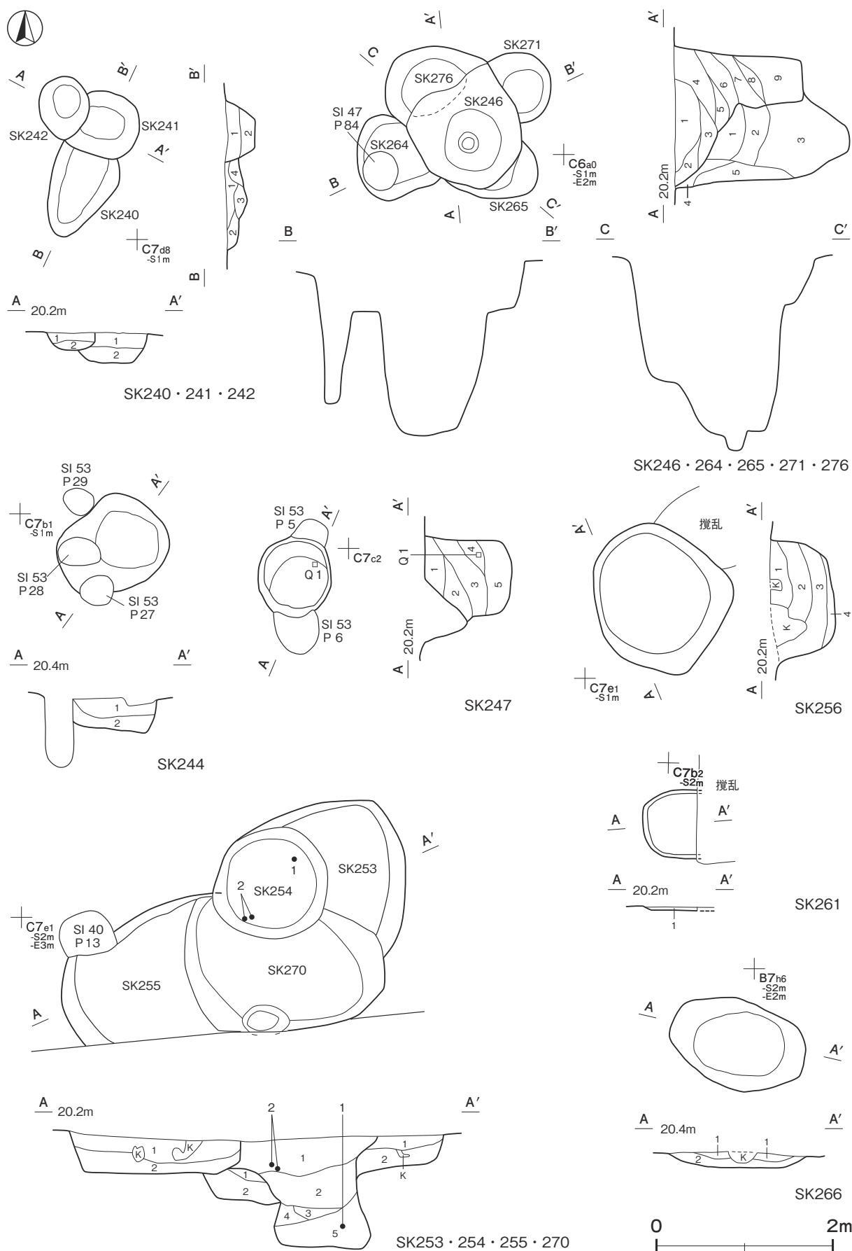
第 237 図 縄文時代の土坑実測図 (16)
