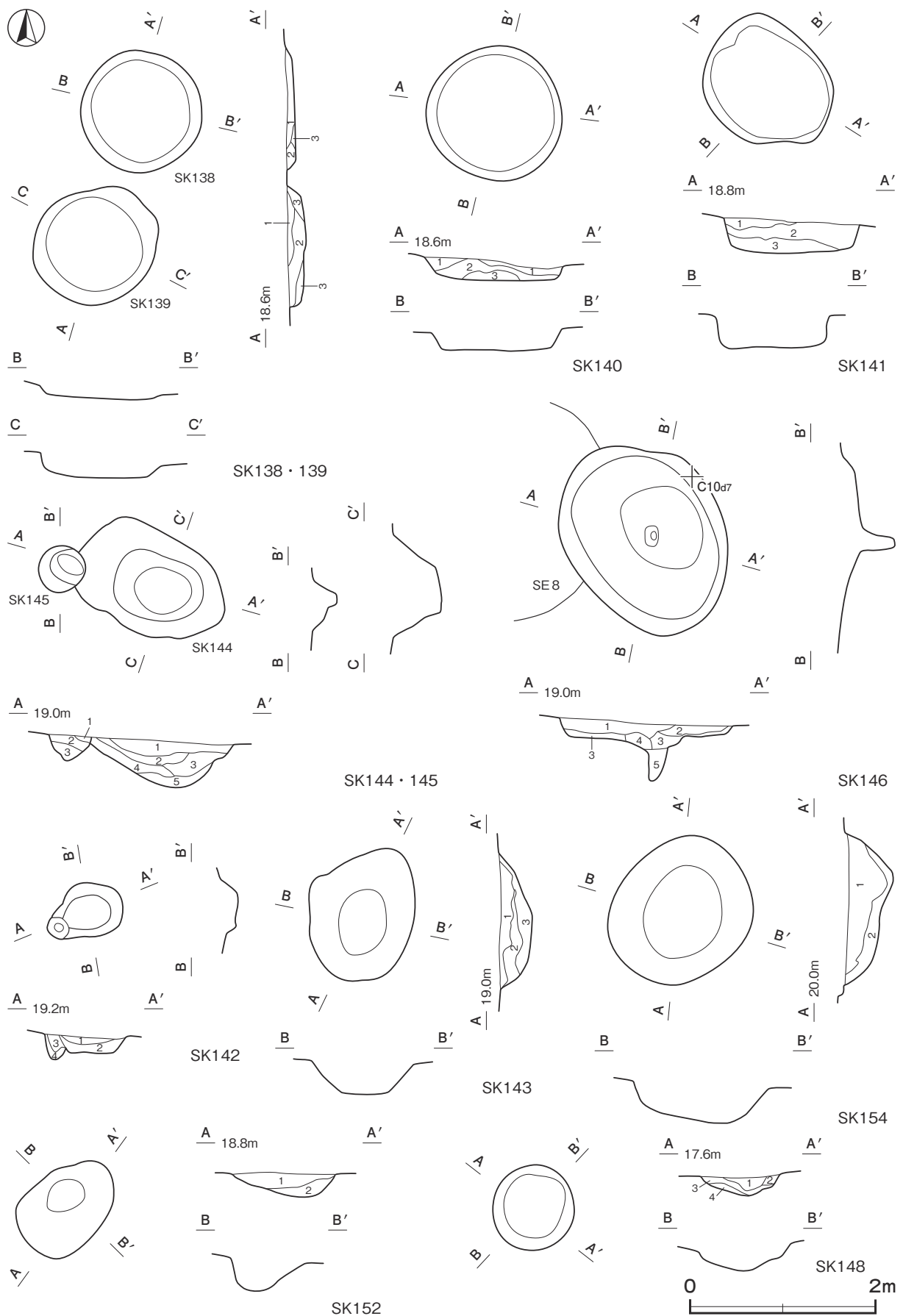
第 443 図 その他の土坑実測図(4)
