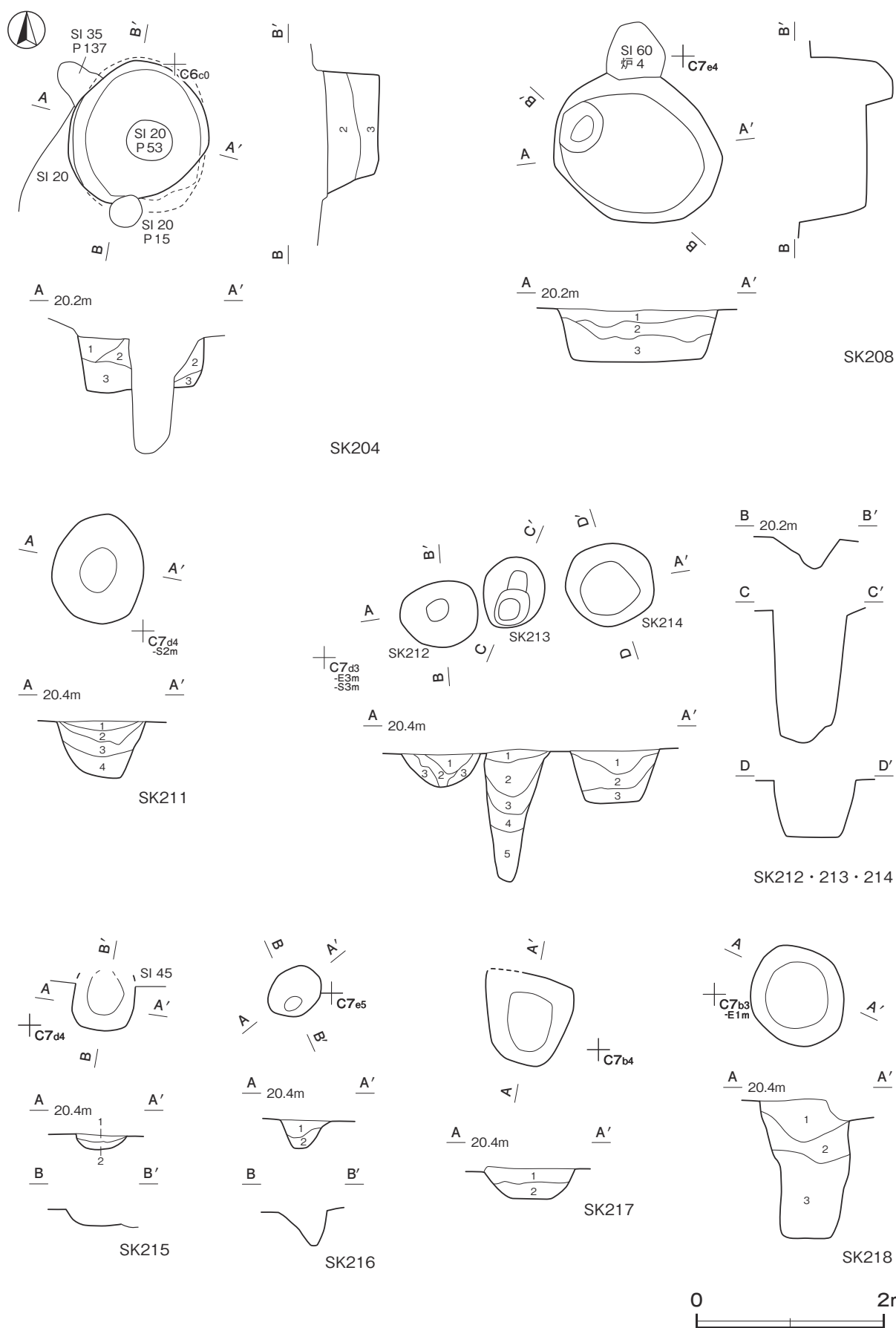
第 235 図 縄文時代の土坑実測図 (14)
