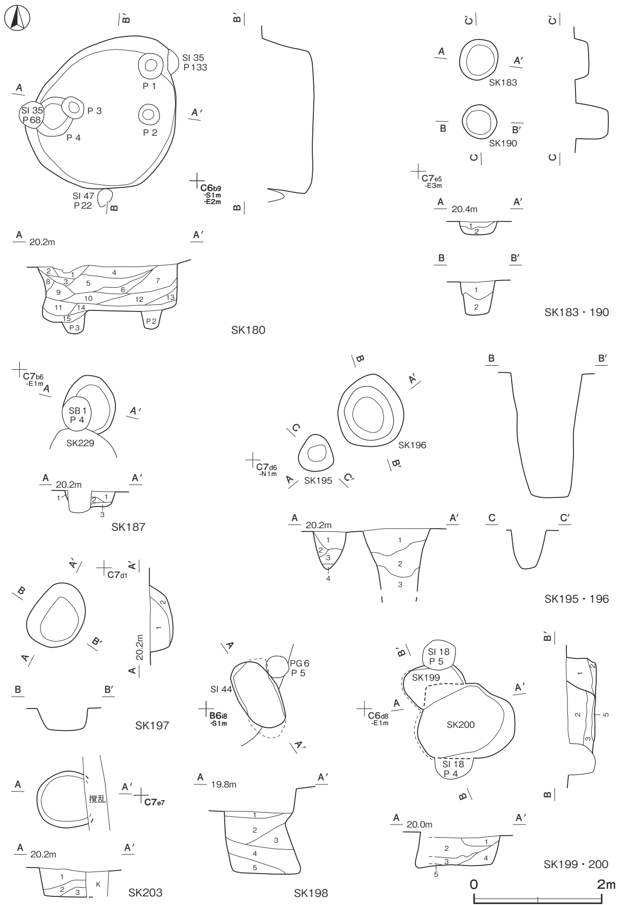
第 234 図 縄文時代の土坑実測図 (13)
