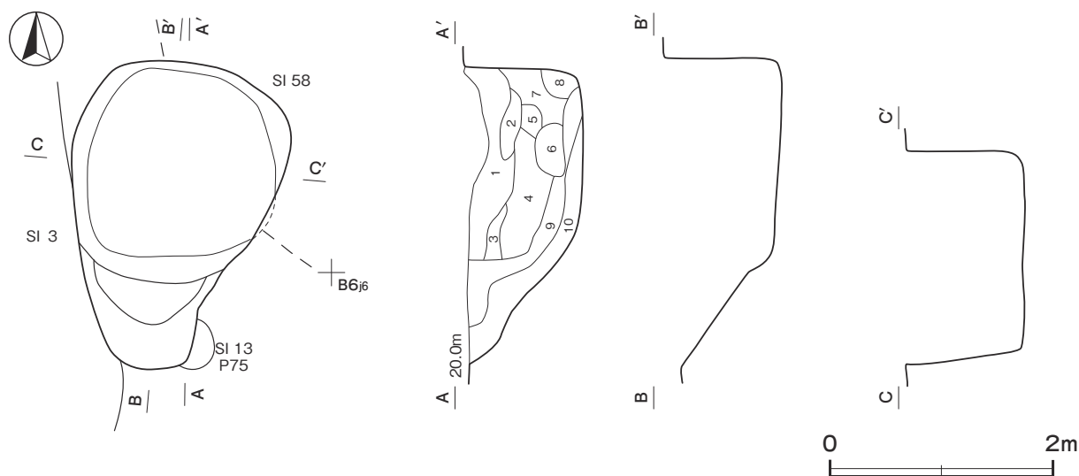
第 325 図 第 1 号地下式坑実測図
