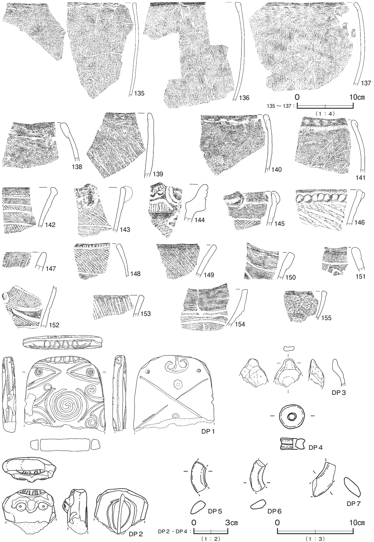
第 29 图 第 4 · 55 号竖穴建物跡出土遺物実測図 (5)
