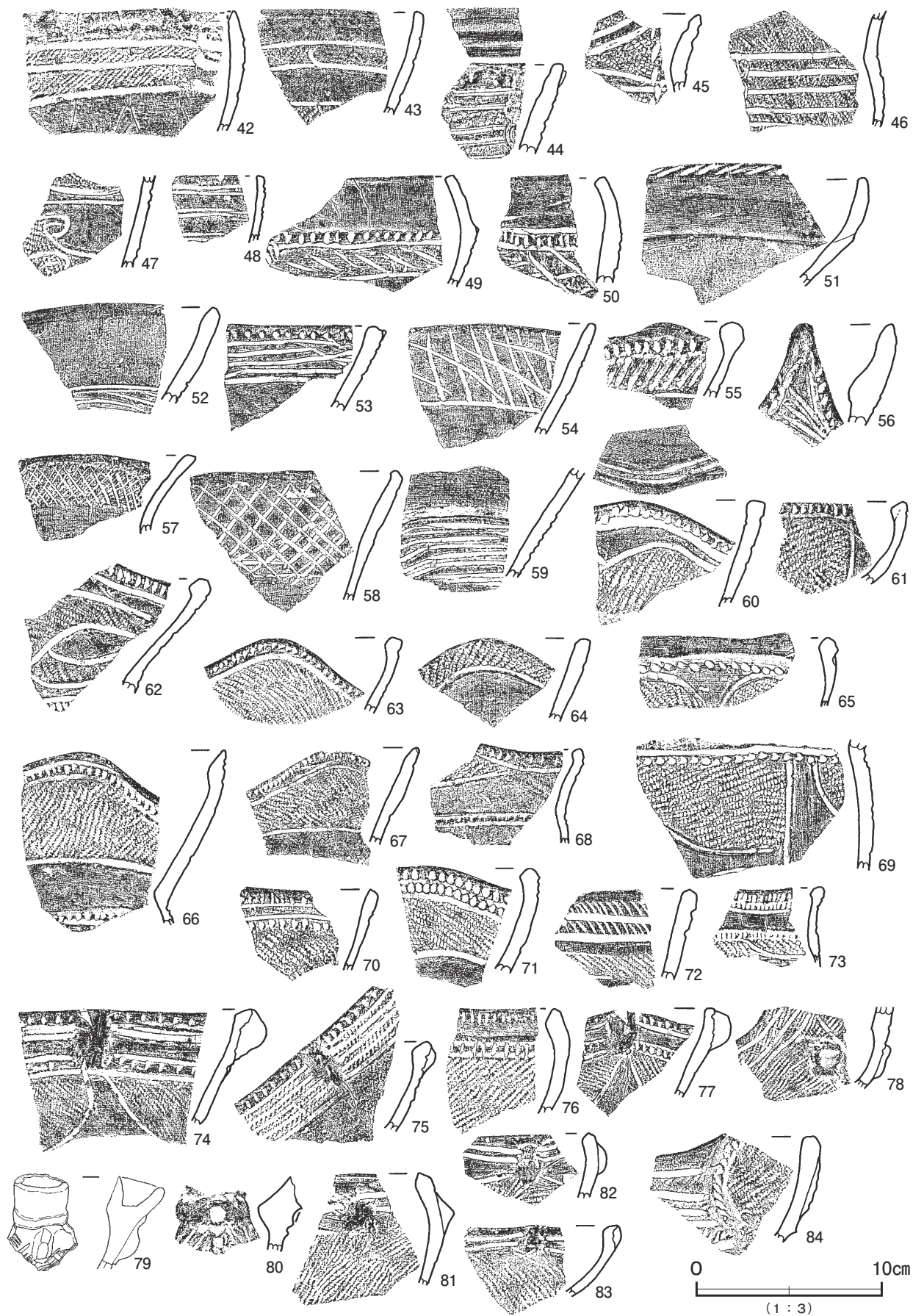
第 48 图 第 6 号竖穴建物跡出土遺物実測图 (3)
