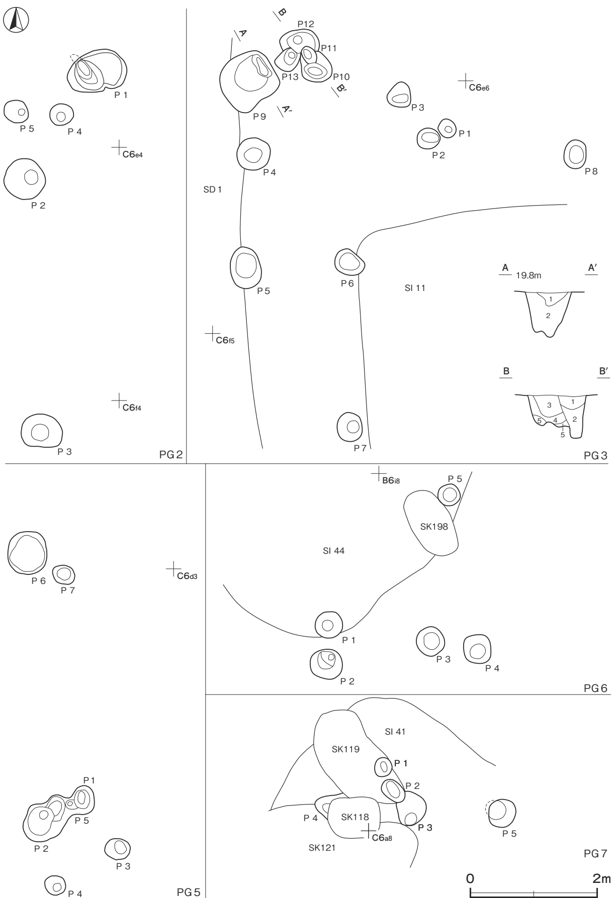
第 262 図 第 2・3・5～7号ピット群実測図
