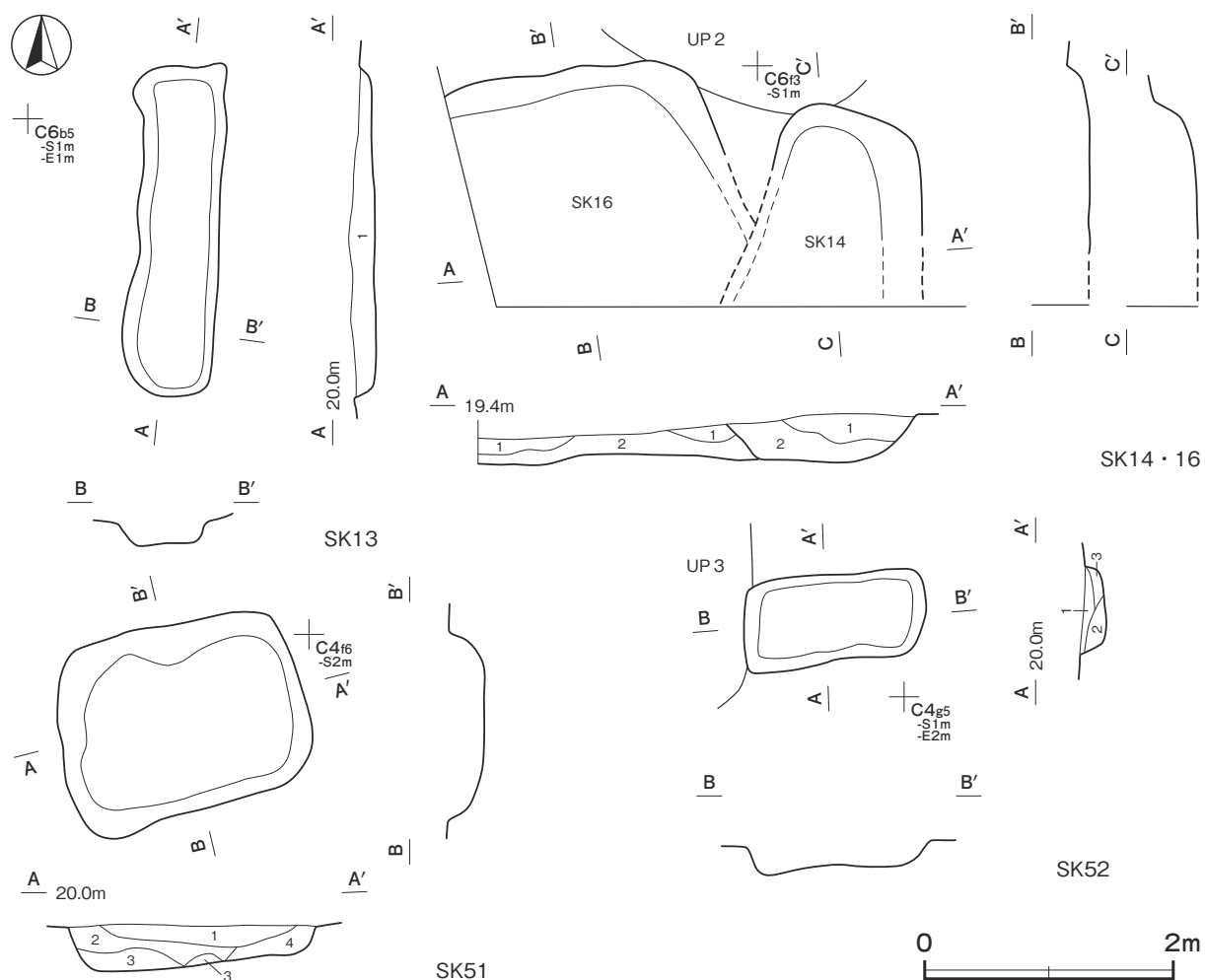
第 335 图 室町時代土坑实测图 (1)
