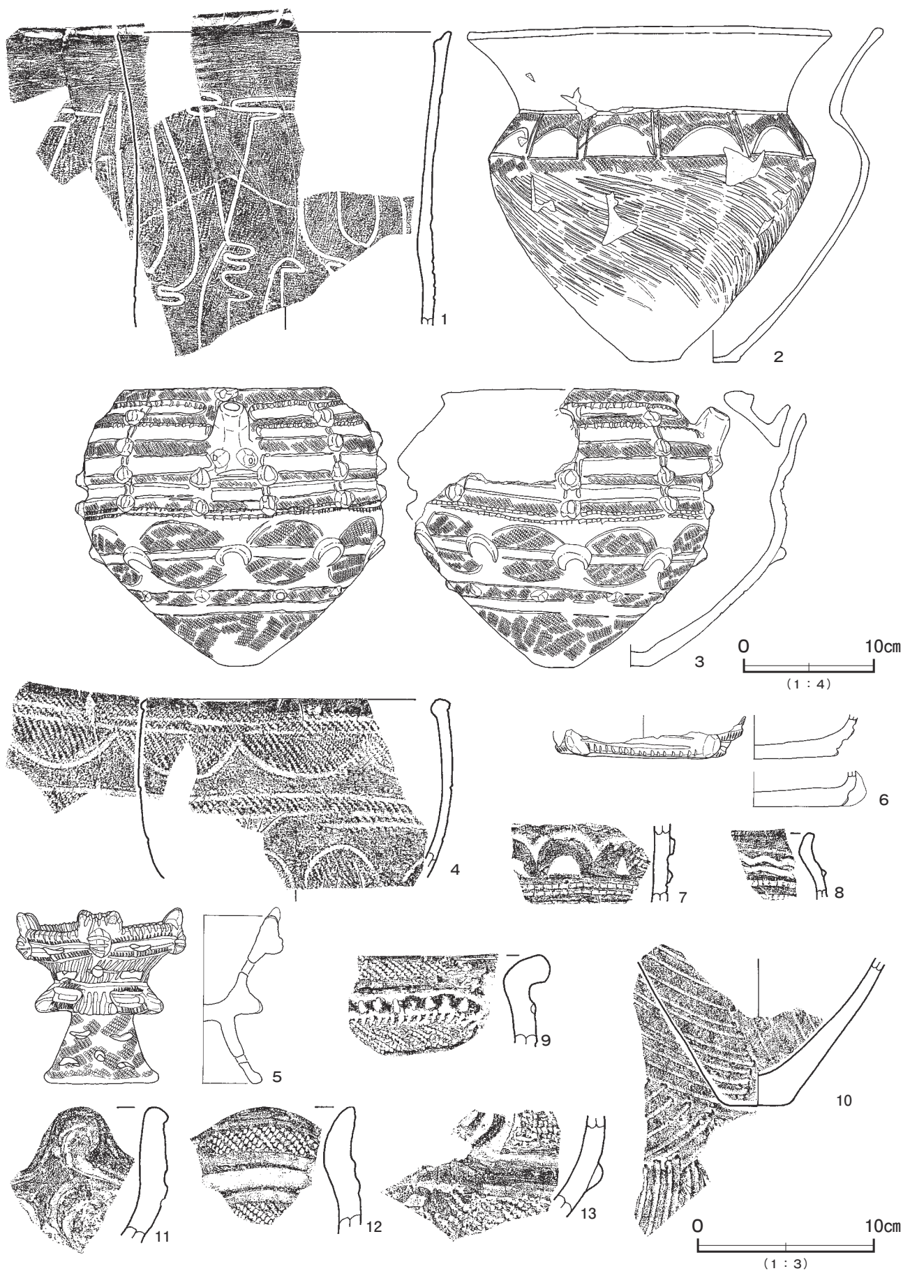
第 88 图 第 13 号竖穴建物跡出土遺物実測图 (1)
