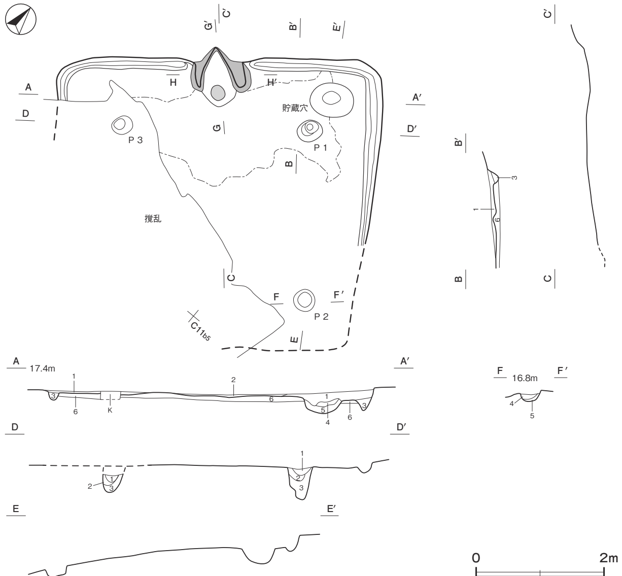
第 371 図 第 43 号 貯蔵穴 建物跡 実測図
