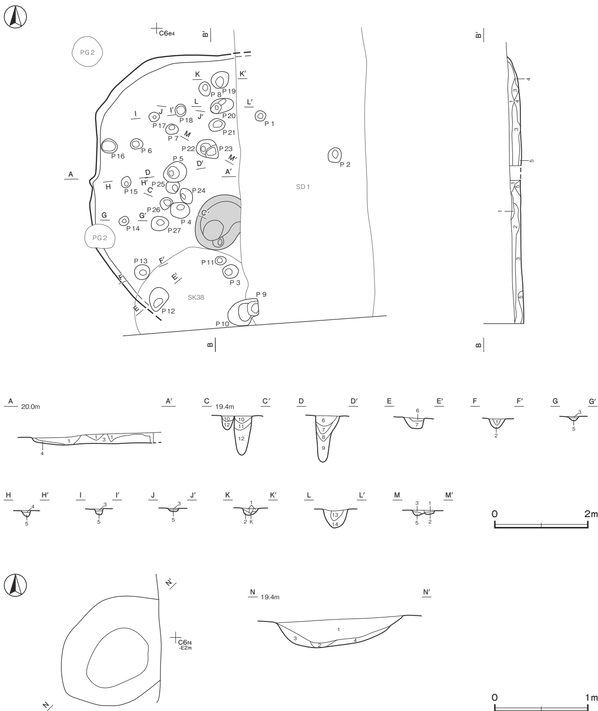
第 93 図 第 14 号 豎穴 建物跡 実測図
