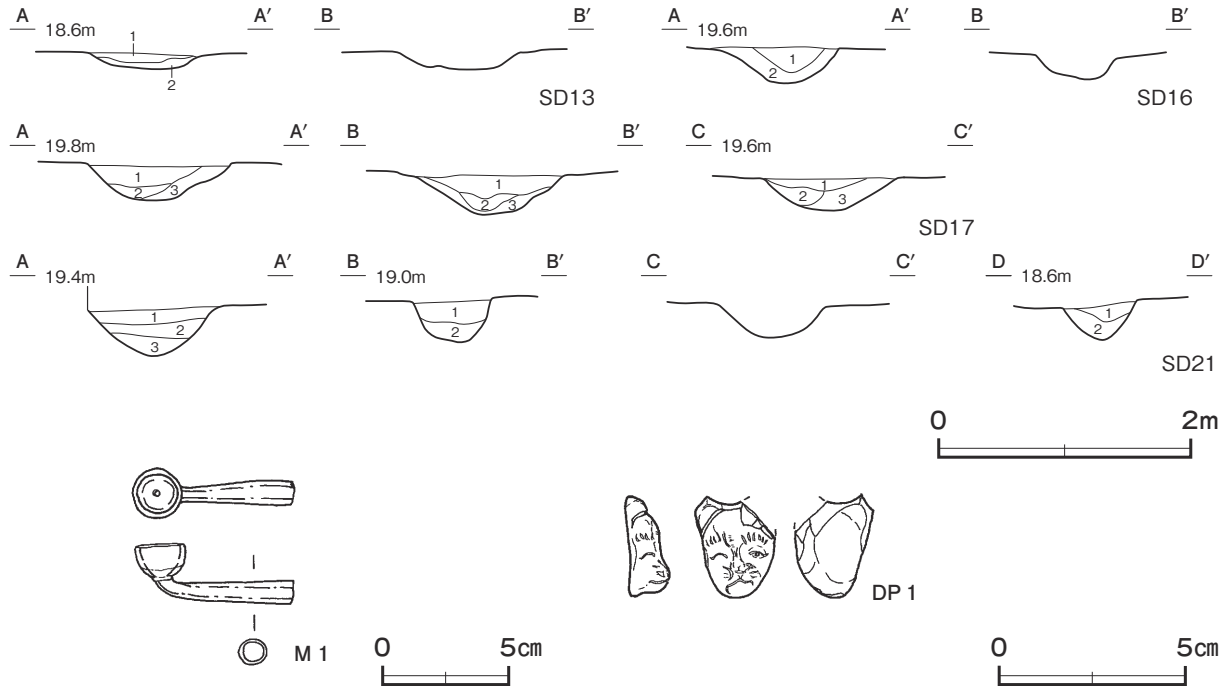
第448図 第13・16・17・21号溝跡・出土遺物実測図
