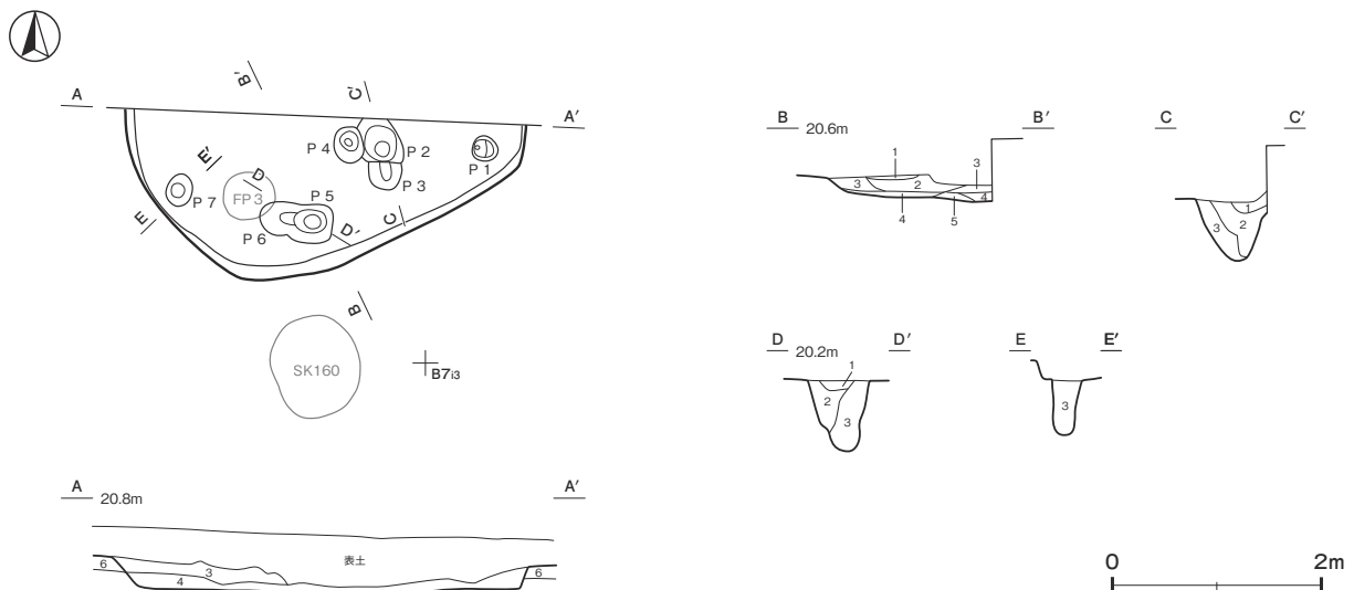
第 199 図 第 49 号竪穴建物跡実測図
