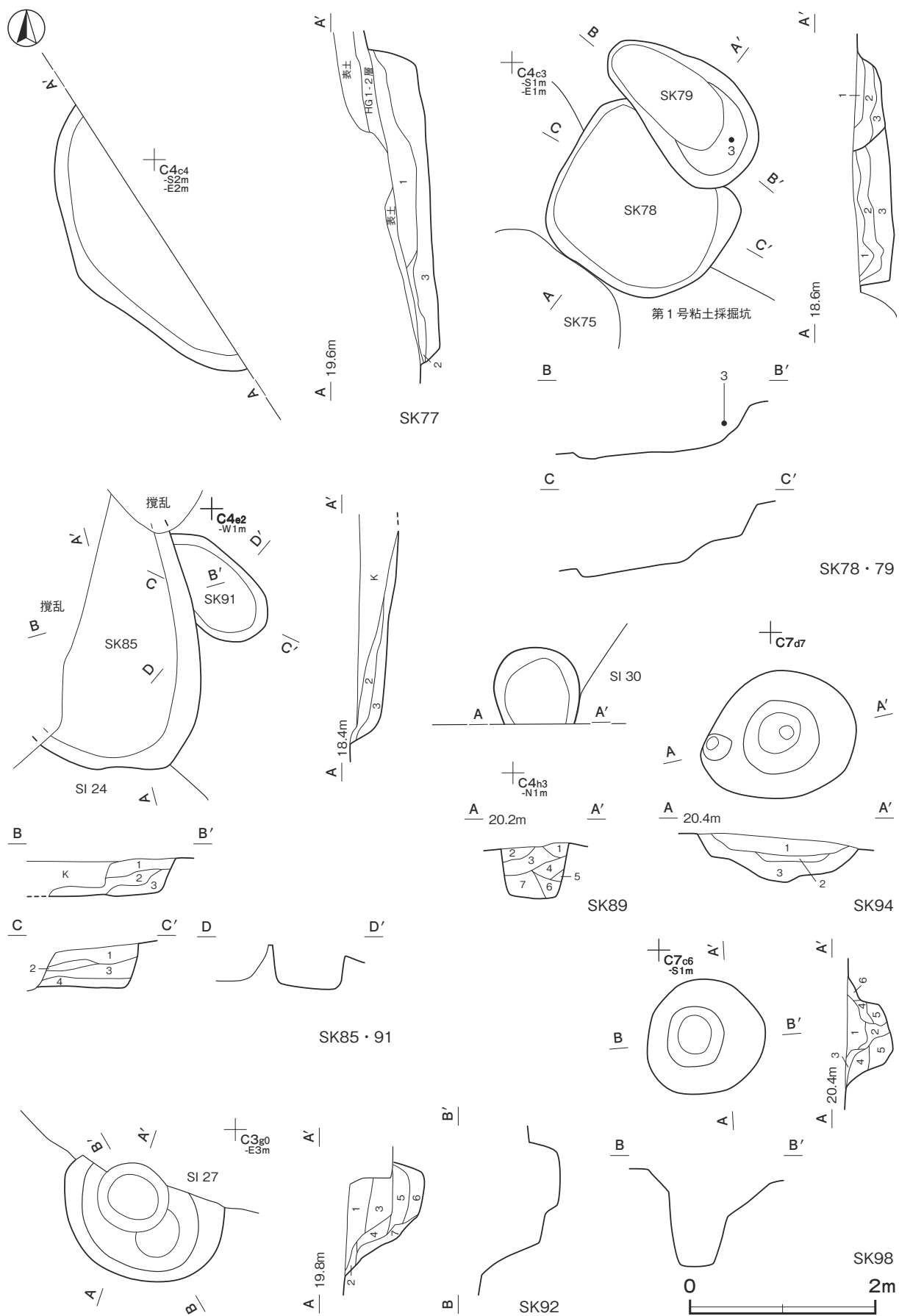
第 228 図 縄文時代の土坑実測図 (7)
