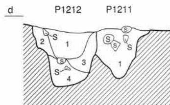
P1212 1 10YR3/2黒褐色土 しまり強 粘性あり 白色粒子多量 2 10YR3/1黒褐色土 しまり強 粘性あり 白色粒子多量 版築 3 10YR2/3暗褐色土 しまり弱 粘性あり 4 10YR2/2黒褐色土 しまり弱 粘性あり 白色粒子少量 小礫多量 P1211 1 10YR3/3暗褐色土 しまり強 粘性あり 白色粒子少量 礫多量
