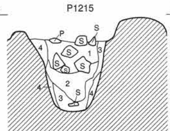
1 10YR2/2黒褐色土 しまり強 粘性あり 白色粒子・小礫多量 炭化粒少量 埋め戻し 2 10YR3/3暗褐色土 しまり強 粘性あり 白色粒子少量 3 10YR3/3暗褐色土 しまりなし 粘性弱 2より砂多量 4 10YR4/2灰黄褐色土 しまり強 粘性なし 砂質土 版築
