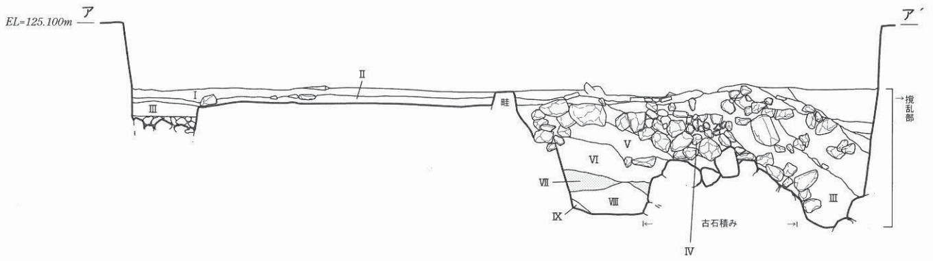
第8図 北グリッド中央畦南壁土層図
