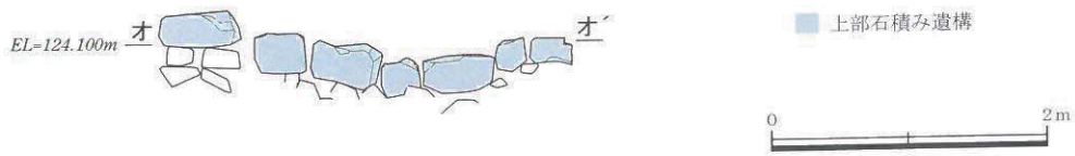
第14図 上部石積み西壁立面図
