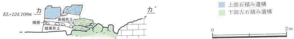
第15図 上部石積みと下部古石積みの北壁立面図
