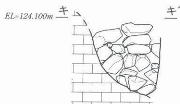
第17図 下部古石積み西壁立面図
