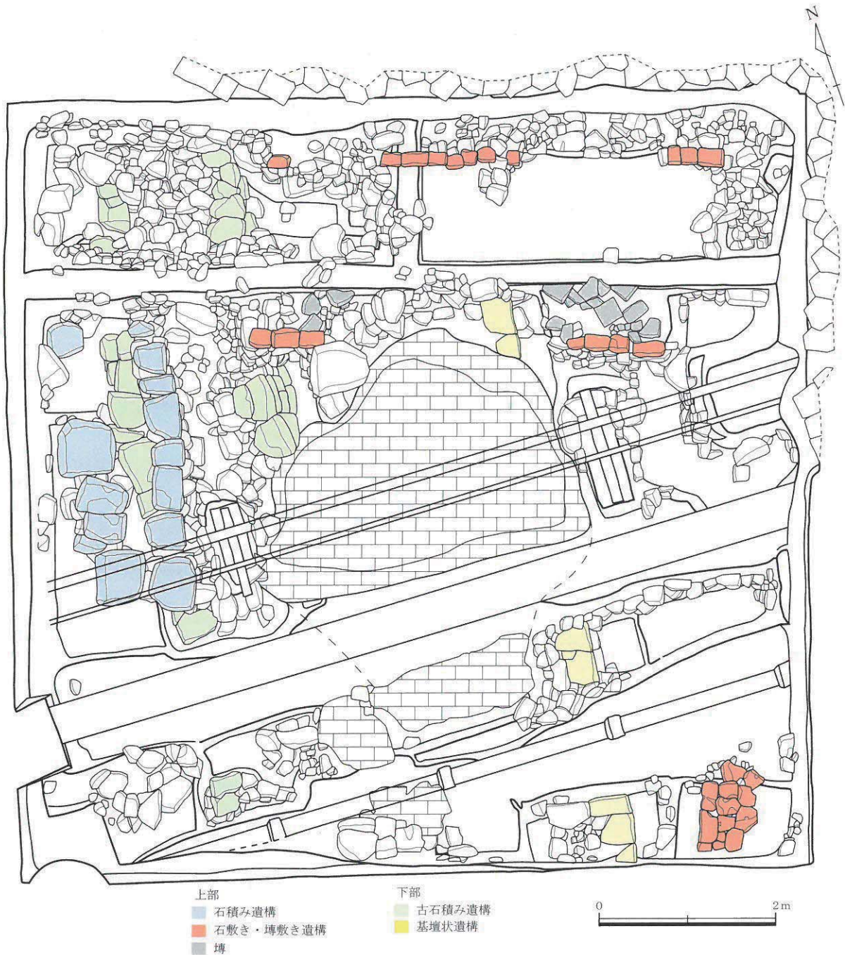
第12図 遺構平面図
