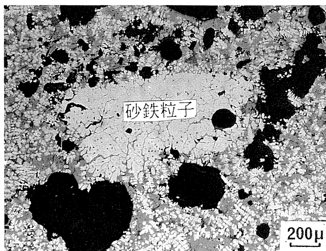
2 ⑤鉄滓の組織
