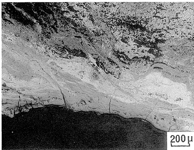
1 ②試料の組織
