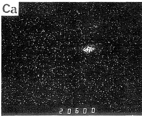
2 ②試料中在物の元素分布 (EPMA)
