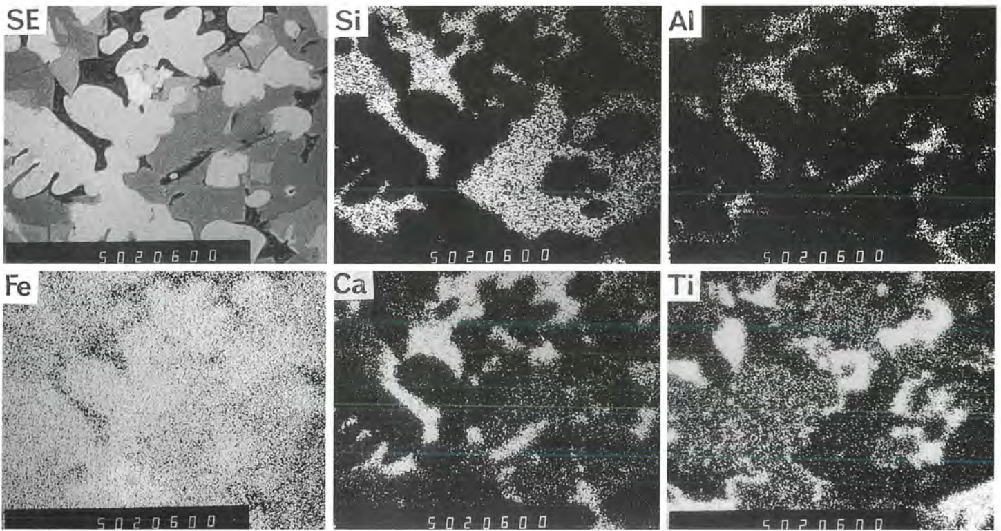
1 ⑤鉄滓の元素分布 (EPMA)
