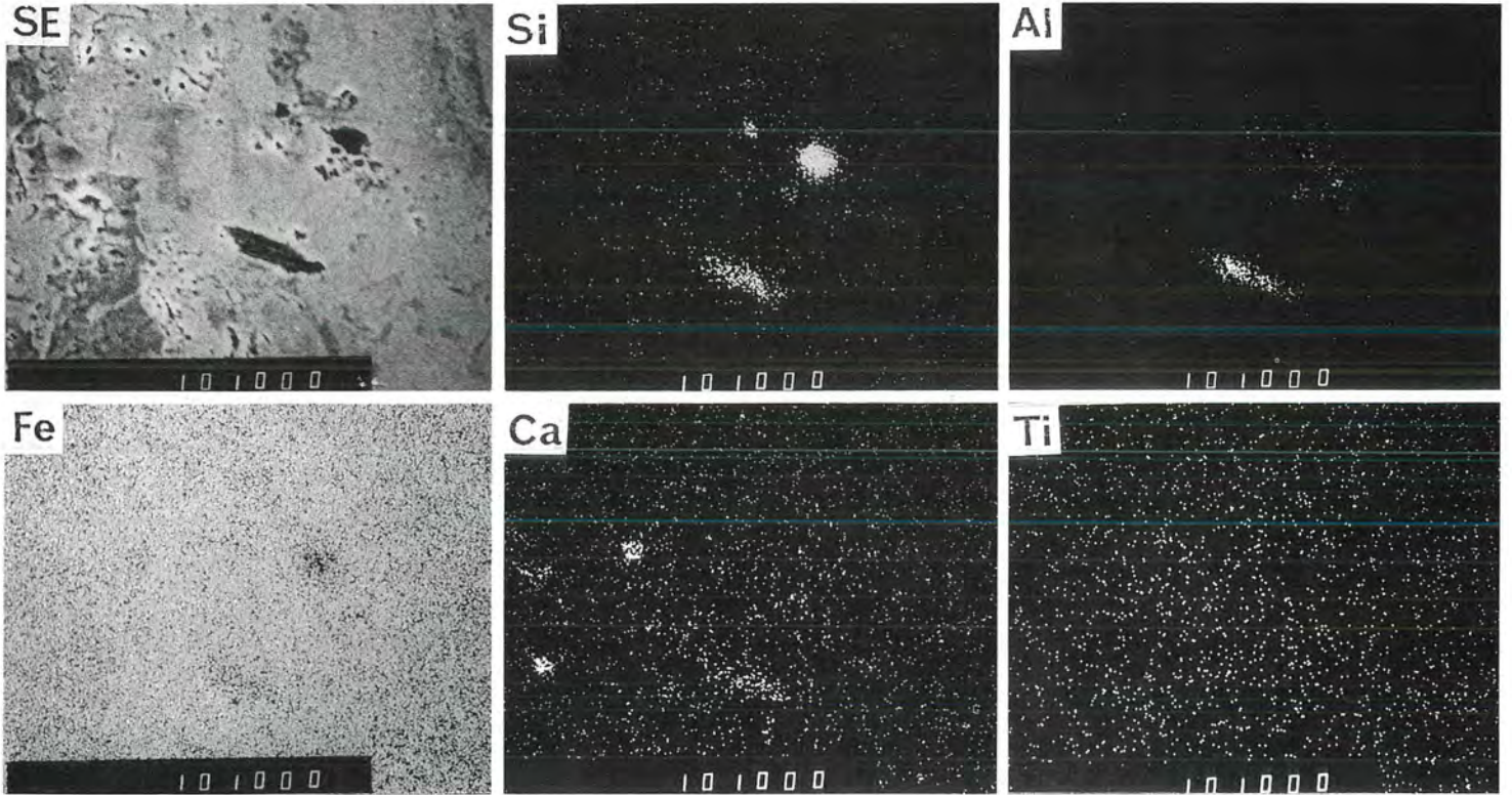
1 ⑩試料中に存在する介在物の元素分布 (EPMA)
