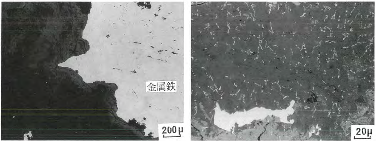
2 ⑬試料の断面組織
