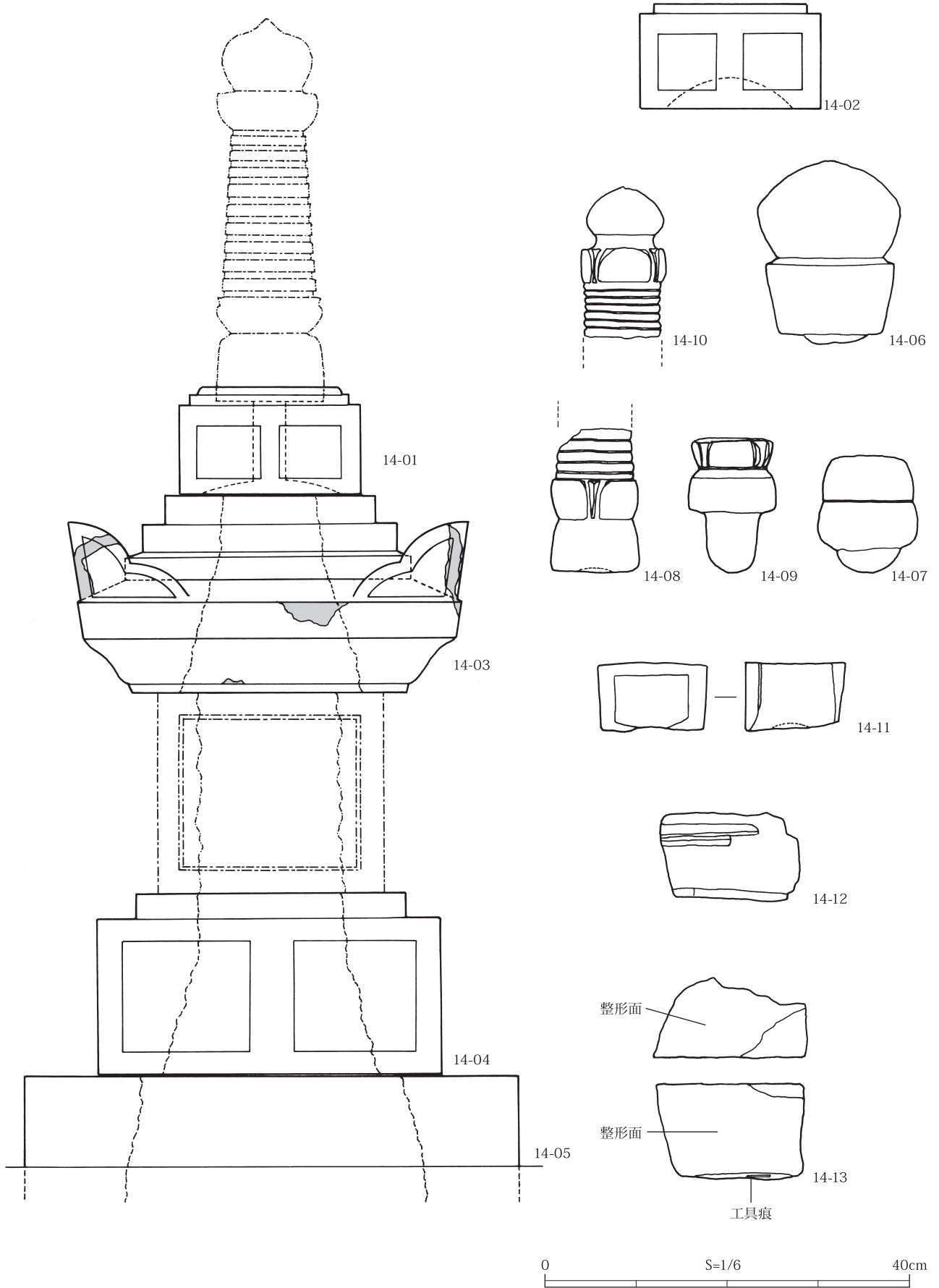
図版 13 石造物実測図・拓本 (13)
