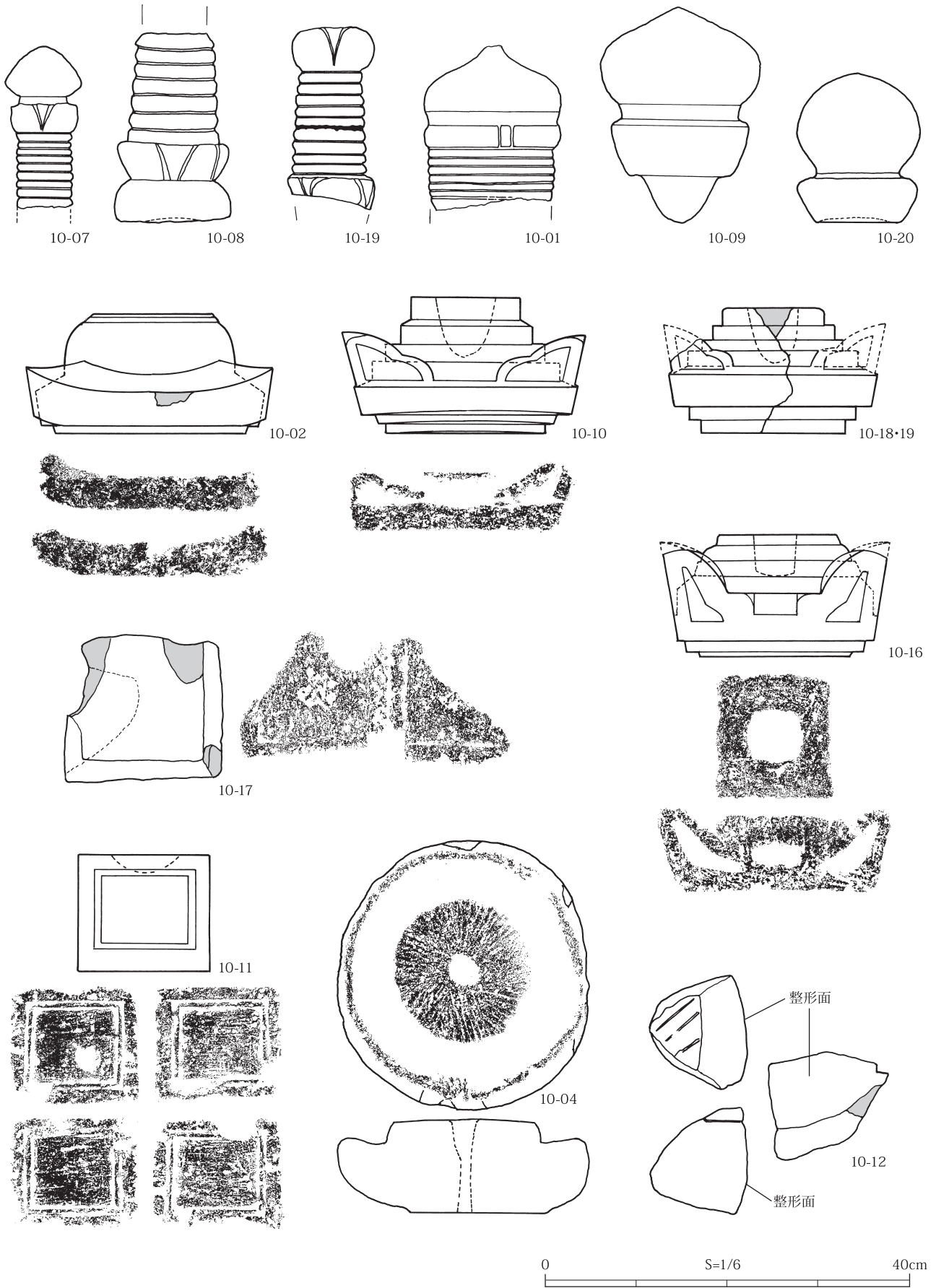
図版 10 石造物実測図・拓本 (10)
