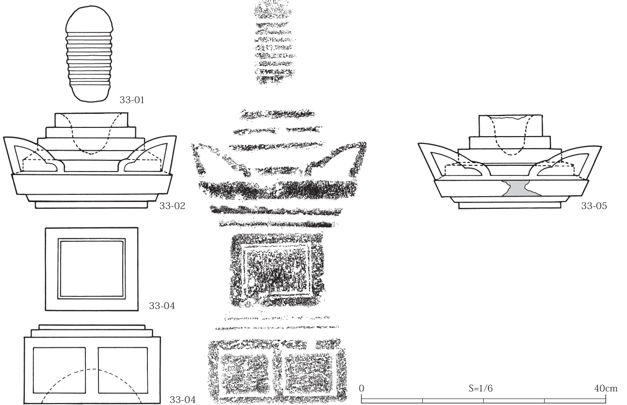
図版 18 石造物実測図・拓本 (18)
