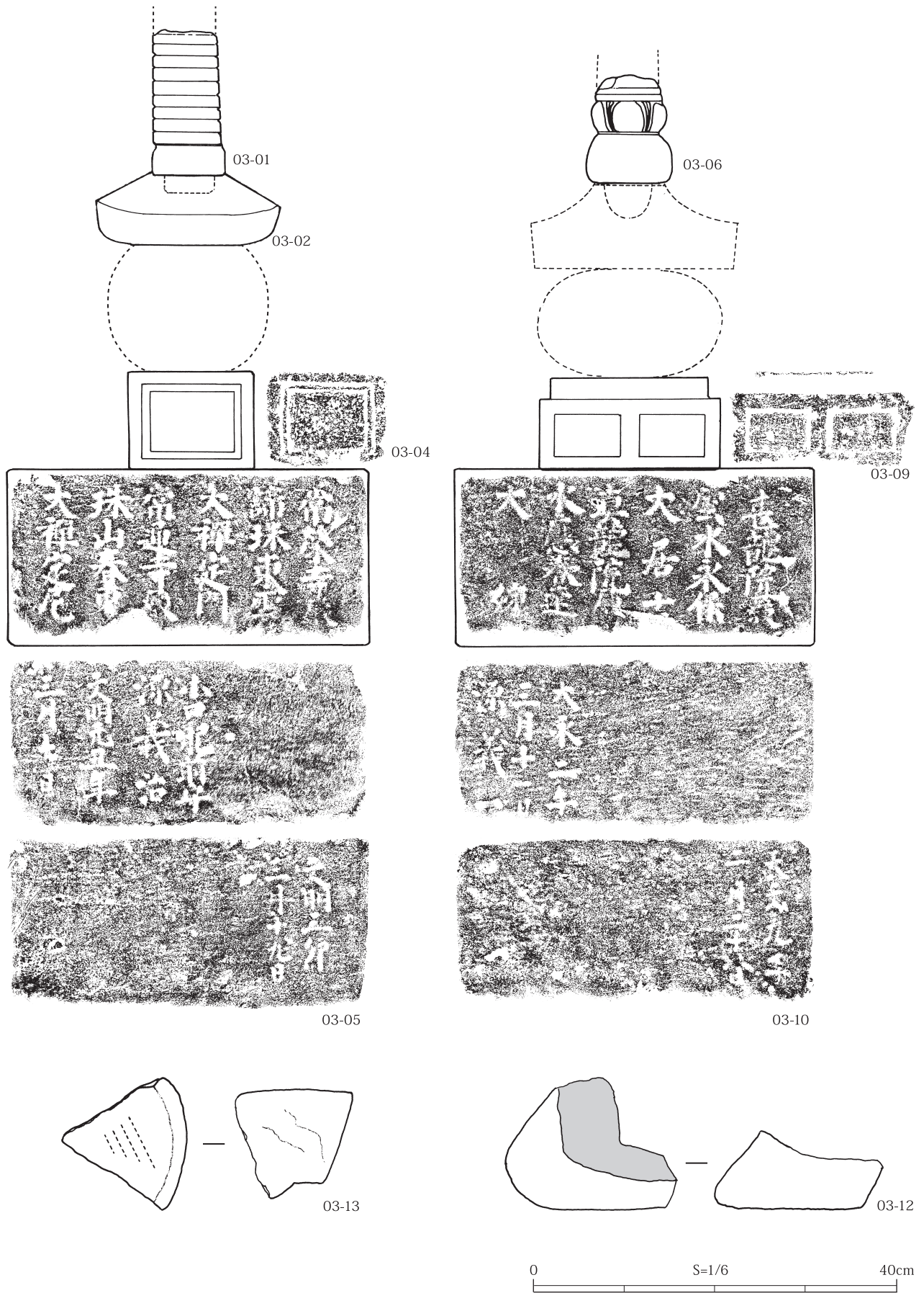
図版4 石造物実測図・拓本(4)
