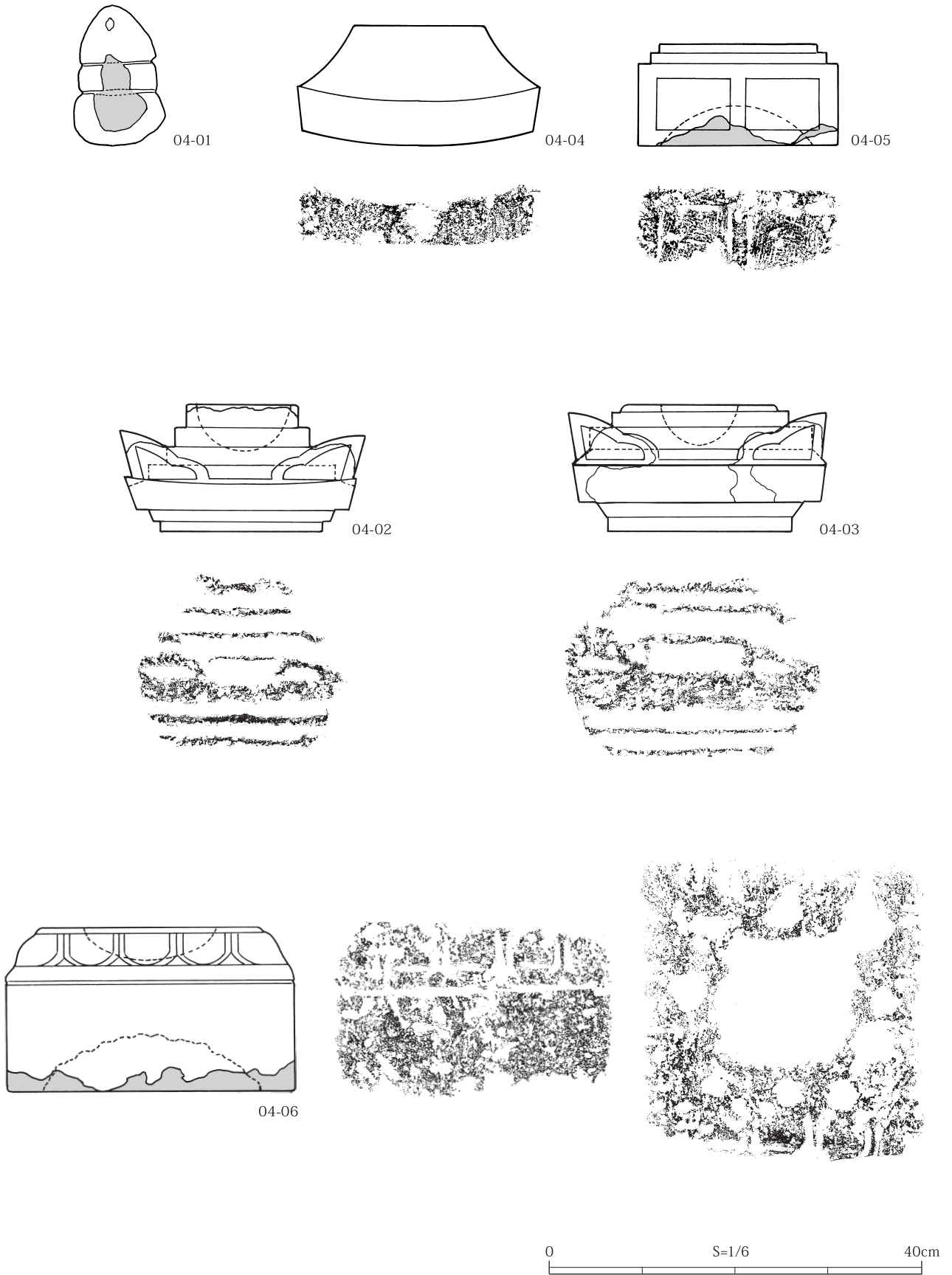
图版 5 石造物実測図・拓本 (5)
