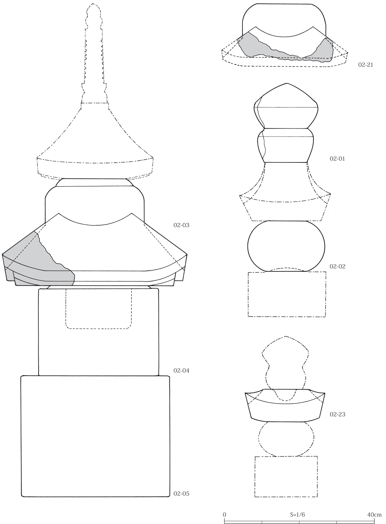
図版2 石造物実測図・拓本(2)
