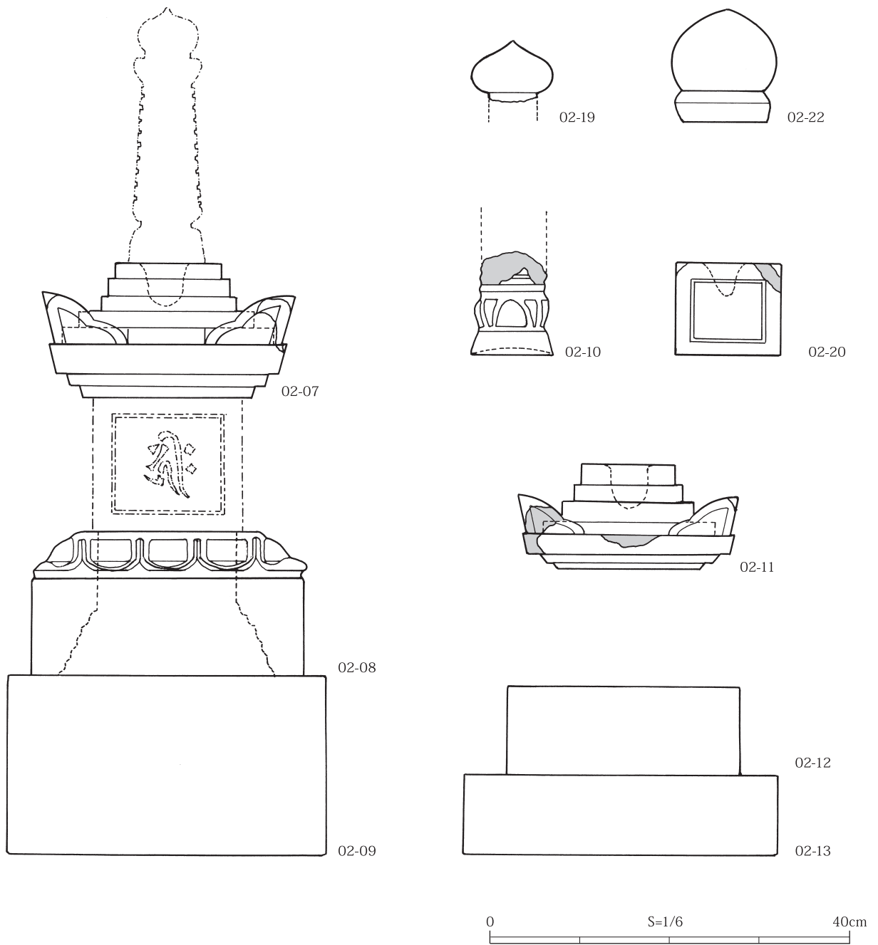
図版3 石造物実測図・拓本(3)
