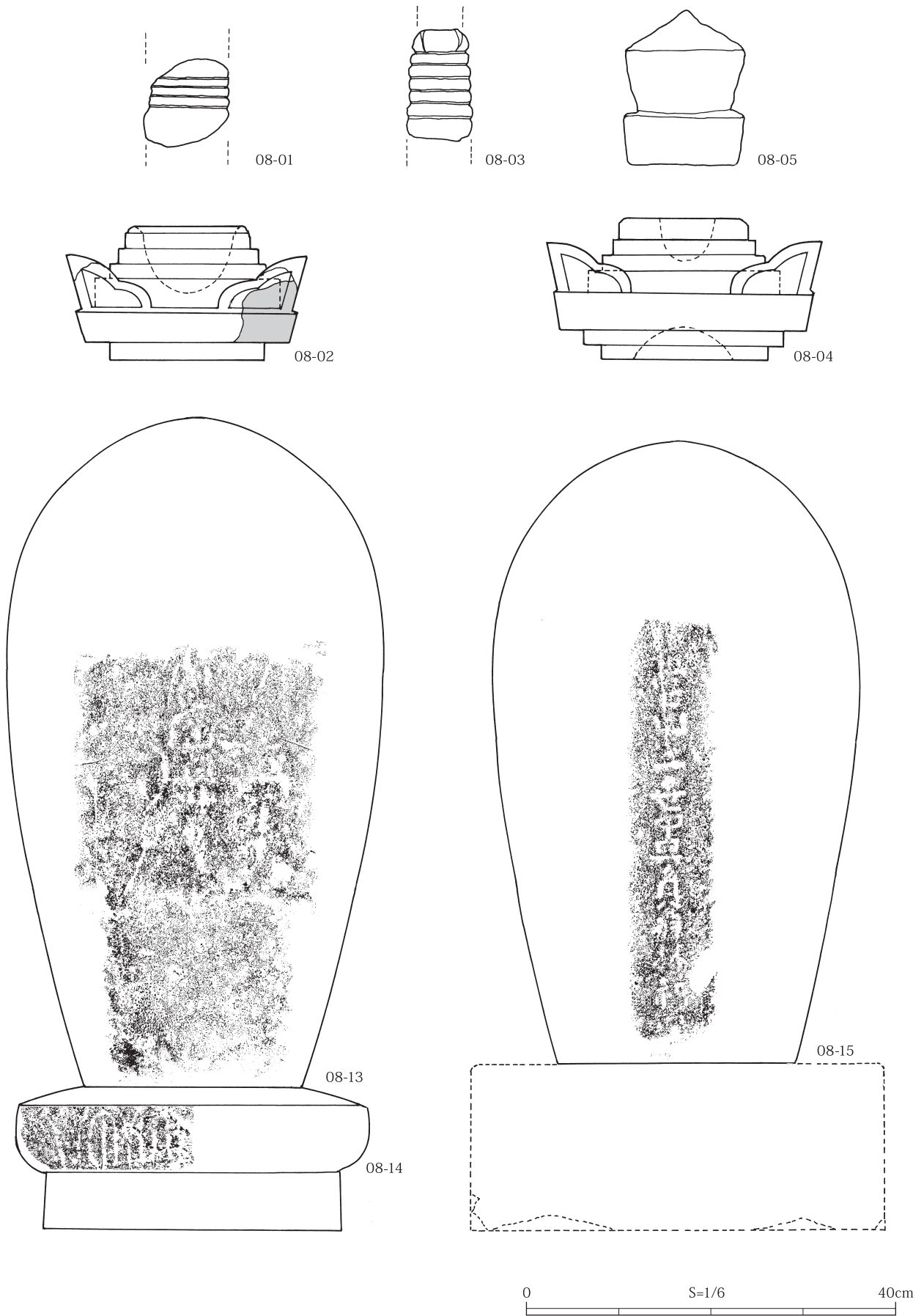
図版8 石造物実測図・拓本（8）
