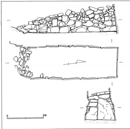
やつおもて 9号墳石室実測図
