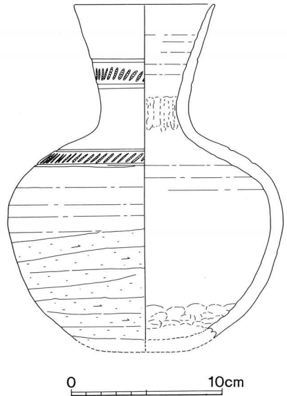
やつおもて 10号墳出土須恵器
