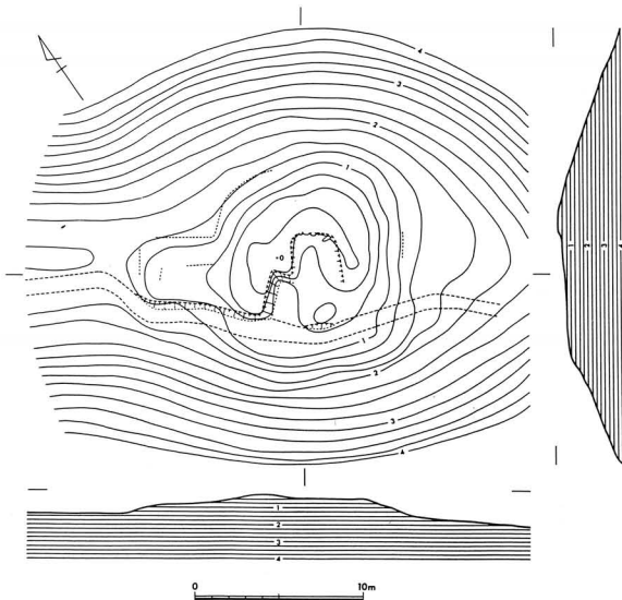
やつおもて 10号墳実測図
