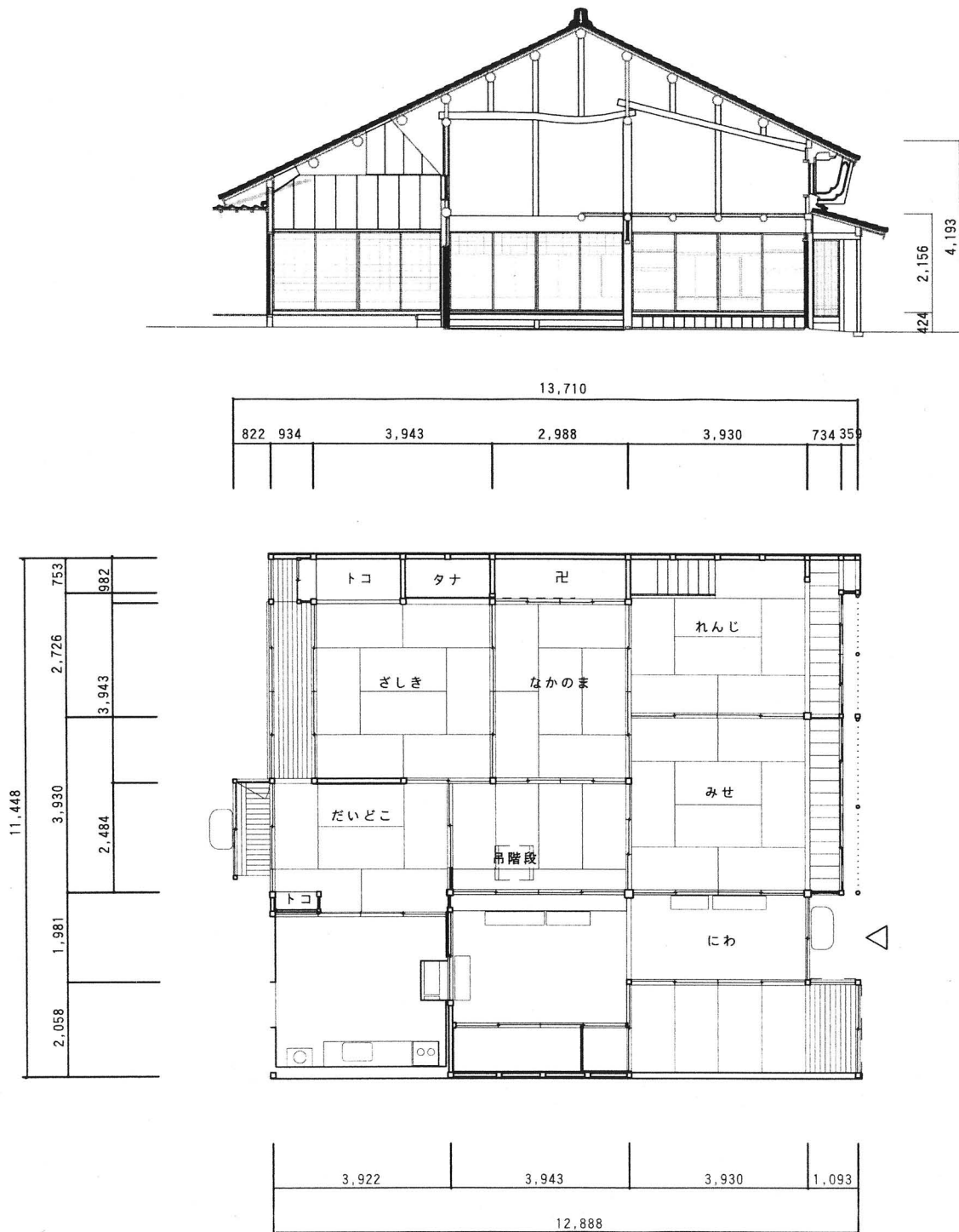
石田家住宅 立面図・平面図
