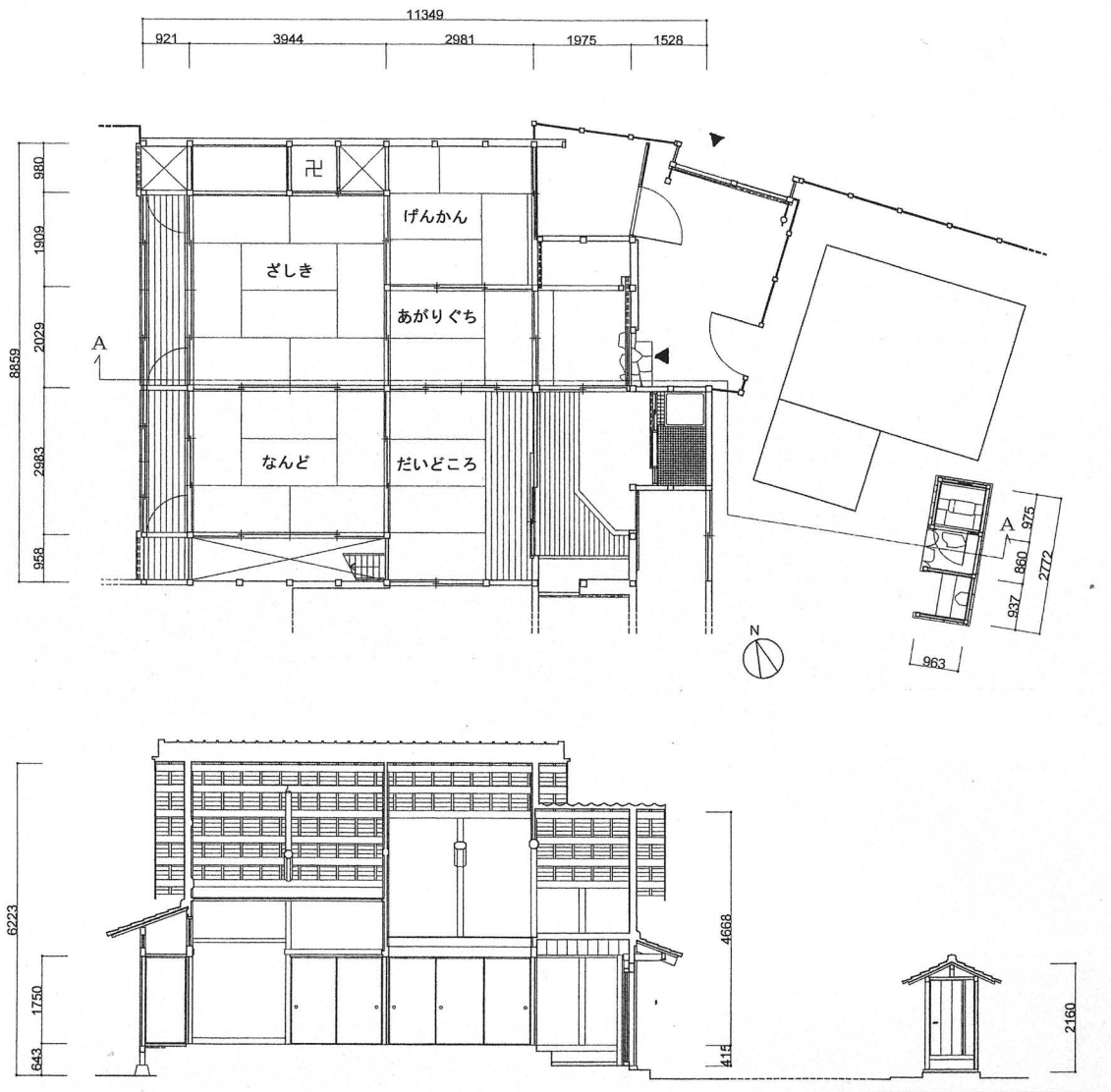
瀧谷家住宅 平面図・立面図
