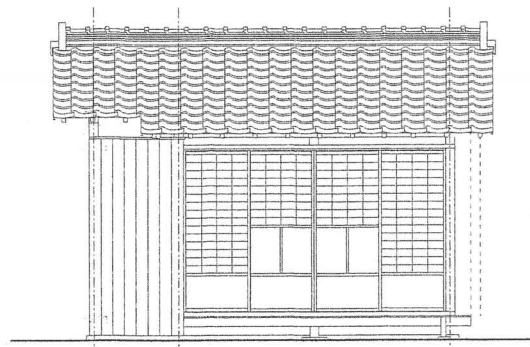
辻番所北側立面図
