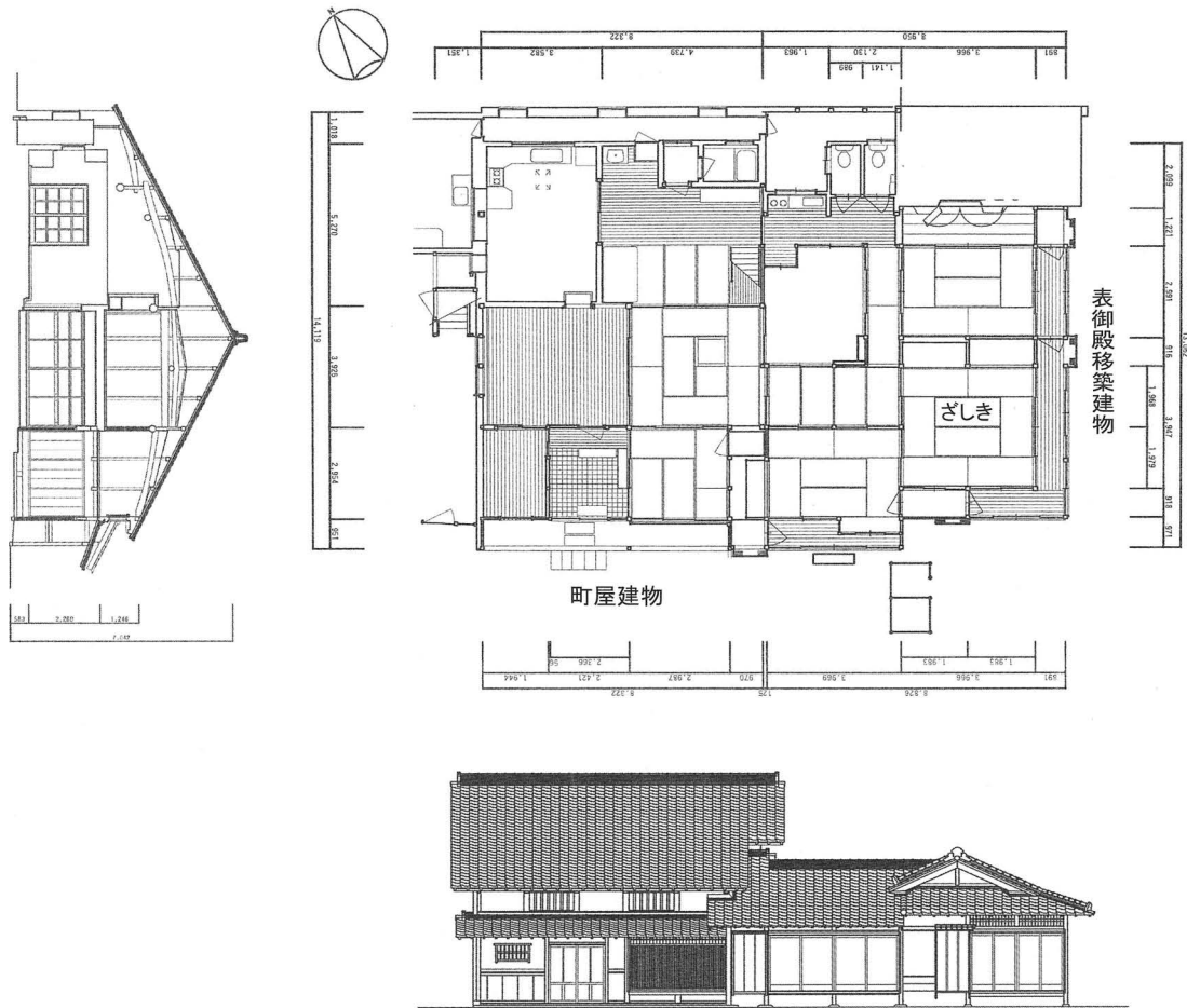
佐々木家住宅平面図・断面図
