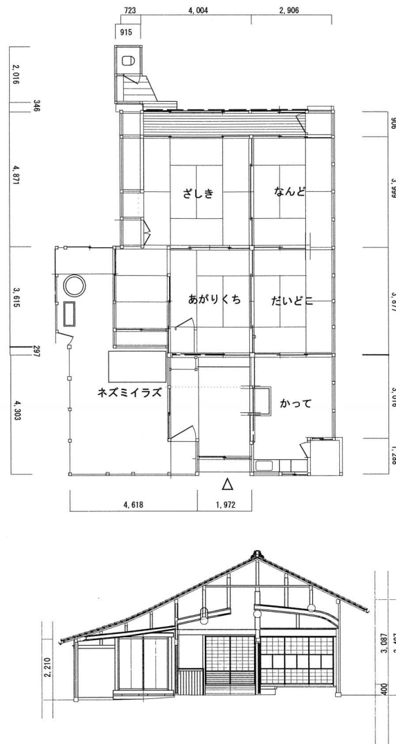
吉居家住宅平面図・断面図
