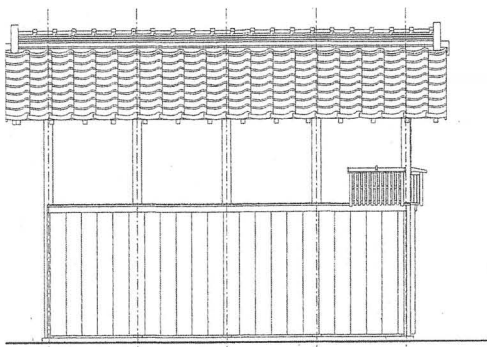
辻番所南側立面図
