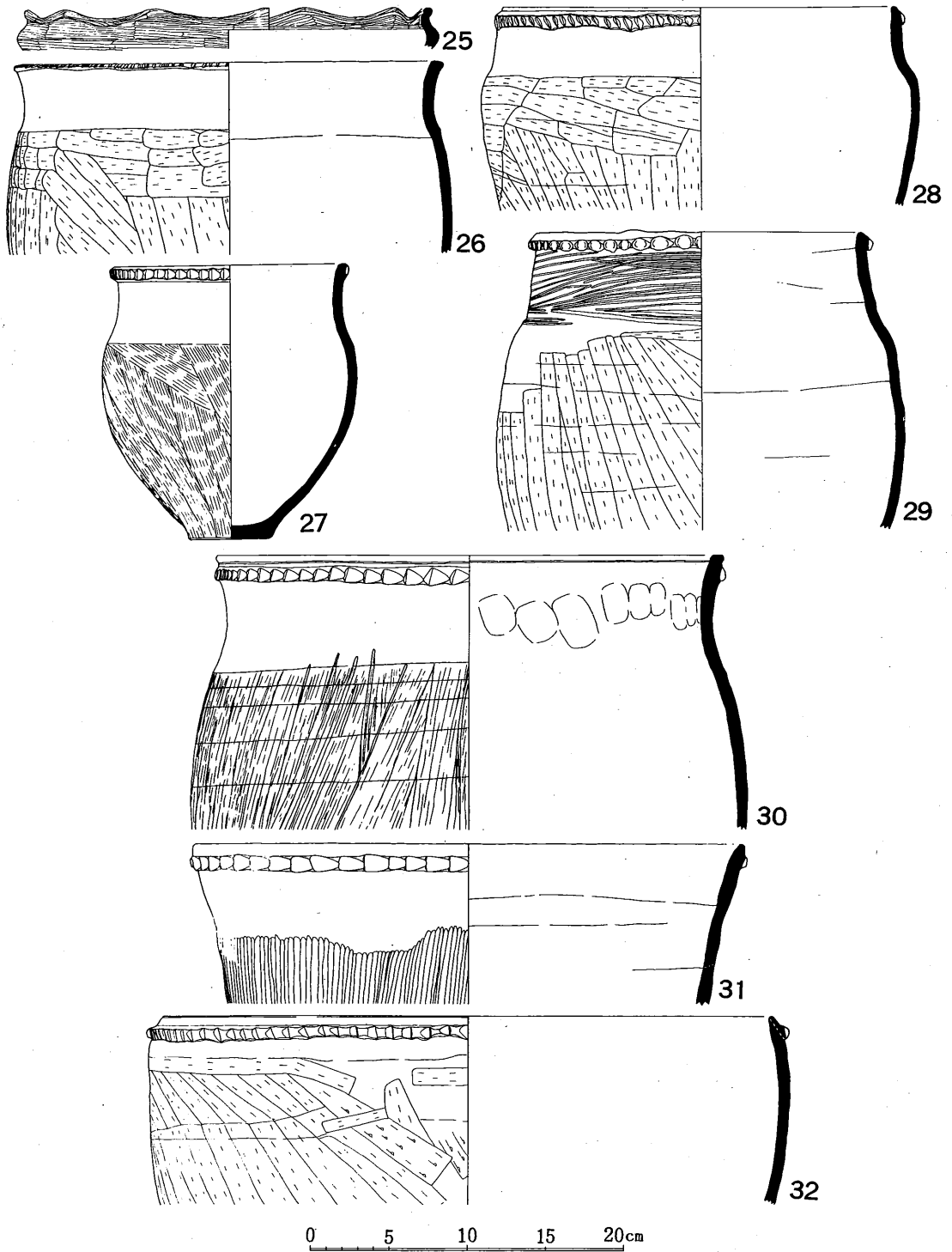
第6圖 出土遺物實測圖
