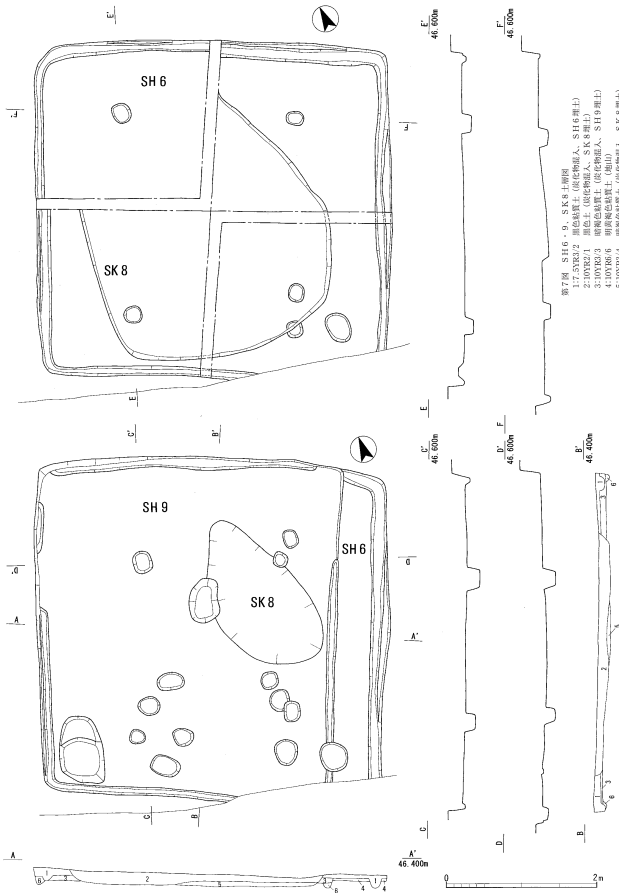
第7圖 SH6・9、SK8実測圖
