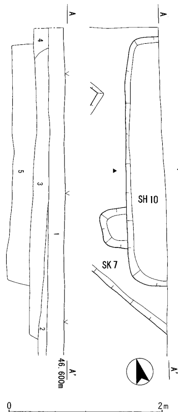
第8図 SH10、SK7実測図 (1:50)
