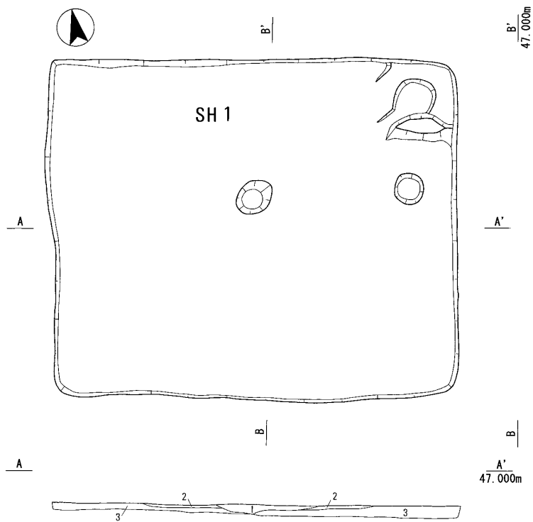
第4図 SH1実測図
