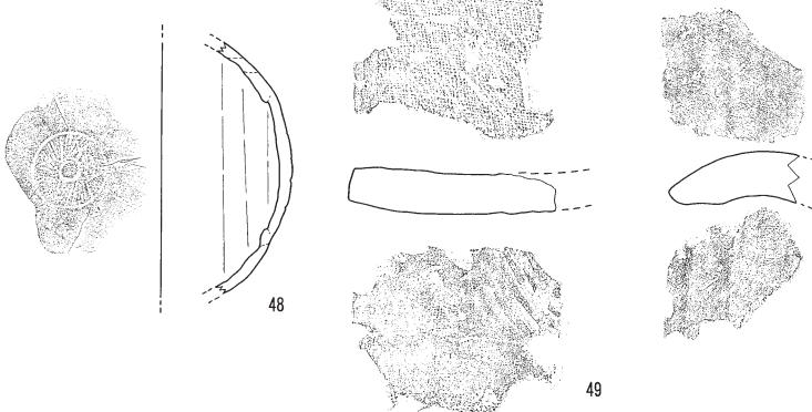
第9図 出土遺物実測図 (1 : 4) (47は 1 : 2)
