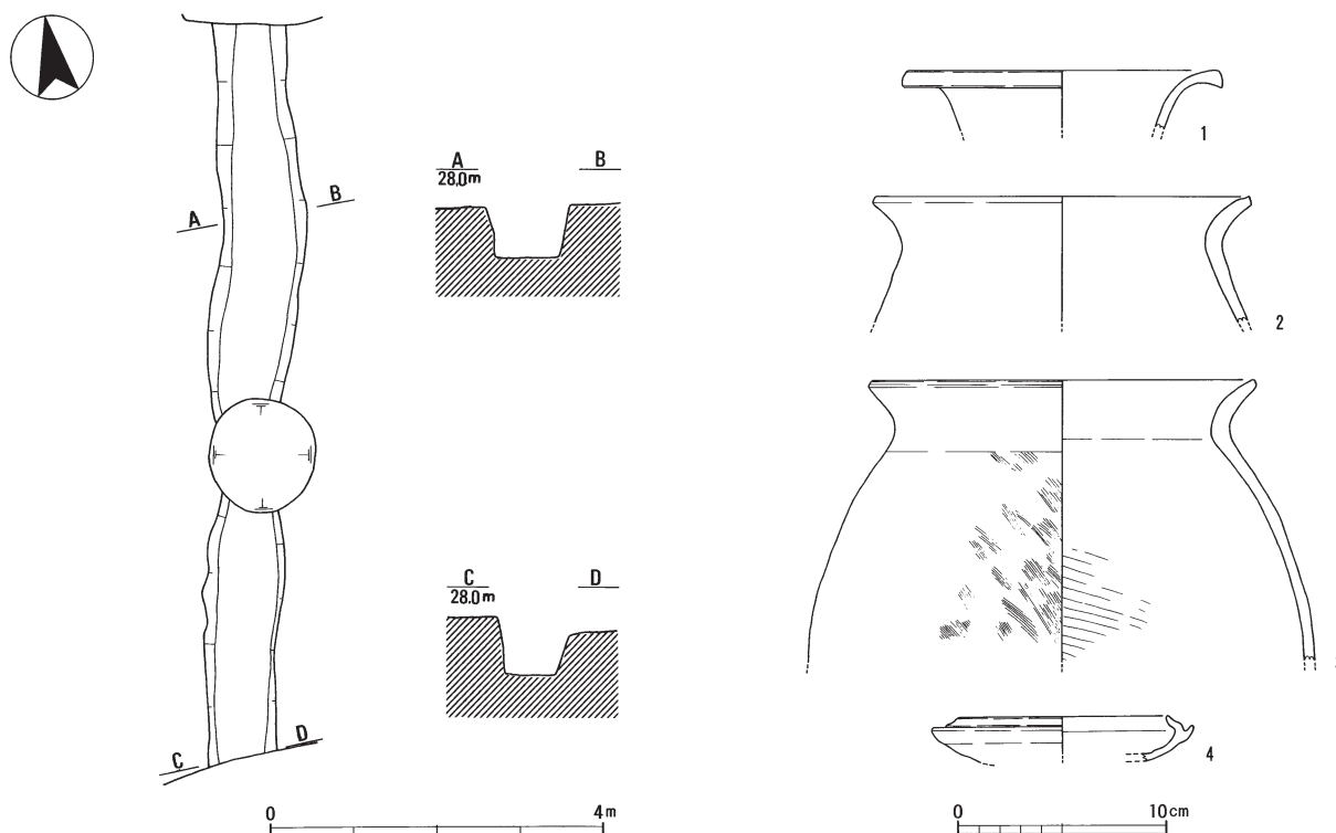
第7図 S D 1平面図・断面図(1:100)及び出土遺物実測図(1:4)
