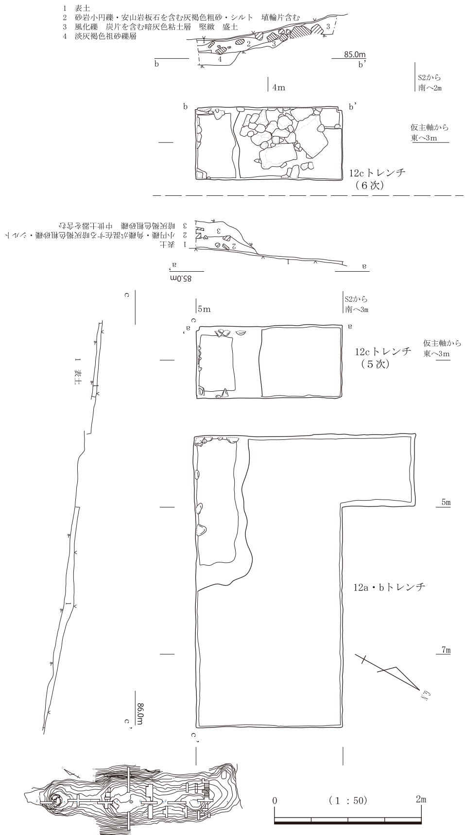
図3-21 12トレンチ平・断面図
