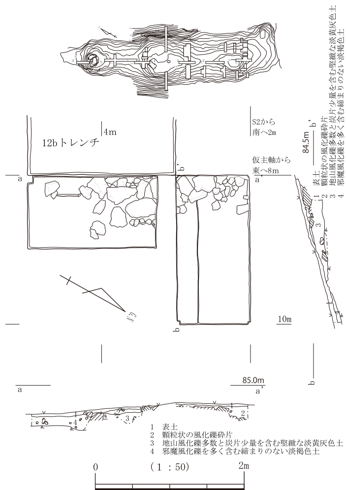
図3-28 19トレンチ平・断面図
