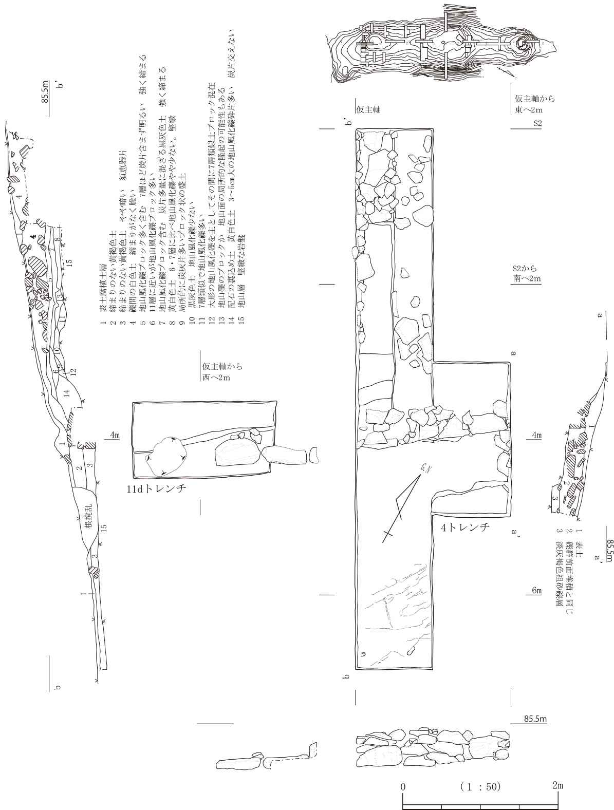
図3-20 4トレンチ平・断面図
