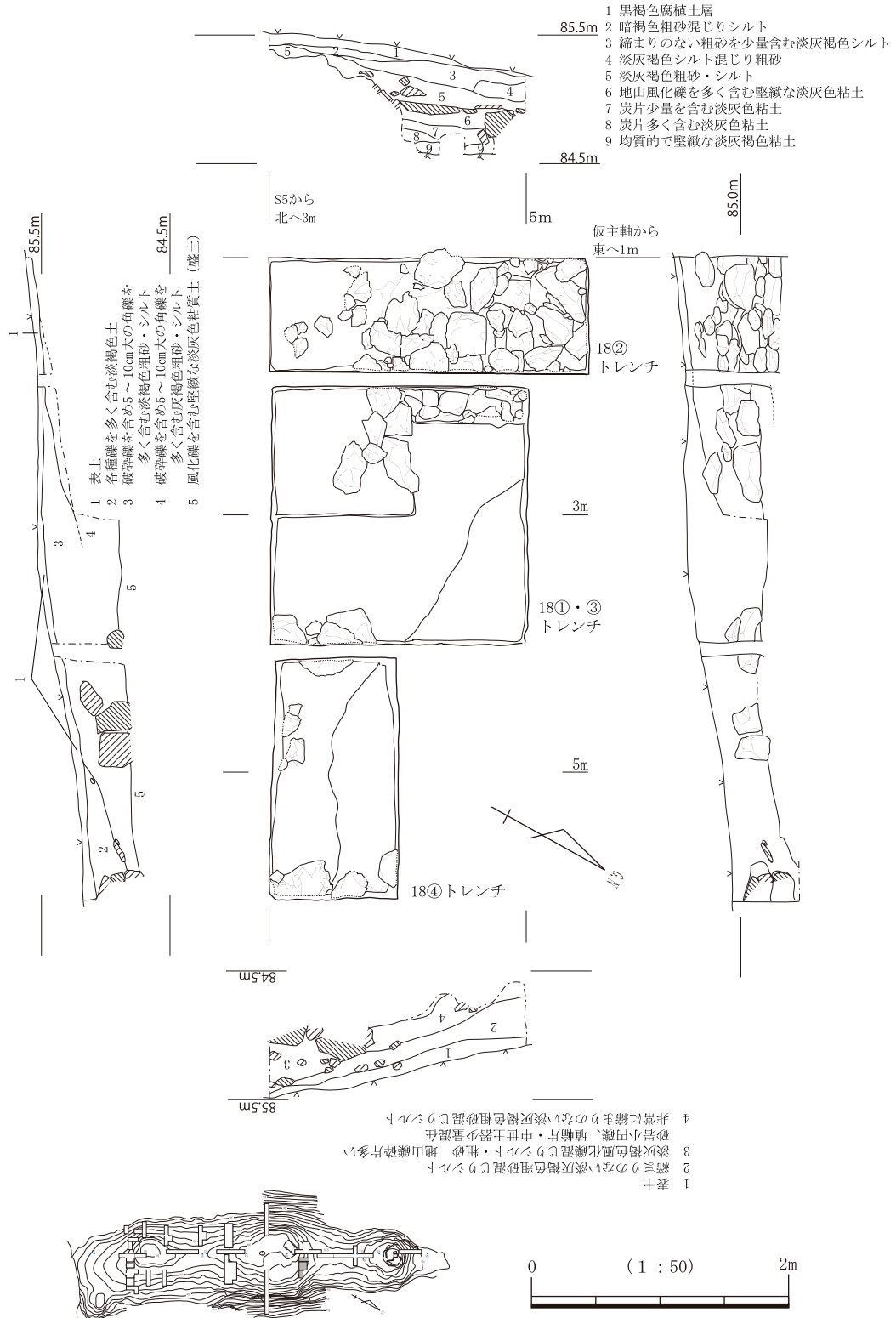
図3-5 18トレンチ平・断面図
