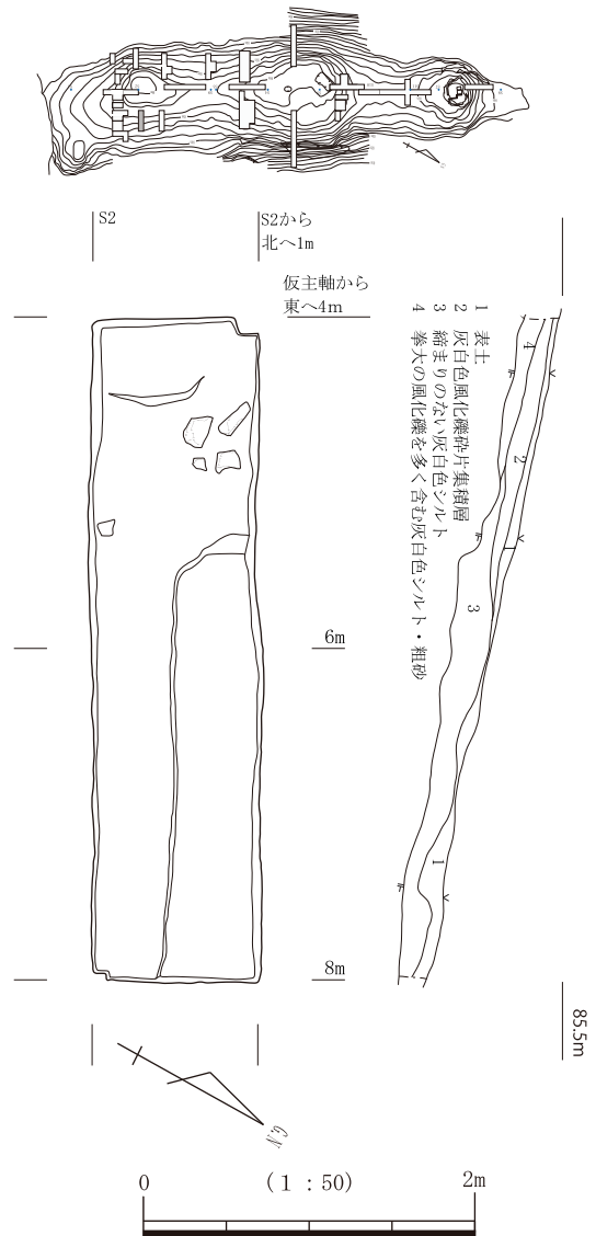
図3-29 13トレンチ平・断面図
