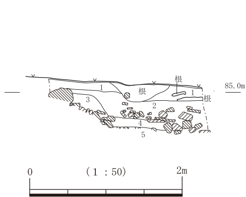
土層図3
