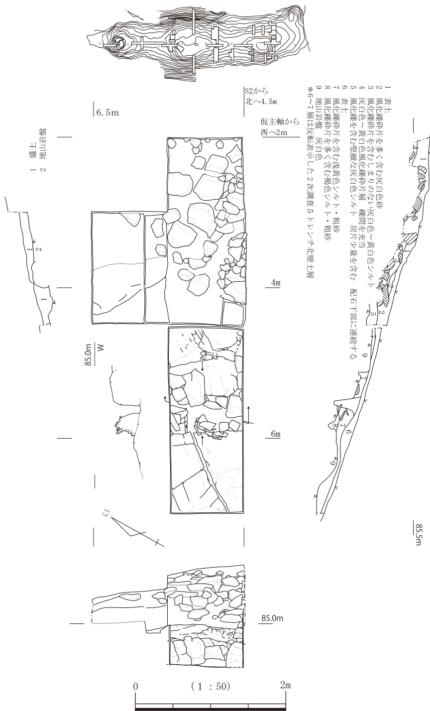
図3-25 5トレンチ平・断面図
