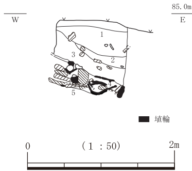
土層図2
