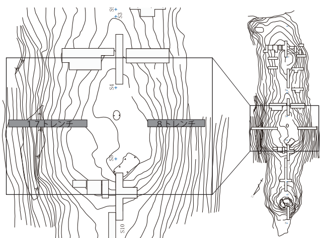
図3-6 後円部側面トレンチ配置
