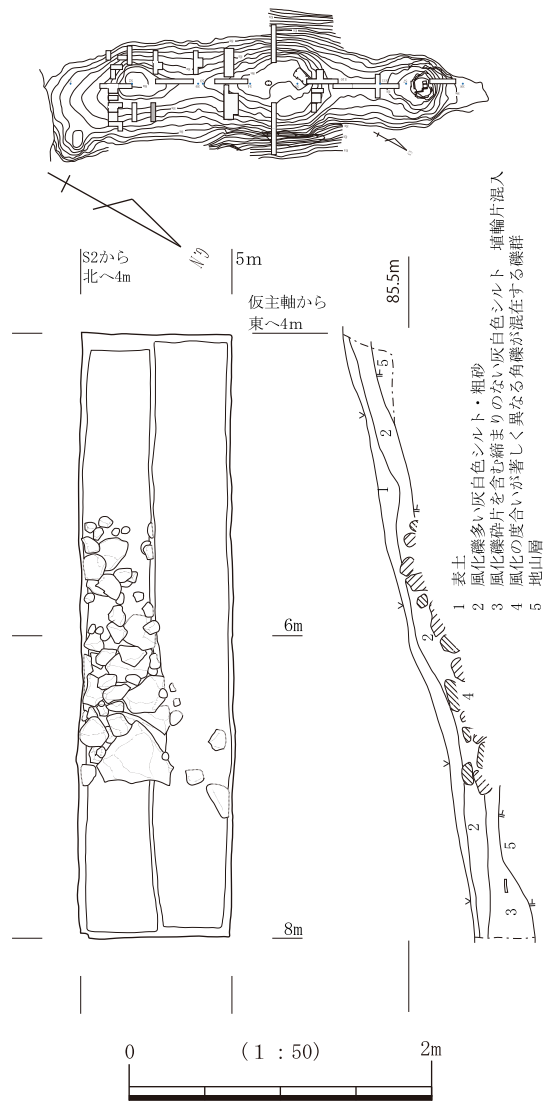
図3-30 14トレンチ平・断面図
