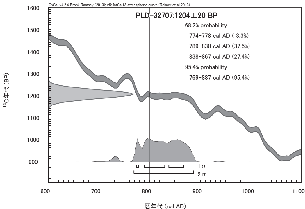
第19図 暦年較正結果
