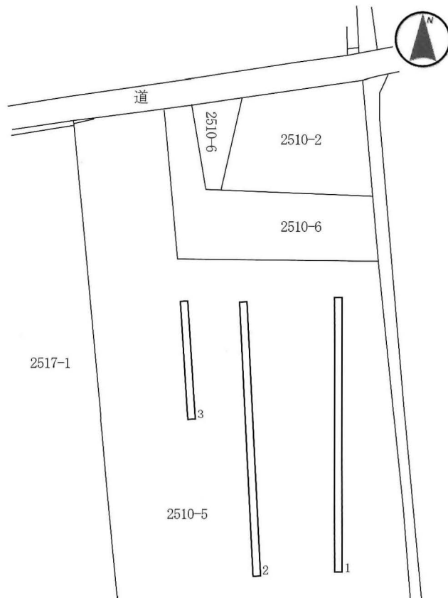
トレンチ設定図 1:1,000
