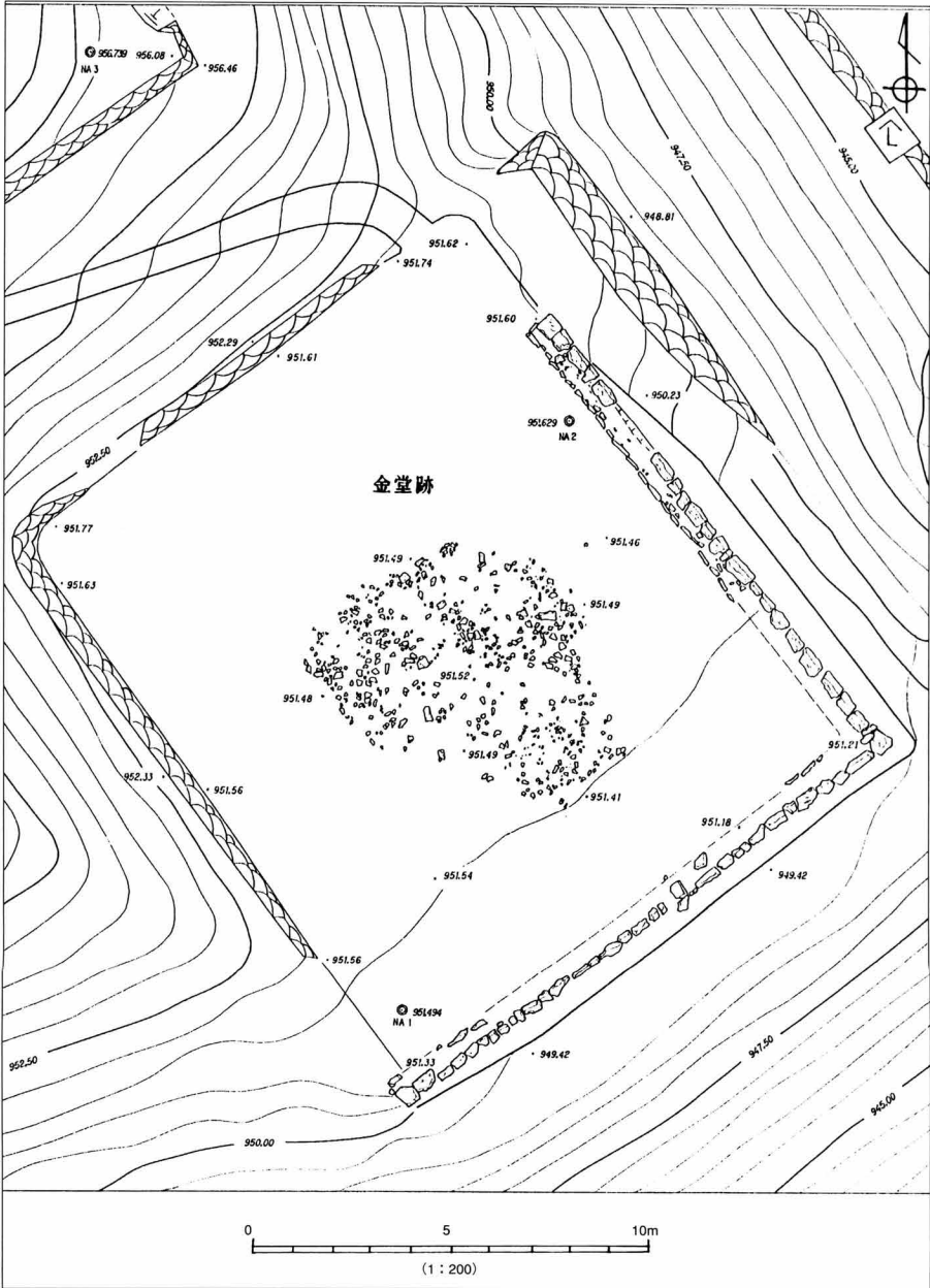
第3図 金堂面全体図
