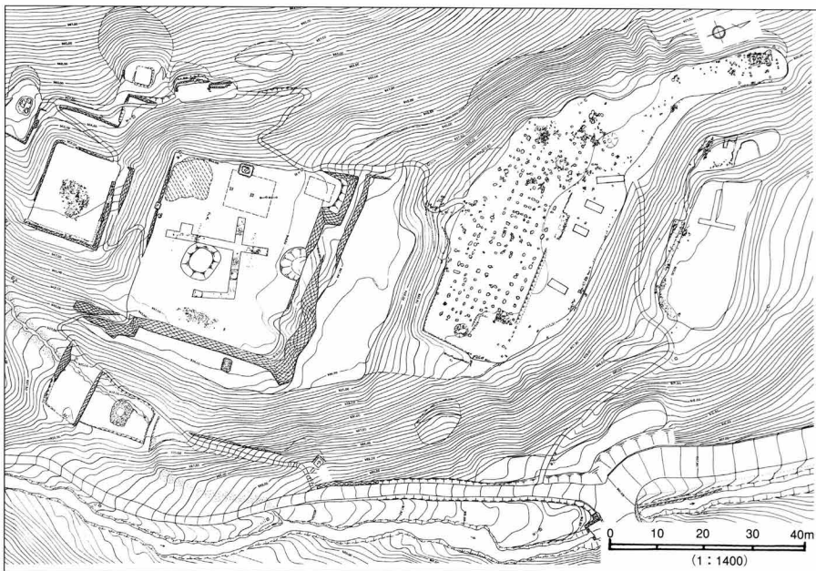
第2図 若澤寺跡全体図
