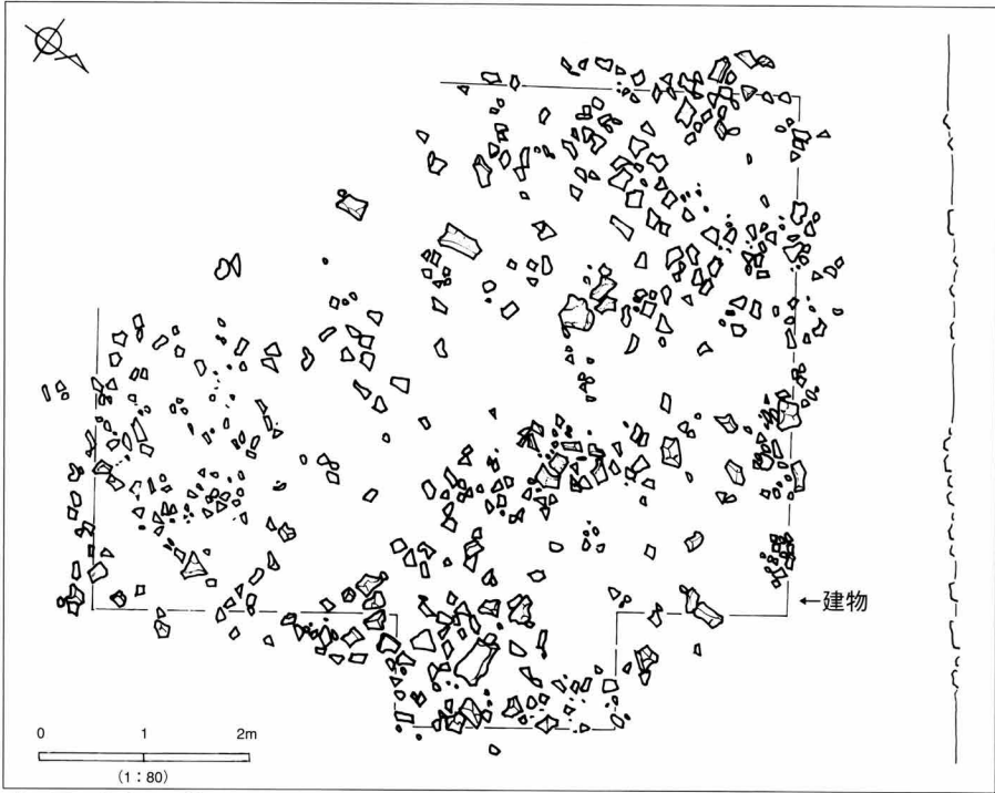
第4図 金堂面の集石図
