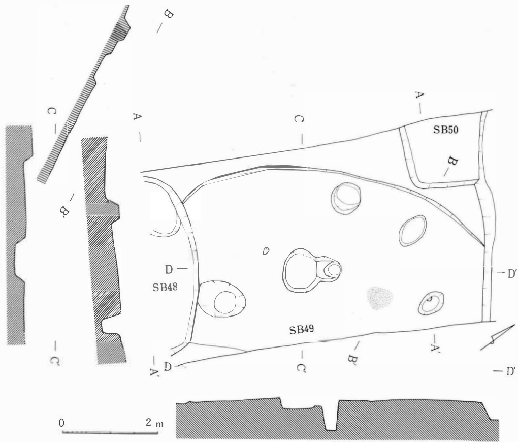
III-179 49号住居址実測図
