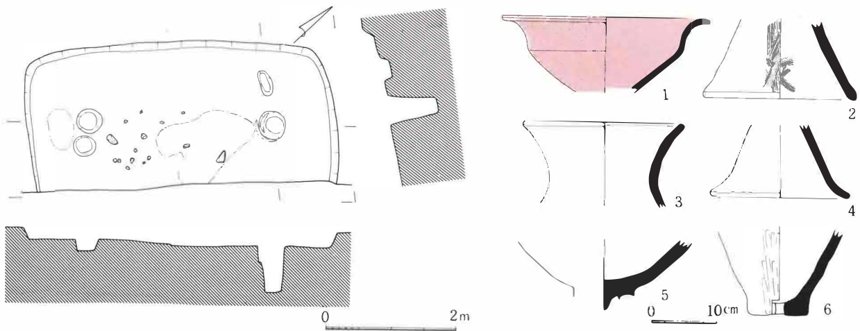
III-227 31号住居址実測図・出土土器
