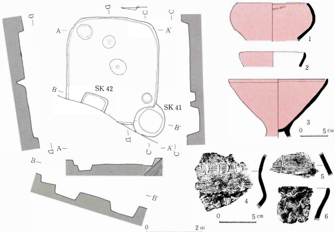
III-272 91号住居址実測図・出土土器
