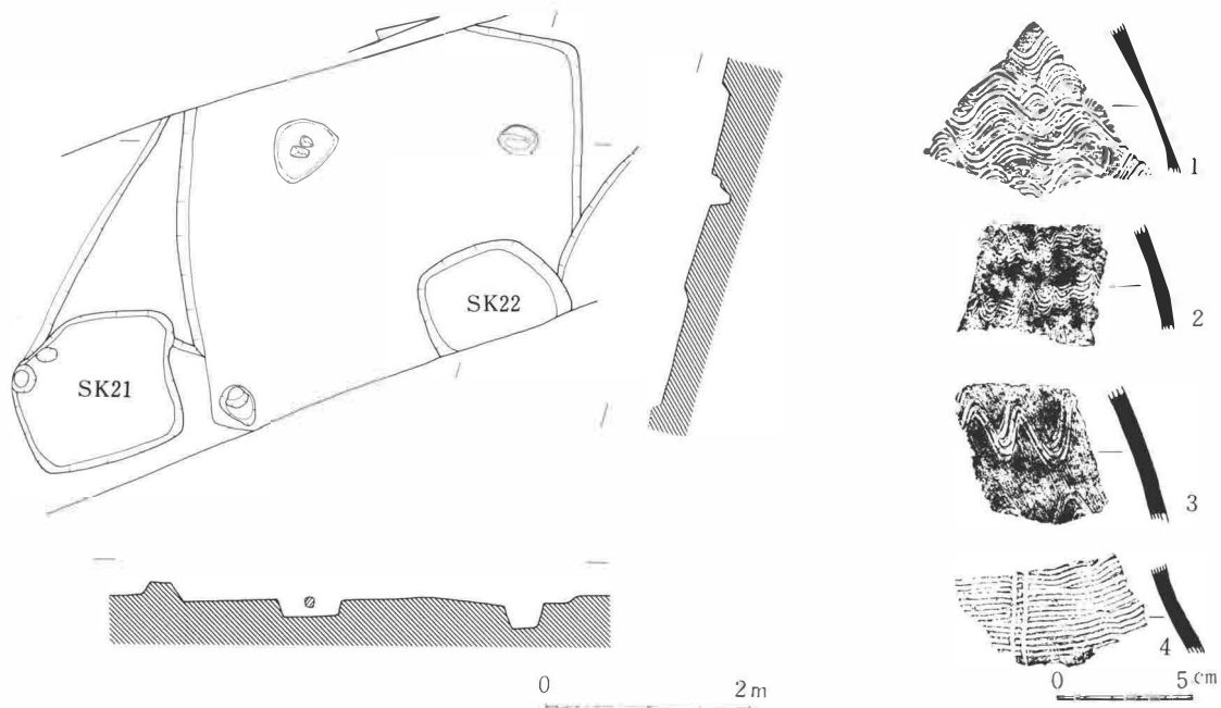
III-255 64号住居址実測図・出土土器
