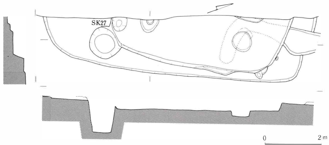
III-257 71号・72号住居址実測図
