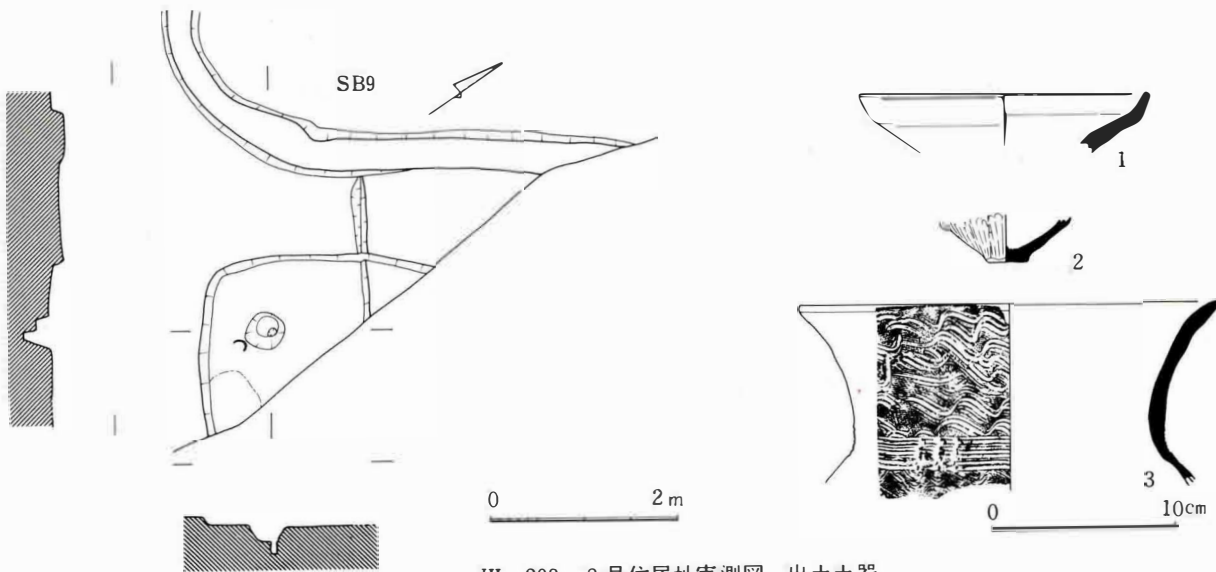
III-203 8号住居址実測図, 出土土器
