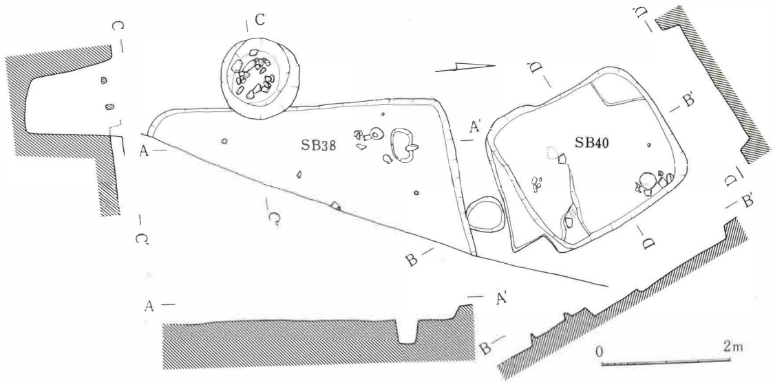
III-235 38号·40号住居址实测图
