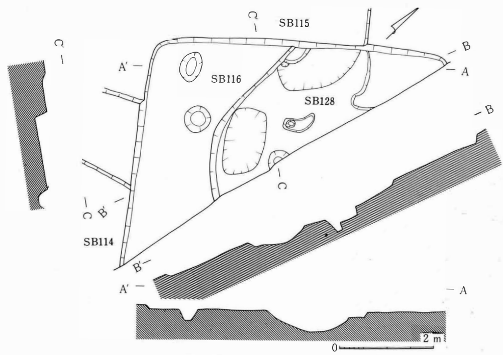
III-182 128号住居址実測図
