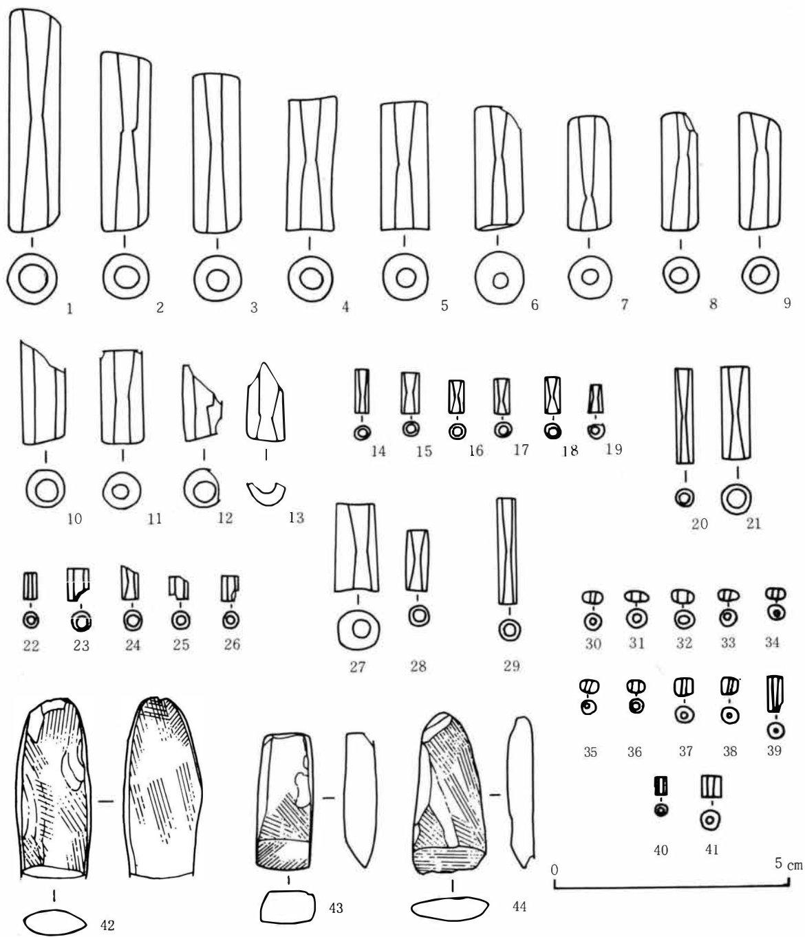
III-166 玉類(1~41), 小形片刃石斧(42~44)
