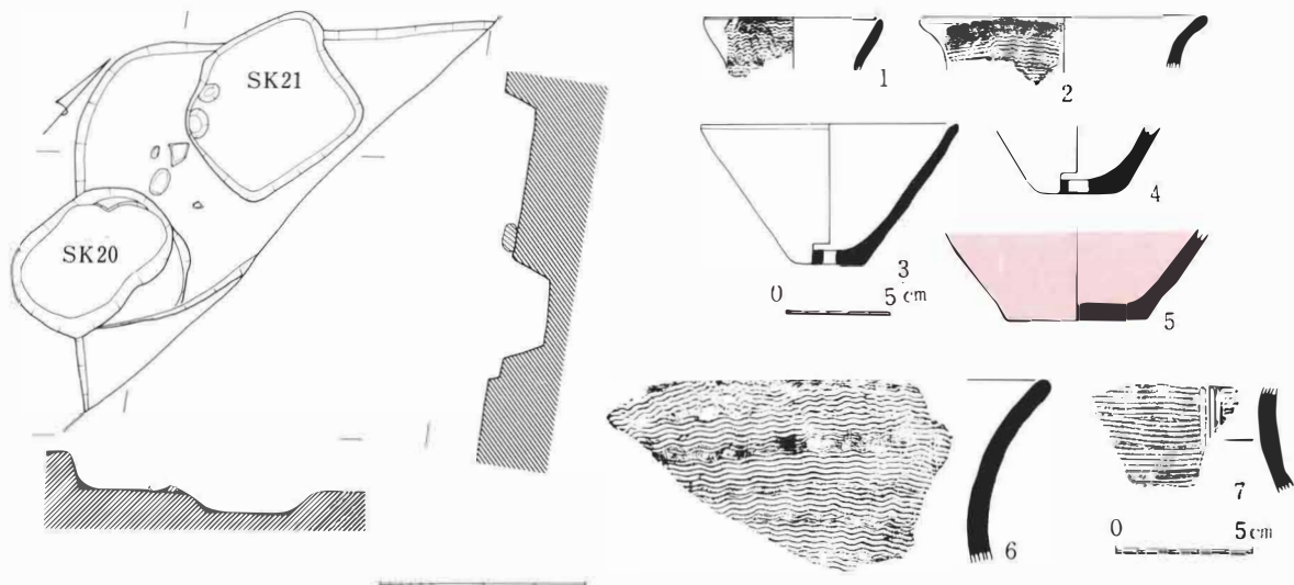
III-254 63号住居址実測図・出土土器
