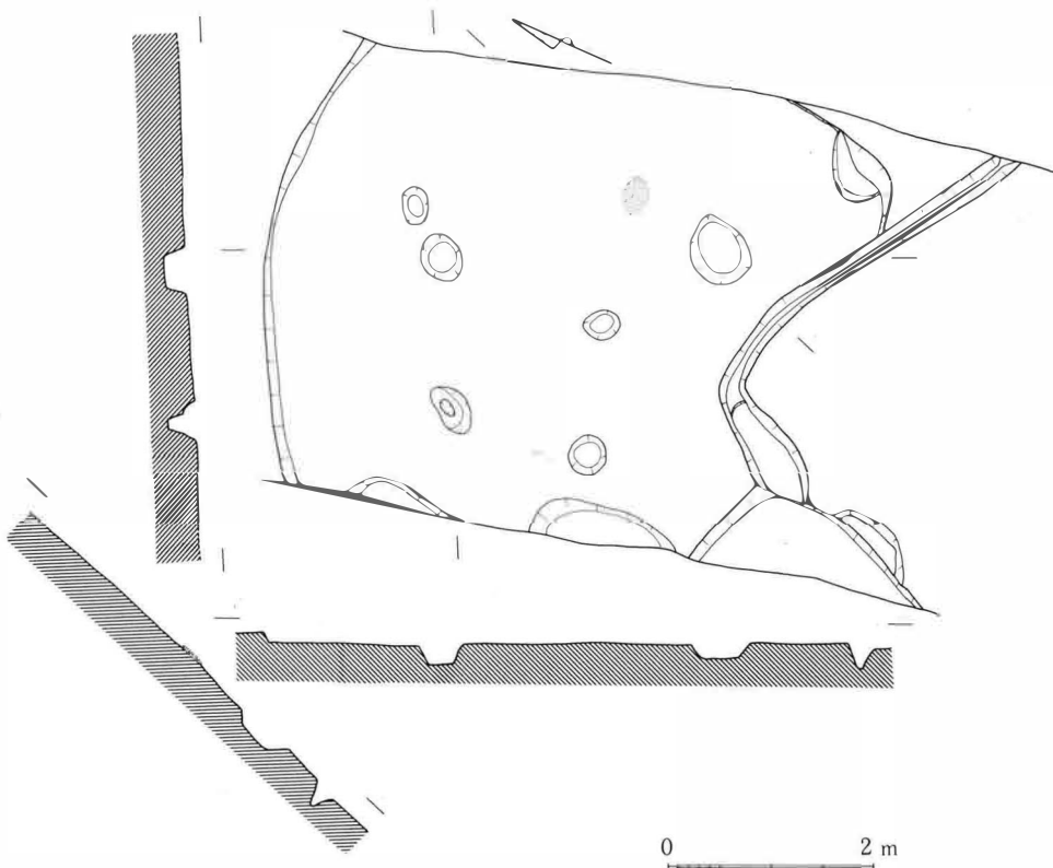
III-199 7号住居址実測図
