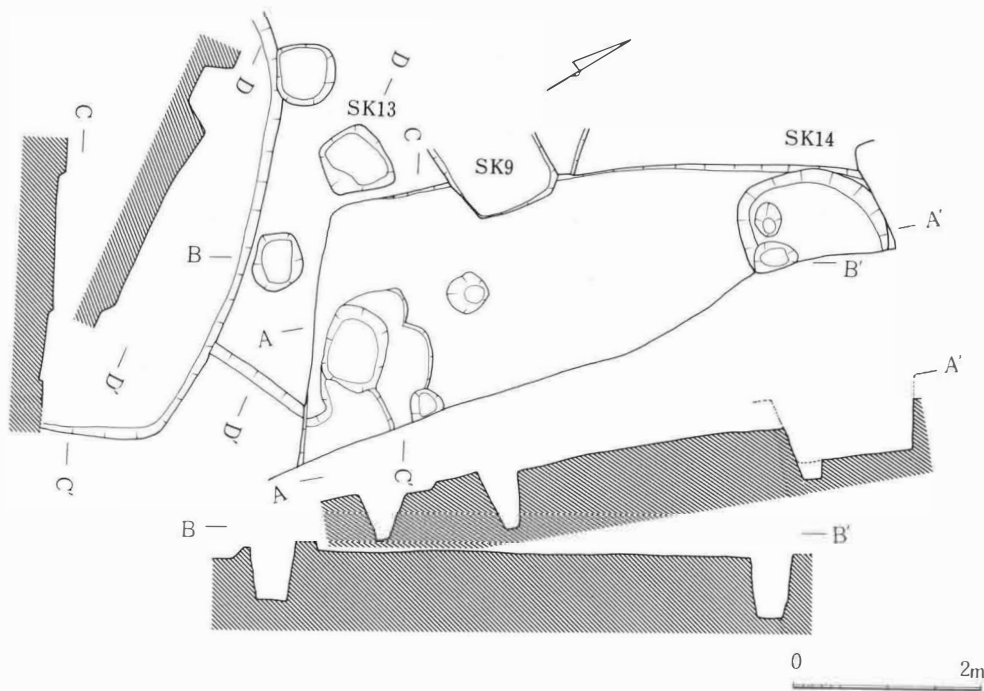
III-218 21号住居址, 土壇13・14実測図
