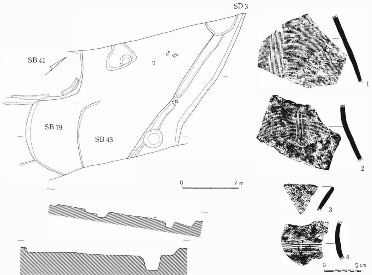
III-265 79号住居址実測図・出土土器
