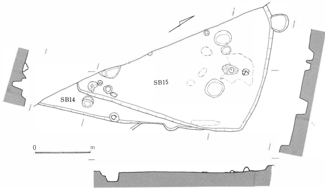
III-210 14号・15号住居址実測図
