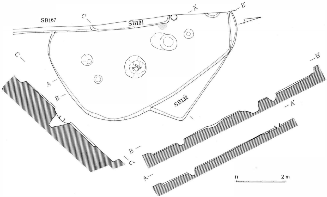
III-172 109号・131号・132号住居址実測図
