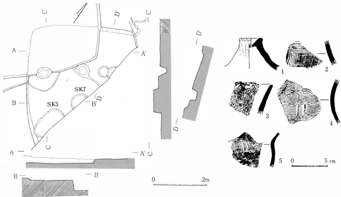
III-224 27号住居址実測図・出土土器
