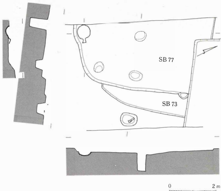
III-260 73号・77号住居址実測図
