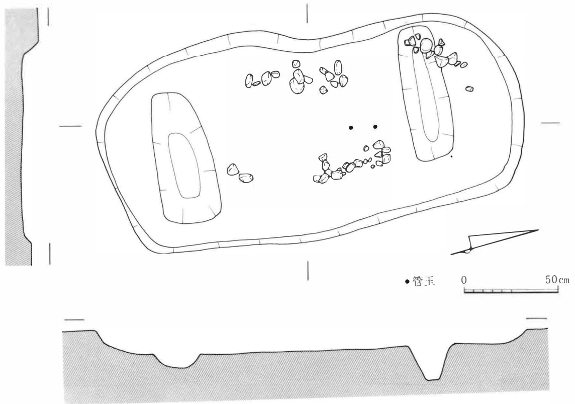
III-139 15号木棺墓実測図
