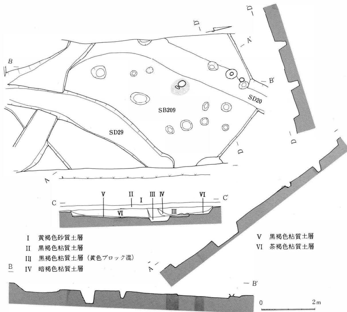
III-187 209号住居址, 29号溝址実測図
