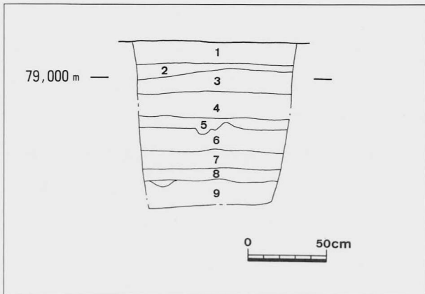
第14図 調査区1 南壁土層図
