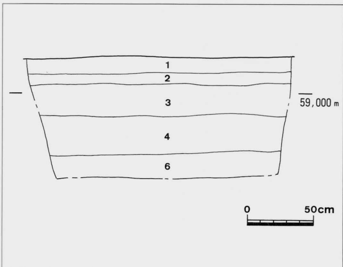
第10図 調査区2 西壁土層図
