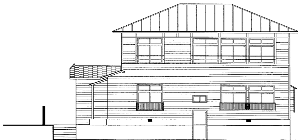
南立面图 S=1:100×0.7
