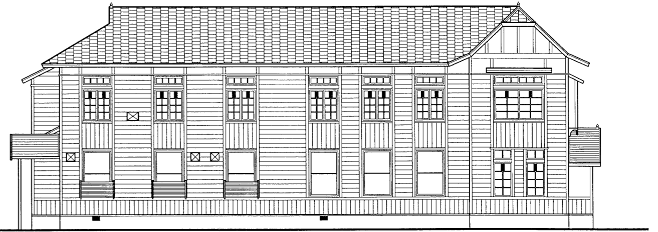
南立面图 S=1:100×0.7
