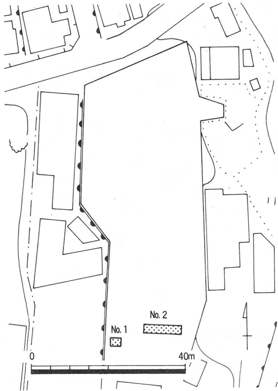
第21図 トレンチ位置図 (TRK 88-3)
