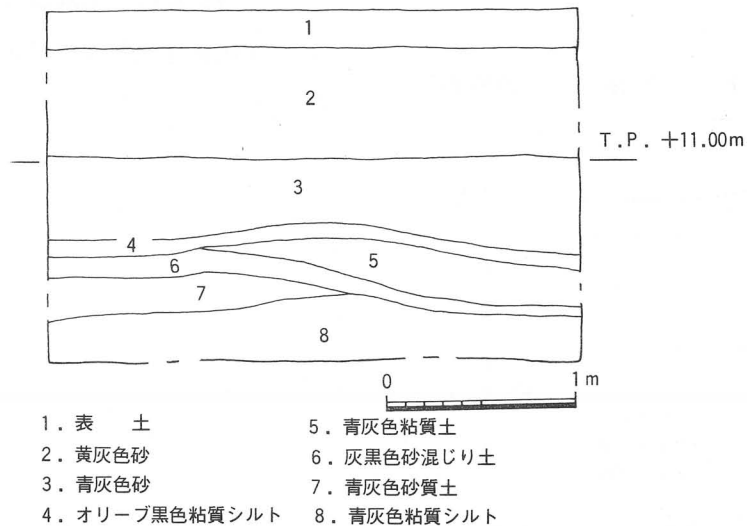
第20図 東壁土層断面図 (TRK 88-2)
