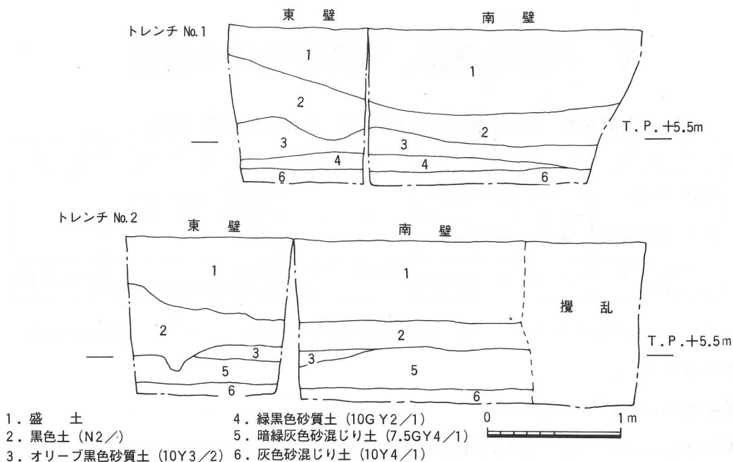
第11図 土層断面図 (K SM88-4)
