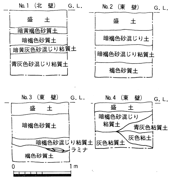
第3図 土層断面図 (NGT88-2)
