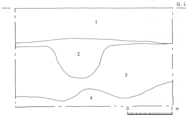
第6図 東壁土層断面図 (NGT88-5)
