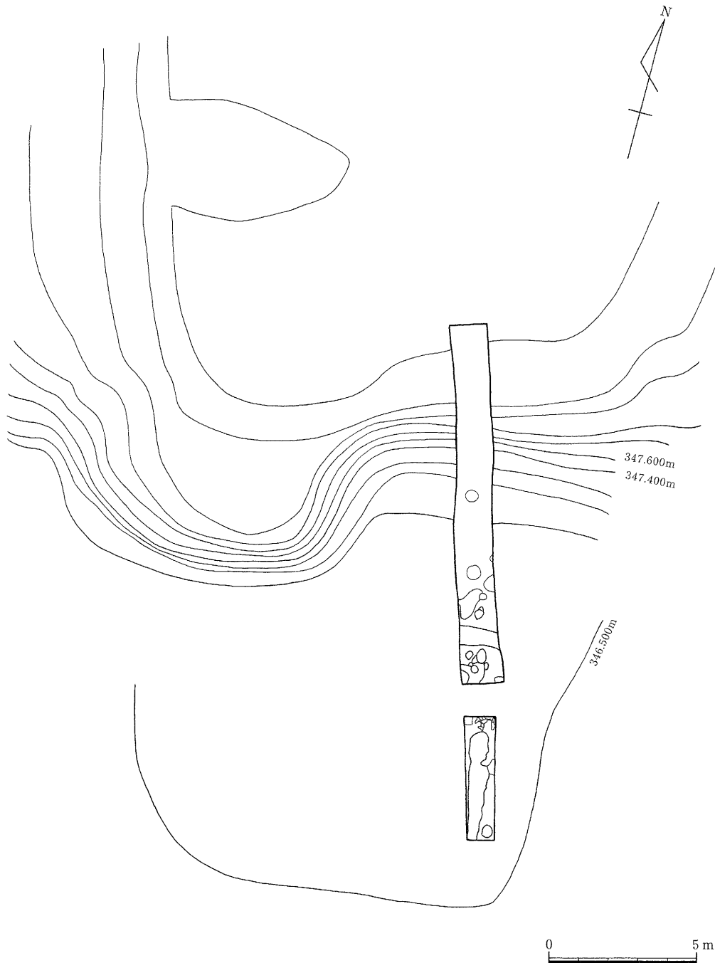
第11図 平成18・19年度調査区周辺図 (1/180)
