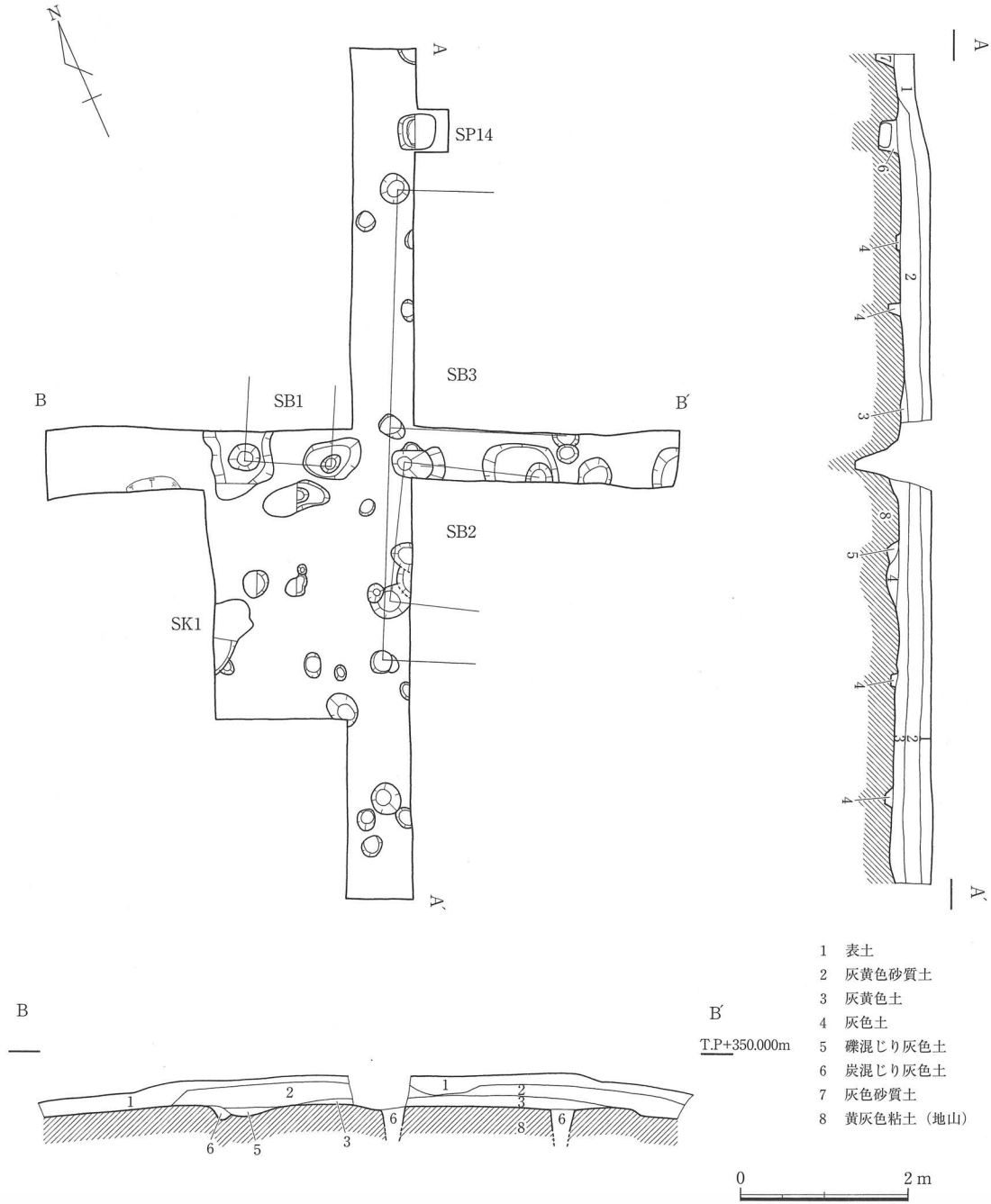
第3図 平成17年度調査区遺構配置図 (1/80)
