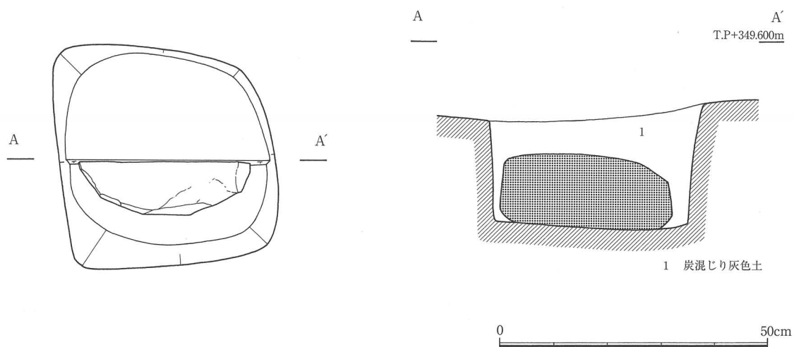
第4図 S P 14平面図・断面図 (1/10)
