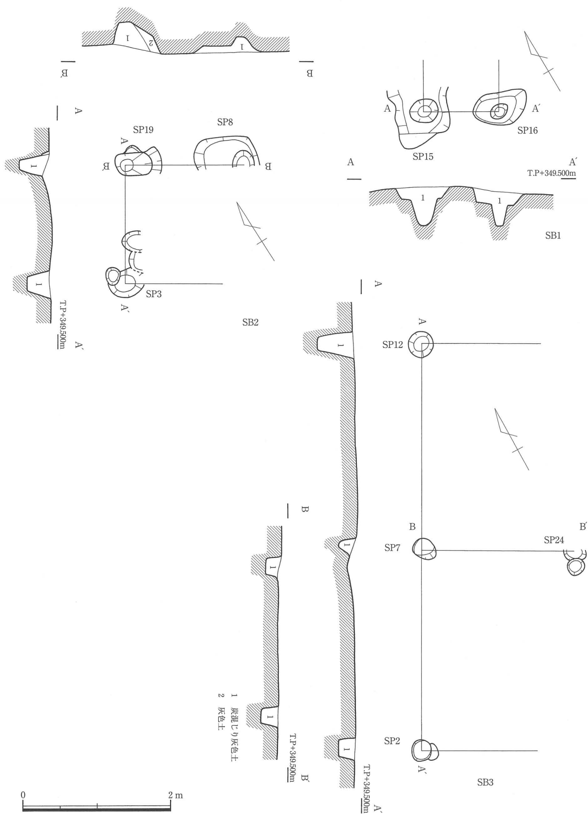
第5図 SB1・2・3平面図・断面図 (1/50)
