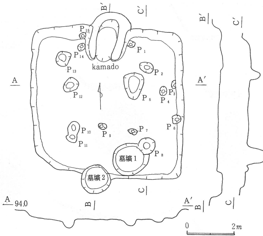
第12図 第3号住居跡実測図
