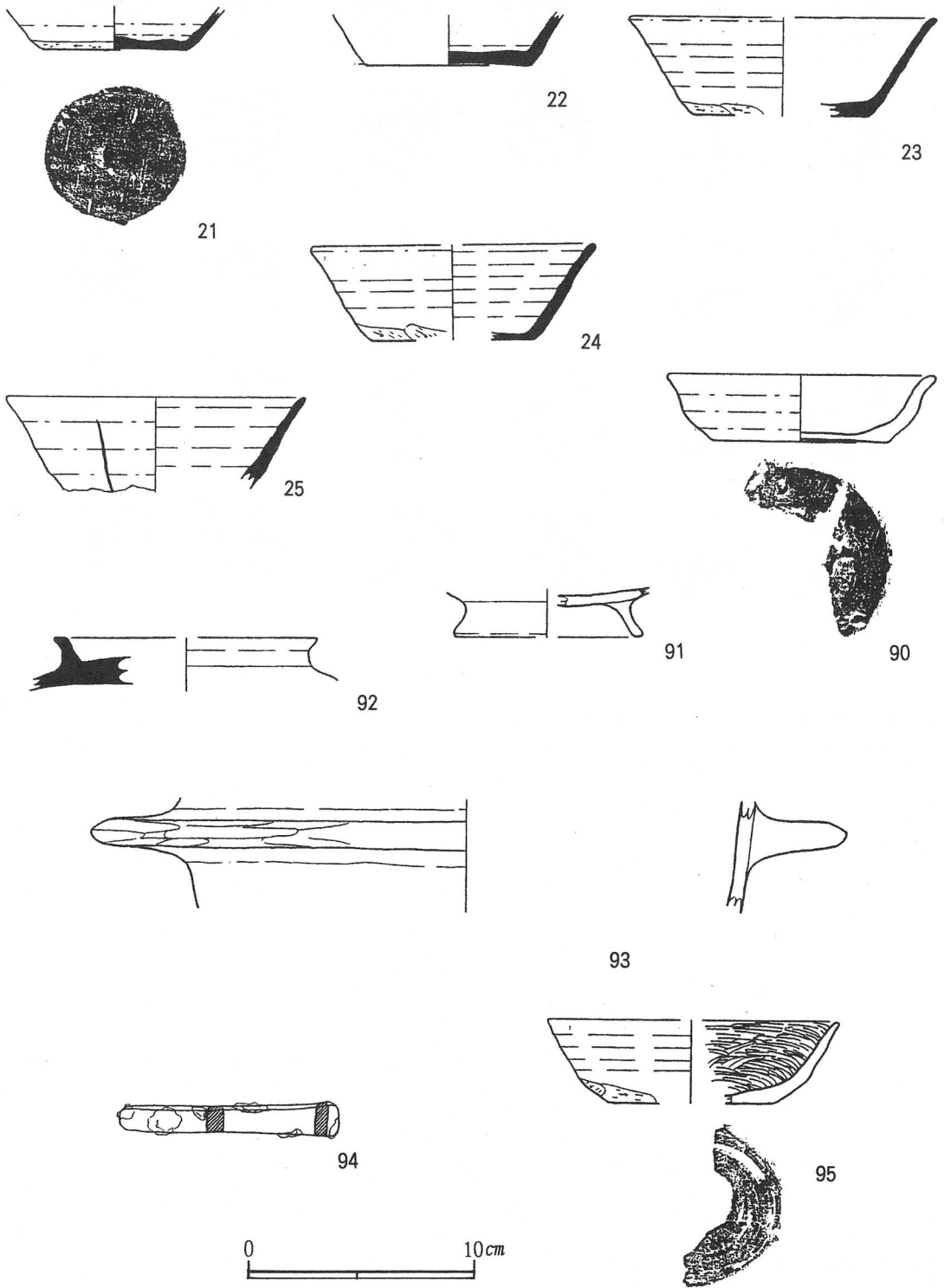
第22図 遺構外出土遺物実測図
