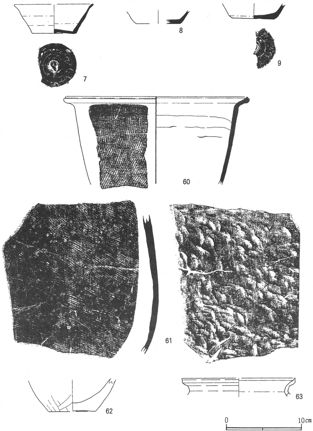
第11图 第2号住居跡出土遺物実測図
