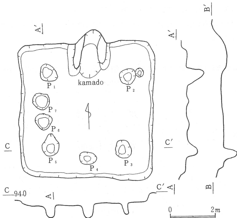
第6図 第1号住居跡実測図
