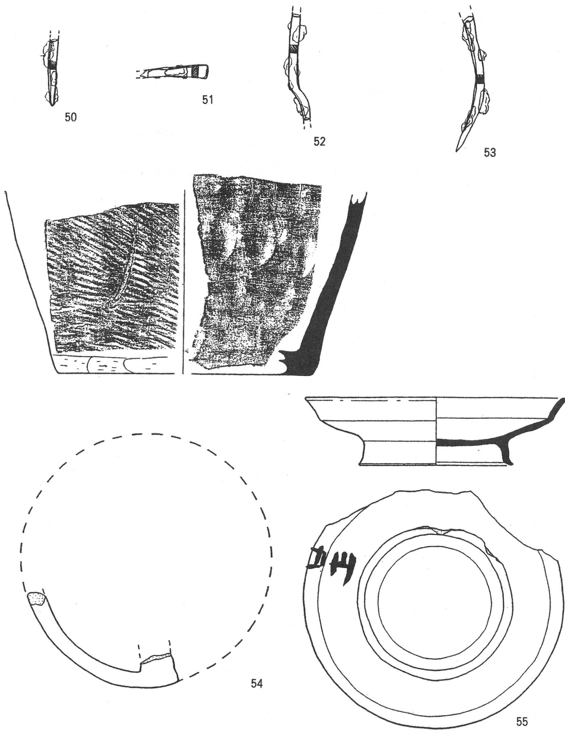
第9图 第1号住居跡出土遺物実測図(3)
