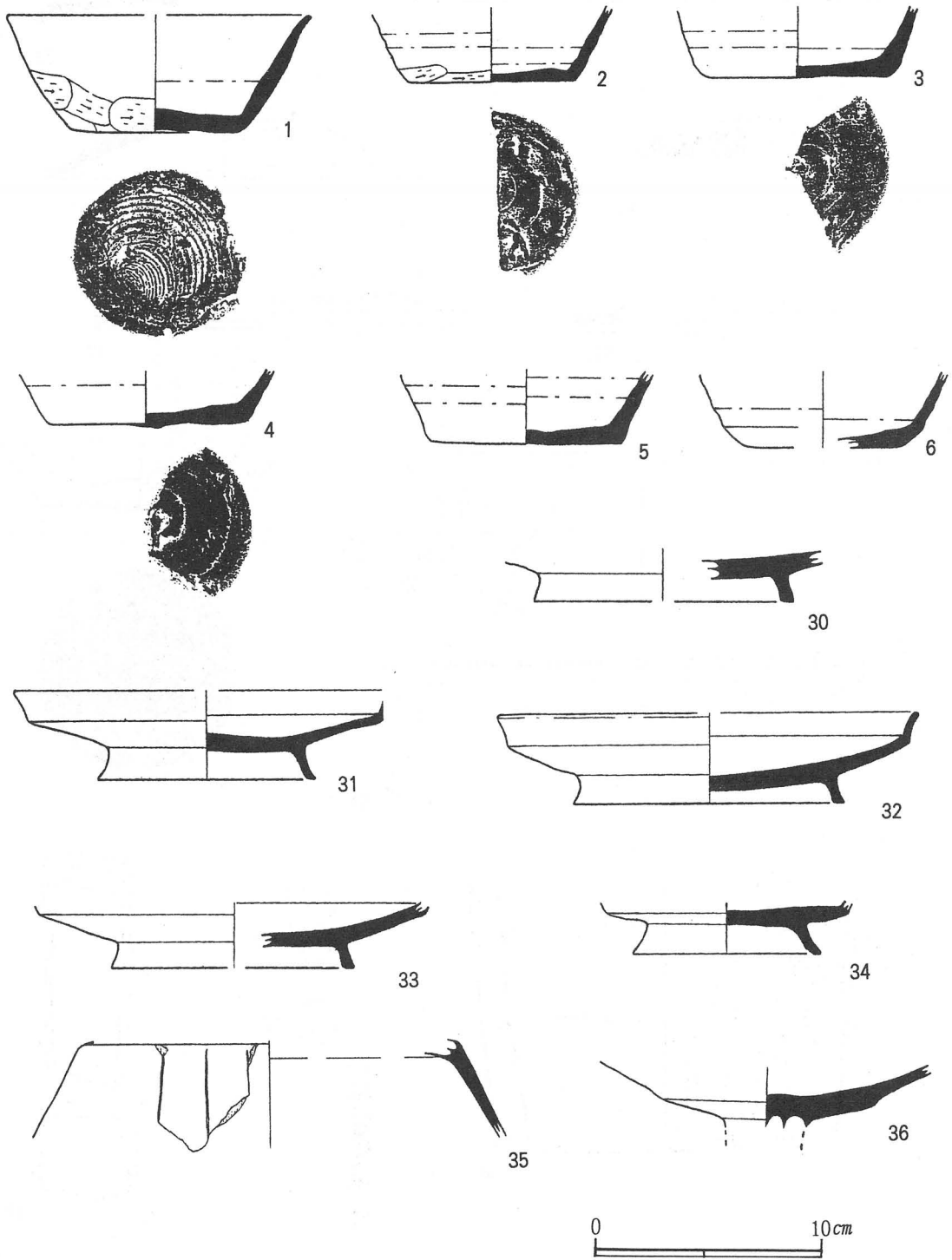
第7图 第1号住居跡出土遺物実測図(1)
