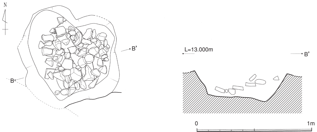
第 15 図 2 号道路跡実測図
