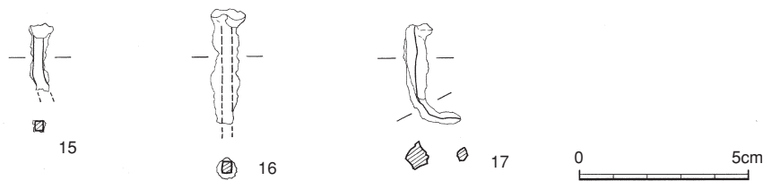
第18図 2区出土遺物実測図3
