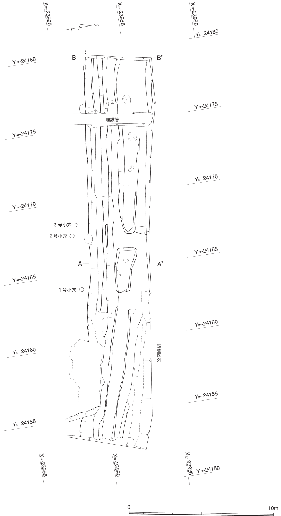
第6図 1号溝状遺構実測図1
