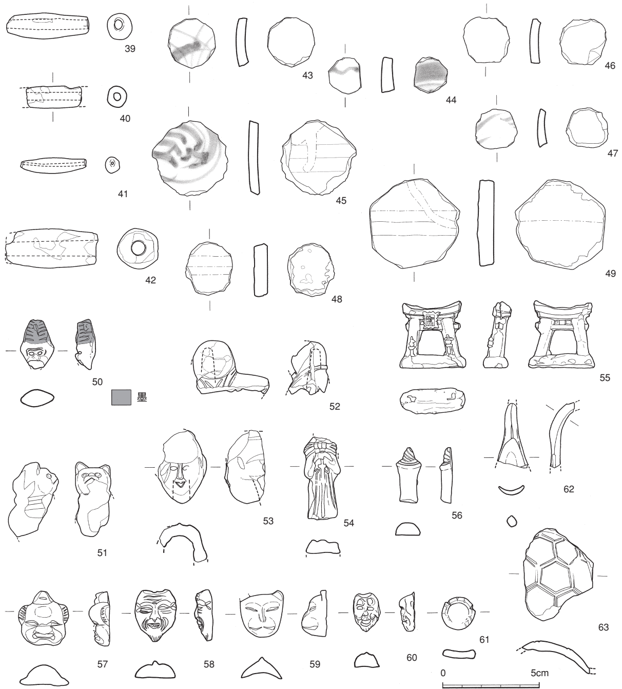
第14図 1区出土遺物実測図5
