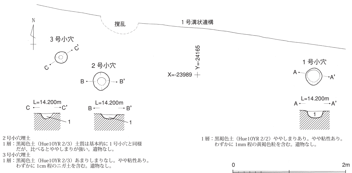
第9図 1号・2号・3号小穴実測図
