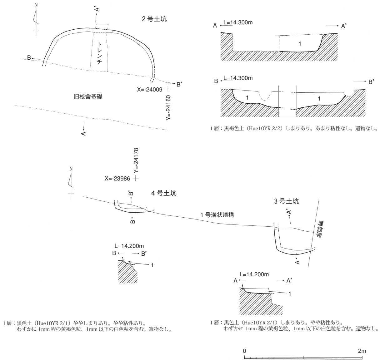
第8図 2号・3号・4号土坑実測図
