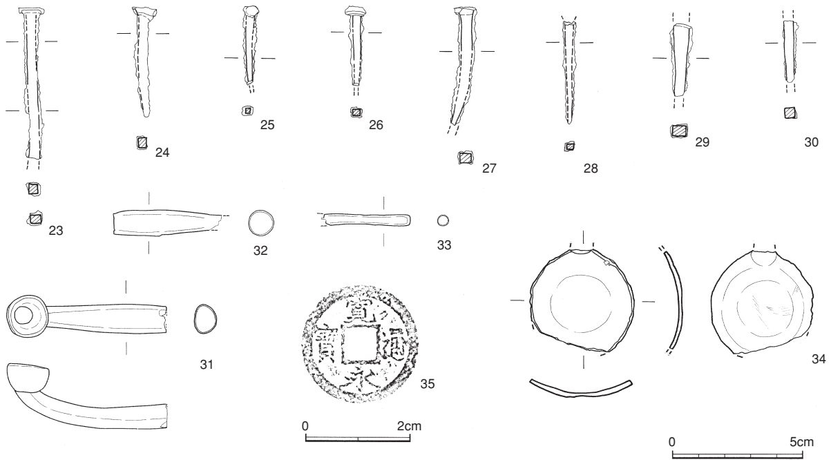
第12図 1区出土遺物実測図3
