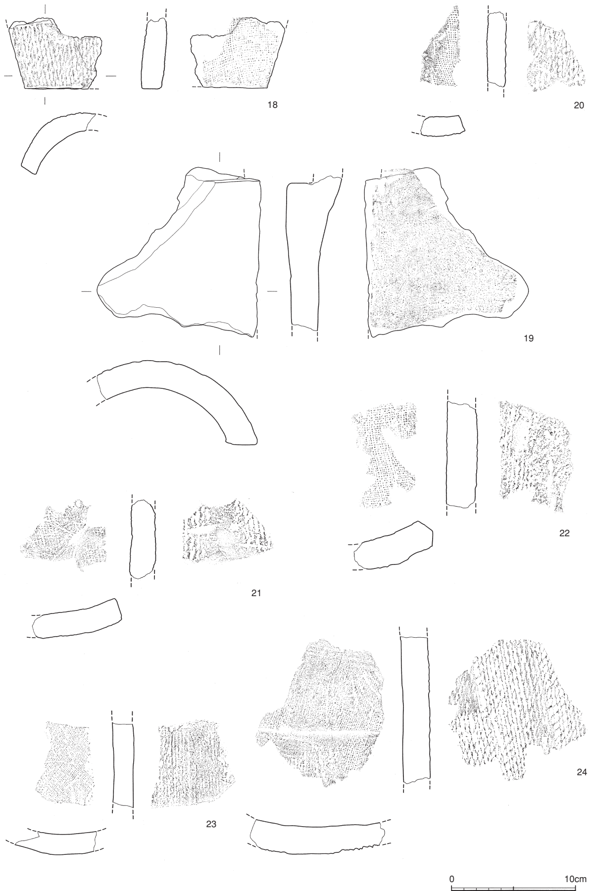
第19図 2区出土遺物実測図4
