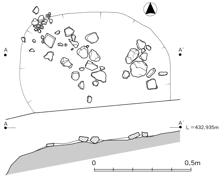
第9図 1号集石遺構図
