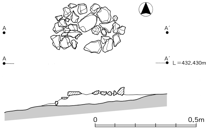
第12図 4号集石遺構図
