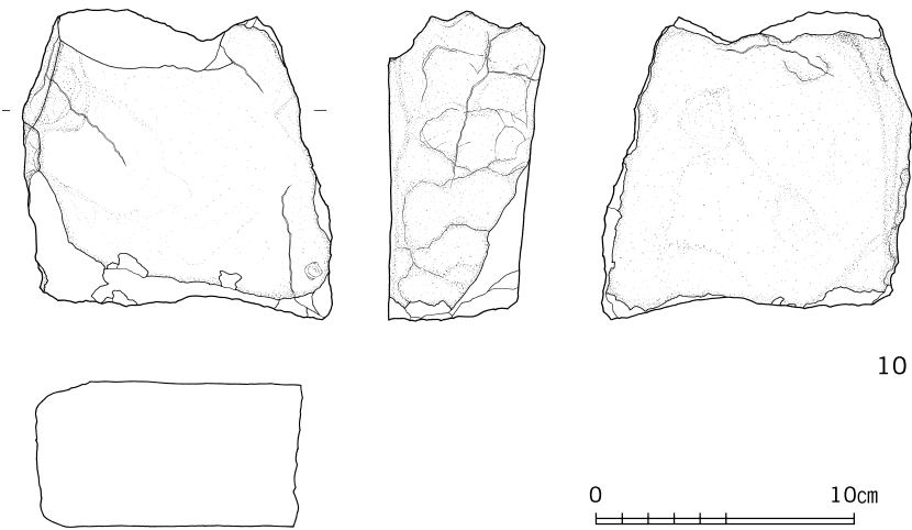
第 23 図 遺物実測図 (石器②)
