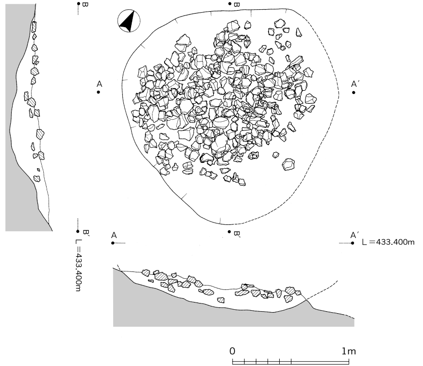
第15図 7号集石遺構図
