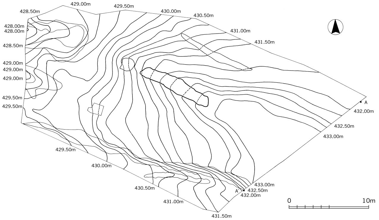
第 6 図 調査区地形測量図
