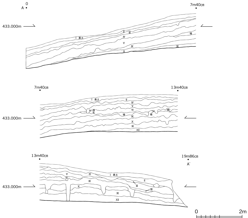
第5図 調査区土層断面図
