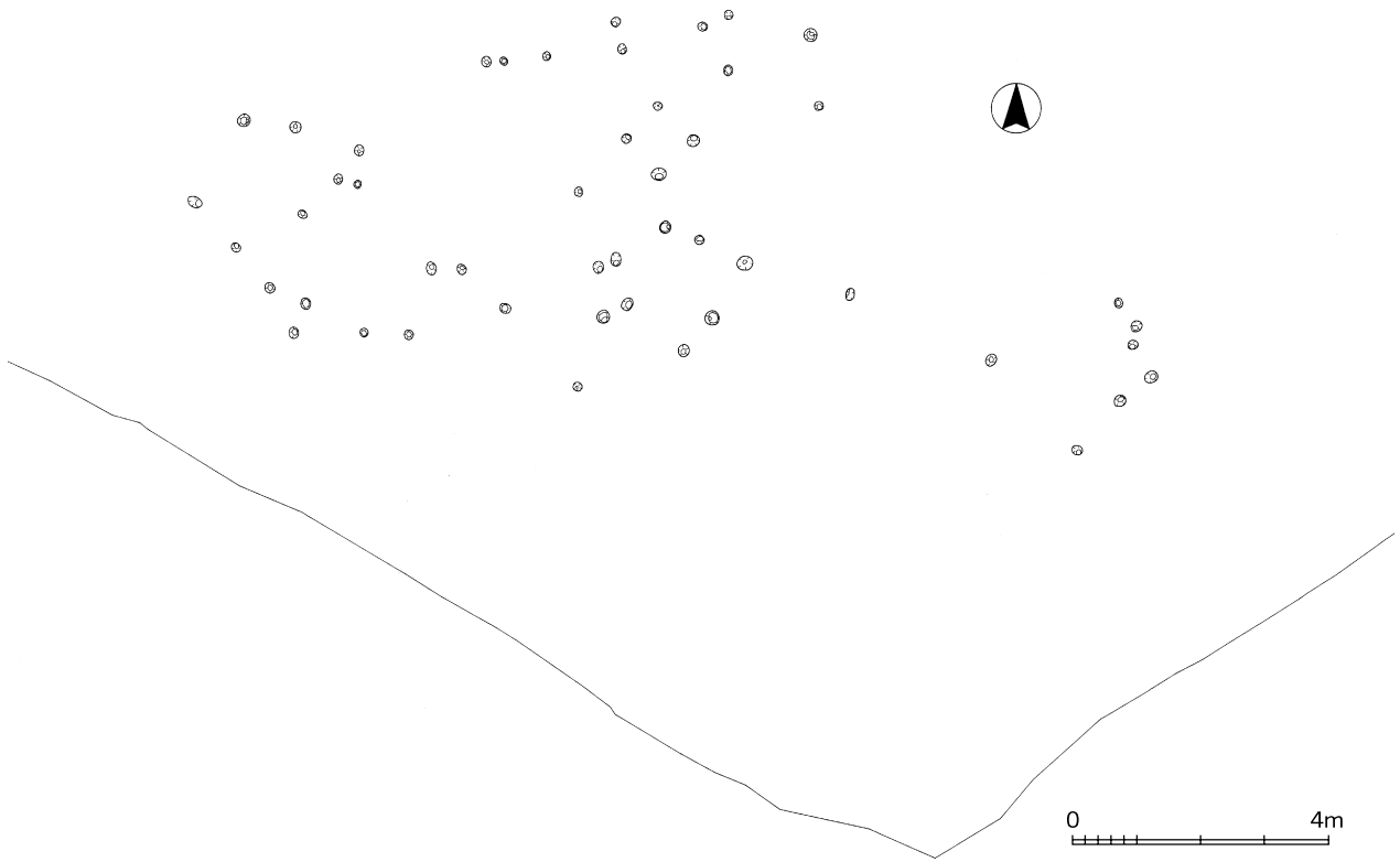
第19図 西側ピット群平面図
