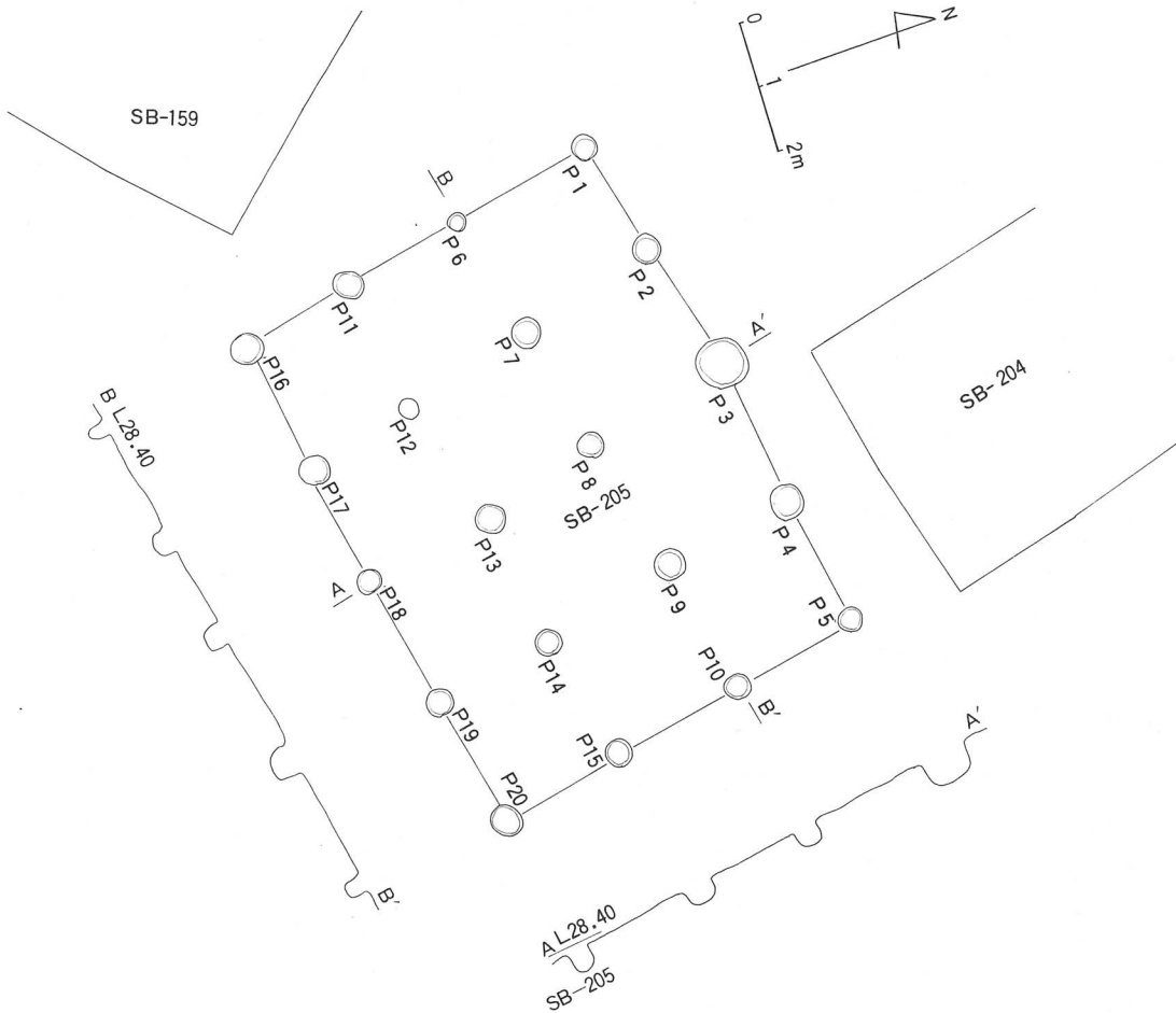
第5図 ①第205号掘立柱建物遺構平面実測図
