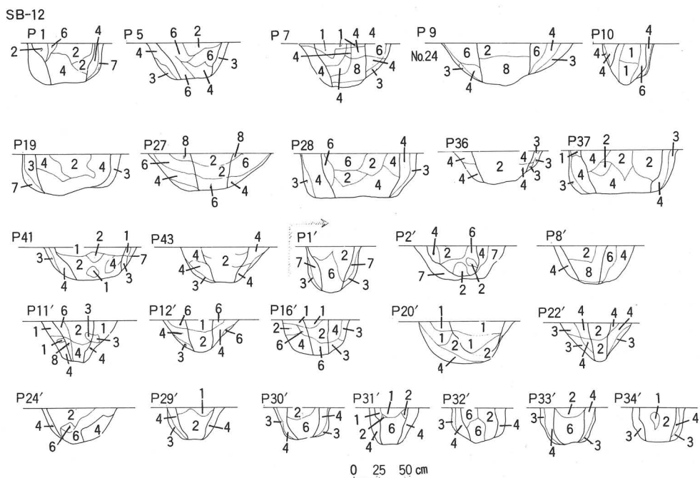
第9図 ～②第12号遺構柱穴セクション
