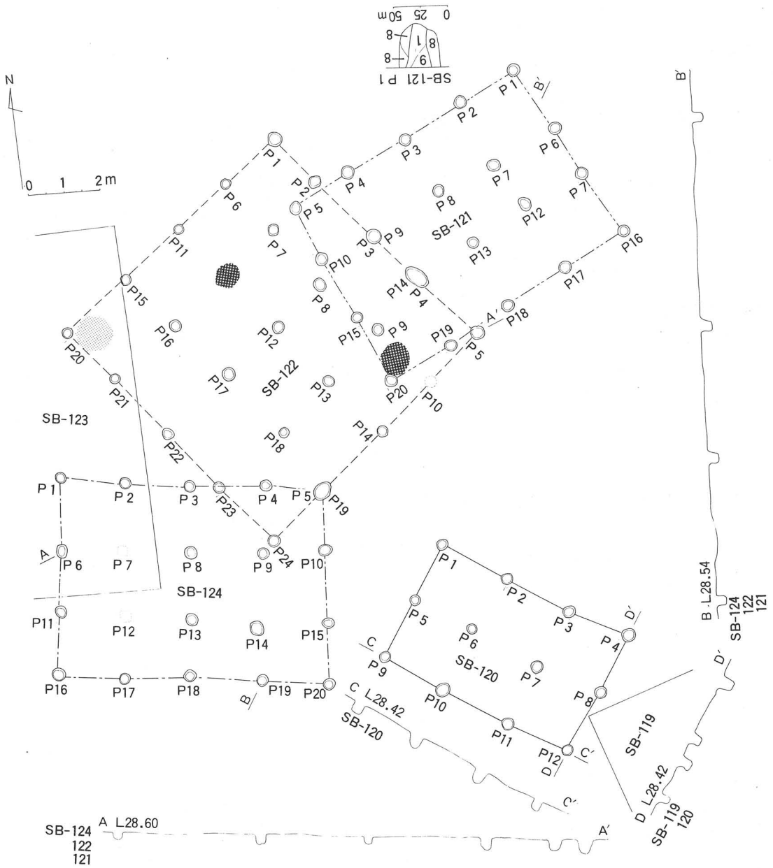
第36图 第120号, 121号, 122号, 124号掘立柱建物遺構平面実測図
