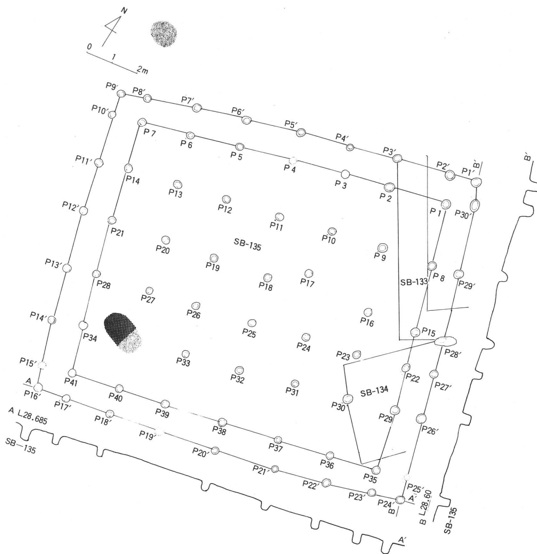
第41图 第135号掘立柱建物遺構平面実測図
