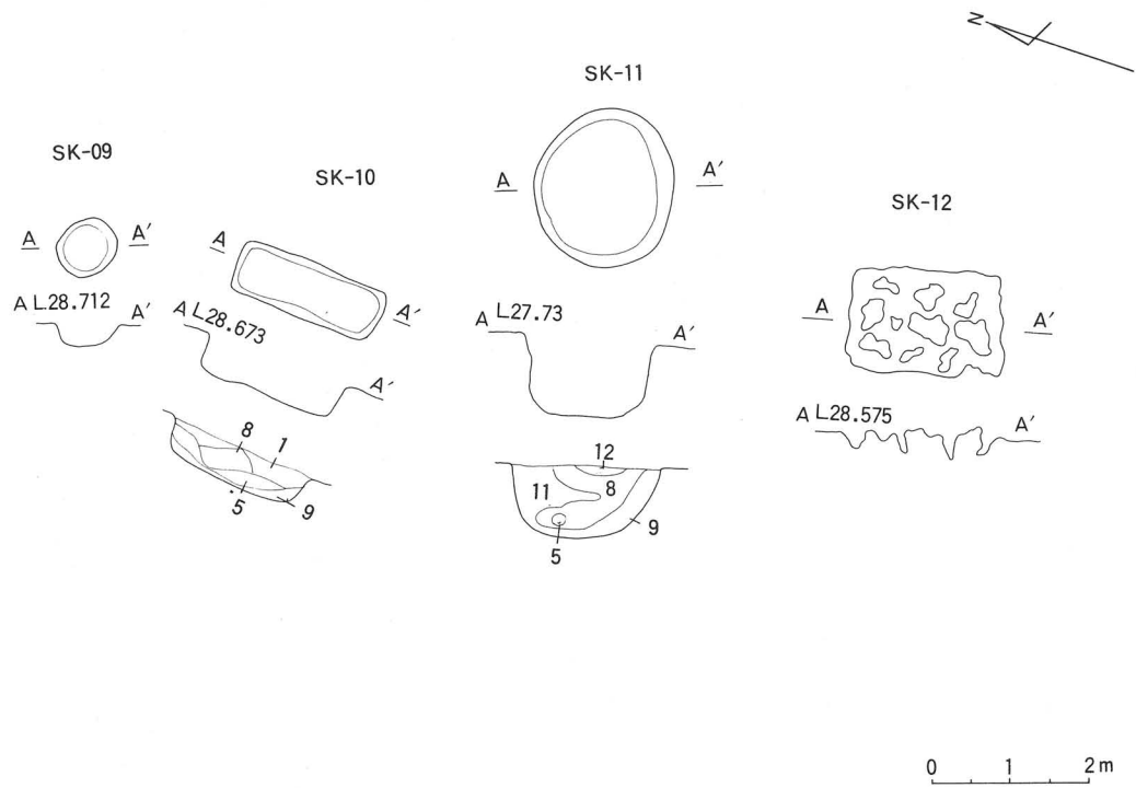
第61図 第9号, 10号, 11号, 12号土壇状遺構平面実測図
