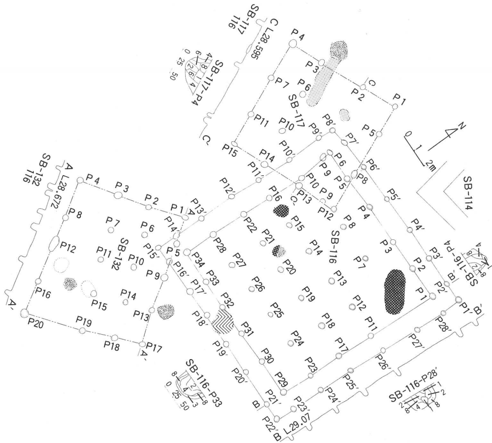
第34図 第116号, 117号, 132号掘立柱建物遺構平面実測図
