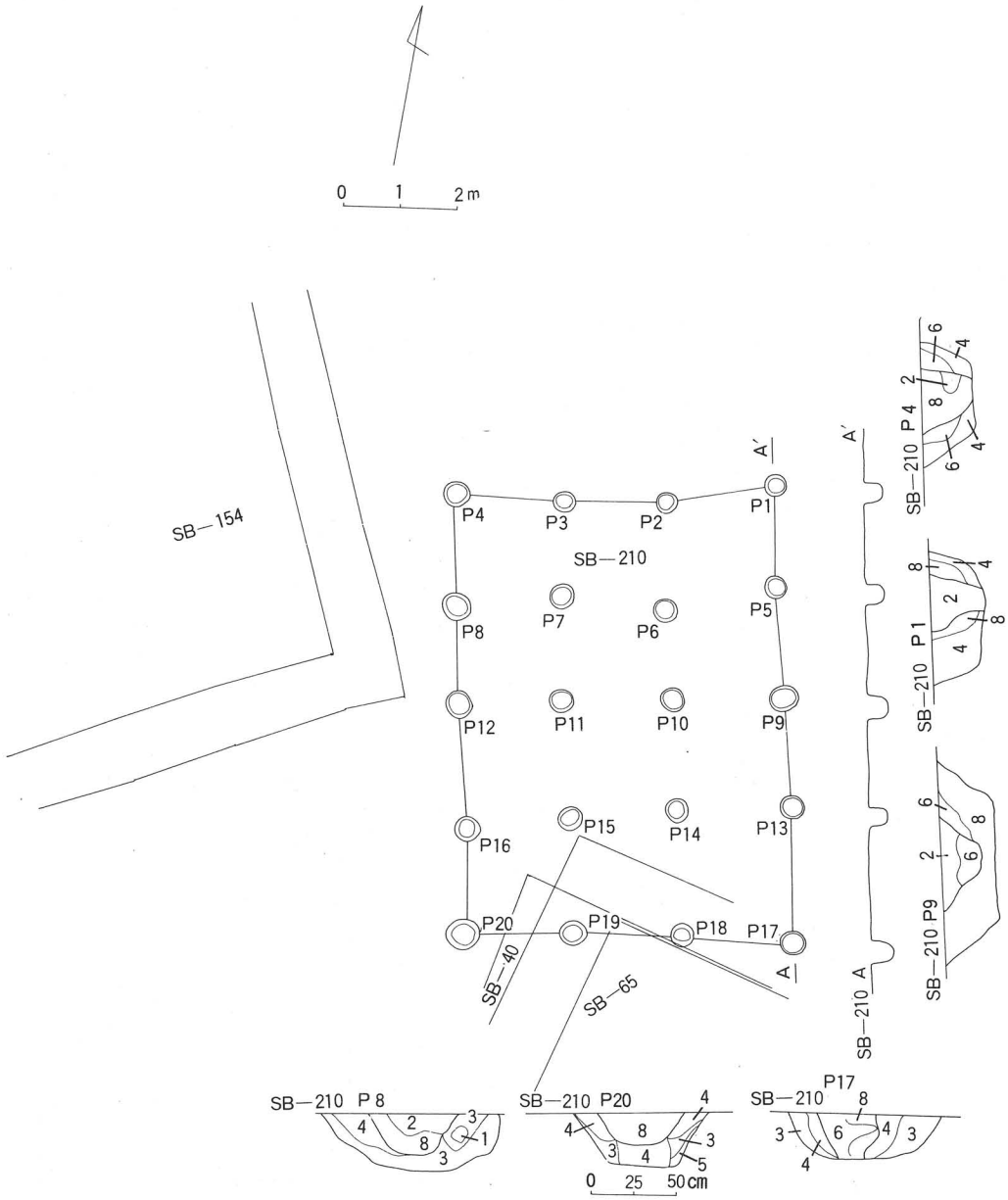
第 8 图 第210号掘立柱建物遺構平面実測図
