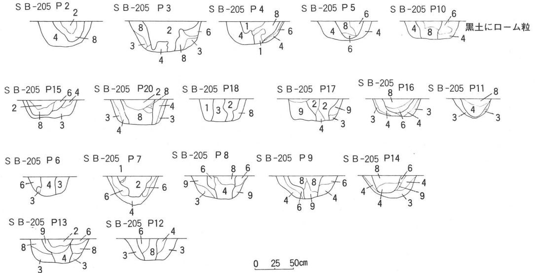
第5図 ～②第205号遺構柱穴セクション
