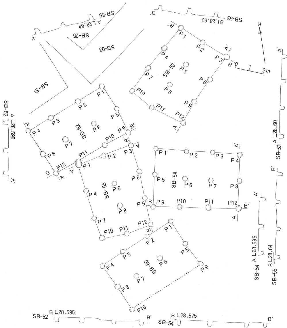
第19图 第52号, 53号, 54号, 55号, 60号掘立柱建物遺構平面実測図
