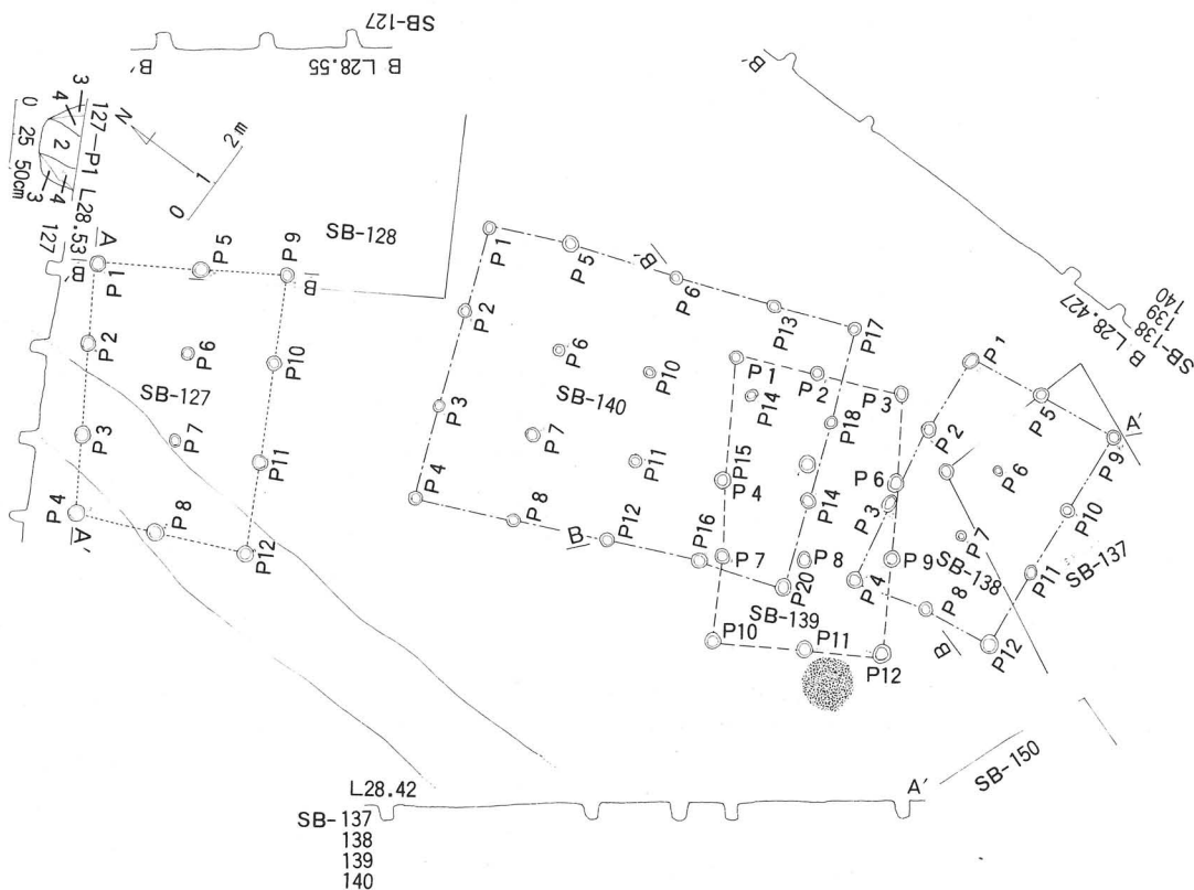
第38図 第127号, 138号, 139号, 140号掘立柱建物遺構平面実測図
