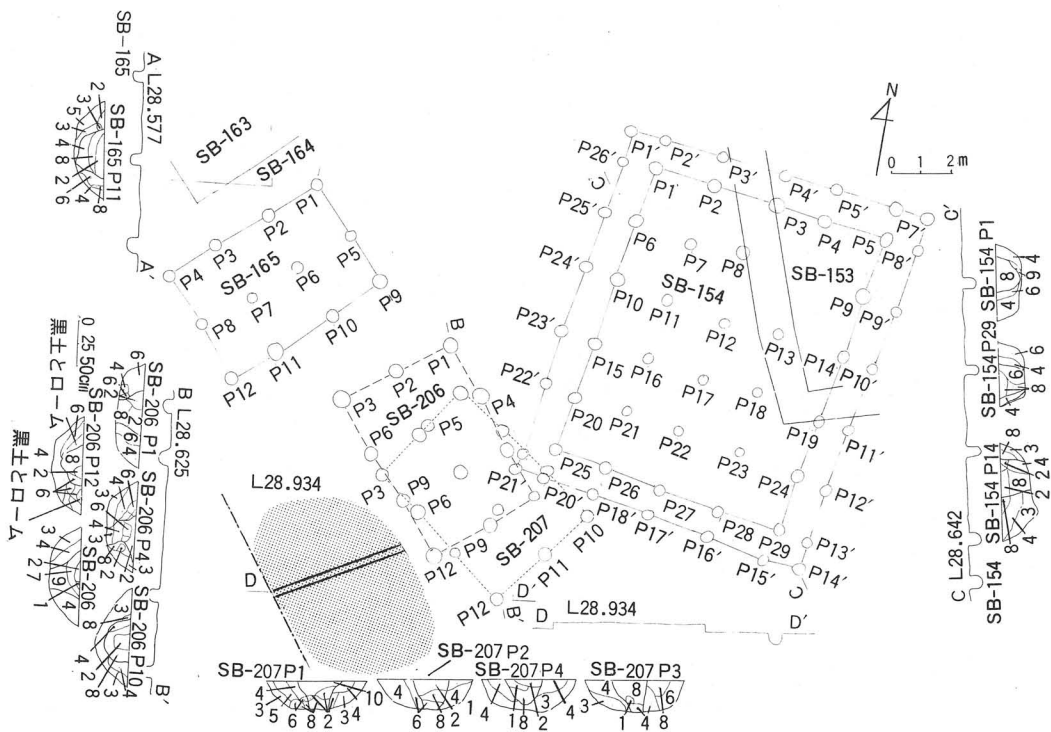
第6図 第154号, 165号, 206号, 207号掘立柱建物遺構平面実測図
