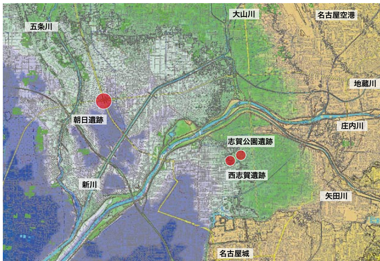
図 1.4-2 朝日遺跡と周辺の地形復原 (国土地理院数値地図 5m メッシュ「濃尾平野」を利用。青色は海拔 2m 未満、緑色は 5m、褐色は 10m を表示)
