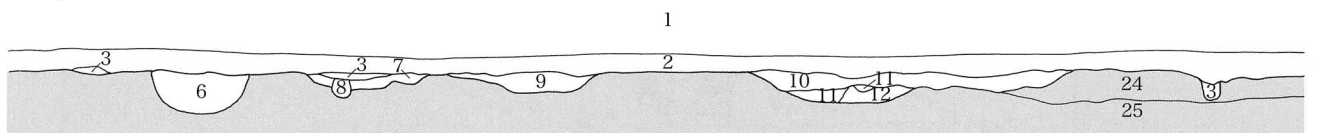
H J 第 541 次調査 東発掘区旧流路部分土層断面図 (1/80)
