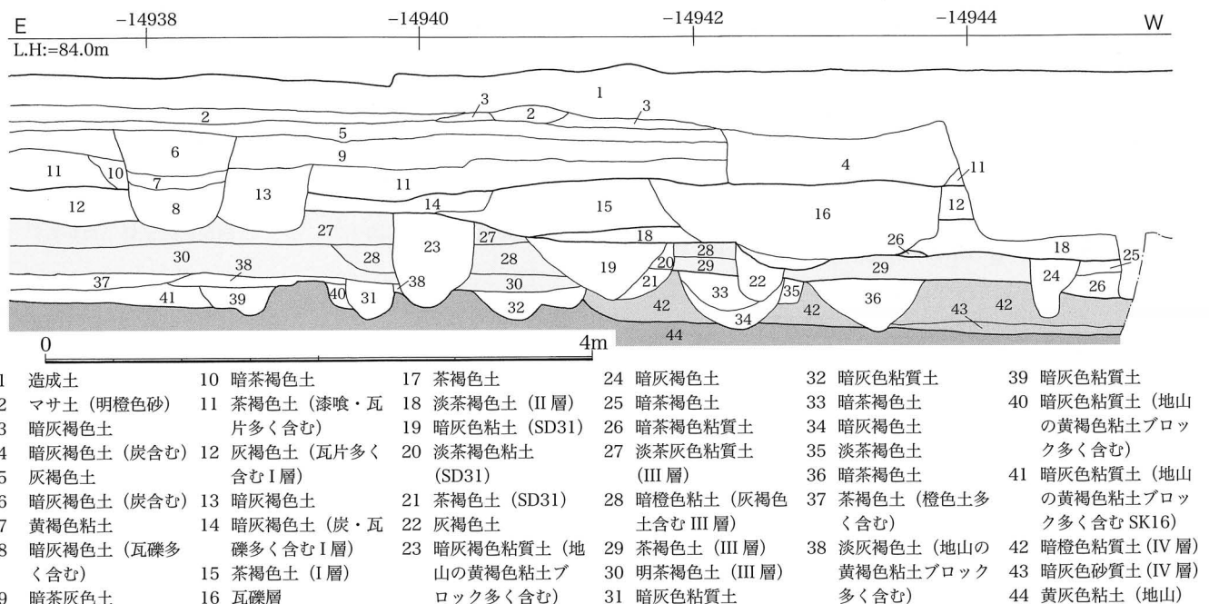
HJ 第531次調査 第1発掘区南壁土層図 (1/50)
