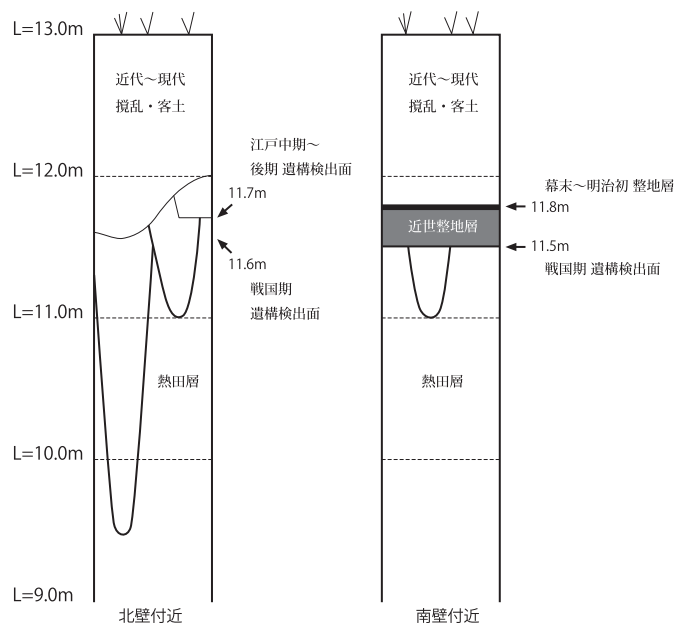
図9 基本層序概念図
