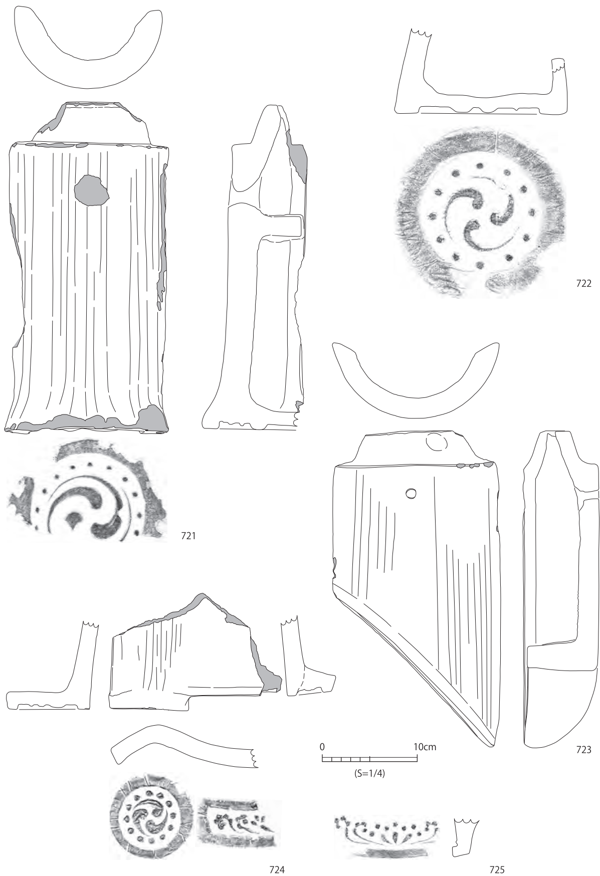
图 69 389SK 出土軒丸瓦·丸瓦·軒棧瓦 (S=1/4)
