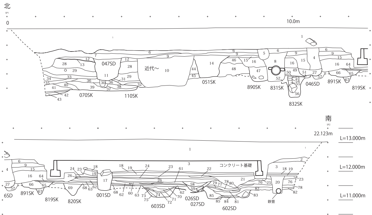
図 11 東壁 土層断面図 -1 (S=1/80)
