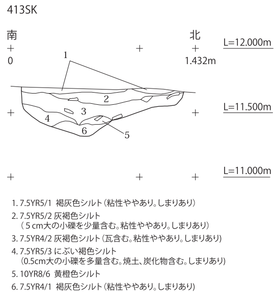
図 24 土坑 413SK 断面図 (S=1/30)
