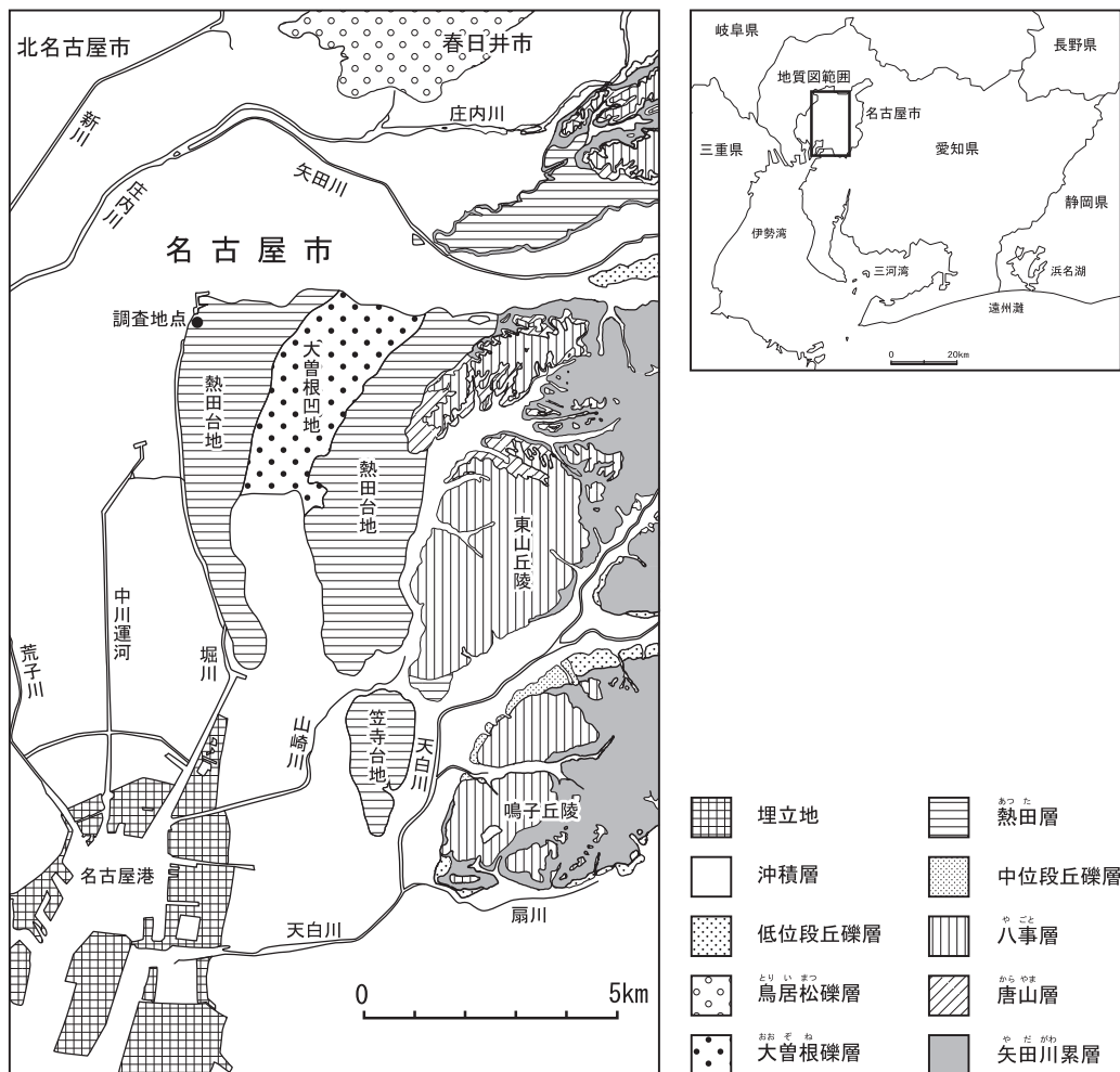
図4 名古屋城三の丸遺跡周辺の地質図
