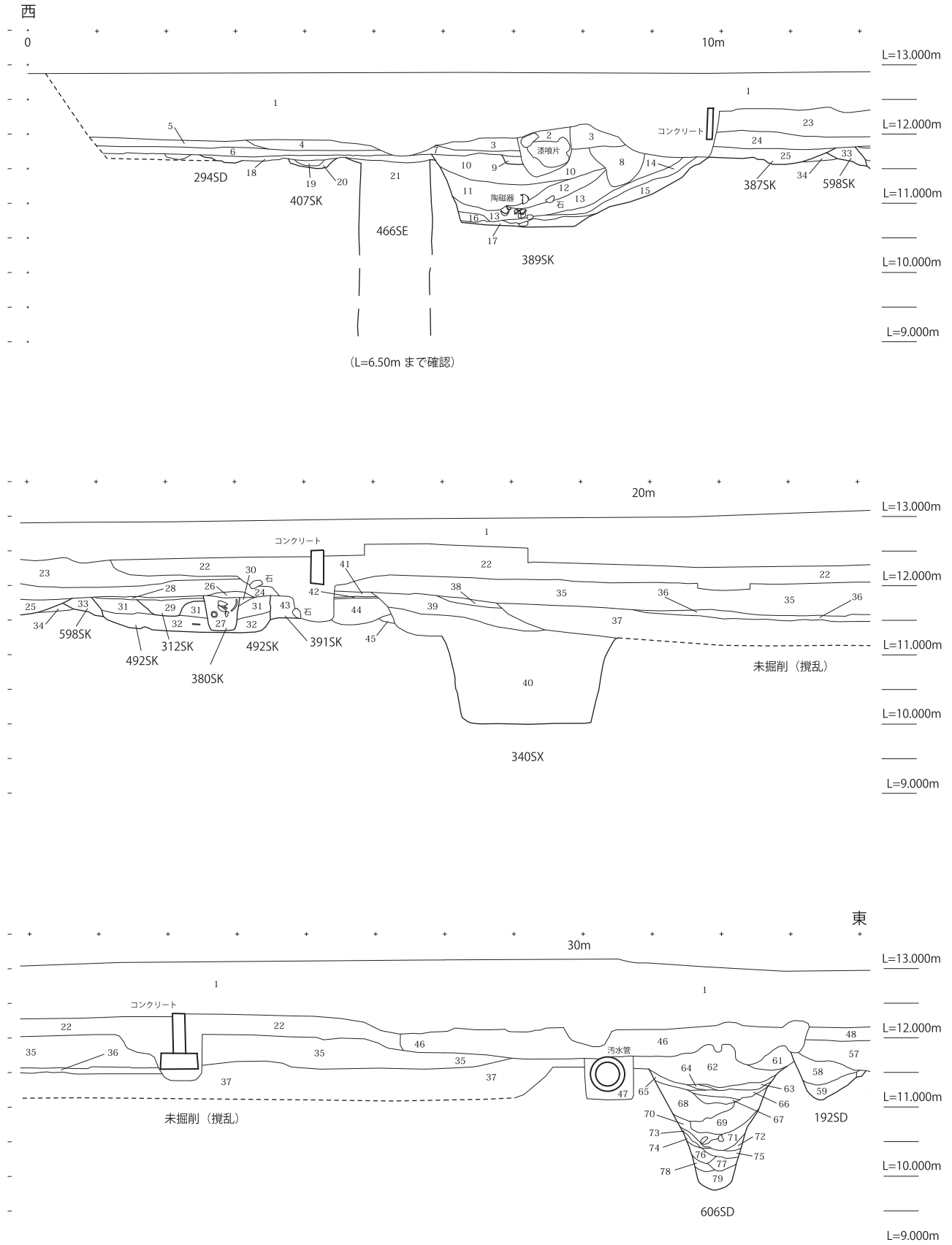
図 13 北壁 土層断面図 -1 (S=1/80)
