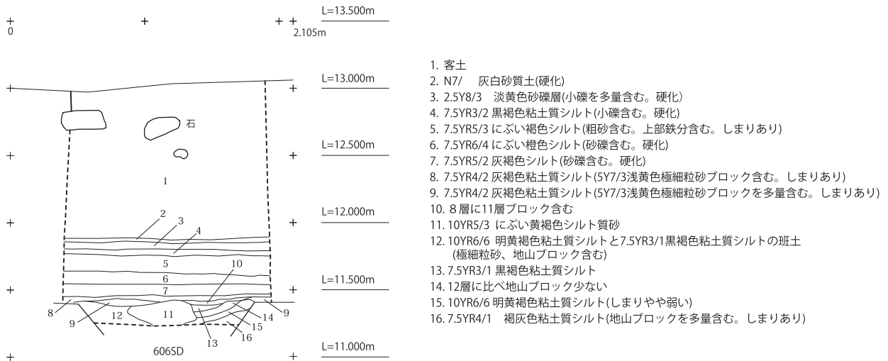
図 10 南壁 土層断面図 -1 (S=1/40)
