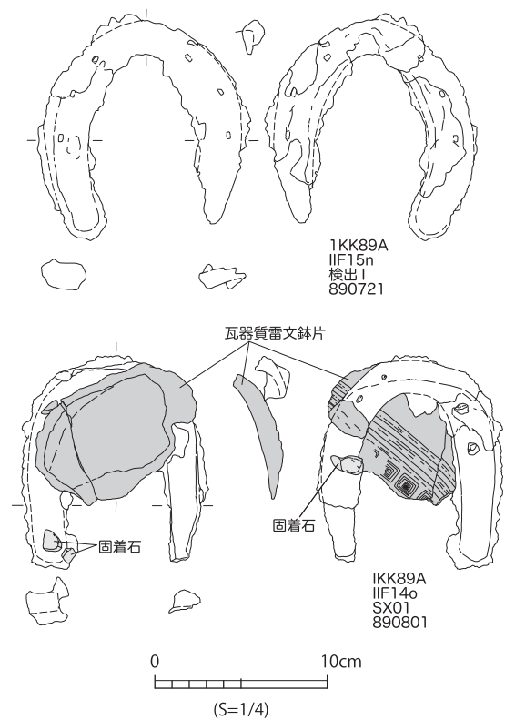
図89 勝川遺跡出土蹄鉄 (S=1/4)
