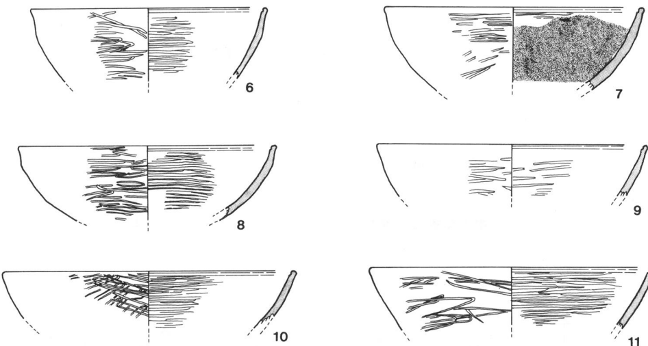
第1 拡張区 3層
