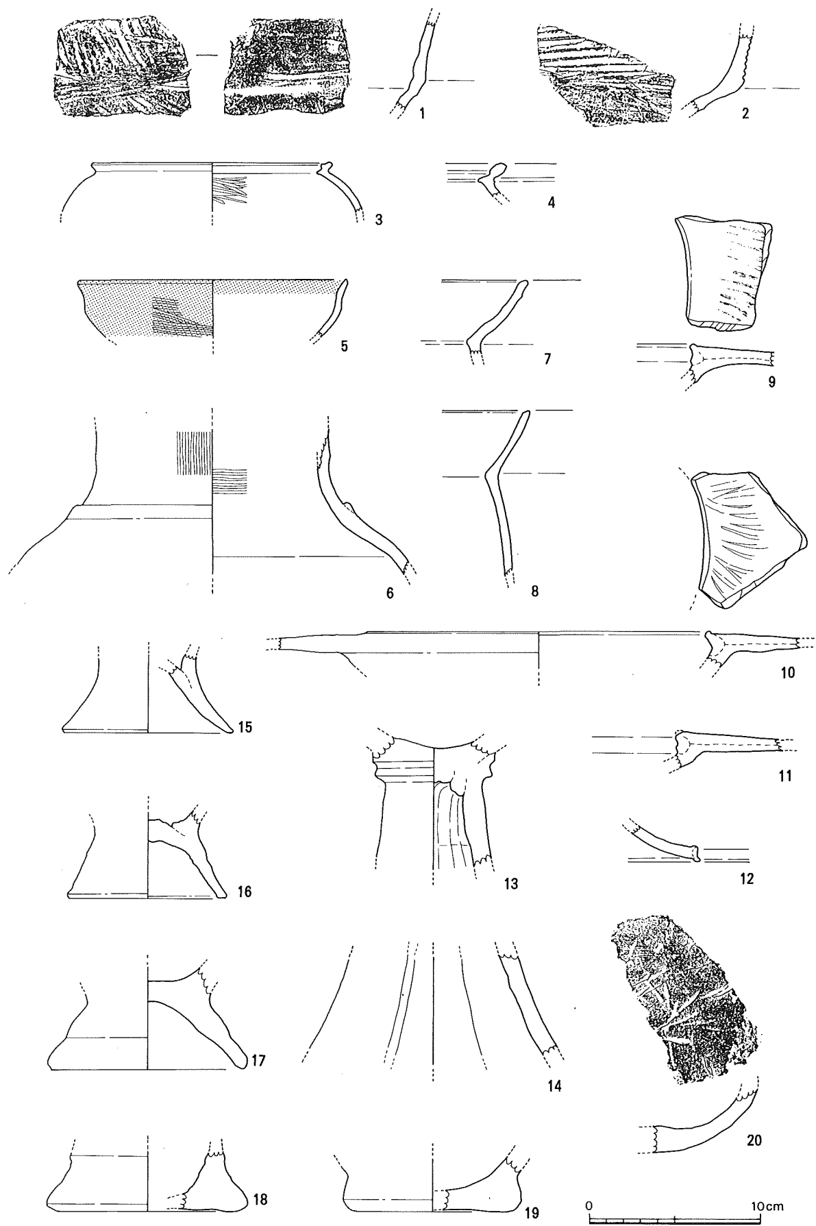
第8图 土器实测图① (S=1/3)
