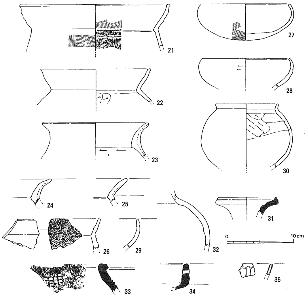
第9図 土器実測図② (S = 1 / 3)
