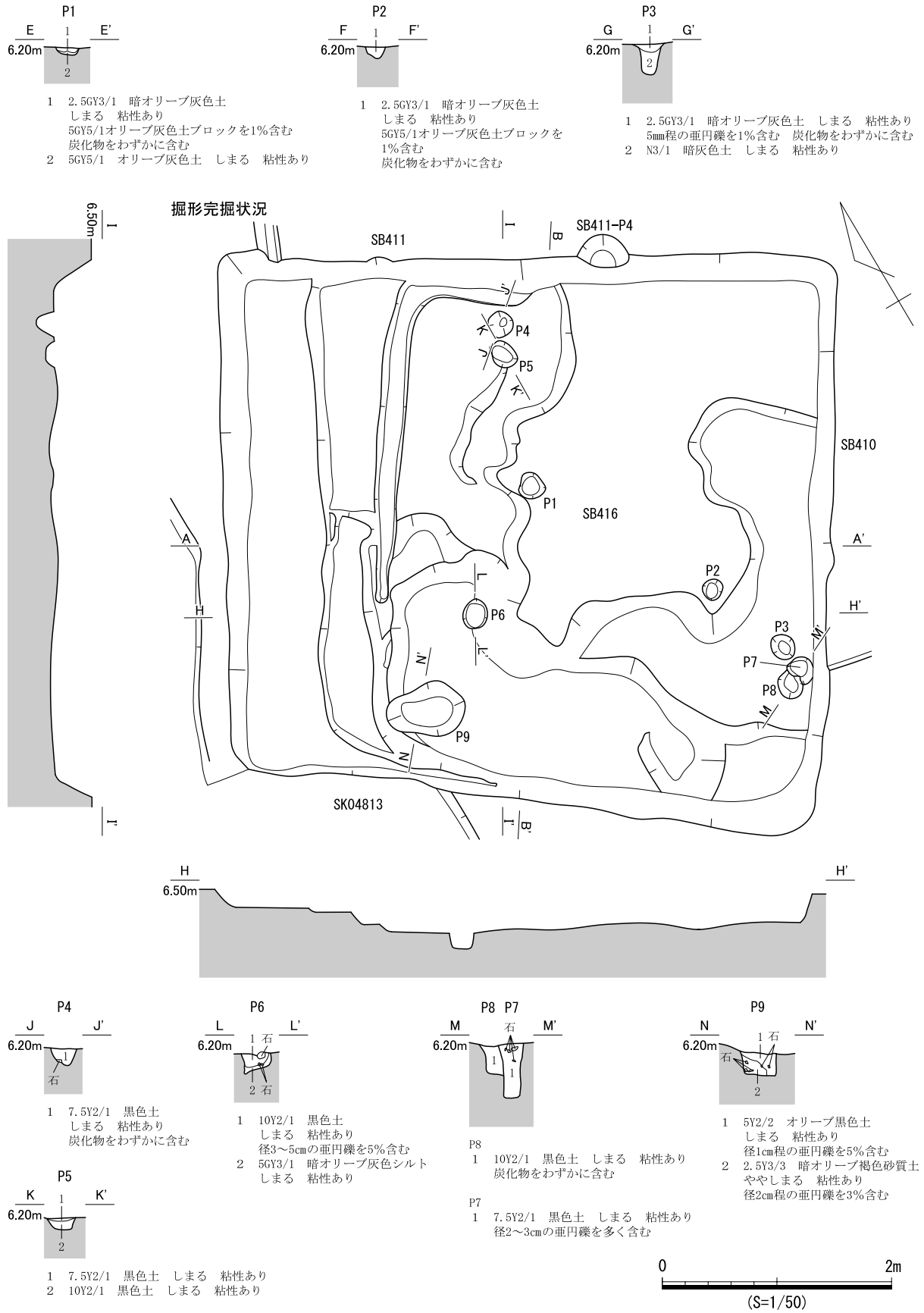
図 773 SB416 遺構図 (2)
