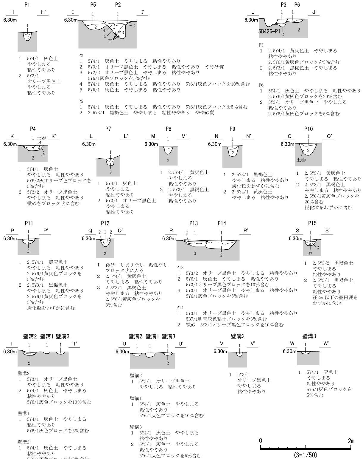
図 803 SB427 遺構図 (2)
