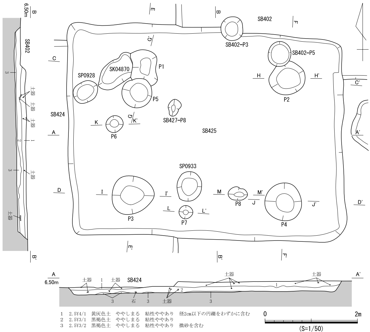
図 797 SB425 遺構図 (1)
