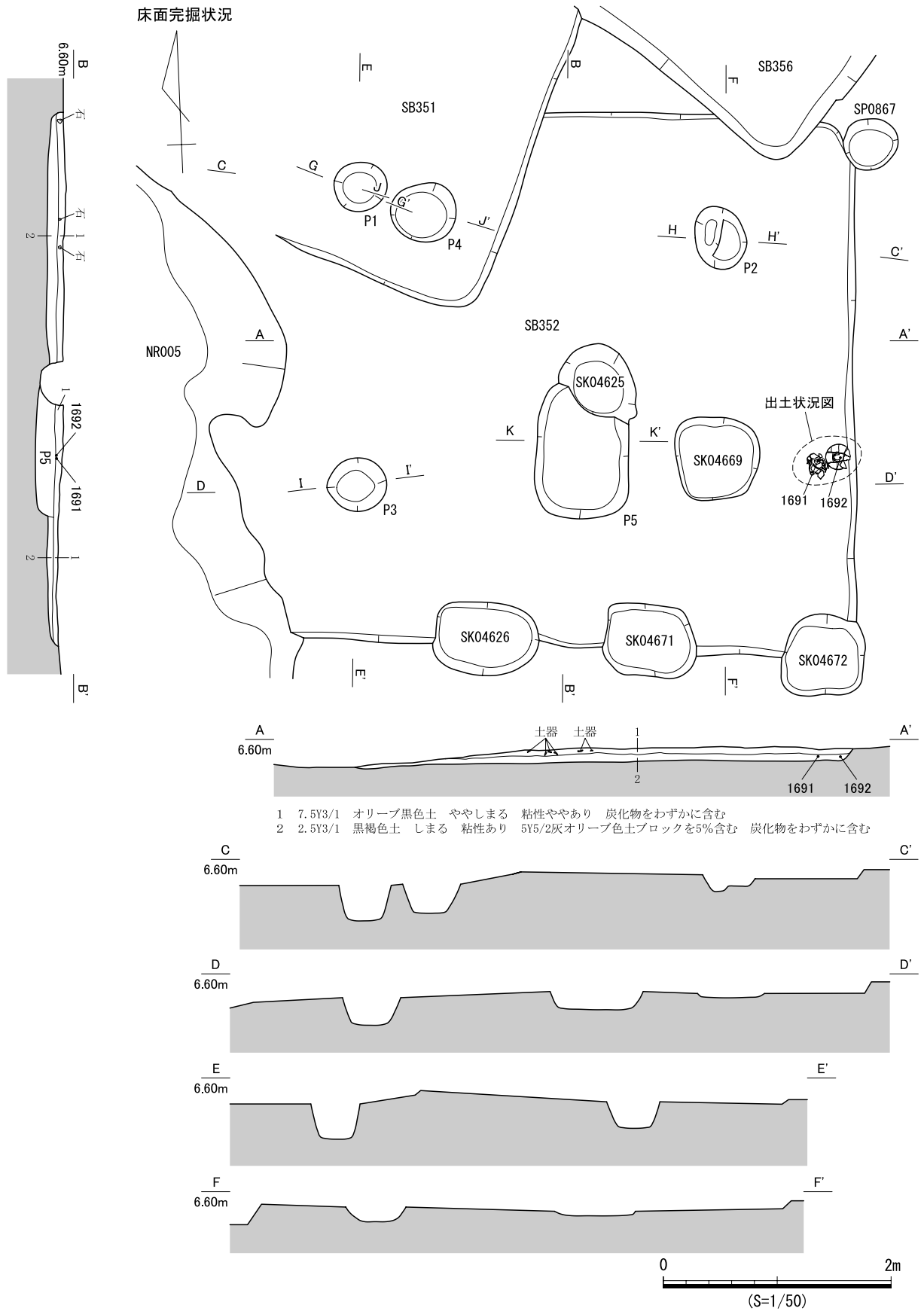
図 614 SB352 遺構図 (1)
