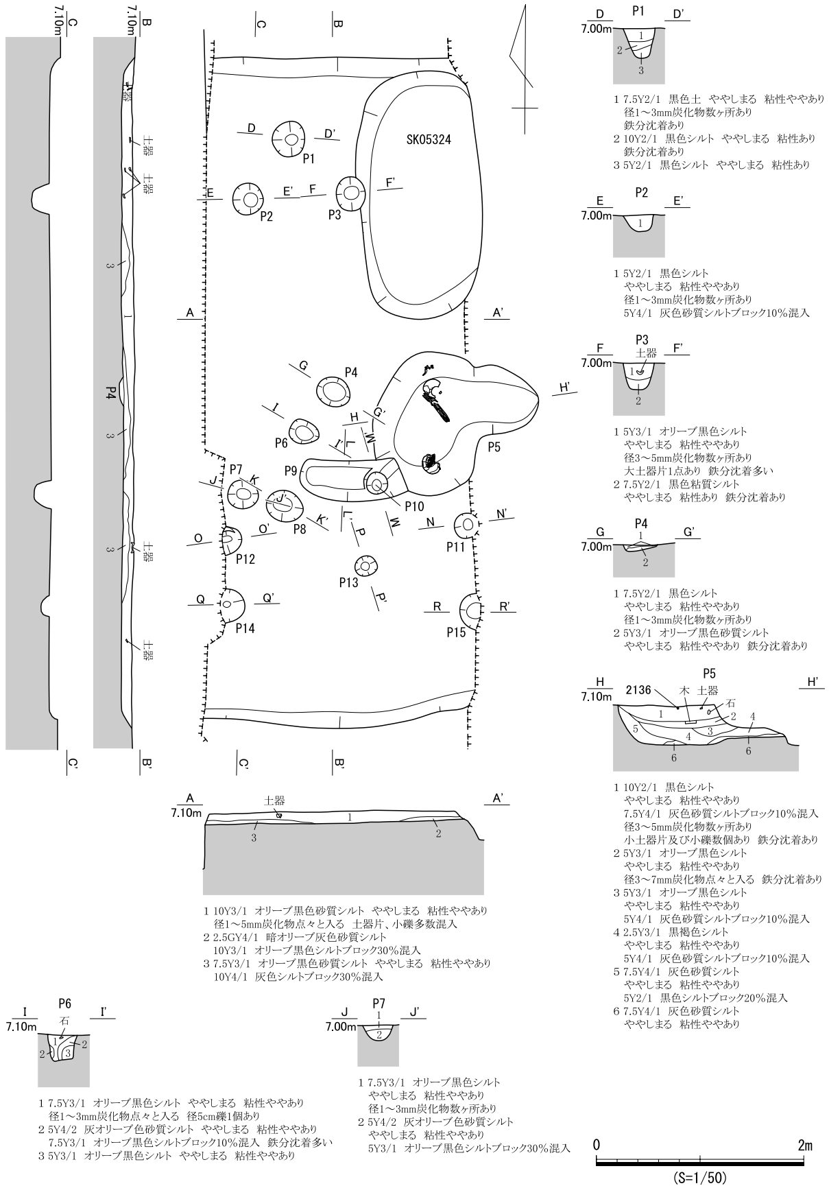
図 857 SB451 遺構図 (1)
