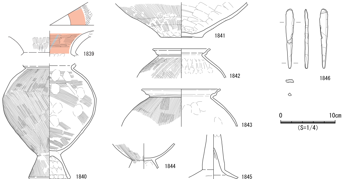
図 682 SB379 遺物実測図
