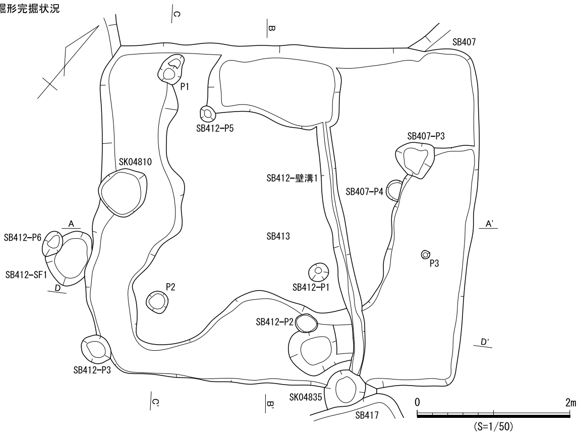
図 767 SB413 遺構図（2）
