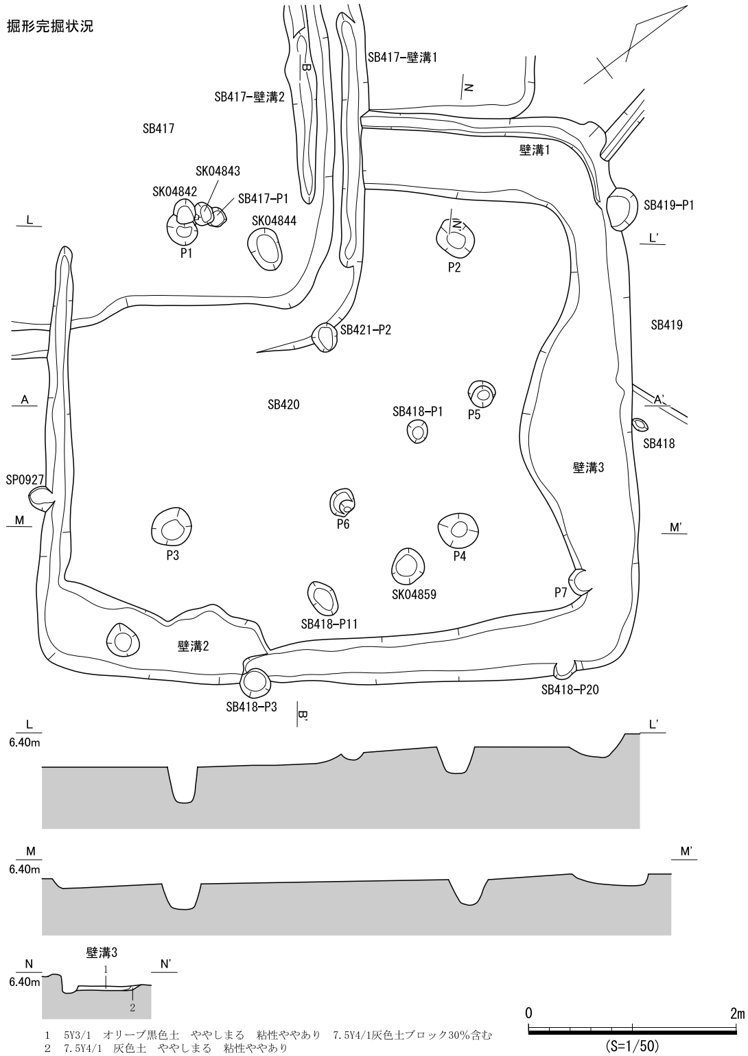
図 786 SB420 遺構図 (3)
