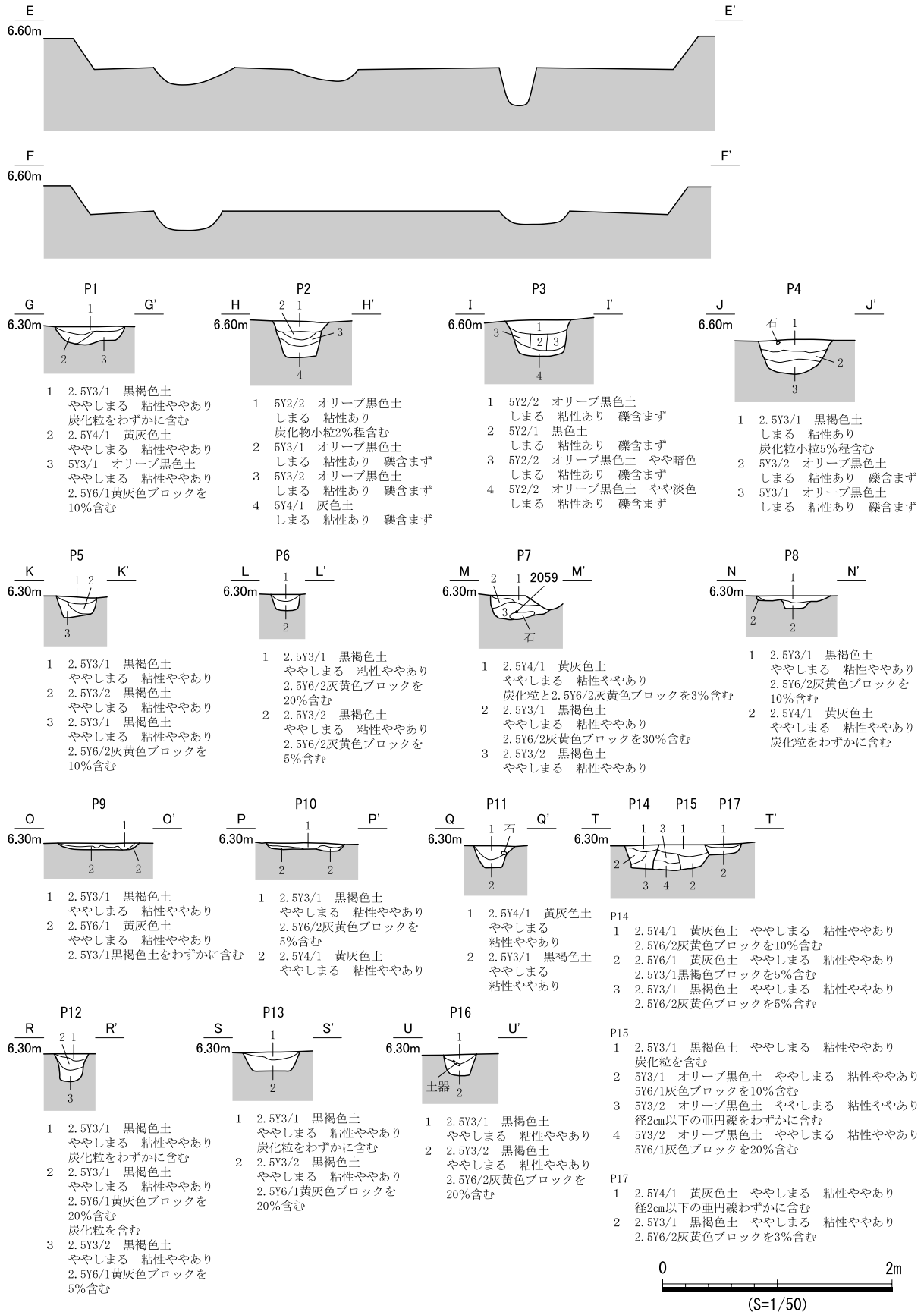
図 809 SB429 遺構図 (2)
