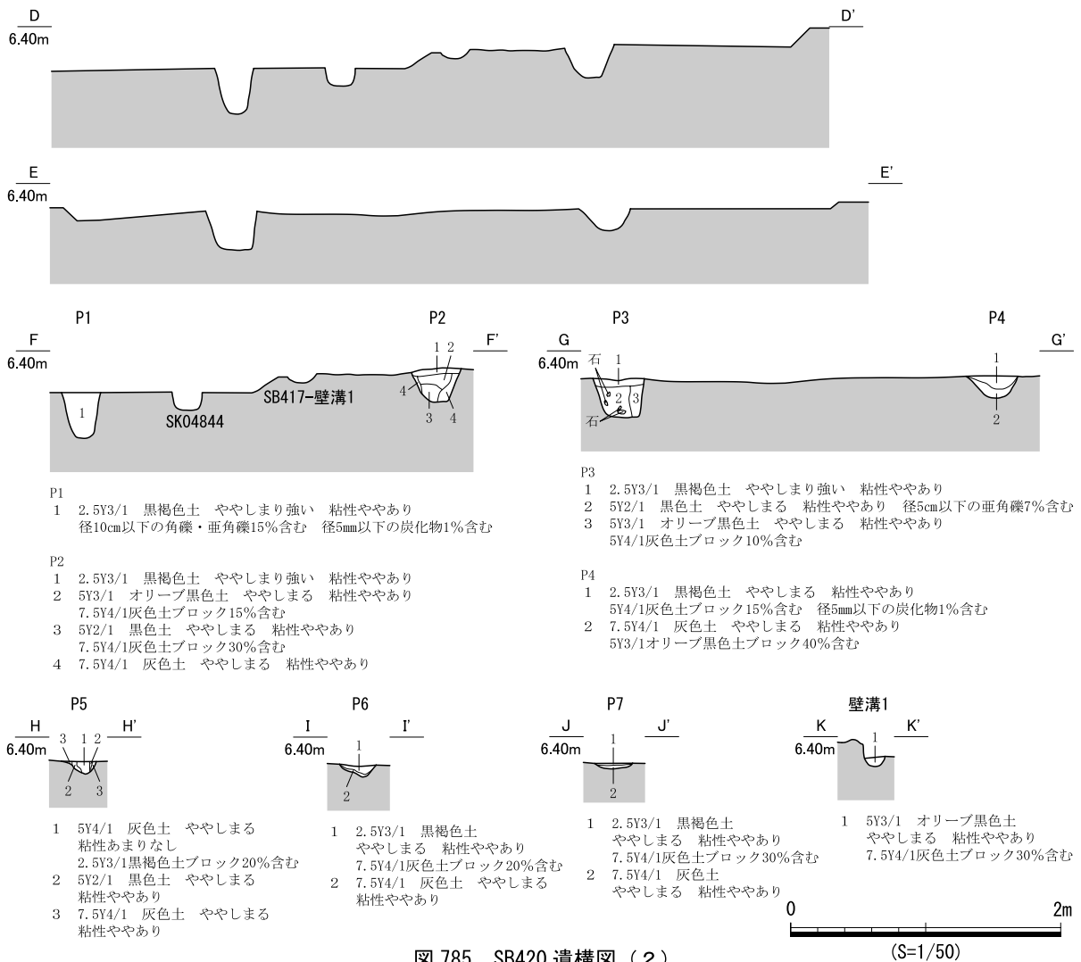
図 785 SB420 遺構図 (2)
