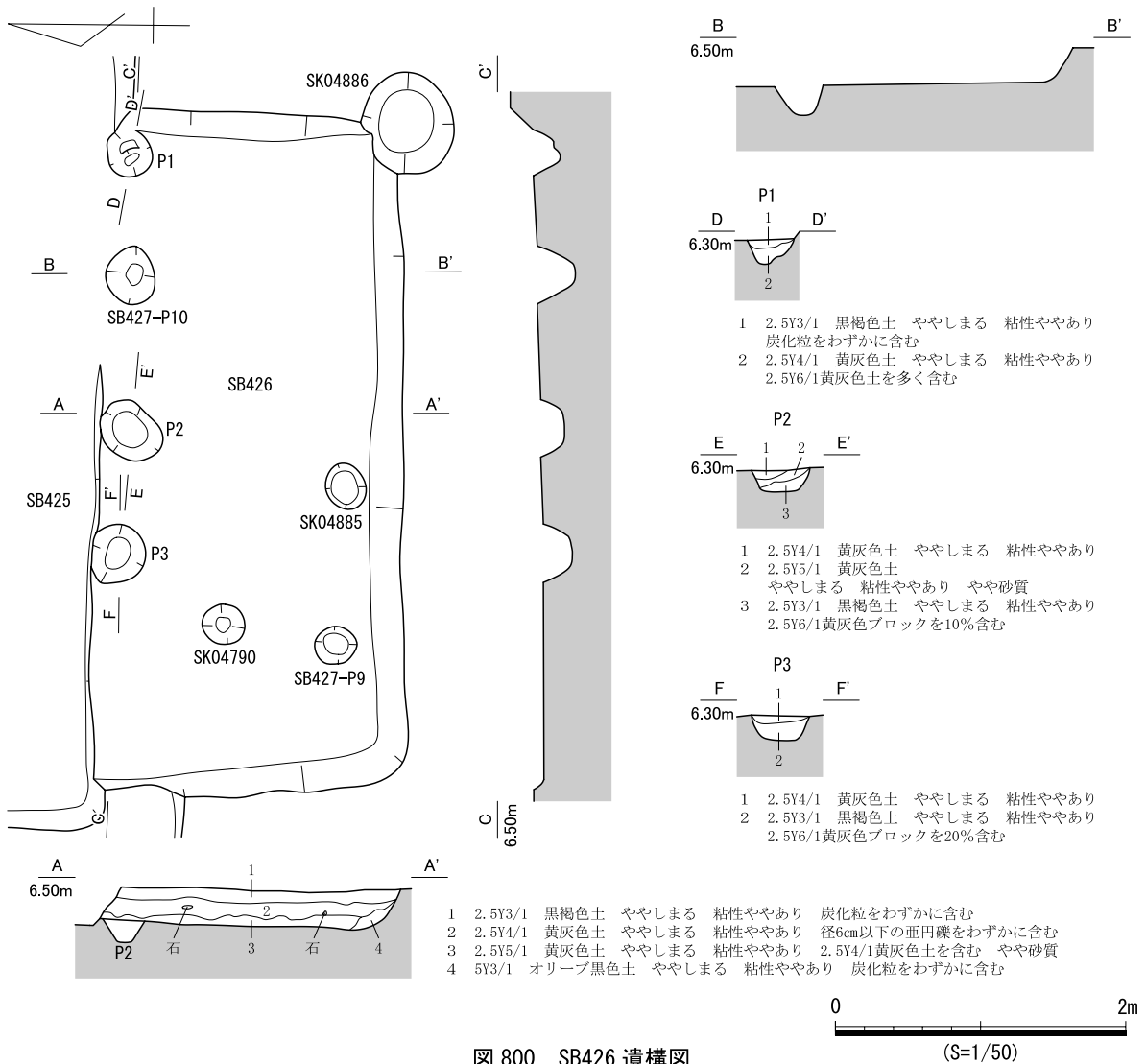
図 800 SB426 遺構図
