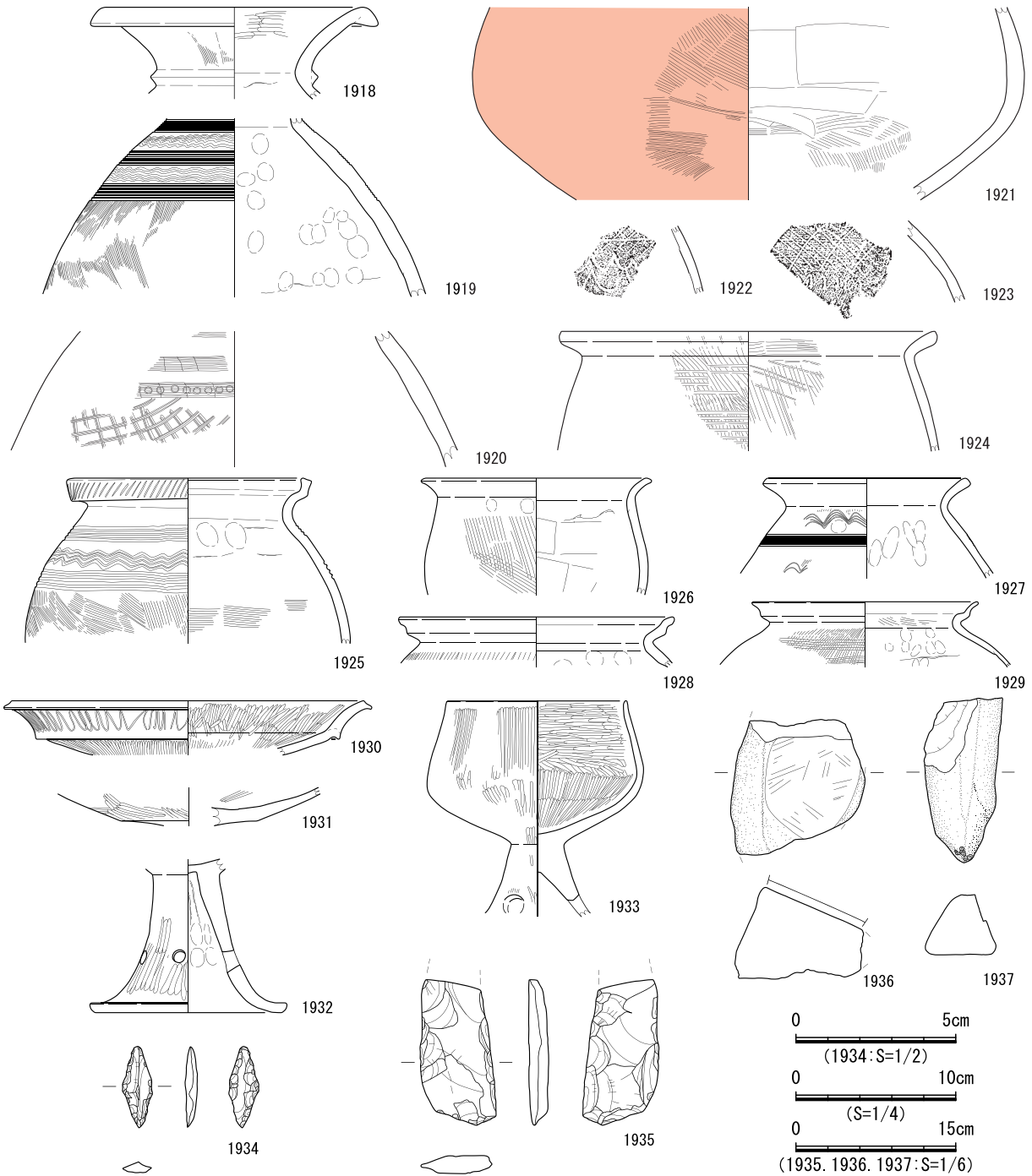
図 743 SB404 遺物実測図
