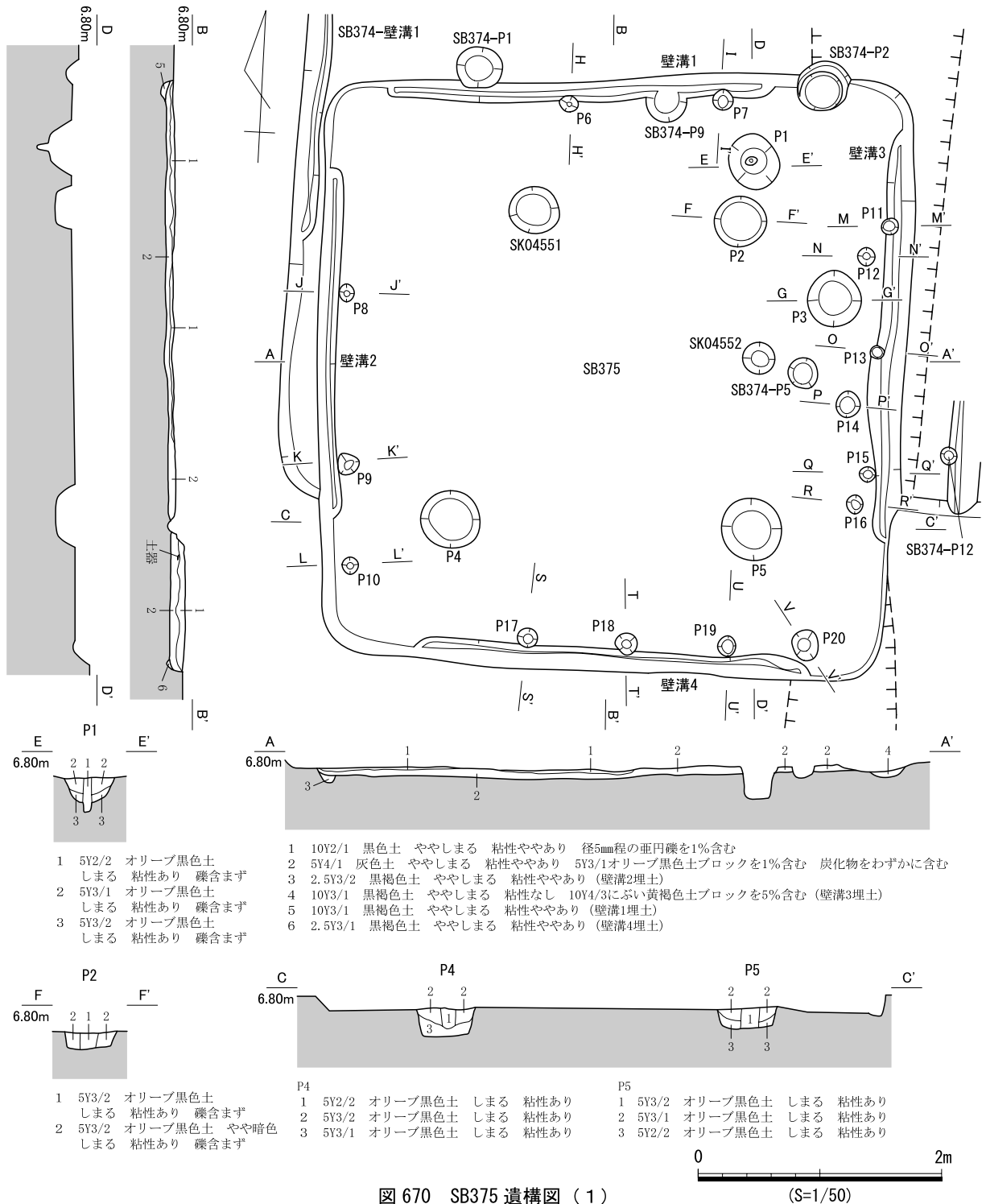
図 670 SB375 遺構図 (1)
