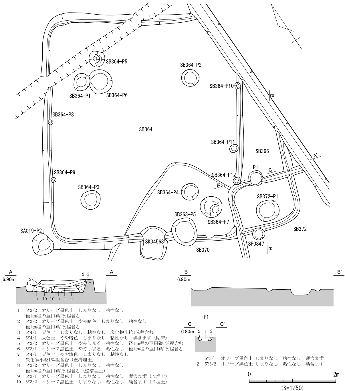
図 650 SB366 遺構図
