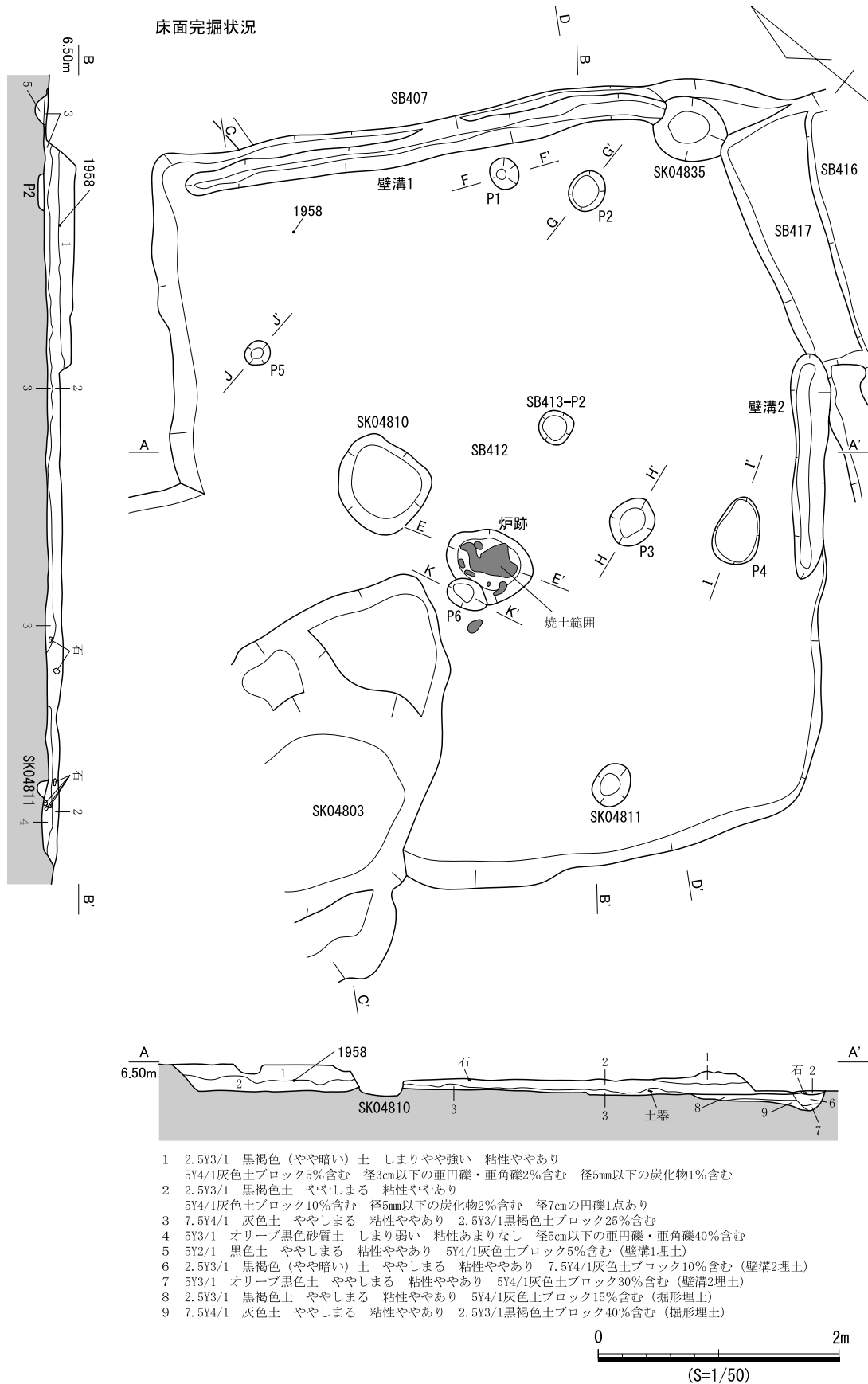
図 761 SB412 遺構図 (1)
