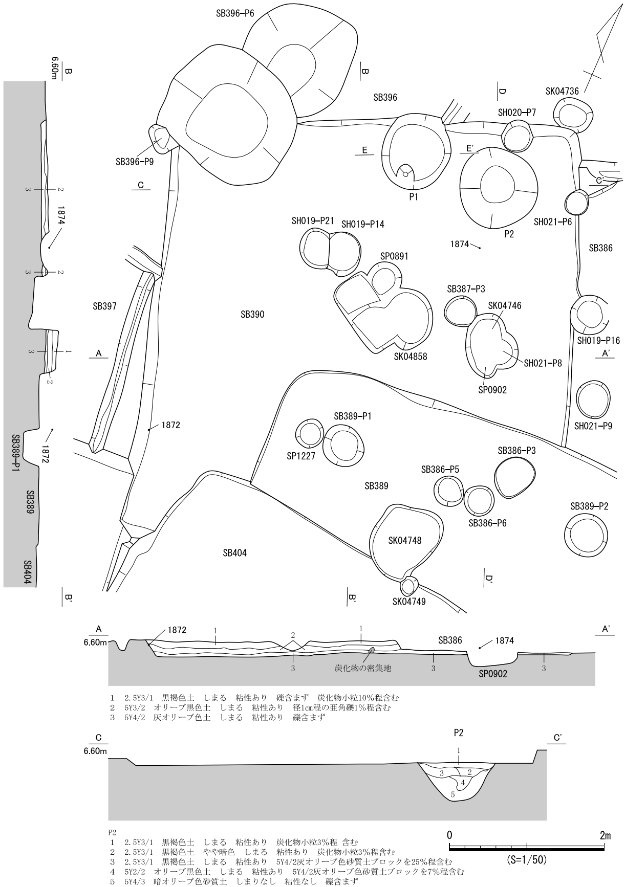
図 709 SB390 遺構図 (1)
