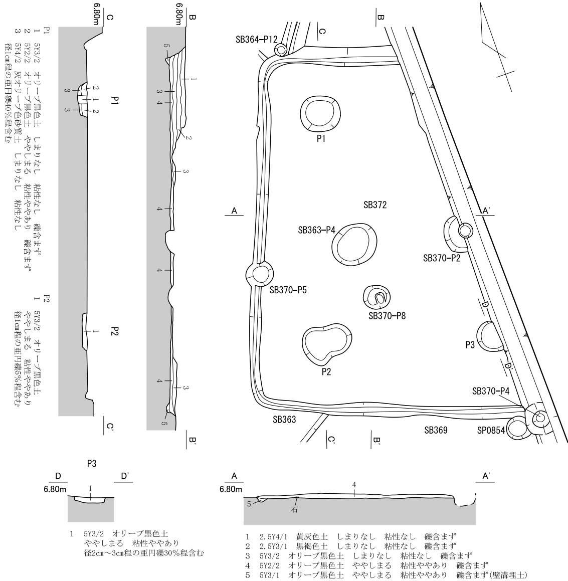
図 662 SB372 遺構図
