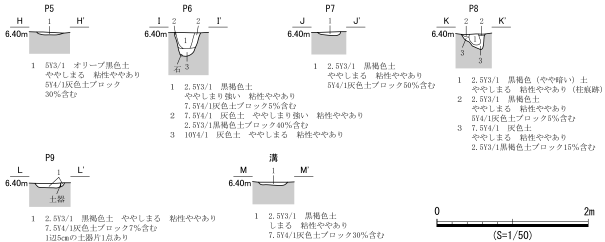
図 770 SB415 遺構図 (2)
