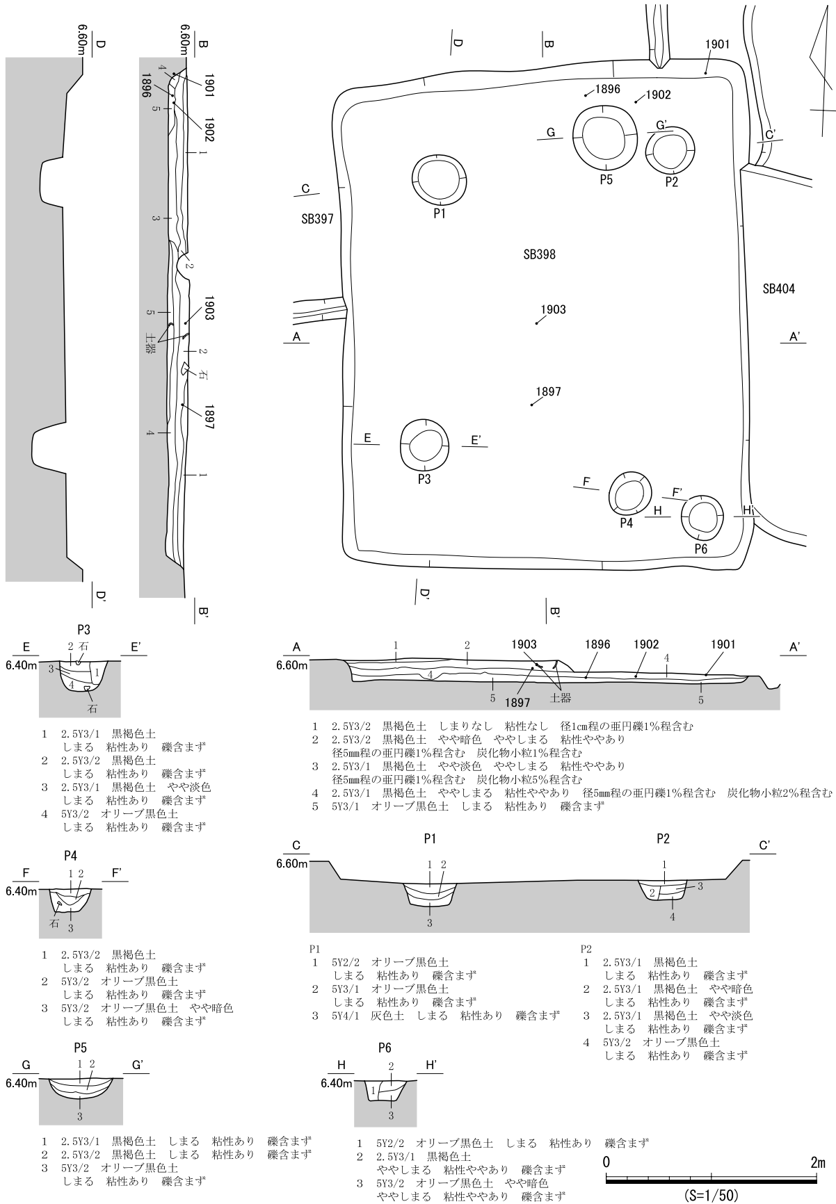
図 729 SB398 遺構図
