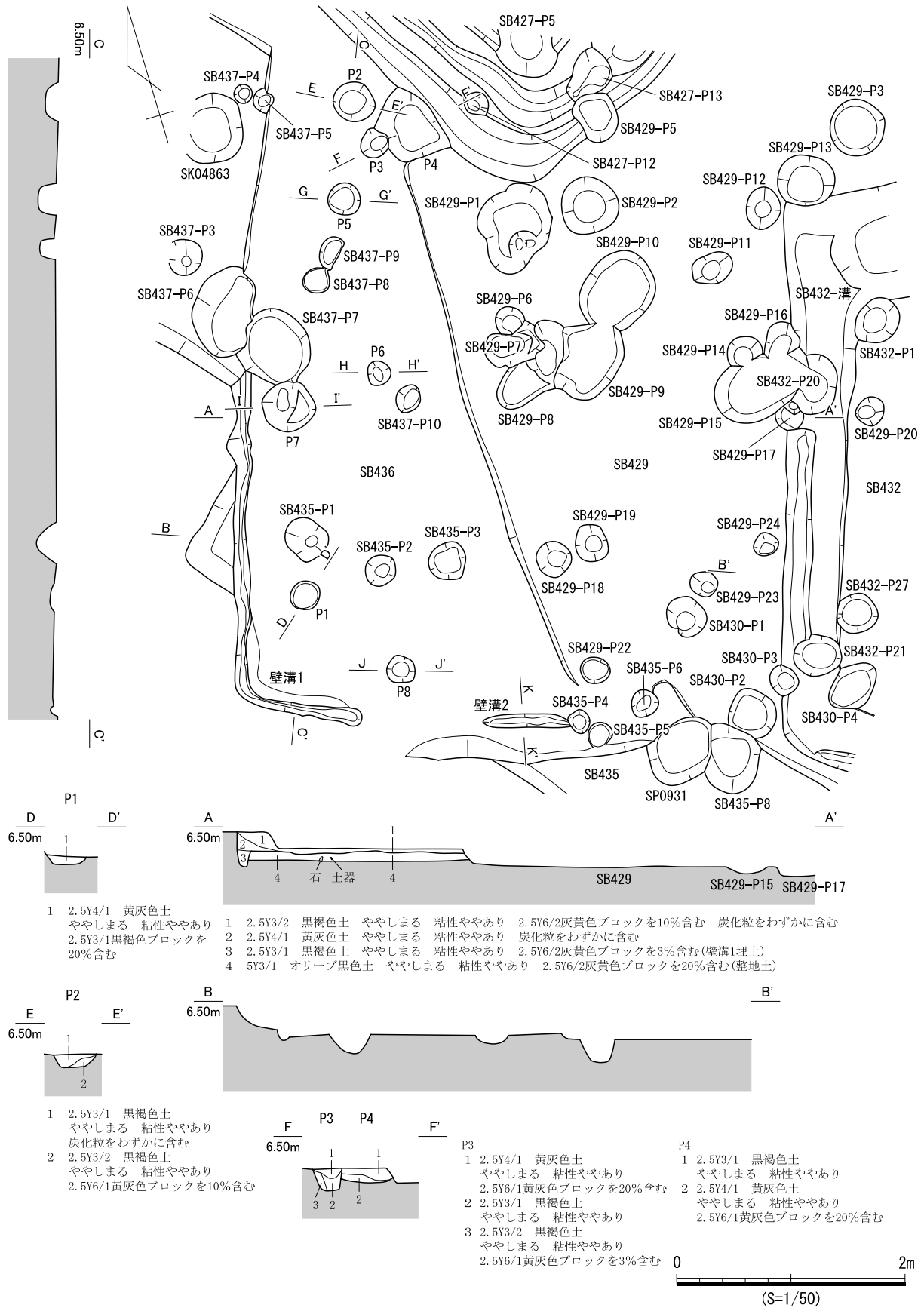
図 828 SB436 遺構図 (1)
