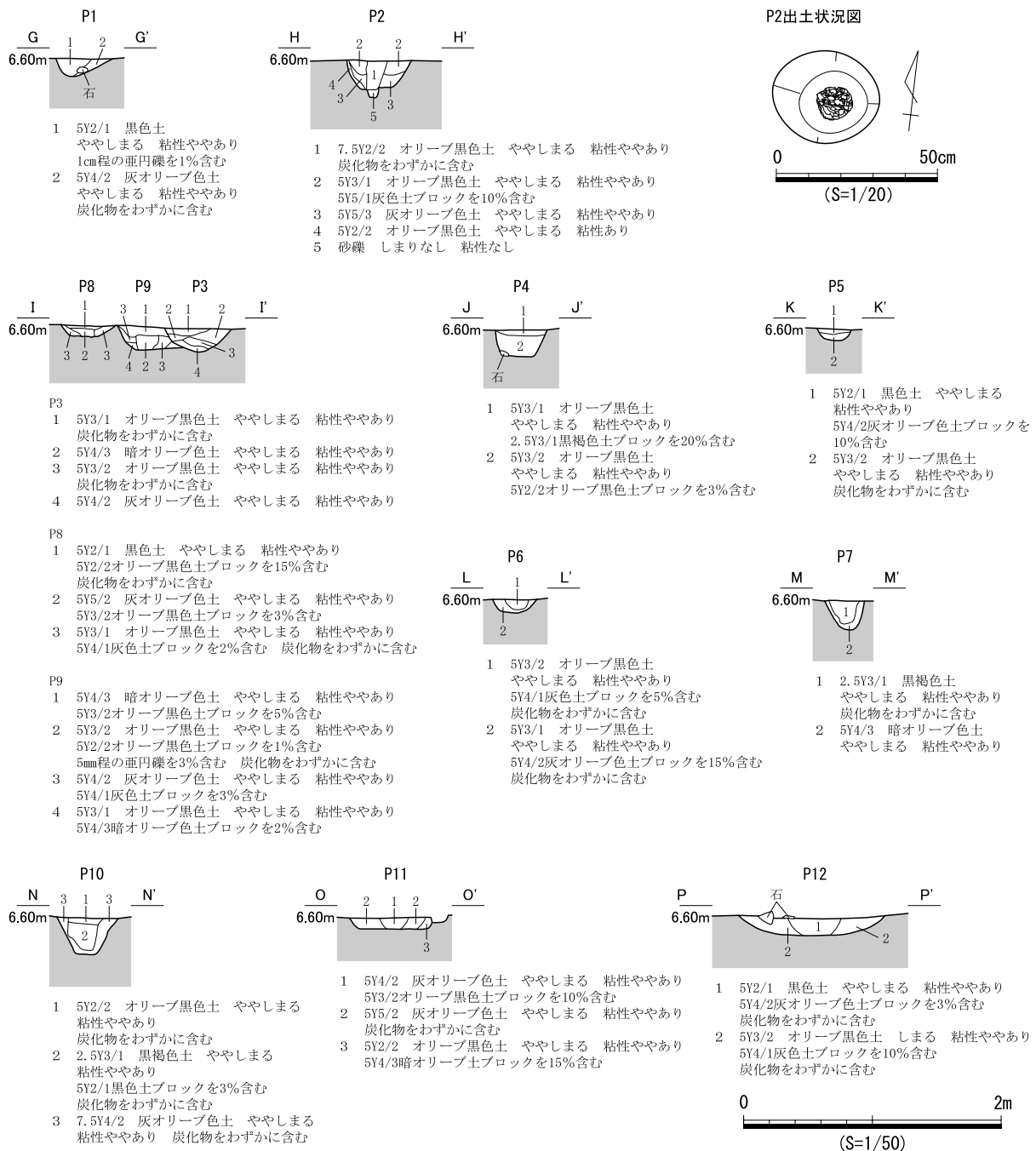
図 633 SB360 遺構図 (2)
