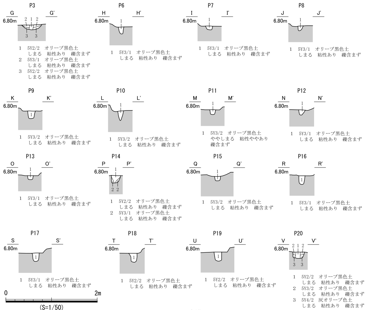
図 672 SB375 遺構図 (2)
