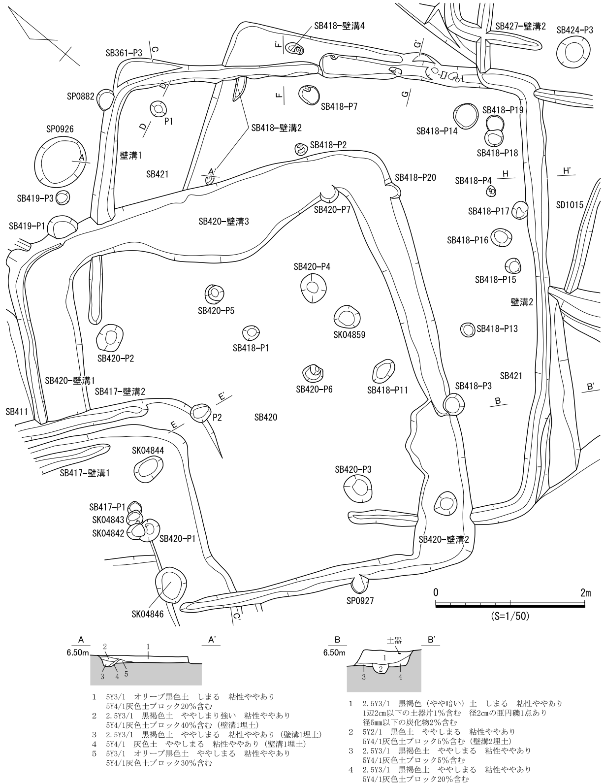
図 787 SB421 遺構図 (1)
