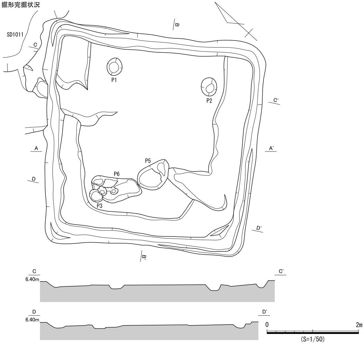
図 790 SB422 遺構図 (2)
