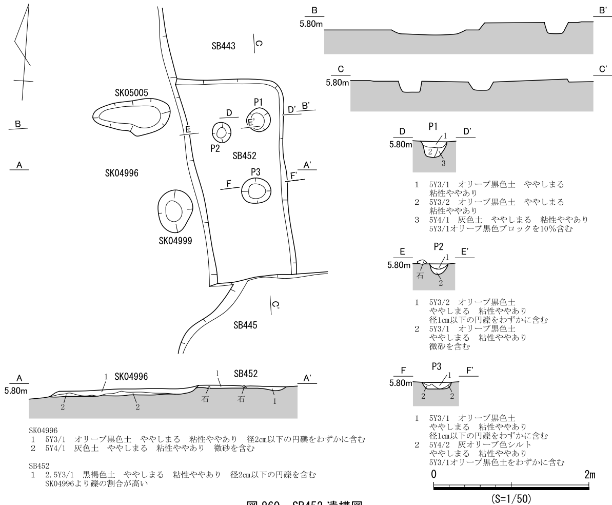
図 860 SB452 遺構図
