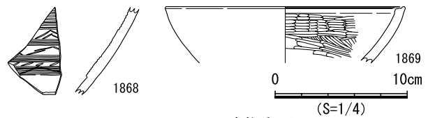
図705 SB388 遺物実測図
