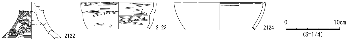
図 851 SB448 遺物実測図
