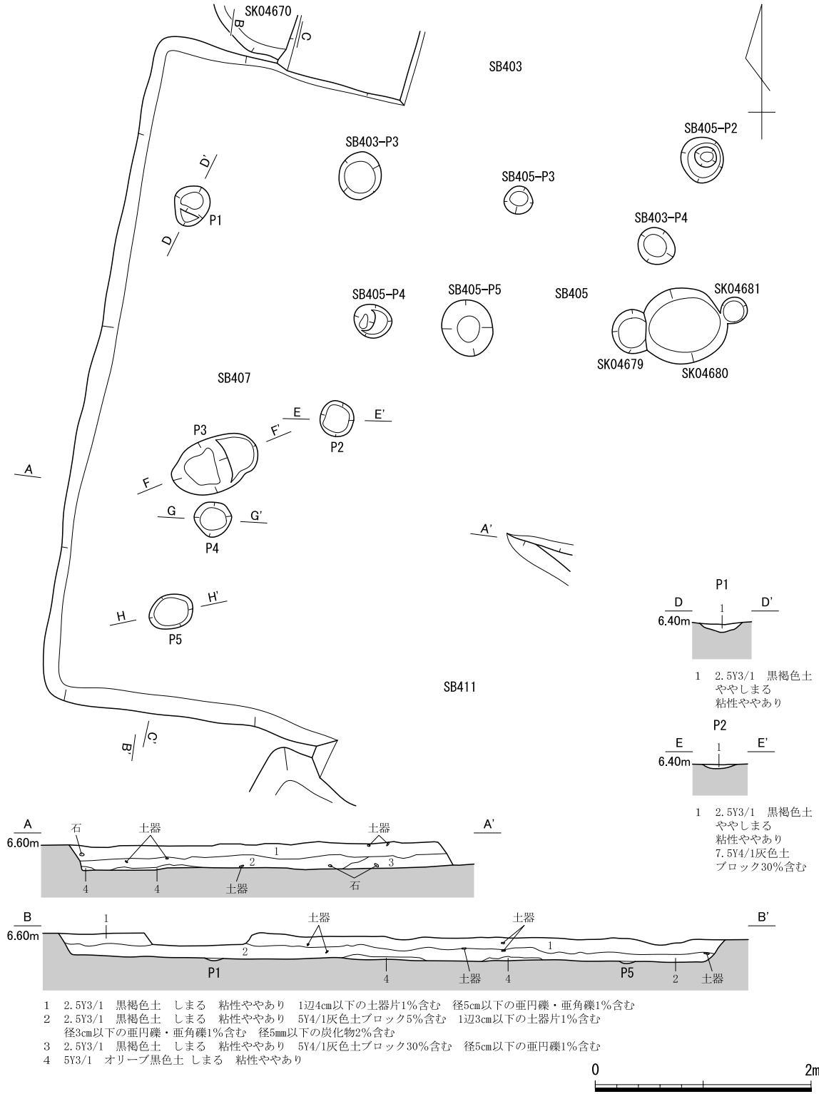
図748 SB407 遺構図(1)
