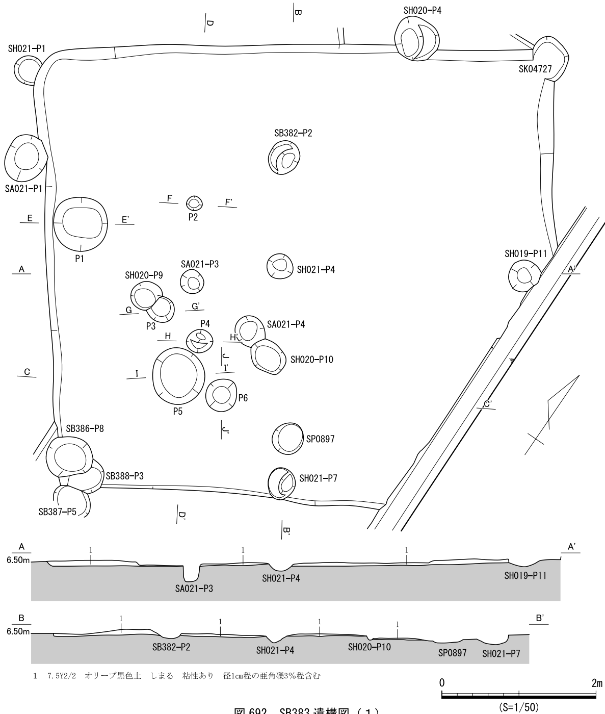
図 692 SB383 遺構図 (1)
