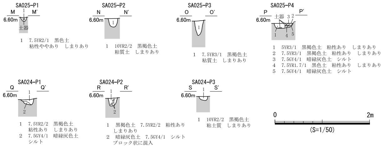
図 794 SB423 遺構図 (2)
