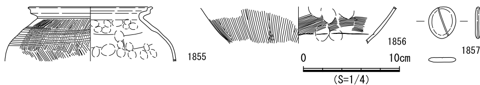
図 690 SB382 遺物実測図
