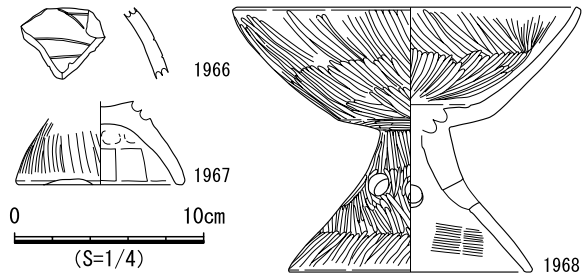
図 774 SB416 遺物実測図
