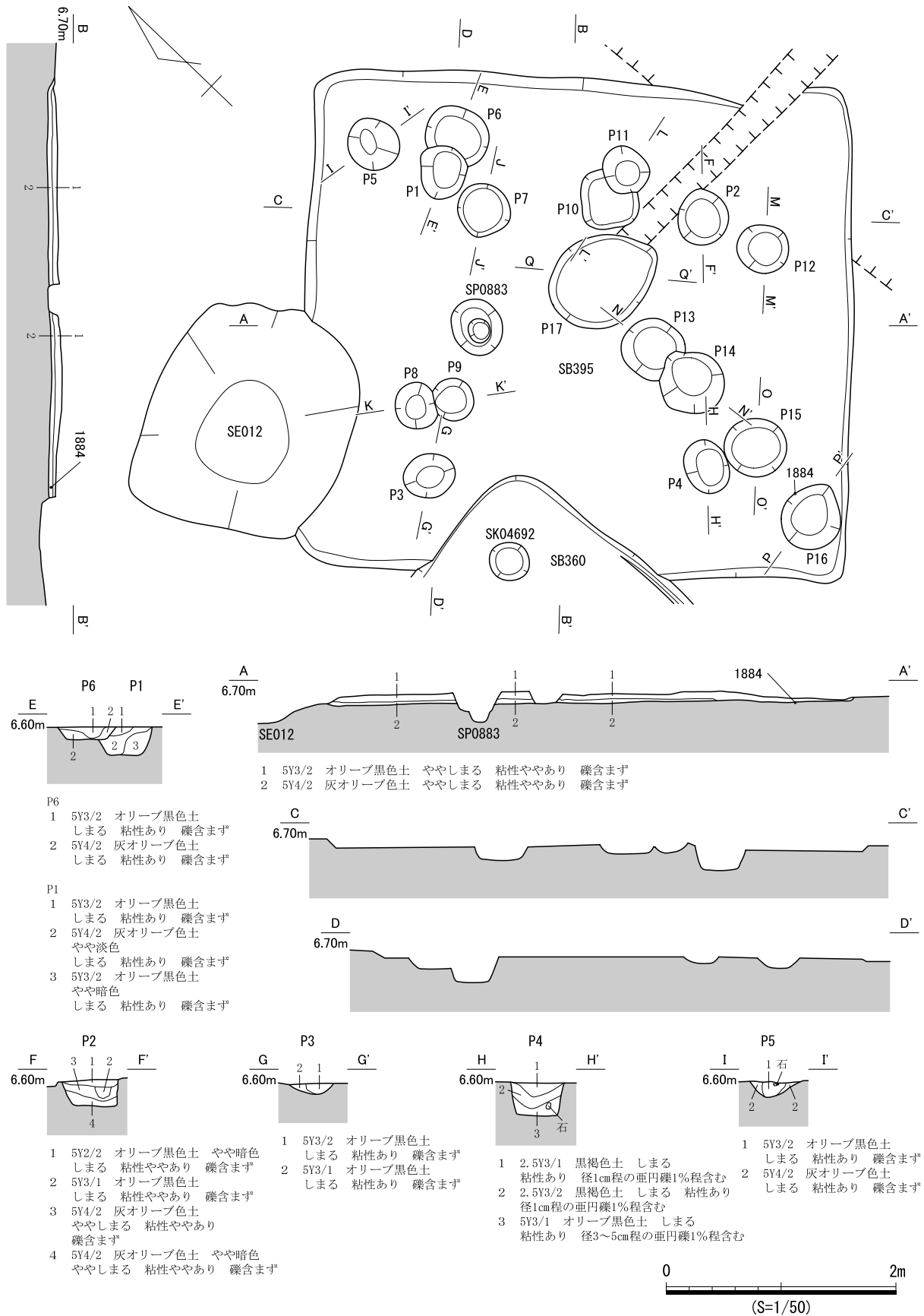
図 722 SB395 遺構図 (1)
