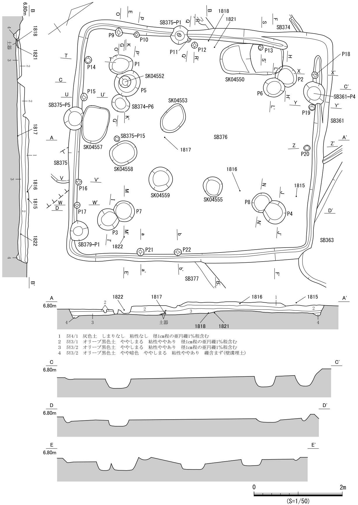
図 674 SB376 遺構図 (1)
