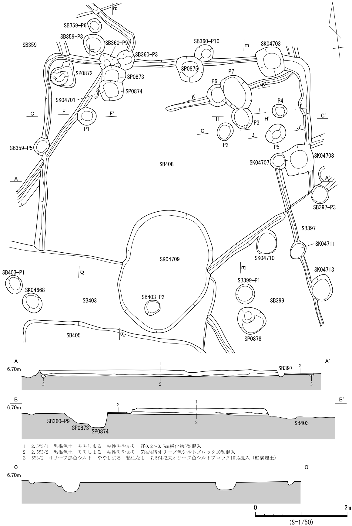
図 751 SB408 遺構図 (1)
