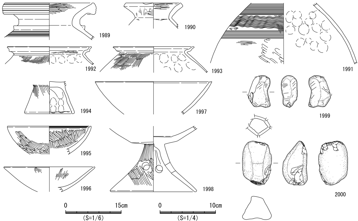
図 795 SB424 遺物実測図
