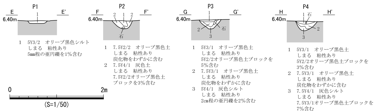
図 624 SB356 遺構図 (2)
