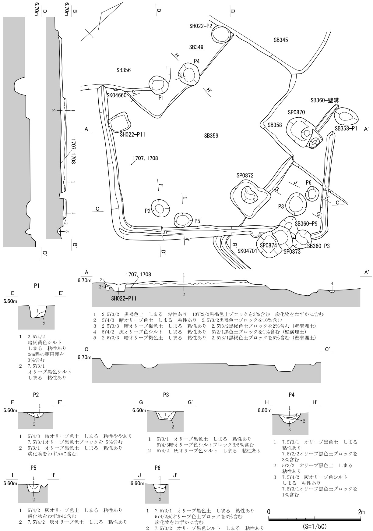
図 631 SB359 遺構図
