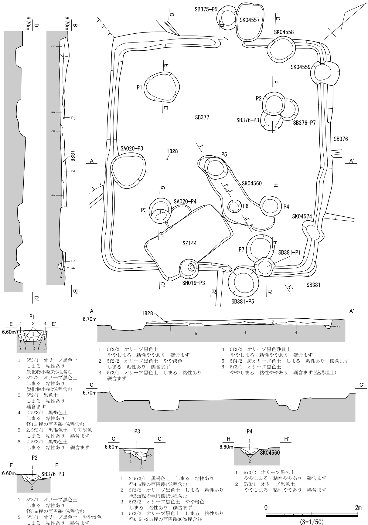
図 677 SB377 遺構図 (1)
