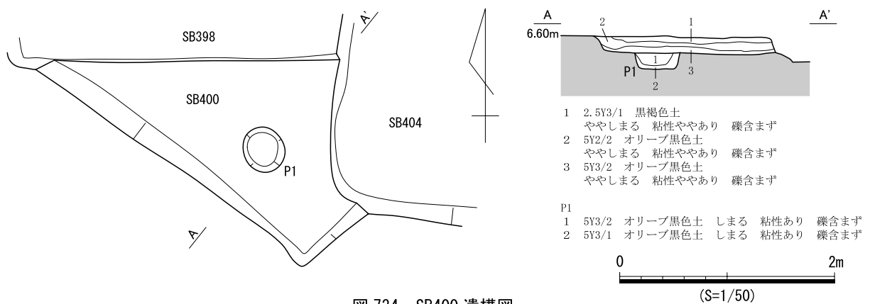
図 734 SB400 遺構図
