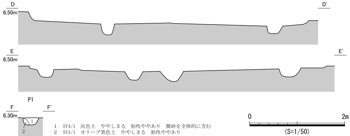
図 807 SB428 遺構図 (2)
