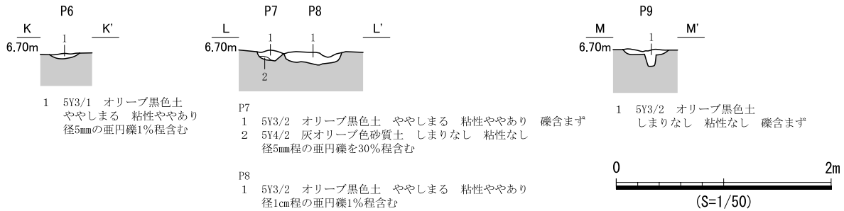
図 665 SB373 遺構図(2)
