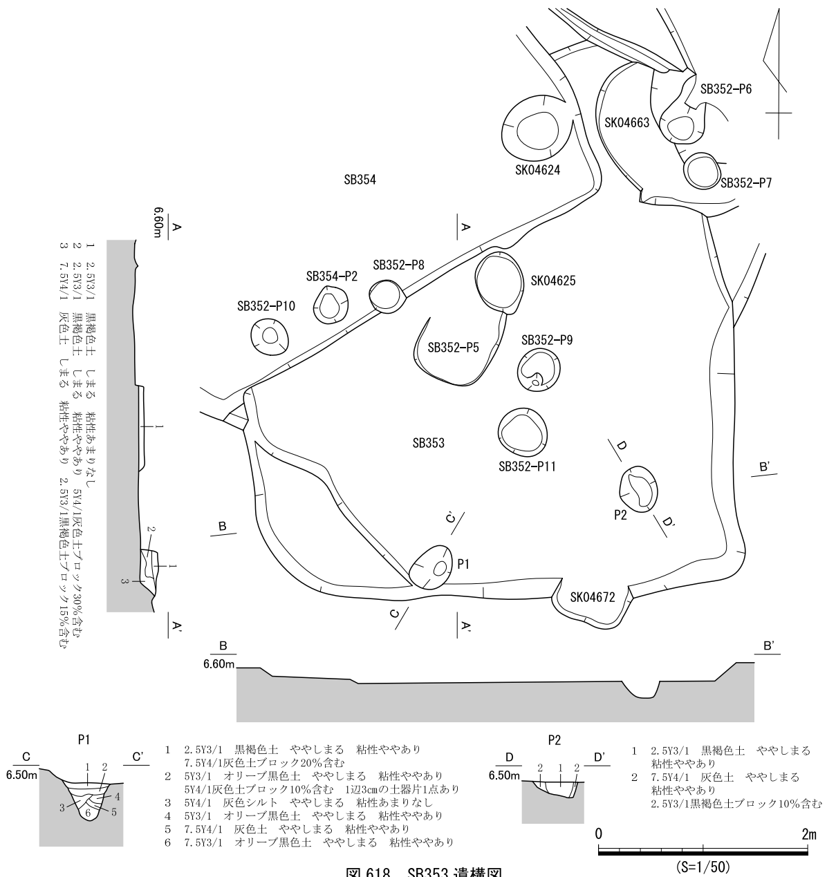
図 618 SB353 遺構図
