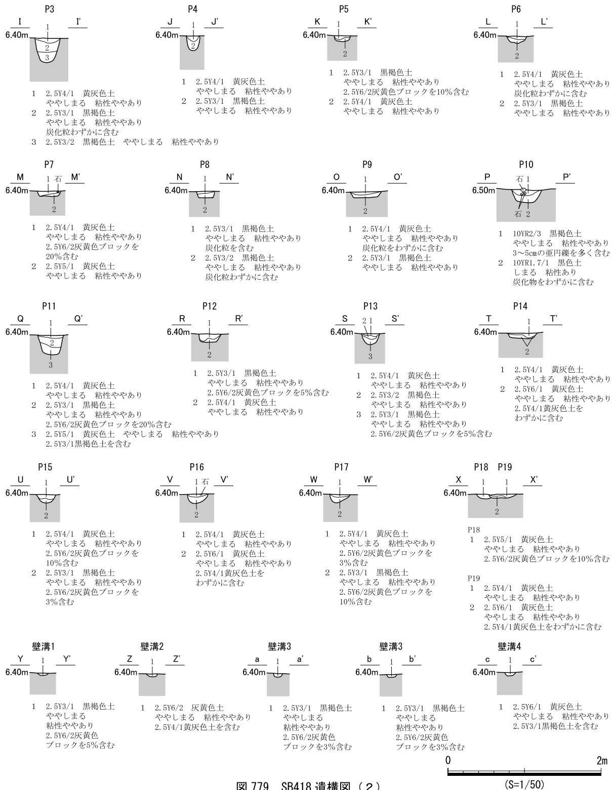
図 779 SB418 遺構図 (2)
