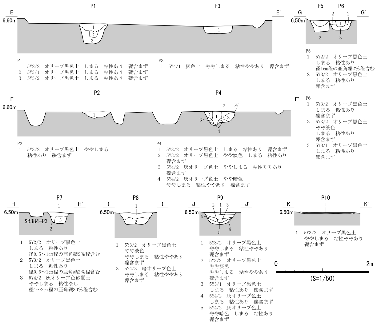
図701 SB386 遺構図(2)
