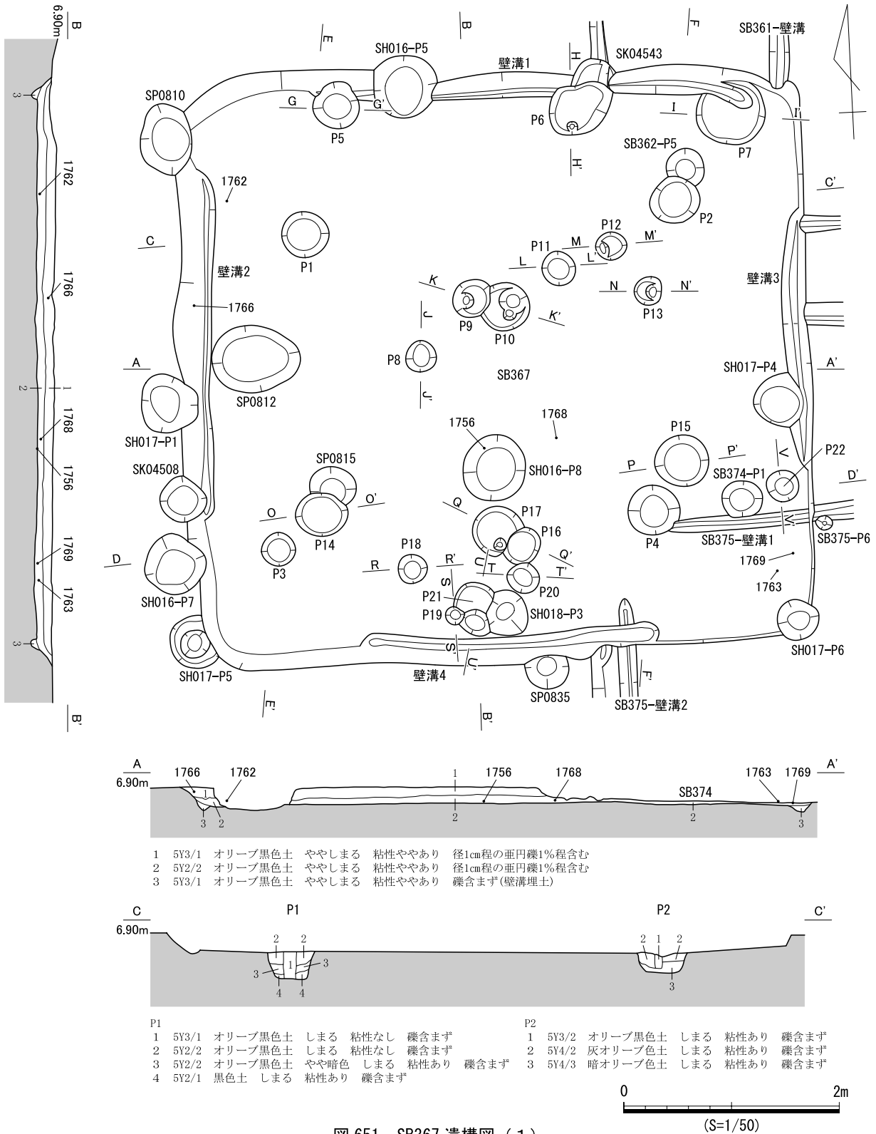
図 651 SB367 遺構図 (1)
