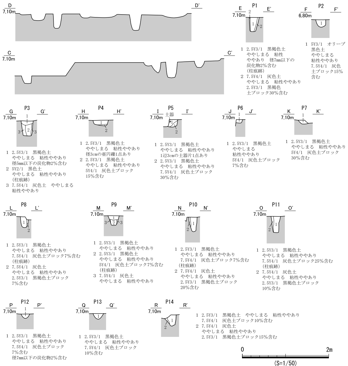
図 865 SB454 遺構図 (2)
