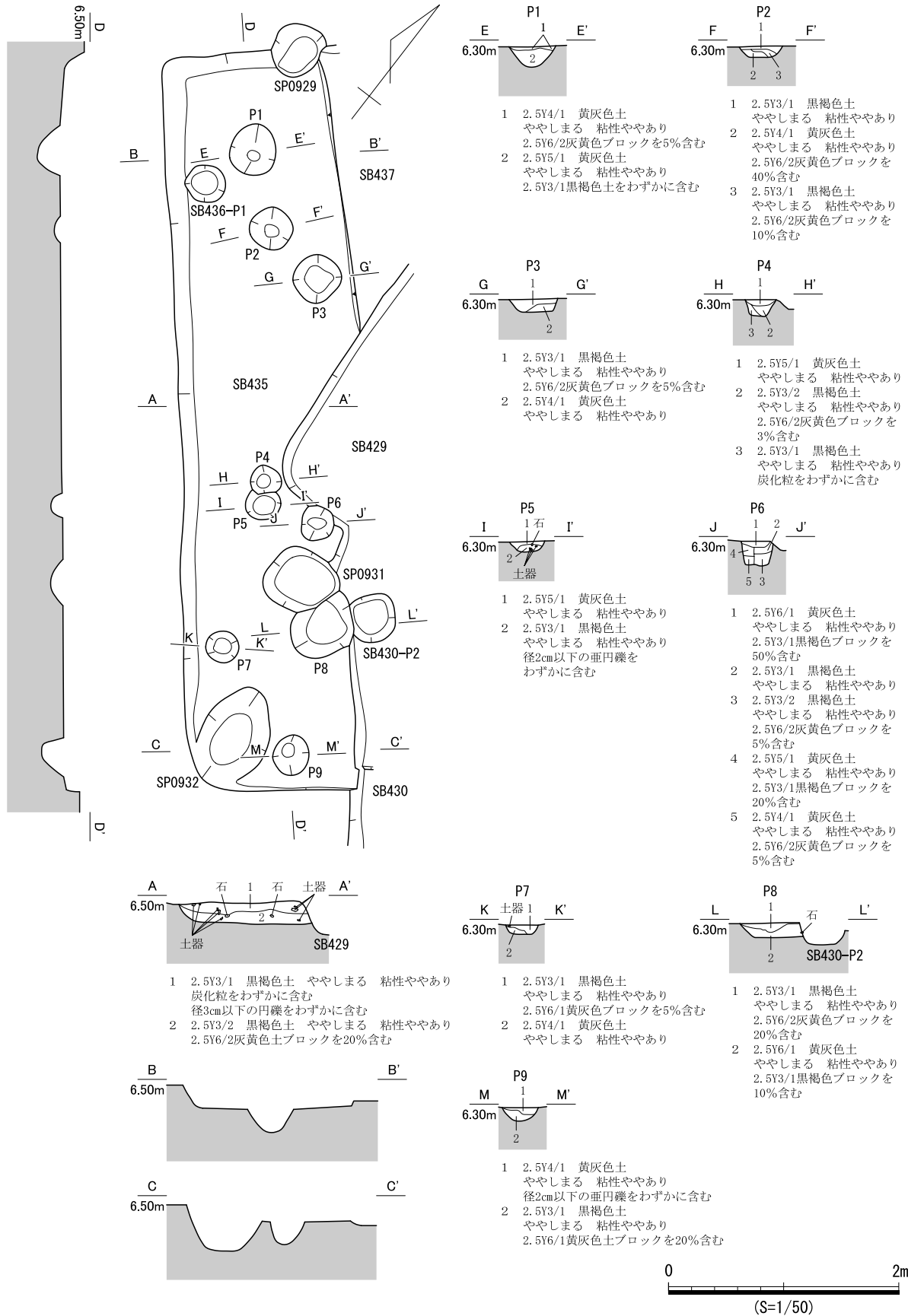
図 827 SB435 遺構図
