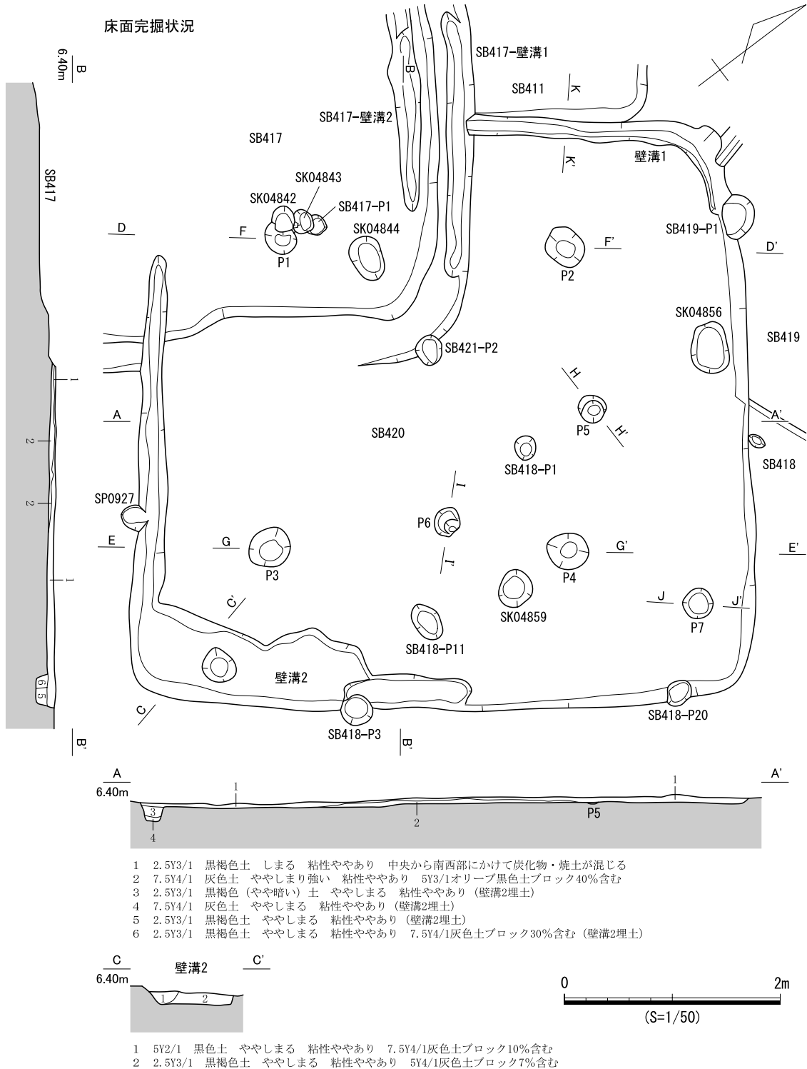
図783 SB420 遺構図(1)
