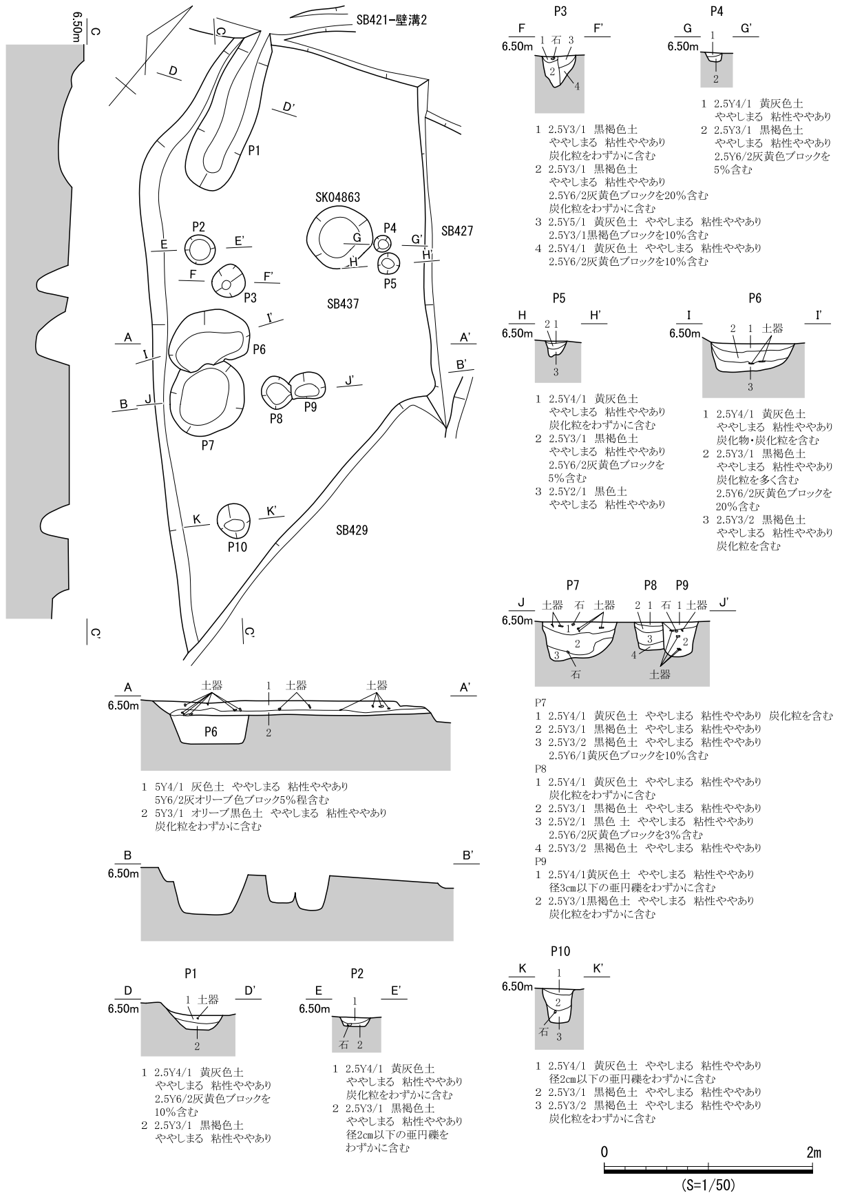
図 831 SB437 遺構図
