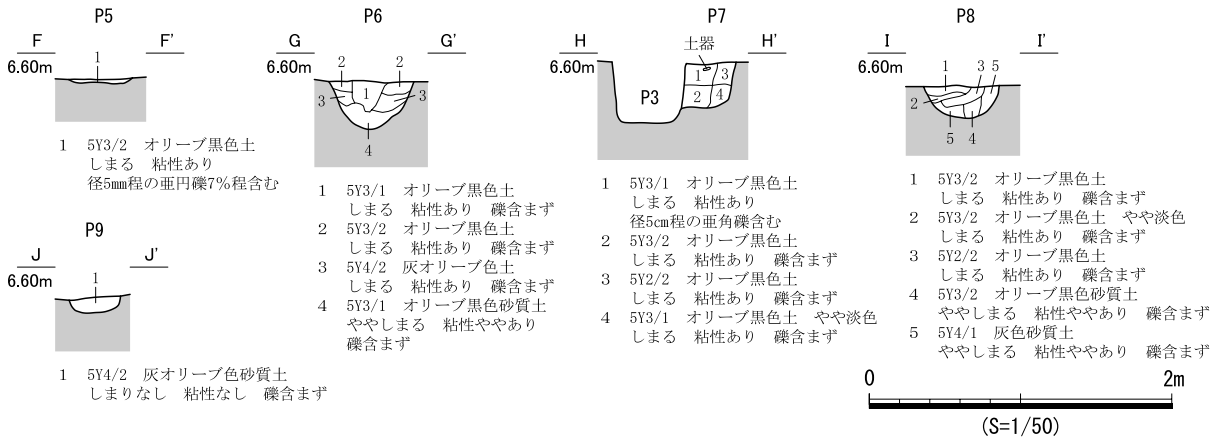
図 681 SB378 遺構図 (2)
