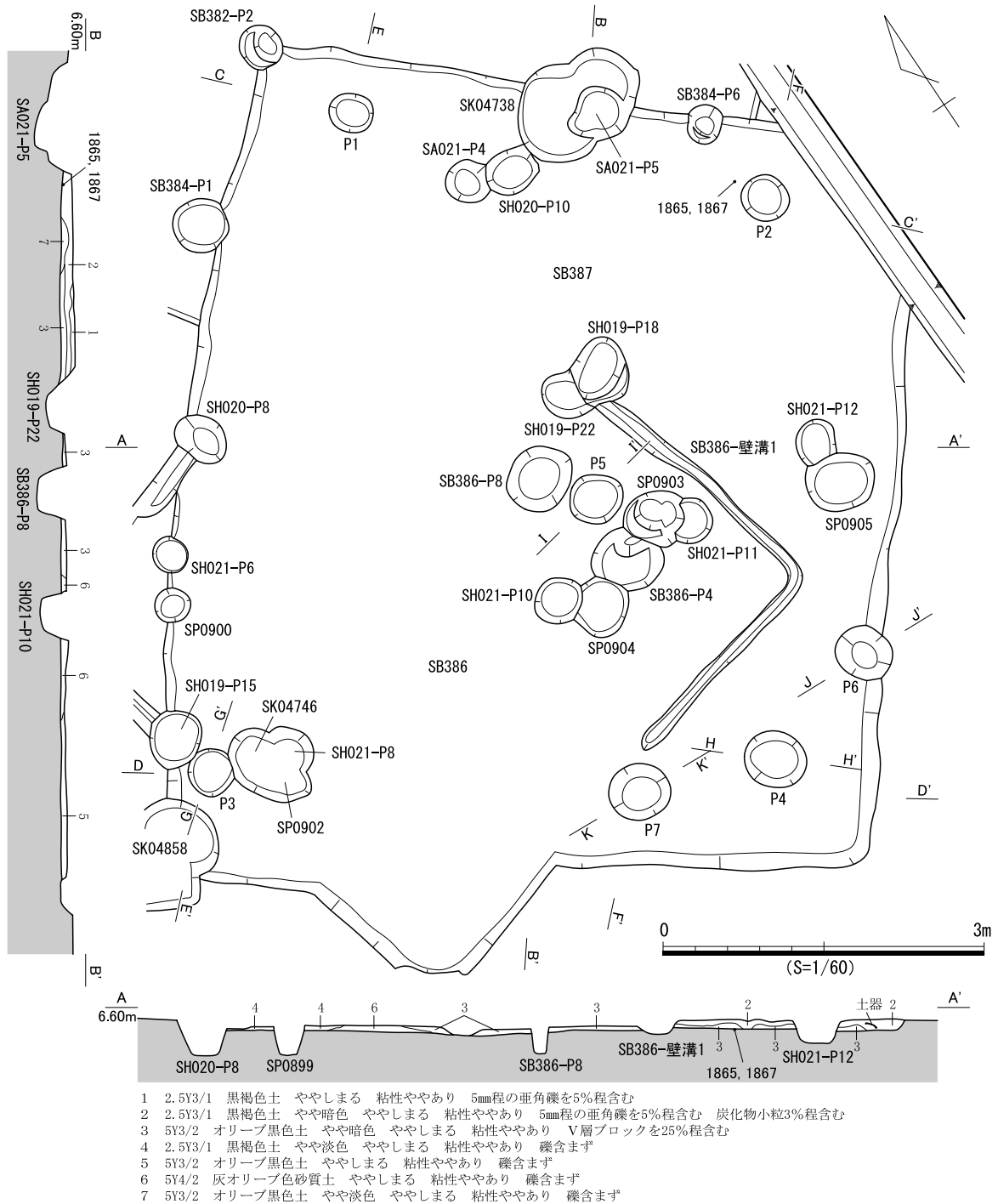
図702 SB387遺構図(1)
