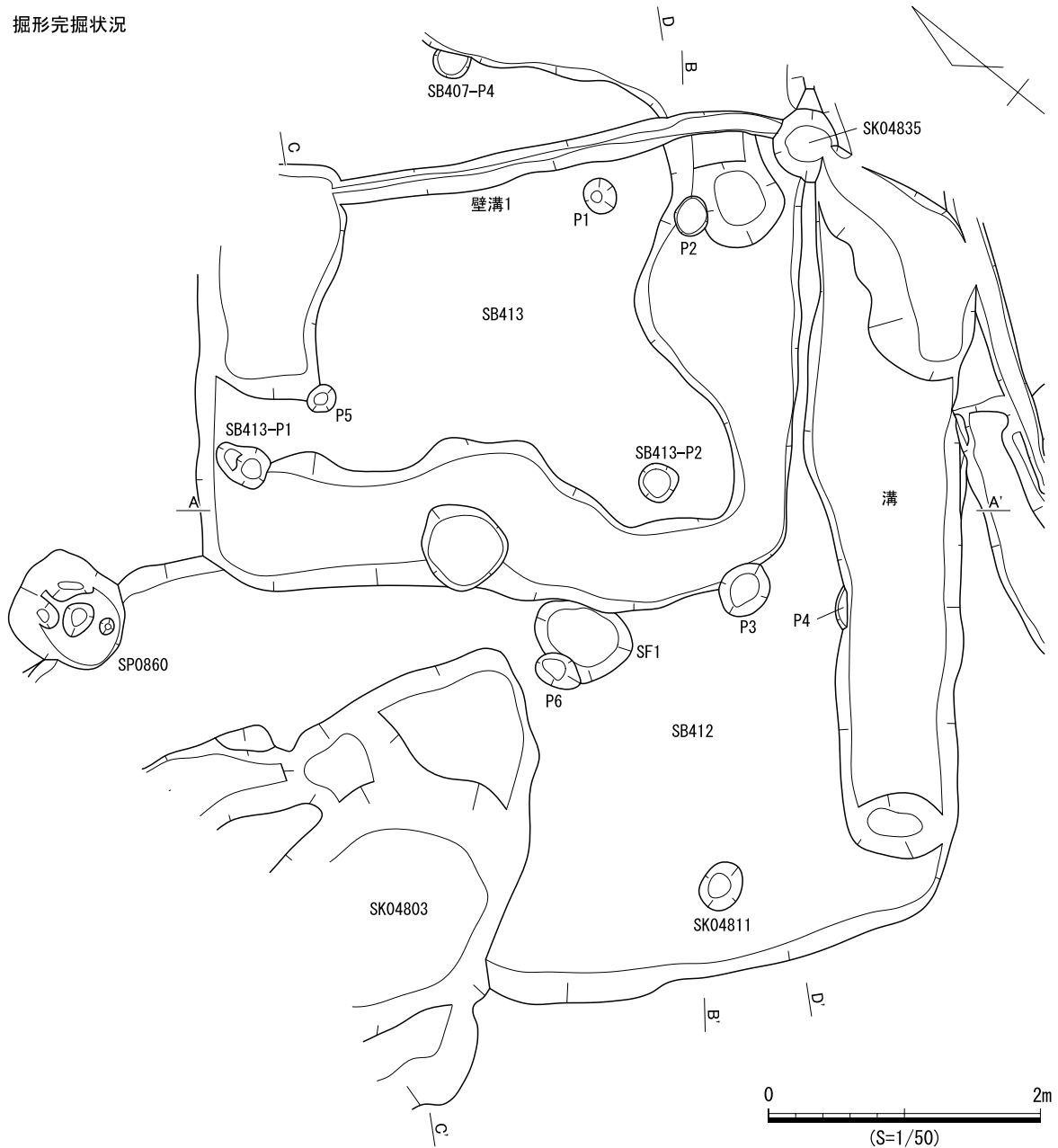
図 764 SB412 遺構図 (3)
