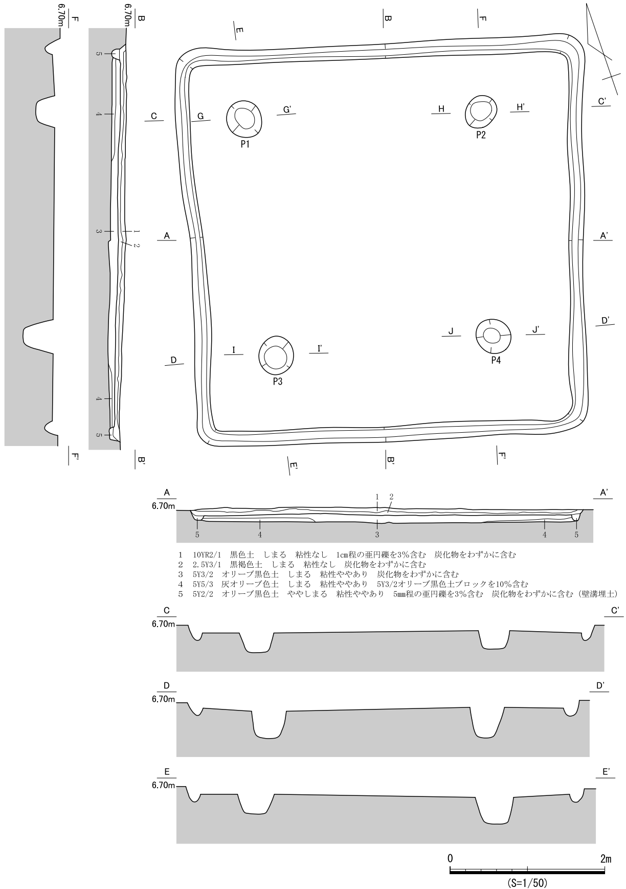
図 739 SB403 遺構図 (1)
