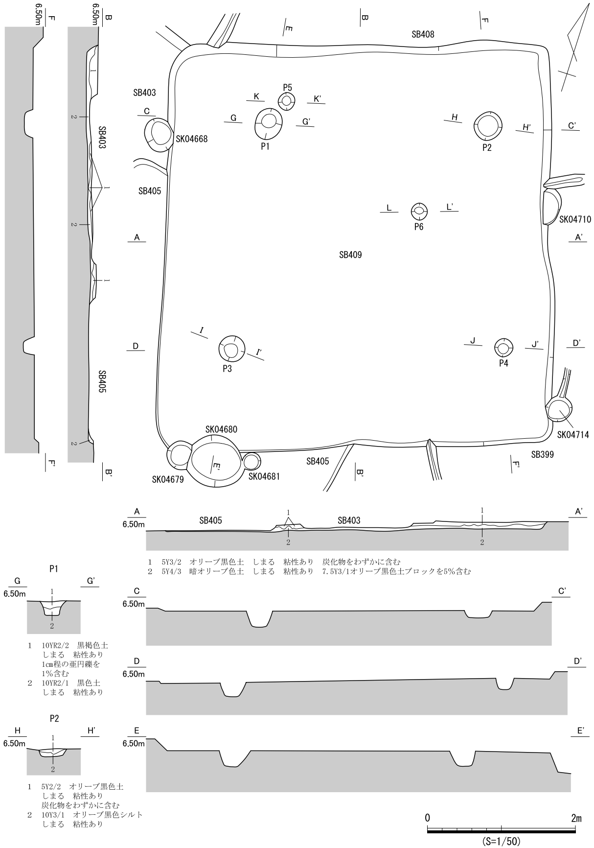
図 754 SB409 遺構図 (1)
