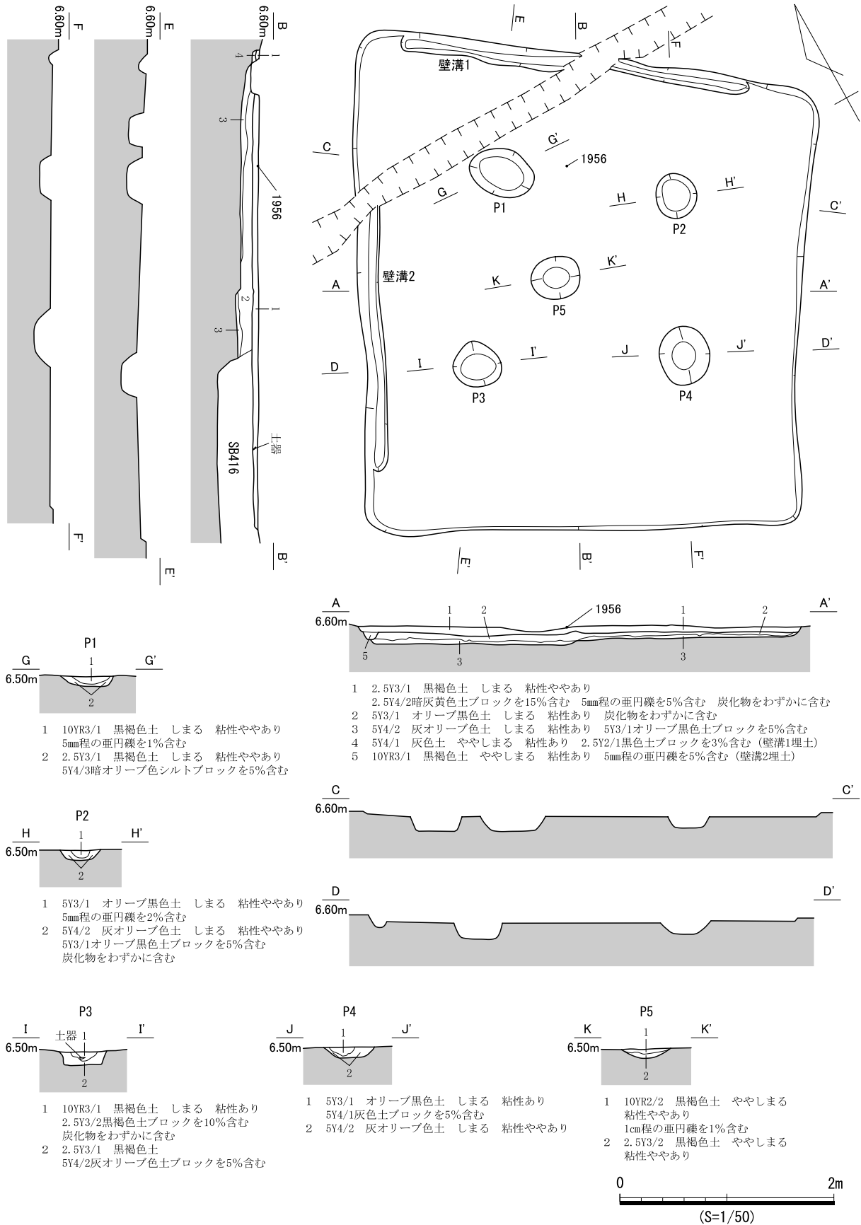
図 760 SB416 遺構図
