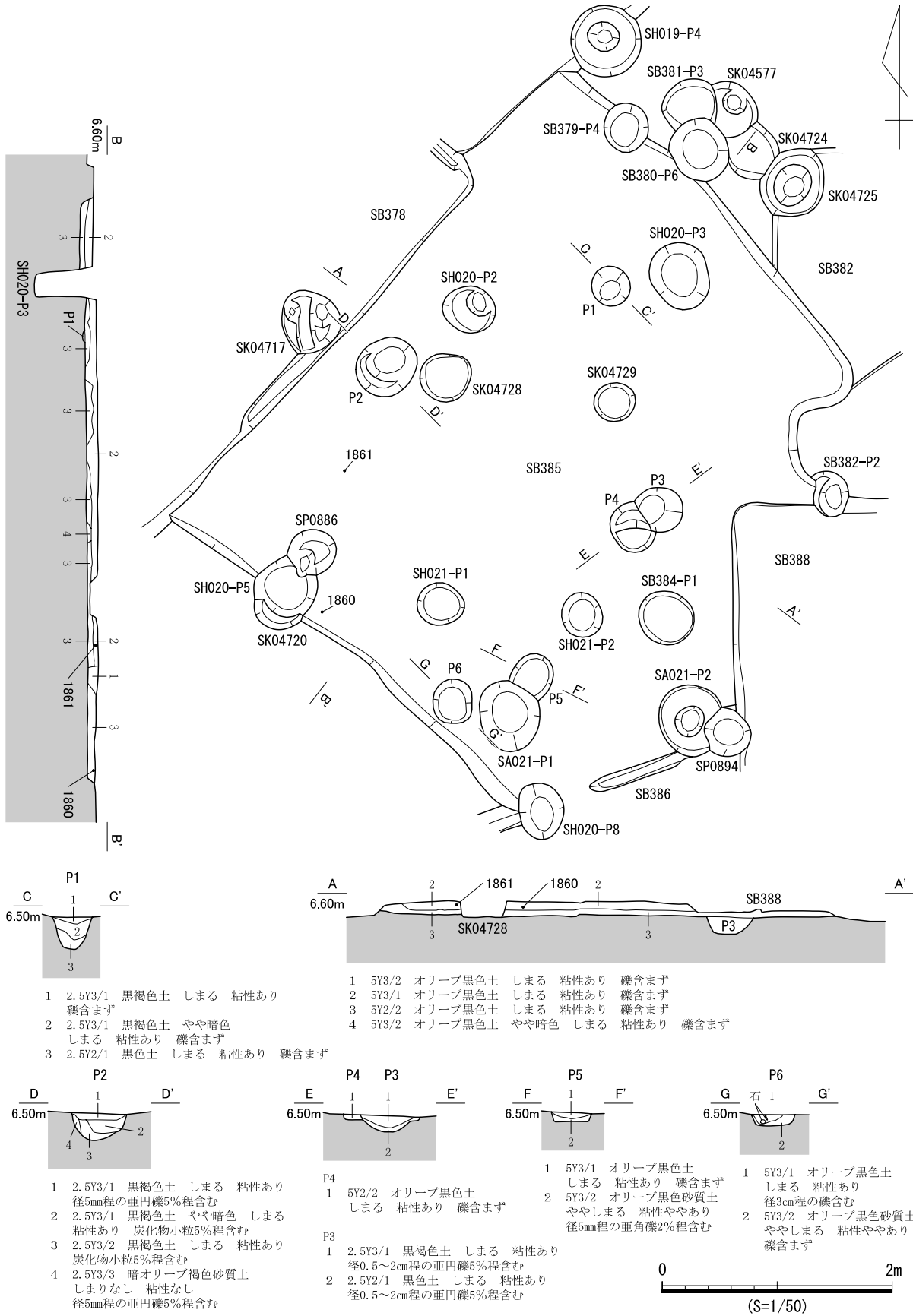
図 698 SB385 遺構図
