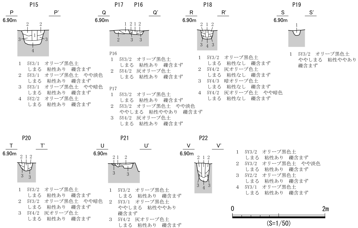
図 653 SB367 遺構図 (3)
