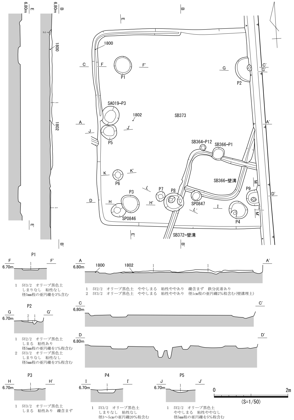
図 664 SB373 遺構図 (1)
