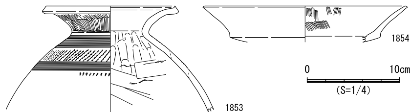
図 687 SB381 遺物実測図
