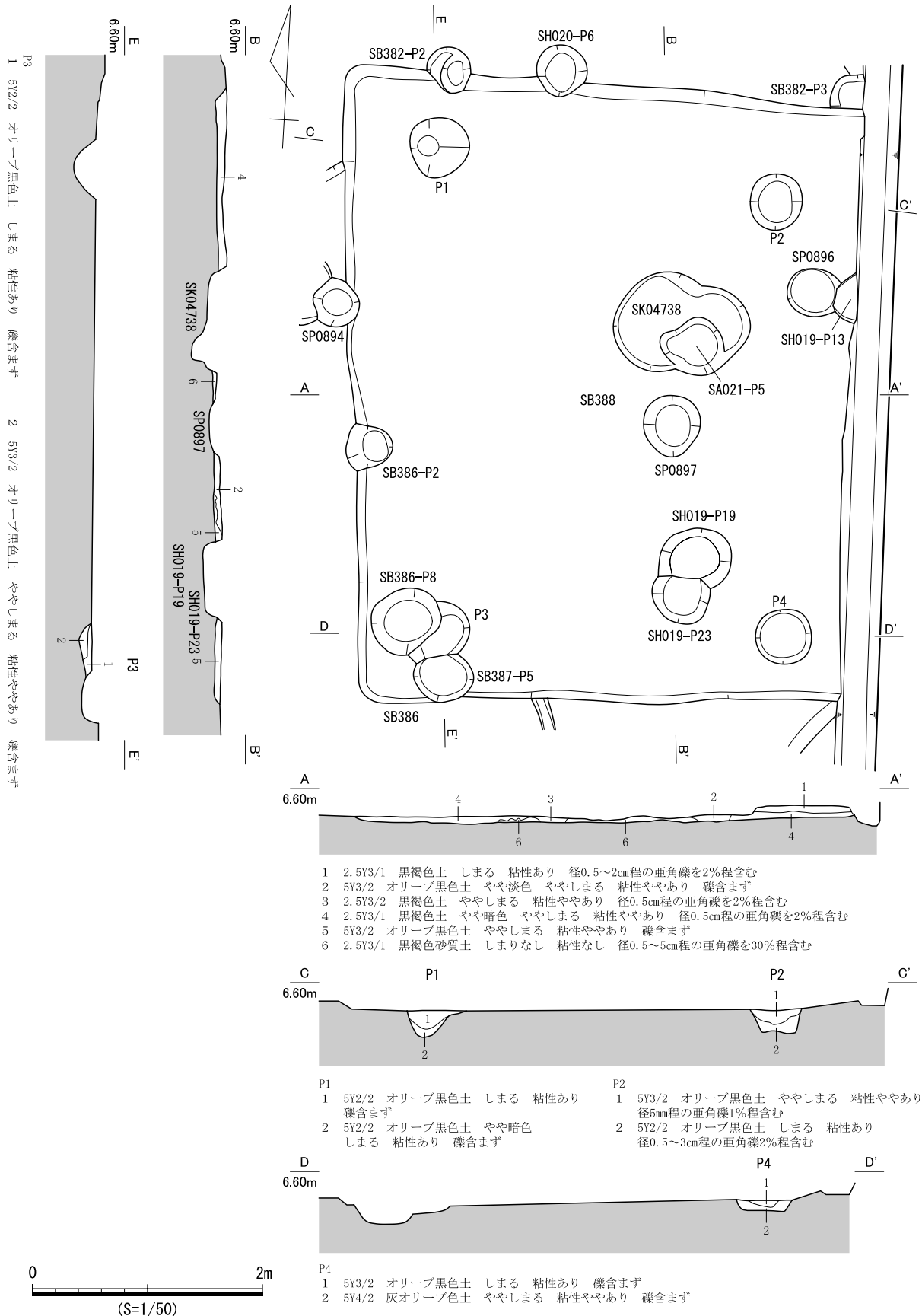
図 707 SB388 遺構図
