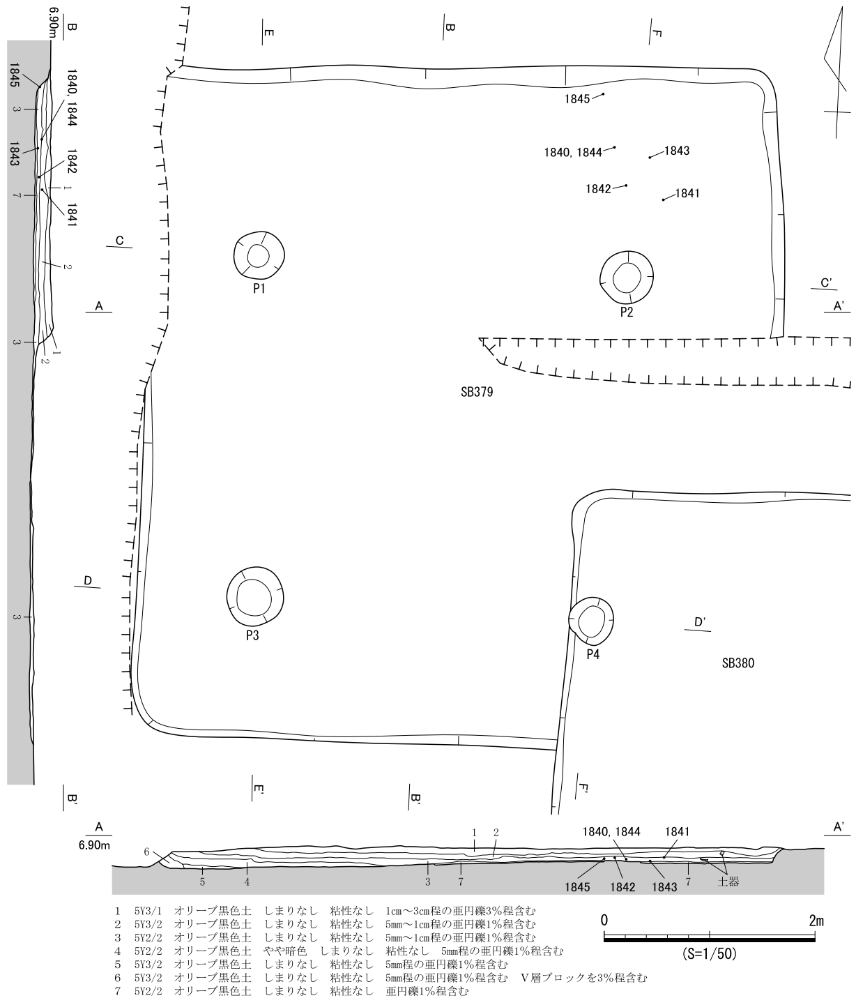
図 683 SB379 遺構図 (1)
