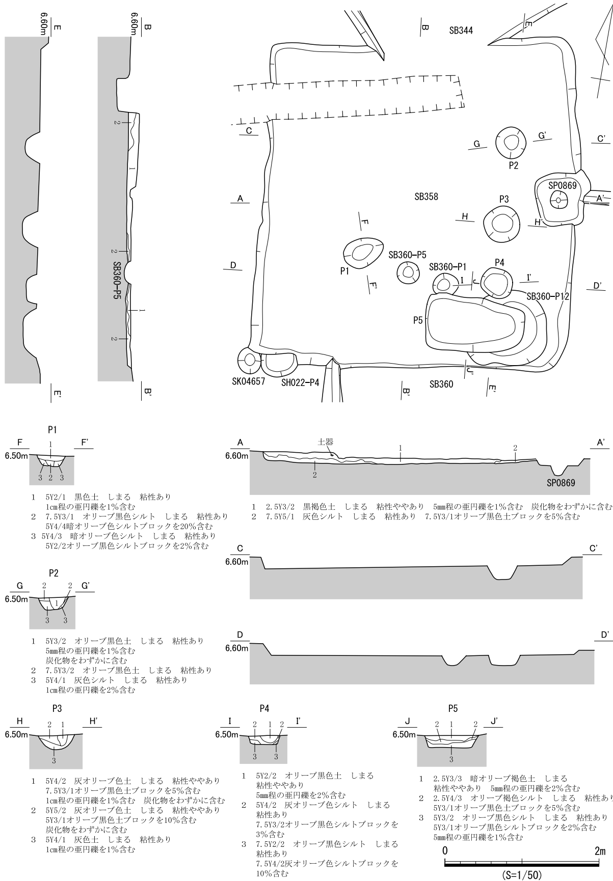
図 628 SB358 遺構図
