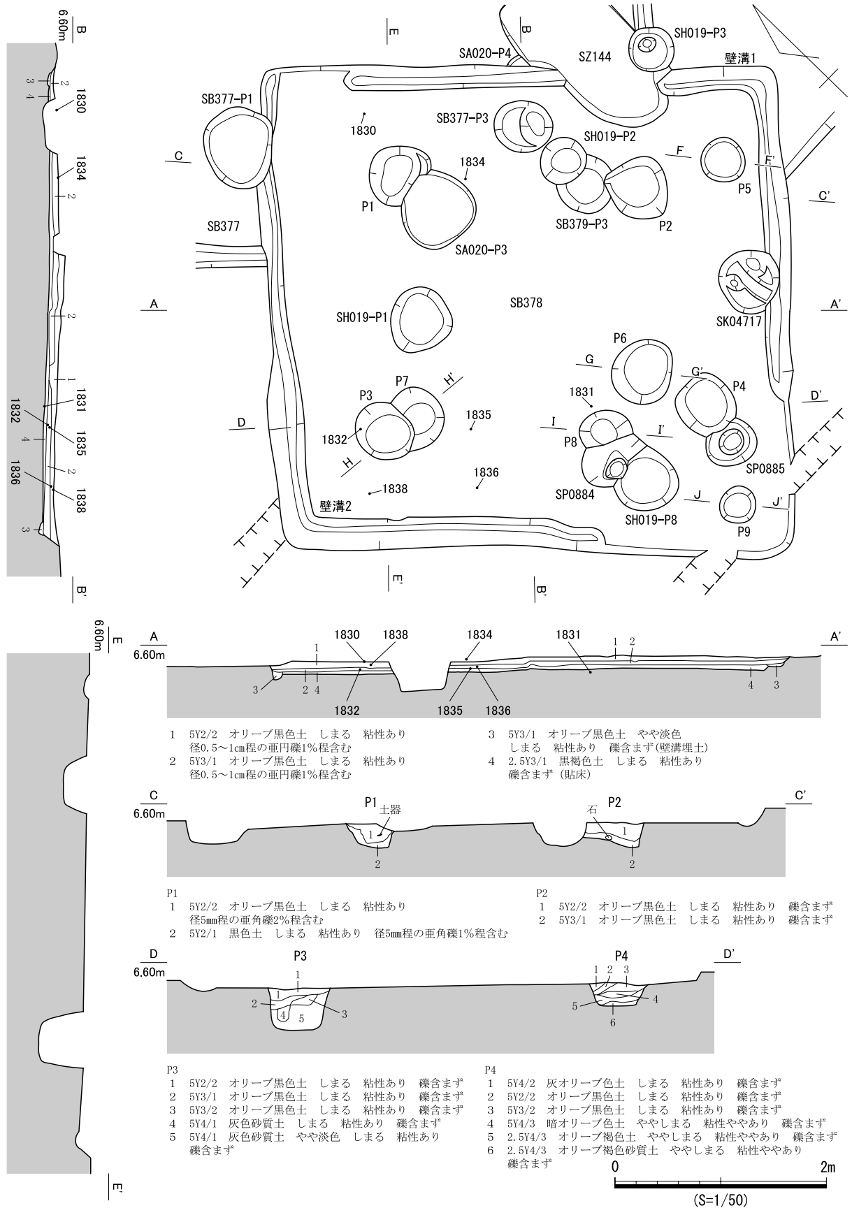
図 680 SB378 遺構図 (1)
