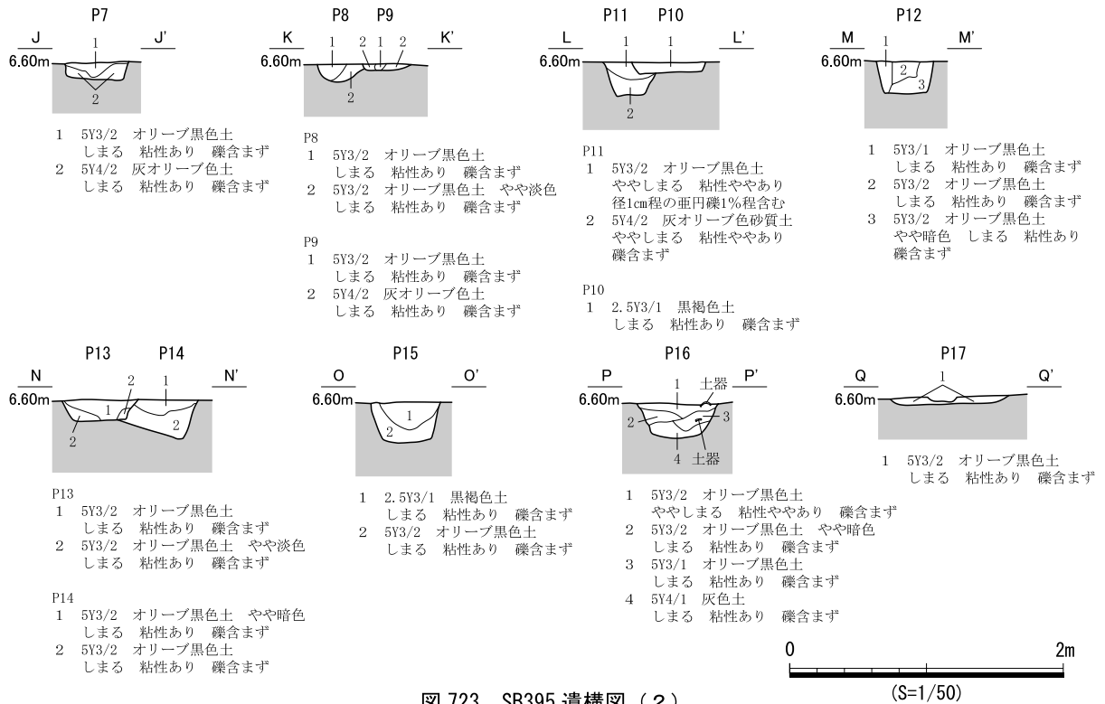
図 723 SB395 遺構図 (2)
