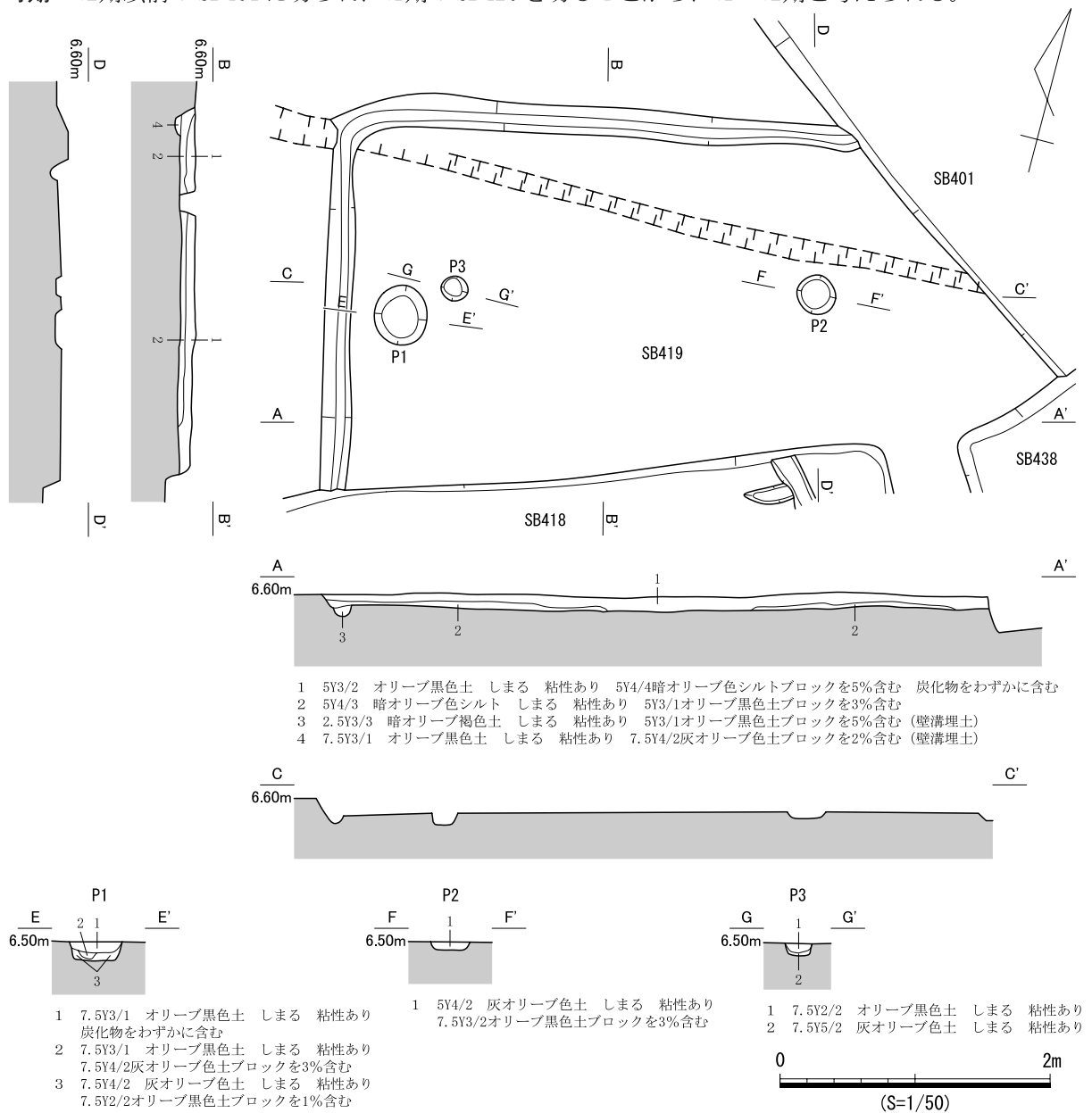
図782 SB419 遺構図
