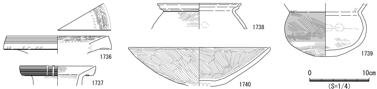
図643 SB364 遺物実測図
