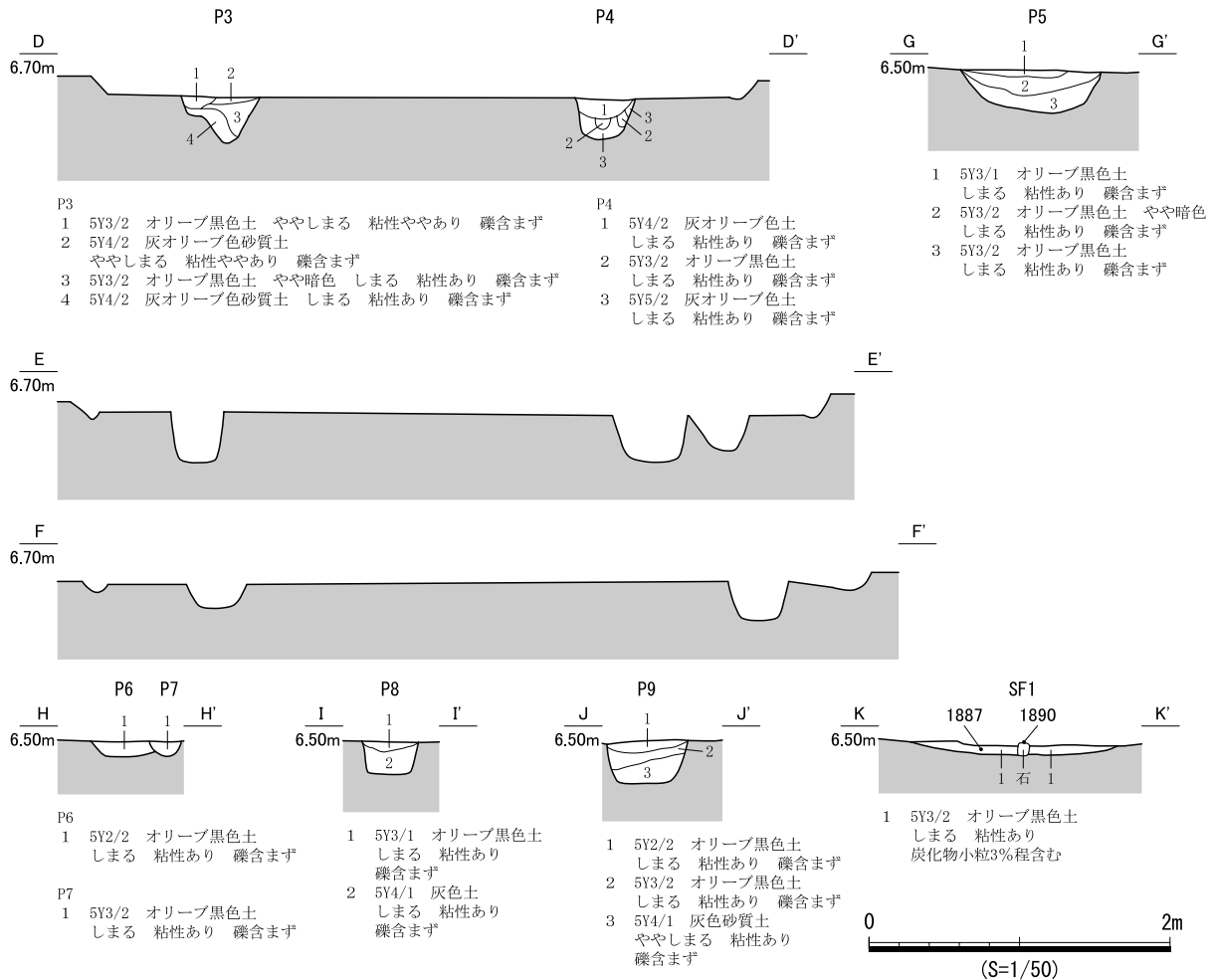
図 725 SB396 遺構図 (2)
