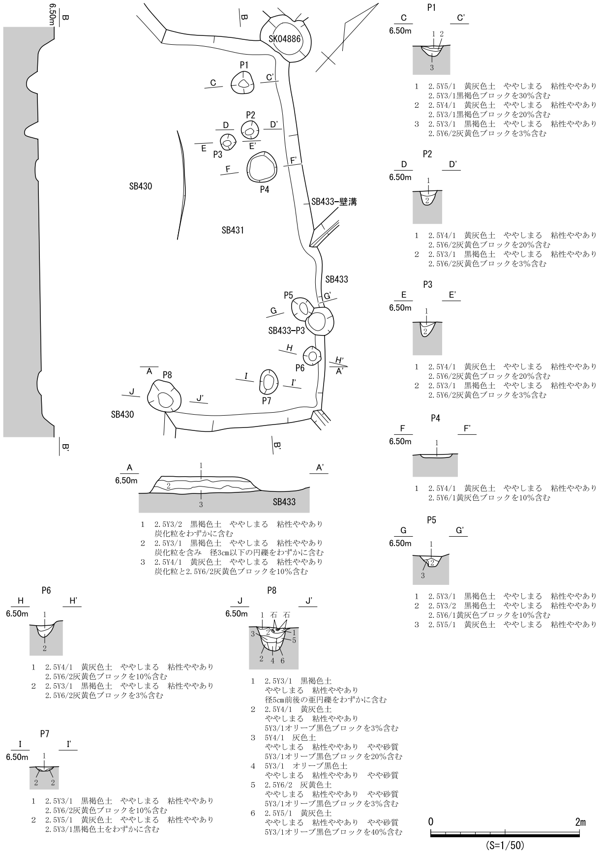
図 816 SB431 遺構図
