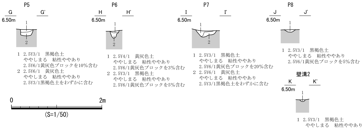
図 829 SB436 遺構図 (2)
