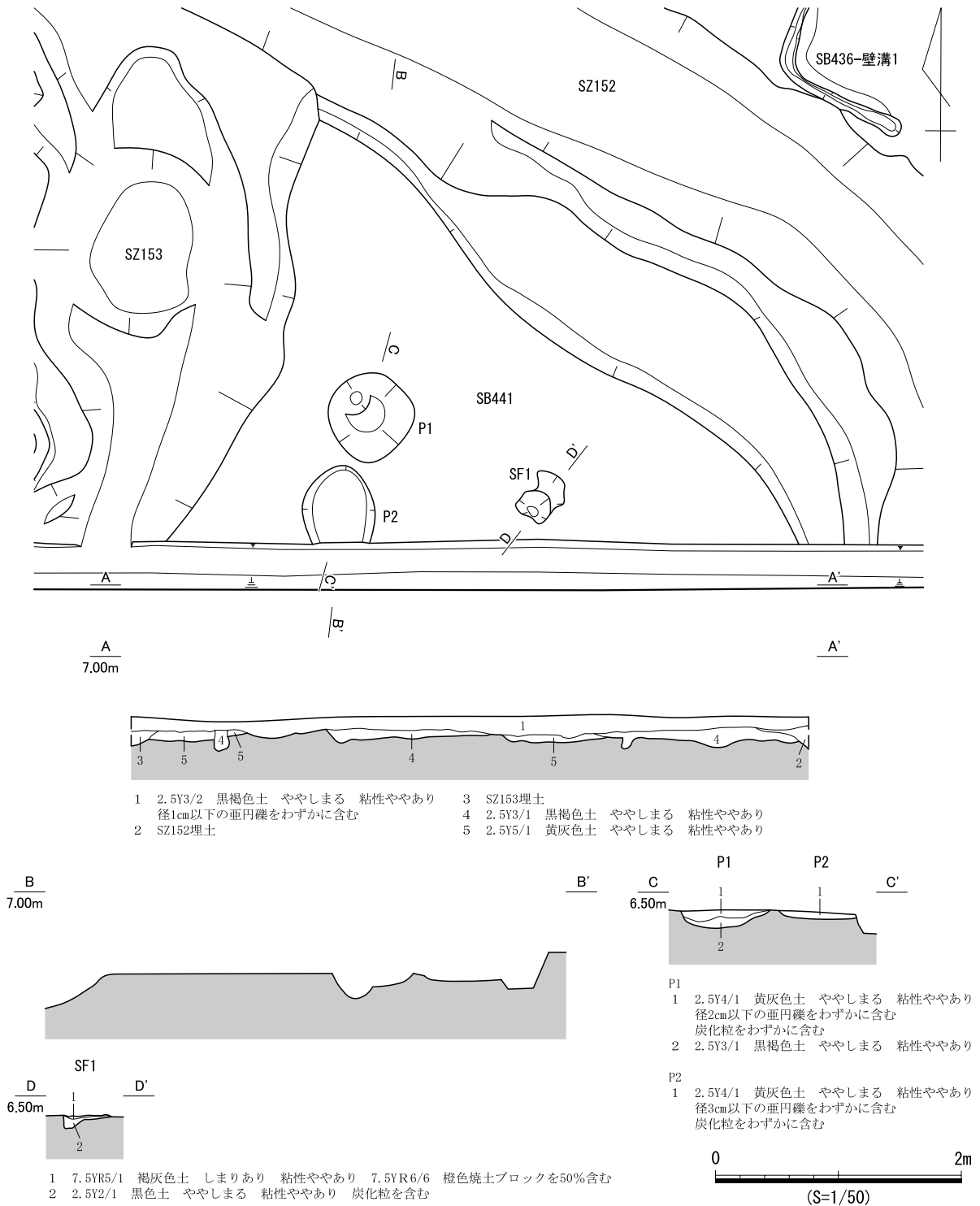
図 838 SB441 遺構図
