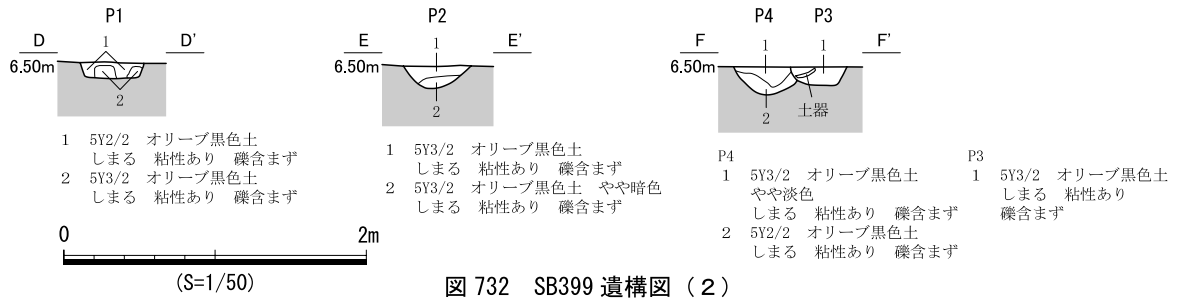
図 732 SB399 遺構図 (2)
