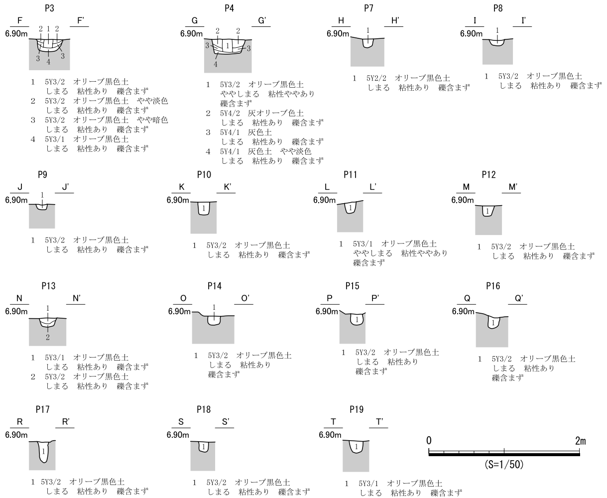
図 639 SB362 遺構図 (2)
