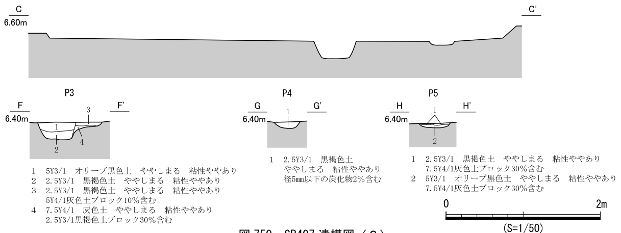
図 750 SB407 遺構図 (2)
