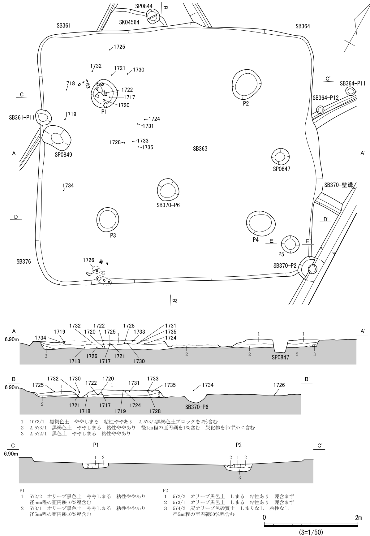
図 640 SB363 遺構図 (1)
