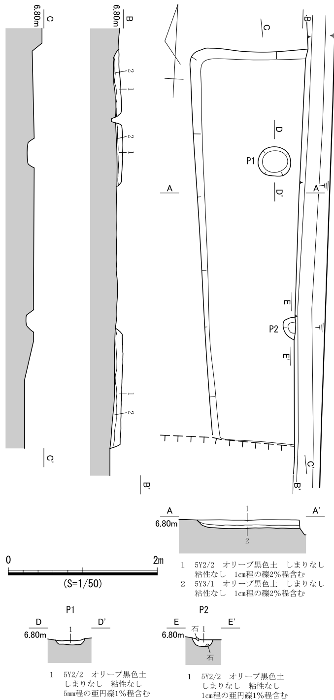
図 657 SB369 遺構図
