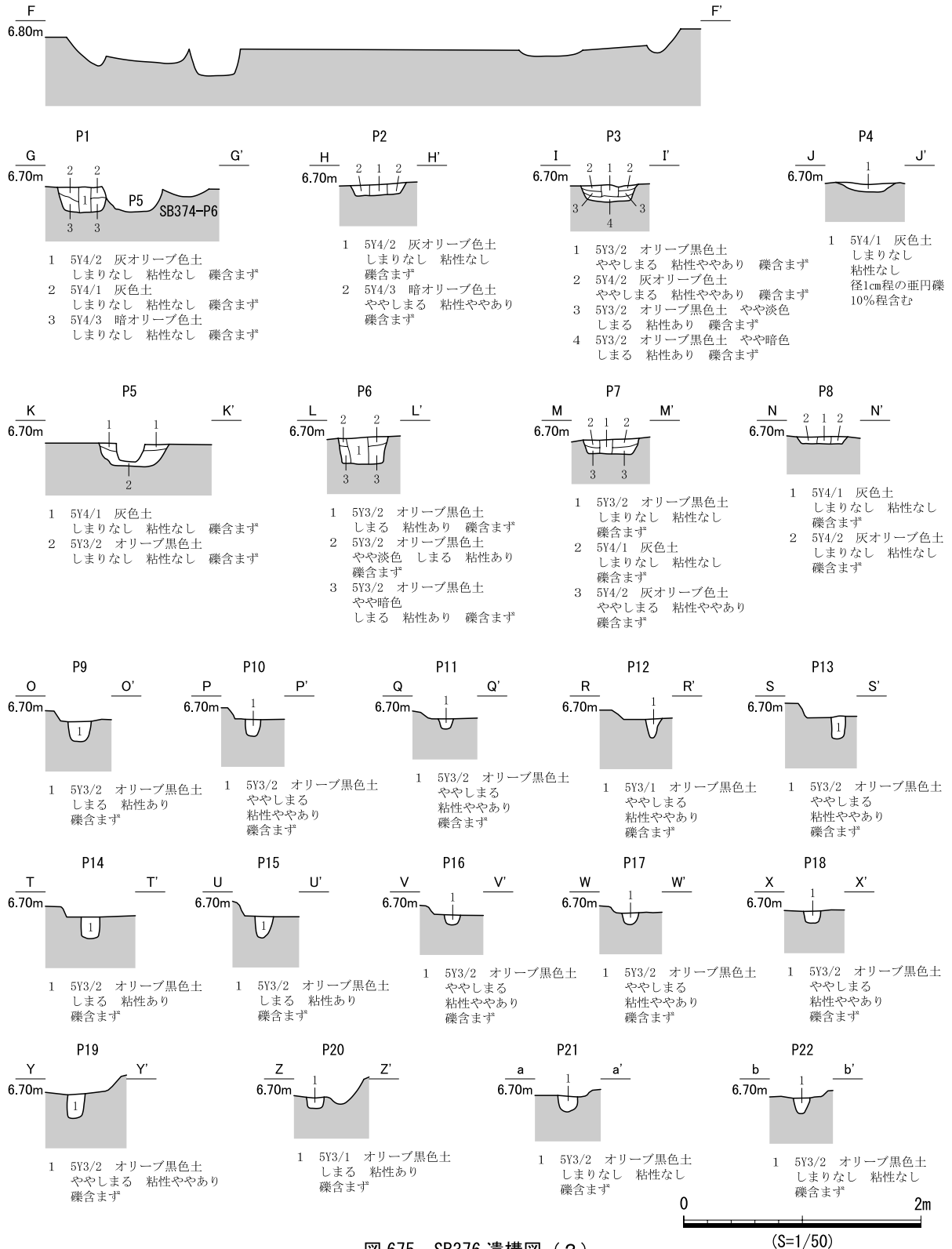
図 675 SB376 遺構図 (2)
