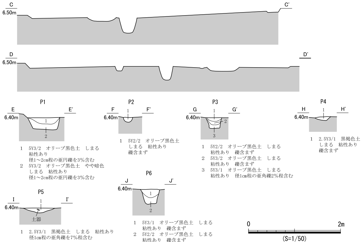
図 693 SB383 遺構図 (2)
