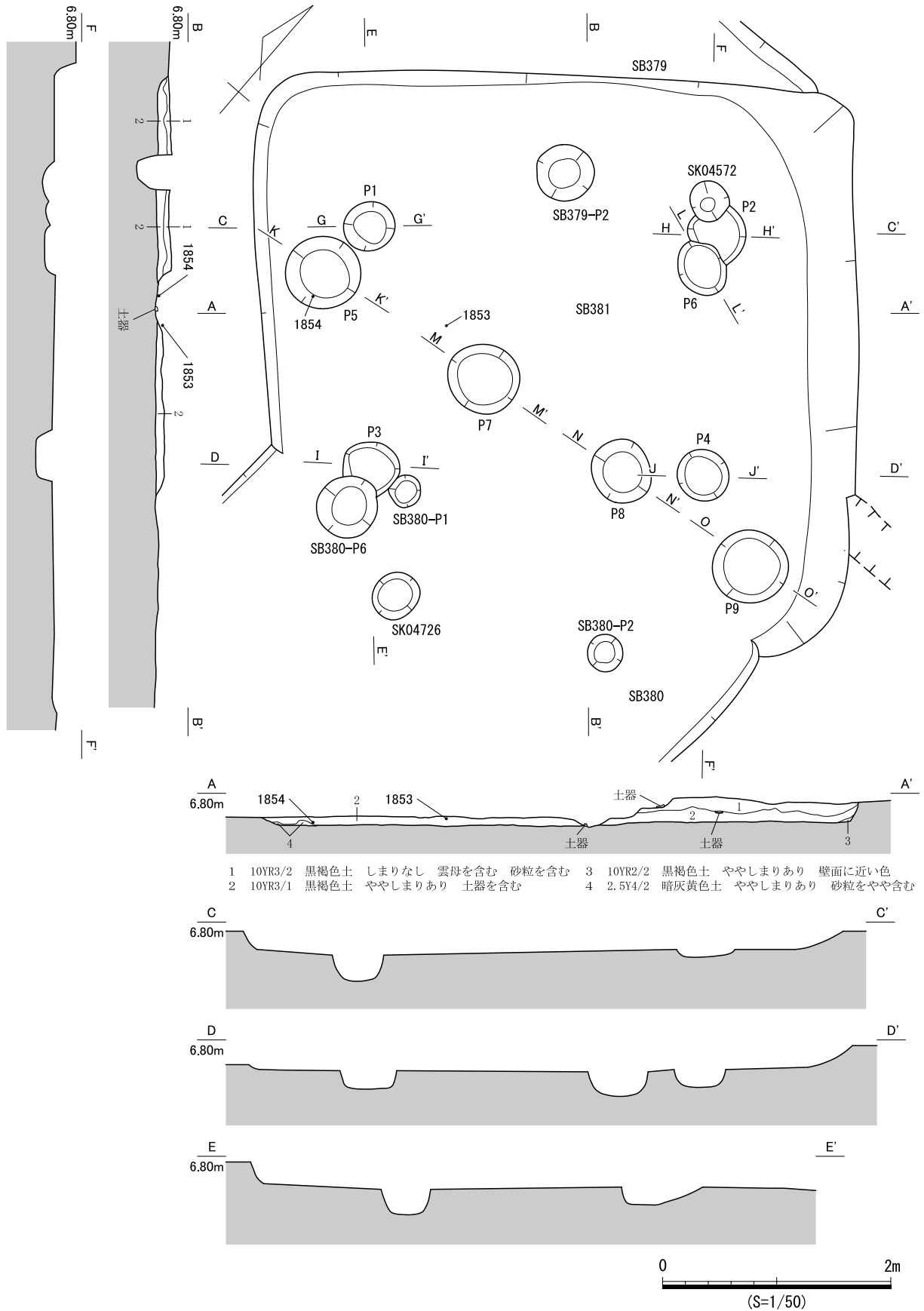
図 688 SB381 遺構図 (1)
