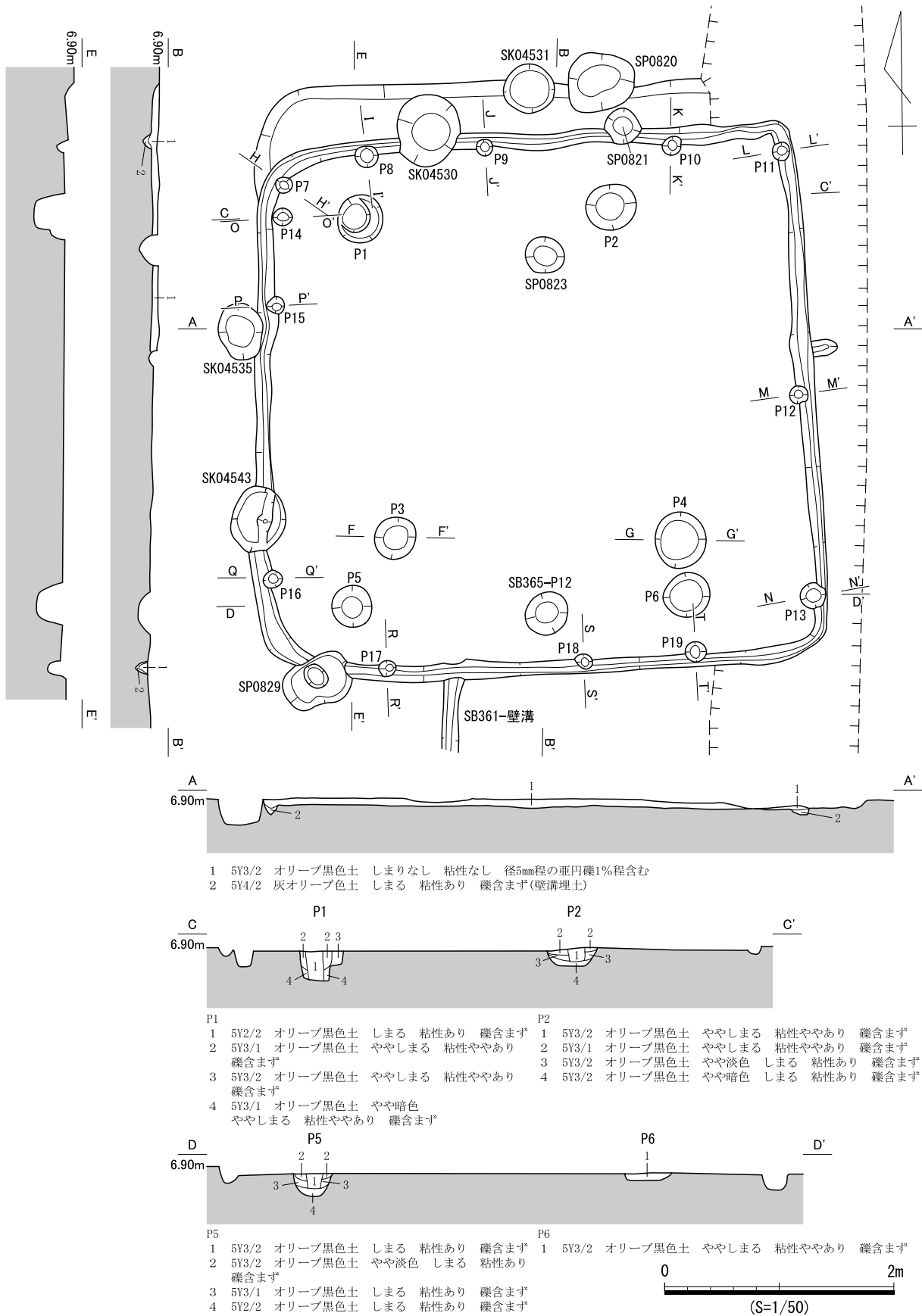
図 638 SB362 遺構図 (1)
