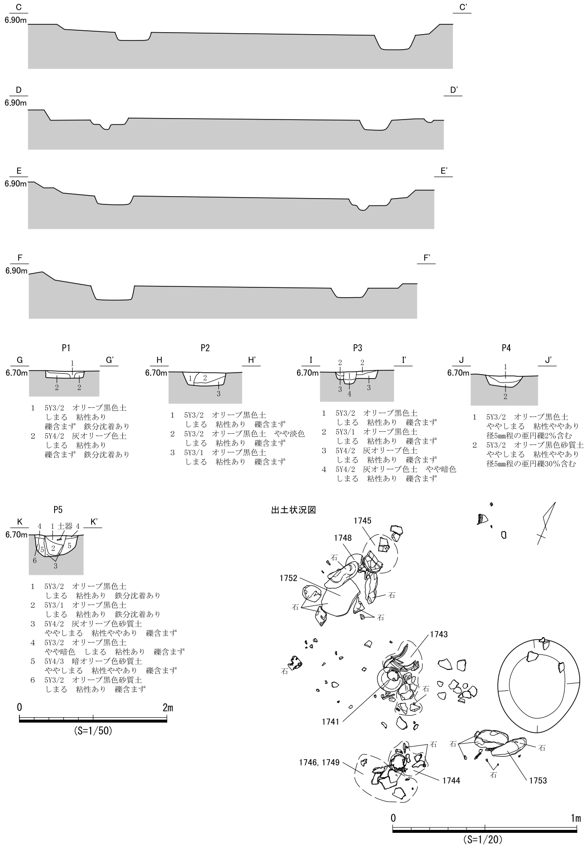
図 647 SB365 遺構図 (2)
