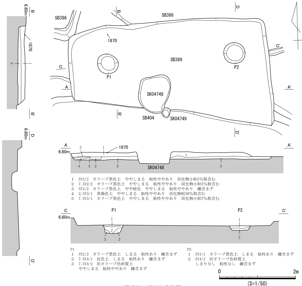
図 708 SB389 遺構図
