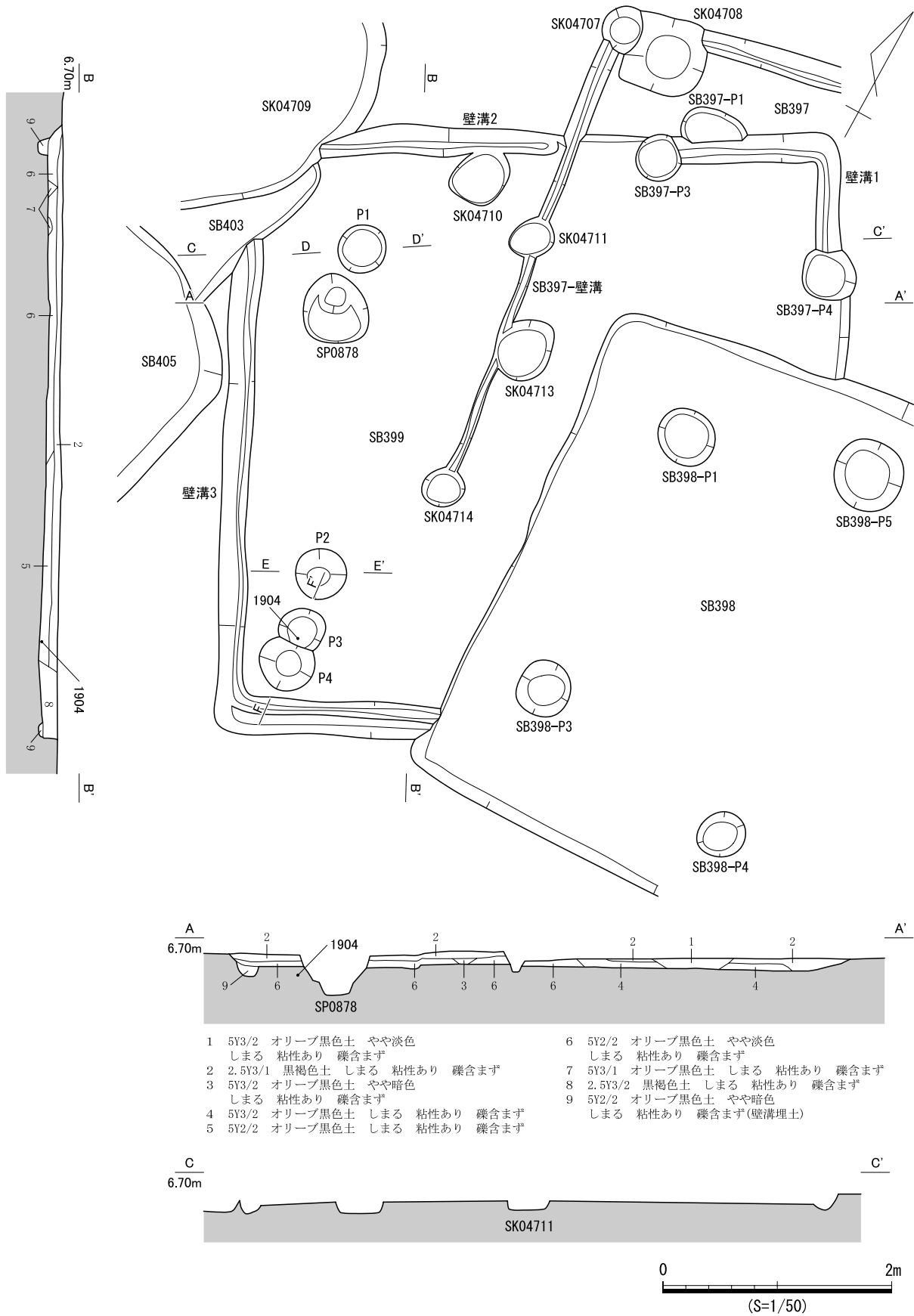
図 731 SB399 遺構図 (1)
