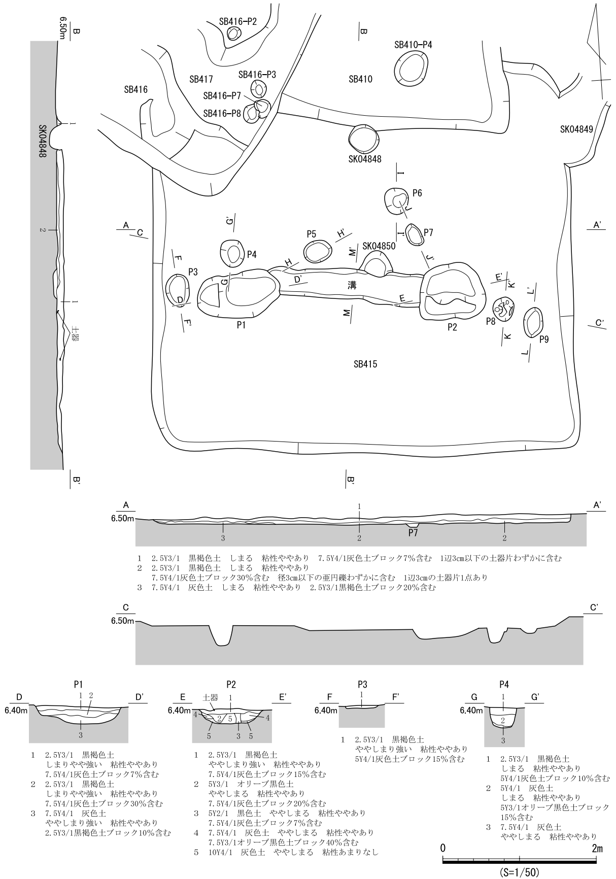
図 769 SB415 遺構図 (1)
