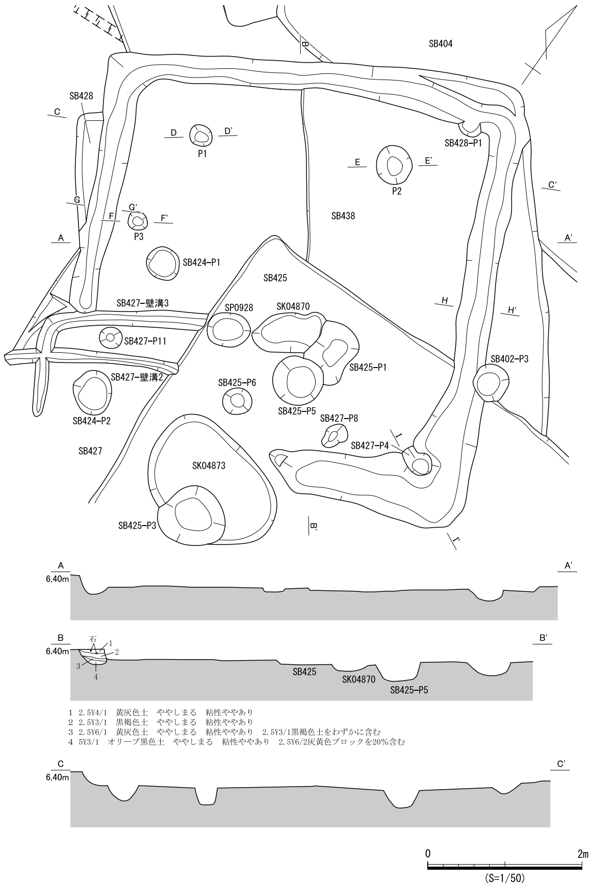
図 832 SB438 遺構図 (1)
