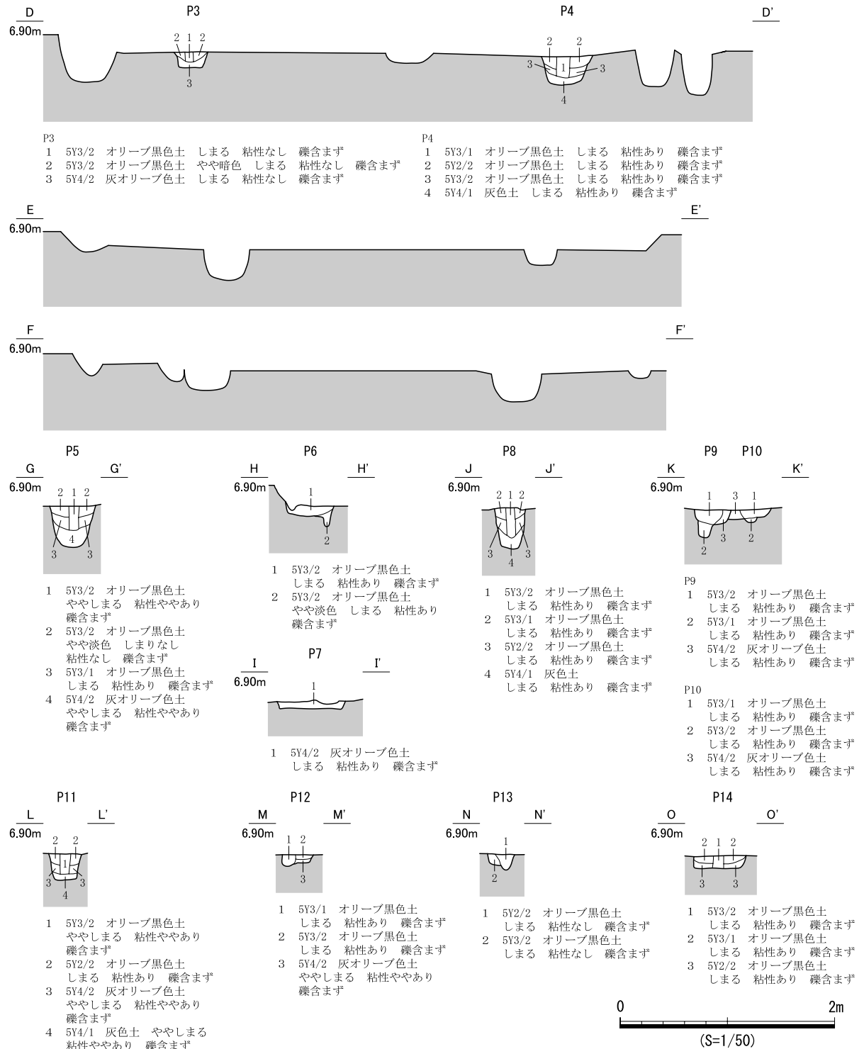
図 652 SB367 遺構図 (2)
