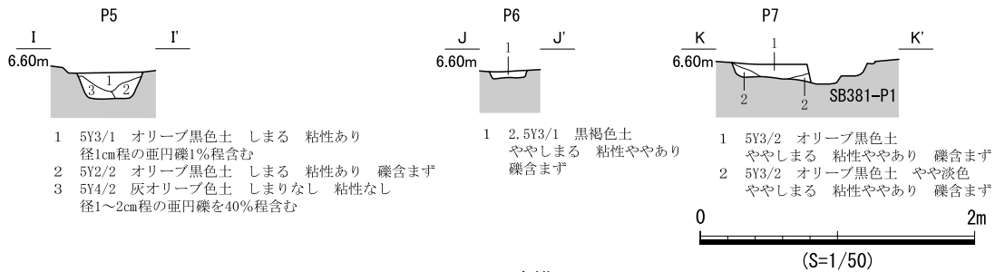
図 678 SB377 遺構図 (2)
