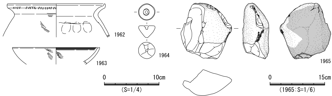
図 771 SB415 遺物実測図
