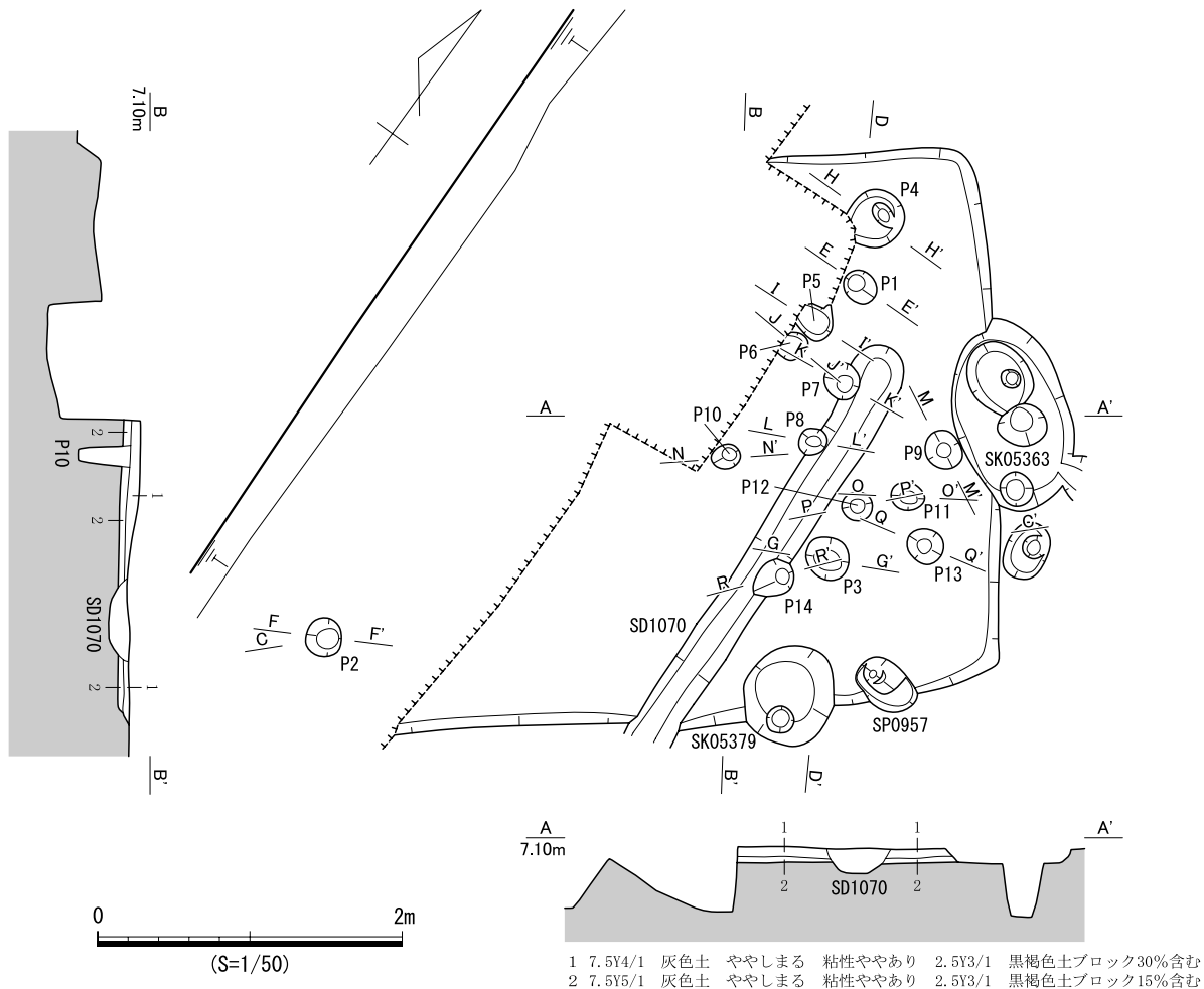
図 864 SB454 遺構図 (1)
