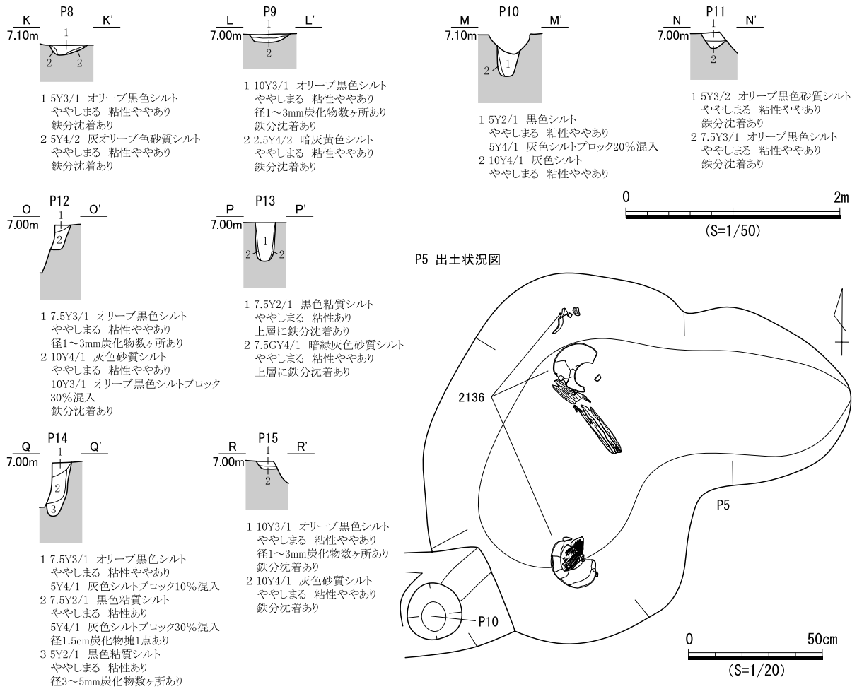
図 858 SB451 遺構図 (2)
