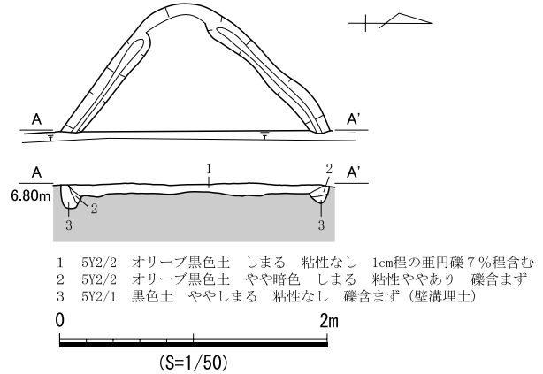
図 655 SB368 遺構図
