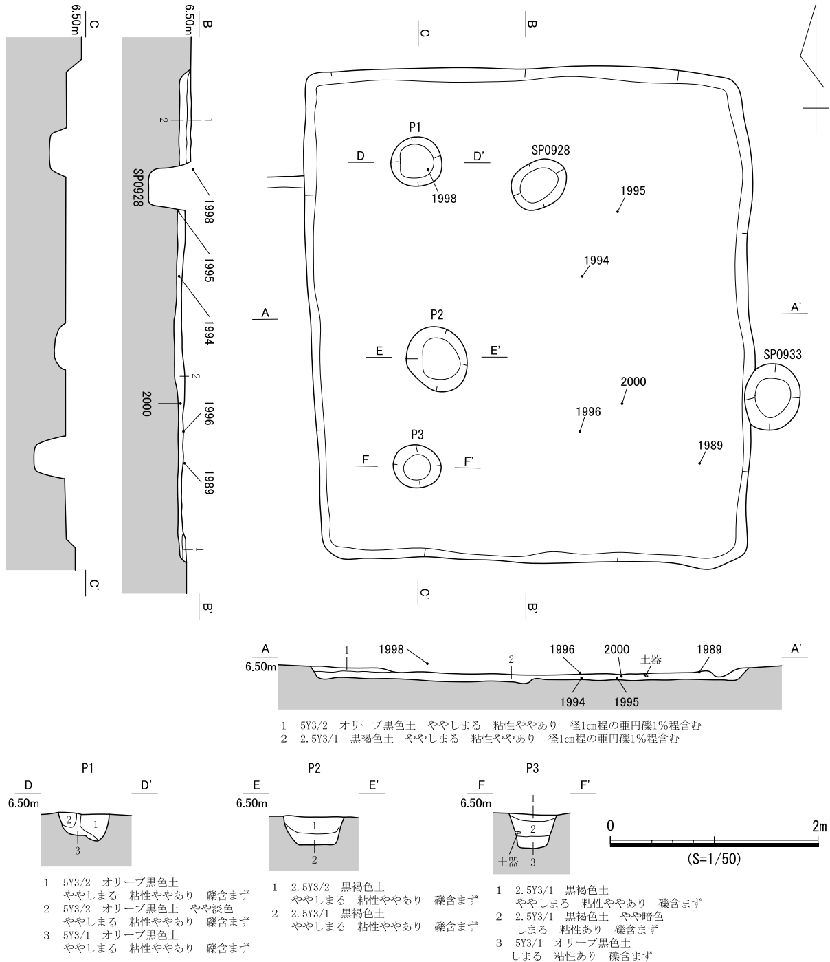
図 796 SB424 遺構図
