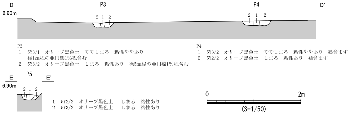
図 641 SB363 遺構図 (2)
