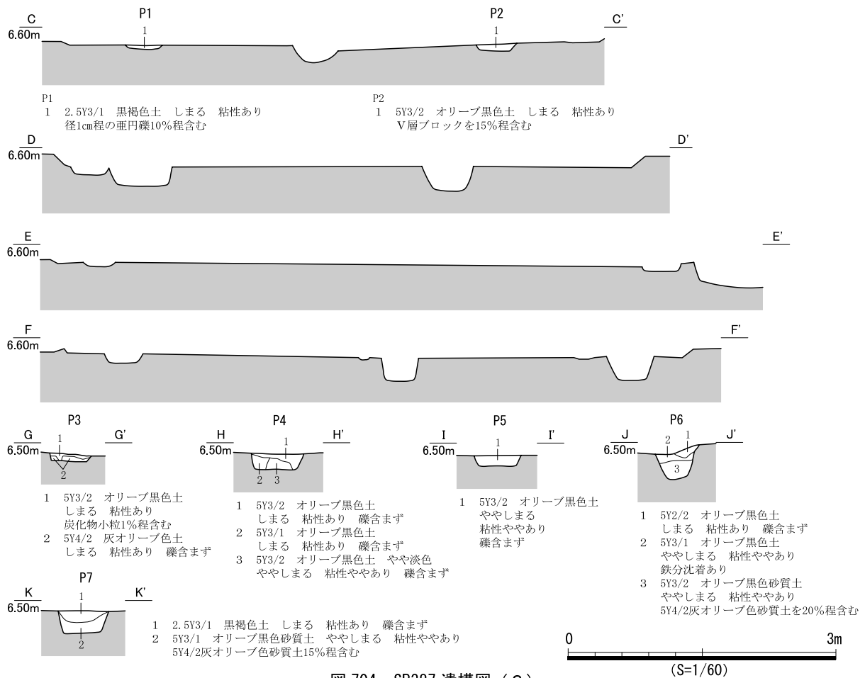
図 704 SB387 遺構図 (2)
