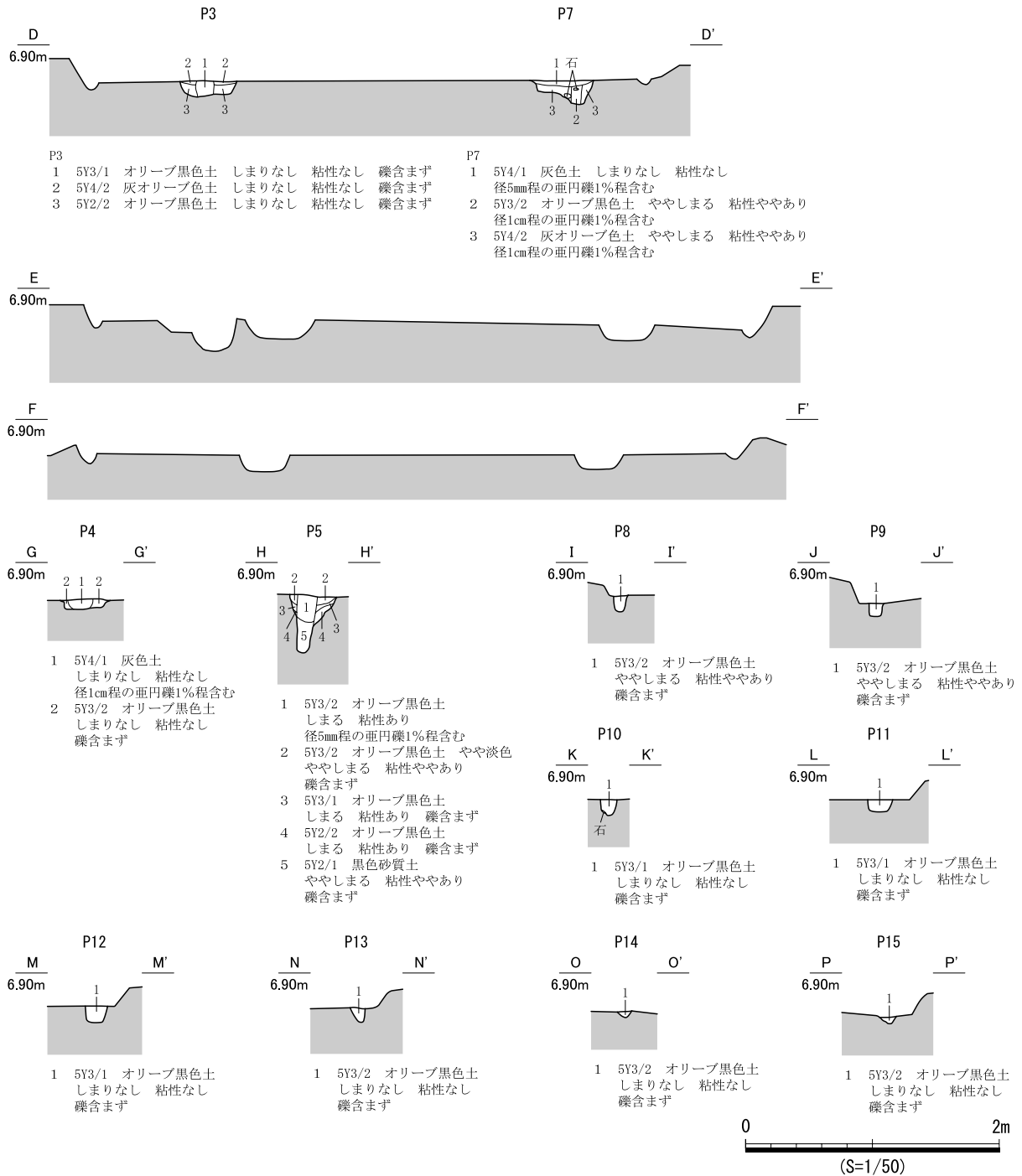
図 645 SB364 遺構図 (2)
