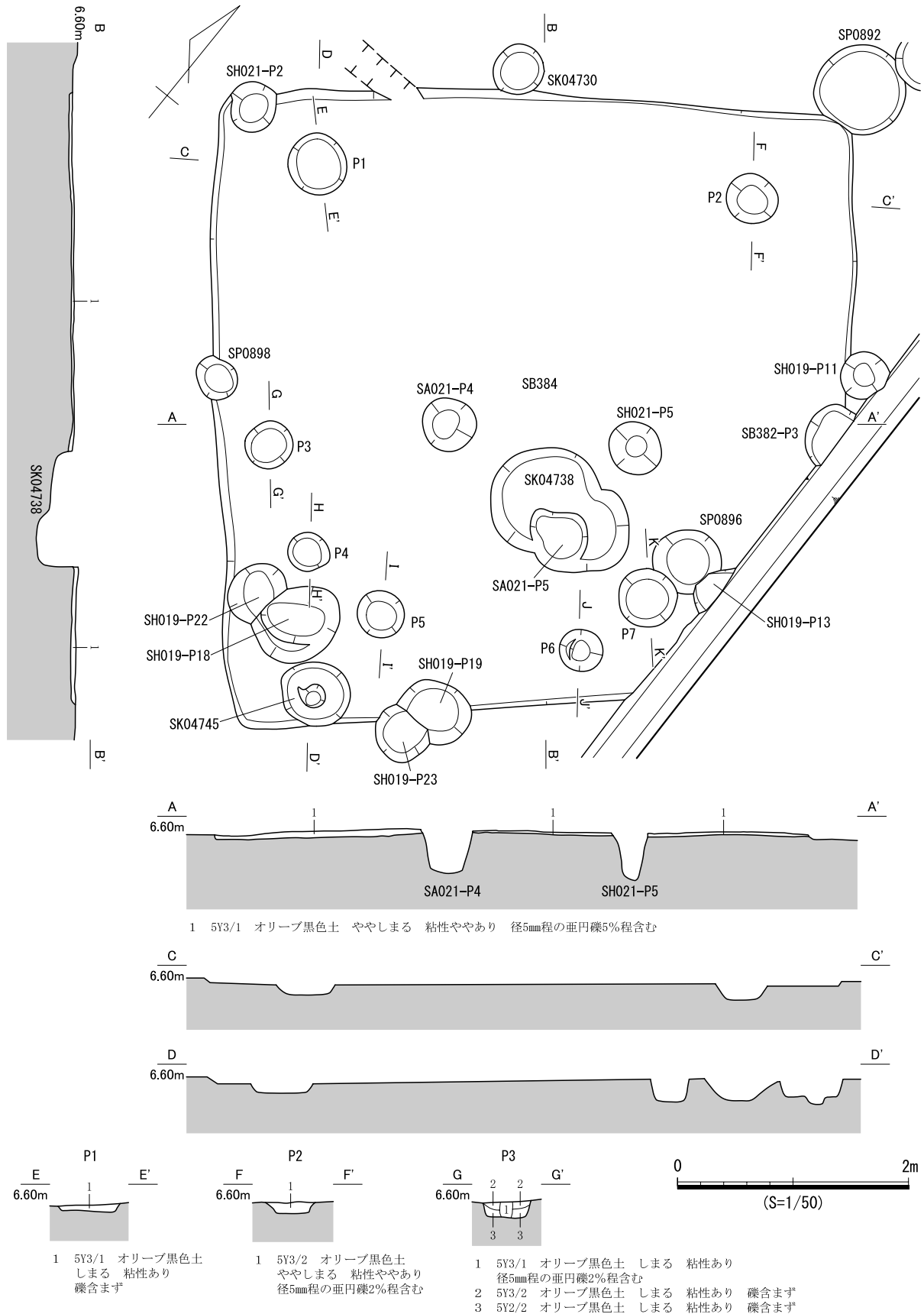
図 695 SB384 遺構図 (1)
