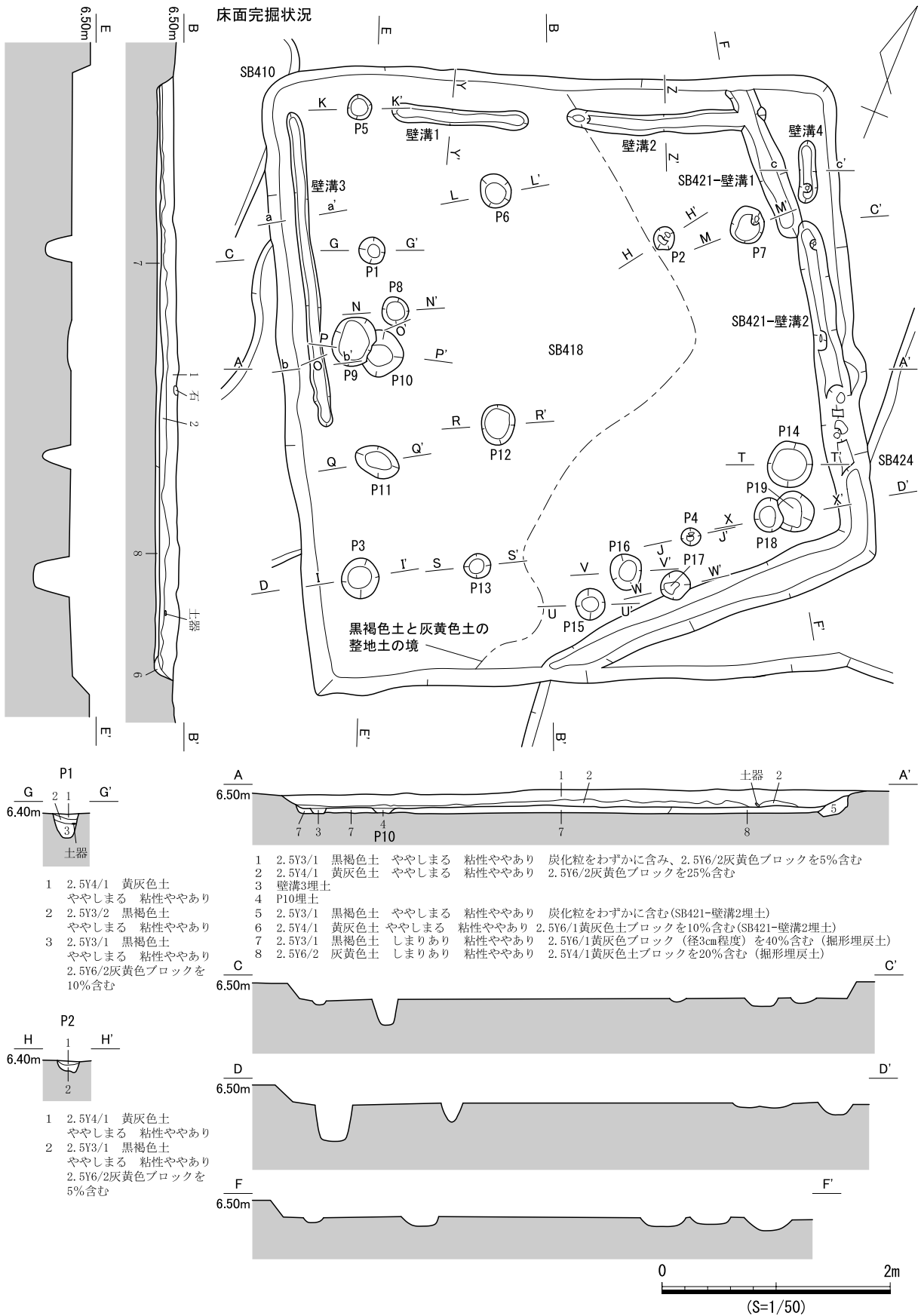
図 778 SB418 遺構図 (1)
