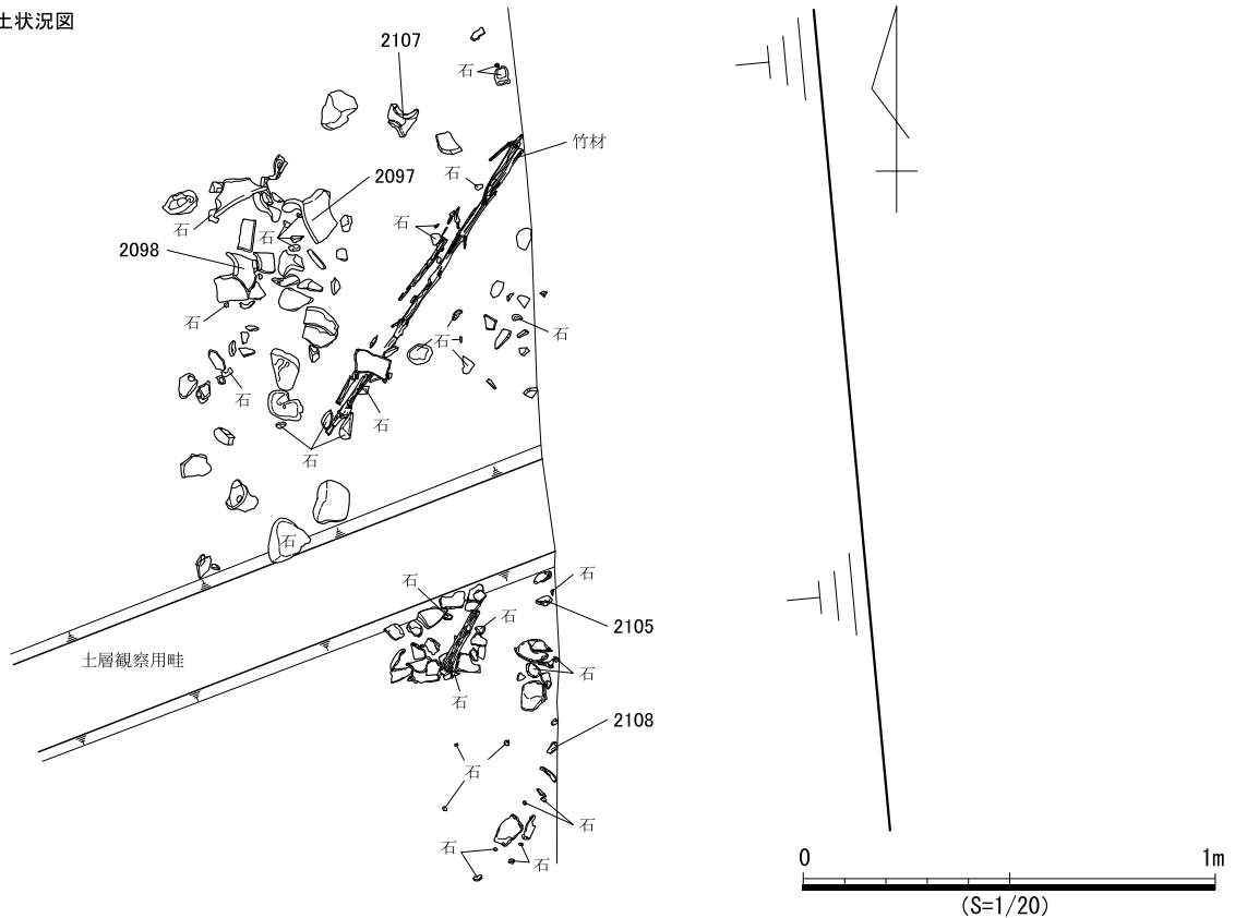
図 845 SB444 遺構図 (2)
