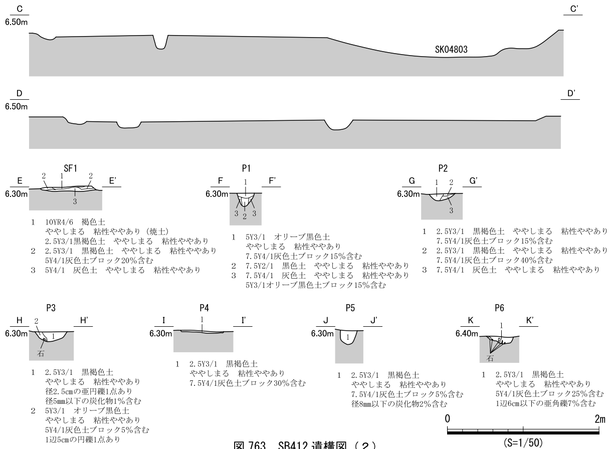
図 763 SB412 遺構図 (2)
