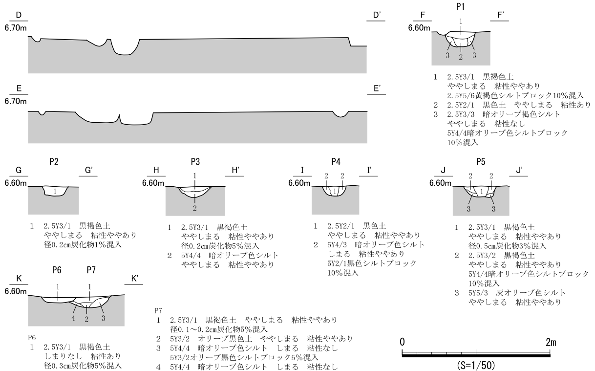
図 753 SB408 遺構図 (2)
