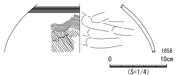
図 694 SB384 遺物実測図
