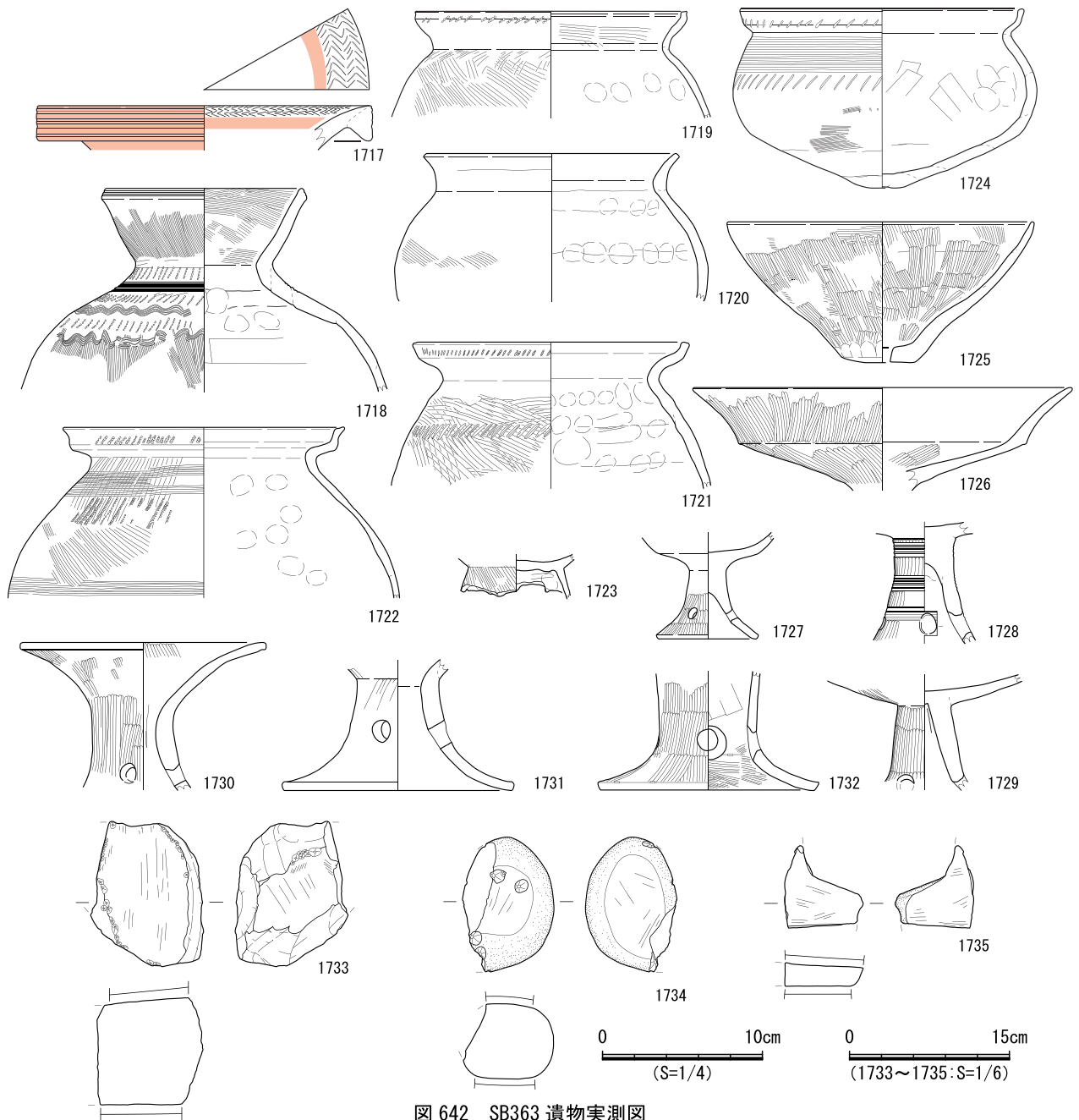
図 642 SB363 遺物実測図
