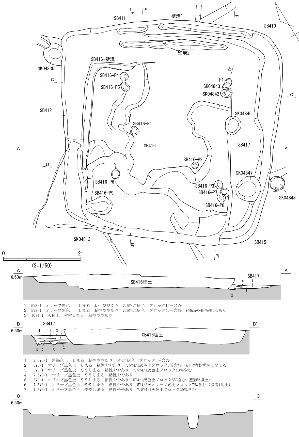
図 776 SB417 遺構図 (1)
