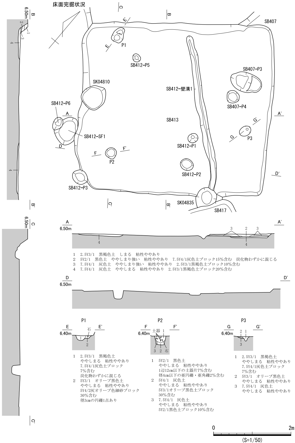
図 765 SB413 遺構図 (1)
