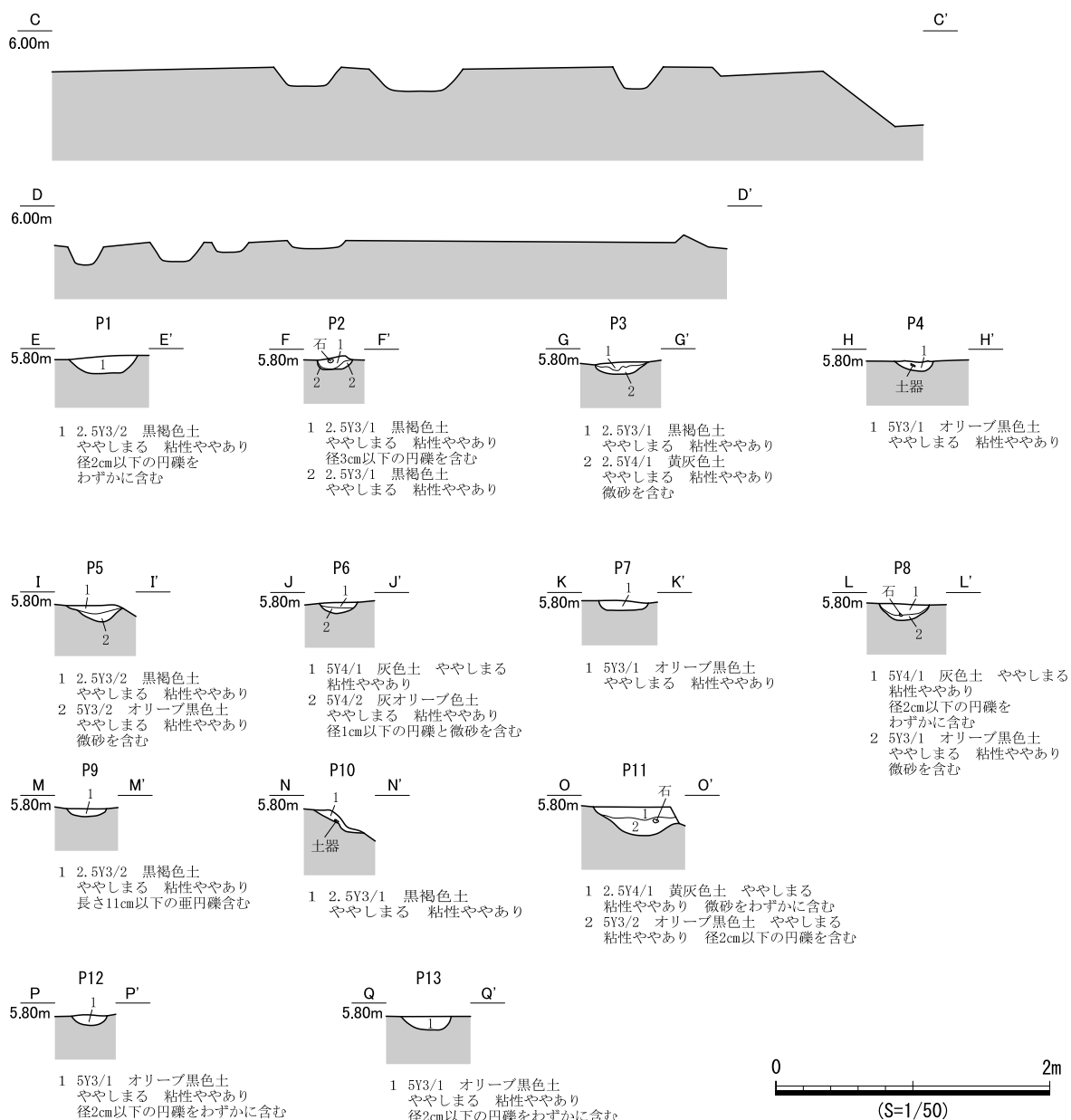
図 842 SB443 遺構図 (2)
