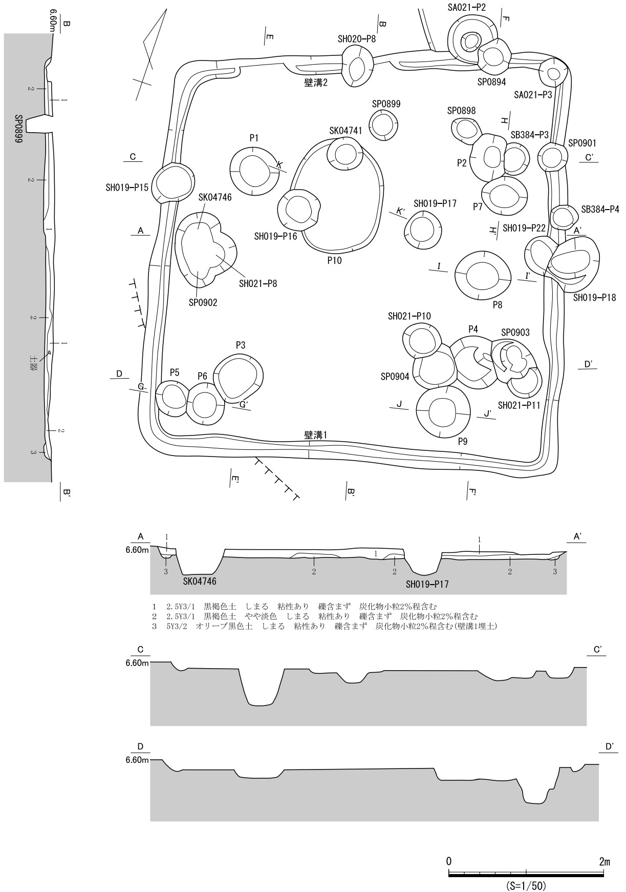
図 699 SB386 遺構図 (1)
