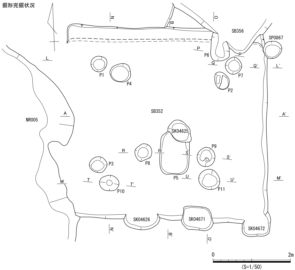
図 615 SB352 遺構図 (2)
