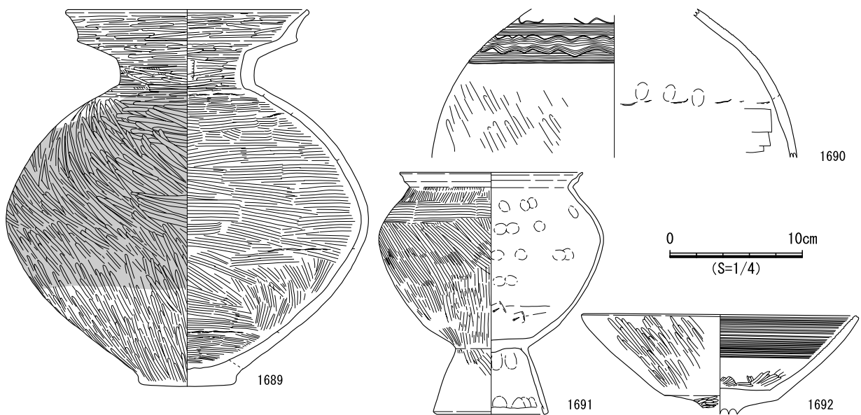
図 617 SB352 遺物実測図
