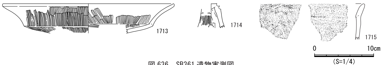
図 636 SB361 遺物実測図
