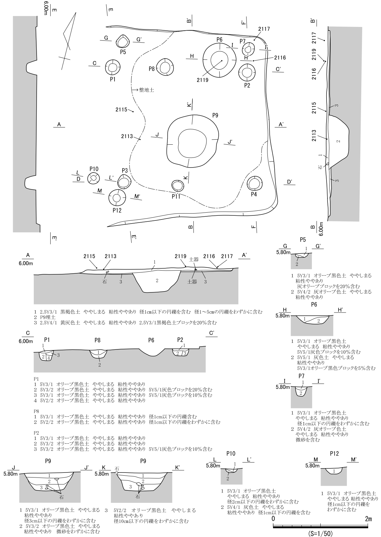
図 847 SB445 遺構図 (1)
