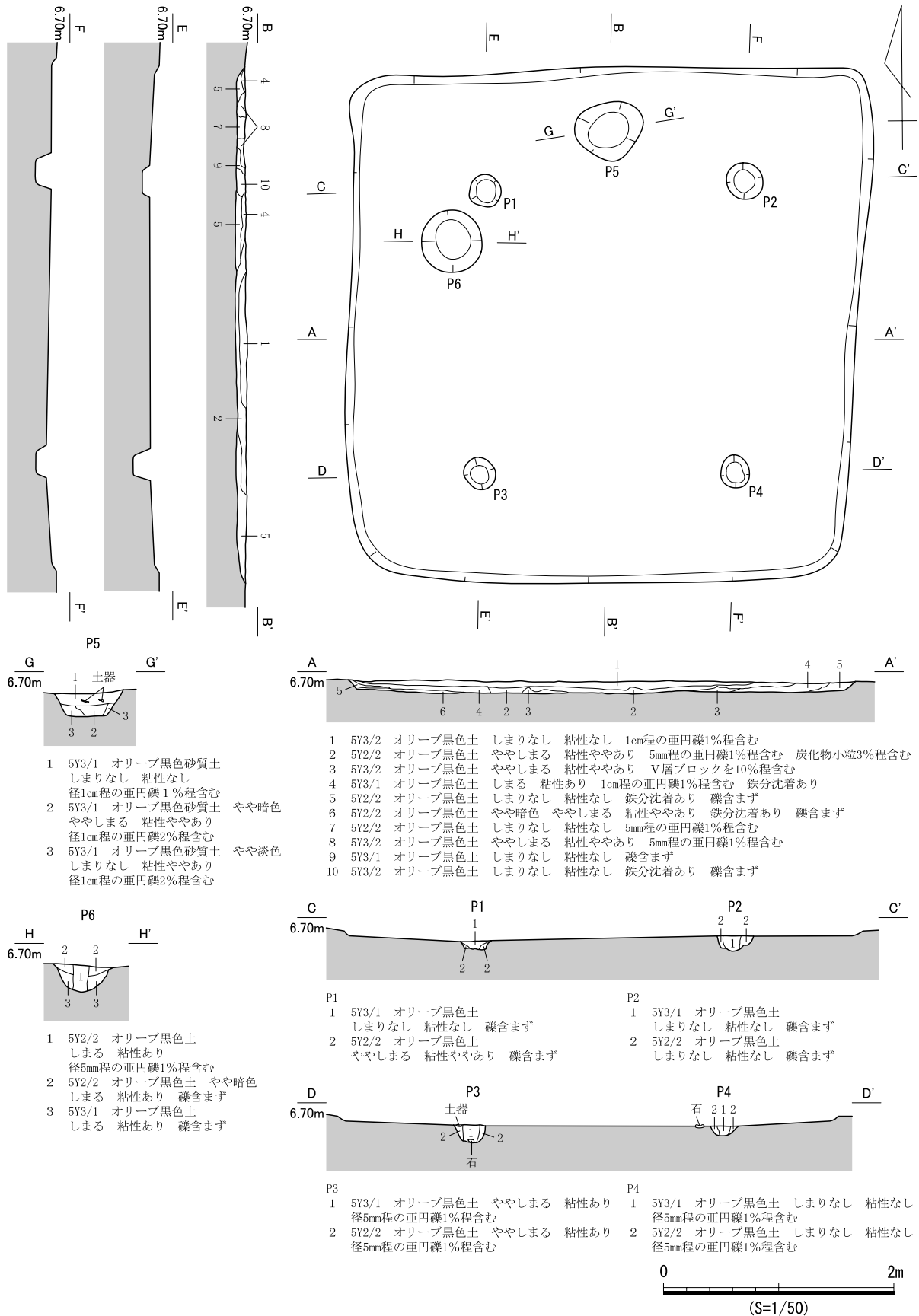
図 685 SB380 遺構図
