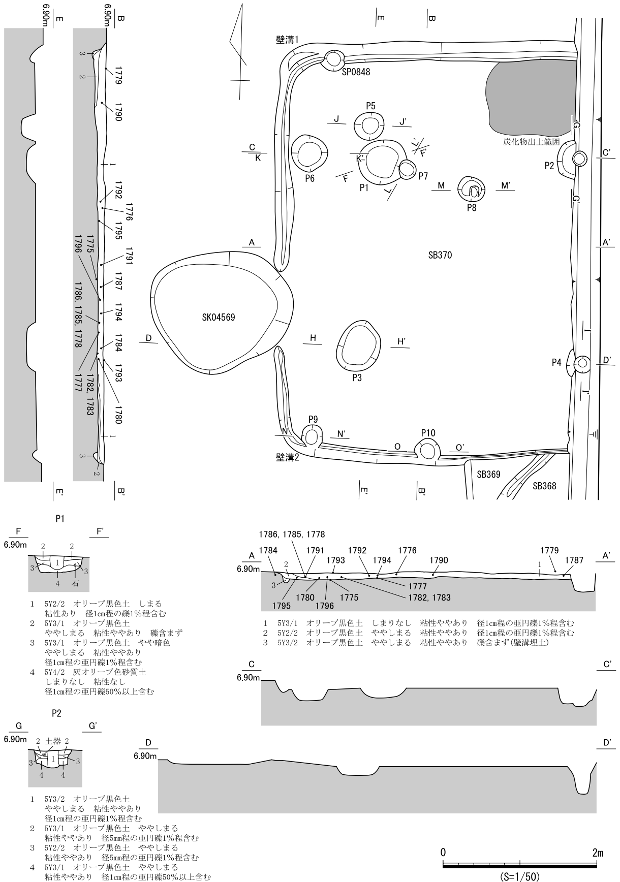
図 658 SB370 遺構図 (1)
