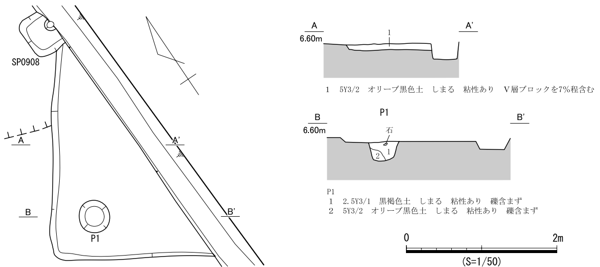
図 712 SB391 遺構図
