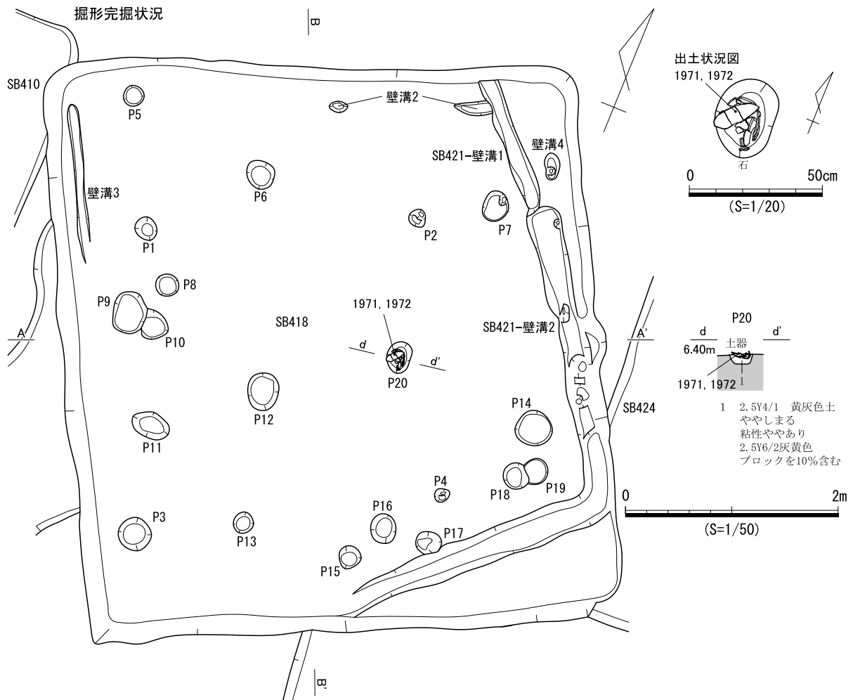
図 780 SB418 遺構図 (3)
