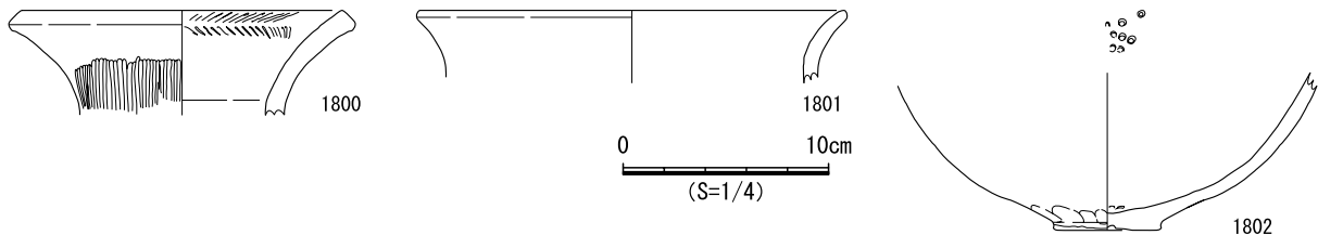
図 666 SB373 遺物実測図
