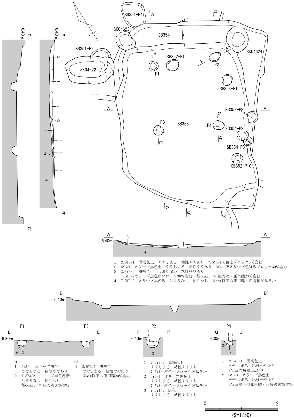
図 622 SB355 遺構図
