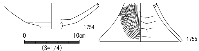
図649 SB366 遺物実測図
