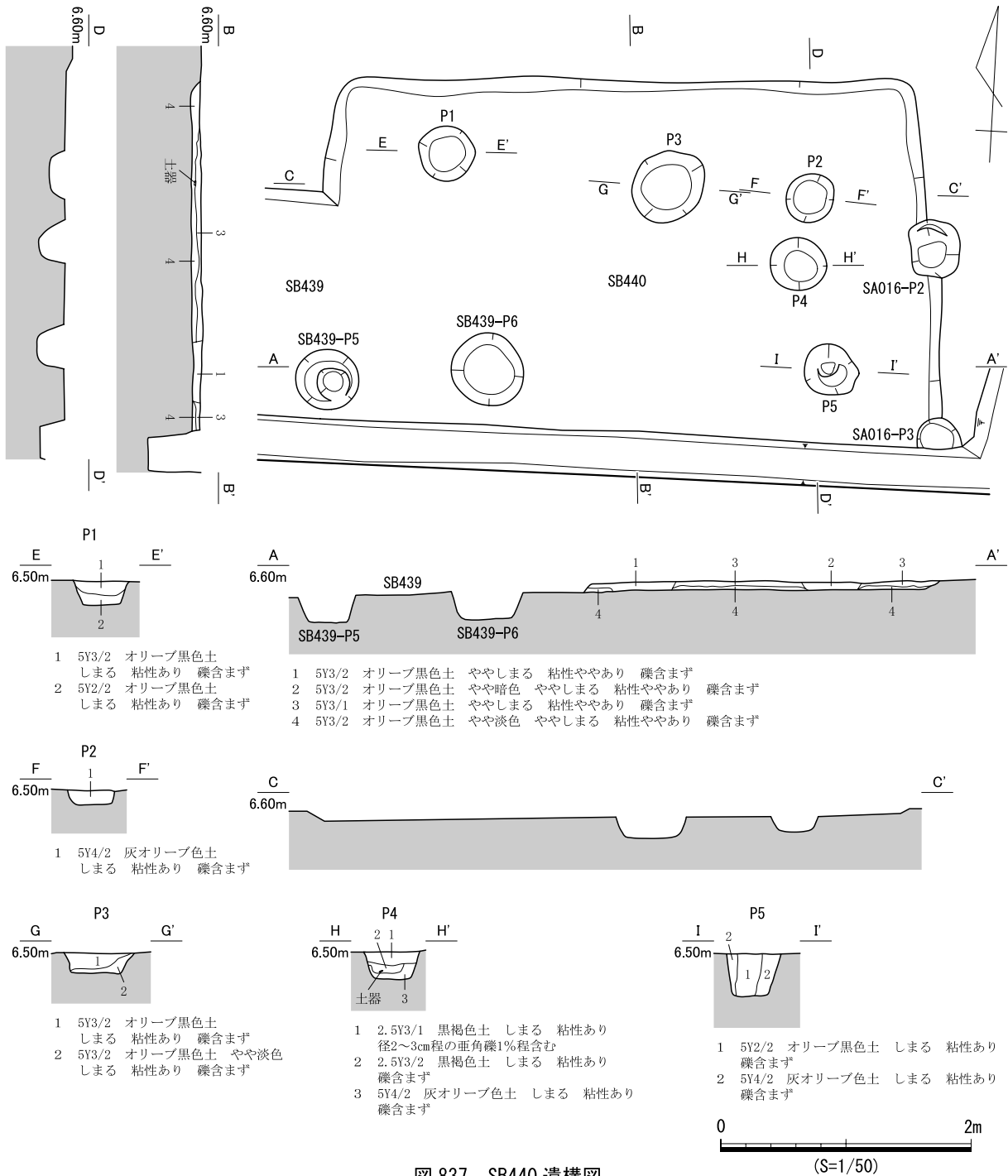
図 837 SB440 遺構図
