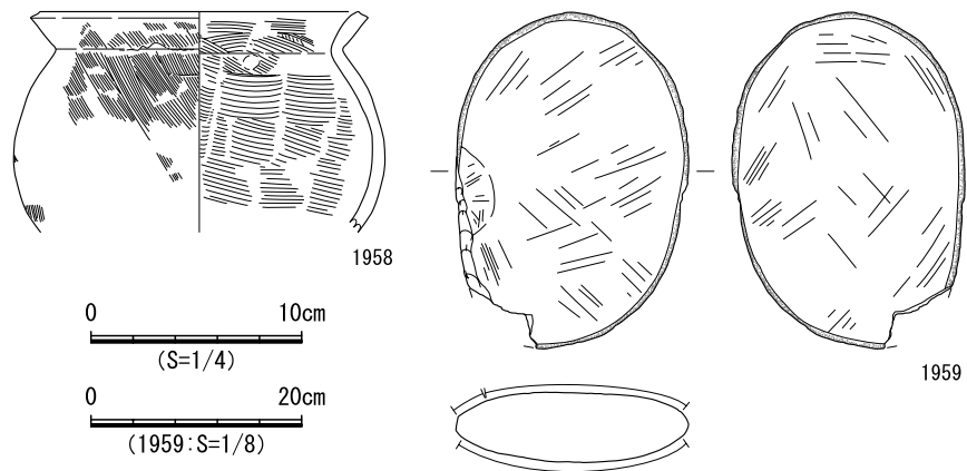
図 762 SB412 遺物実測図
