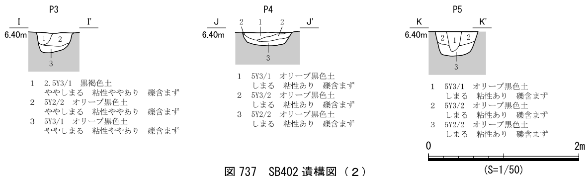
図 737 SB402 遺構図 (2)
