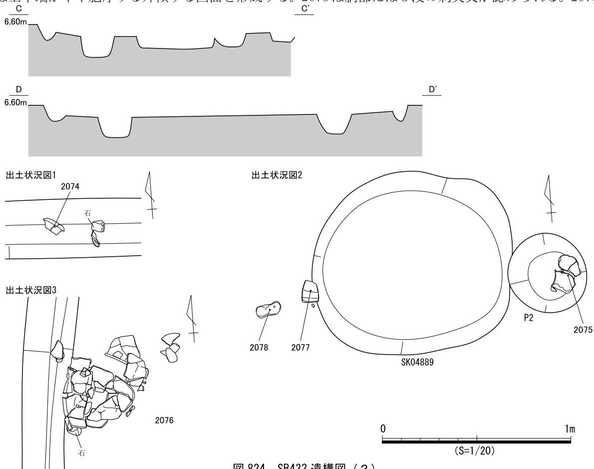
図 824 SB433 遺構図（2）
