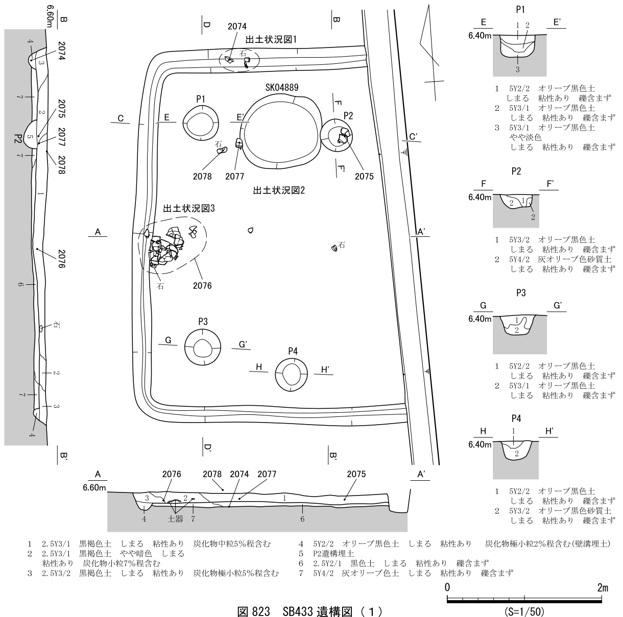
図 823 SB433 遺構図 (1)
