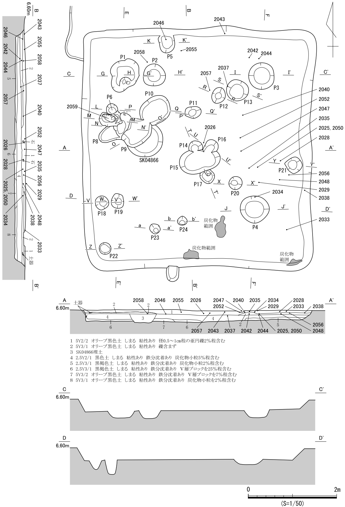
図 808 SB429 遺構図 (1)
