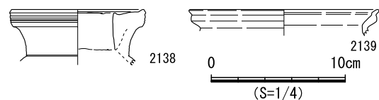
図 861 SB453 遺物実測図
