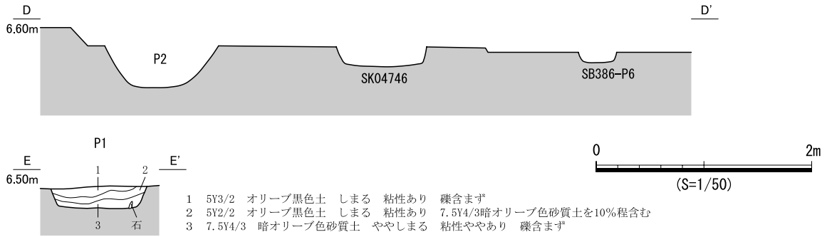
図 710 SB390 遺構図 (2)
