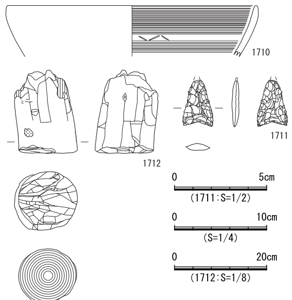
図 630 SB360 遺物実測図
