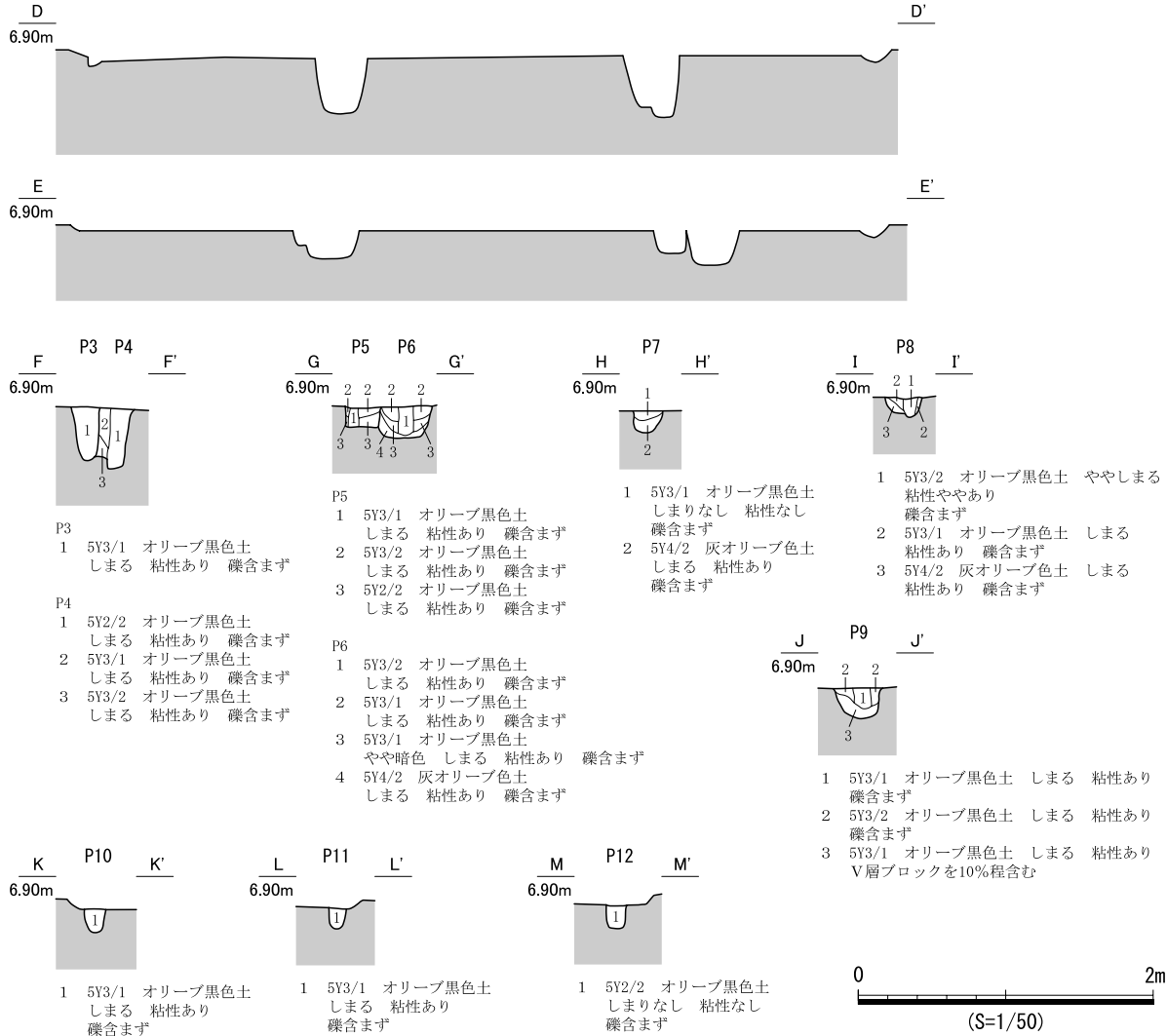
図 668 SB374 遺構図 (2)
