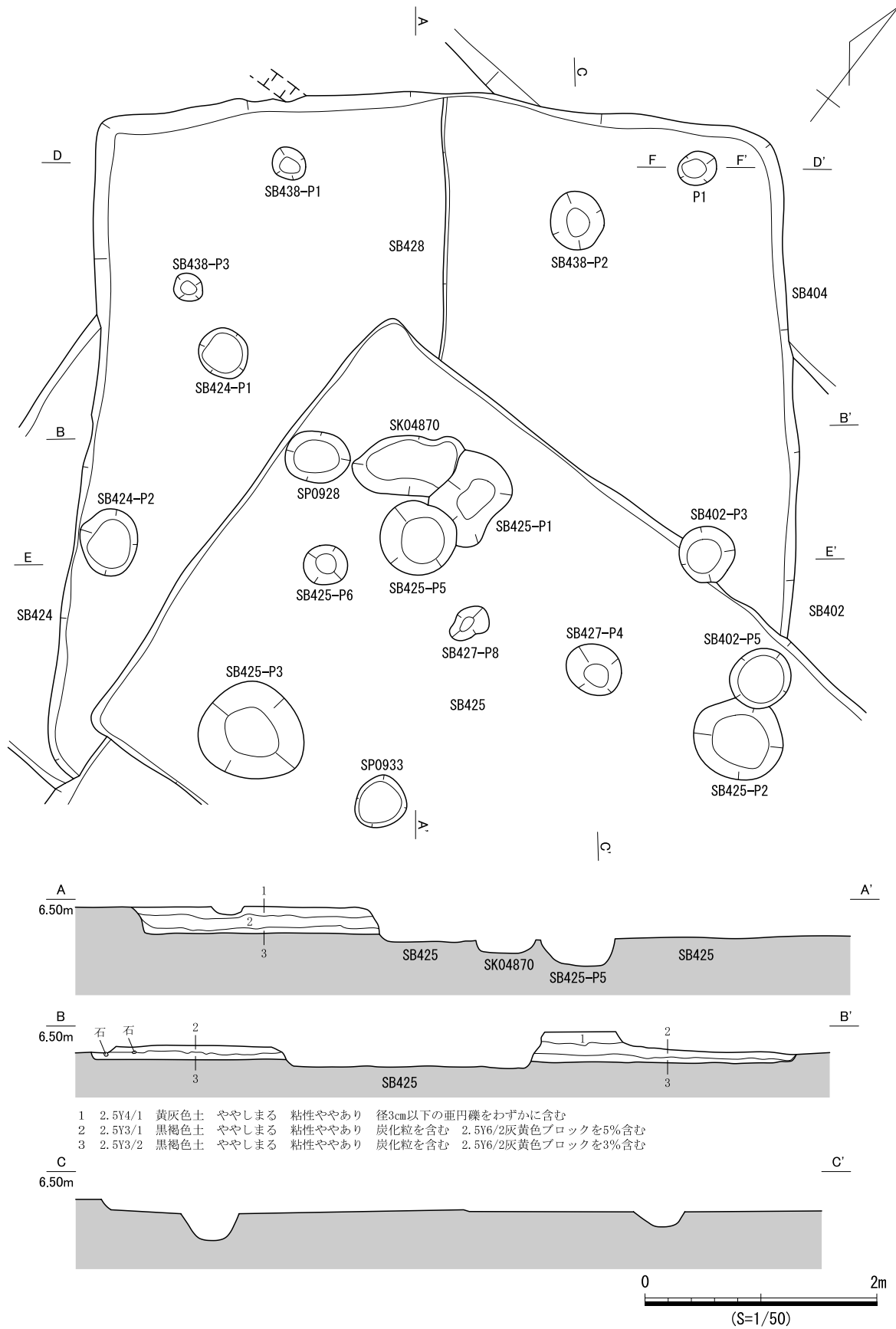
図 806 SB428 遺構図 (1)
