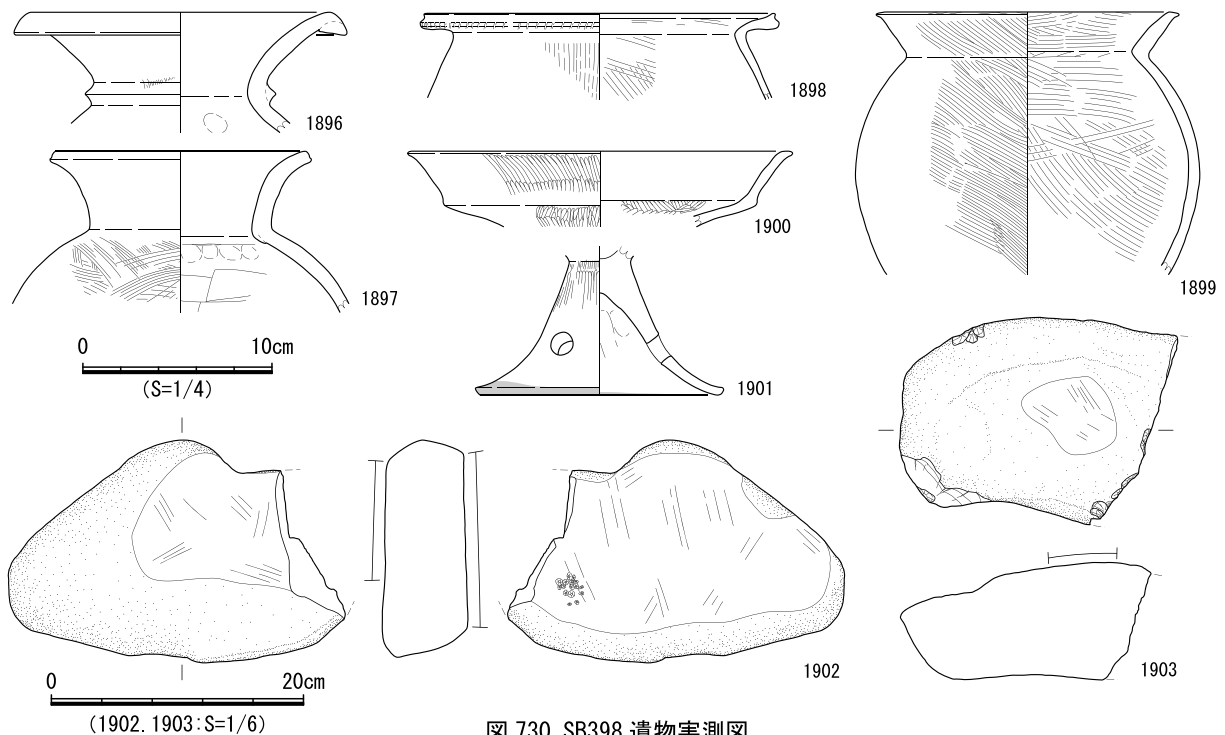
図 730 SB398 遺物実測図
