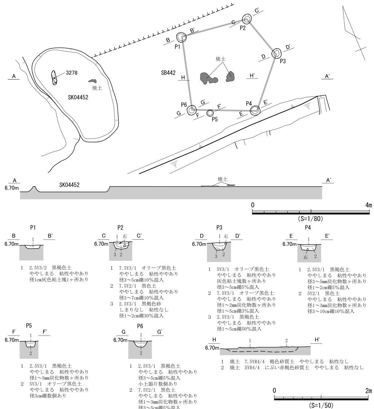
図 840 SB442 遺構図
