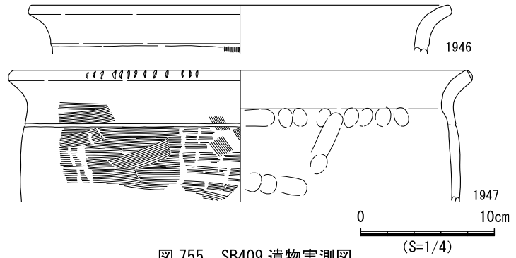
図 755 SB409 遺物実測図
