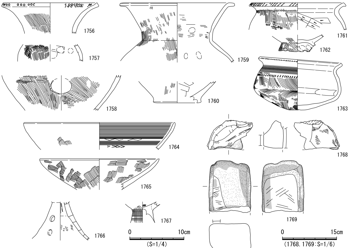
図 654 SB367 遺物実測図
