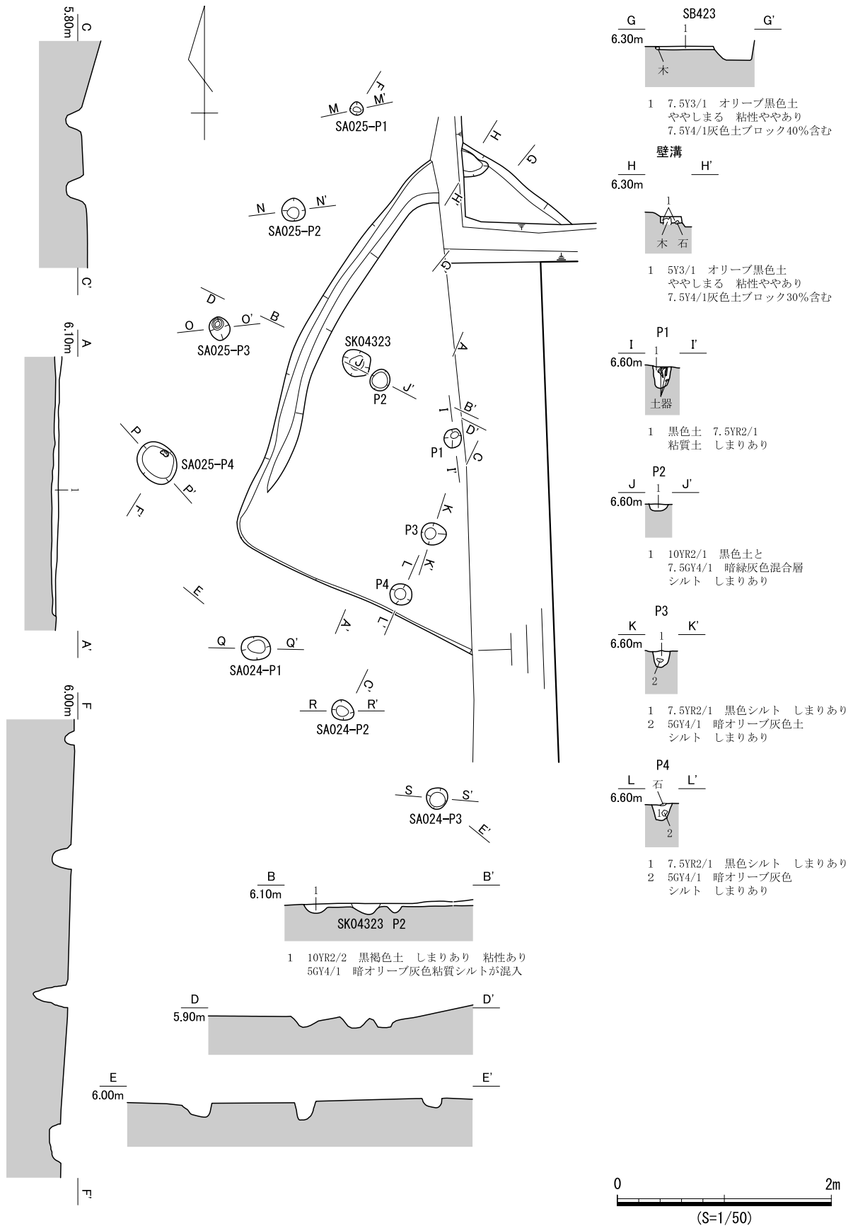
図 793 SB423 遺構図 (1)
