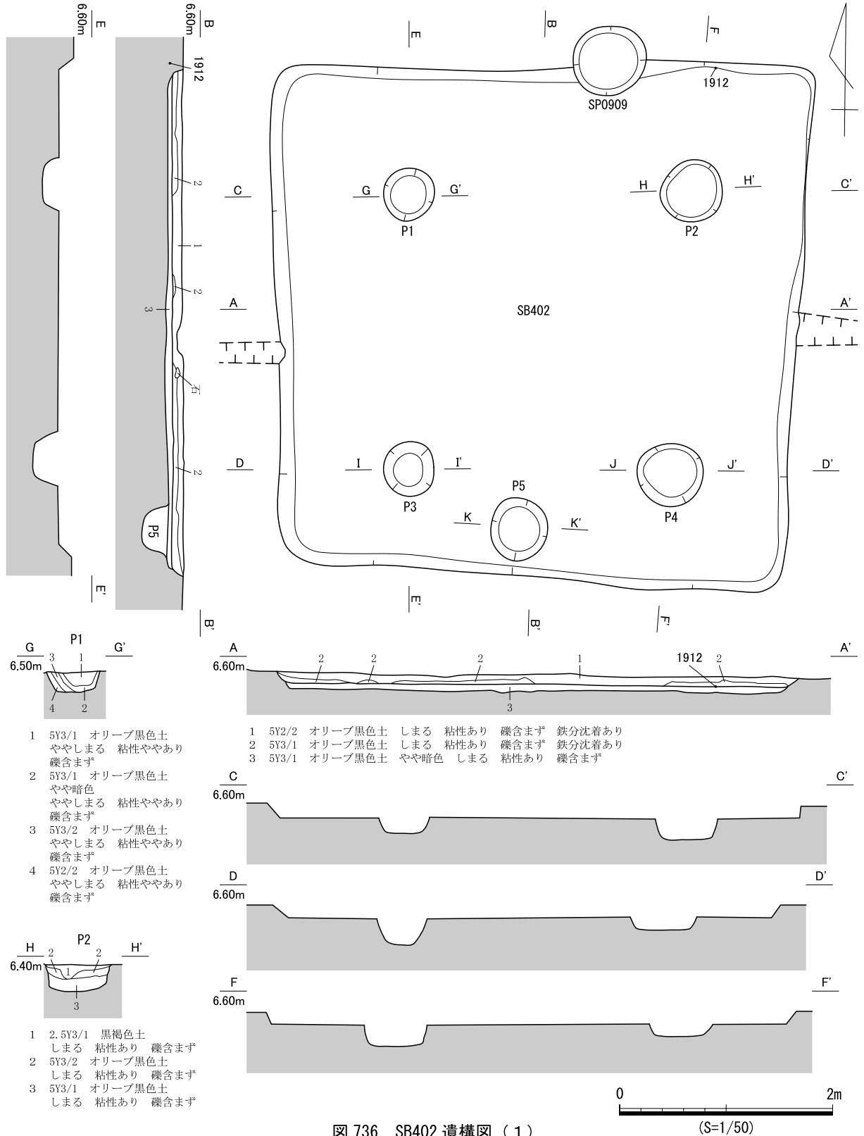
図 736 SB402 遺構図 (1)
