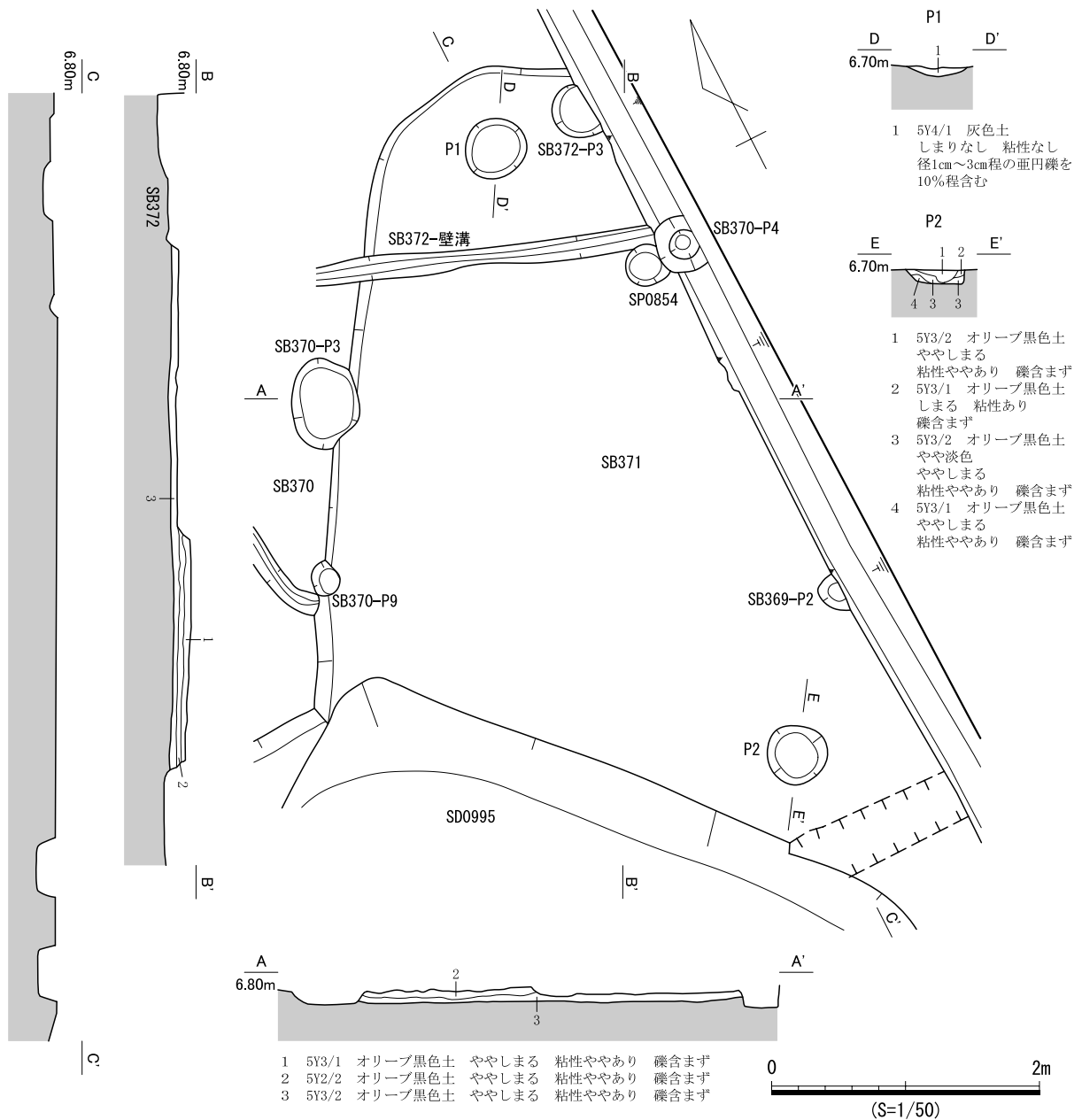
図 661 SB371 遺構図
