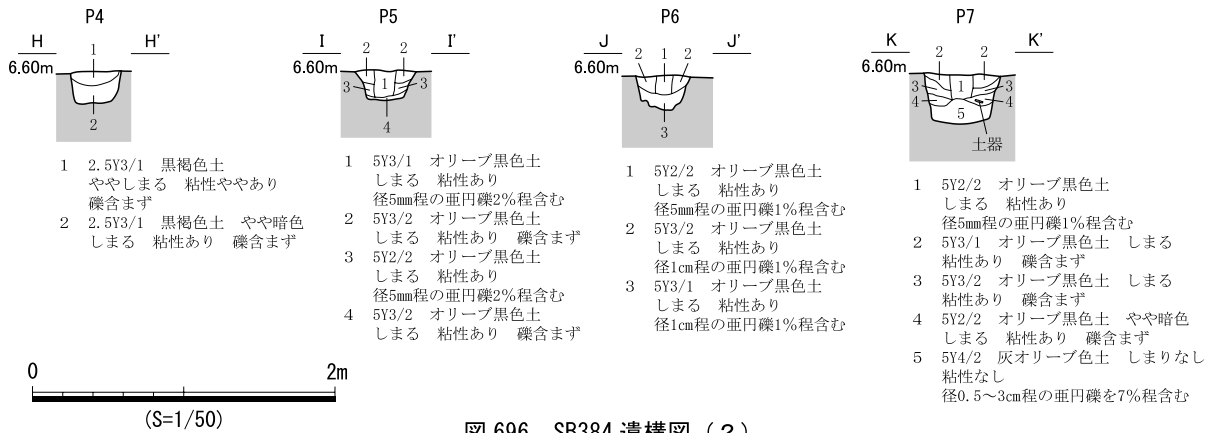
図 696 SB384 遺構図 (2)
