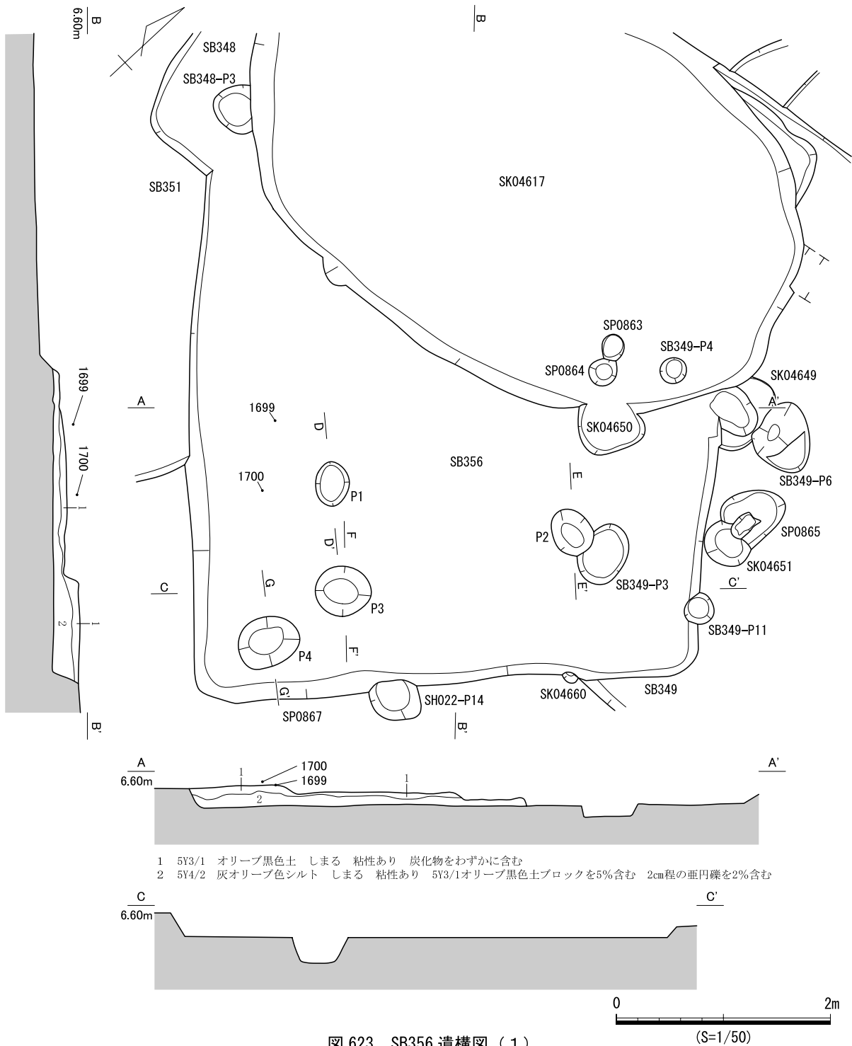
図 623 SB356 遺構図 (1)
