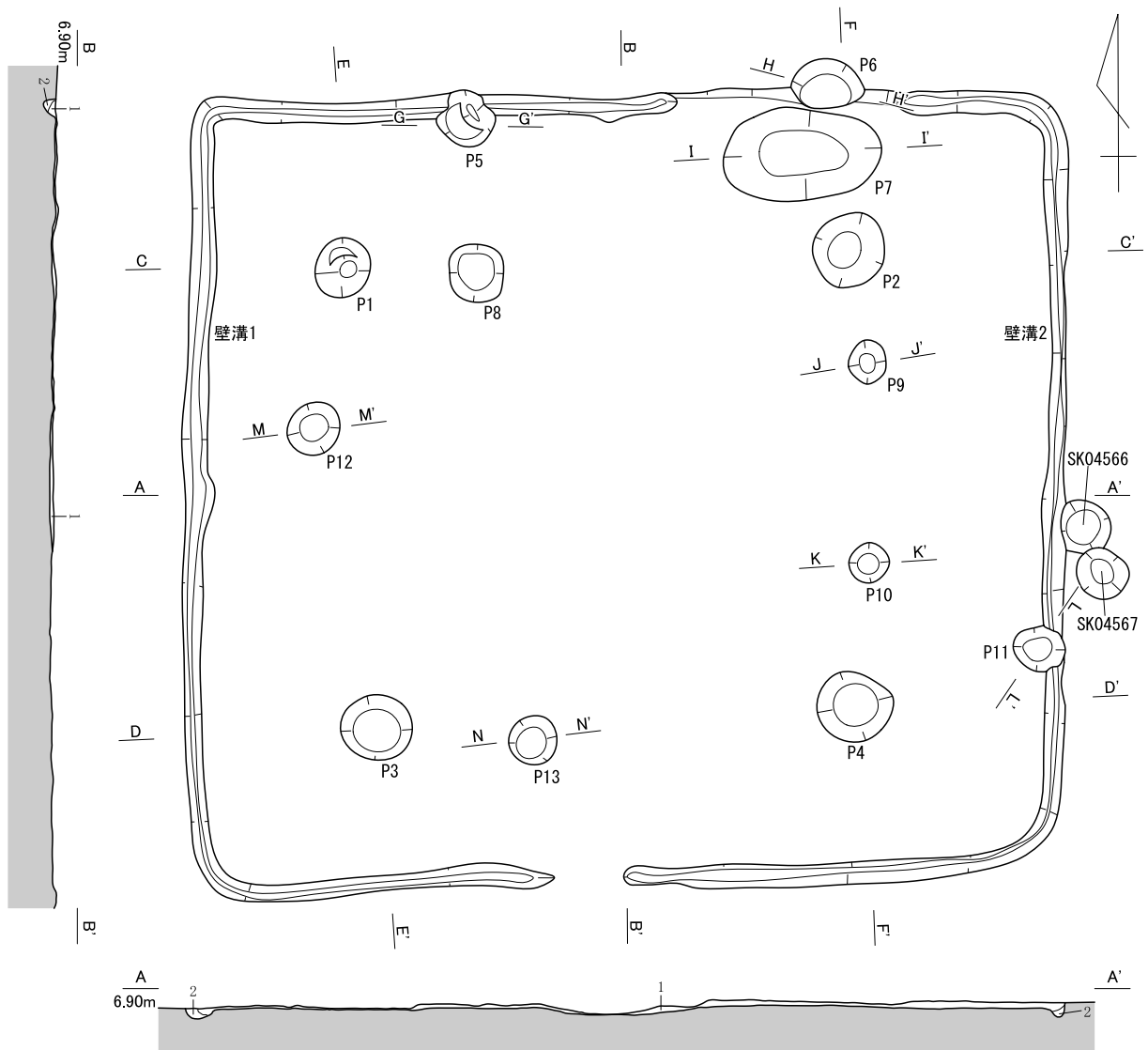
図 634 SB361 遺構図 (1)
