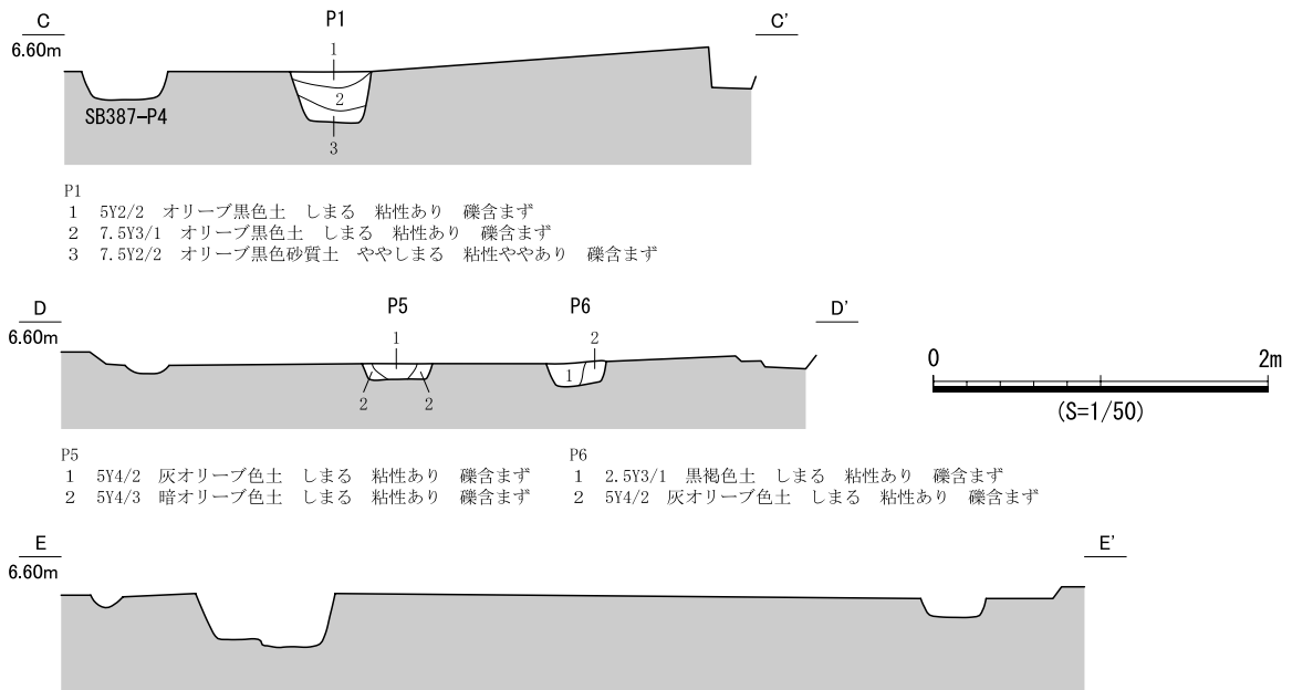
図 715 SB392 遺構図 (2)
