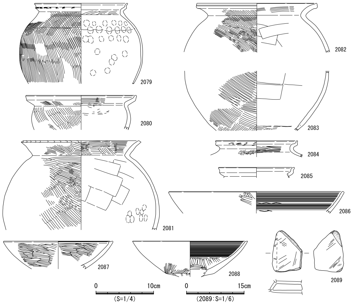
図 830 SB437 遺物実測図
