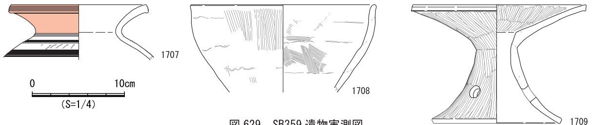
図 629 SB359 遺物実測図
