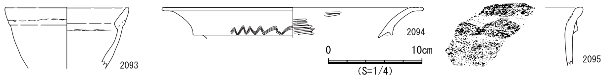
図 843 SB443 遺物実測図
