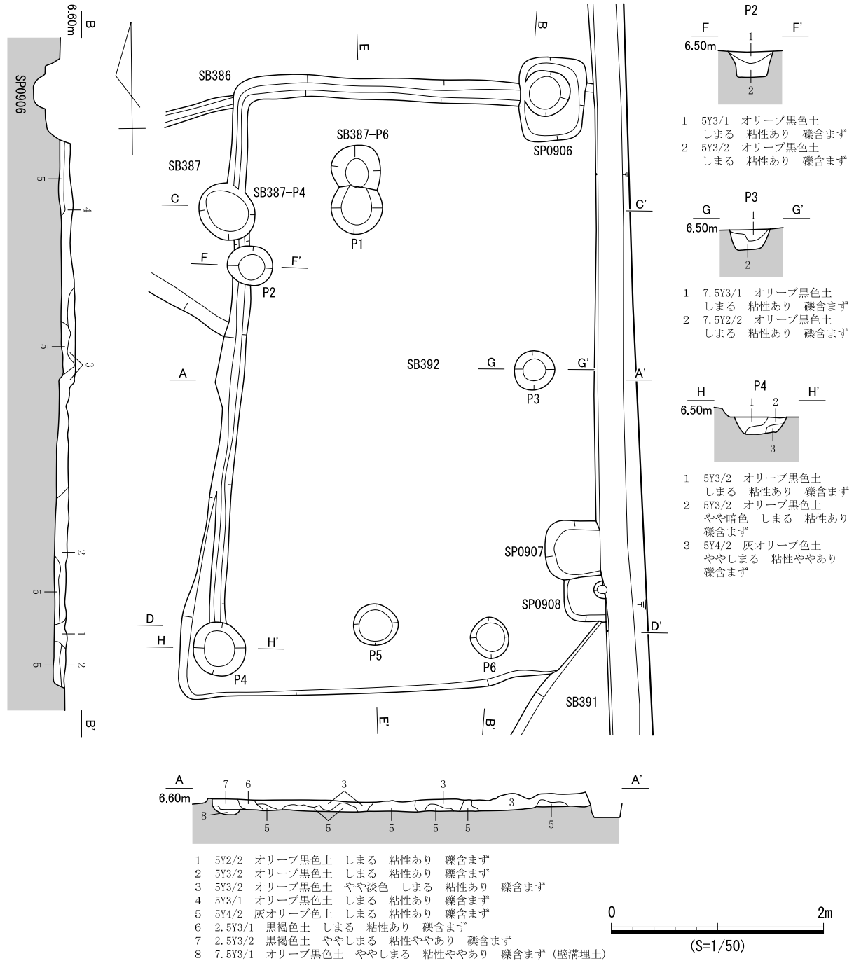
図713 SB392 遺構図 (1)
