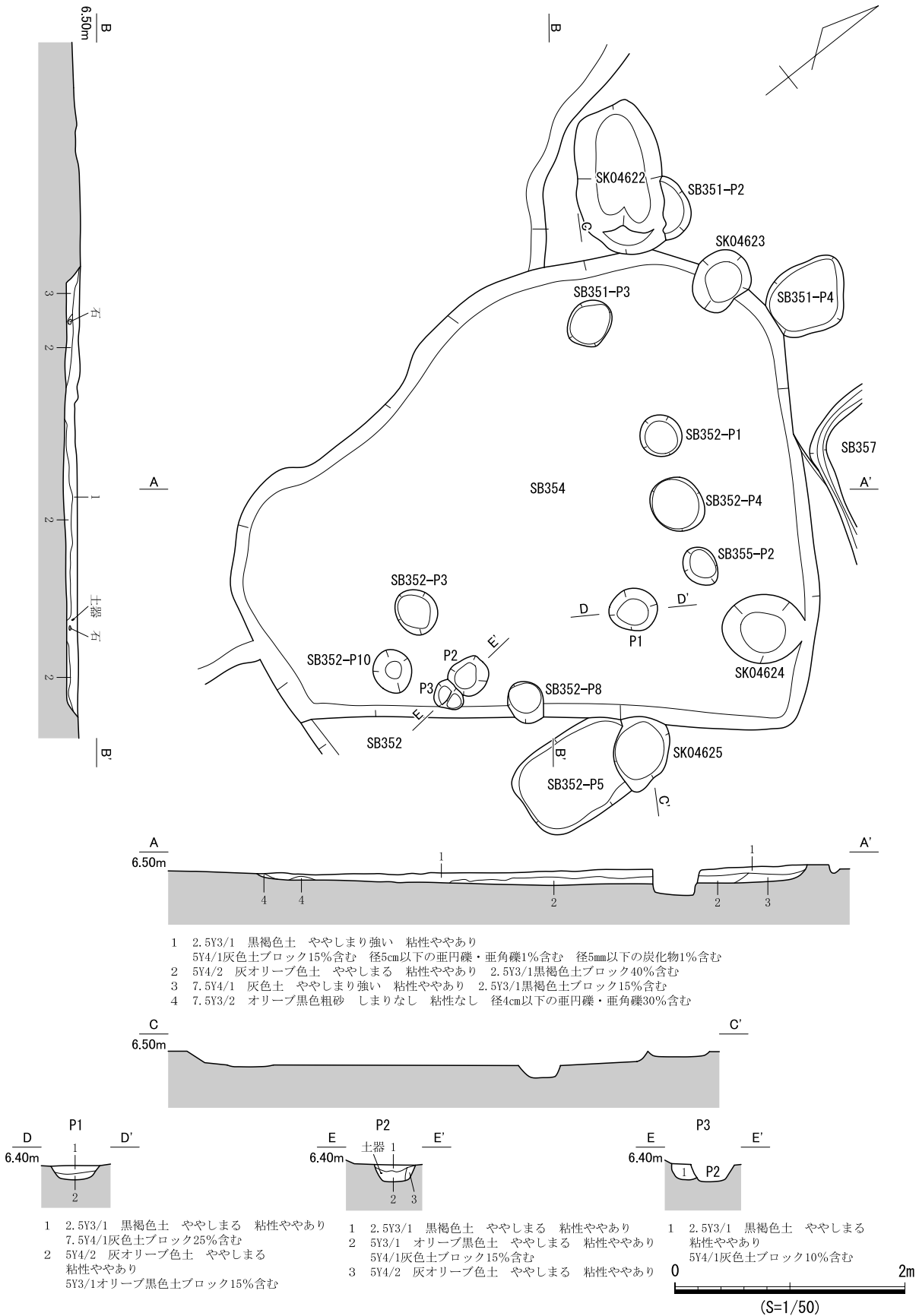
図 621 SB354 遺構図
