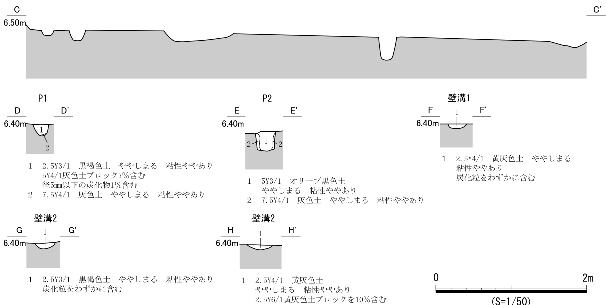
図 788 SB421 遺構図 (2)
