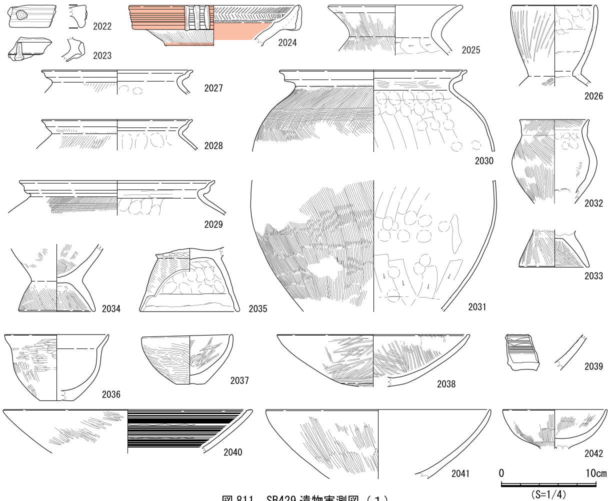
図 811 SB429 遺物実測図 (1)
