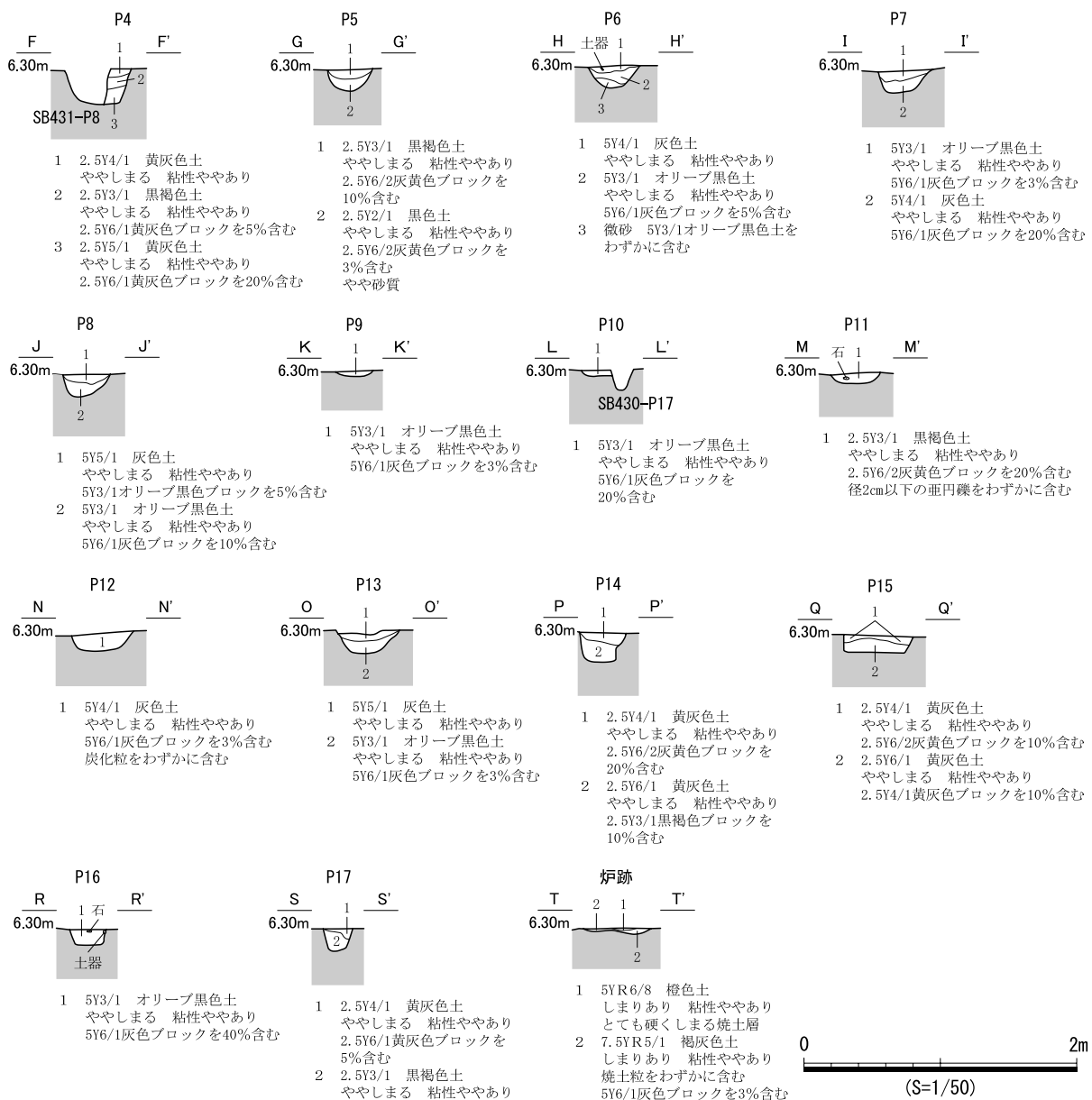
図 819 SB432 遺構図（2）
