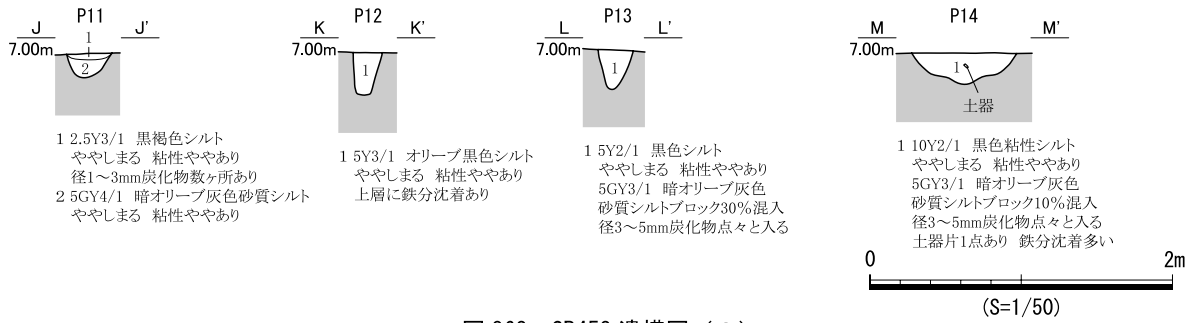
図 863 SB453 遺構図 (2)
