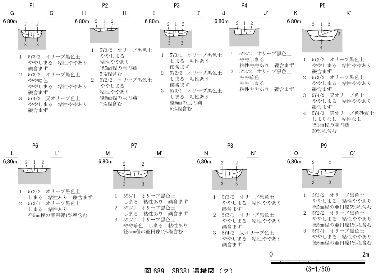
図 689 SB381 遺構図 (2)
