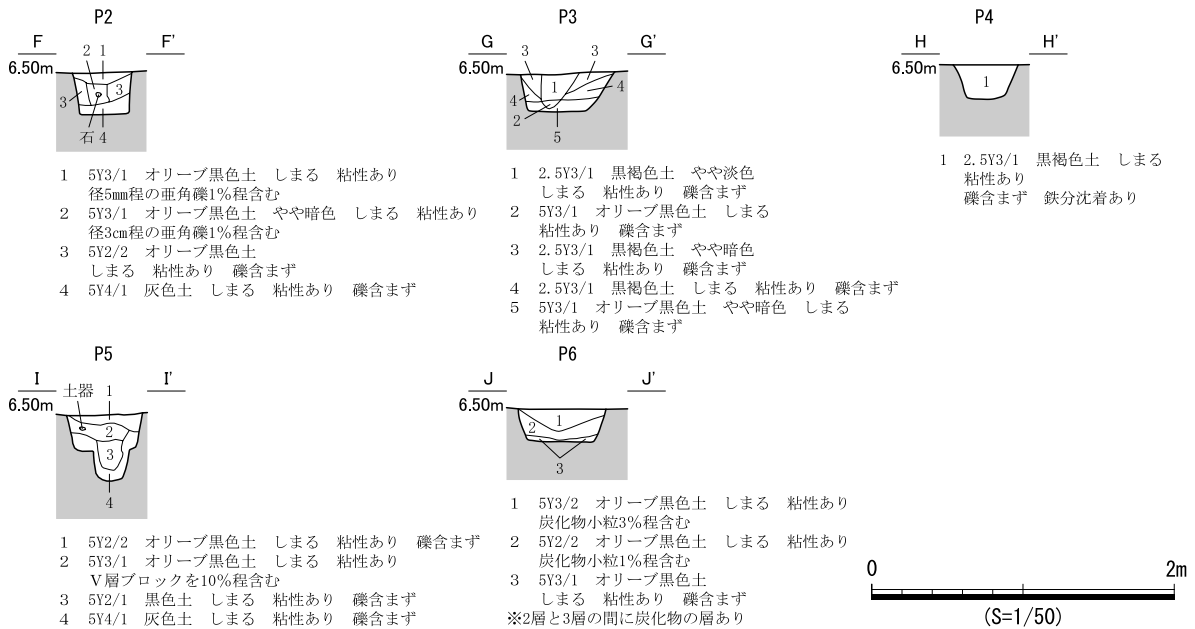
図 836 SB439 遺構図 (2)
