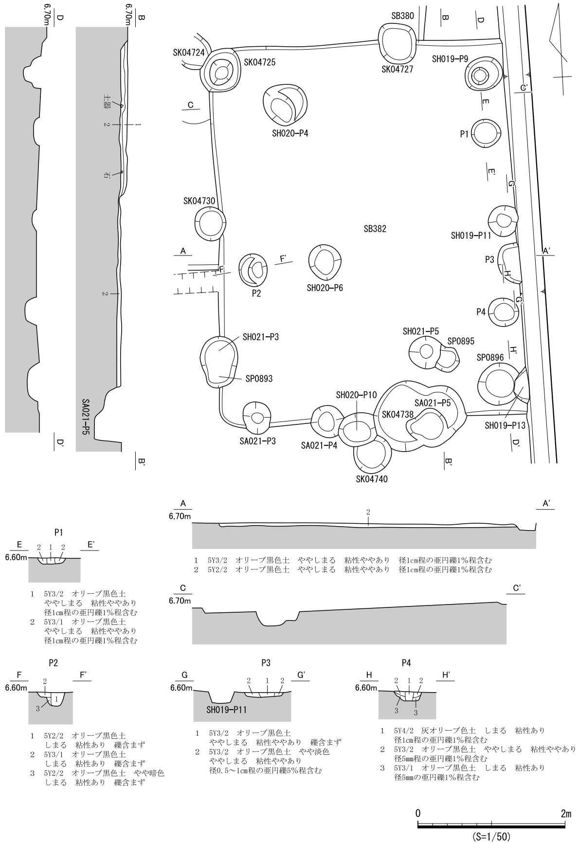
図 691 SB382 遺構図
