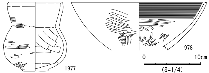
図 784 SB420 遺物実測図
