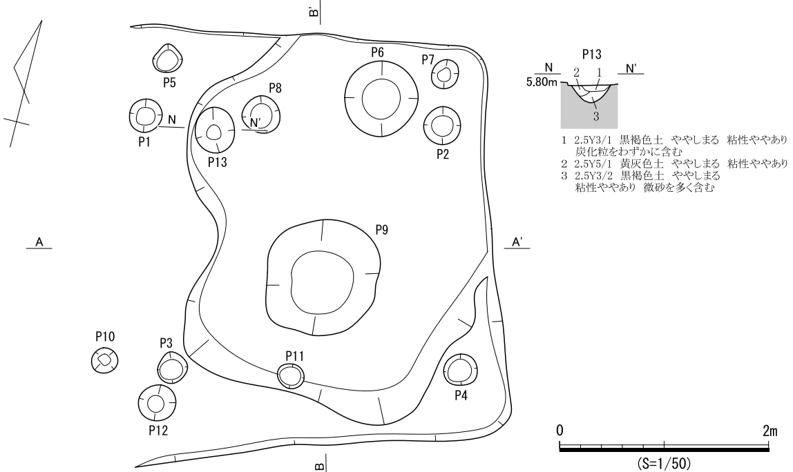
図 848 SB445 遺構図 (2)
