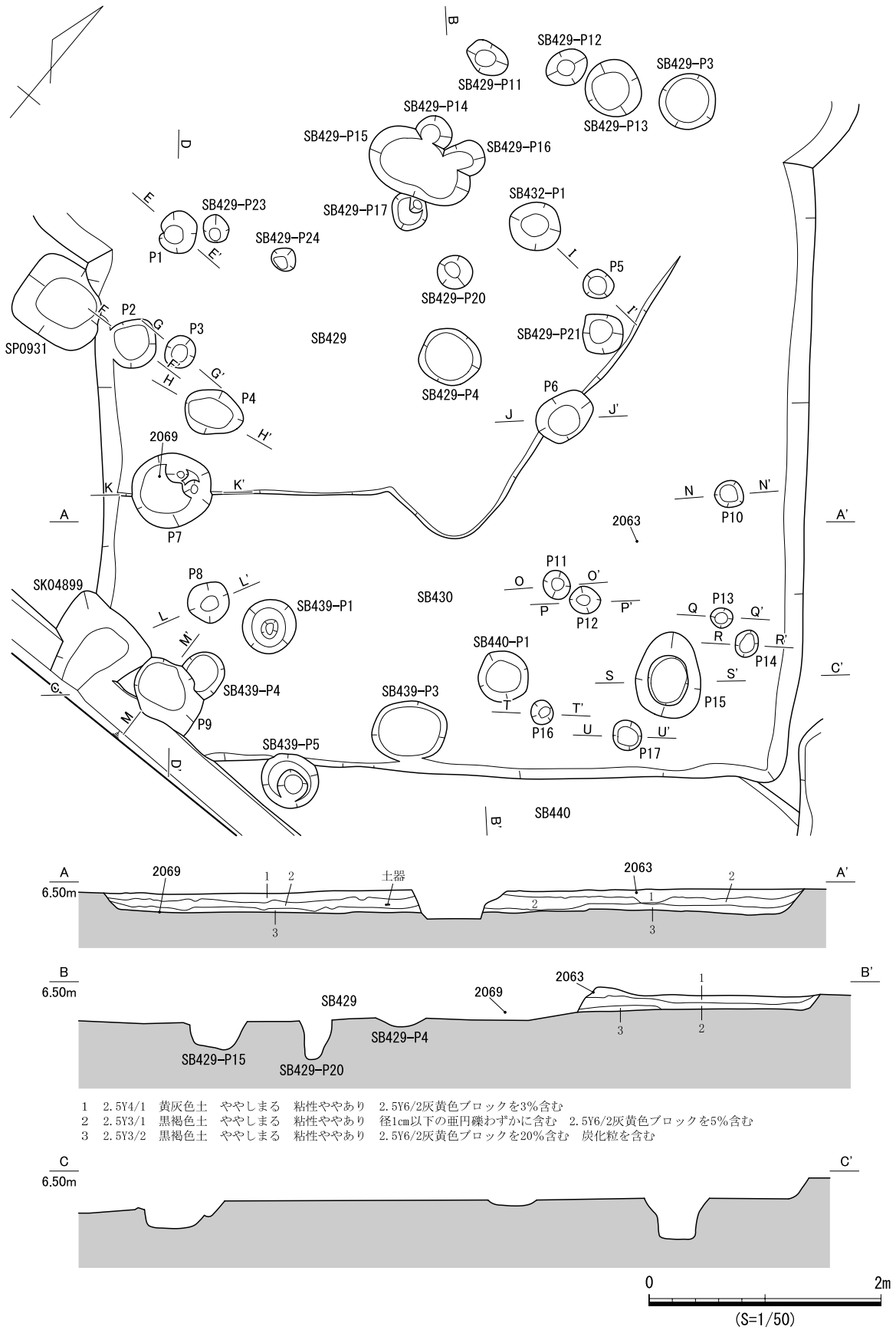
図 814 SB430 遺構図 (1)
