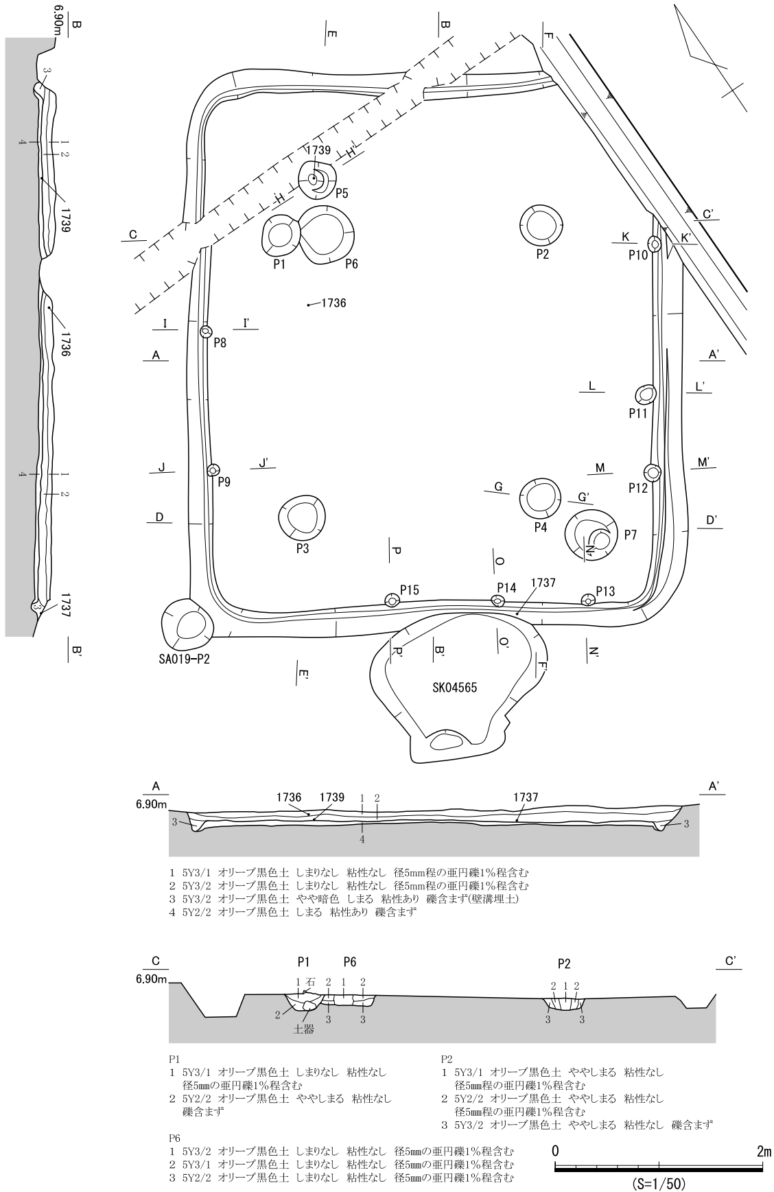
図 644 SB364 遺構図 (1)
