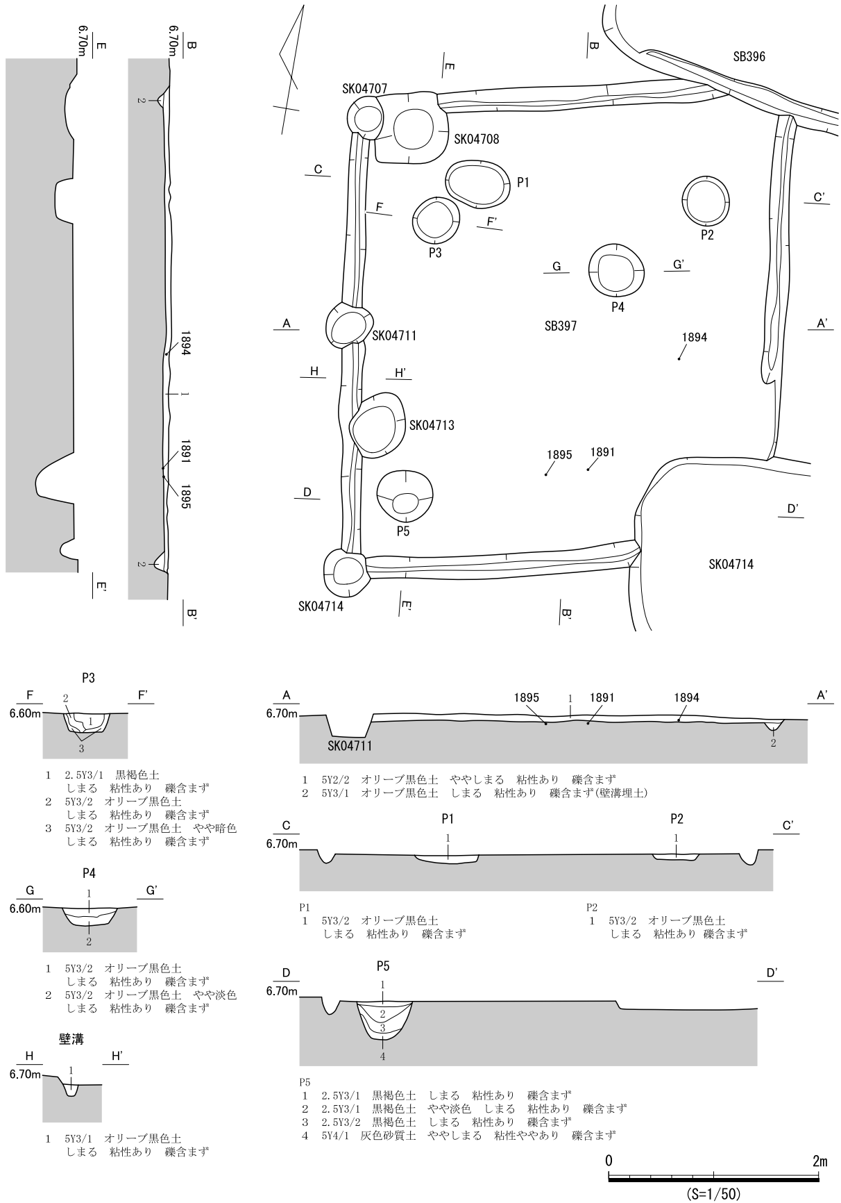
図 728 SB397 遺構図
