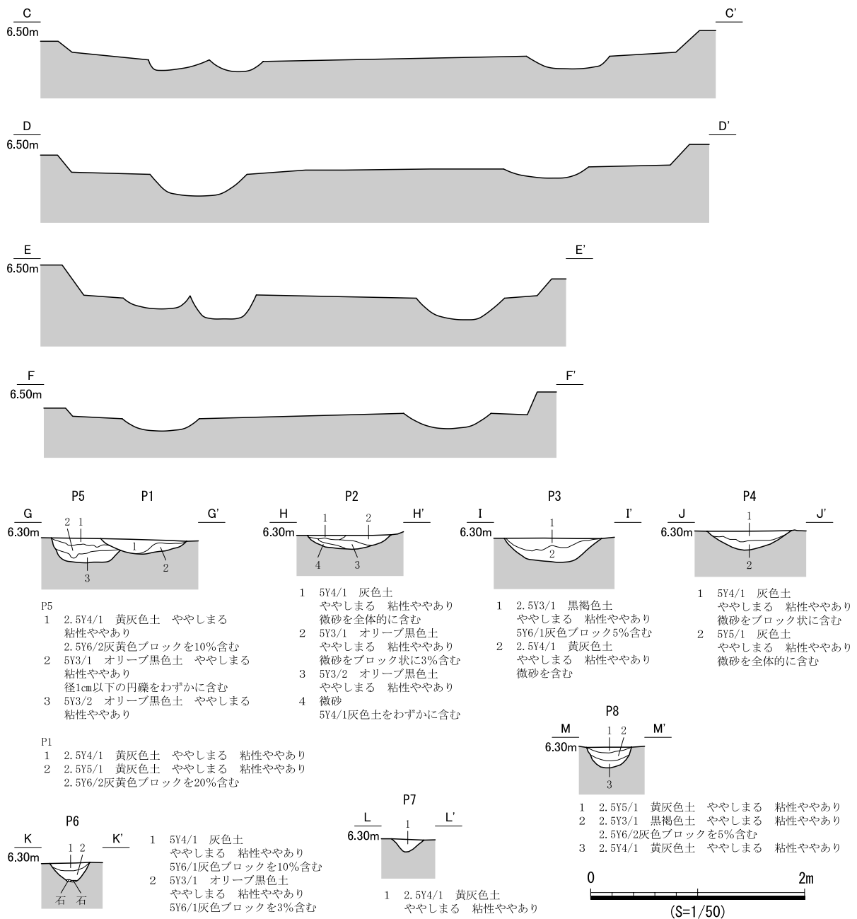
図 799 SB425 遺構図 (2)
