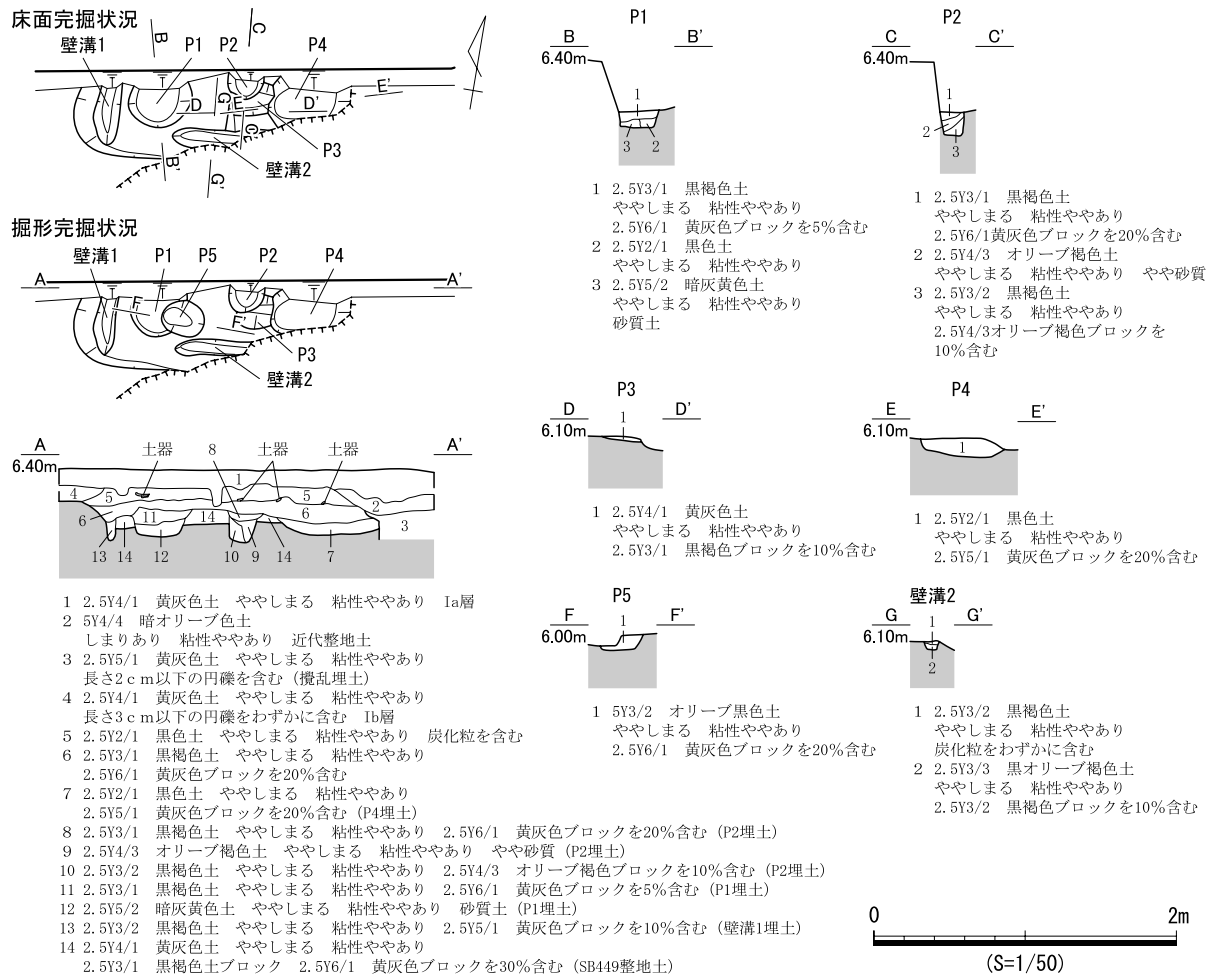
図 852 SB449 遺構図
