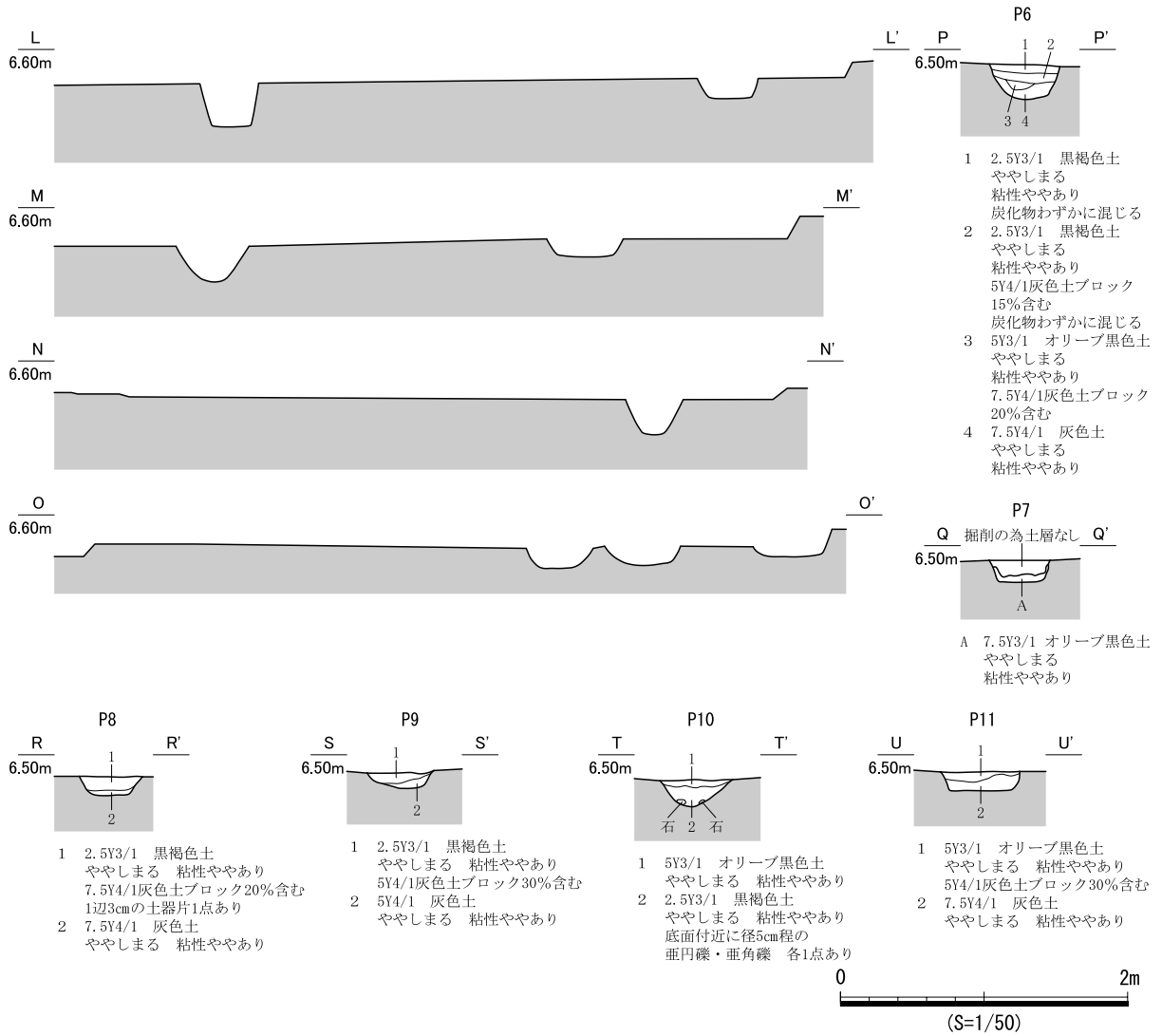
図 616 SB352 遺構図 (3)
