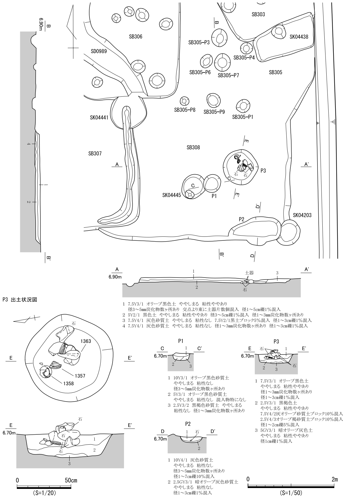
図 506 SB308 遺構図
