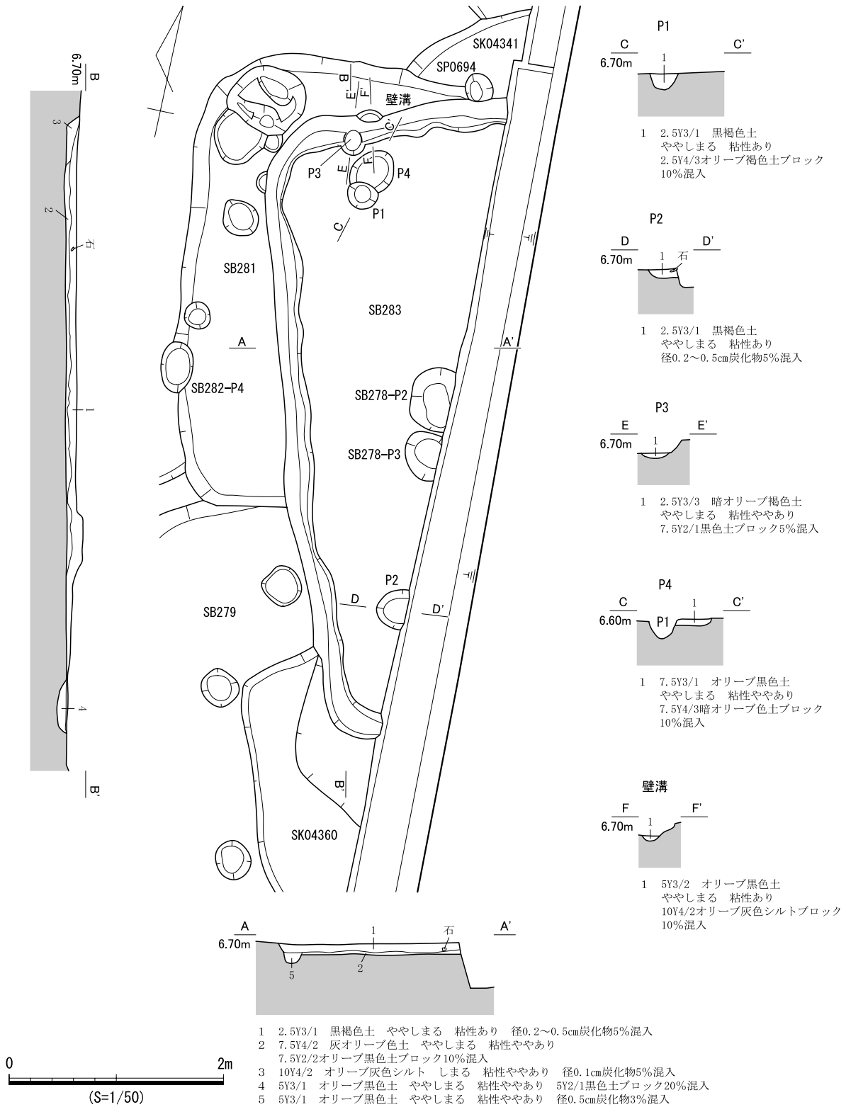
図 450 SB283 遺構図
