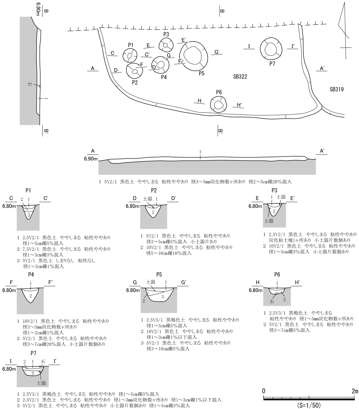
図 538 SB322 遺構図
