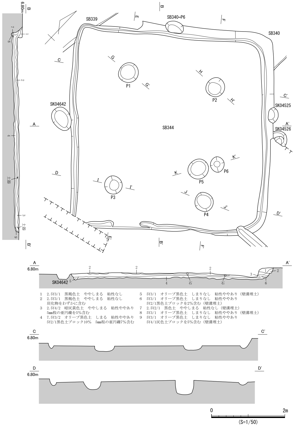
図 598 SB344 遺構図 (1)
