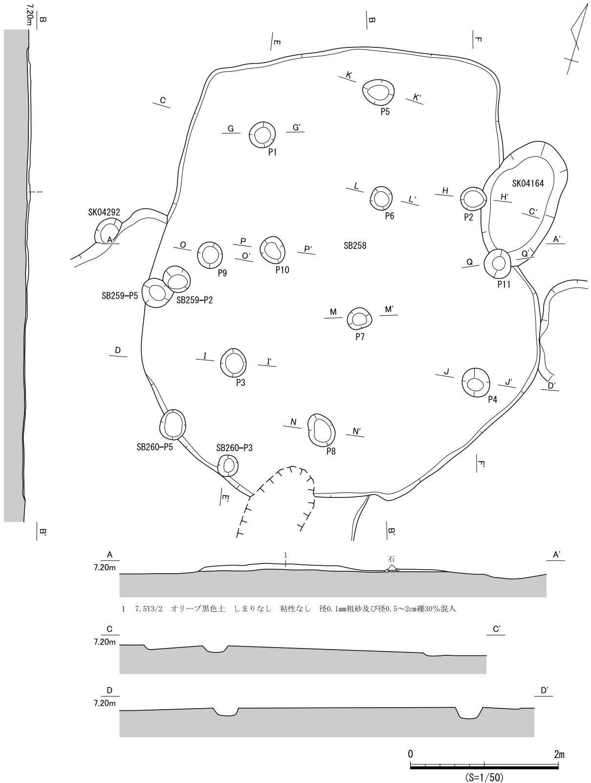
図388 SB258 遺構図(1)
