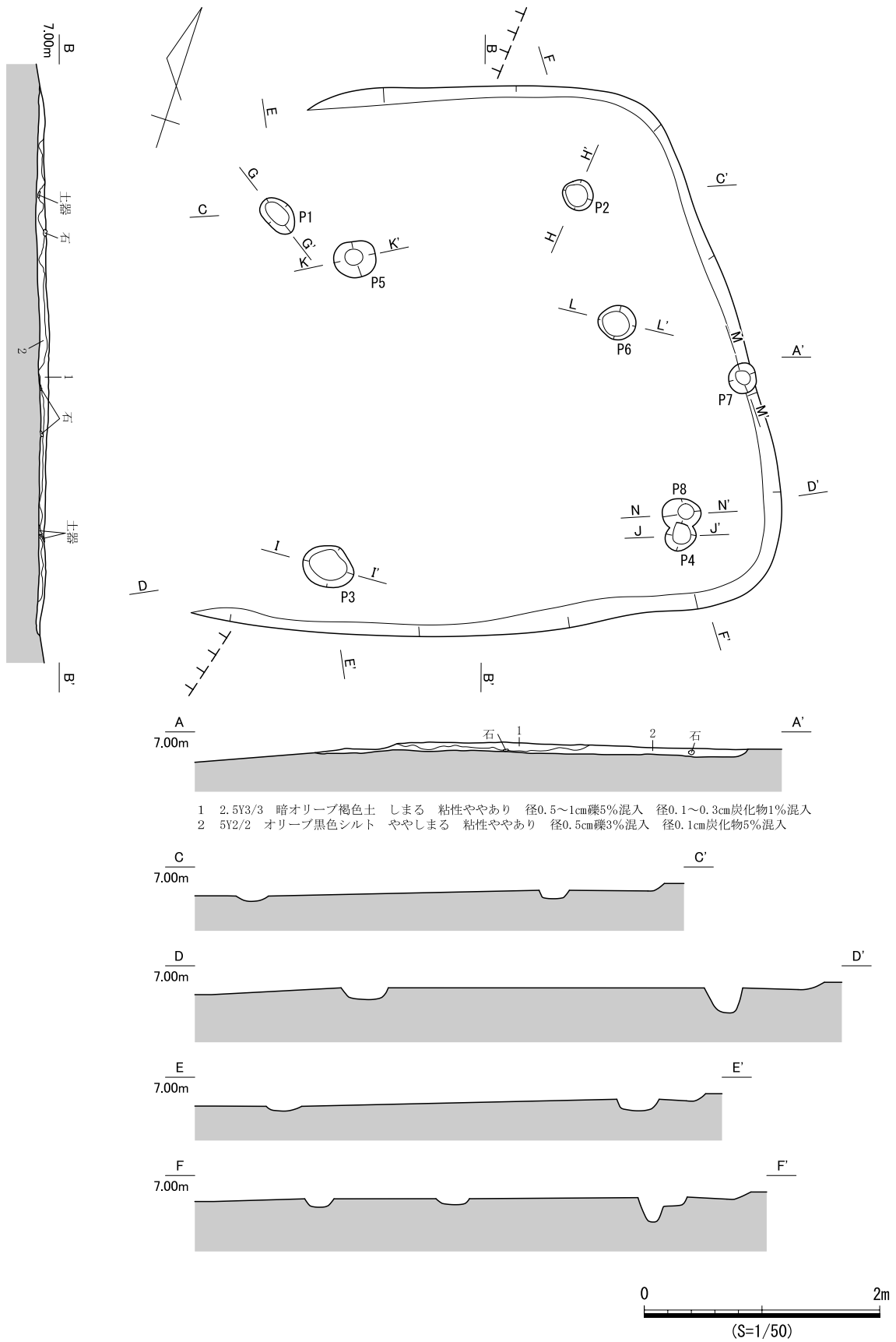
図 411 SB267 遺構図 (1)
