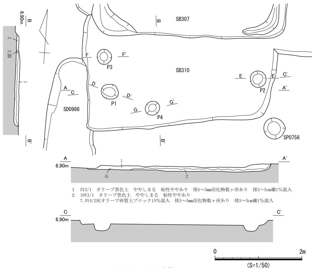
図508 SB310遺構図(1)
