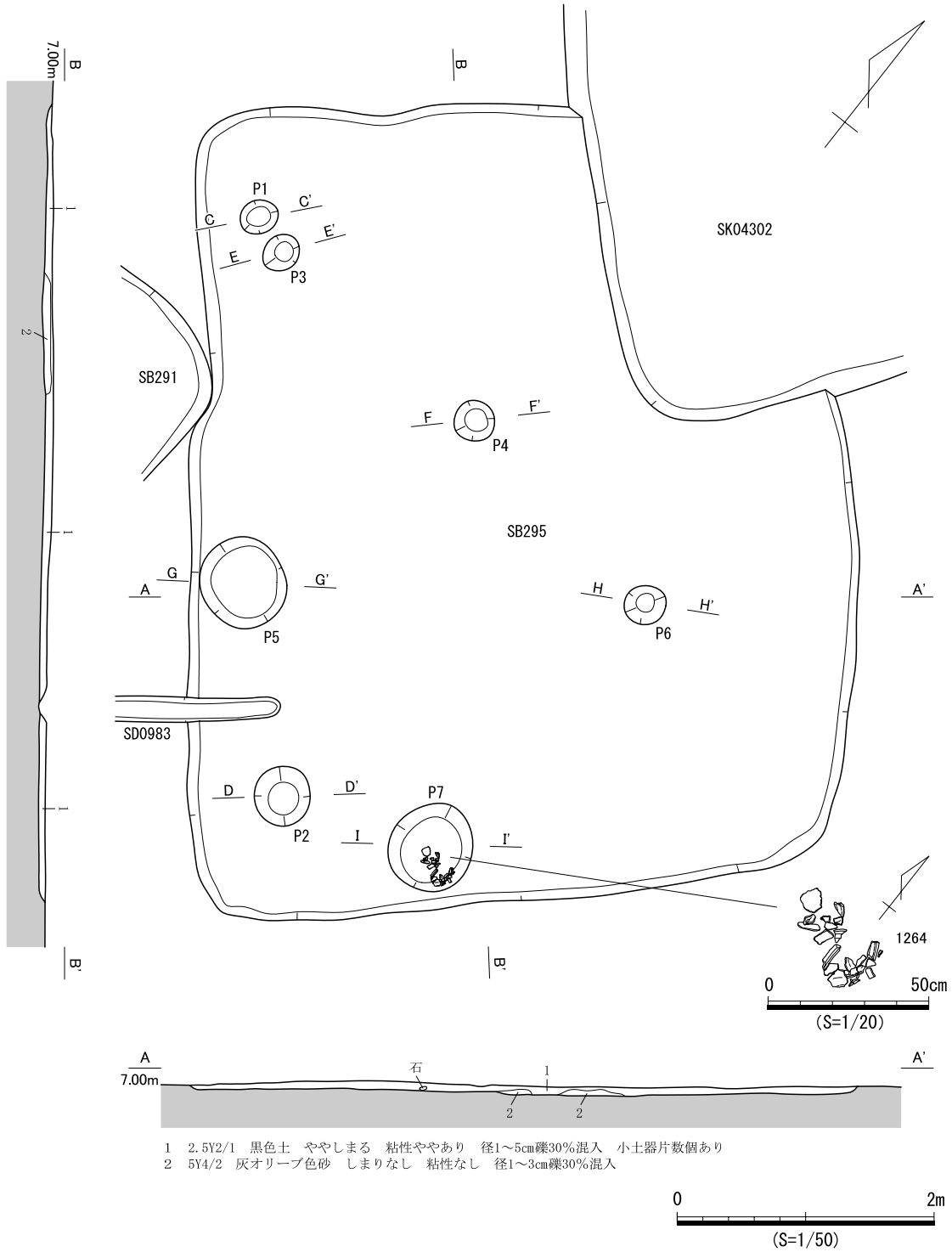
図472 SB295 遺構図(1)
