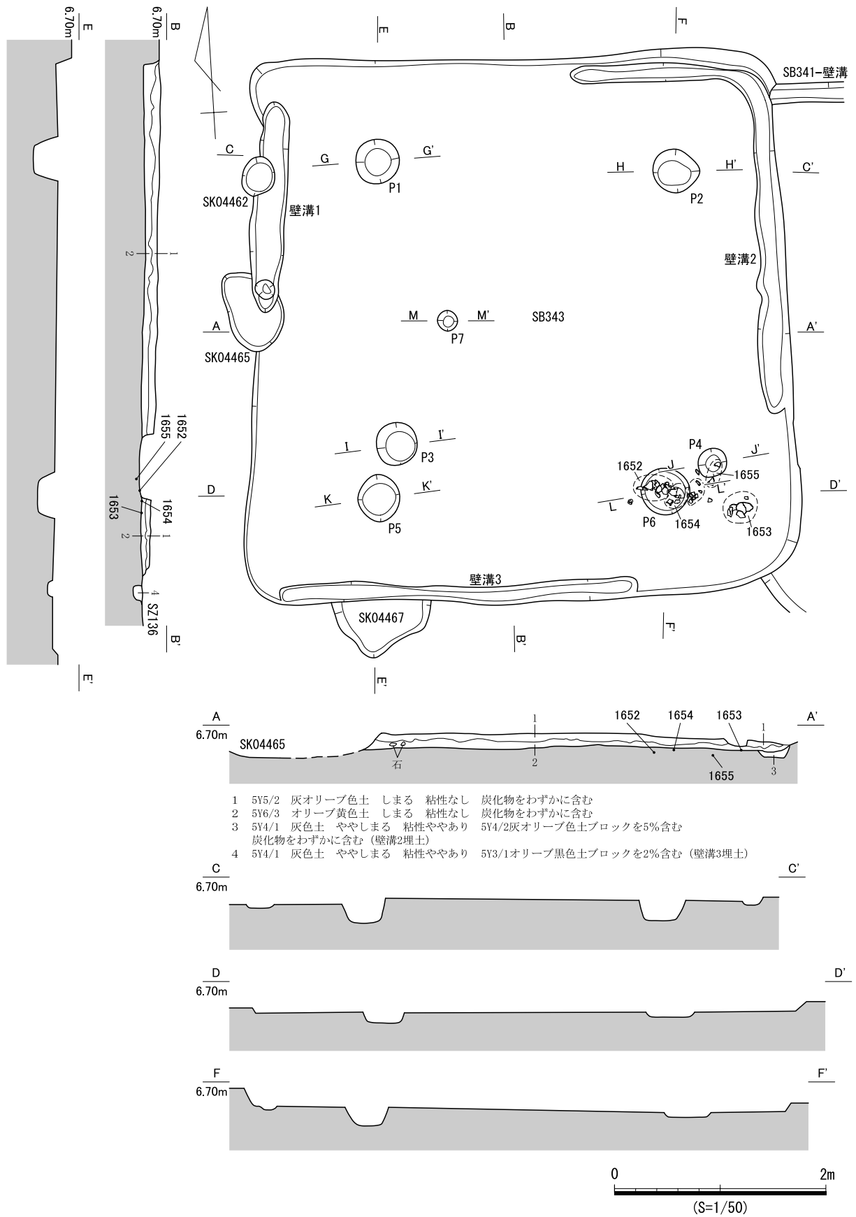
図 594 SB343 遺構図 (1)
