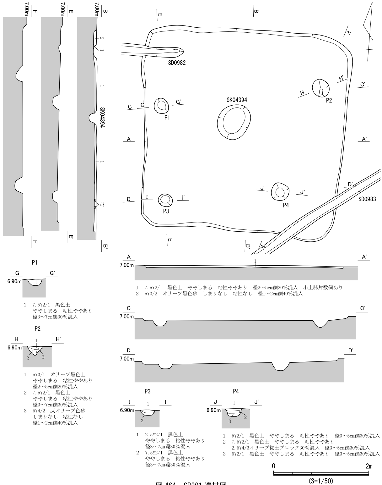
図 464 SB291 遺構図
