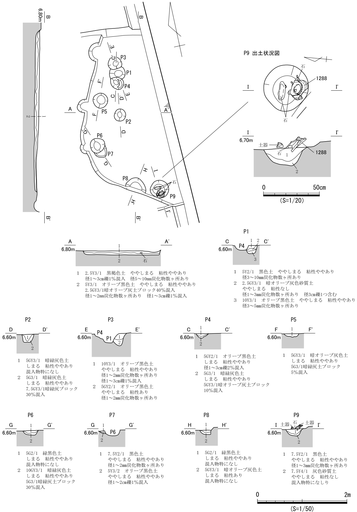
図 485 SB300 遺構図
