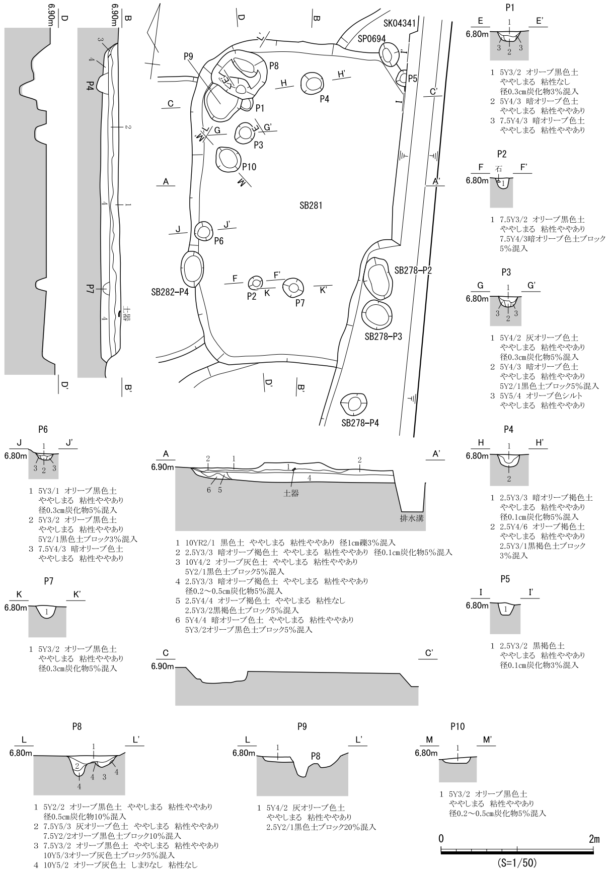
図 446 SB281 遺構図
