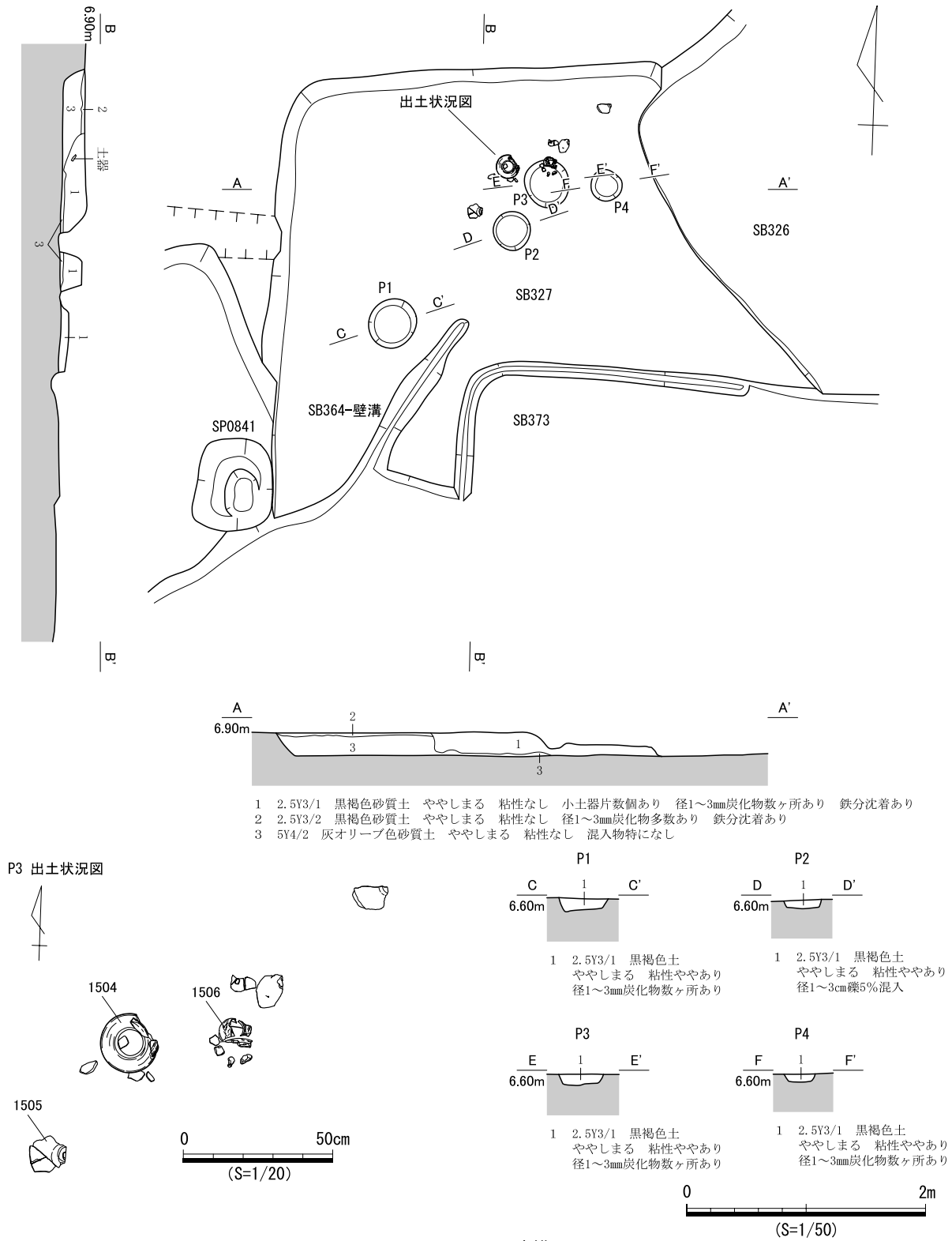
図 551 SB327 遺構図
