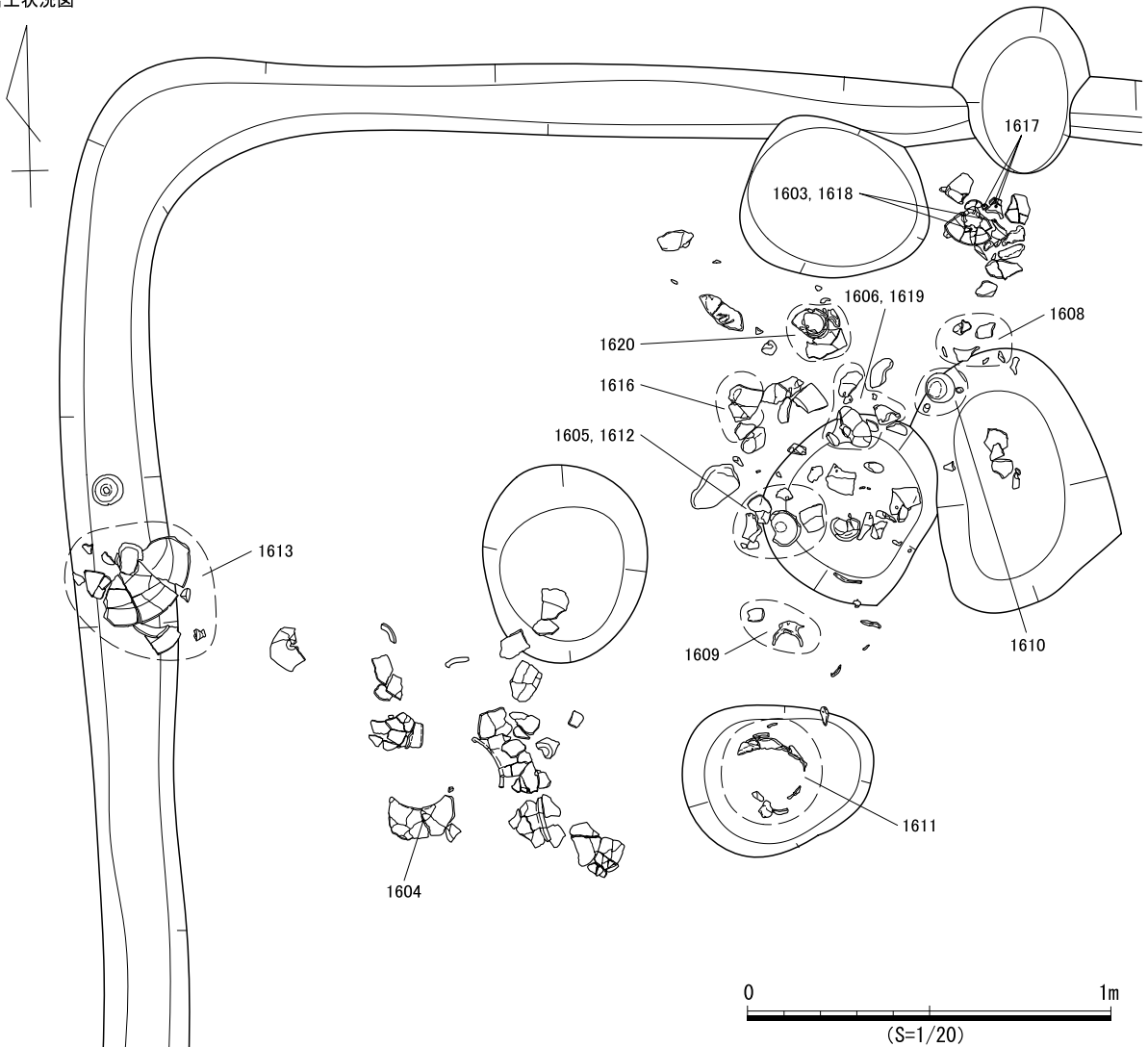
図 589 SB341 遺構図 (2)
