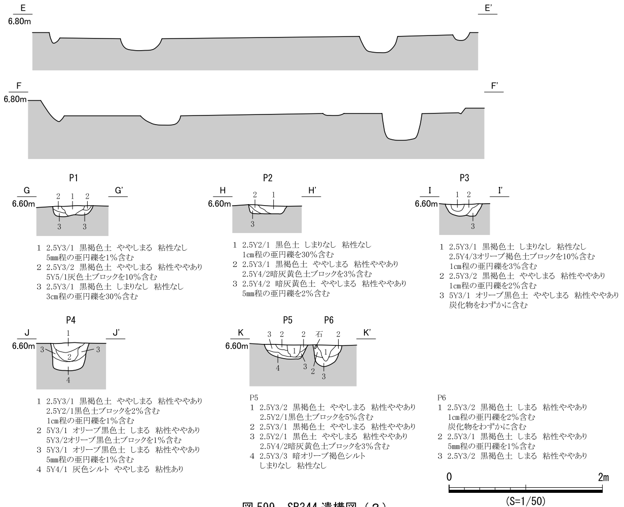
図 599 SB344 遺構図 (2)
