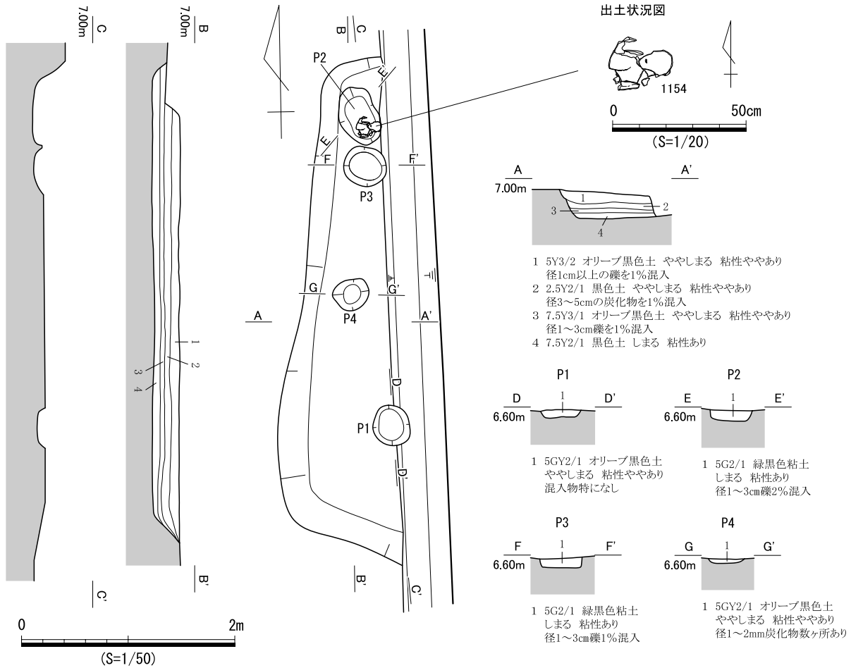
図437 SB278 遺構図
