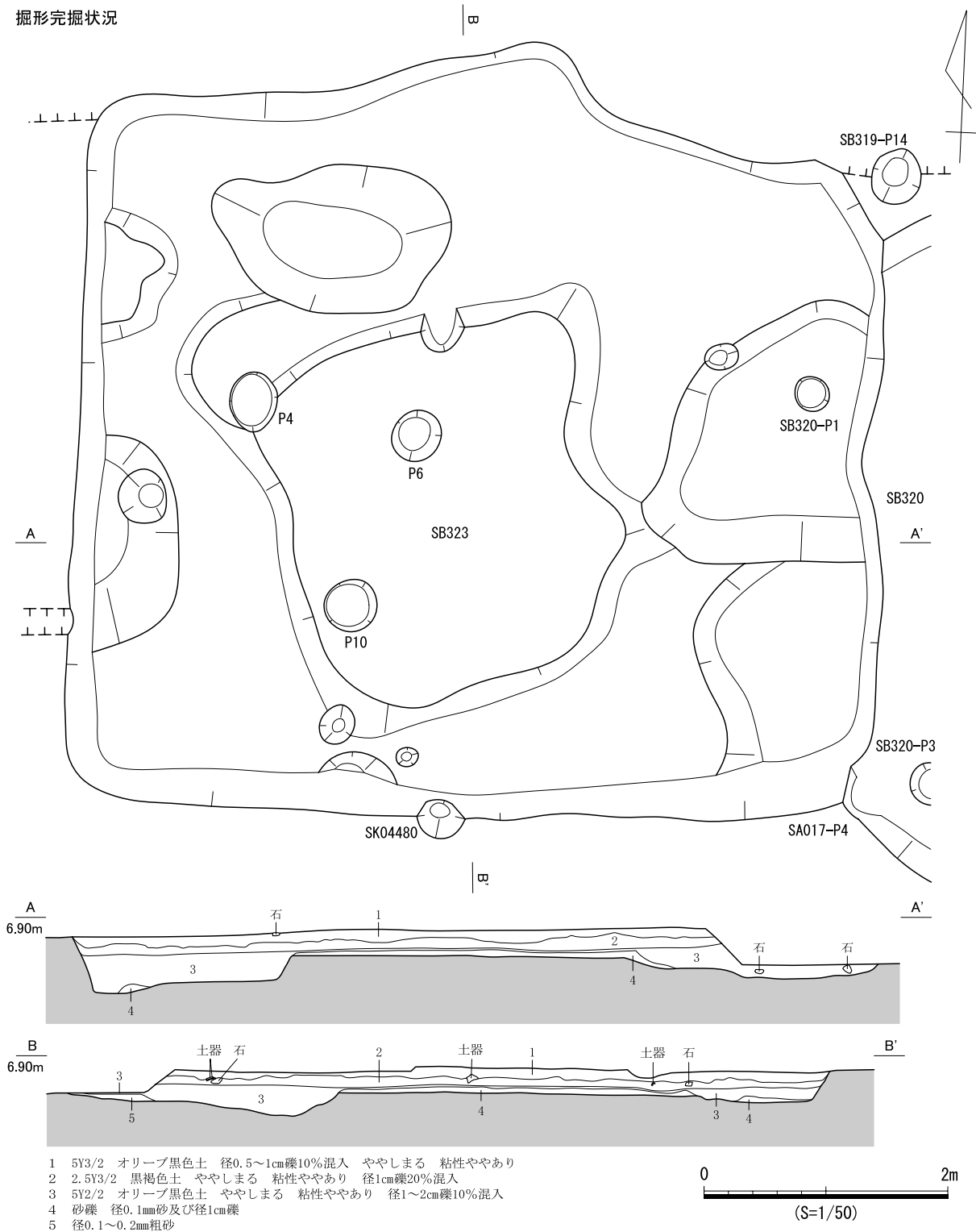
図 541 SB323 遺構図 (2)
