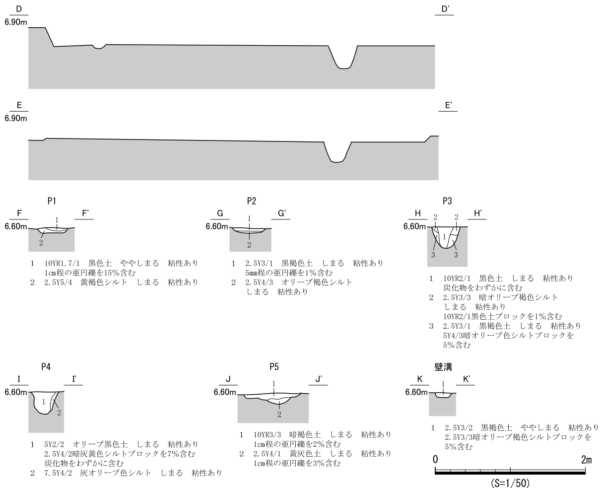
図 592 SB342 遺構図 (2)
