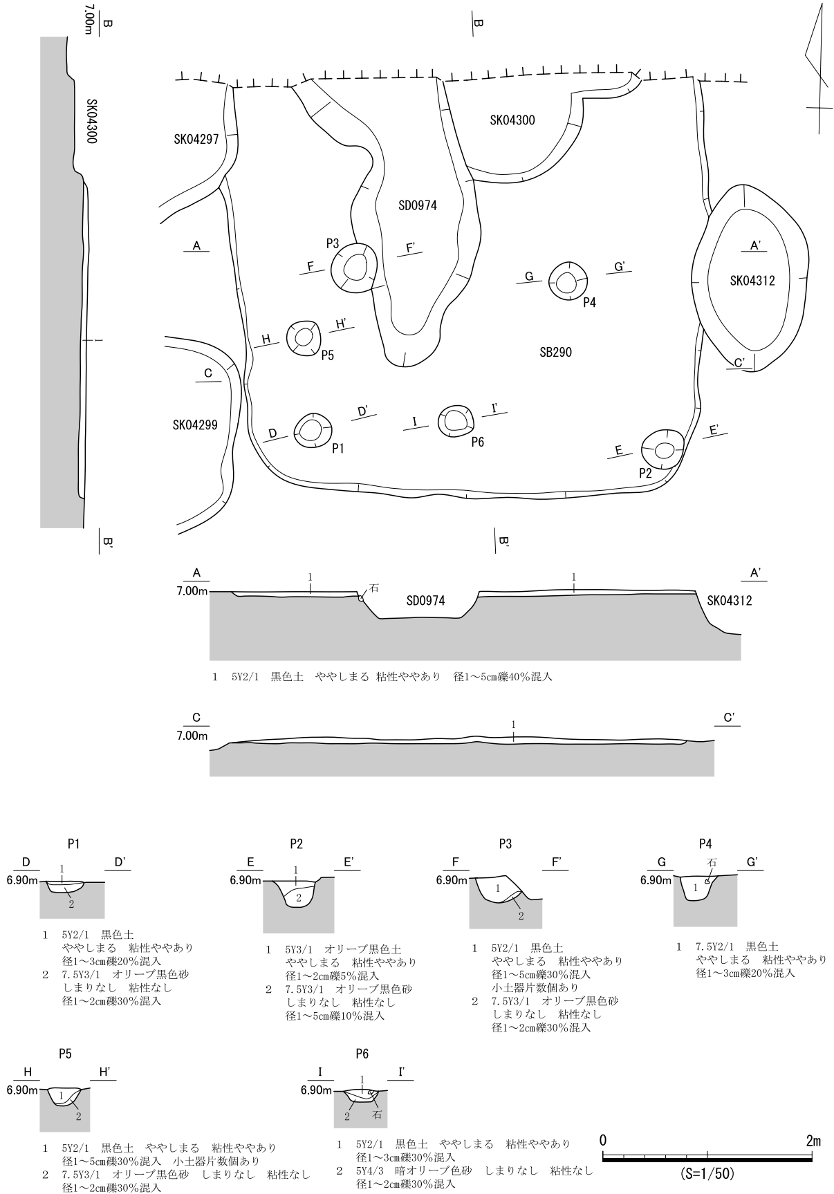
図 463 SB290 遺構図
