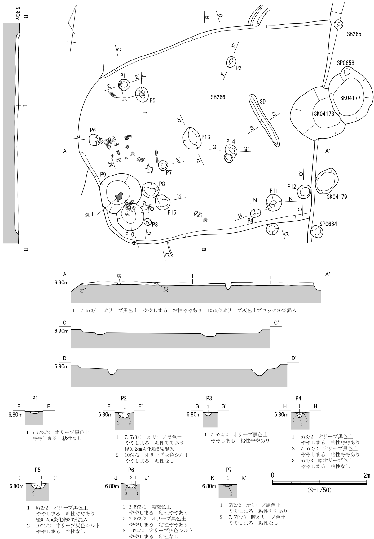
図 408 SB266 遺構図 (1)
