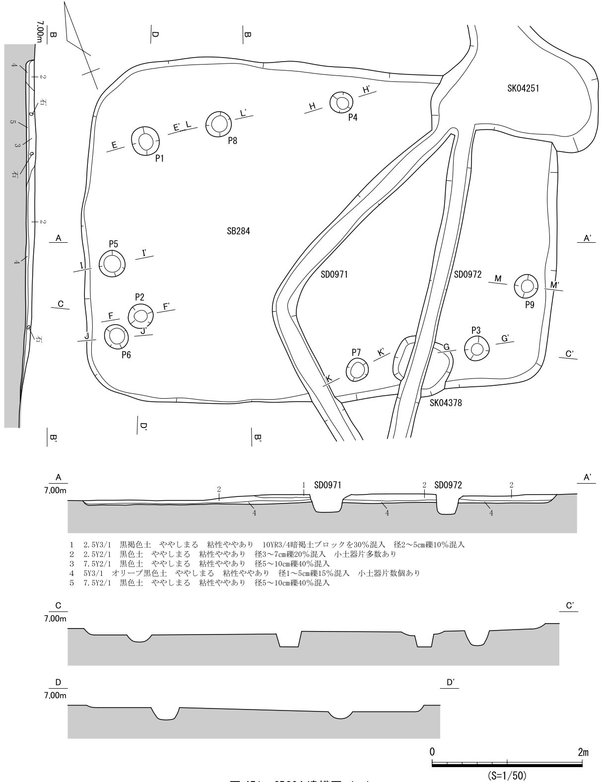
図451 SB284 遺構図(1)
