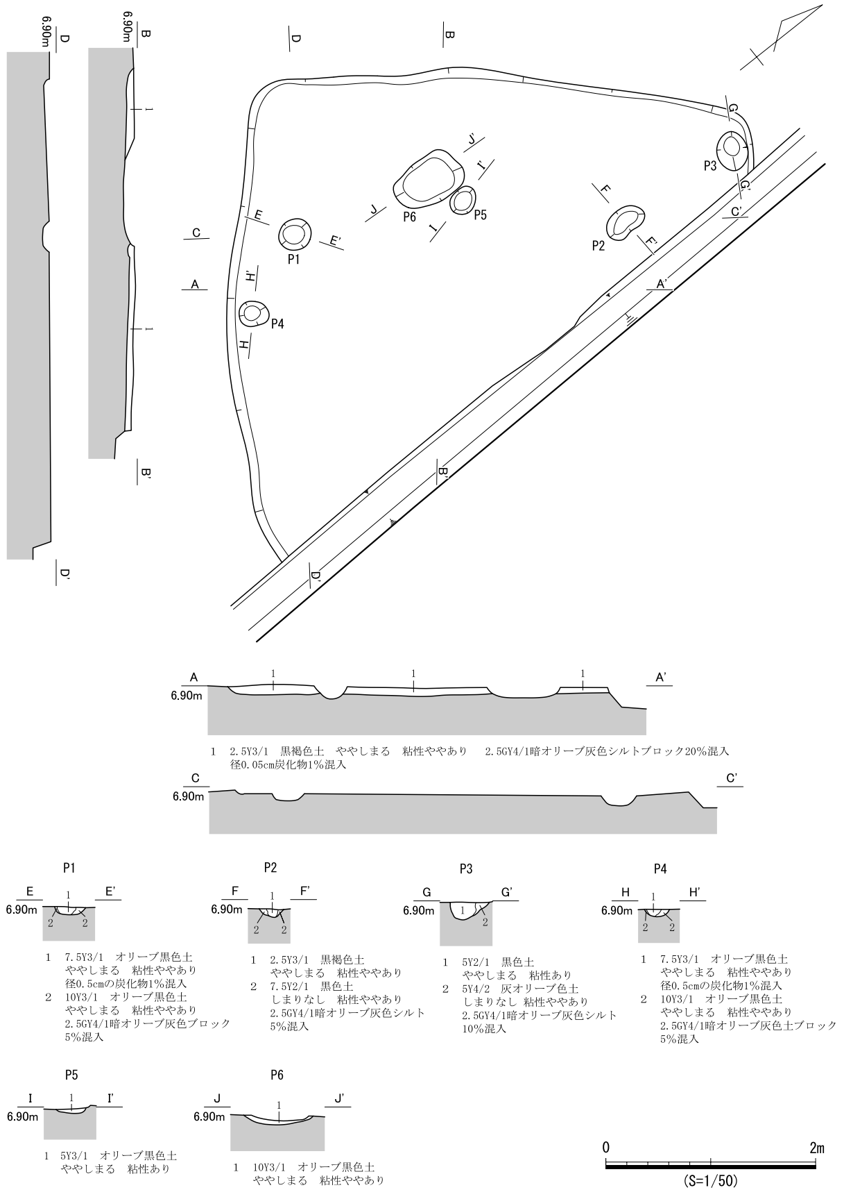
図 415 SB269 遺構図
