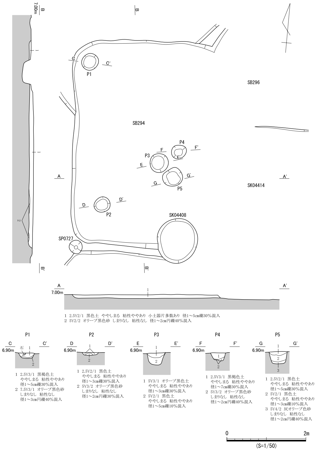
図 471 SB294 遺構図
