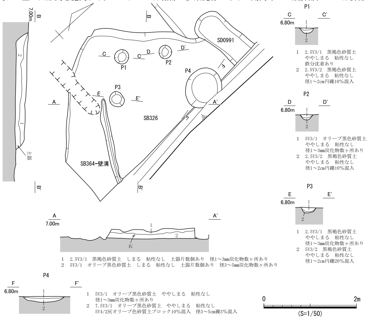
図 548 SB326 遺構図
