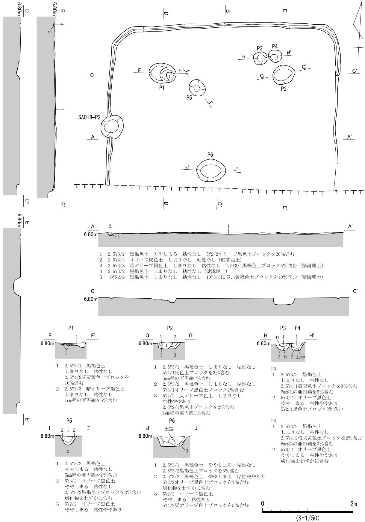
図 587 SB340 遺構図
