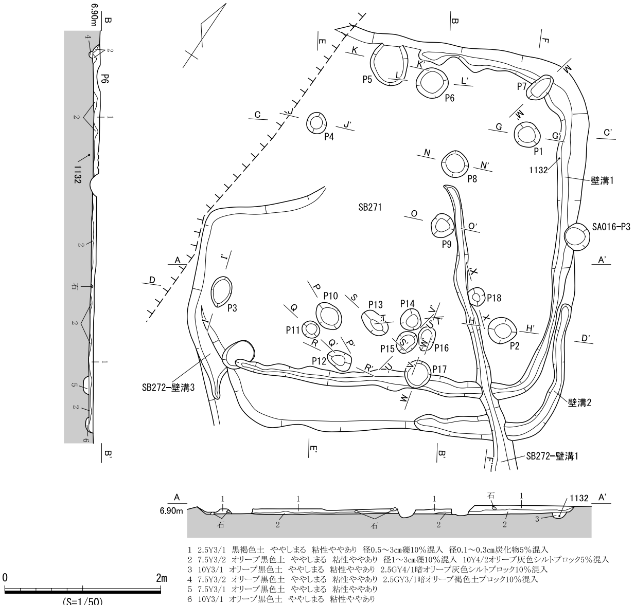
図419 SB271 遺構図(1)
