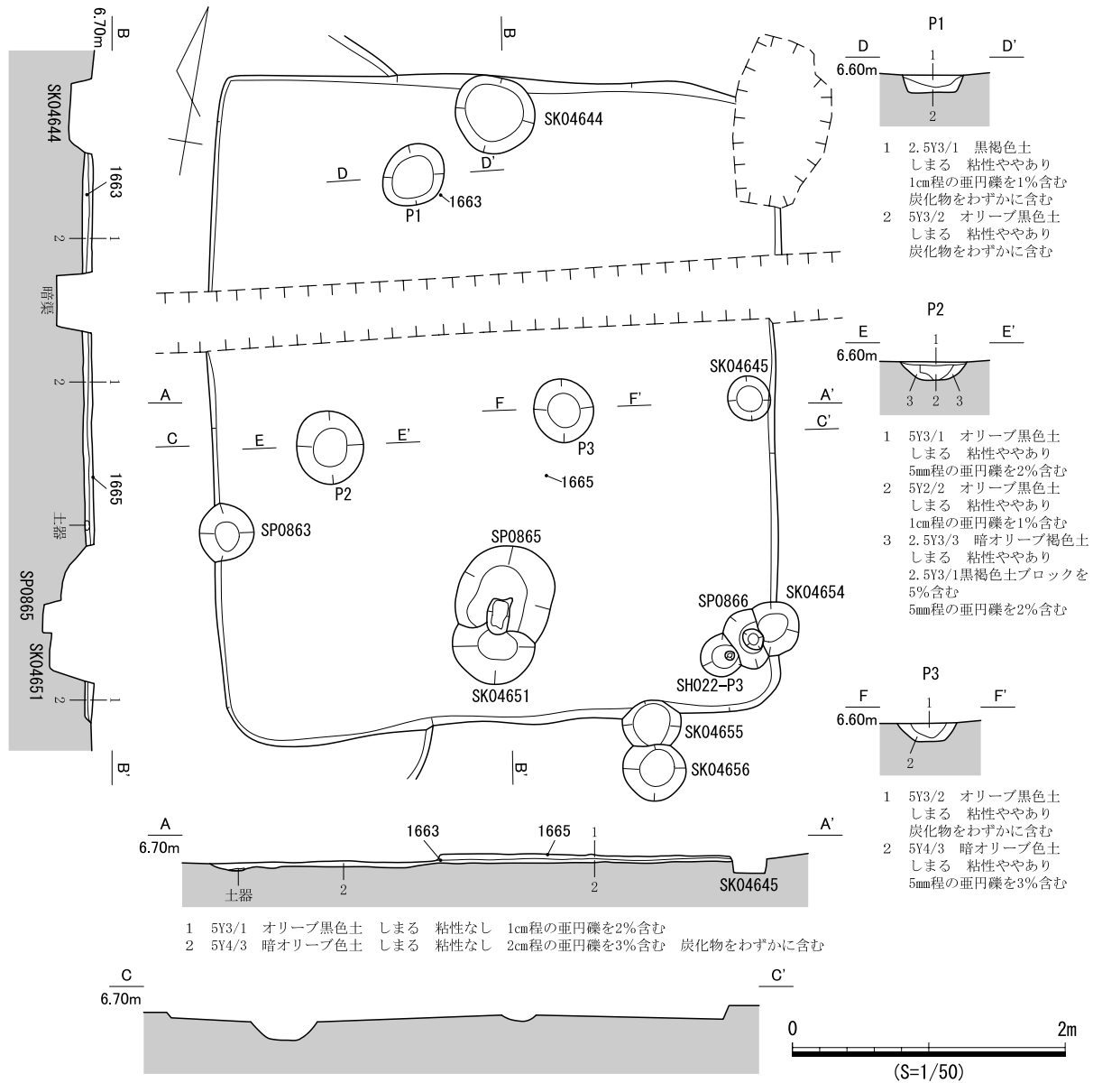
図 600 SB345 遺構図
