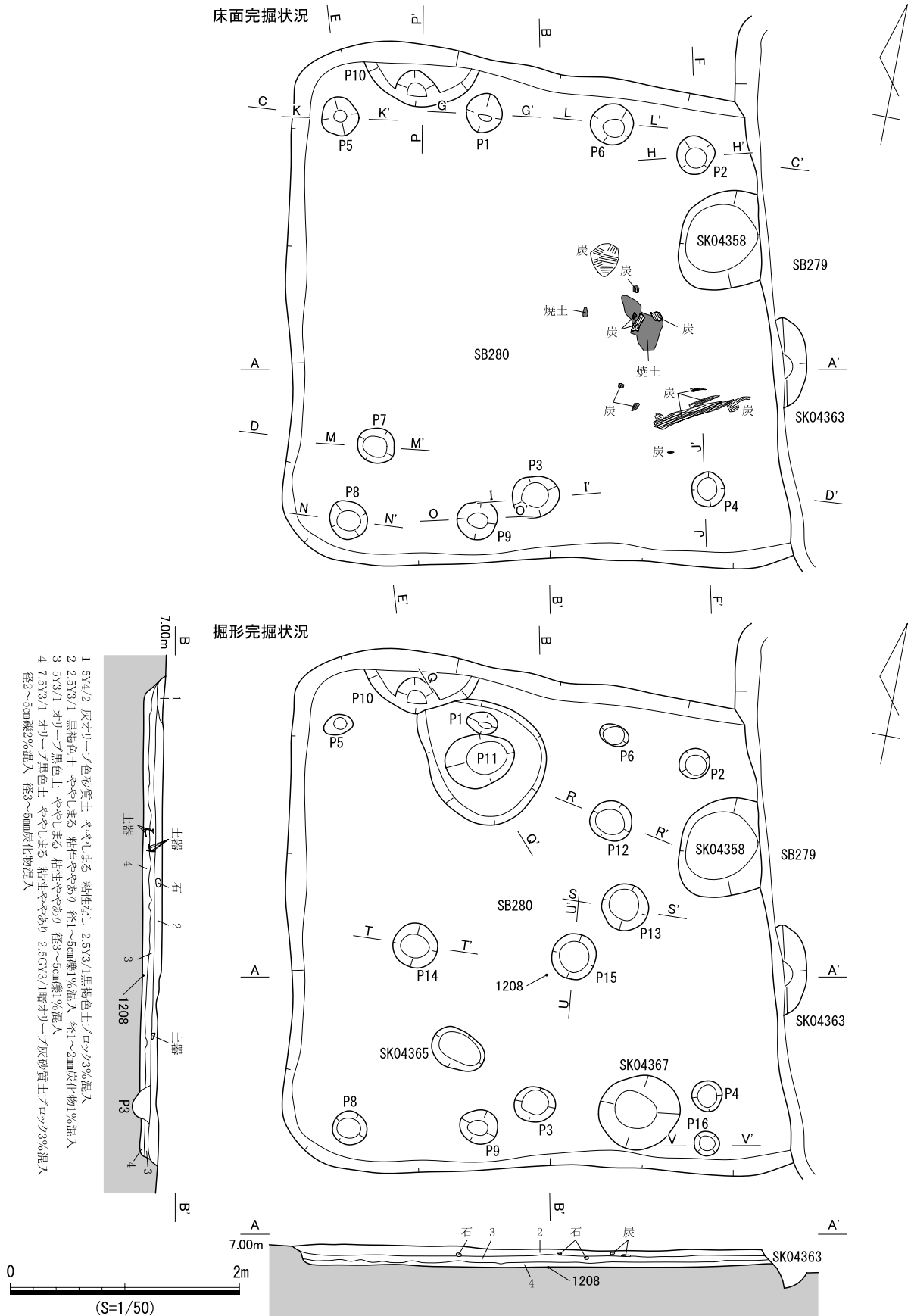
図 440 SB280 遺構図 (1)
