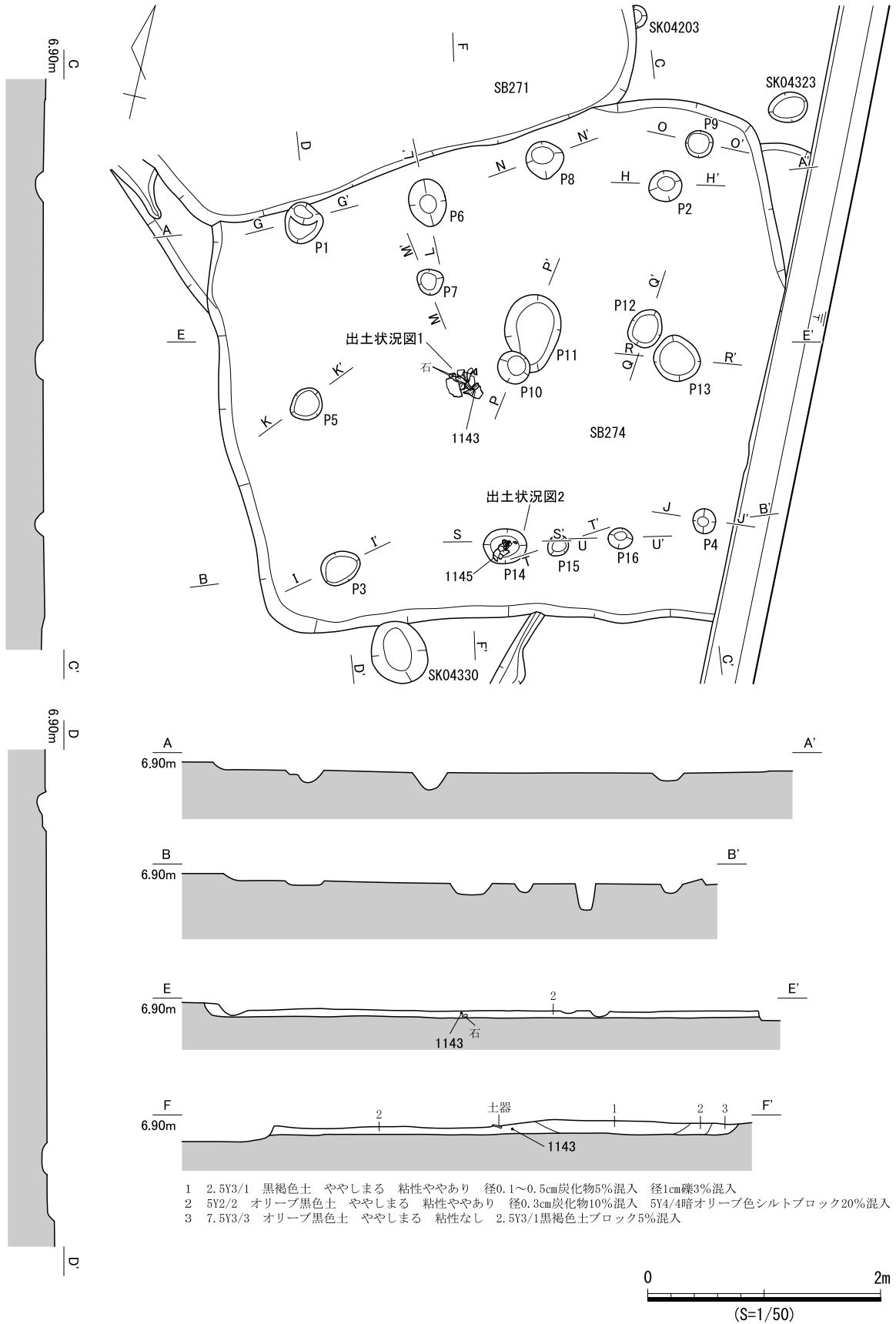
図427 SB274 遺構図(1)
