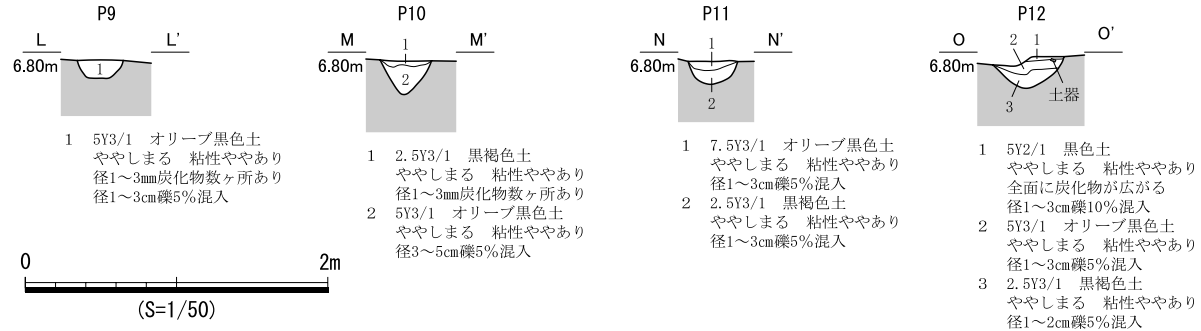
図 515 SB312 遺構図 (2)
