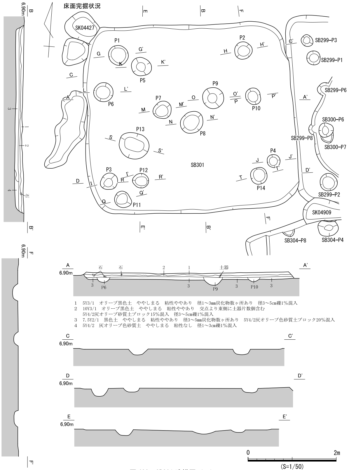
図 488 SB301 遺構図 (1)
