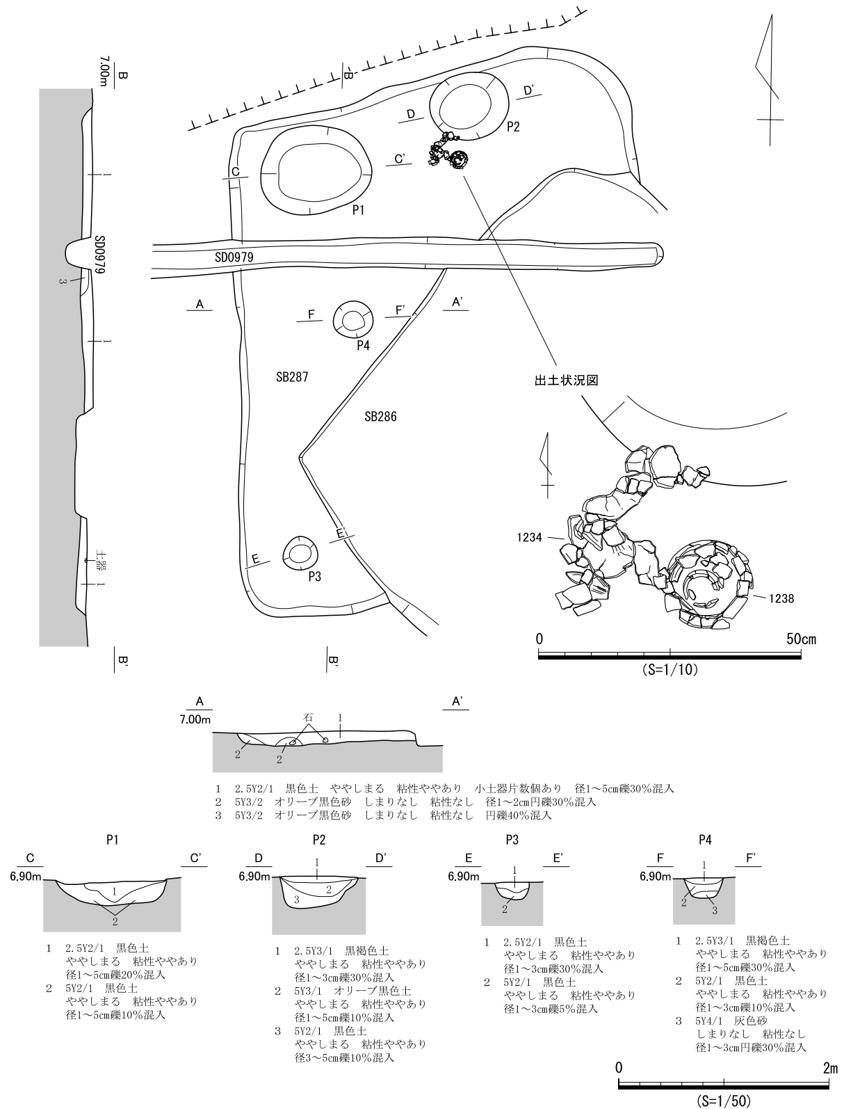
図 458 SB287 遺構図
