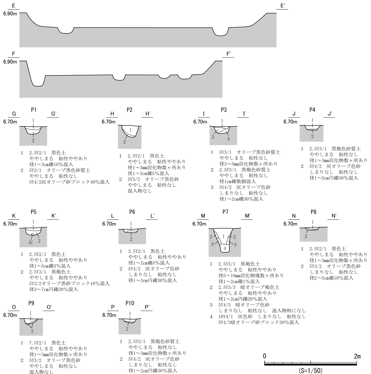
図 534 SB320 遺構図 (2)
