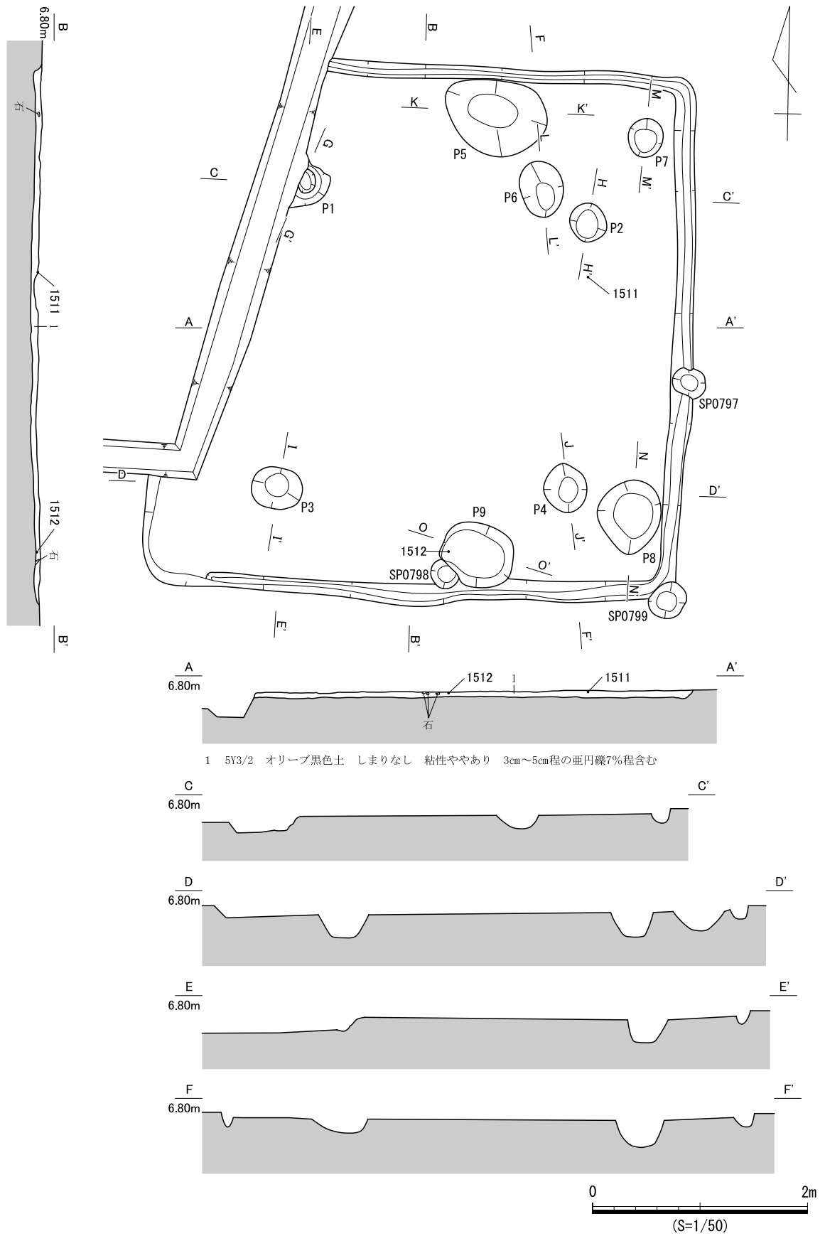
図 552 SB328 遺構図 (1)
