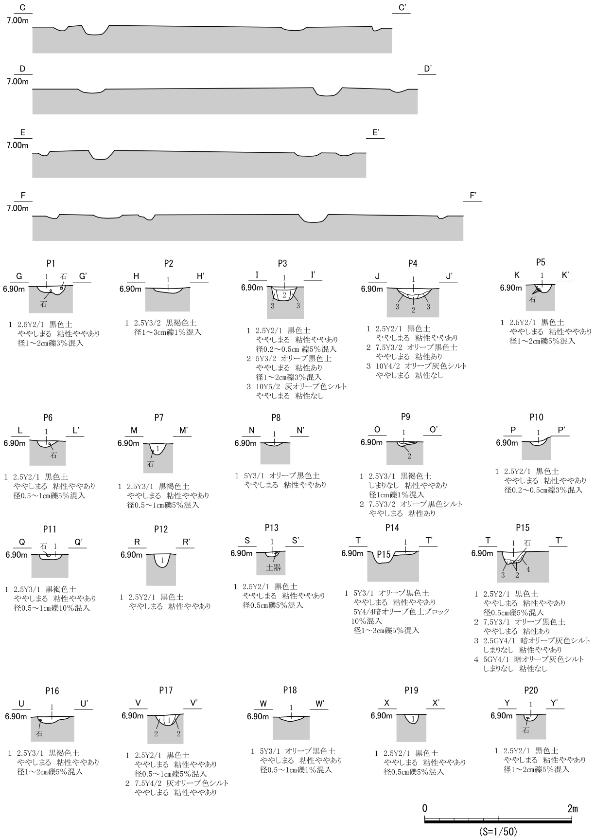
図 434 SB276 遺構図 (2)
