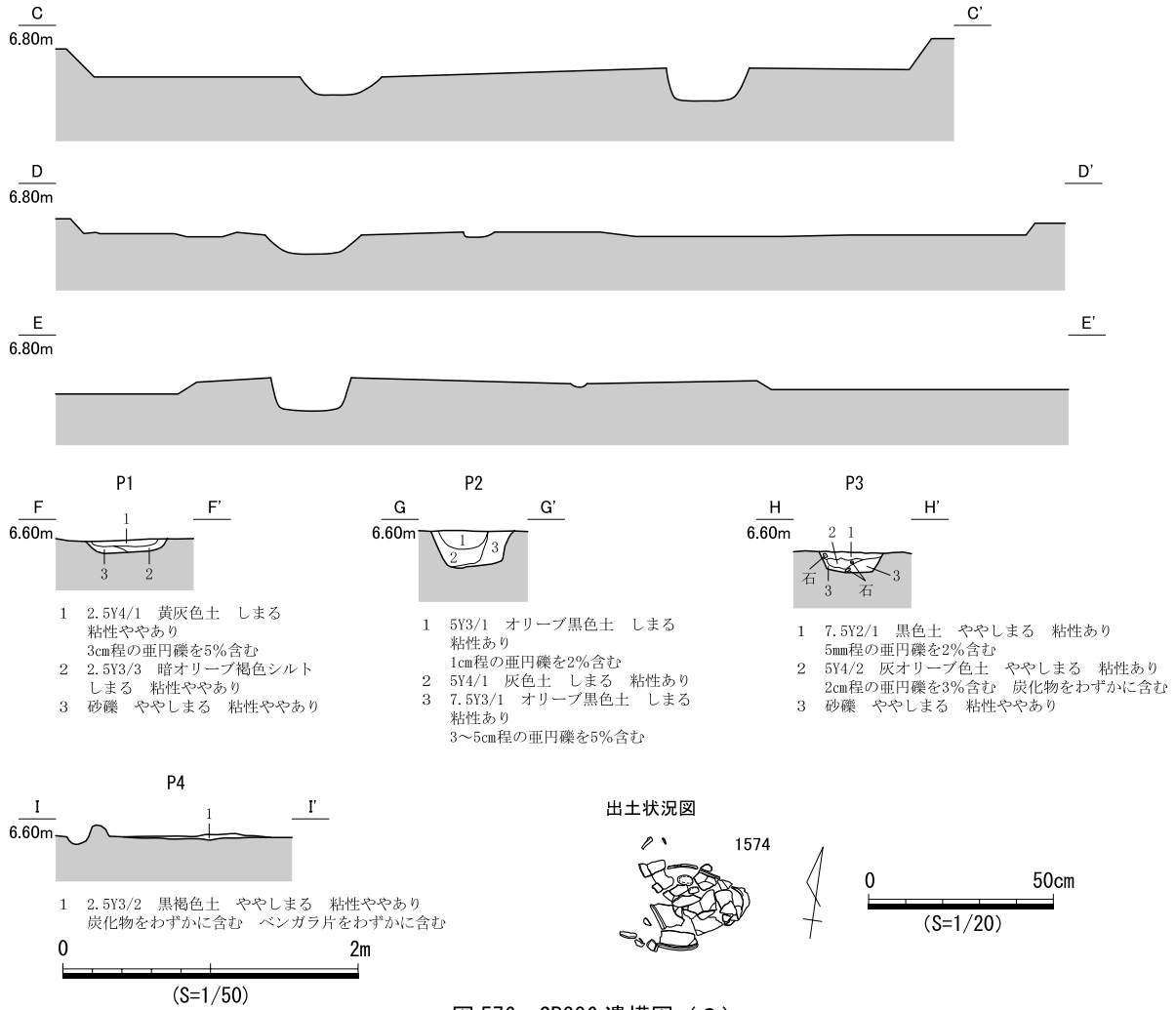
図 576 SB336 遺構図 (3)
