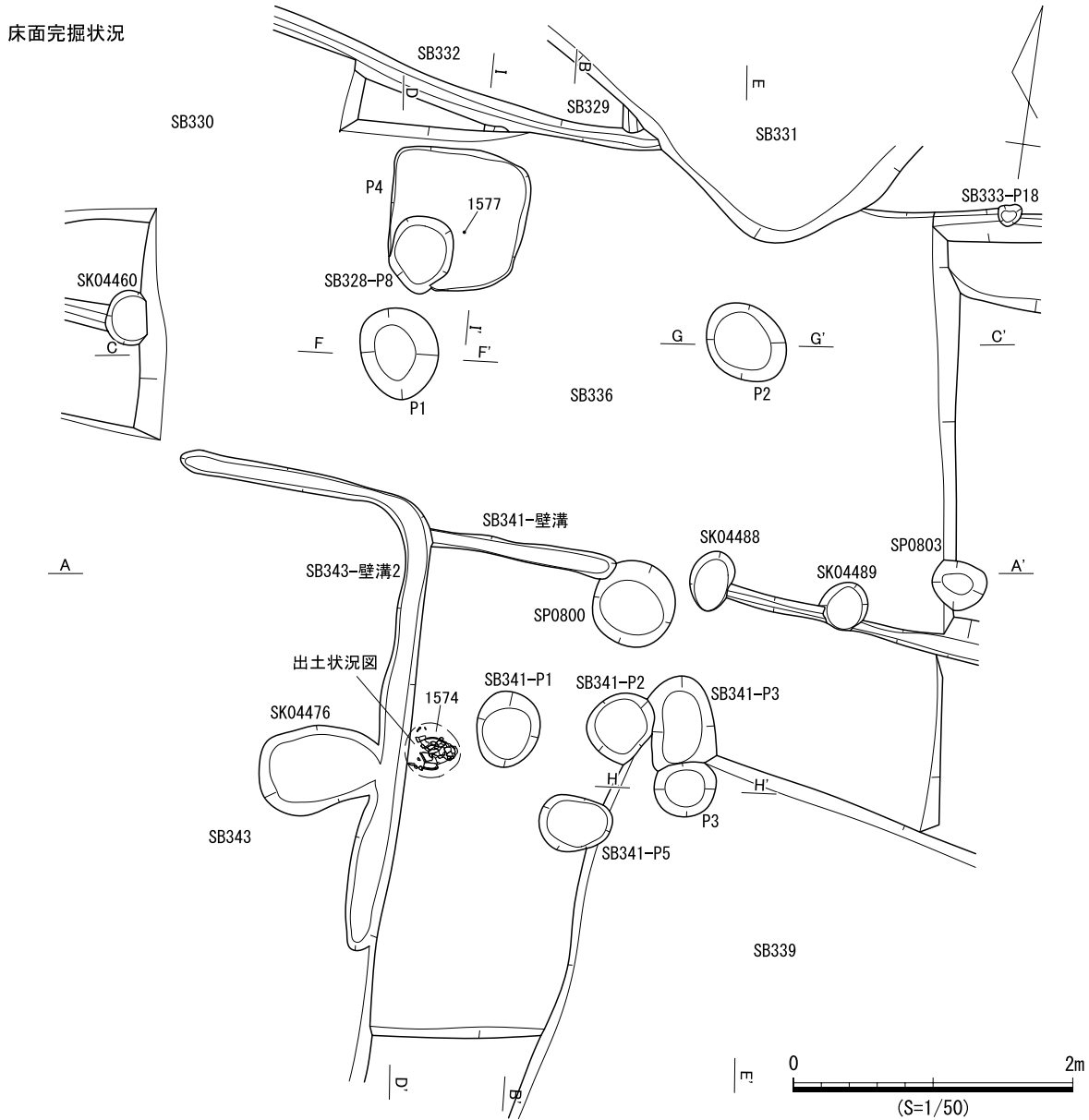
図 574 SB336 遺構図 (1)
