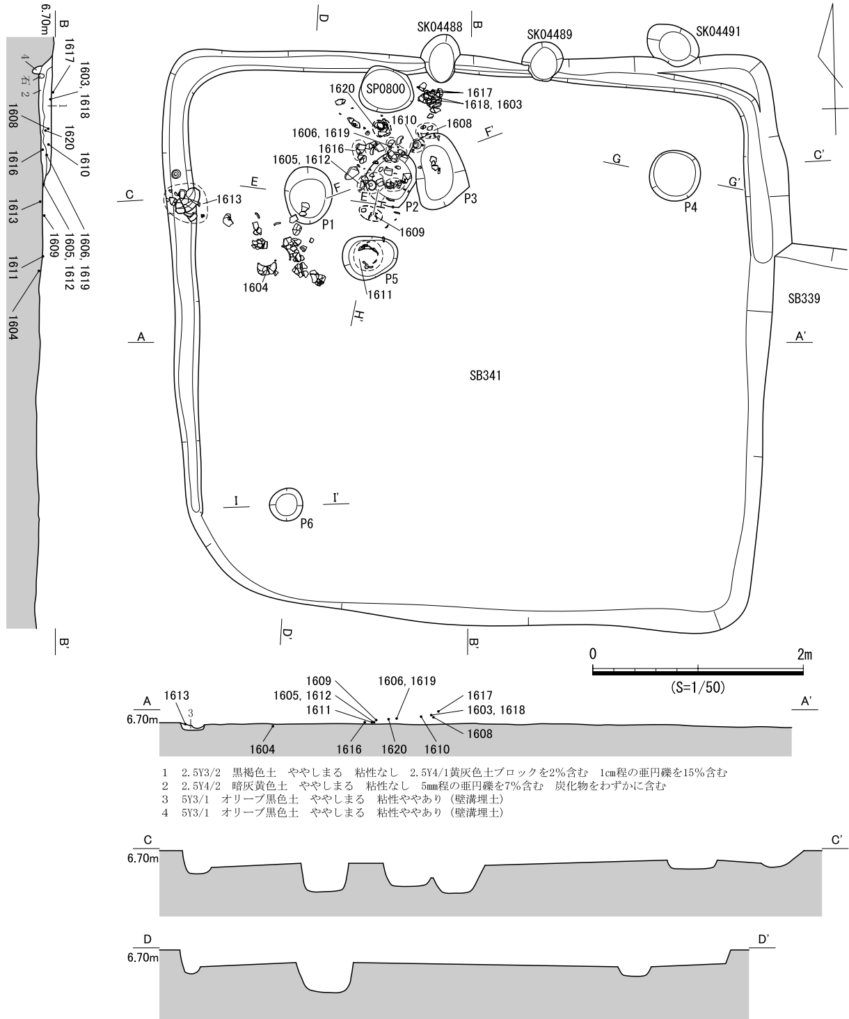
図 588 SB341 遺構図 (1)
