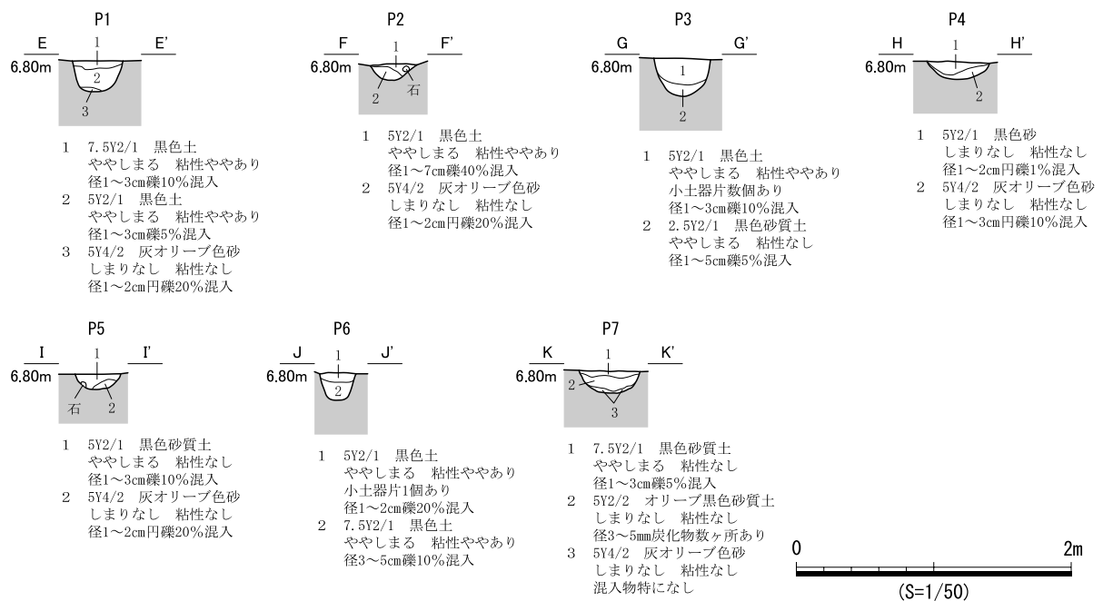
図 476 SB296 遺構図 (2)
