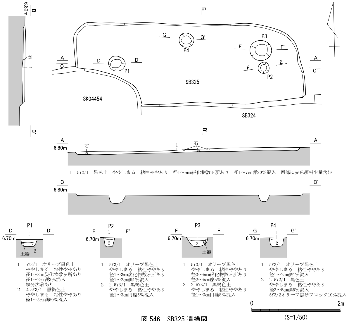
図 546 SB325 遺構図
