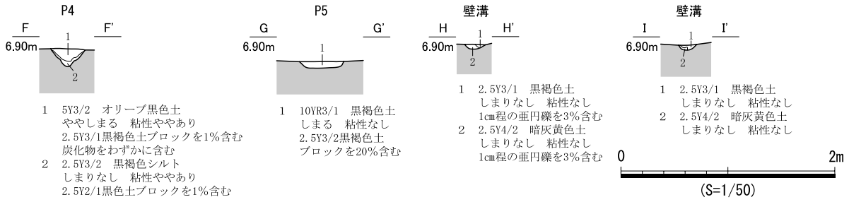
図 573 SB335 遺構図 (2)
