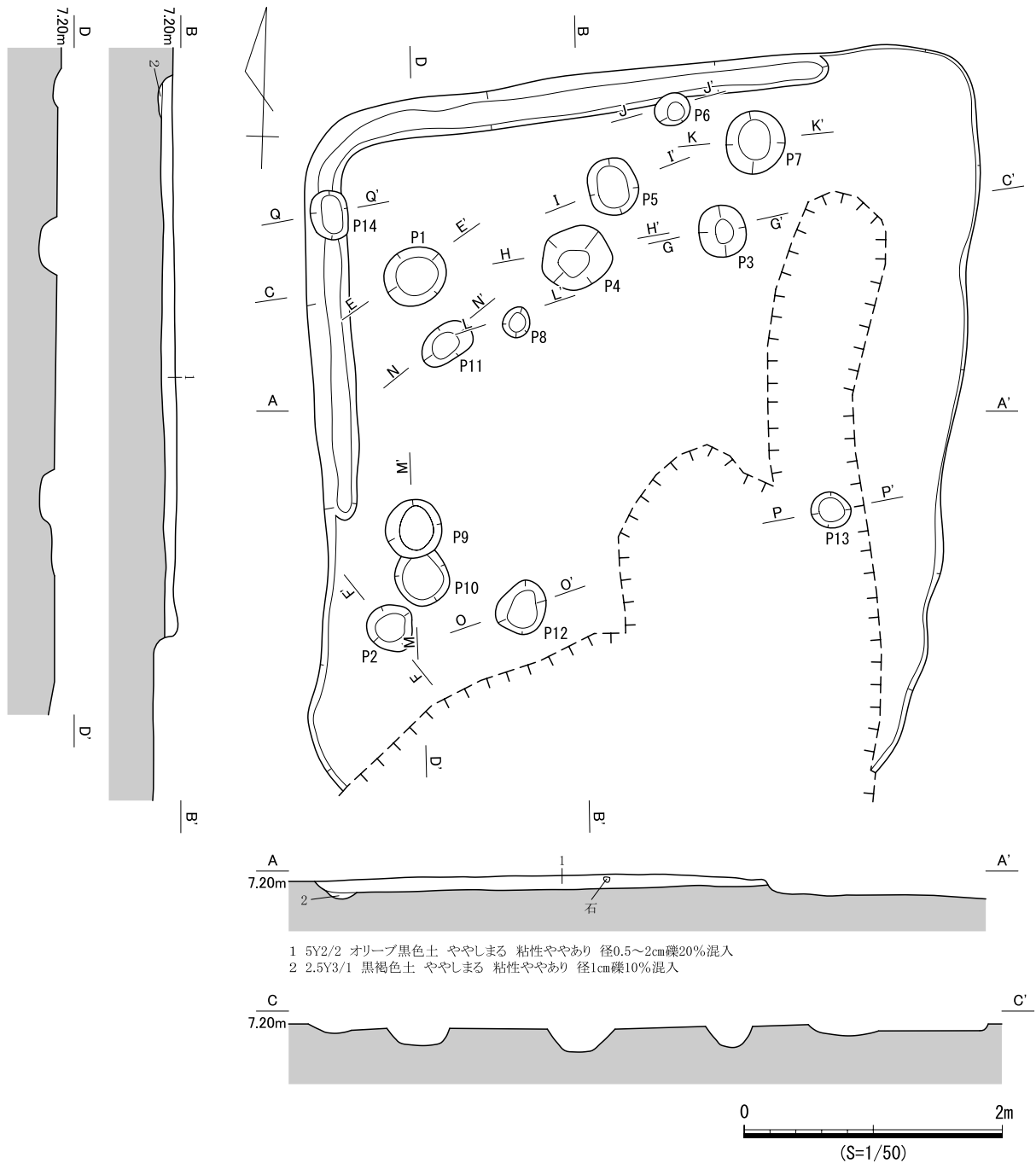
図393 SB260 遺構図(1)
