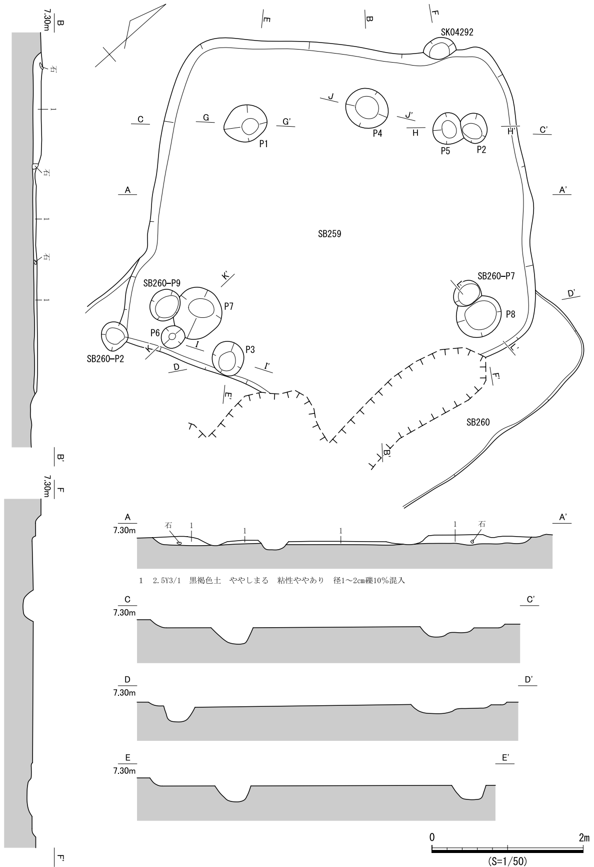
図 392 SB259 遺構図 (2)
