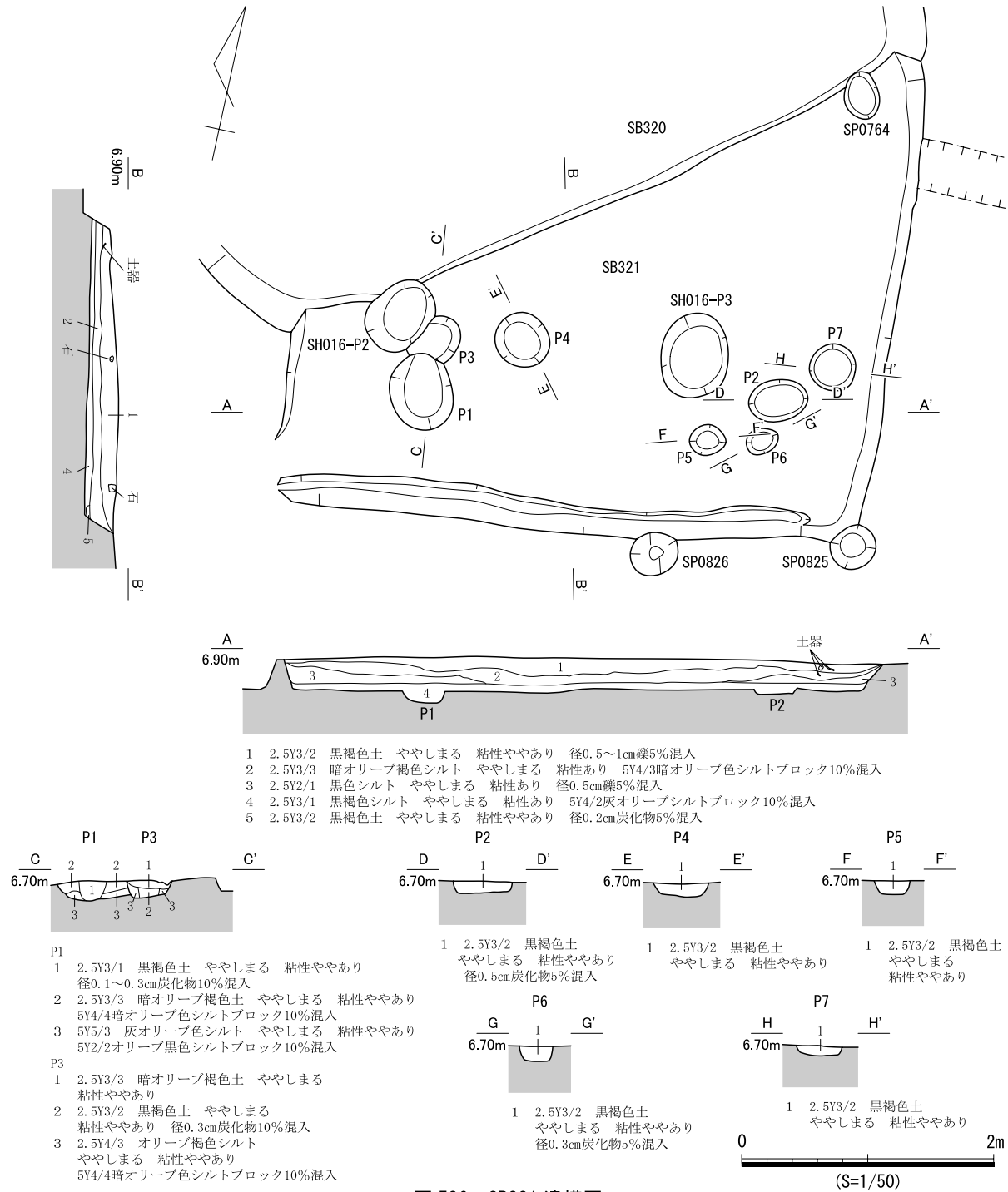
図 536 SB321 遺構図
