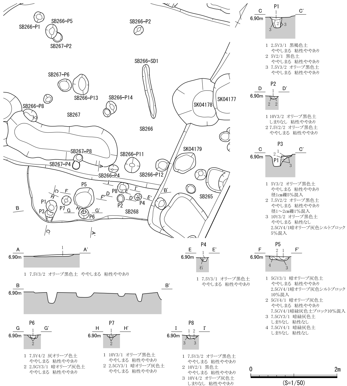
図 414 SB268 遺構図
