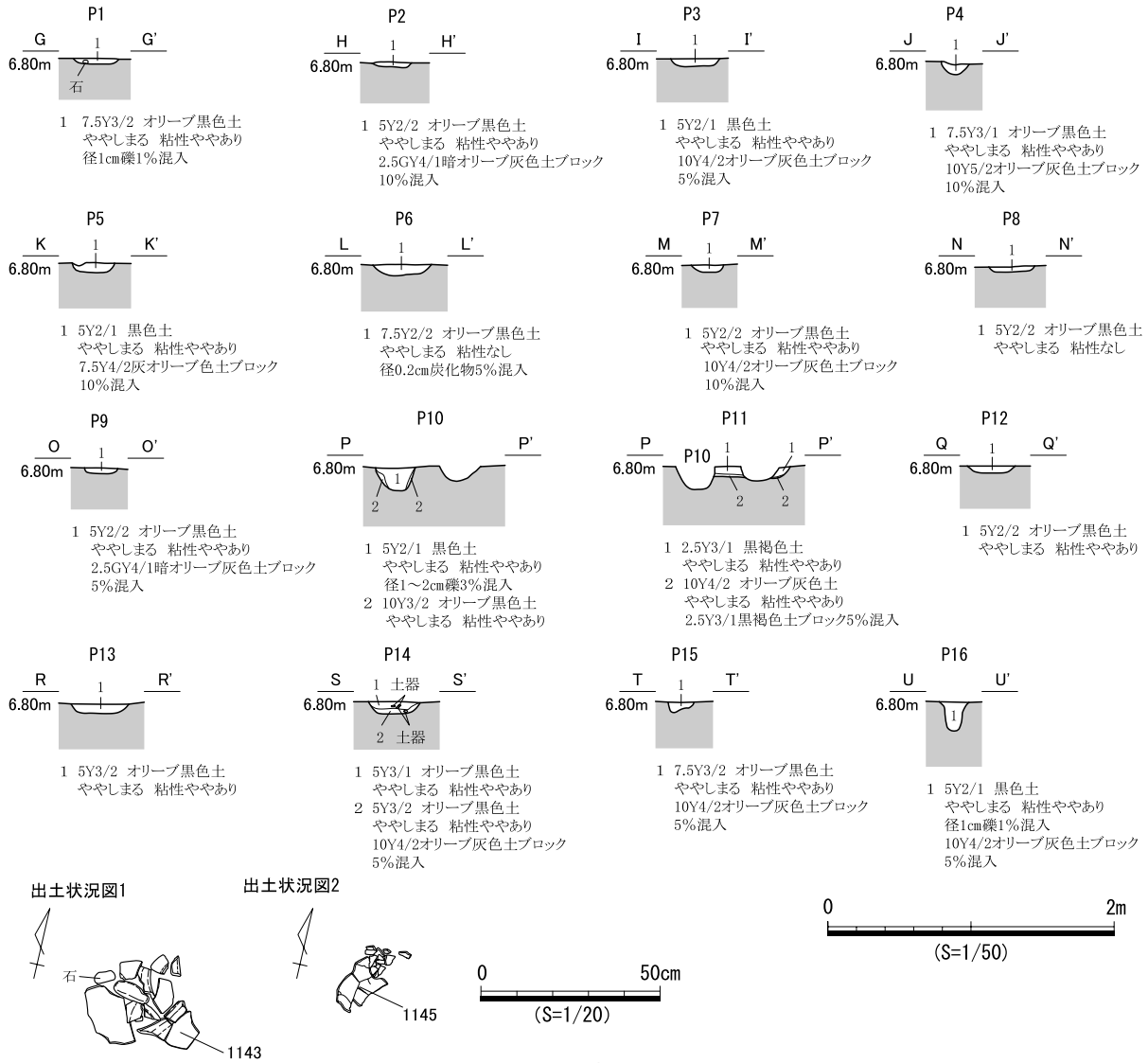
図 428 SB274 遺構図 (2)
