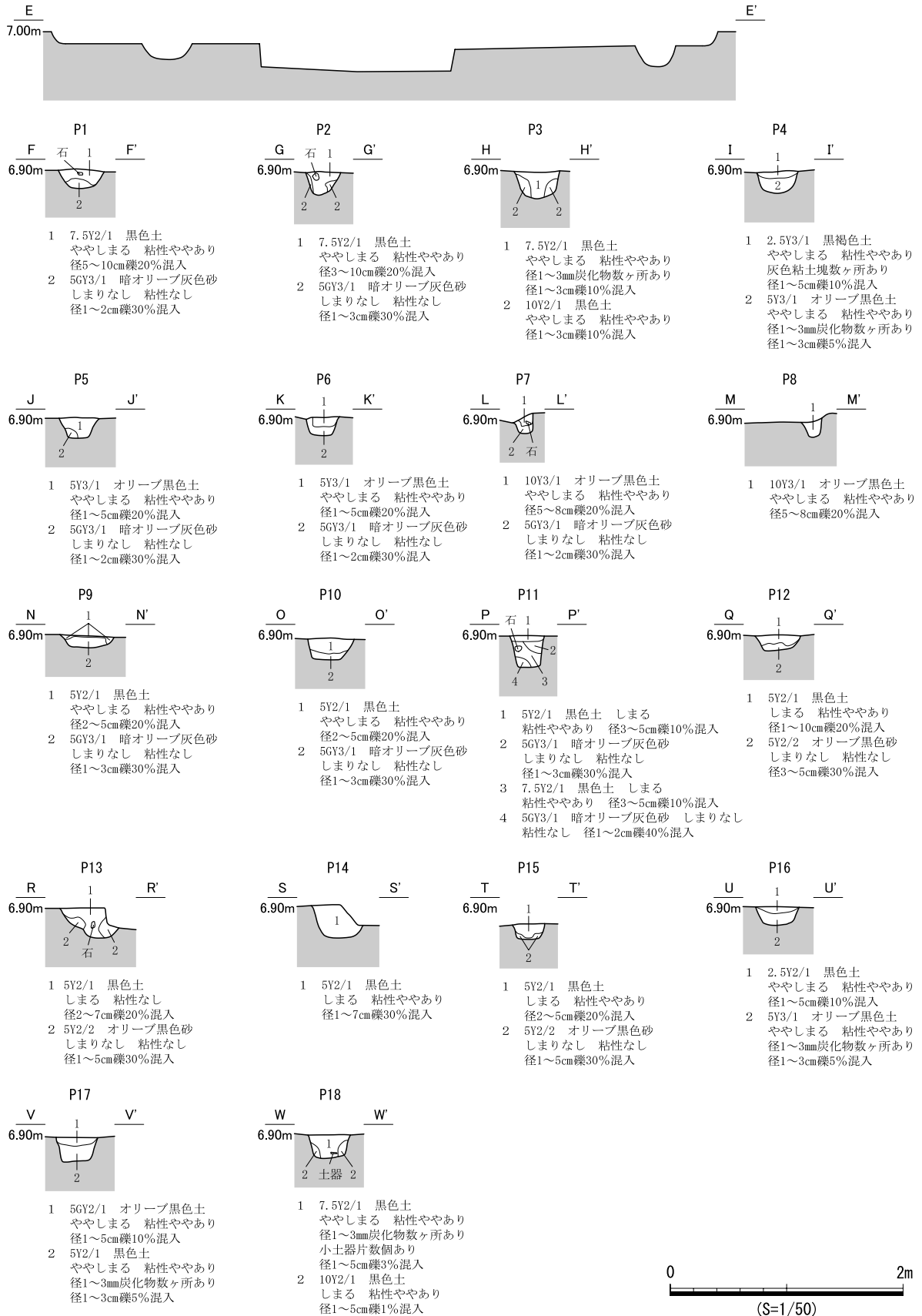
図 532 SB319 遺構図 (2)
