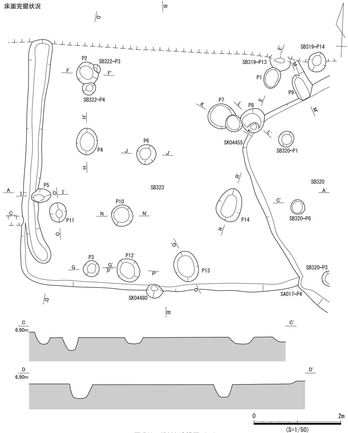
図540 SB323 遺構図(1)
