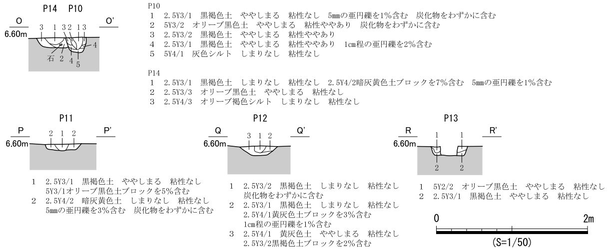
図 584 SB339 遺構図 (3)
