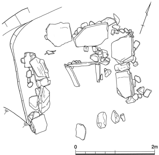
第5図 ST1001石棺状石組検出状況平面図 (S=1/50)
