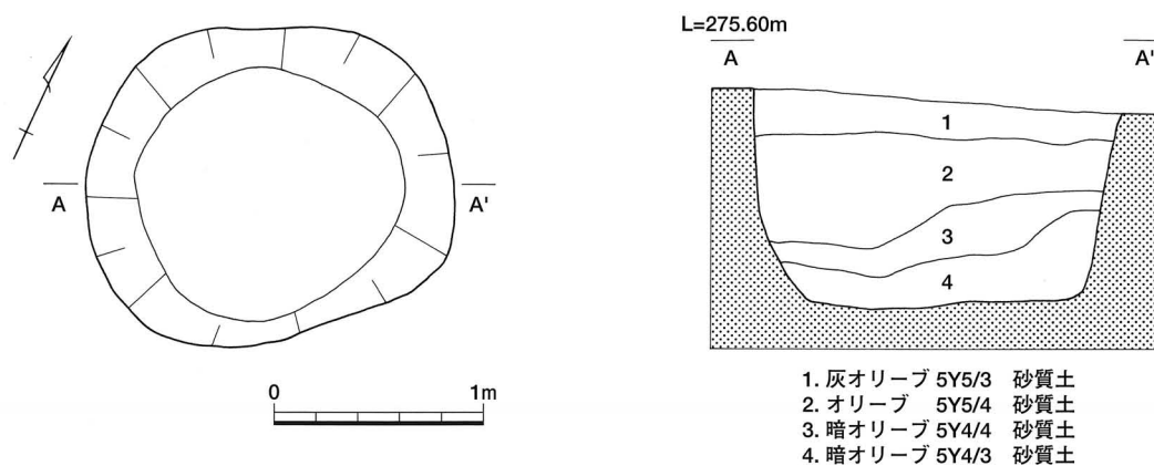
第3図 SE1001平・断面図 (S=1/40)
