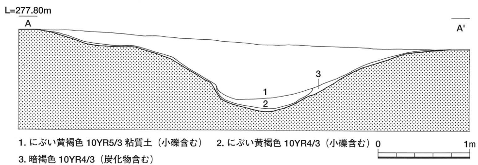
第2図 和田遺跡遺構配置図 (S=1/300) ・SR1001断面図 (S=1/80)
