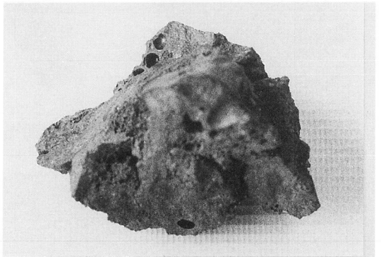
SK05内出土の鉄滓拡大 (×1.5)
