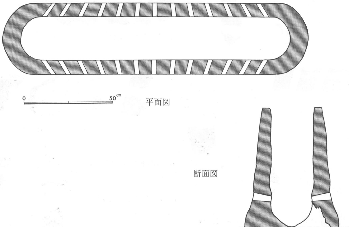
第10図 羽森遺跡製鉄炉復原図
