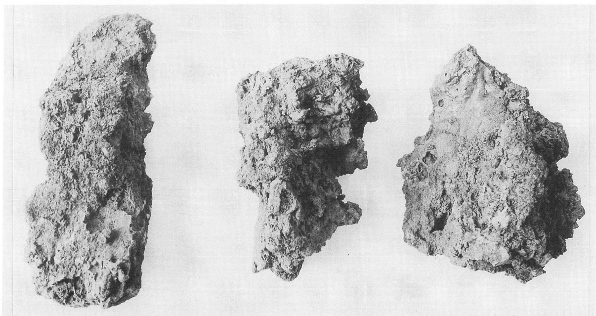
製鉄炉内出土の鉄滓外観
