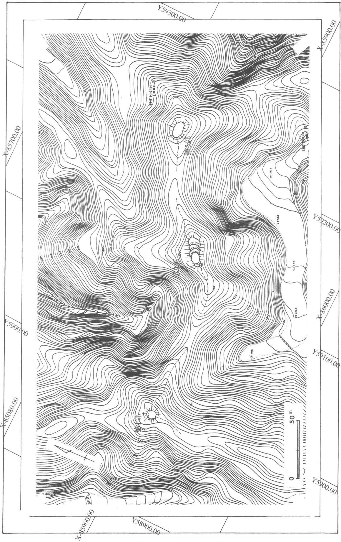
第3图 羽森城跡山頂部郭群配置図
