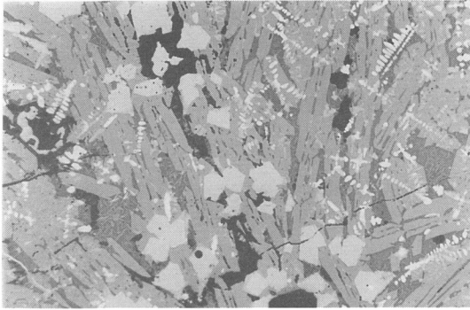
写真9 資料No.4鉄塊 (×100)
