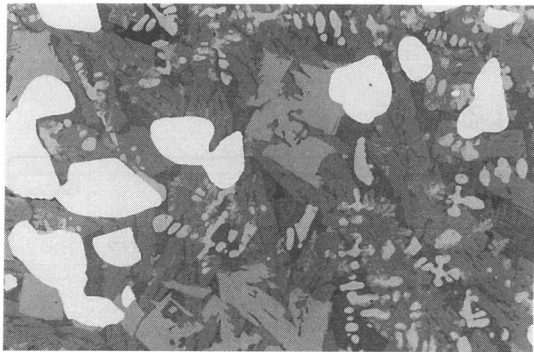
写真7-1 資料No.21号炉鉄塊 (×100)
