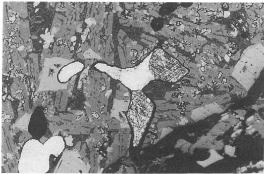
写真7-2 資料No.21号炉鉄塊ニイタル腐食 (×100)
