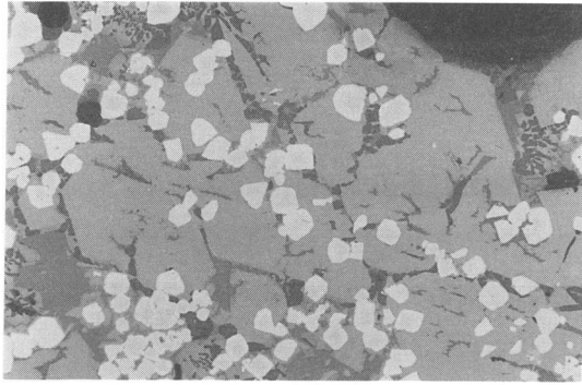
写真6 資料No.1鉄滓 (×100)
